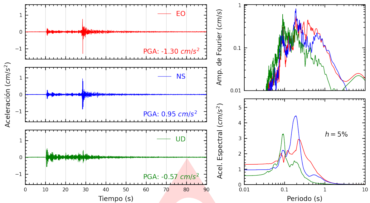
Figura A.1: Registros tiempo-historia, espectros de Fourier y de respuesta en las direcciones EO, NS y vertical de la estación UNIA. Sismo de Contamana, Ucayali - Loreto de 2022-08-19, 14:06:52 (Hora local)
