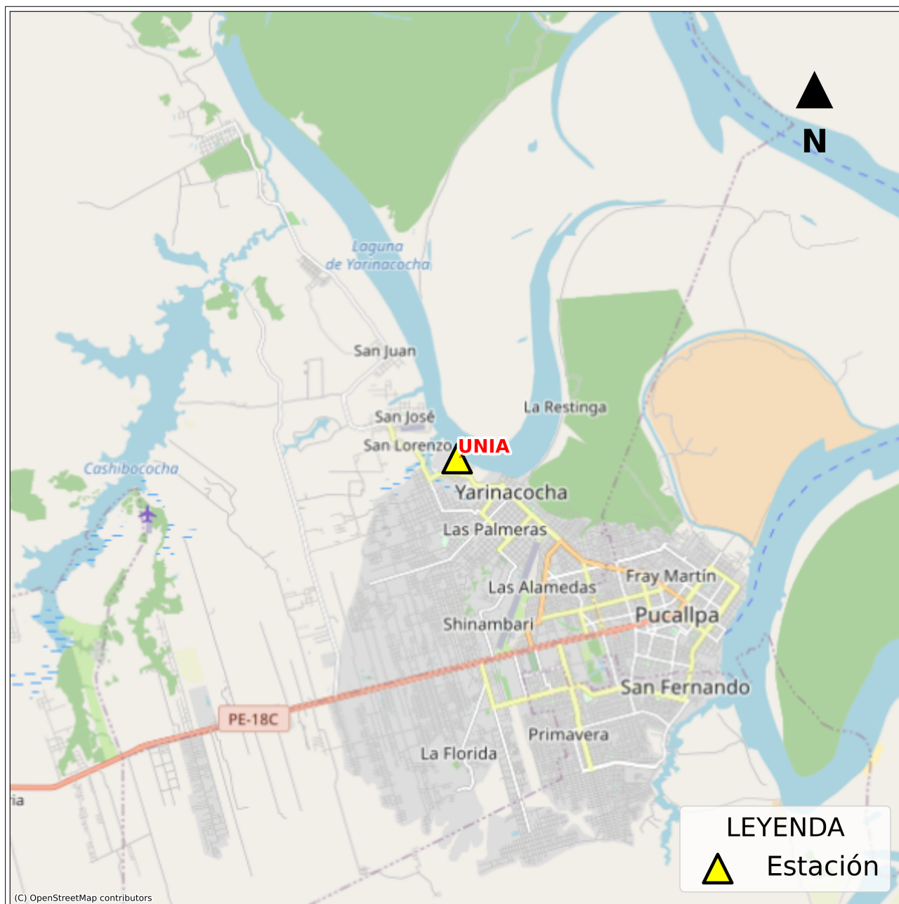
Figura 2: Mapa de ubicación de la(s) estación(es) acelerográfica(s) correspondiente(s) al Sismo de Contamana, Ucayali - Loreto del 19 de agosto de 2022 a las 14:06:52 (hora local)
