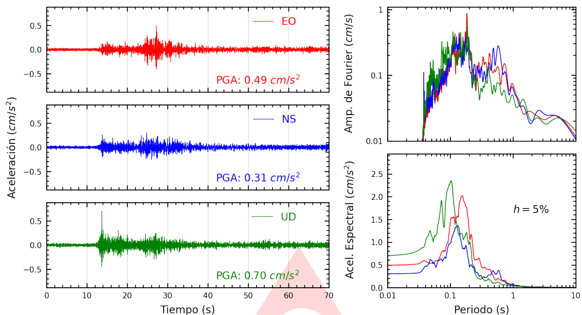
Figura A.1: Registros tiempo-historia, espectros de Fourier y de respuesta en las direcciones EO, NS y vertical de la estación UNICA. Sismo de Ica, Ica - Ica del 2022-10-28, 13:52:58 (Hora local)
