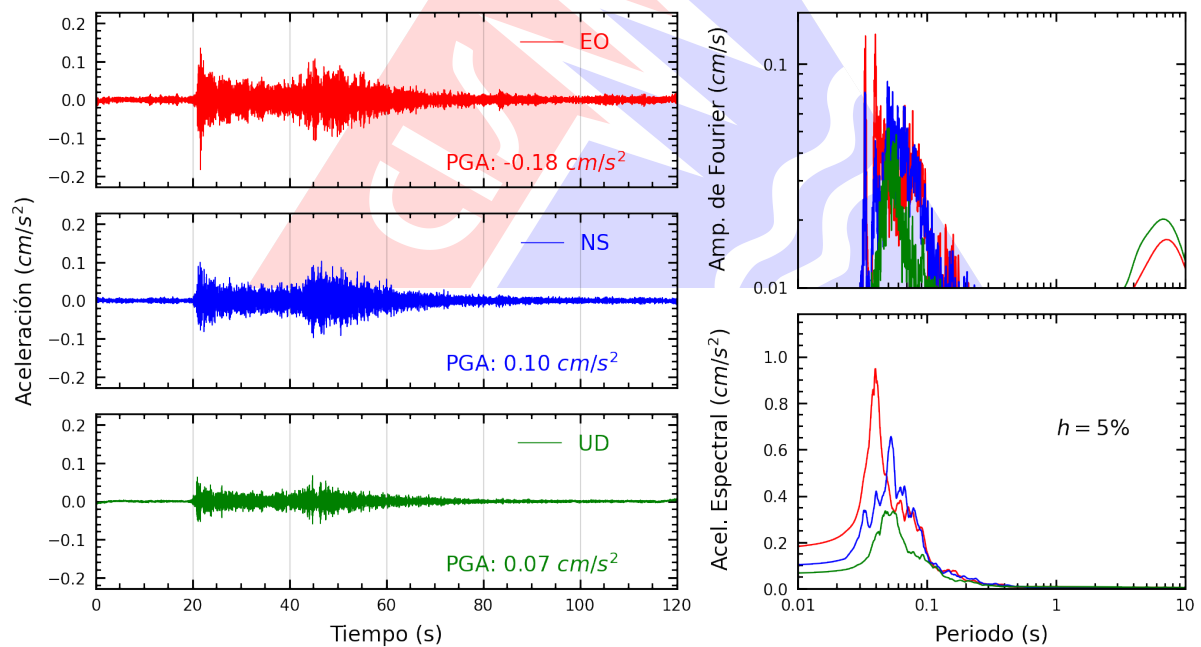
Figura A.2: Registros tiempo-historia, espectros de Fourier y de respuesta en las direcciones EO, NS y vertical de la estación UNAM. Sismo de Aplao, Castilla - Arequipa del 2022-11-22, 01:29:37 (Hora local)
