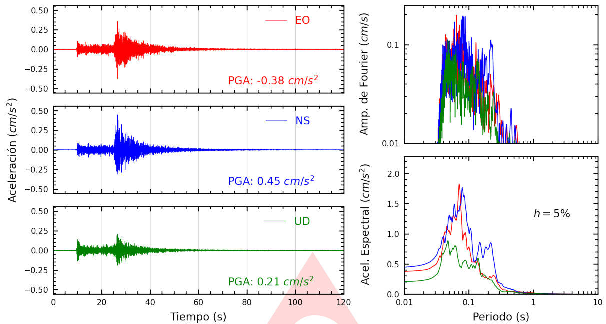
Figura A.1: Registros tiempo-historia, espectros de Fourier y de respuesta en las direcciones EO, NS y vertical de la estación UNSA. Sismo de Aplao, Castilla - Arequipa del 2022-11-22, 01:29:37 (Hora local)
