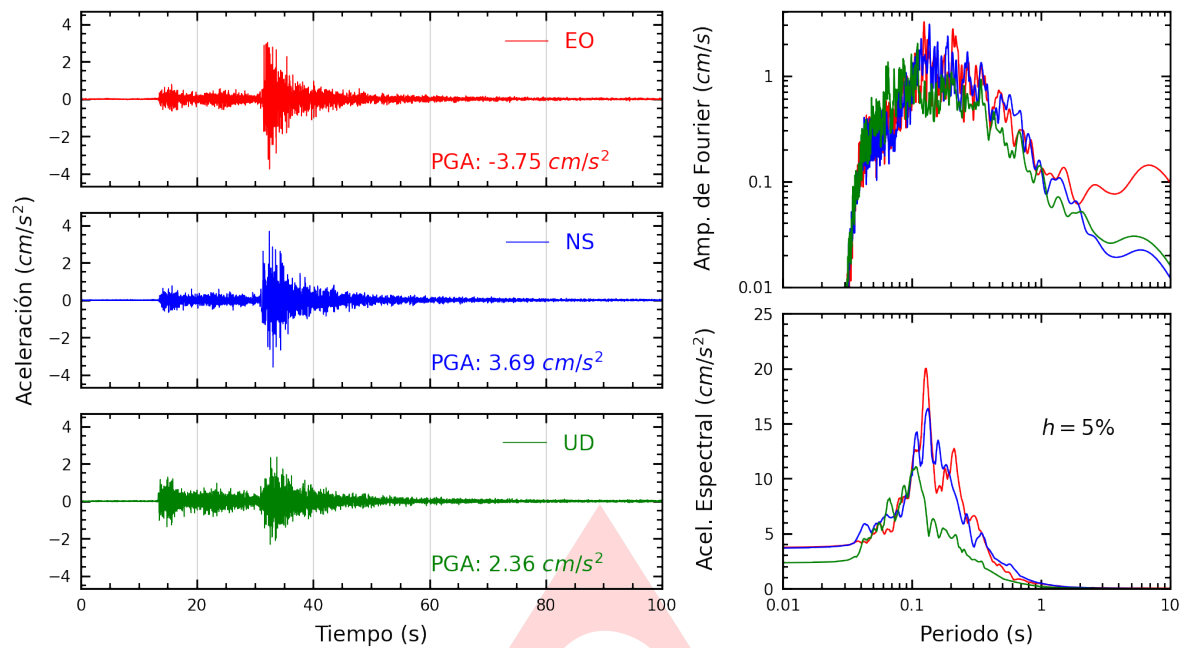
Figura A.1: Registros tiempo-historia, espectros de Fourier y de respuesta en las direcciones EO, NS y vertical de la estación UJBG3. Sismo de Calana, Tacna - Tacna del 2022-12-03, 06:45:29 (Hora local)
