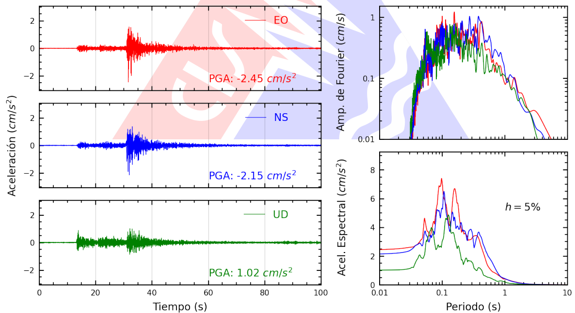
Figura A.2: Registros tiempo-historia, espectros de Fourier y de respuesta en las direcciones EO, NS y vertical de la estación UJBG2. Sismo de Calana, Tacna - Tacna del 2022-12-03, 06:45:29 (Hora local)
