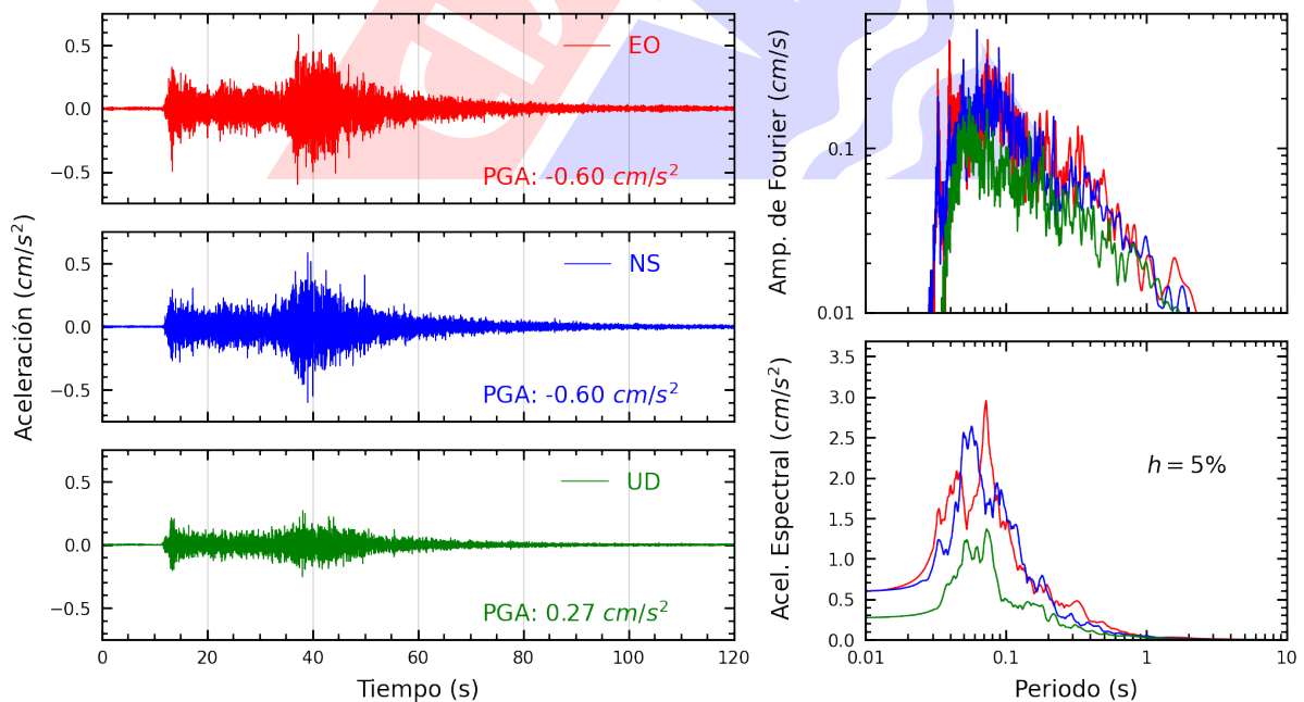
Figura A.4: Registros tiempo-historia, espectros de Fourier y de respuesta en las direcciones EO, NS y vertical de la estación UNAM. Sismo de Calana, Tacna - Tacna del 2022-12-03, 06:45:29 (Hora local)
