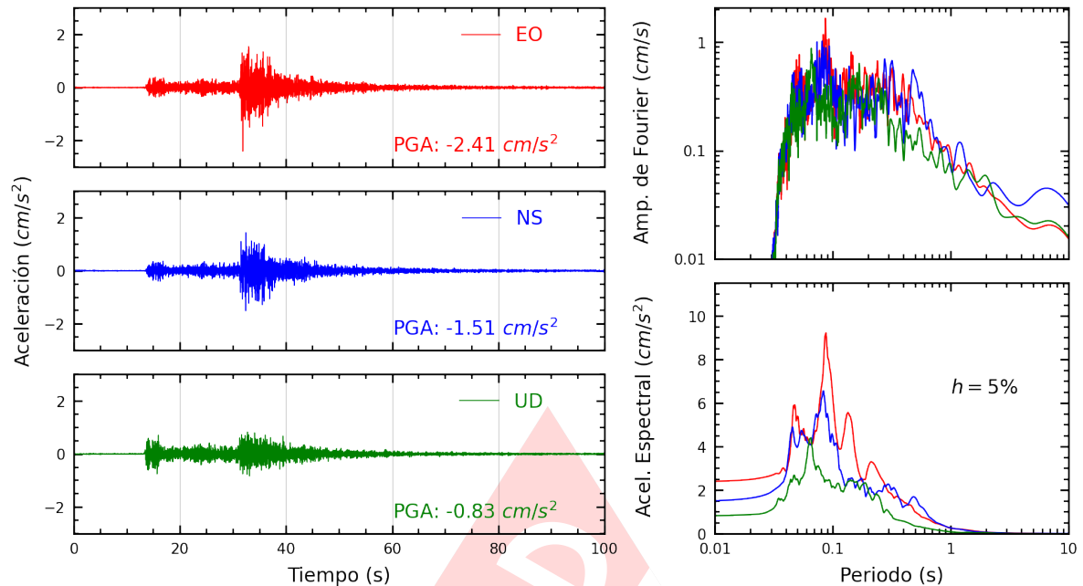
Figura A.3: Registros tiempo-historia, espectros de Fourier y de respuesta en las direcciones EO, NS y vertical de la estación CREY. Sismo de Calana, Tacna - Tacna del 2022-12-03, 06:45:29 (Hora local)
