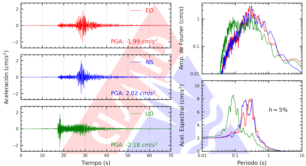
Figura A.3: Registros tiempo-historia, espectros de Fourier y de respuesta en las direcciones EO, NS y vertical de la estación UNIPE. Sismo de Sullana, Sullana - Piura del 2022-12-11, 16:00:04 (Hora local)
