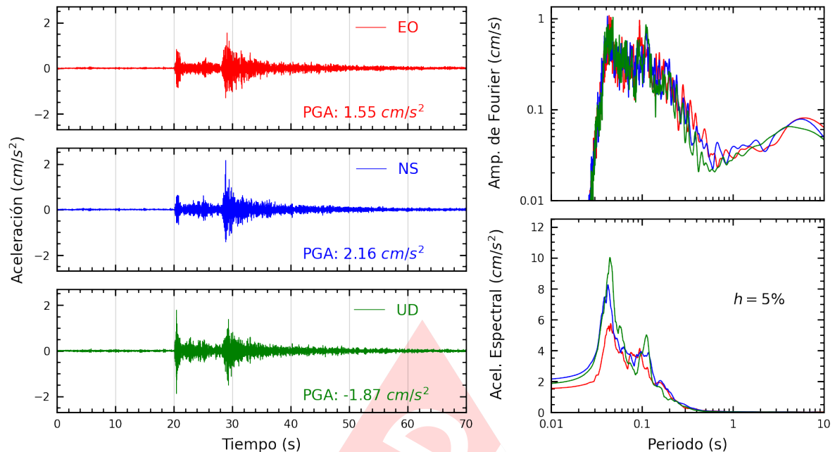
Figura A.17: Registros tiempo-historia, espectros de Fourier y de respuesta en las direcciones EO, NS y vertical de la estación USMP. Sismo de Ancon, Lima - Lima del 2022-12-19, 20:30:07 (Hora local)
