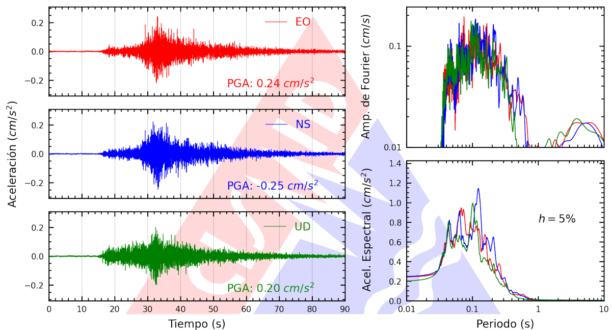
Figura A.35: Registros tiempo-historia, espectros de Fourier y de respuesta en las direcciones EO, NS y vertical de la estación CARAL. Sismo de Ancon, Lima - Lima del 2022-12-19, 20:30:07 (Hora local)
