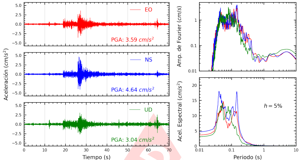
Figura A.9: Registros tiempo-historia, espectros de Fourier y de respuesta en las direcciones EO, NS y vertical de la estación CARAB. Sismo de Ancon, Lima - Lima del 2022-12-19, 20:30:07 (Hora local)
