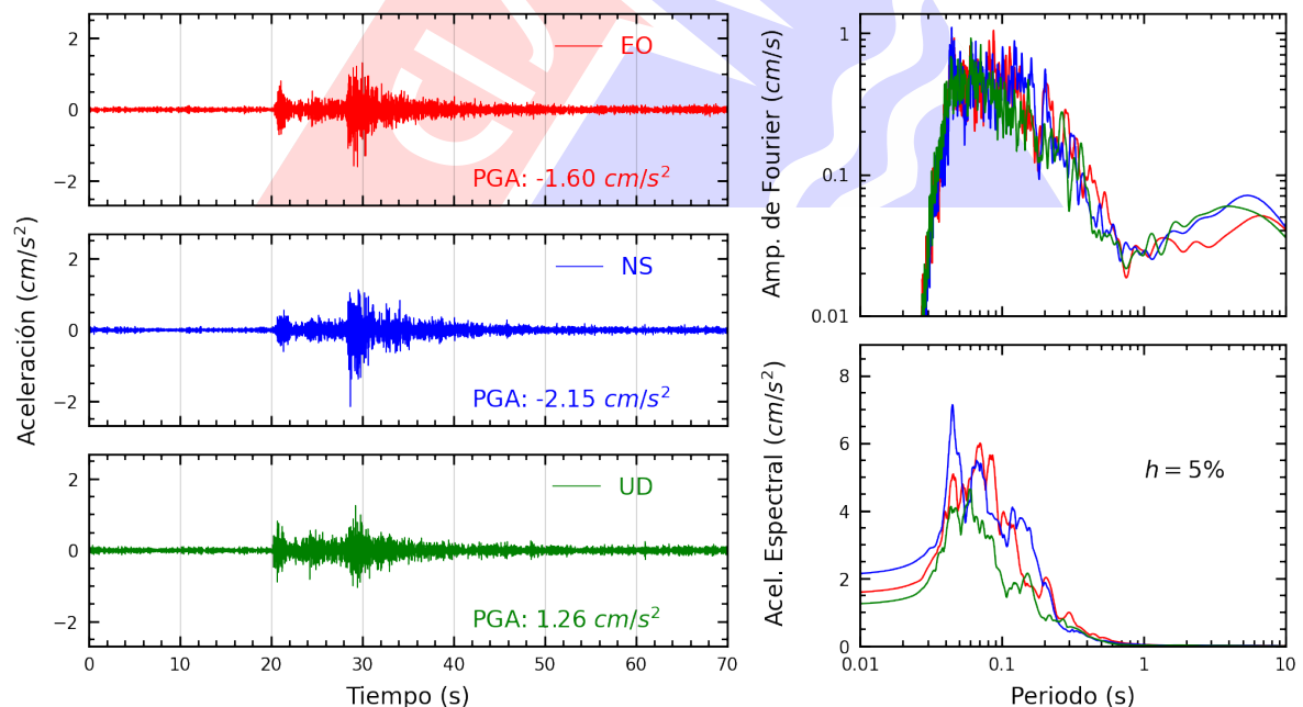
Figura A.18: Registros tiempo-historia, espectros de Fourier y de respuesta en las direcciones EO, NS y vertical de la estación URPE. Sismo de Ancon, Lima - Lima del 2022-12-19, 20:30:07 (Hora local)
