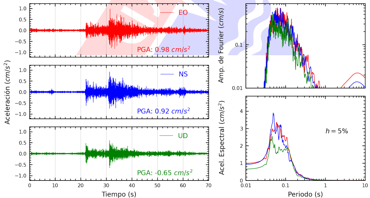
Figura A.32: Registros tiempo-historia, espectros de Fourier y de respuesta en las direcciones EO, NS y vertical de la estación PACHA. Sismo de Ancon, Lima - Lima del 2022-12-19, 20:30:07 (Hora local)
