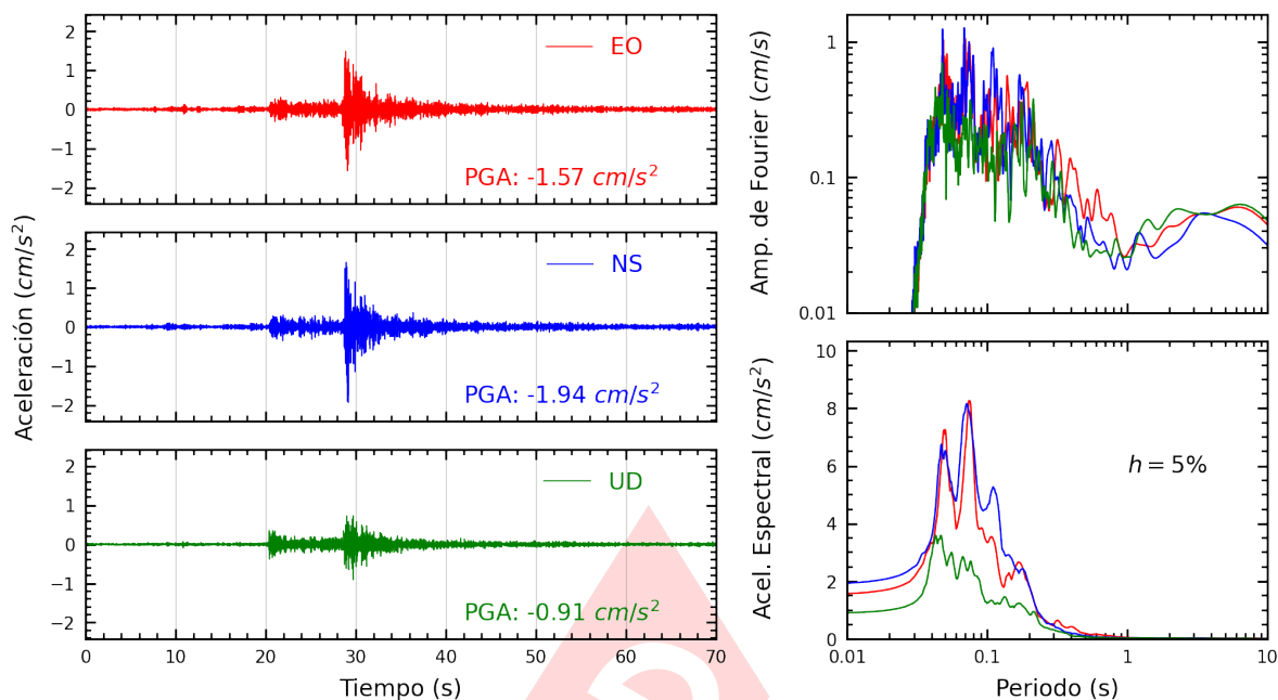
Figura A.21: Registros tiempo-historia, espectros de Fourier y de respuesta en las direcciones EO, NS y vertical de la estación UPCVI. Sismo de Ancon, Lima - Lima del 2022-12-19, 20:30:07 (Hora local)
