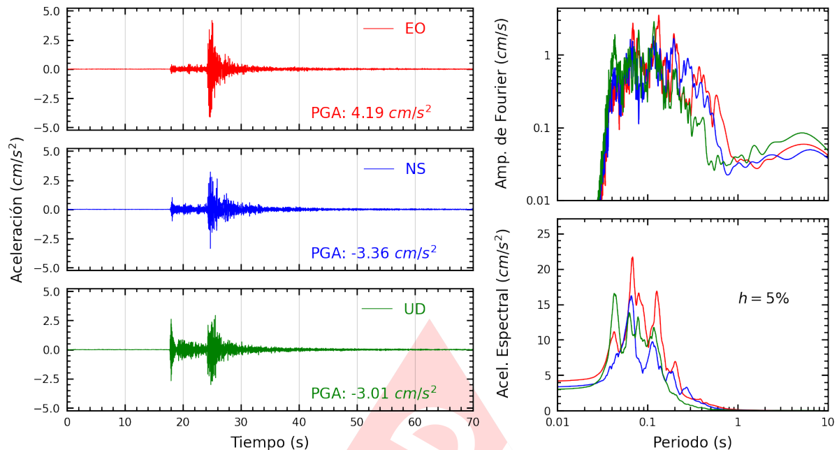
Figura A.11: Registros tiempo-historia, espectros de Fourier y de respuesta en las direcciones EO, NS y vertical de la estación VHAYA. Sismo de Ancon, Lima - Lima del 2022-12-19, 20:30:07 (Hora local)
