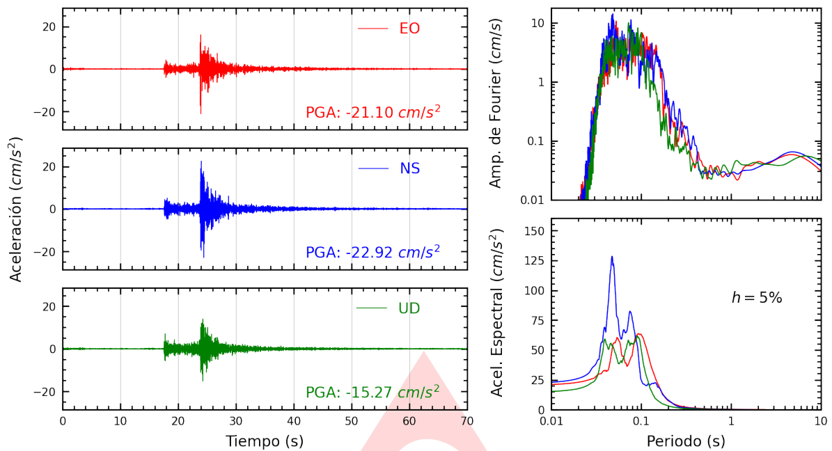
Figura A.1: Registros tiempo-historia, espectros de Fourier y de respuesta en las direcciones EO, NS y vertical de la estación SROSA. Sismo de Ancon, Lima - Lima del 2022-12-19, 20:30:07 (Hora local)
