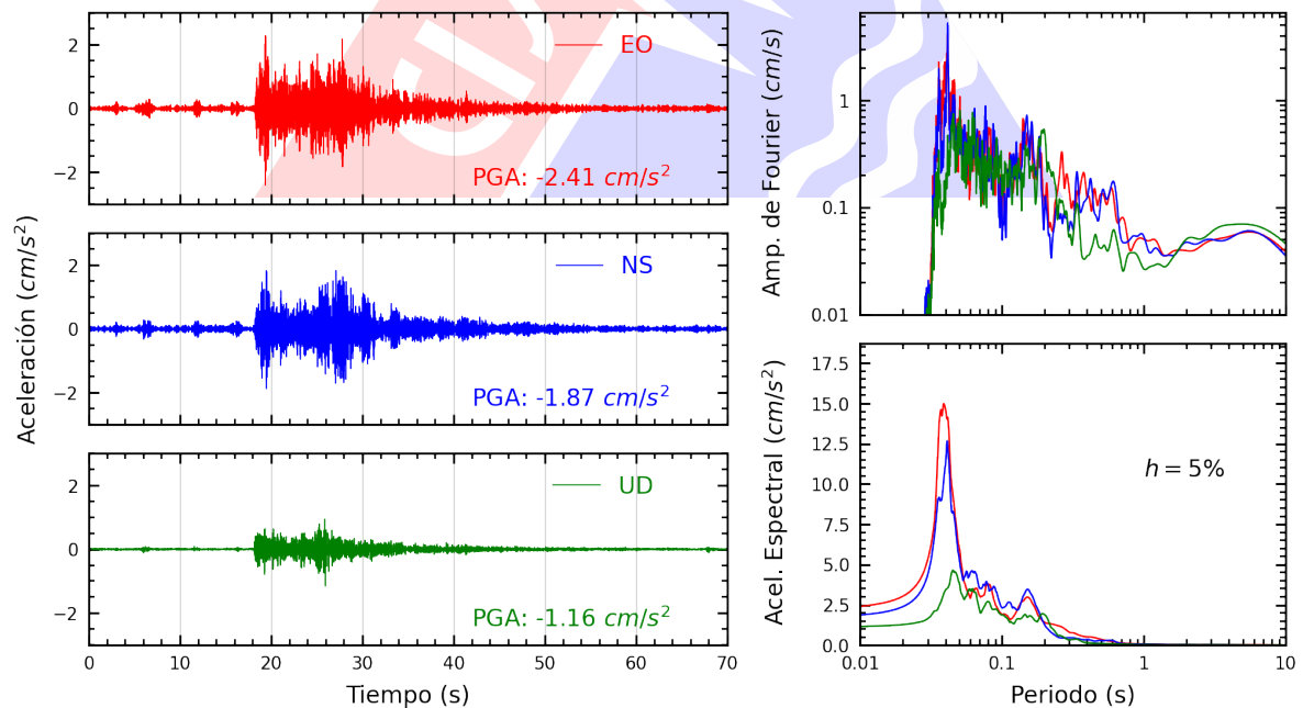
Figura A.14: Registros tiempo-historia, espectros de Fourier y de respuesta en las direcciones EO, NS y vertical de la estación DHNPE. Sismo de Ancon, Lima - Lima del 2022-12-19, 20:30:07 (Hora local)
