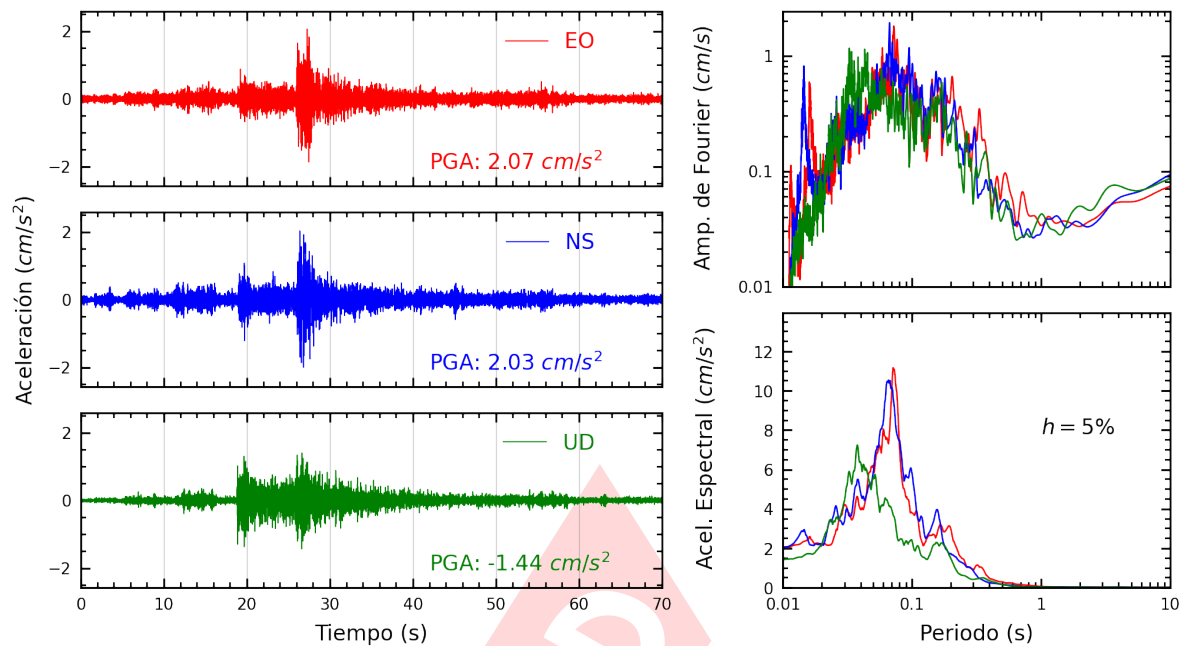
Figura A.19: Registros tiempo-historia, espectros de Fourier y de respuesta en las direcciones EO, NS y vertical de la estación UPCSM. Sismo de Ancon, Lima - Lima del 2022-12-19, 20:30:07 (Hora local)
