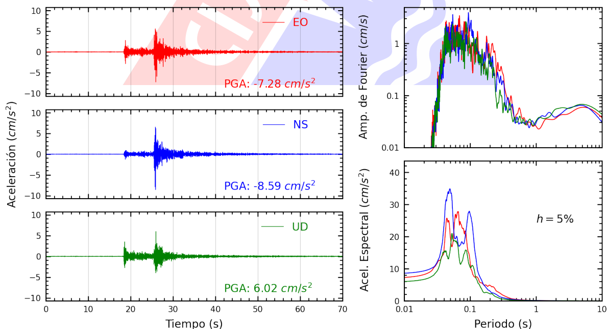
Figura A.4: Registros tiempo-historia, espectros de Fourier y de respuesta en las direcciones EO, NS y vertical de la estación INDEP. Sismo de Ancon, Lima - Lima del 2022-12-19, 20:30:07 (Hora local)
