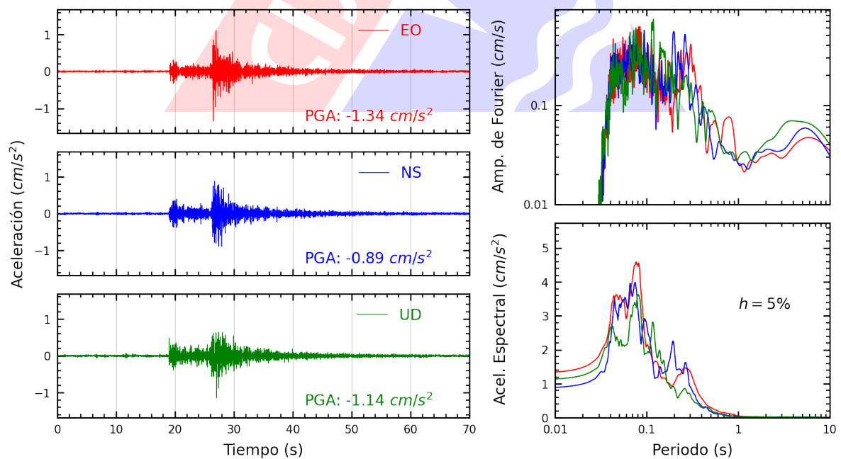
Figura A.28: Registros tiempo-historia, espectros de Fourier y de respuesta en las direcciones EO, NS y vertical de la estación UNFV. Sismo de Ancon, Lima - Lima del 2022-12-19, 20:30:07 (Hora local)
