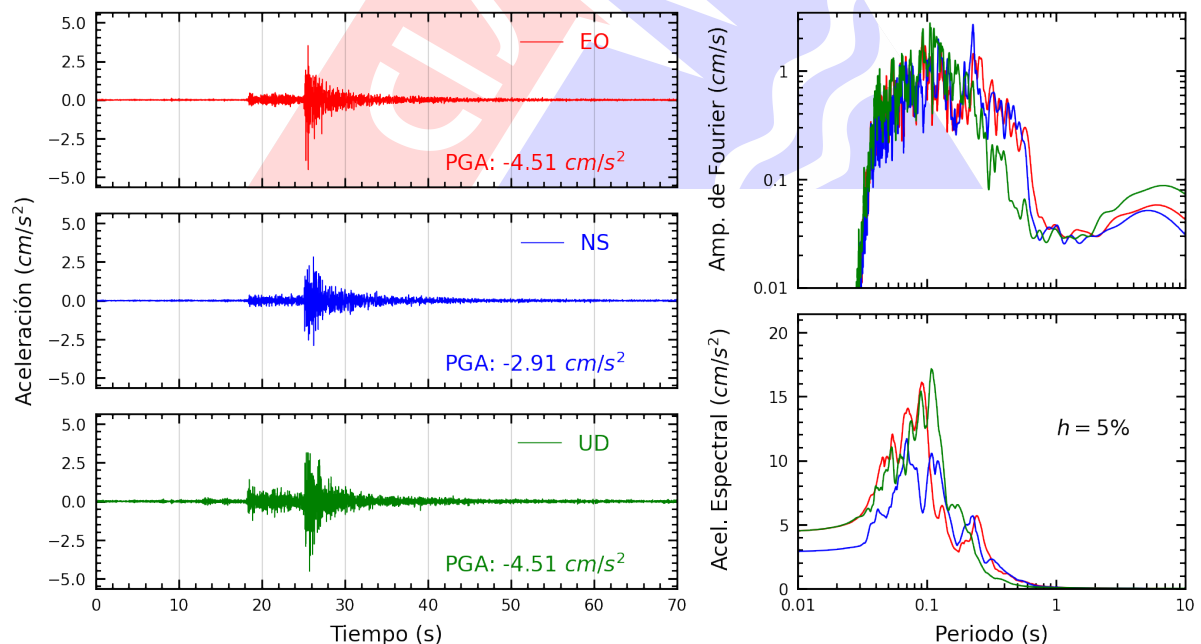
Figura A.10: Registros tiempo-historia, espectros de Fourier y de respuesta en las direcciones EO, NS y vertical de la estación MDPP. Sismo de Ancon, Lima - Lima del 2022-12-19, 20:30:07 (Hora local)
