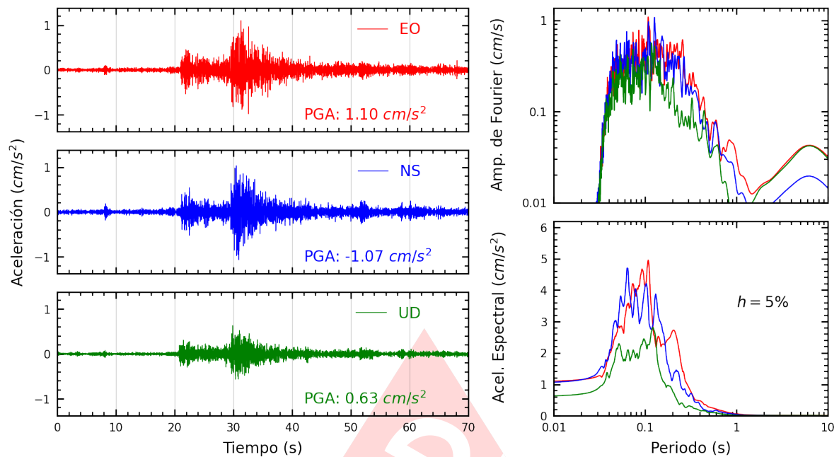
Figura A.31: Registros tiempo-historia, espectros de Fourier y de respuesta en las direcciones EO, NS y vertical de la estación BRISA. Sismo de Ancon, Lima - Lima del 2022-12-19, 20:30:07 (Hora local)
