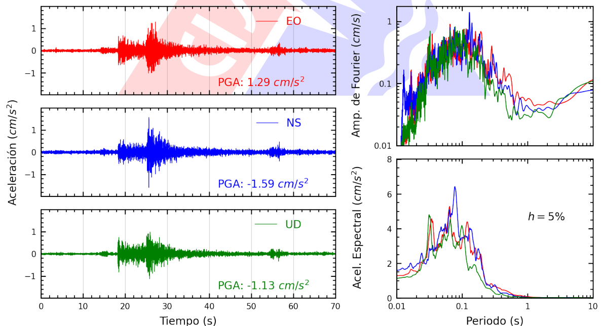
Figura A.24: Registros tiempo-historia, espectros de Fourier y de respuesta en las direcciones EO, NS y vertical de la estación NISTA. Sismo de Ancon, Lima - Lima del 2022-12-19, 20:30:07 (Hora local)
