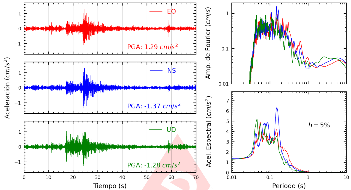
Figura A.27: Registros tiempo-historia, espectros de Fourier y de respuesta en las direcciones EO, NS y vertical de la estación PRADO. Sismo de Ancon, Lima - Lima del 2022-12-19, 20:30:07 (Hora local)
