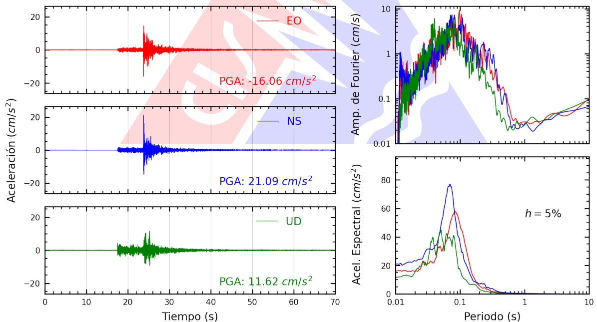
Figura A.2: Registros tiempo-historia, espectros de Fourier y de respuesta en las direcciones EO, NS y vertical de la estación ANCON. Sismo de Ancon, Lima - Lima del 2022-12-19, 20:30:07 (Hora local)
