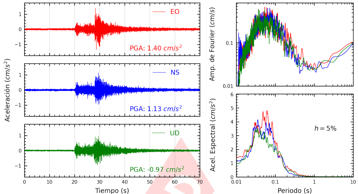
Figura A.25: Registros tiempo-historia, espectros de Fourier y de respuesta en las direcciones EO, NS y vertical de la estación SERVI. Sismo de Ancon, Lima - Lima del 2022-12-19, 20:30:07 (Hora local)
