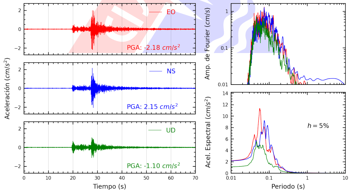
Figura A.16: Registros tiempo-historia, espectros de Fourier y de respuesta en las direcciones EO, NS y vertical de la estación ATARJ. Sismo de Ancon, Lima - Lima del 2022-12-19, 20:30:07 (Hora local)
