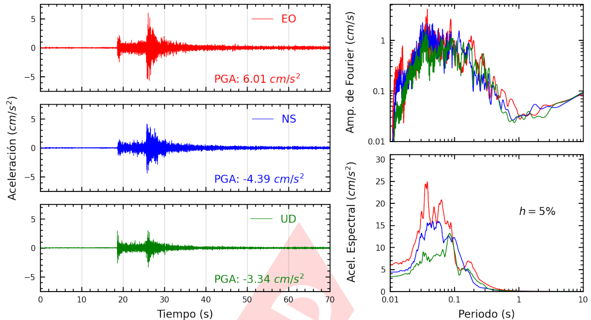
Figura A.5: Registros tiempo-historia, espectros de Fourier y de respuesta en las direcciones EO, NS y vertical de la estación COMAS. Sismo de Ancon, Lima - Lima del 2022-12-19, 20:30:07 (Hora local)
