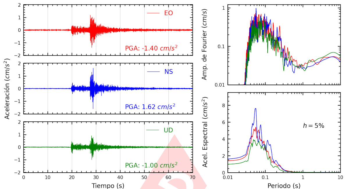
Figura A.23: Registros tiempo-historia, espectros de Fourier y de respuesta en las direcciones EO, NS y vertical de la estación INICT. Sismo de Ancon, Lima - Lima del 2022-12-19, 20:30:07 (Hora local)
