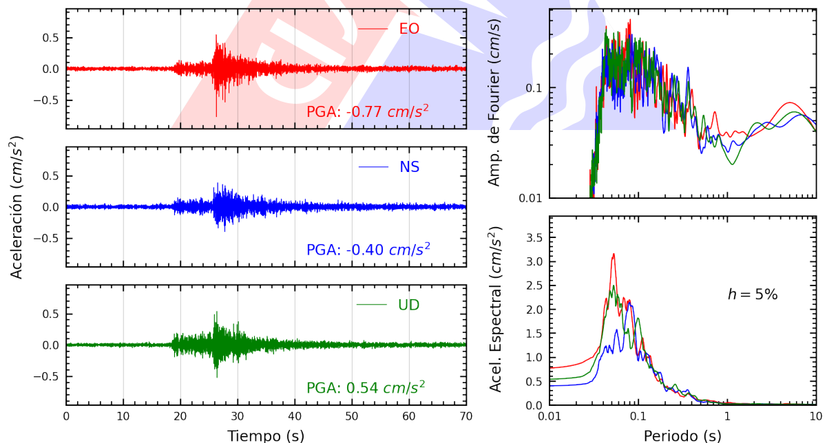
Figura A.34: Registros tiempo-historia, espectros de Fourier y de respuesta en las direcciones EO, NS y vertical de la estación BONDY. Sismo de Ancon, Lima - Lima del 2022-12-19, 20:30:07 (Hora local)
