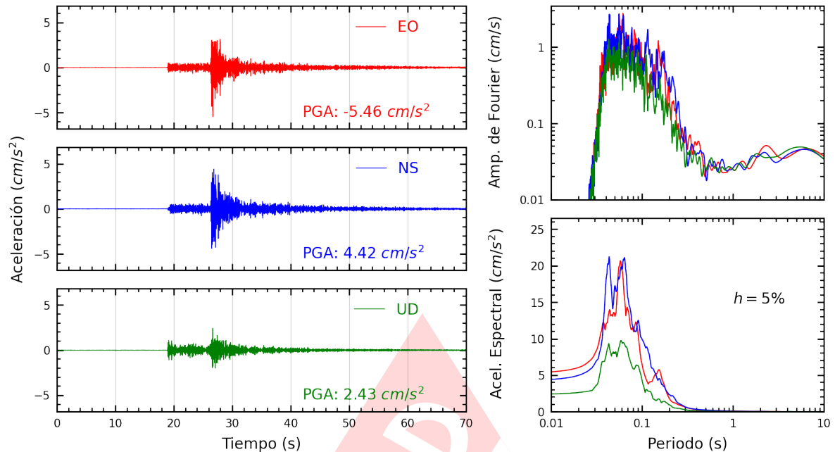
Figura A.7: Registros tiempo-historia, espectros de Fourier y de respuesta en las direcciones EO, NS y vertical de la estación IPEN. Sismo de Ancon, Lima - Lima del 2022-12-19, 20:30:07 (Hora local)
