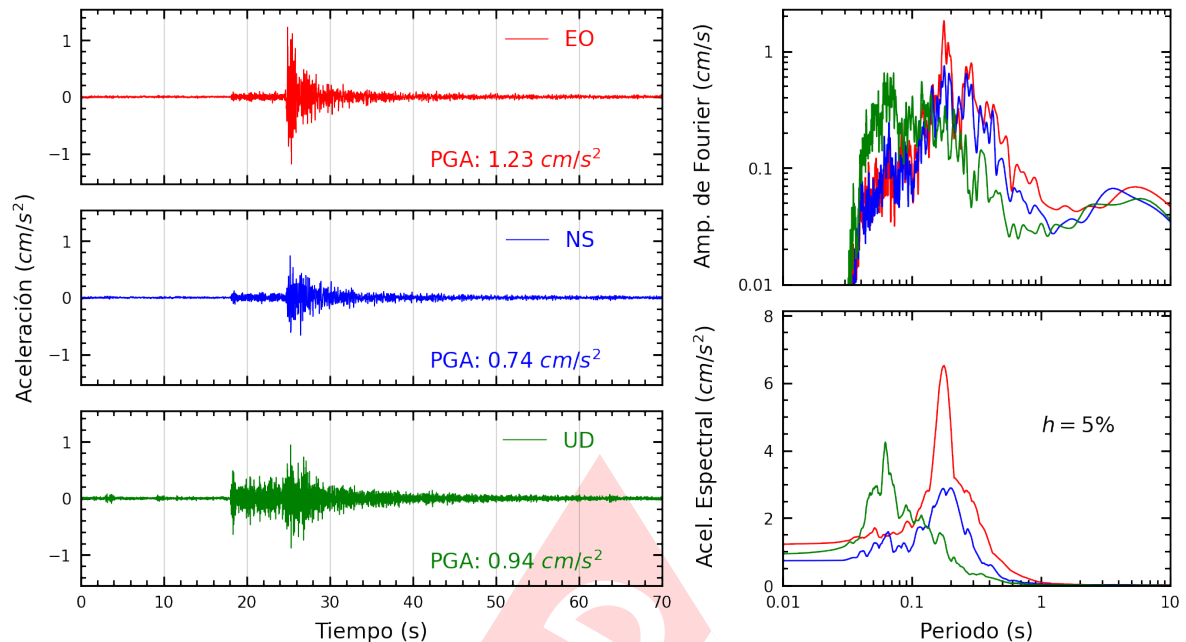
Figura A.29: Registros tiempo-historia, espectros de Fourier y de respuesta en las direcciones EO, NS y vertical de la estación ACAPU. Sismo de Ancon, Lima - Lima del 2022-12-19, 20:30:07 (Hora local)
