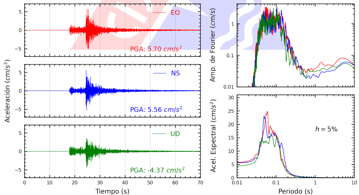
Figura A.6: Registros tiempo-historia, espectros de Fourier y de respuesta en las direcciones EO, NS y vertical de la estación AMORE. Sismo de Ancon, Lima - Lima del 2022-12-19, 20:30:07 (Hora local)
