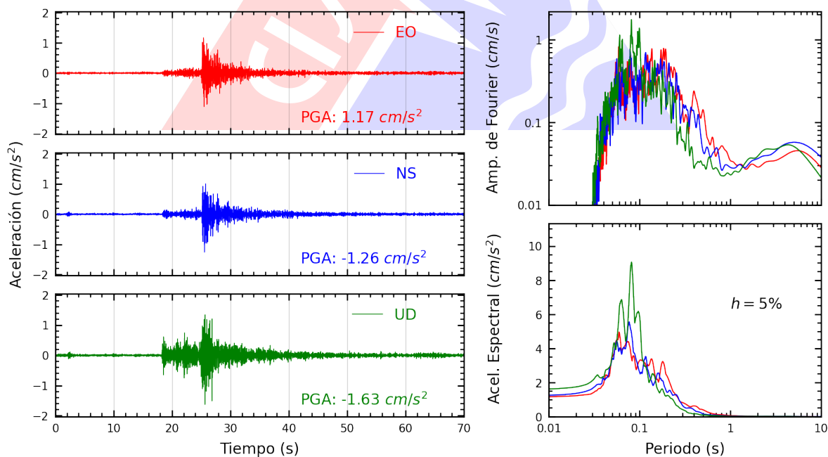
Figura A.22: Registros tiempo-historia, espectros de Fourier y de respuesta en las direcciones EO, NS y vertical de la estación RAMON. Sismo de Ancon, Lima - Lima del 2022-12-19, 20:30:07 (Hora local)
