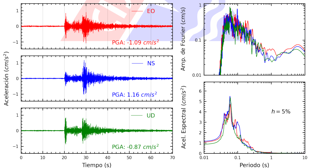
Figura A.30: Registros tiempo-historia, espectros de Fourier y de respuesta en las direcciones EO, NS y vertical de la estación IMCA. Sismo de Ancon, Lima - Lima del 2022-12-19, 20:30:07 (Hora local)
