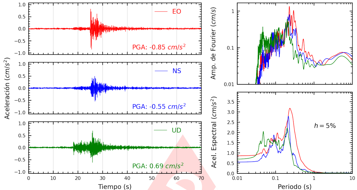
Figura A.33: Registros tiempo-historia, espectros de Fourier y de respuesta en las direcciones EO, NS y vertical de la estación DSML. Sismo de Ancon, Lima - Lima del 2022-12-19, 20:30:07 (Hora local)
