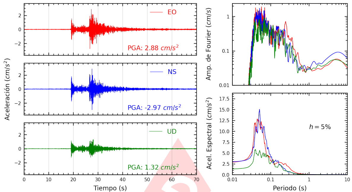
Figura A.13: Registros tiempo-historia, espectros de Fourier y de respuesta en las direcciones EO, NS y vertical de la estación CEPRE. Sismo de Ancon, Lima - Lima del 2022-12-19, 20:30:07 (Hora local)
