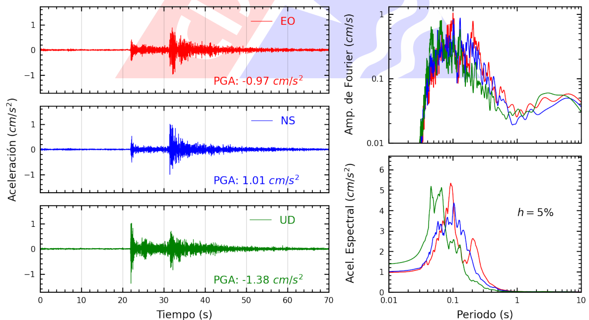
Figura A.26: Registros tiempo-historia, espectros de Fourier y de respuesta en las direcciones EO, NS y vertical de la estación USILP. Sismo de Ancon, Lima - Lima del 2022-12-19, 20:30:07 (Hora local)
