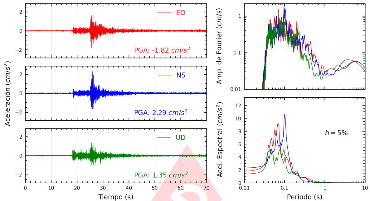
Figura A.15: Registros tiempo-historia, espectros de Fourier y de respuesta en las direcciones EO, NS y vertical de la estación MADRE. Sismo de Ancon, Lima - Lima del 2022-12-19, 20:30:07 (Hora local)
