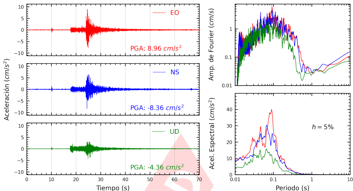
Figura A.3: Registros tiempo-historia, espectros de Fourier y de respuesta en las direcciones EO, NS y vertical de la estación DEFEN. Sismo de Ancon, Lima - Lima del 2022-12-19, 20:30:07 (Hora local)
