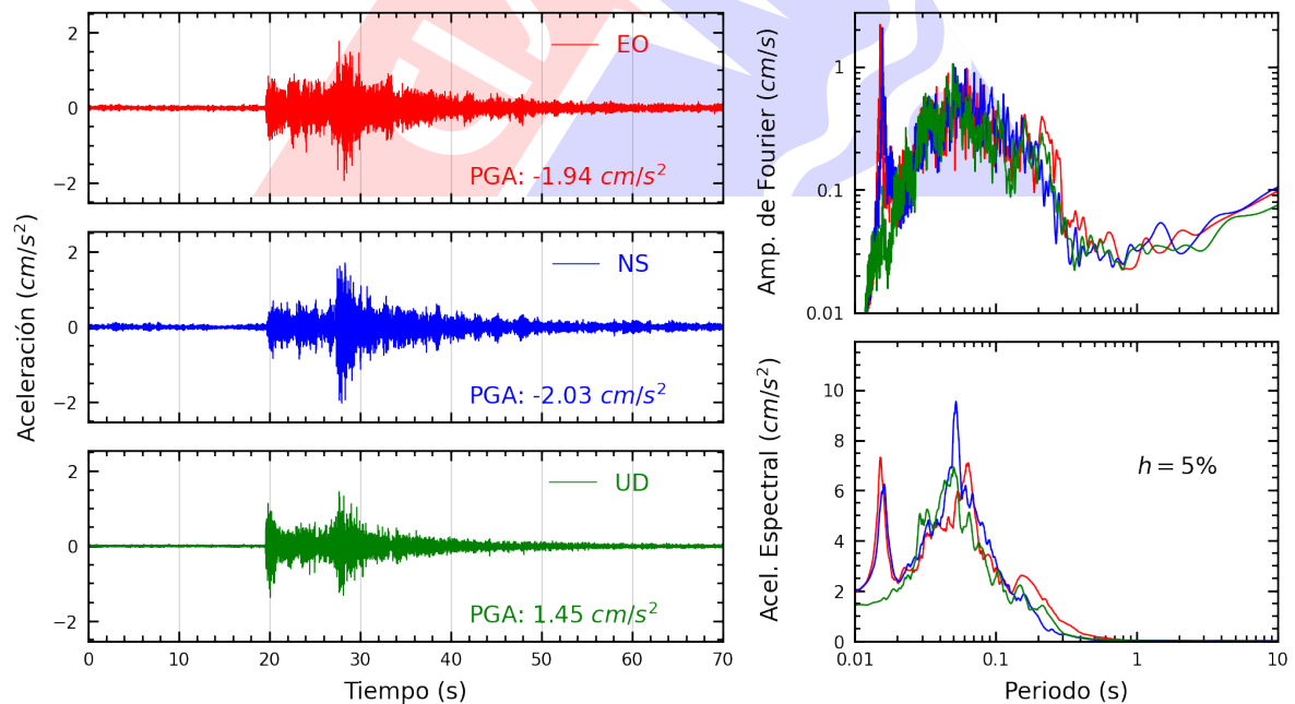
Figura A.20: Registros tiempo-historia, espectros de Fourier y de respuesta en las direcciones EO, NS y vertical de la estación CENEP. Sismo de Ancon, Lima - Lima del 2022-12-19, 20:30:07 (Hora local)
