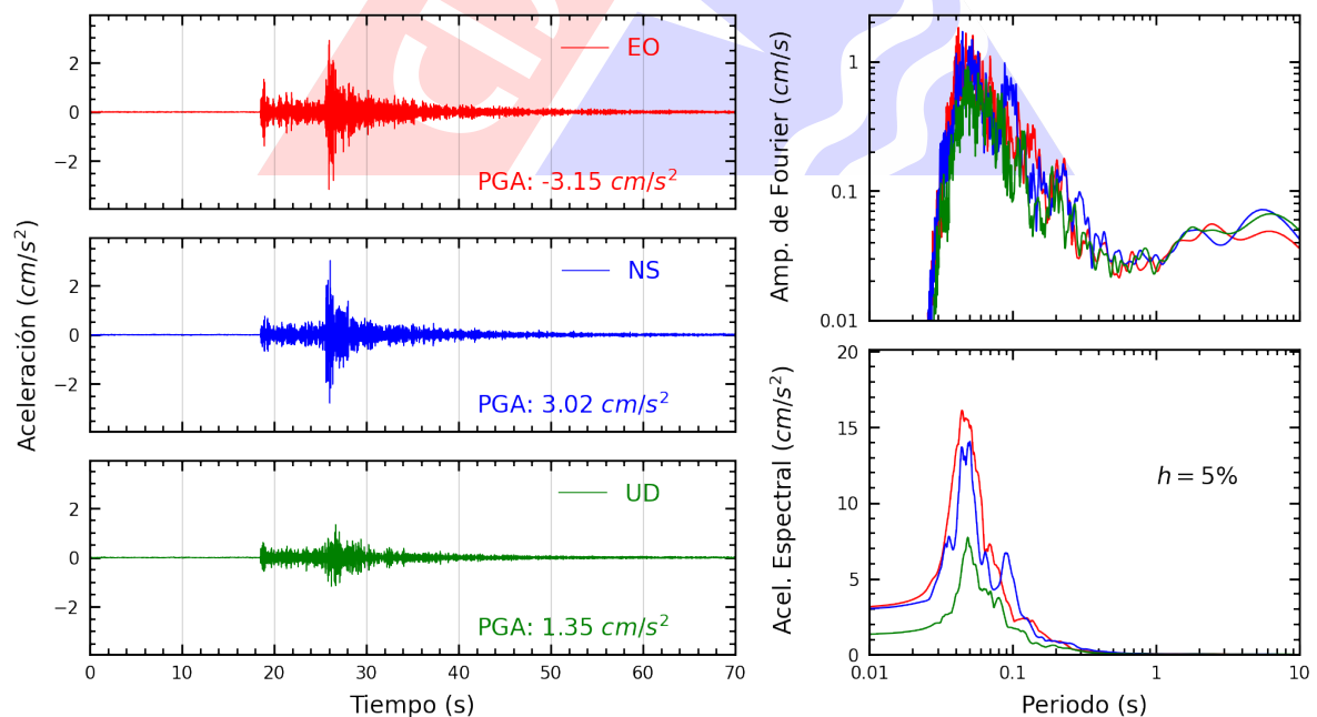
Figura A.12: Registros tiempo-historia, espectros de Fourier y de respuesta en las direcciones EO, NS y vertical de la estación UCSS. Sismo de Ancon, Lima - Lima del 2022-12-19, 20:30:07 (Hora local)
