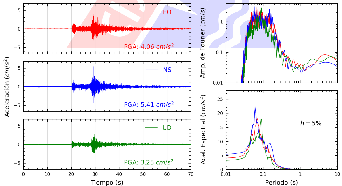
Figura A.8: Registros tiempo-historia, espectros de Fourier y de respuesta en las direcciones EO, NS y vertical de la estación USILM. Sismo de Ancon, Lima - Lima del 2022-12-19, 20:30:07 (Hora local)
