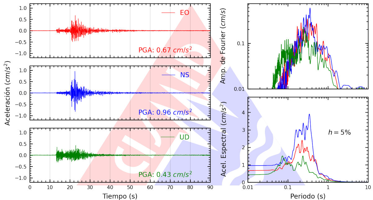
Figura A.3: Registros tiempo-historia, espectros de Fourier y de respuesta en las direcciones EO, NS y vertical de la estación UNIPE. Sismo de Sullana, Sullana - Piura del 2023-01-17, 13:33:51 (Hora local)
