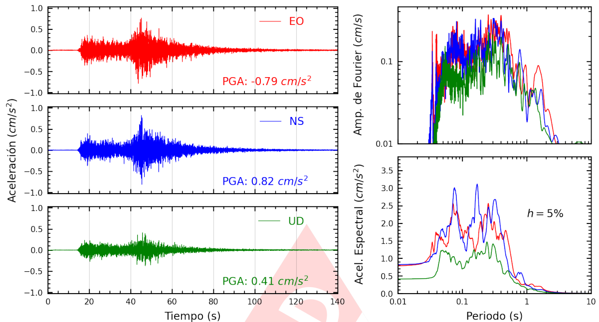
Figura A.3: Registros tiempo-historia, espectros de Fourier y de respuesta en las direcciones EO, NS y vertical de la estación UNAM. Sismo de Tacna, Tacna - Tacna del 2023-02-03, 04:50:50 (Hora local)
