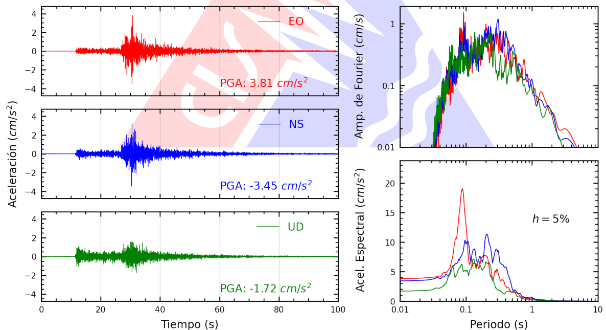
Figura A.2: Registros tiempo-historia, espectros de Fourier y de respuesta en las direcciones EO, NS y vertical de la estación UJBG2. Sismo de Tacna, Tacna - Tacna del 2023-02-03, 04:50:50 (Hora local)
