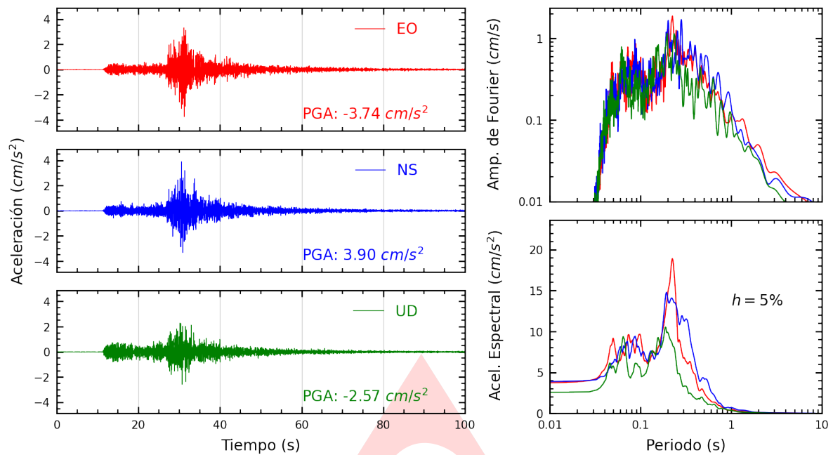
Figura A.1: Registros tiempo-historia, espectros de Fourier y de respuesta en las direcciones EO, NS y vertical de la estación CREY. Sismo de Tacna, Tacna - Tacna del 2023-02-03, 04:50:50 (Hora local)
