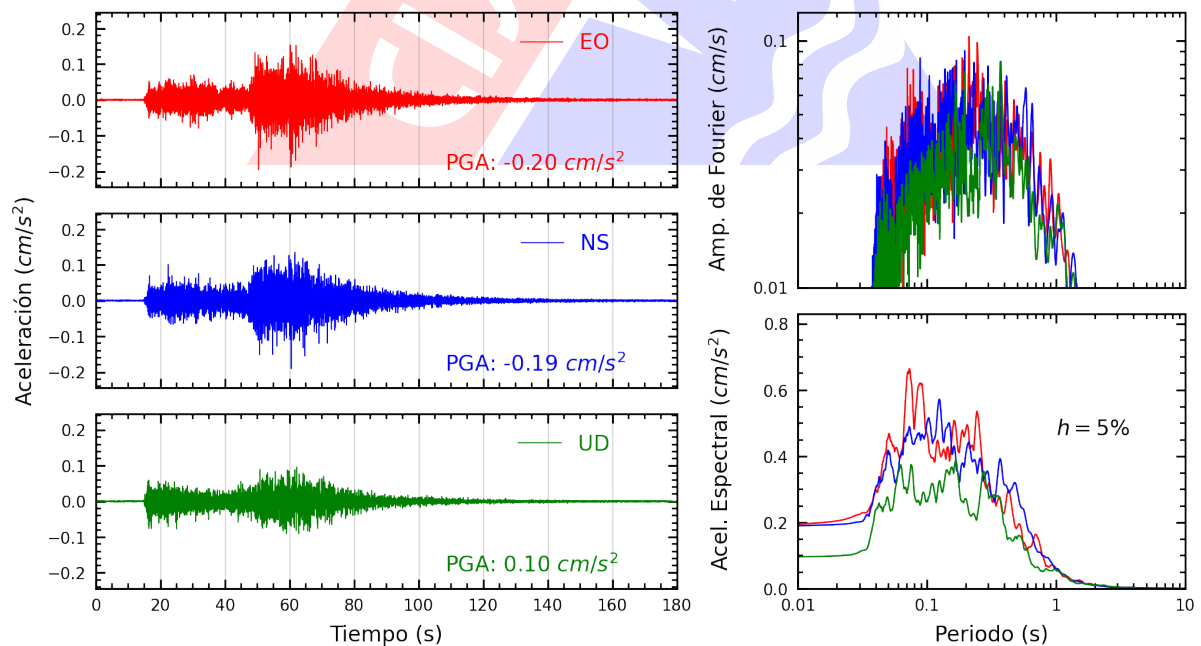
Figura A.4: Registros tiempo-historia, espectros de Fourier y de respuesta en las direcciones EO, NS y vertical de la estación UNSA. Sismo de Tacna, Tacna - Tacna del 2023-02-03, 04:50:50 (Hora local)
