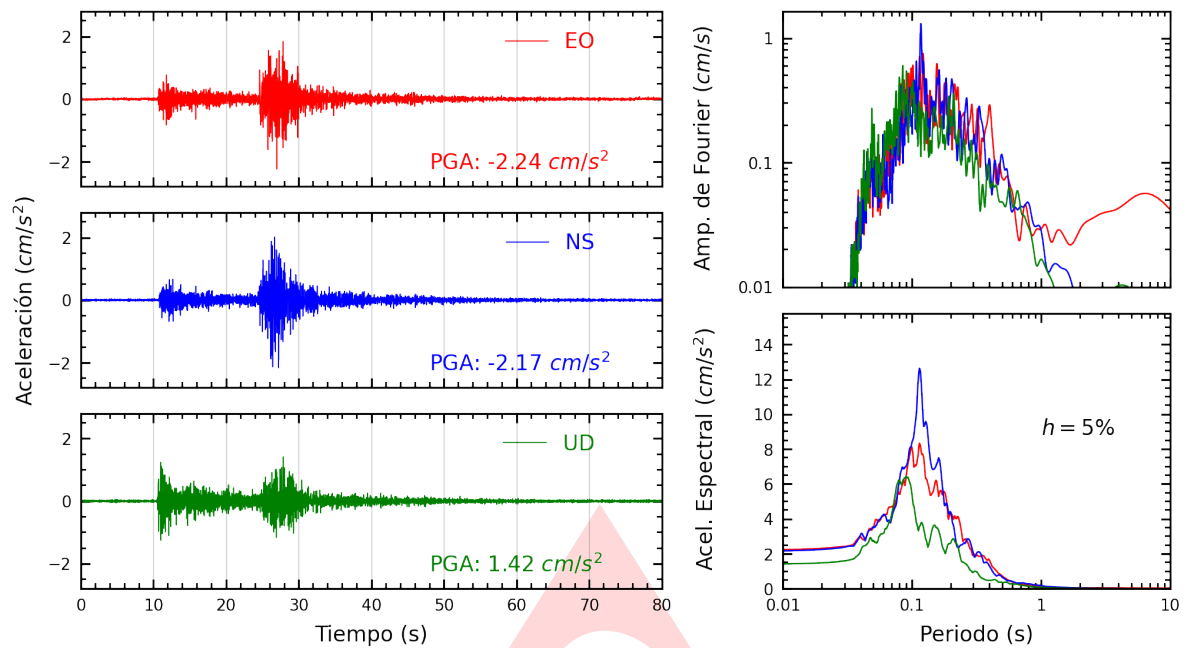
Figura A.1: Registros tiempo-historia, espectros de Fourier y de respuesta en las direcciones EO, NS y vertical de la estación UJBG3. Sismo de Calana, Tacna - Tacna del 2023-05-25, 15:20:12 (Hora local)
