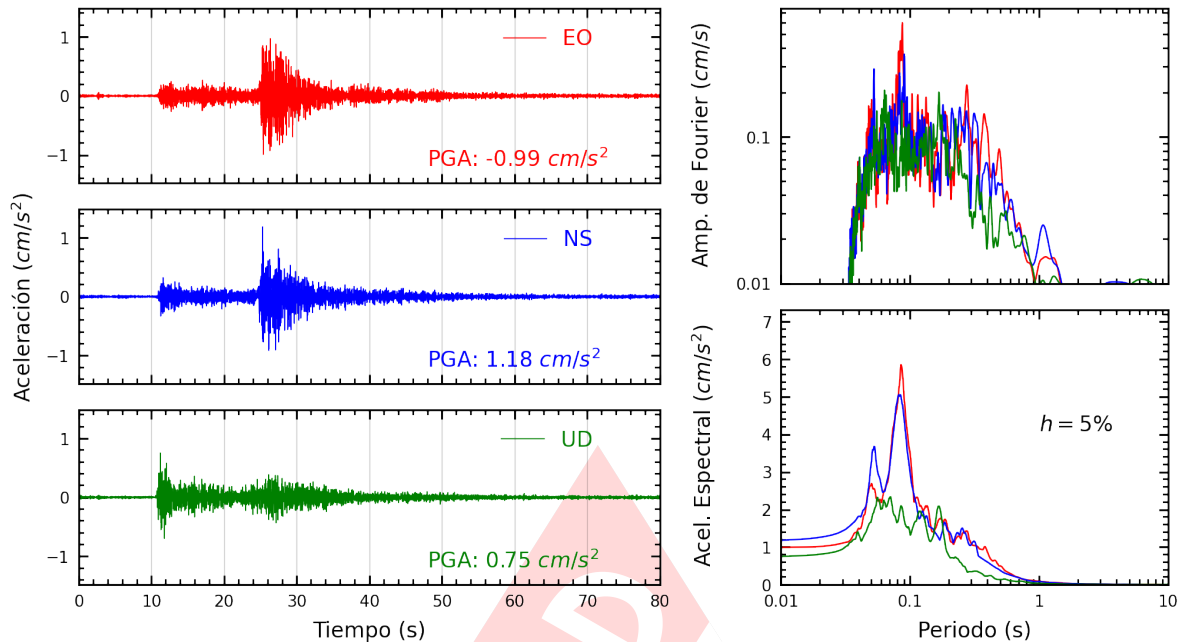
Figura A.3: Registros tiempo-historia, espectros de Fourier y de respuesta en las direcciones EO, NS y vertical de la estación CREY. Sismo de Calana, Tacna - Tacna del 2023-05-25, 15:20:12 (Hora local)
