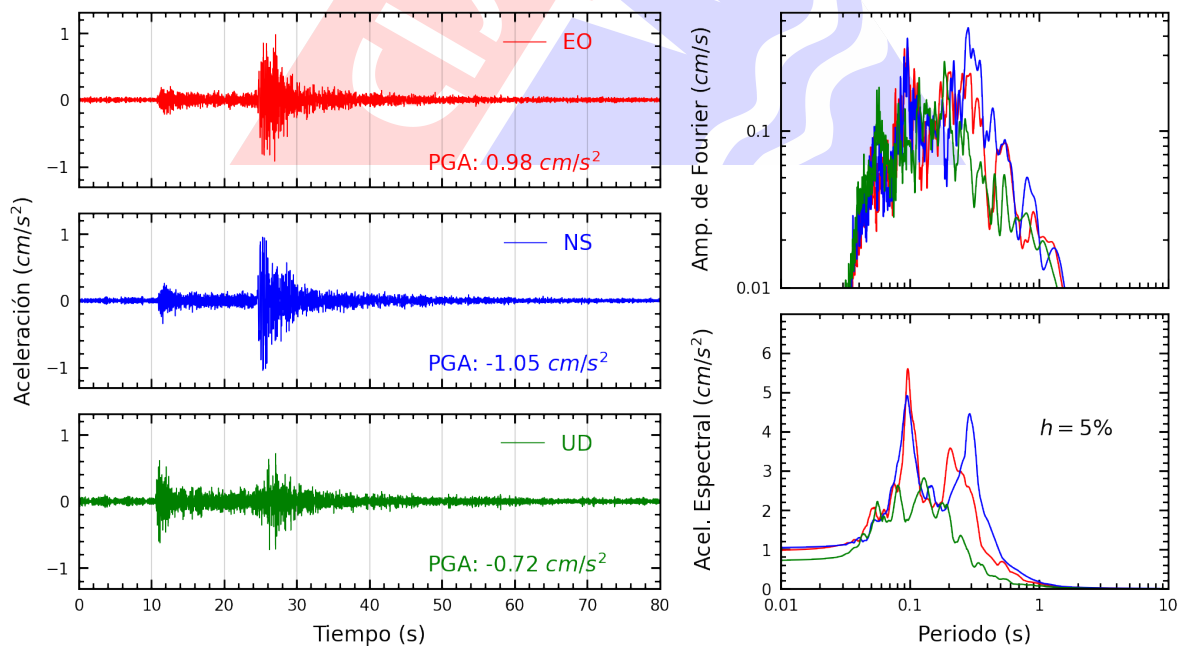
Figura A.4: Registros tiempo-historia, espectros de Fourier y de respuesta en las direcciones EO, NS y vertical de la estación UJBG2. Sismo de Calana, Tacna - Tacna del 2023-05-25, 15:20:12 (Hora local)
