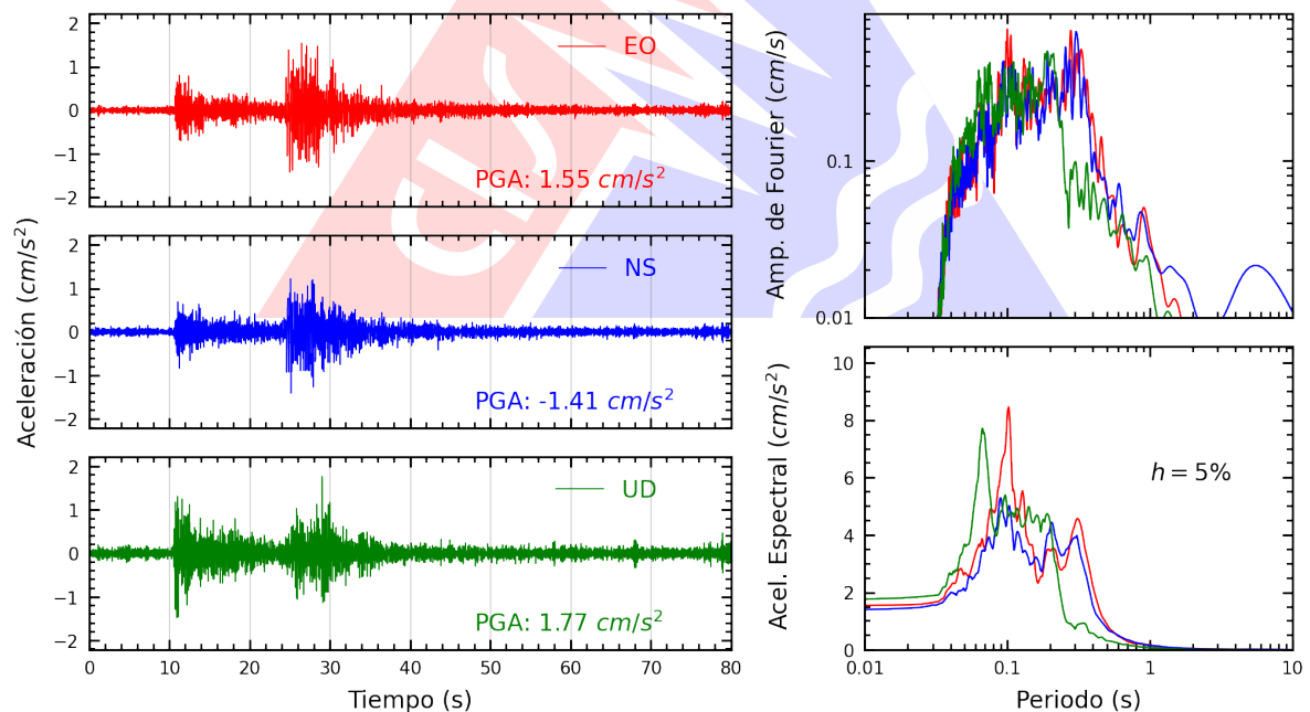
Figura A.2: Registros tiempo-historia, espectros de Fourier y de respuesta en las direcciones EO, NS y vertical de la estación SCTAC. Sismo de Calana, Tacna - Tacna del 2023-05-25, 15:20:12 (Hora local)
