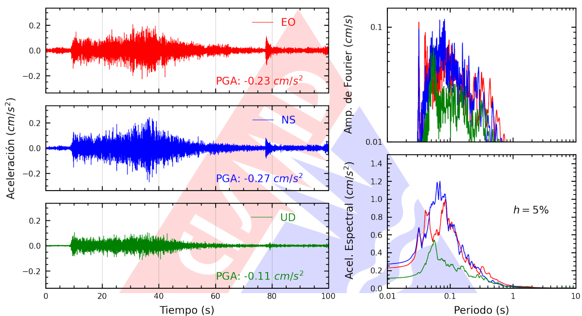
Figura A.5: Registros tiempo-historia, espectros de Fourier y de respuesta en las direcciones EO, NS y vertical de la estación UNAM. Sismo de Calana, Tacna - Tacna del 2023-05-25, 15:20:12 (Hora local)
