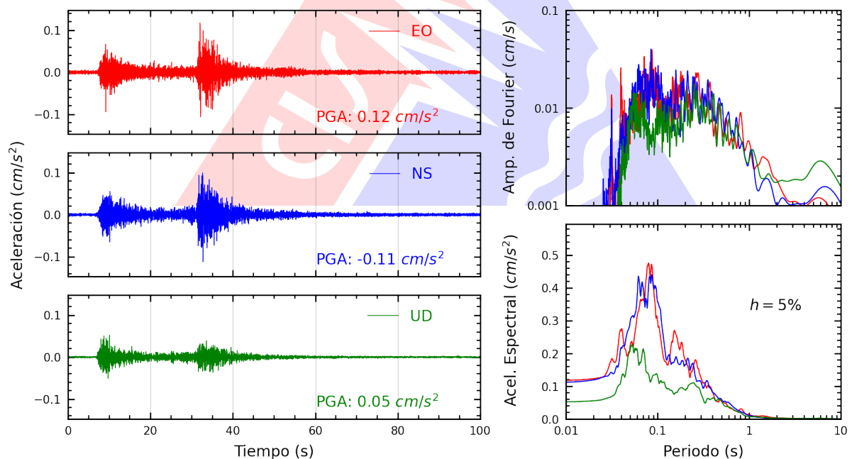
Figura A.2: Registros tiempo-historia, espectros de Fourier y de respuesta en las direcciones EO, NS y vertical de la estación UNAM. Sismo de Maca, Caylloma - Arequipa del 2023-06-03, 00:01:13 (Hora local)
