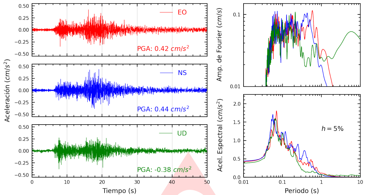
Figura A.1: Registros tiempo-historia, espectros de Fourier y de respuesta en las direcciones EO, NS y vertical de la estación SCARQ. Sismo de Maca, Caylloma - Arequipa del 2023-06-03, 00:01:13 (Hora local)
