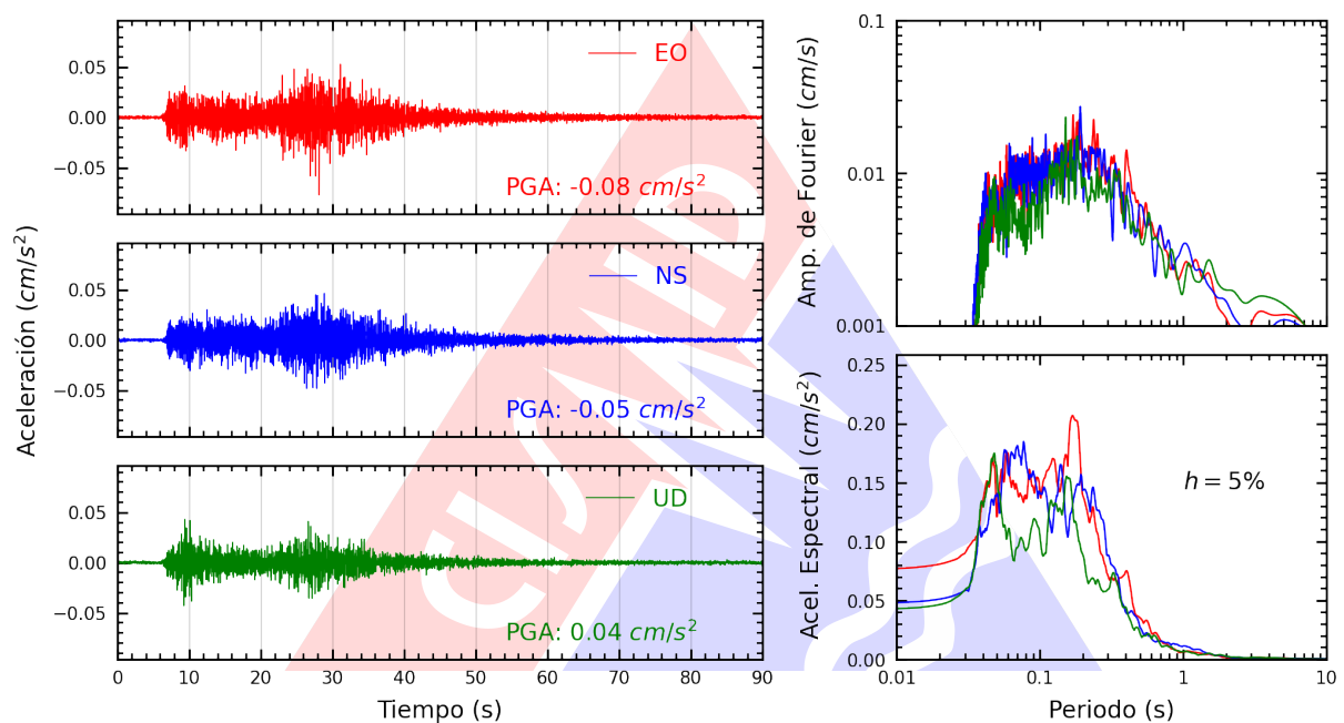
Figura A.3: Registros tiempo-historia, espectros de Fourier y de respuesta en las direcciones EO, NS y vertical de la estación UNSA. Sismo de Maca, Caylloma - Arequipa del 2023-06-03, 00:01:13 (Hora local)
