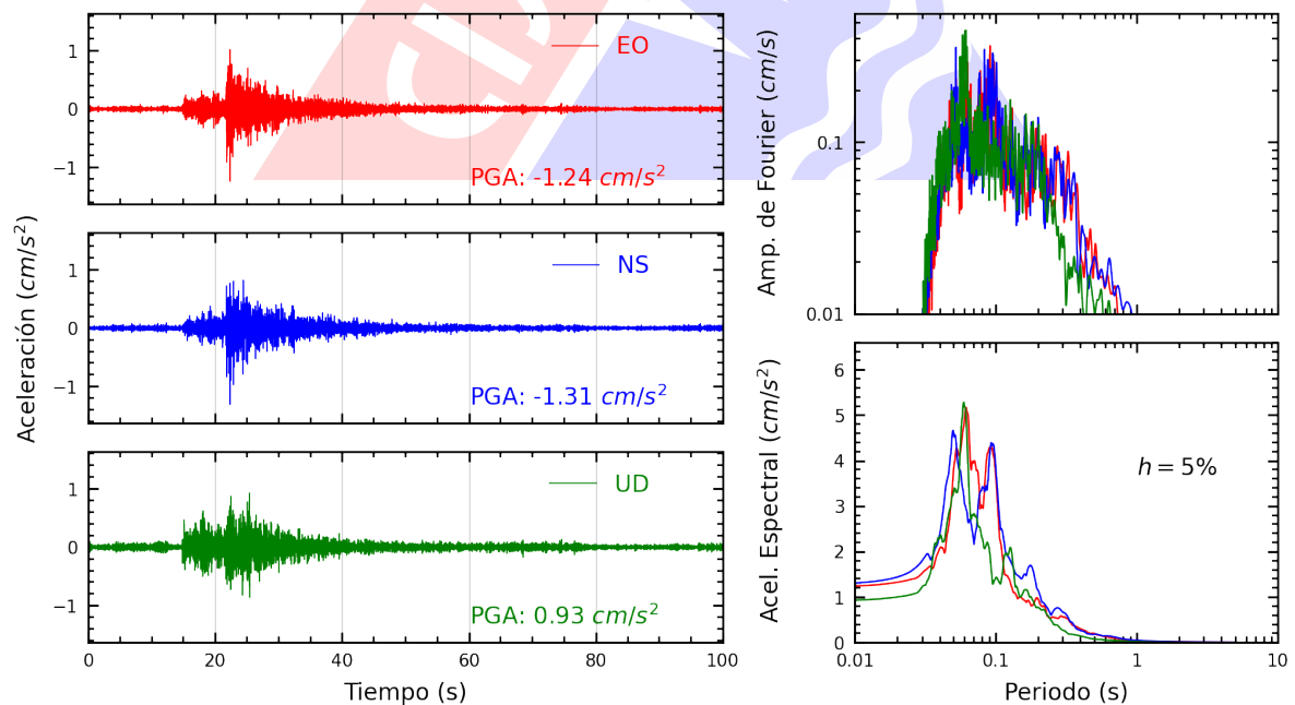
Figura A.4: Registros tiempo-historia, espectros de Fourier y de respuesta en las direcciones EO, NS y vertical de la estación UJBG2. Sismo de Tacna, Tacna - Tacna del 2023-06-15, 16:32:04 (Hora local)
