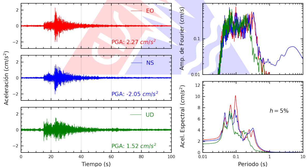
Figura A.2: Registros tiempo-historia, espectros de Fourier y de respuesta en las direcciones EO, NS y vertical de la estación SCTAC. Sismo de Tacna, Tacna - Tacna del 2023-06-15, 16:32:04 (Hora local)
