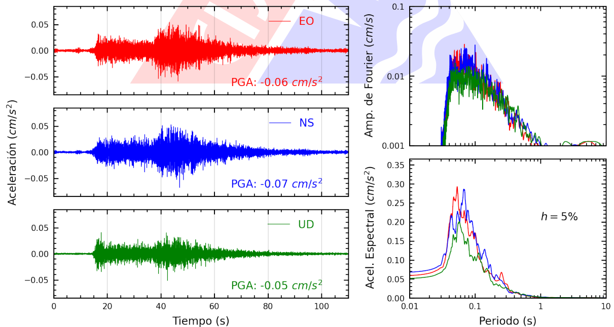
Figura A.6: Registros tiempo-historia, espectros de Fourier y de respuesta en las direcciones EO, NS y vertical de la estación UNSA. Sismo de Tacna, Tacna - Tacna del 2023-06-15, 16:32:04 (Hora local)
