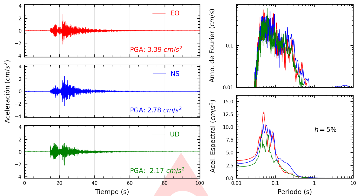
Figura A.1: Registros tiempo-historia, espectros de Fourier y de respuesta en las direcciones EO, NS y vertical de la estación CREY. Sismo de Tacna, Tacna - Tacna del 2023-06-15, 16:32:04 (Hora local)
