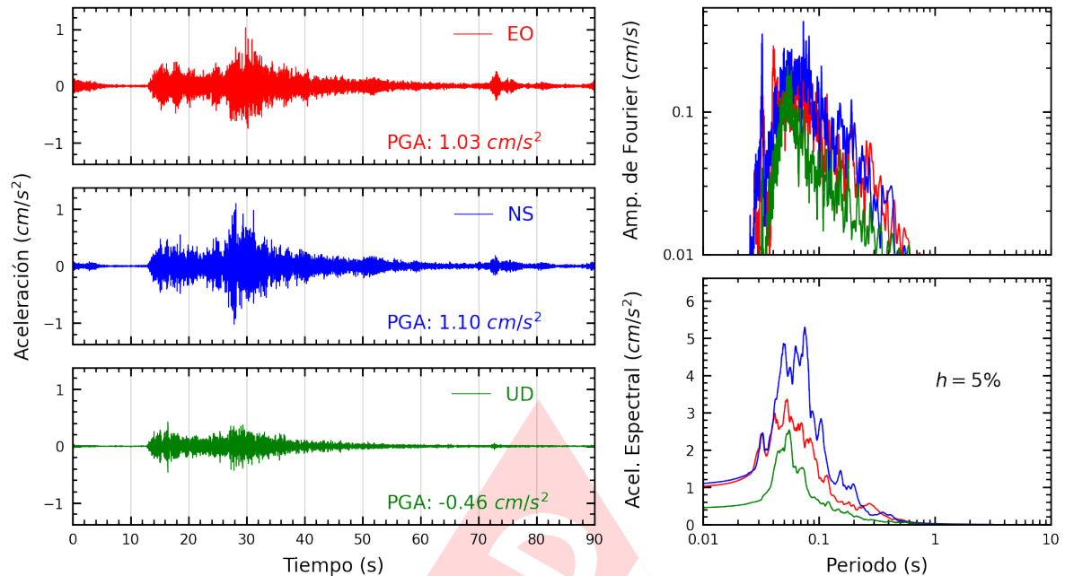
Figura A.5: Registros tiempo-historia, espectros de Fourier y de respuesta en las direcciones EO, NS y vertical de la estación UNAM. Sismo de Tacna, Tacna - Tacna del 2023-06-15, 16:32:04 (Hora local)
