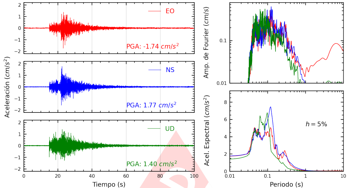
Figura A.3: Registros tiempo-historia, espectros de Fourier y de respuesta en las direcciones EO, NS y vertical de la estación UJBG3. Sismo de Tacna, Tacna - Tacna del 2023-06-15, 16:32:04 (Hora local)
