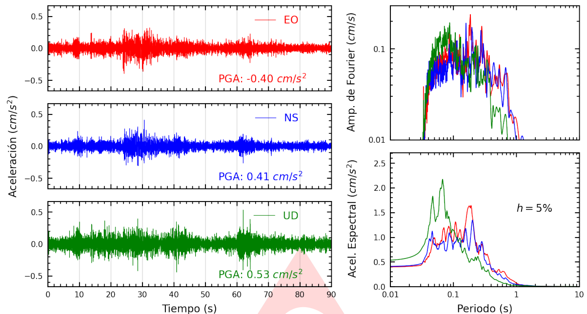
Figura A.1: Registros tiempo-historia, espectros de Fourier y de respuesta en las direcciones EO, NS y vertical de la estación SCICA. Sismo de Palpa, Palpa - Ica del 2023-08-14, 15:13:50 (Hora local)
