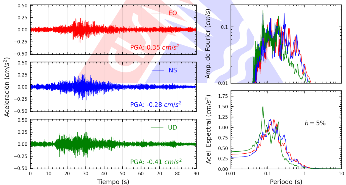
Figura A.2: Registros tiempo-historia, espectros de Fourier y de respuesta en las direcciones EO, NS y vertical de la estación UNICA. Sismo de Palpa, Palpa - Ica del 2023-08-14, 15:13:50 (Hora local)
