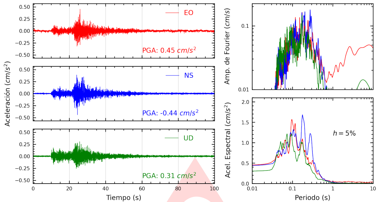
Figura A.1: Registros tiempo-historia, espectros de Fourier y de respuesta en las direcciones EO, NS y vertical de la estación UJBG3. Sismo de Tacna, Tacna - Tacna del 2023-08-27, 03:27:32 (Hora local)
