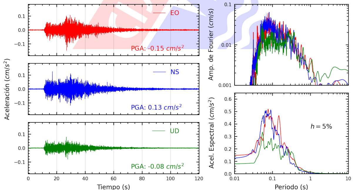
Figura A.4: Registros tiempo-historia, espectros de Fourier y de respuesta en las direcciones EO, NS y vertical de la estación UNAM. Sismo de Tacna, Tacna - Tacna del 2023-08-27, 03:27:32 (Hora local)
