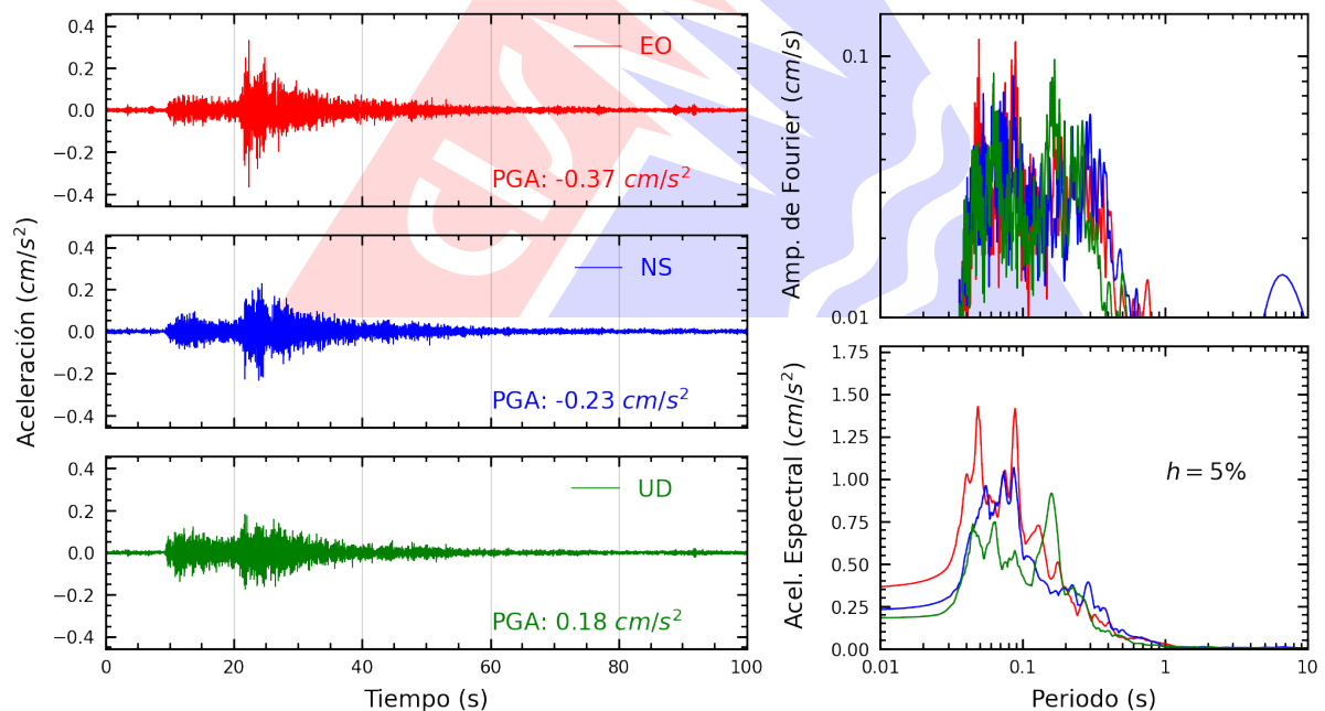
Figura A.2: Registros tiempo-historia, espectros de Fourier y de respuesta en las direcciones EO, NS y vertical de la estación CREY. Sismo de Tacna, Tacna - Tacna del 2023-08-27, 03:27:32 (Hora local)
