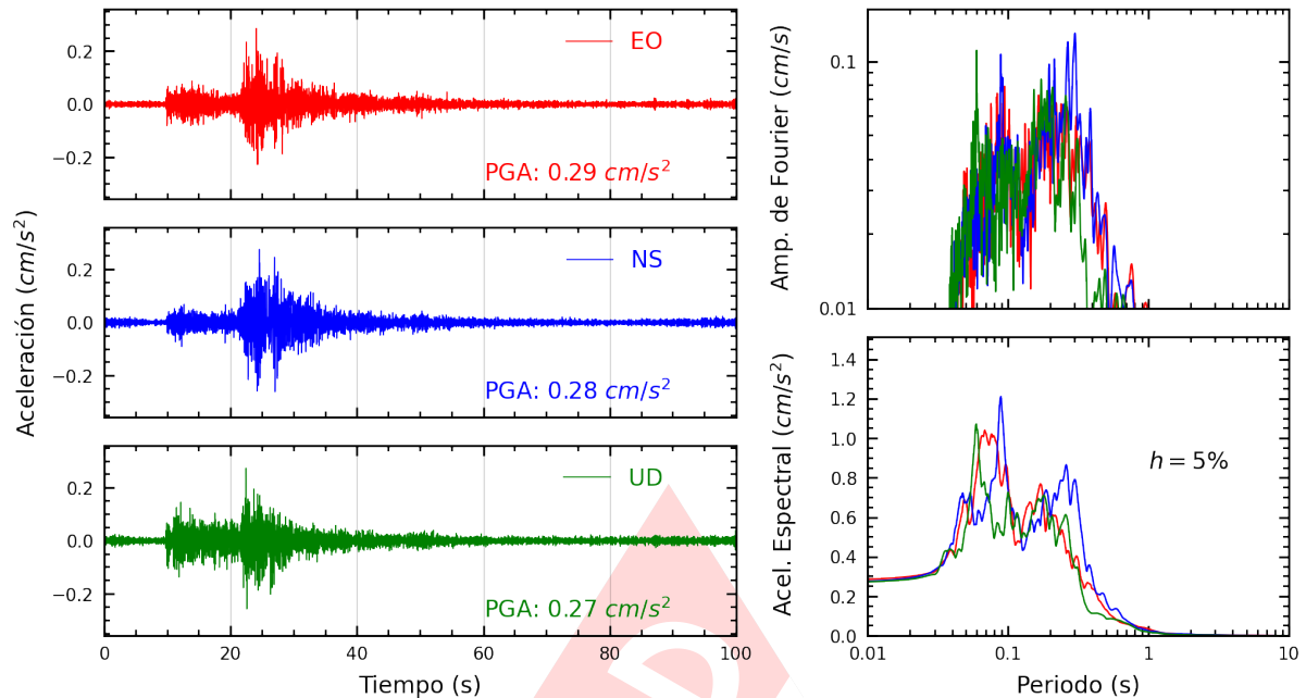
Figura A.3: Registros tiempo-historia, espectros de Fourier y de respuesta en las direcciones EO, NS y vertical de la estación UJBG2. Sismo de Tacna, Tacna - Tacna del 2023-08-27, 03:27:32 (Hora local)
