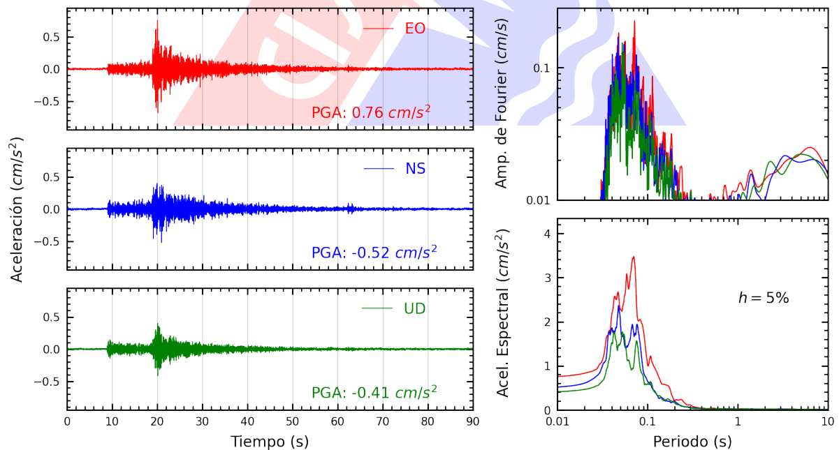
Figura A.14: Registros tiempo-historia, espectros de Fourier y de respuesta en las direcciones EO, NS y vertical de la estación FICPE. Sismo de Chilca, Cañete - Lima del 2023-09-07, 01:53:09 (Hora local)
