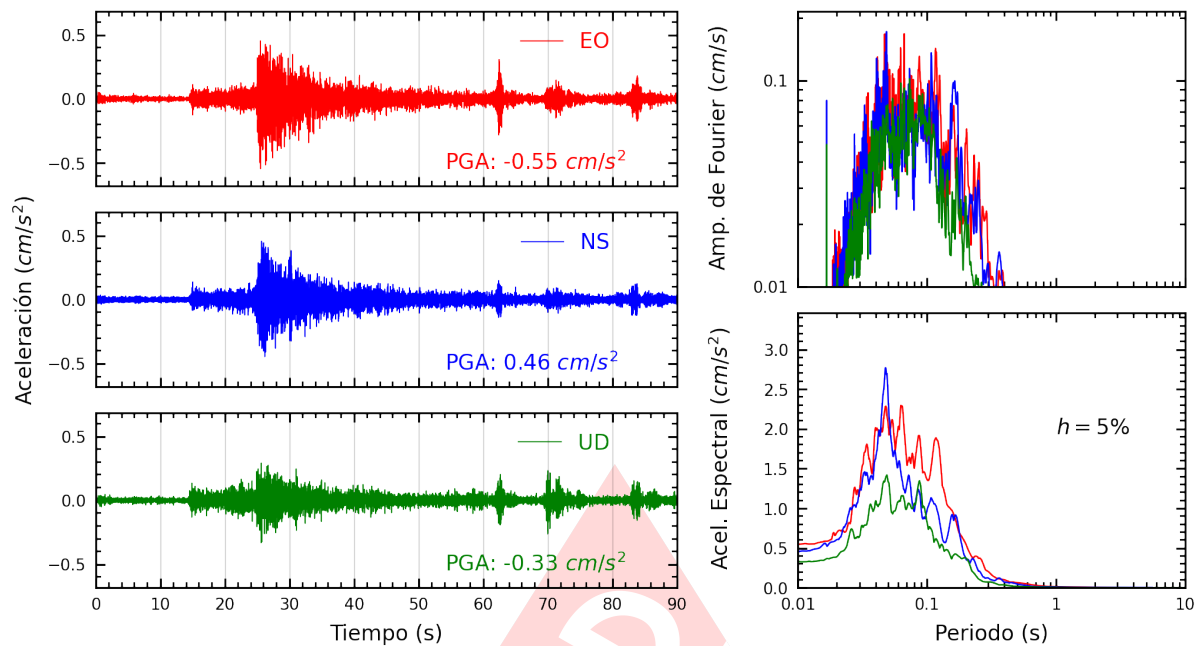
Figura A.21: Registros tiempo-historia, espectros de Fourier y de respuesta en las direcciones EO, NS y vertical de la estación SCOLI. Sismo de Chilca, Cañete - Lima del 2023-09-07, 01:53:09 (Hora local)
