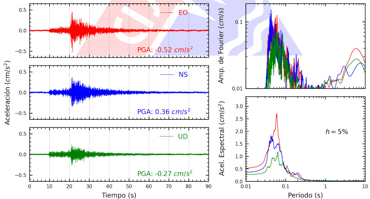
Figura A.22: Registros tiempo-historia, espectros de Fourier y de respuesta en las direcciones EO, NS y vertical de la estación COMAS. Sismo de Chilca, Cañete - Lima del 2023-09-07, 01:53:09 (Hora local)
