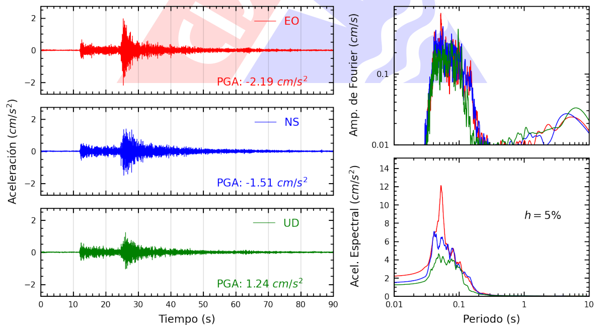
Figura A.4: Registros tiempo-historia, espectros de Fourier y de respuesta en las direcciones EO, NS y vertical de la estación SROSA. Sismo de Chilca, Cañete - Lima del 2023-09-07, 01:53:09 (Hora local)
