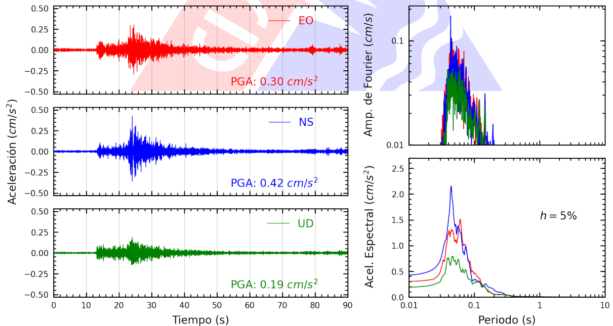
Figura A.26: Registros tiempo-historia, espectros de Fourier y de respuesta en las direcciones EO, NS y vertical de la estación BORJA. Sismo de Chilca, Cañete - Lima del 2023-09-07, 01:53:09 (Hora local)
