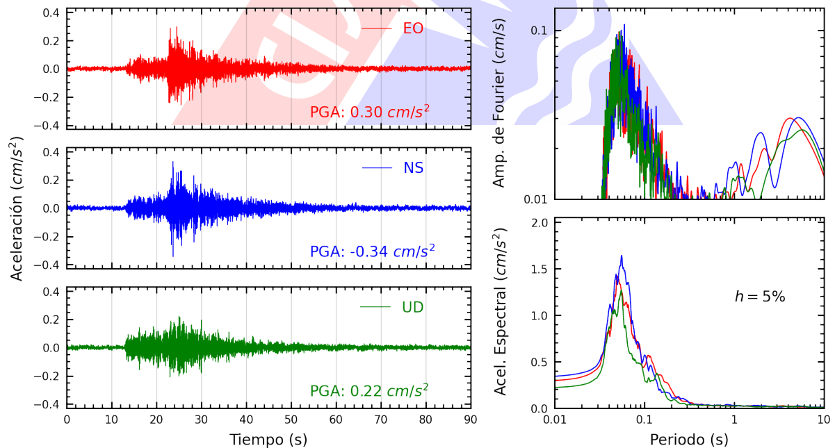
Figura A.30: Registros tiempo-historia, espectros de Fourier y de respuesta en las direcciones EO, NS y vertical de la estación CENEP. Sismo de Chilca, Cañete - Lima del 2023-09-07, 01:53:09 (Hora local)
