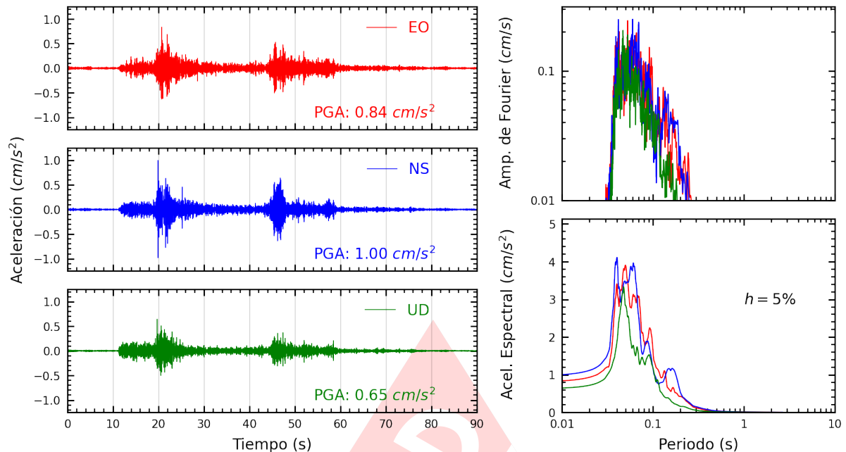
Figura A.9: Registros tiempo-historia, espectros de Fourier y de respuesta en las direcciones EO, NS y vertical de la estación PACHA. Sismo de Chilca, Cañete - Lima del 2023-09-07, 01:53:09 (Hora local)
