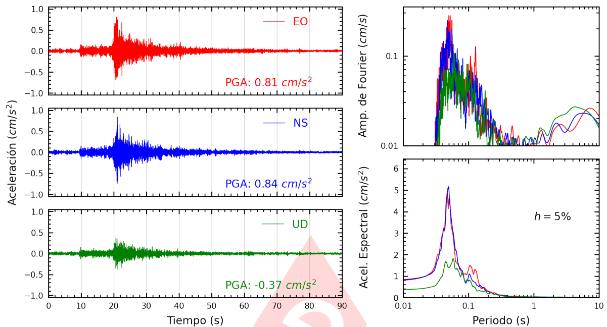
Figura A.13: Registros tiempo-historia, espectros de Fourier y de respuesta en las direcciones EO, NS y vertical de la estación OLIVO. Sismo de Chilca, Cañete - Lima del 2023-09-07, 01:53:09 (Hora local)
