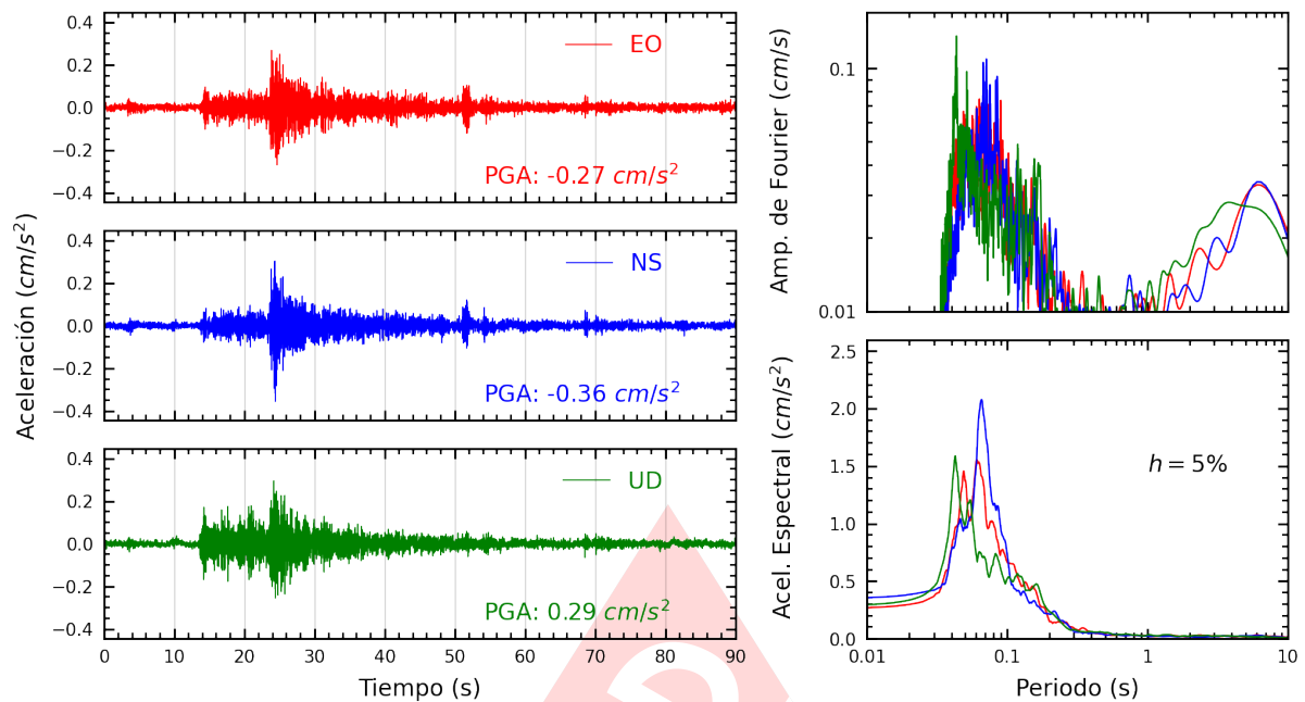
Figura A.27: Registros tiempo-historia, espectros de Fourier y de respuesta en las direcciones EO, NS y vertical de la estación UPCS. Sismo de Chilca, Cañete - Lima del 2023-09-07, 01:53:09 (Hora local)
