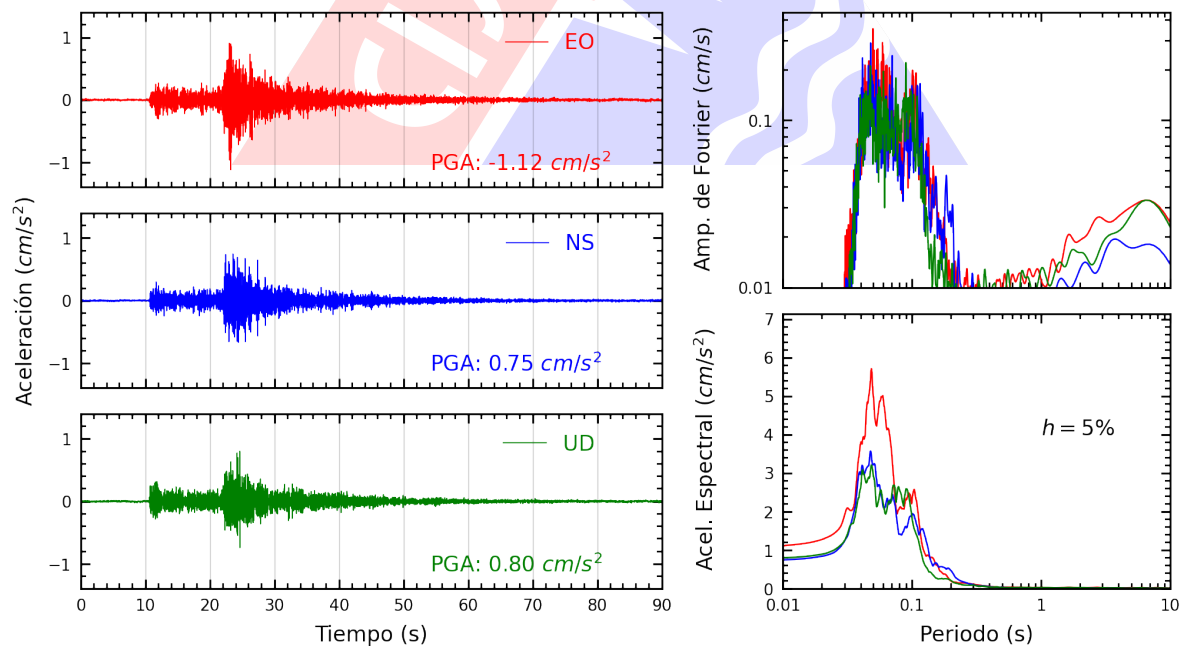
Figura A.6: Registros tiempo-historia, espectros de Fourier y de respuesta en las direcciones EO, NS y vertical de la estación AMORE. Sismo de Chilca, Cañete - Lima del 2023-09-07, 01:53:09 (Hora local)
