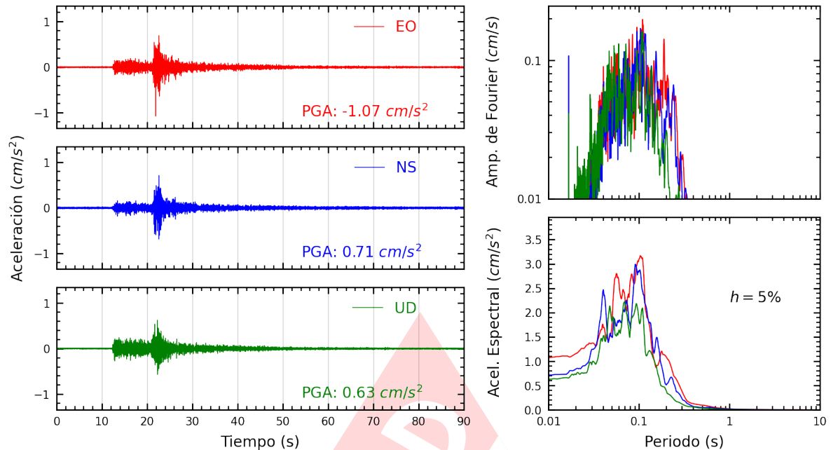
Figura A.7: Registros tiempo-historia, espectros de Fourier y de respuesta en las direcciones EO, NS y vertical de la estación SCCHO. Sismo de Chilca, Cañete - Lima del 2023-09-07, 01:53:09 (Hora local)
