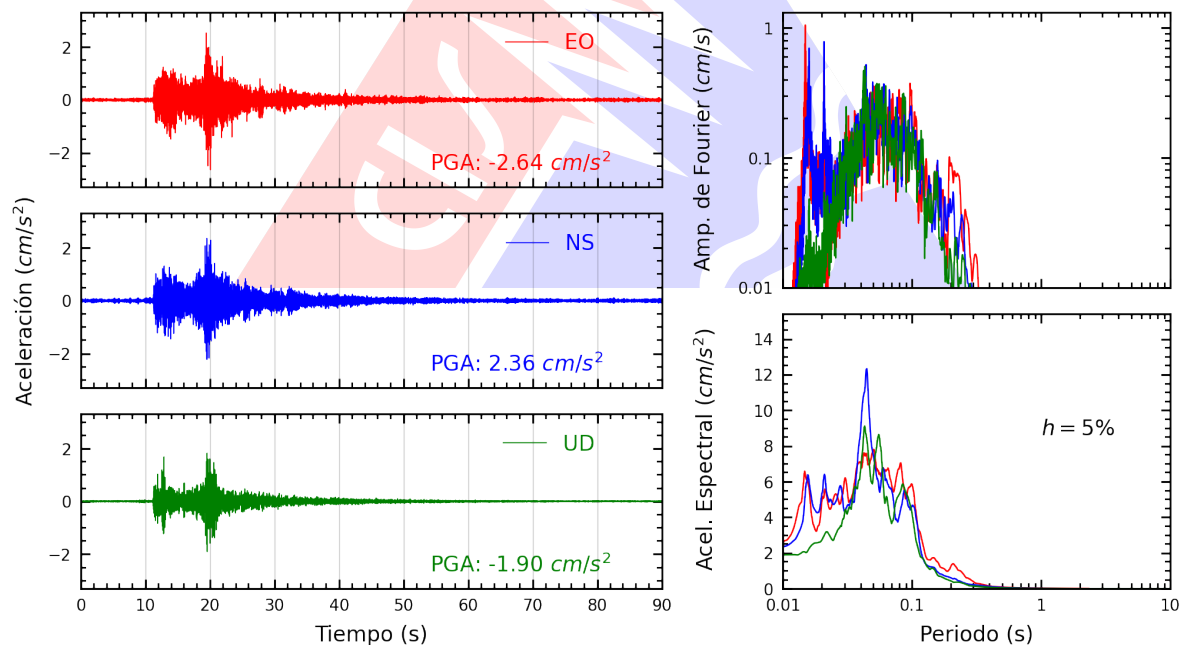
Figura A.2: Registros tiempo-historia, espectros de Fourier y de respuesta en las direcciones EO, NS y vertical de la estación ASIA. Sismo de Chilca, Cañete - Lima del 2023-09-07, 01:53:09 (Hora local)
