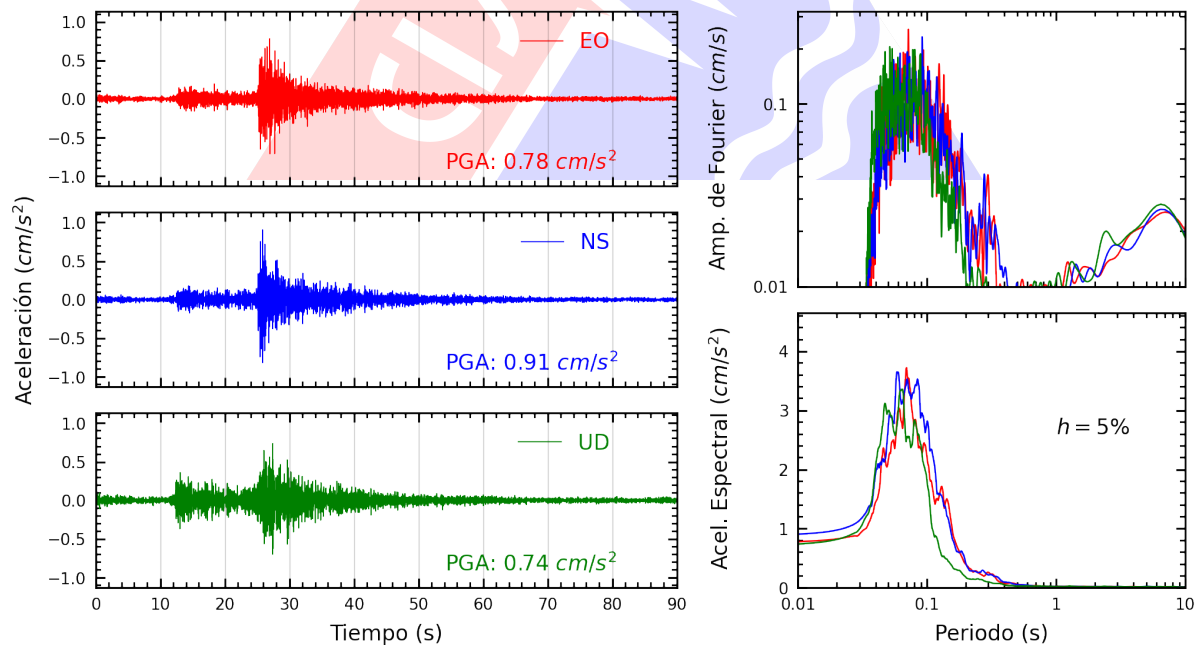
Figura A.12: Registros tiempo-historia, espectros de Fourier y de respuesta en las direcciones EO, NS y vertical de la estación ANCON. Sismo de Chilca, Cañete - Lima del 2023-09-07, 01:53:09 (Hora local)
