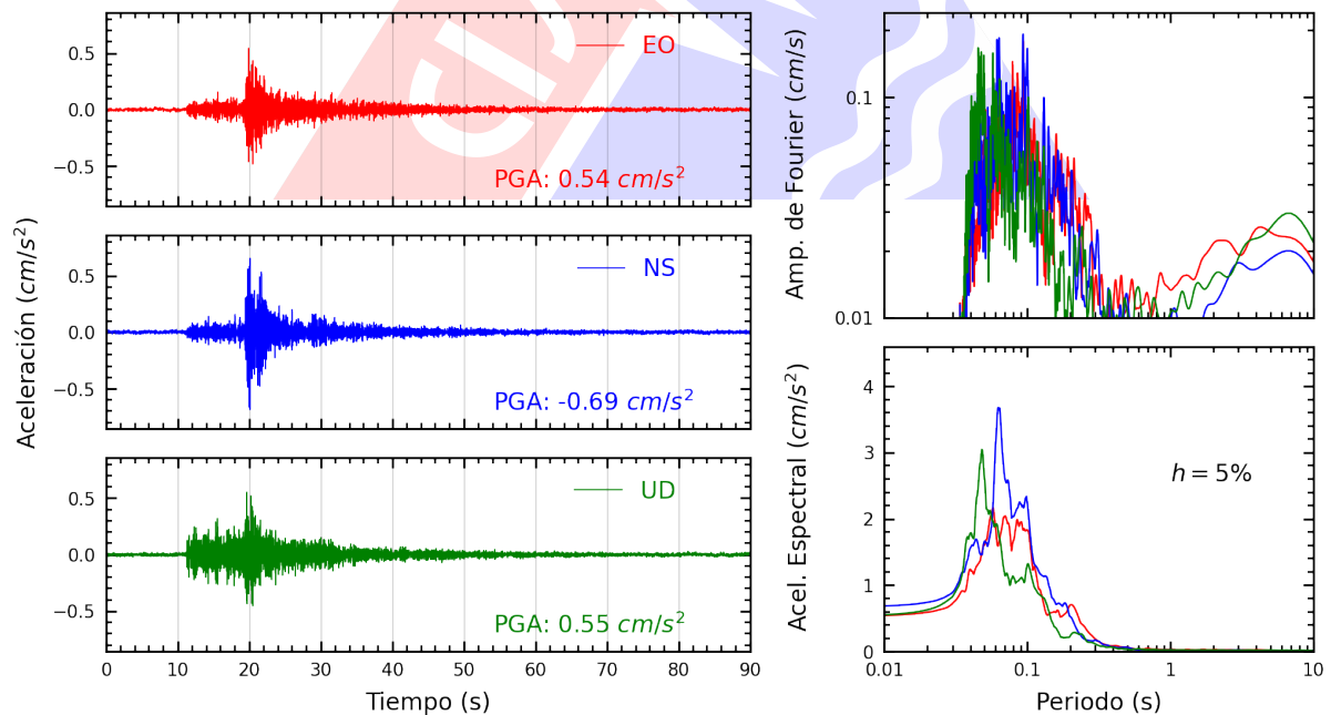
Figura A.18: Registros tiempo-historia, espectros de Fourier y de respuesta en las direcciones EO, NS y vertical de la estación USILP. Sismo de Chilca, Cañete - Lima del 2023-09-07, 01:53:09 (Hora local)
