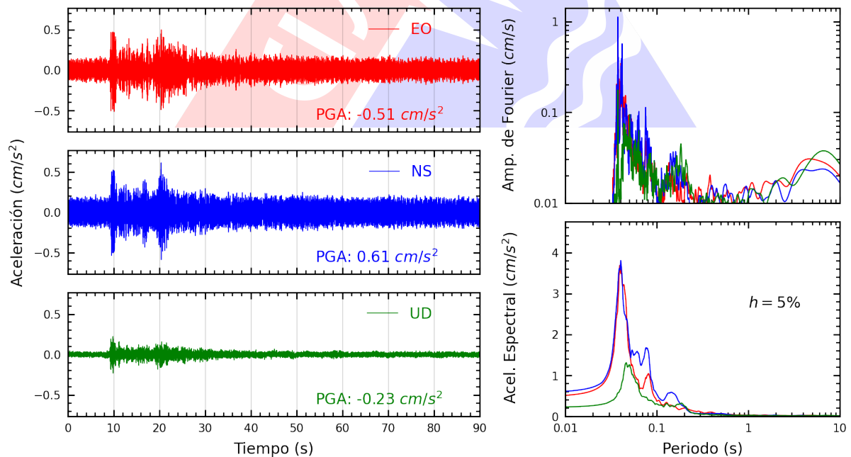
Figura A.20: Registros tiempo-historia, espectros de Fourier y de respuesta en las direcciones EO, NS y vertical de la estación DHNPE. Sismo de Chilca, Cañete - Lima del 2023-09-07, 01:53:09 (Hora local)
