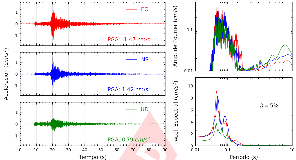
Figura A.5: Registros tiempo-historia, espectros de Fourier y de respuesta en las direcciones EO, NS y vertical de la estación INDEP. Sismo de Chilca, Cañete - Lima del 2023-09-07, 01:53:09 (Hora local)
