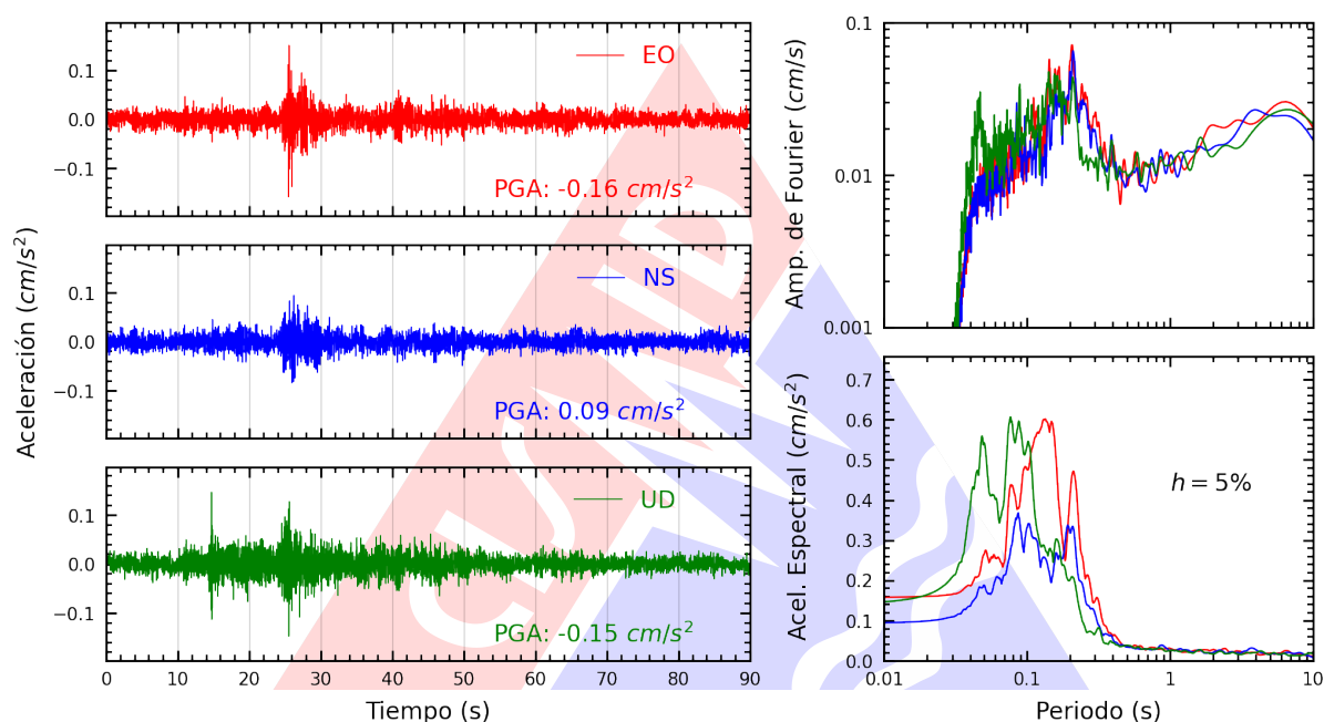
Figura A.35: Registros tiempo-historia, espectros de Fourier y de respuesta en las direcciones EO, NS y vertical de la estación DDMI. Sismo de Chilca, Cañete - Lima del 2023-09-07, 01:53:09 (Hora local)
