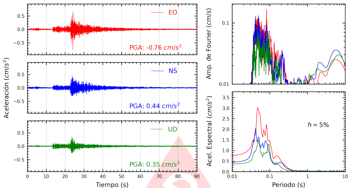
Figura A.15: Registros tiempo-historia, espectros de Fourier y de respuesta en las direcciones EO, NS y vertical de la estación CEPRE. Sismo de Chilca, Cañete - Lima del 2023-09-07, 01:53:09 (Hora local)
