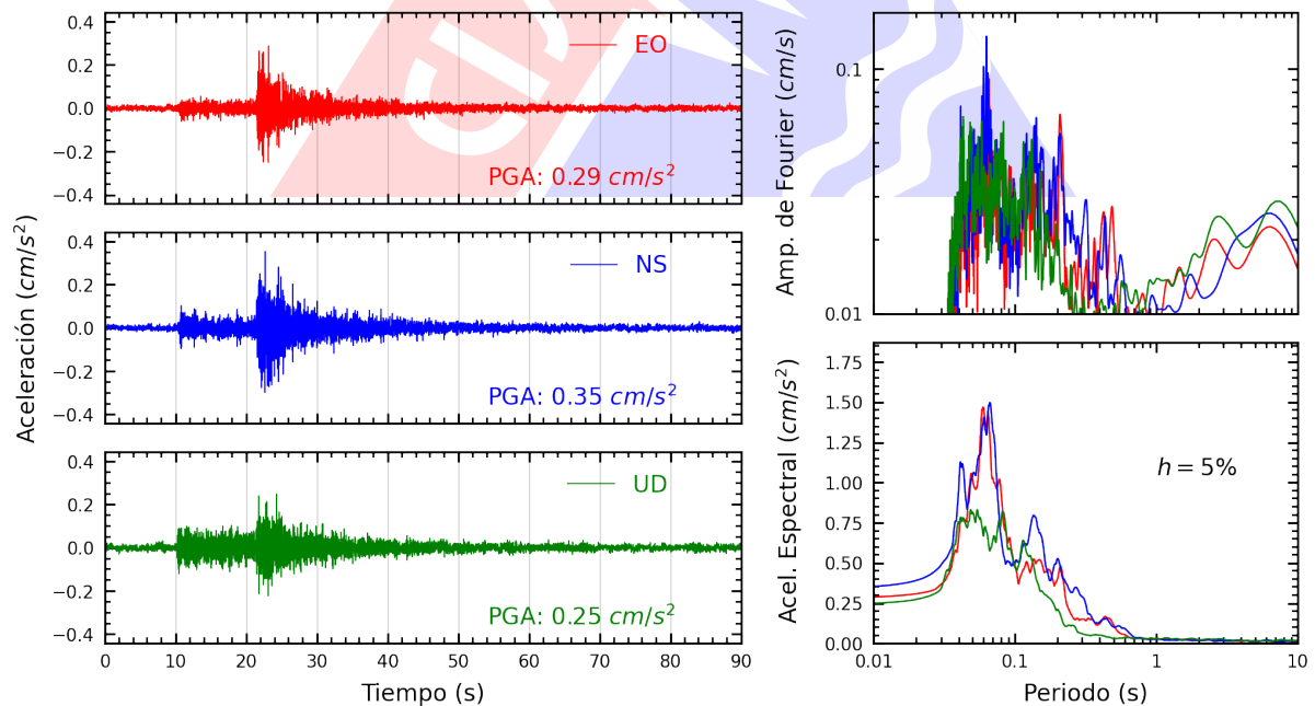
Figura A.28: Registros tiempo-historia, espectros de Fourier y de respuesta en las direcciones EO, NS y vertical de la estación VHAY. Sismo de Chilca, Cañete - Lima del 2023-09-07, 01:53:09 (Hora local)
