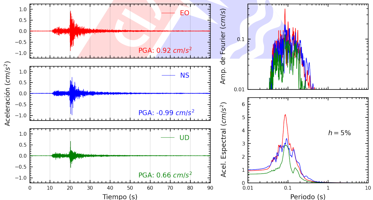
Figura A.10: Registros tiempo-historia, espectros de Fourier y de respuesta en las direcciones EO, NS y vertical de la estación BRISA. Sismo de Chilca, Cañete - Lima del 2023-09-07, 01:53:09 (Hora local)
