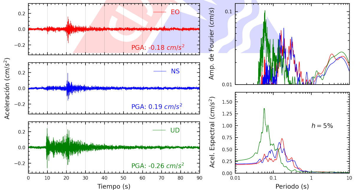
Figura A.32: Registros tiempo-historia, espectros de Fourier y de respuesta en las direcciones EO, NS y vertical de la estación ACAPU. Sismo de Chilca, Cañete - Lima del 2023-09-07, 01:53:09 (Hora local)
