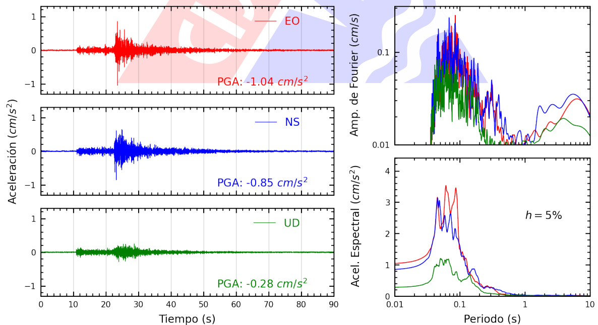
Figura A.8: Registros tiempo-historia, espectros de Fourier y de respuesta en las direcciones EO, NS y vertical de la estación DEFEN. Sismo de Chilca, Cañete - Lima del 2023-09-07, 01:53:09 (Hora local)
