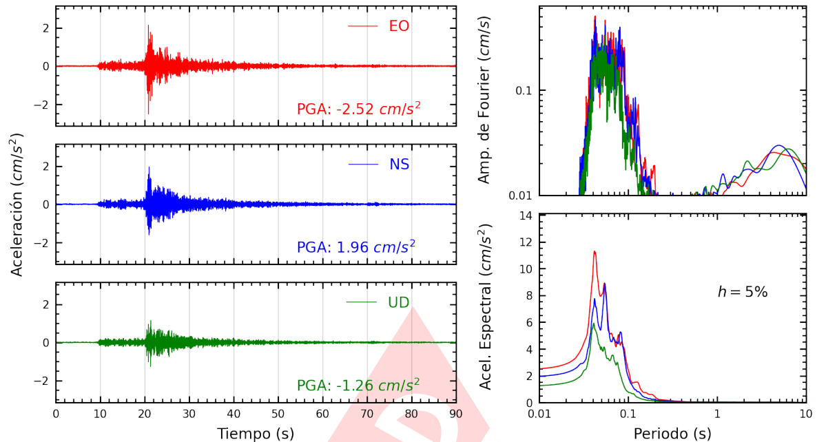
Figura A.3: Registros tiempo-historia, espectros de Fourier y de respuesta en las direcciones EO, NS y vertical de la estación JOSEO. Sismo de Chilca, Cañete - Lima del 2023-09-07, 01:53:09 (Hora local)
