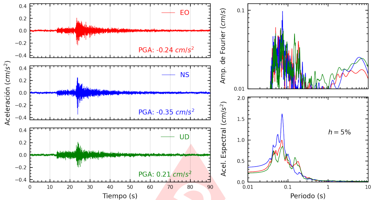
Figura A.29: Registros tiempo-historia, espectros de Fourier y de respuesta en las direcciones EO, NS y vertical de la estación UNFV. Sismo de Chilca, Cañete - Lima del 2023-09-07, 01:53:09 (Hora local)
