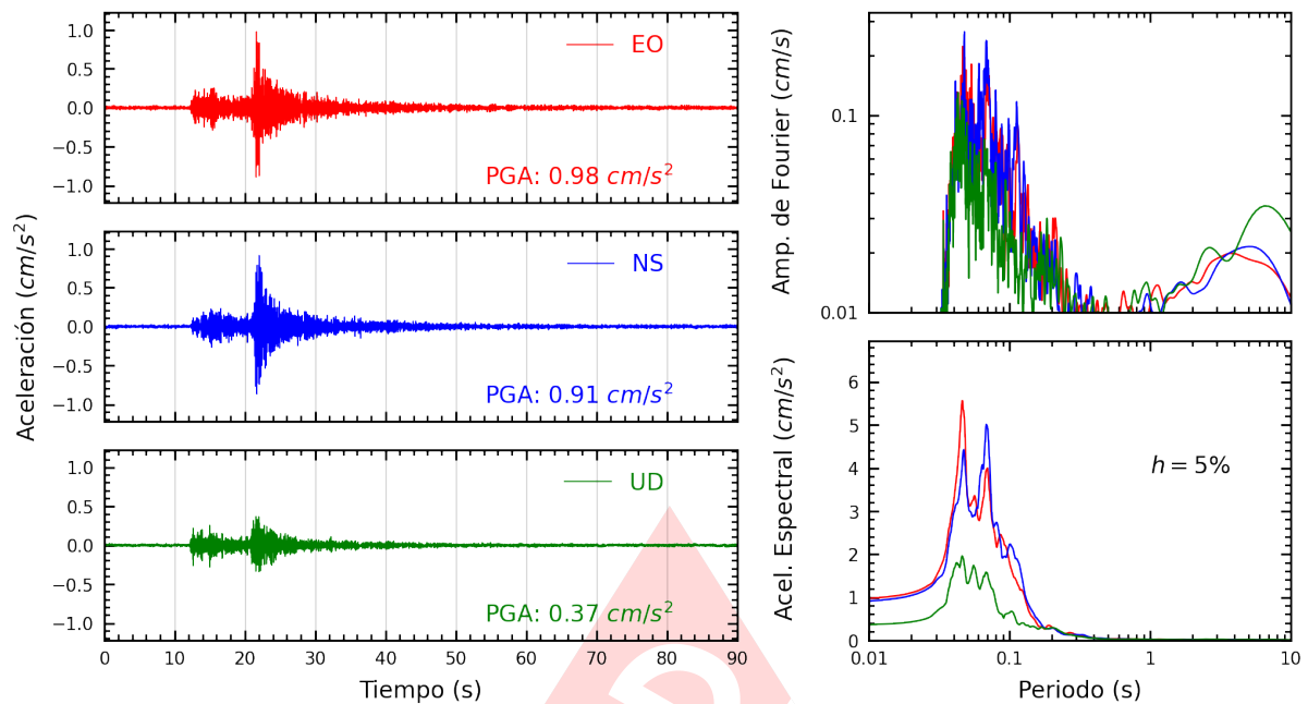
Figura A.11: Registros tiempo-historia, espectros de Fourier y de respuesta en las direcciones EO, NS y vertical de la estación UPCVI. Sismo de Chilca, Cañete - Lima del 2023-09-07, 01:53:09 (Hora local)
