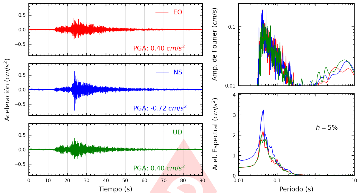
Figura A.17: Registros tiempo-historia, espectros de Fourier y de respuesta en las direcciones EO, NS y vertical de la estación USMP. Sismo de Chilca, Cañete - Lima del 2023-09-07, 01:53:09 (Hora local)
