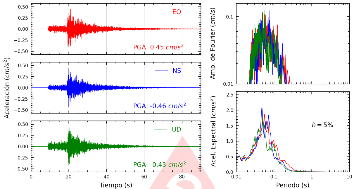
Figura A.23: Registros tiempo-historia, espectros de Fourier y de respuesta en las direcciones EO, NS y vertical de la estación JALV2. Sismo de Chilca, Cañete - Lima del 2023-09-07, 01:53:09 (Hora local)
