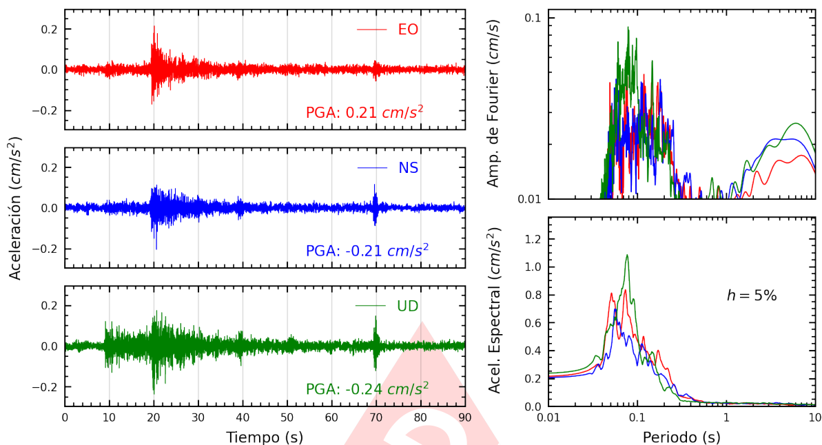
Figura A.33: Registros tiempo-historia, espectros de Fourier y de respuesta en las direcciones EO, NS y vertical de la estación RAMON. Sismo de Chilca, Cañete - Lima del 2023-09-07, 01:53:09 (Hora local)
