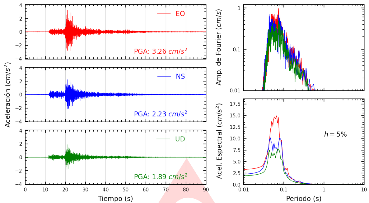
Figura A.1: Registros tiempo-historia, espectros de Fourier y de respuesta en las direcciones EO, NS y vertical de la estación UNTEL. Sismo de Chilca, Cañete - Lima del 2023-09-07, 01:53:09 (Hora local)
