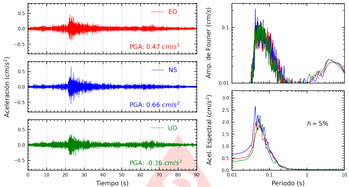
Figura A.19: Registros tiempo-historia, espectros de Fourier y de respuesta en las direcciones EO, NS y vertical de la estación URPPE. Sismo de Chilca, Cañete - Lima del 2023-09-07, 01:53:09 (Hora local)
