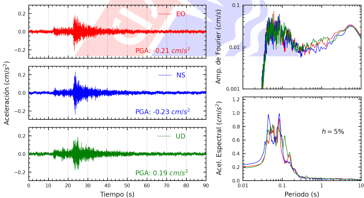
Figura A.34: Registros tiempo-historia, espectros de Fourier y de respuesta en las direcciones EO, NS y vertical de la estación UNMSM. Sismo de Chilca, Cañete - Lima del 2023-09-07, 01:53:09 (Hora local)
