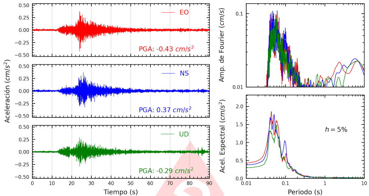
Figura A.25: Registros tiempo-historia, espectros de Fourier y de respuesta en las direcciones EO, NS y vertical de la estación IMCA. Sismo de Chilca, Cañete - Lima del 2023-09-07, 01:53:09 (Hora local)
