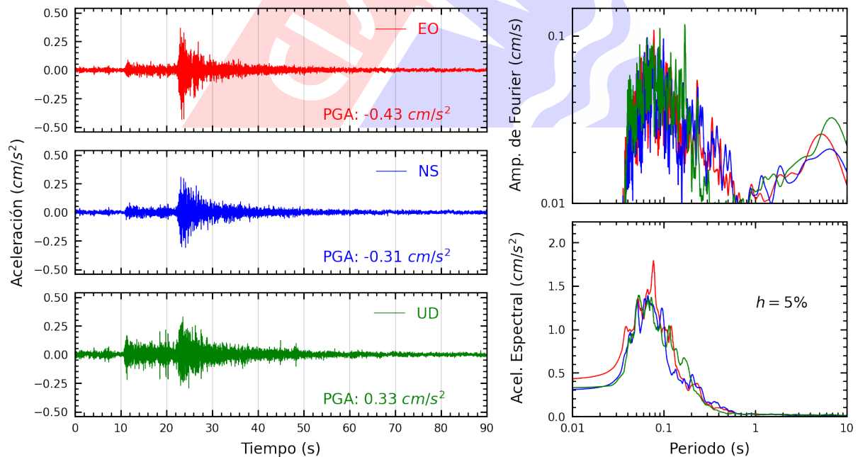
Figura A.24: Registros tiempo-historia, espectros de Fourier y de respuesta en las direcciones EO, NS y vertical de la estación MDPP. Sismo de Chilca, Cañete - Lima del 2023-09-07, 01:53:09 (Hora local)
