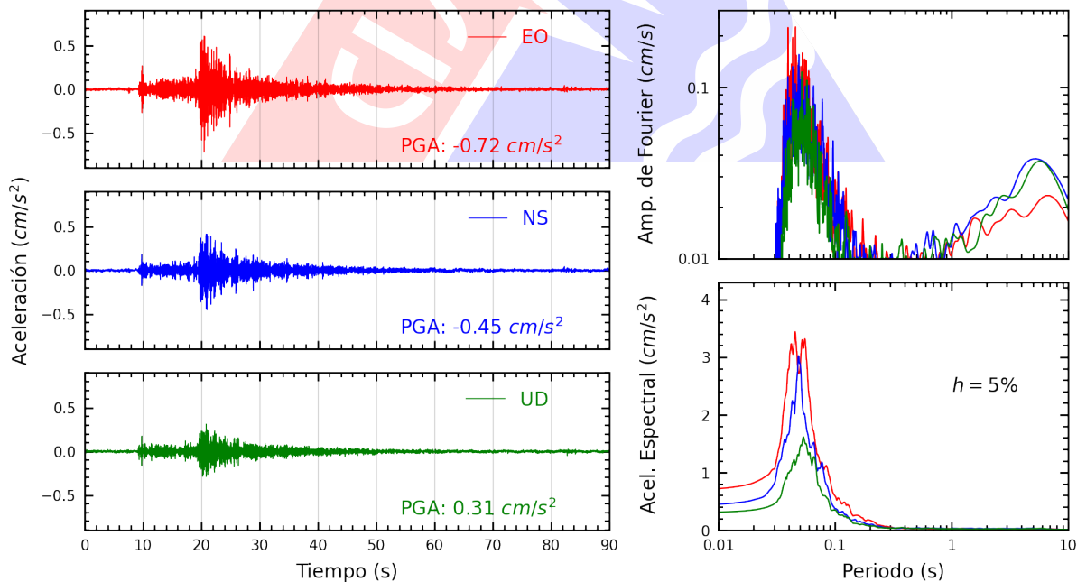
Figura A.16: Registros tiempo-historia, espectros de Fourier y de respuesta en las direcciones EO, NS y vertical de la estación UCSS. Sismo de Chilca, Cañete - Lima del 2023-09-07, 01:53:09 (Hora local)
