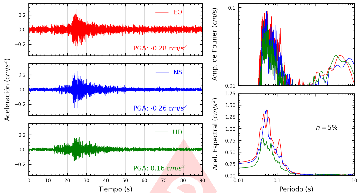
Figura A.31: Registros tiempo-historia, espectros de Fourier y de respuesta en las direcciones EO, NS y vertical de la estación INICT. Sismo de Chilca, Cañete - Lima del 2023-09-07, 01:53:09 (Hora local)
