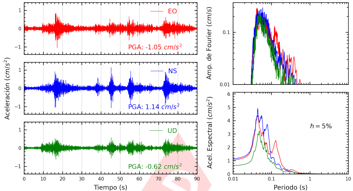
Figura A.5: Registros tiempo-historia, espectros de Fourier y de respuesta en las direcciones EO, NS y vertical de la estación PACHA. Sismo de Chilca, Cañete - Lima del 2023-09-20, 16:44:27 (Hora local)
