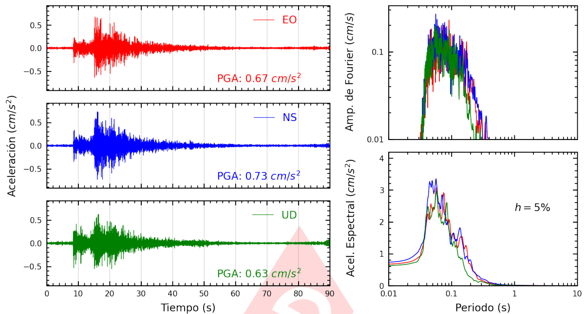
Figura A.11: Registros tiempo-historia, espectros de Fourier y de respuesta en las direcciones EO, NS y vertical de la estación ASIA. Sismo de Chilca, Cañete - Lima del 2023-09-20, 16:44:27 (Hora local)
