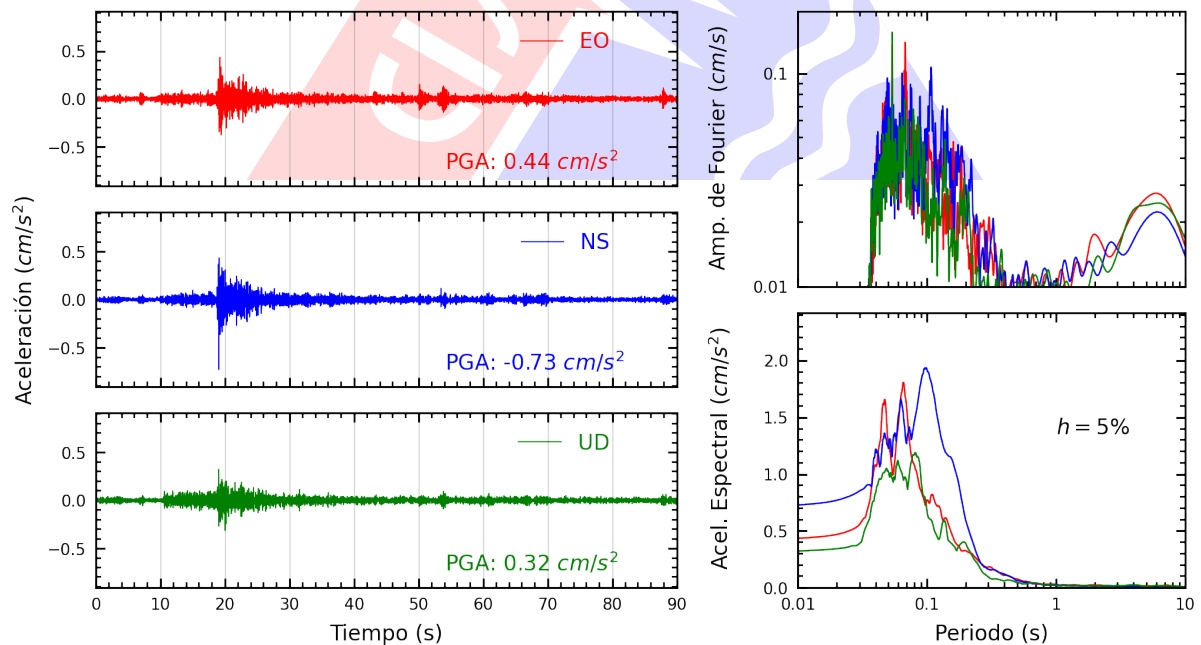
Figura A.12: Registros tiempo-historia, espectros de Fourier y de respuesta en las direcciones EO, NS y vertical de la estación SERVI. Sismo de Chilca, Cañete - Lima del 2023-09-20, 16:44:27 (Hora local)
