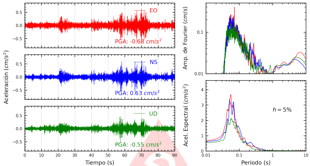
Figura A.13: Registros tiempo-historia, espectros de Fourier y de respuesta en las direcciones EO, NS y vertical de la estación UPCS. Sismo de Chilca, Cañete - Lima del 2023-09-20, 16:44:27 (Hora local)
