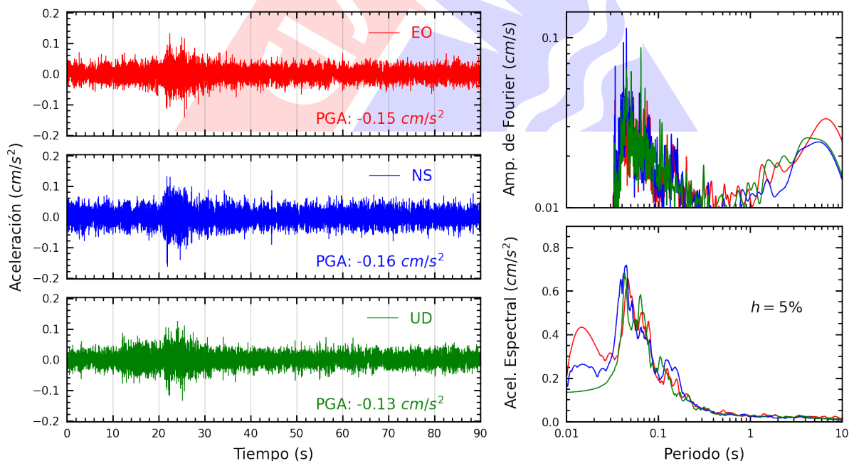
Figura A.30: Registros tiempo-historia, espectros de Fourier y de respuesta en las direcciones EO, NS y vertical de la estación BONDY. Sismo de Chilca, Cañete - Lima del 2023-09-20, 16:44:27 (Hora local)
