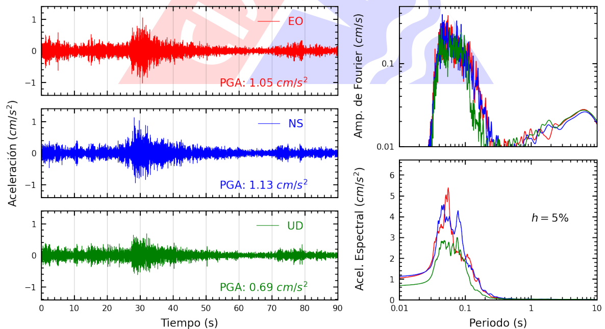
Figura A.6: Registros tiempo-historia, espectros de Fourier y de respuesta en las direcciones EO, NS y vertical de la estación SROSA. Sismo de Chilca, Cañete - Lima del 2023-09-20, 16:44:27 (Hora local)
