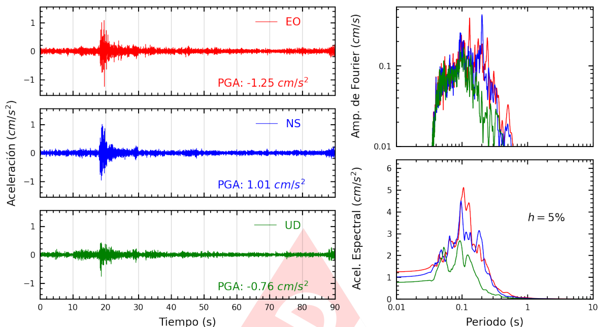
Figura A.3: Registros tiempo-historia, espectros de Fourier y de respuesta en las direcciones EO, NS y vertical de la estación SCCHO. Sismo de Chilca, Cañete - Lima del 2023-09-20, 16:44:27 (Hora local)
