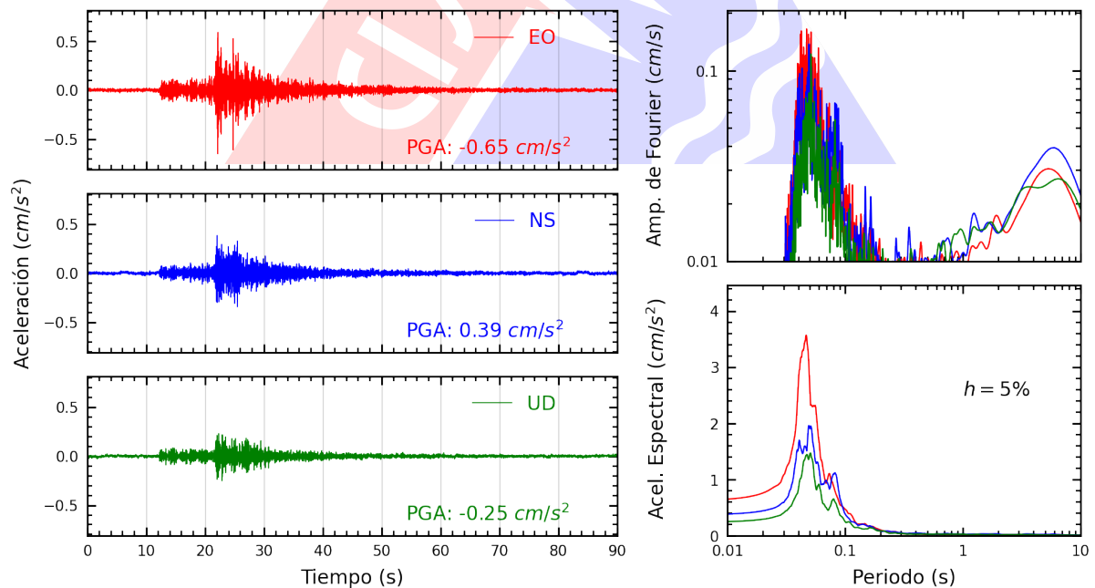
Figura A.14: Registros tiempo-historia, espectros de Fourier y de respuesta en las direcciones EO, NS y vertical de la estación UCSS. Sismo de Chilca, Cañete - Lima del 2023-09-20, 16:44:27 (Hora local)
