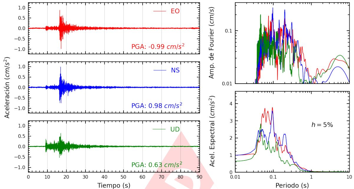
Figura A.7: Registros tiempo-historia, espectros de Fourier y de respuesta en las direcciones EO, NS y vertical de la estación USILP. Sismo de Chilca, Cañete - Lima del 2023-09-20, 16:44:27 (Hora local)
