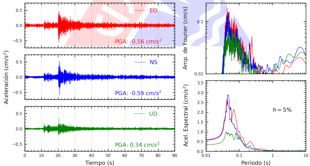
Figura A.16: Registros tiempo-historia, espectros de Fourier y de respuesta en las direcciones EO, NS y vertical de la estación CEPRE. Sismo de Chilca, Cañete - Lima del 2023-09-20, 16:44:27 (Hora local)
