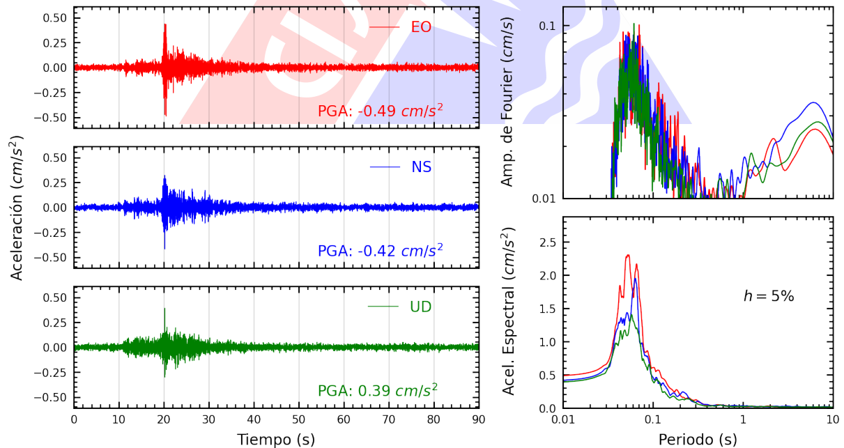
Figura A.18: Registros tiempo-historia, espectros de Fourier y de respuesta en las direcciones EO, NS y vertical de la estación CENEP. Sismo de Chilca, Cañete - Lima del 2023-09-20, 16:44:27 (Hora local)
