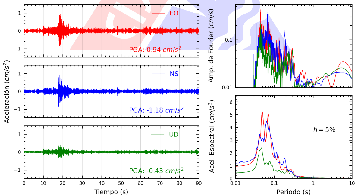
Figura A.4: Registros tiempo-historia, espectros de Fourier y de respuesta en las direcciones EO, NS y vertical de la estación UPCVI. Sismo de Chilca, Cañete - Lima del 2023-09-20, 16:44:27 (Hora local)
