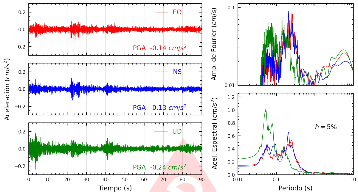
Figura A.27: Registros tiempo-historia, espectros de Fourier y de respuesta en las direcciones EO, NS y vertical de la estación DSMI. Sismo de Chilca, Cañete - Lima del 2023-09-20, 16:44:27 (Hora local)
