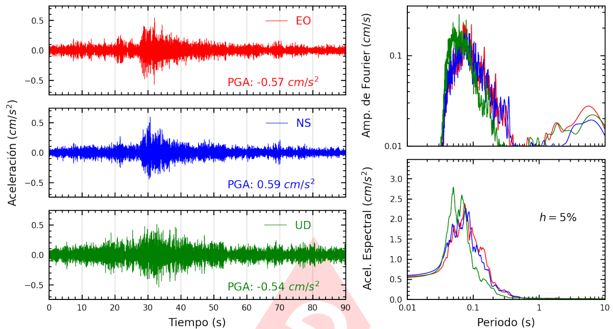
Figura A.15: Registros tiempo-historia, espectros de Fourier y de respuesta en las direcciones EO, NS y vertical de la estación ANCON. Sismo de Chilca, Cañete - Lima del 2023-09-20, 16:44:27 (Hora local)
