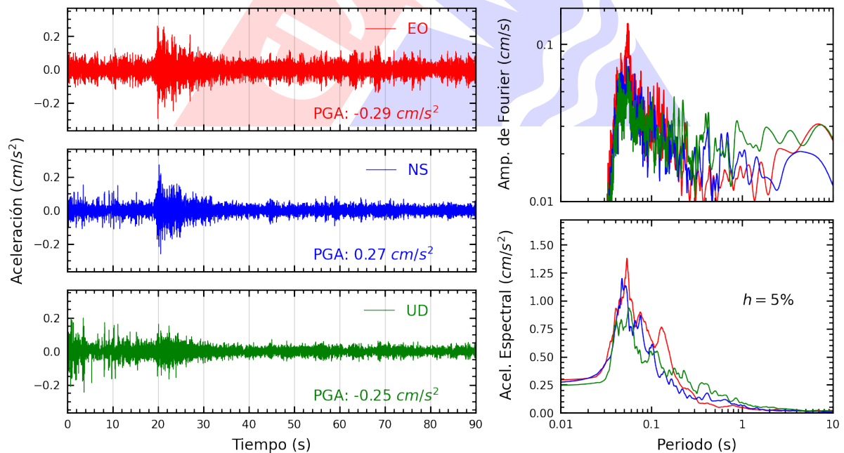
Figura A.26: Registros tiempo-historia, espectros de Fourier y de respuesta en las direcciones EO, NS y vertical de la estación INICT. Sismo de Chilca, Cañete - Lima del 2023-09-20, 16:44:27 (Hora local)
