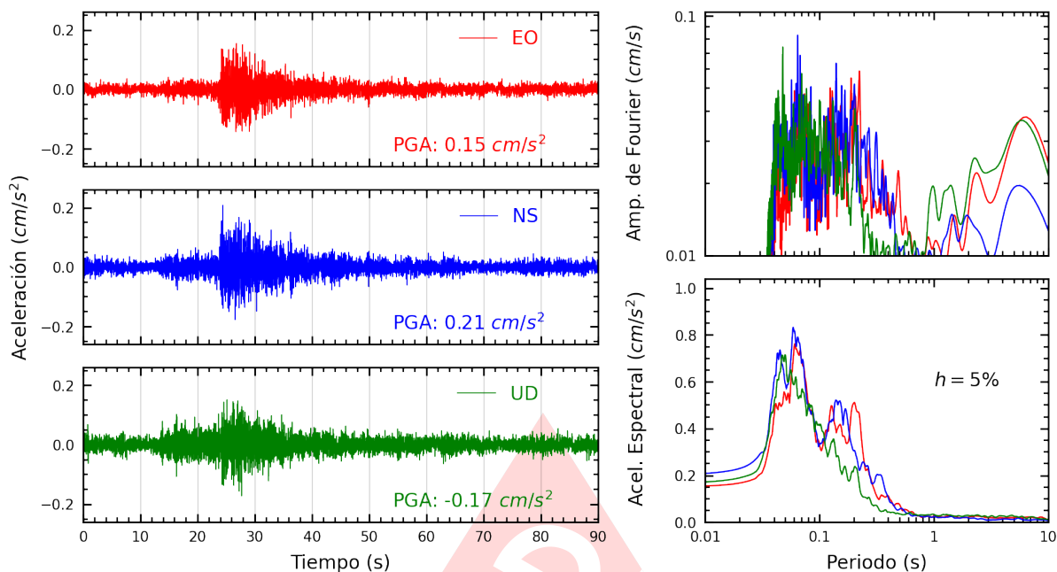
Figura A.29: Registros tiempo-historia, espectros de Fourier y de respuesta en las direcciones EO, NS y vertical de la estación VHAYA. Sismo de Chilca, Cañete - Lima del 2023-09-20, 16:44:27 (Hora local)
