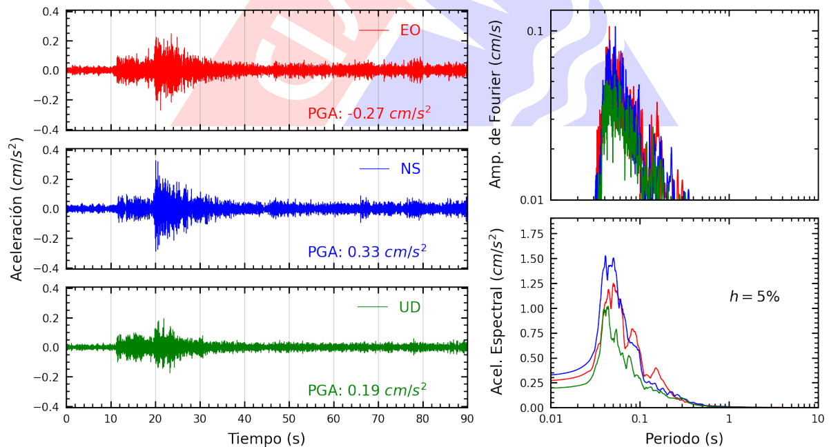
Figura A.22: Registros tiempo-historia, espectros de Fourier y de respuesta en las direcciones EO, NS y vertical de la estación BORJA. Sismo de Chilca, Cañete - Lima del 2023-09-20, 16:44:27 (Hora local)
