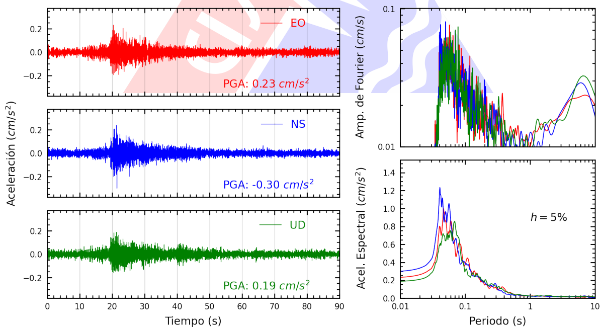
Figura A.24: Registros tiempo-historia, espectros de Fourier y de respuesta en las direcciones EO, NS y vertical de la estación IMCA. Sismo de Chilca, Cañete - Lima del 2023-09-20, 16:44:27 (Hora local)
