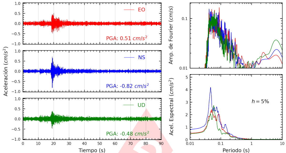
Figura A.9: Registros tiempo-historia, espectros de Fourier y de respuesta en las direcciones EO, NS y vertical de la estación URPE. Sismo de Chilca, Cañete - Lima del 2023-09-20, 16:44:27 (Hora local)
