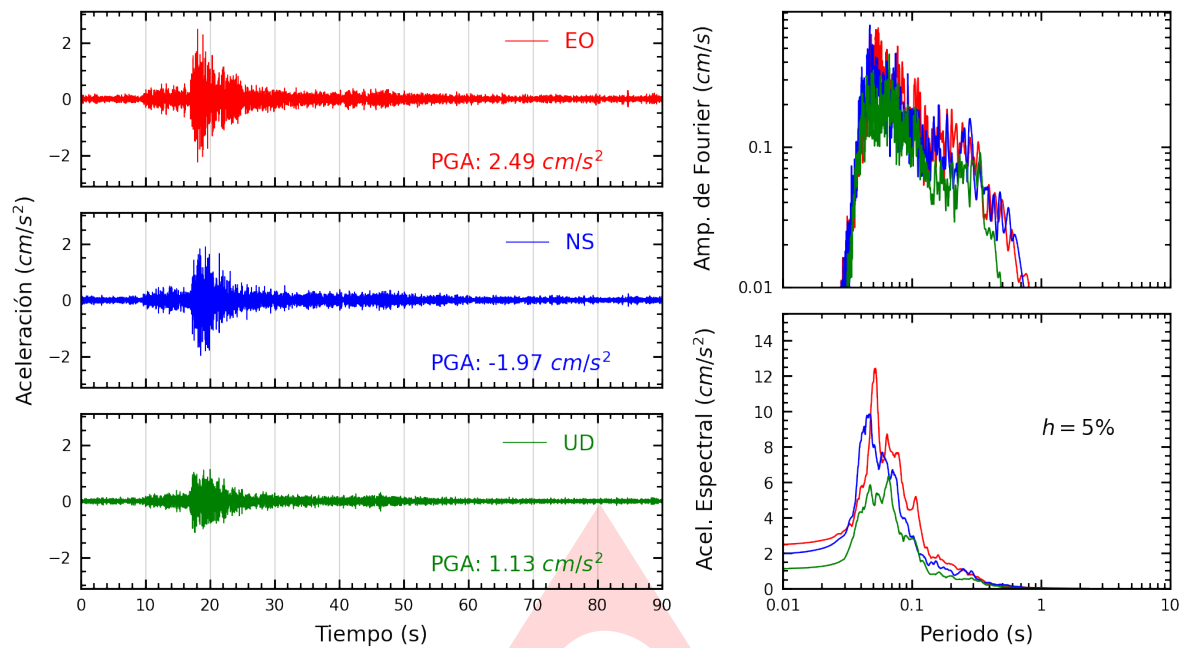
Figura A.1: Registros tiempo-historia, espectros de Fourier y de respuesta en las direcciones EO, NS y vertical de la estación UNTEL. Sismo de Chilca, Cañete - Lima del 2023-09-20, 16:44:27 (Hora local)
