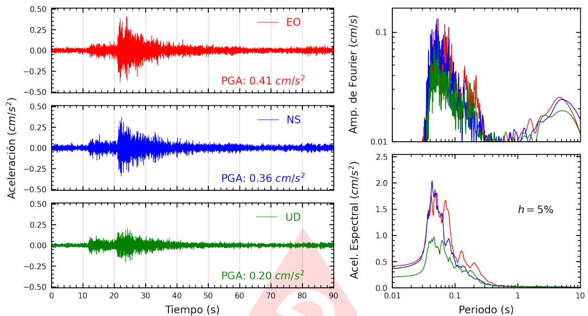
Figura A.21: Registros tiempo-historia, espectros de Fourier y de respuesta en las direcciones EO, NS y vertical de la estación FICPE. Sismo de Chilca, Cañete - Lima del 2023-09-20, 16:44:27 (Hora local)
