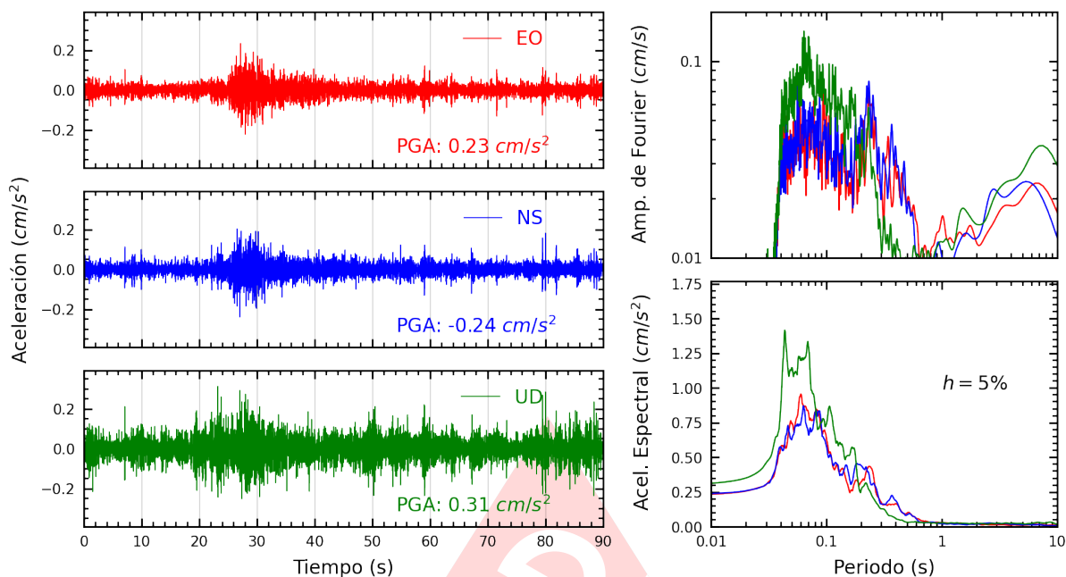
Figura A.23: Registros tiempo-historia, espectros de Fourier y de respuesta en las direcciones EO, NS y vertical de la estación MDPP. Sismo de Chilca, Cañete - Lima del 2023-09-20, 16:44:27 (Hora local)
