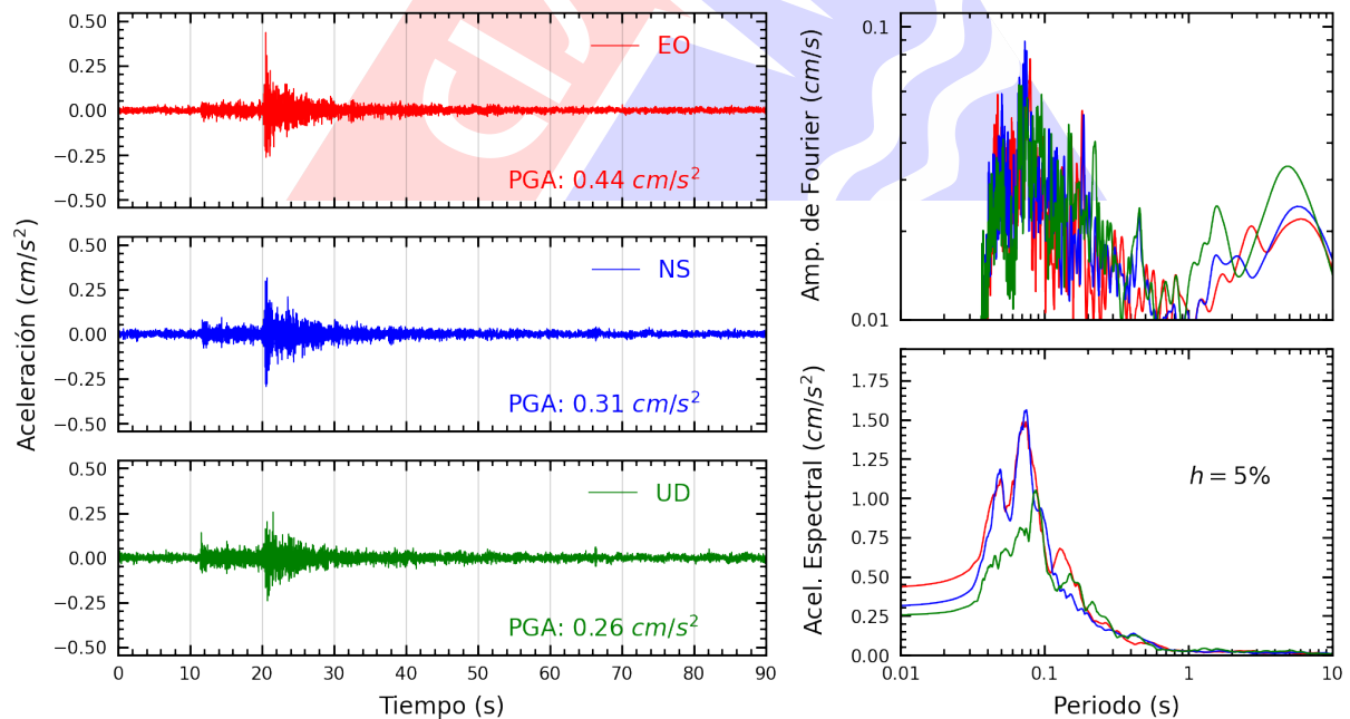
Figura A.20: Registros tiempo-historia, espectros de Fourier y de respuesta en las direcciones EO, NS y vertical de la estación UNFV. Sismo de Chilca, Cañete - Lima del 2023-09-20, 16:44:27 (Hora local)
