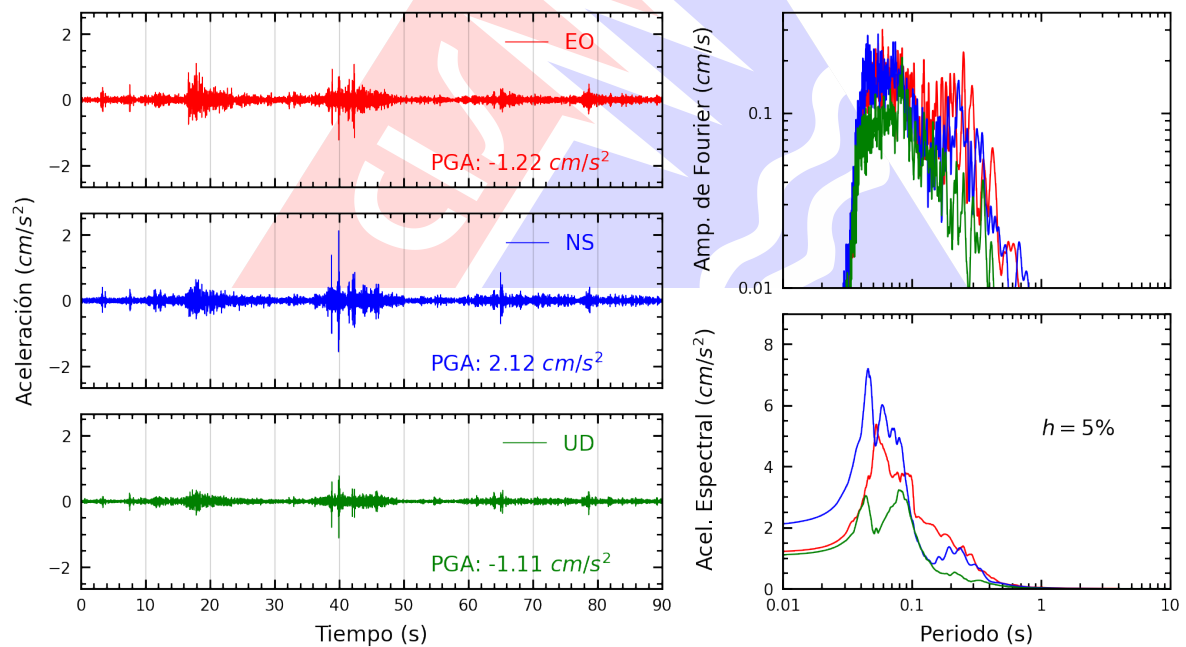
Figura A.2: Registros tiempo-historia, espectros de Fourier y de respuesta en las direcciones EO, NS y vertical de la estación BRISA. Sismo de Chilca, Cañete - Lima del 2023-09-20, 16:44:27 (Hora local)
