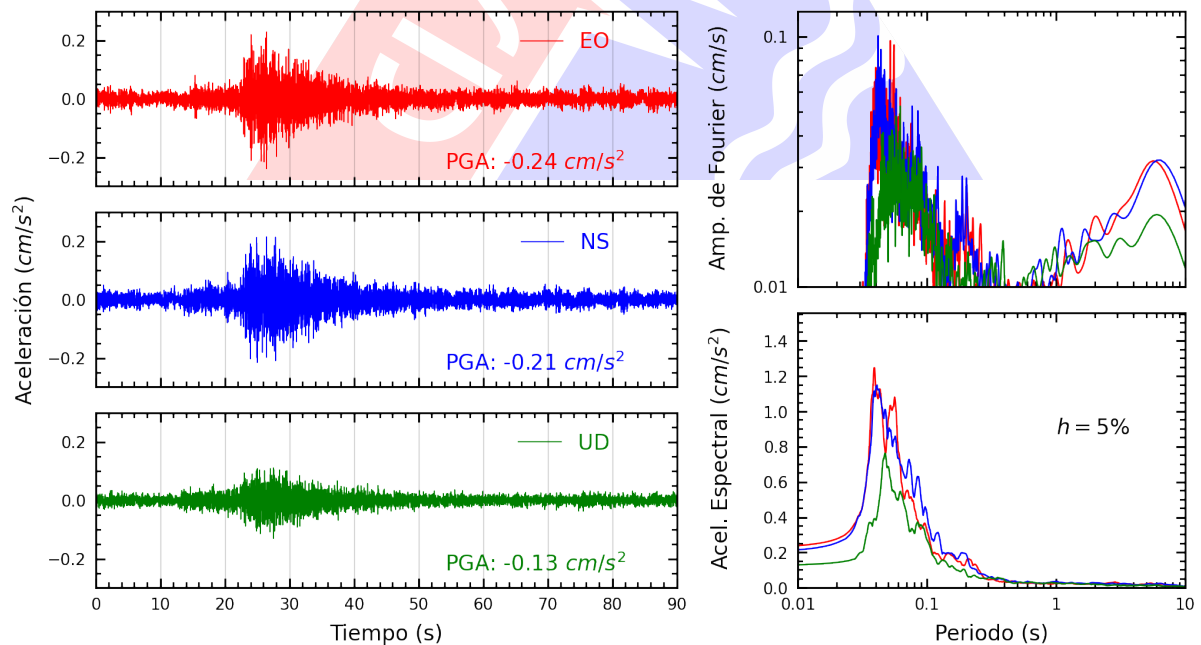
Figura A.28: Registros tiempo-historia, espectros de Fourier y de respuesta en las direcciones EO, NS y vertical de la estación COMAS. Sismo de Chilca, Cañete - Lima del 2023-09-20, 16:44:27 (Hora local)
