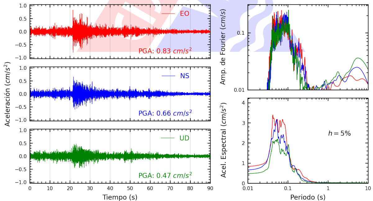
Figura A.8: Registros tiempo-historia, espectros de Fourier y de respuesta en las direcciones EO, NS y vertical de la estación INDEP. Sismo de Chilca, Cañete - Lima del 2023-09-20, 16:44:27 (Hora local)
