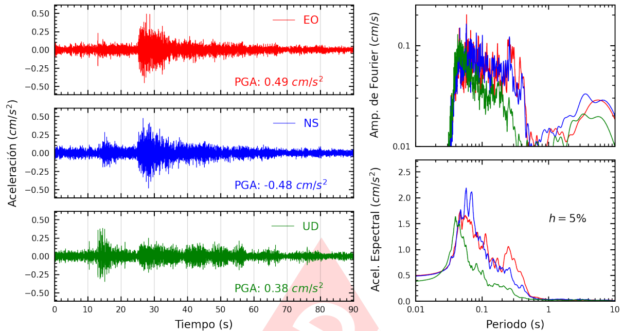
Figura A.17: Registros tiempo-historia, espectros de Fourier y de respuesta en las direcciones EO, NS y vertical de la estación DEFEN. Sismo de Chilca, Cañete - Lima del 2023-09-20, 16:44:27 (Hora local)
