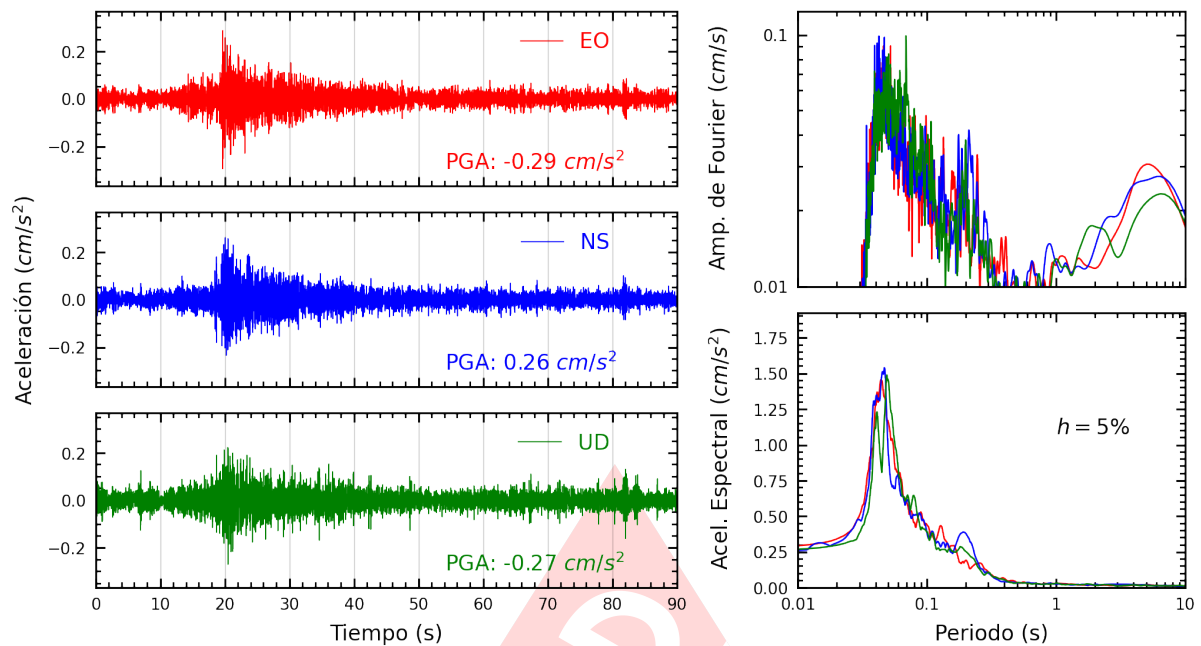
Figura A.25: Registros tiempo-historia, espectros de Fourier y de respuesta en las direcciones EO, NS y vertical de la estación USMP. Sismo de Chilca, Cañete - Lima del 2023-09-20, 16:44:27 (Hora local)
