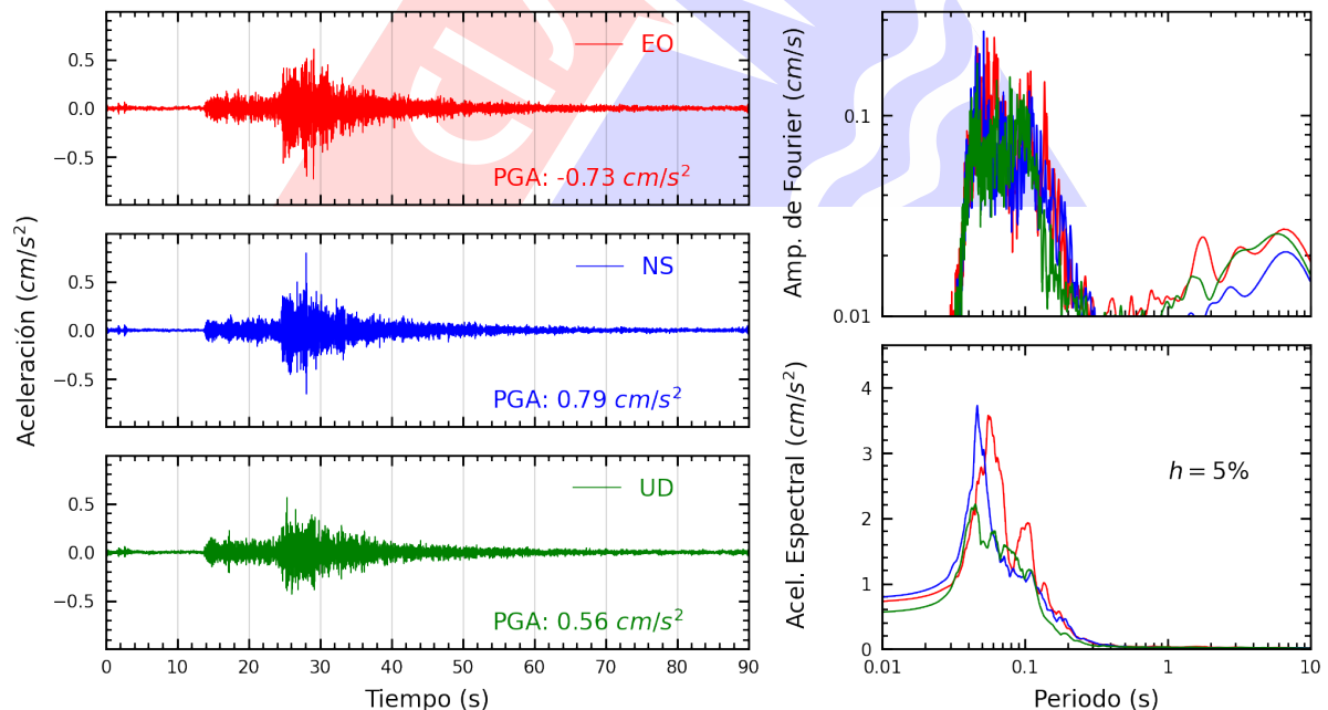
Figura A.10: Registros tiempo-historia, espectros de Fourier y de respuesta en las direcciones EO, NS y vertical de la estación AMORE. Sismo de Chilca, Cañete - Lima del 2023-09-20, 16:44:27 (Hora local)
