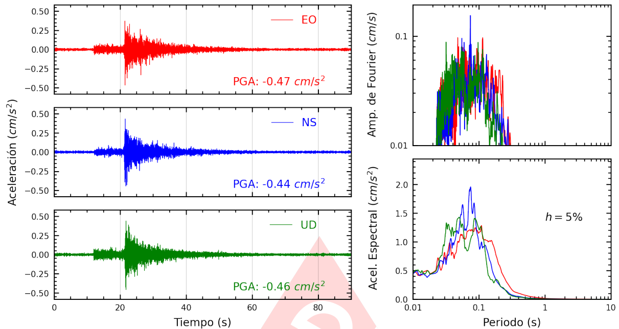
Figura A.19: Registros tiempo-historia, espectros de Fourier y de respuesta en las direcciones EO, NS y vertical de la estación JALV2. Sismo de Chilca, Cañete - Lima del 2023-09-20, 16:44:27 (Hora local)
