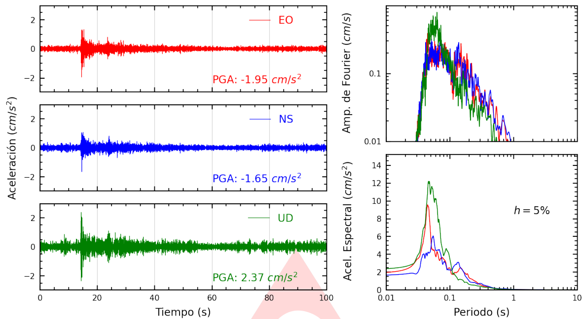
Figura A.1: Registros tiempo-historia, espectros de Fourier y de respuesta en las direcciones EO, NS y vertical de la estación SCAR2. Sismo de La Capilla, General Sanchez Cerro - Moquegua del 2023-09-21, 13:28:10 (Hora local)
