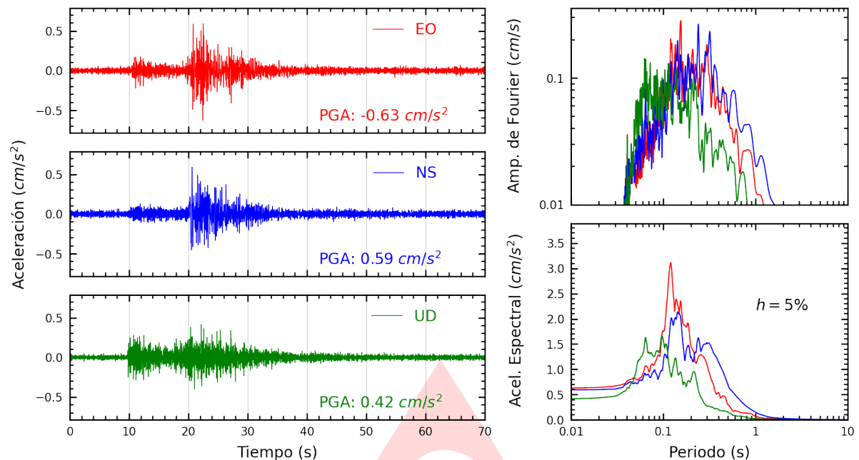
Figura A.1: Registros tiempo-historia, espectros de Fourier y de respuesta en las direcciones EO, NS y vertical de la estación UNAAA. Sismo de Moyobamba, Moyobamba - San Martín del 2023-09-21, 15:55:59 (Hora local)
