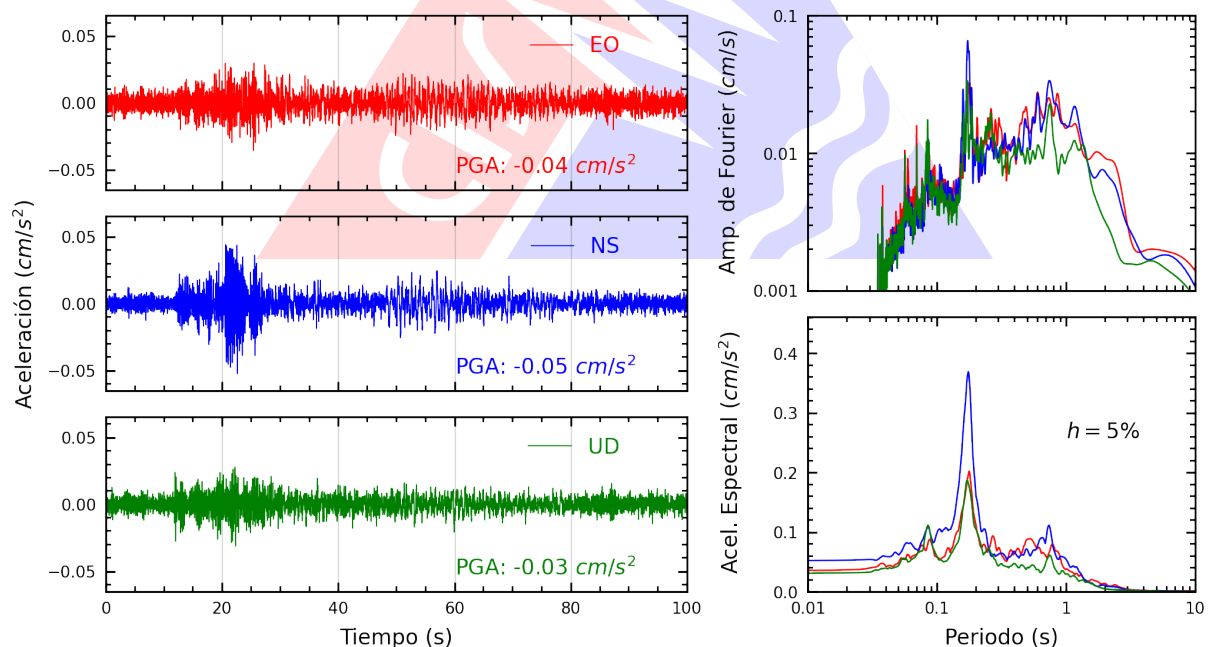
Figura A.2: Registros tiempo-historia, espectros de Fourier y de respuesta en las direcciones EO, NS y vertical de la estación UNC. Sismo de Moyobamba, Moyobamba - San Martín del 2023-09-21, 15:55:59 (Hora local)
