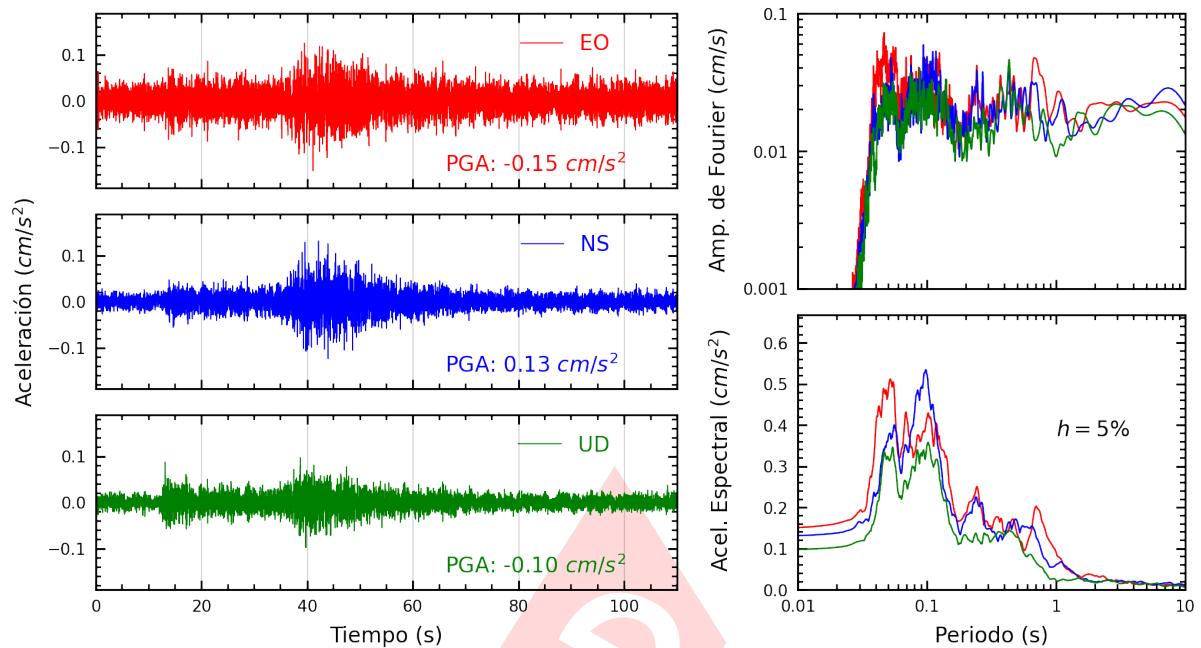
Figura A.27: Registros tiempo-historia, espectros de Fourier y de respuesta en las direcciones EO, NS y vertical de la estación INICT. Sismo de Huancavelica, Huancavelica - Huancavelica del 2023-10-03, 02:40:16 (Hora local)
