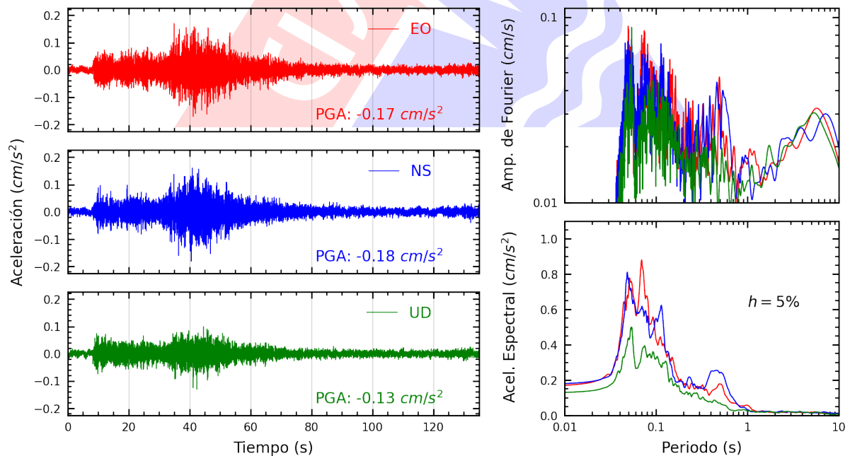
Figura A.22: Registros tiempo-historia, espectros de Fourier y de respuesta en las direcciones EO, NS y vertical de la estación FICPE. Sismo de Huancavelica, Huancavelica - Huancavelica del 2023-10-03, 02:40:16 (Hora local)
