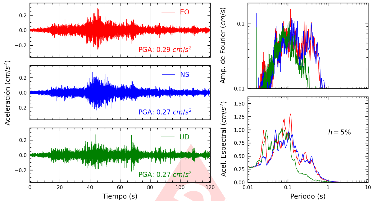
Figura A.11: Registros tiempo-historia, espectros de Fourier y de respuesta en las direcciones EO, NS y vertical de la estación SCOLI. Sismo de Huancavelica, Huancavelica - Huancavelica del 2023-10-03, 02:40:16 (Hora local)
