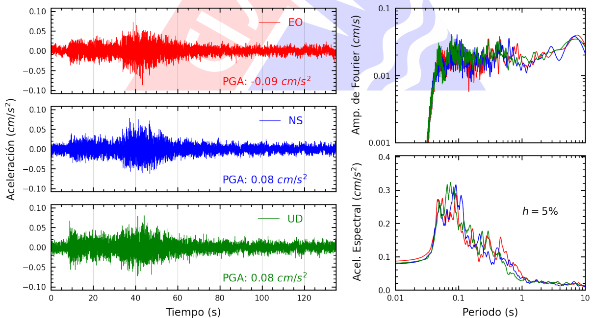
Figura A.34: Registros tiempo-historia, espectros de Fourier y de respuesta en las direcciones EO, NS y vertical de la estación UNFV. Sismo de Huancavelica, Huancavelica - Huancavelica del 2023-10-03, 02:40:16 (Hora local)
