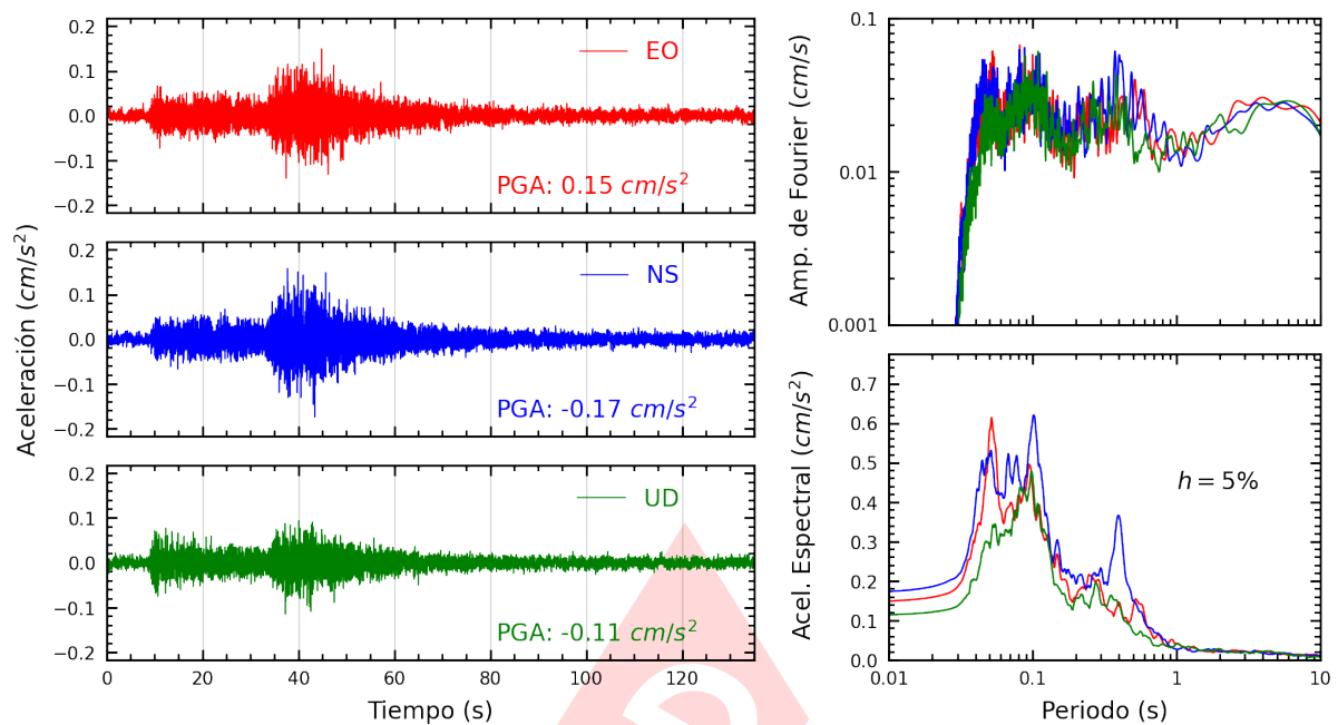
Figura A.25: Registros tiempo-historia, espectros de Fourier y de respuesta en las direcciones EO, NS y vertical de la estación COMAS. Sismo de Huancavelica, Huancavelica - Huancavelica del 2023-10-03, 02:40:16 (Hora local)
