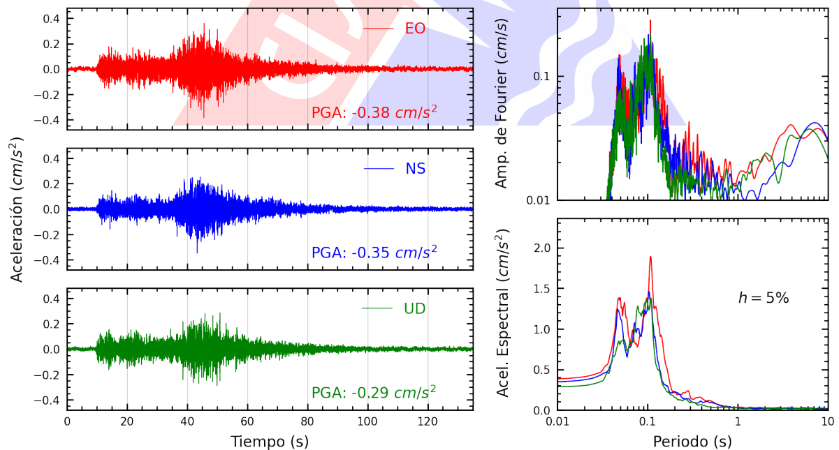
Figura A.6: Registros tiempo-historia, espectros de Fourier y de respuesta en las direcciones EO, NS y vertical de la estación AMORE. Sismo de Huancavelica, Huancavelica - Huancavelica del 2023-10-03, 02:40:16 (Hora local)
