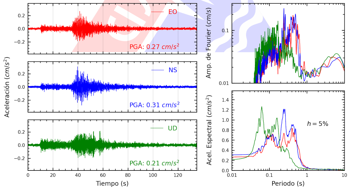
Figura A.10: Registros tiempo-historia, espectros de Fourier y de respuesta en las direcciones EO, NS y vertical de la estación MDPP. Sismo de Huancavelica, Huancavelica - Huancavelica del 2023-10-03, 02:40:16 (Hora local)
