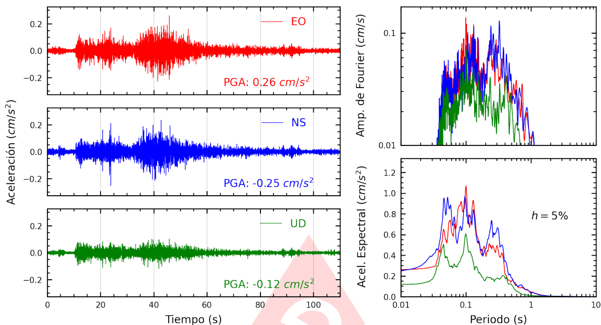
Figura A.13: Registros tiempo-historia, espectros de Fourier y de respuesta en las direcciones EO, NS y vertical de la estación BRISA. Sismo de Huancavelica, Huancavelica - Huancavelica del 2023-10-03, 02:40:16 (Hora local)
