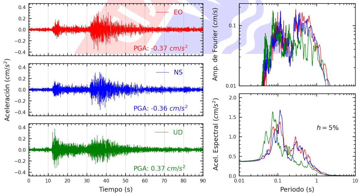
Figura A.8: Registros tiempo-historia, espectros de Fourier y de respuesta en las direcciones EO, NS y vertical de la estación UNICA. Sismo de Huancavelica, Huancavelica - Huancavelica del 2023-10-03, 02:40:16 (Hora local)
