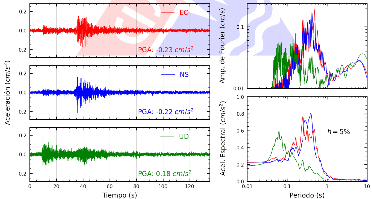
Figura A.16: Registros tiempo-historia, espectros de Fourier y de respuesta en las direcciones EO, NS y vertical de la estación ACAPU. Sismo de Huancavelica, Huancavelica - Huancavelica del 2023-10-03, 02:40:16 (Hora local)
