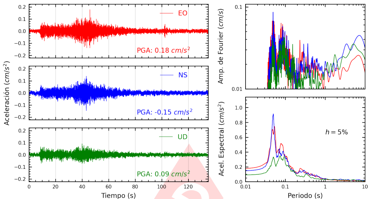
Figura A.23: Registros tiempo-historia, espectros de Fourier y de respuesta en las direcciones EO, NS y vertical de la estación CEPRE. Sismo de Huancavelica, Huancavelica - Huancavelica del 2023-10-03, 02:40:16 (Hora local)
