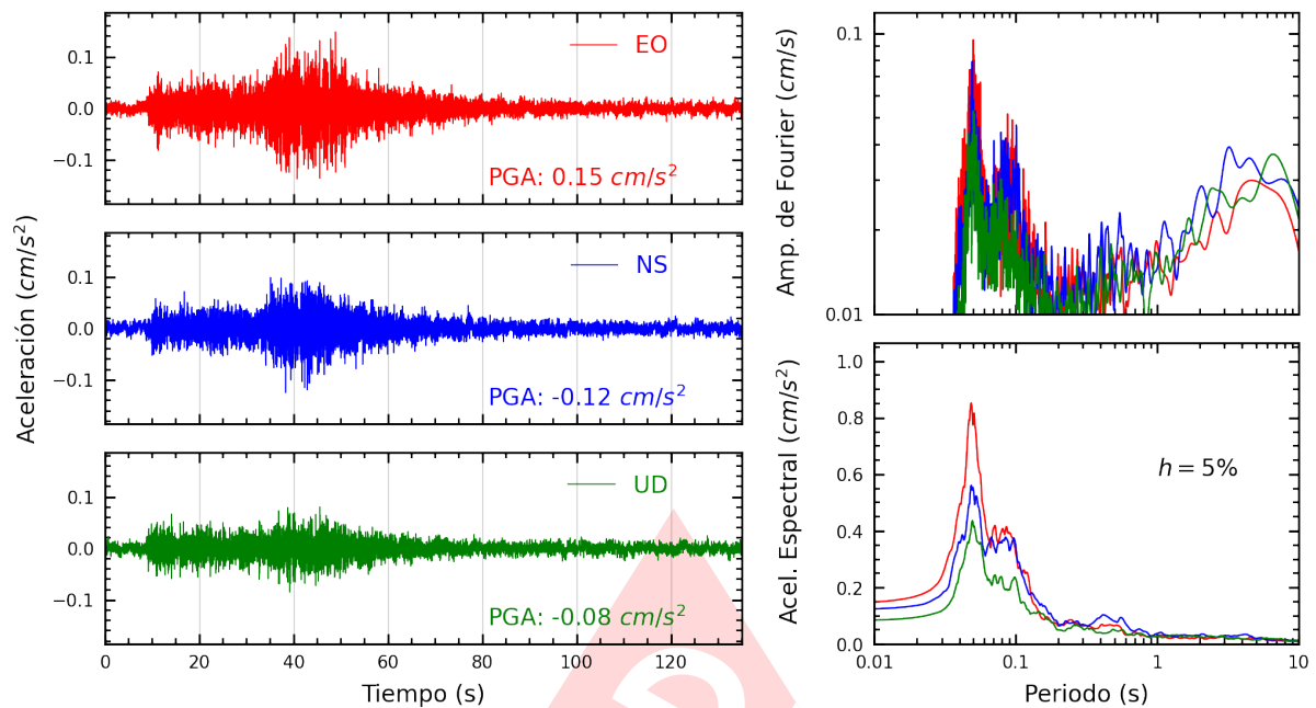
Figura A.29: Registros tiempo-historia, espectros de Fourier y de respuesta en las direcciones EO, NS y vertical de la estación UCSS. Sismo de Huancavelica, Huancavelica - Huancavelica del 2023-10-03, 02:40:16 (Hora local)
