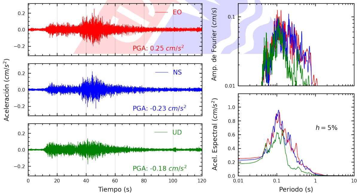
Figura A.14: Registros tiempo-historia, espectros de Fourier y de respuesta en las direcciones EO, NS y vertical de la estación SCCHO. Sismo de Huancavelica, Huancavelica - Huancavelica del 2023-10-03, 02:40:16 (Hora local)
