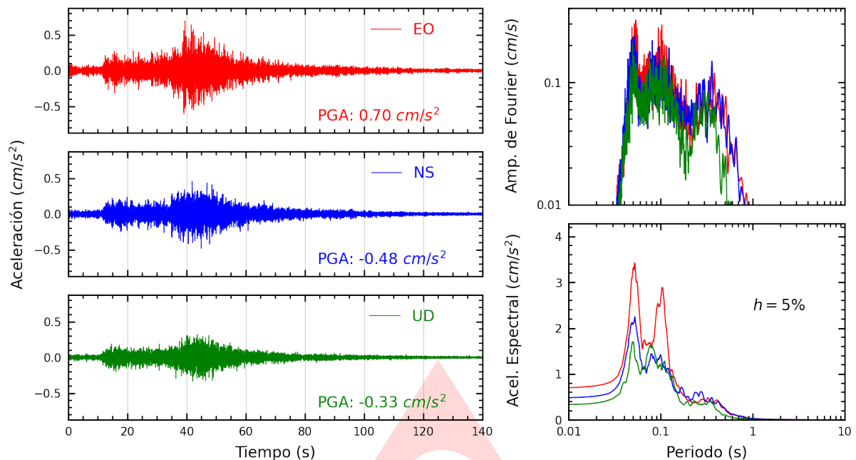
Figura A.1: Registros tiempo-historia, espectros de Fourier y de respuesta en las direcciones EO, NS y vertical de la estación UNTEL. Sismo de Huancavelica, Huancavelica - Huancavelica del 2023-10-03, 02:40:16 (Hora local)
