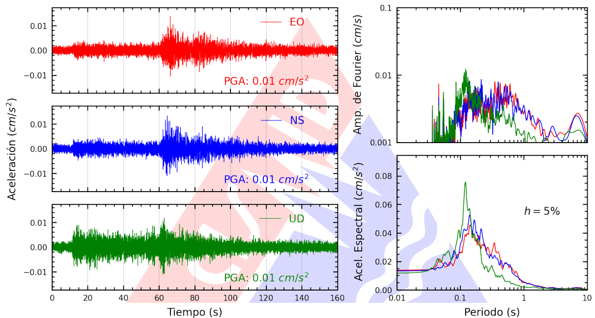
Figura A.35: Registros tiempo-historia, espectros de Fourier y de respuesta en las direcciones EO, NS y vertical de la estación UNIA. Sismo de Huancavelica, Huancavelica - Huancavelica del 2023-10-03, 02:40:16 (Hora local)
