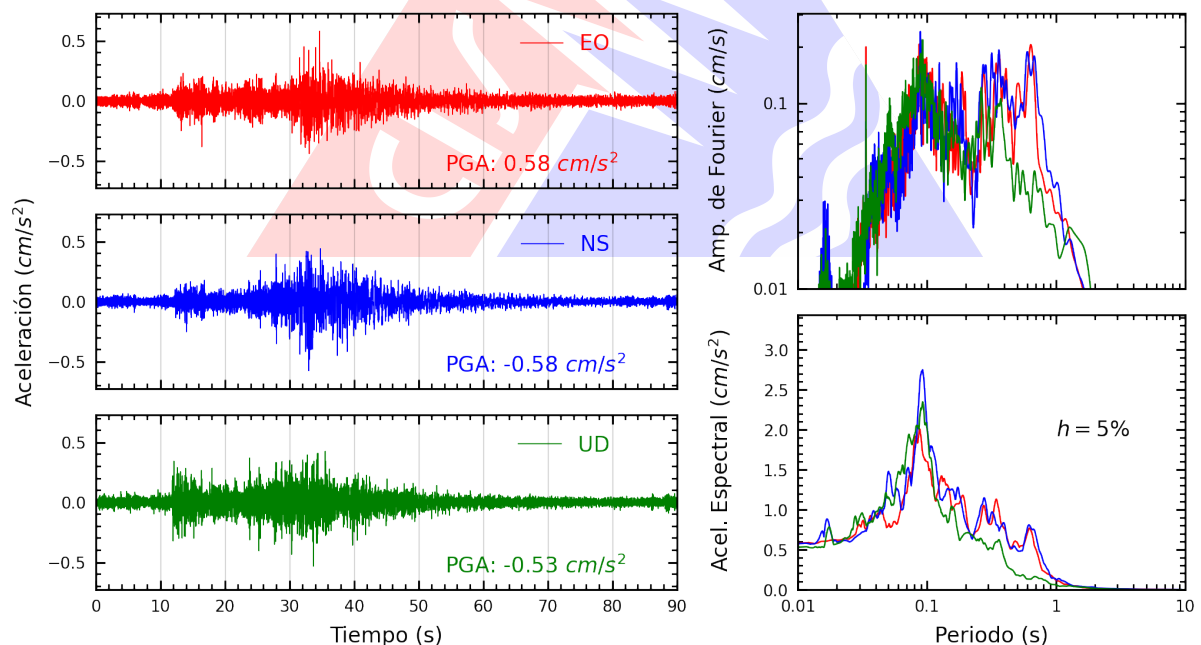
Figura A.2: Registros tiempo-historia, espectros de Fourier y de respuesta en las direcciones EO, NS y vertical de la estación SCICA. Sismo de Huancavelica, Huancavelica - Huancavelica del 2023-10-03, 02:40:16 (Hora local)
