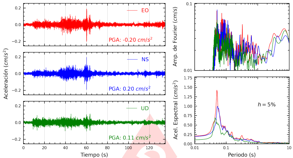
Figura A.19: Registros tiempo-historia, espectros de Fourier y de respuesta en las direcciones EO, NS y vertical de la estación UPCSM. Sismo de Huancavelica, Huancavelica - Huancavelica del 2023-10-03, 02:40:16 (Hora local)
