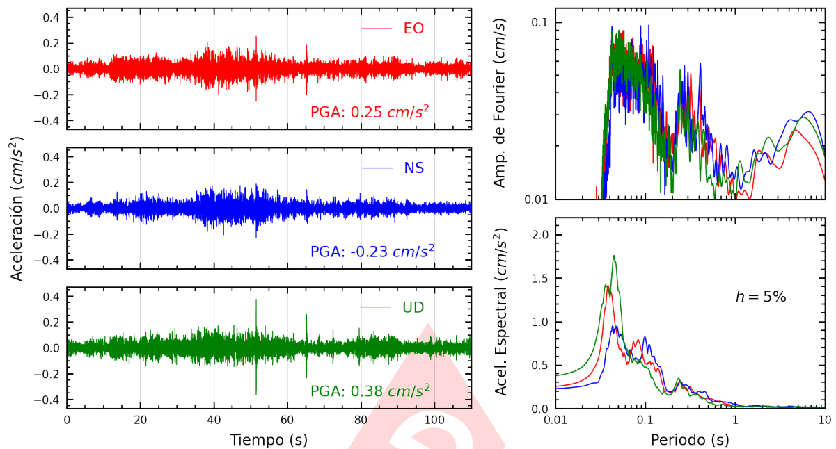
Figura A.7: Registros tiempo-historia, espectros de Fourier y de respuesta en las direcciones EO, NS y vertical de la estación URPE. Sismo de Huancavelica, Huancavelica - Huancavelica del 2023-10-03, 02:40:16 (Hora local)
