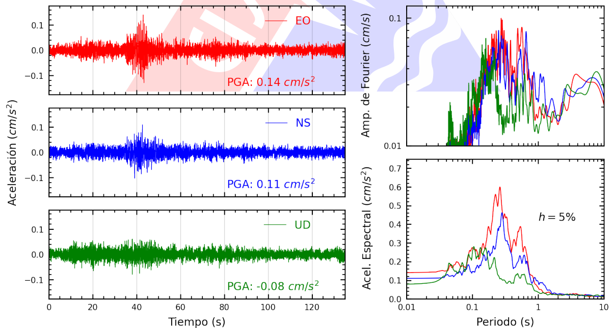
Figura A.30: Registros tiempo-historia, espectros de Fourier y de respuesta en las direcciones EO, NS y vertical de la estación DSMI. Sismo de Huancavelica, Huancavelica - Huancavelica del 2023-10-03, 02:40:16 (Hora local)
