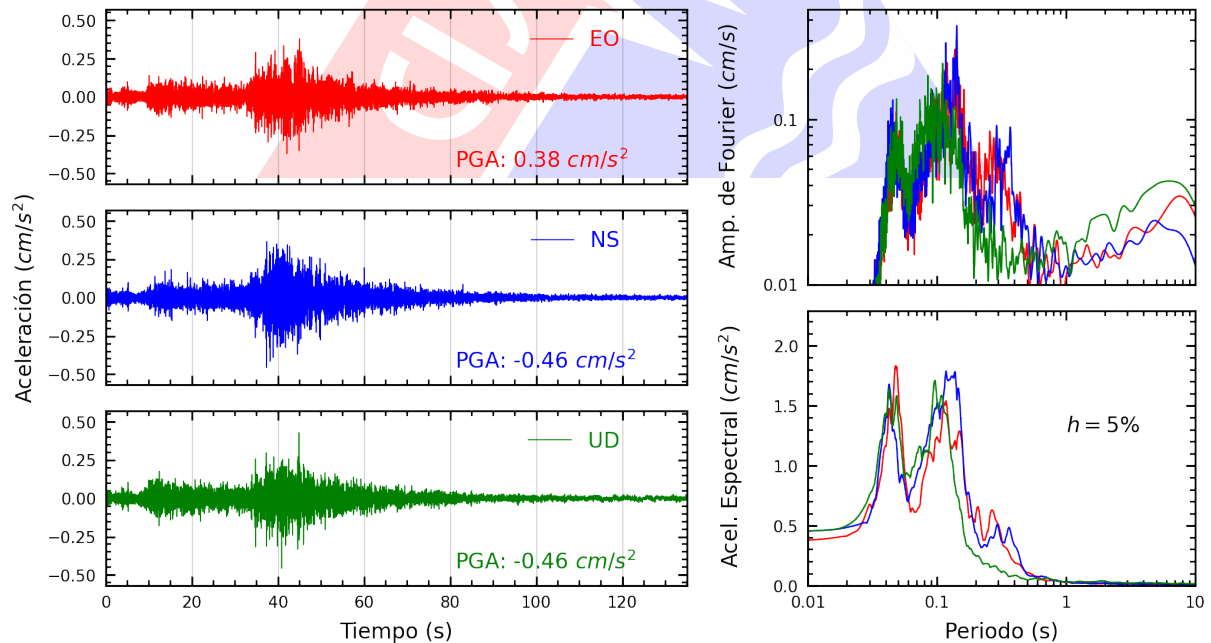
Figura A.4: Registros tiempo-historia, espectros de Fourier y de respuesta en las direcciones EO, NS y vertical de la estación CARAB. Sismo de Huancavelica, Huancavelica - Huancavelica del 2023-10-03, 02:40:16 (Hora local)
