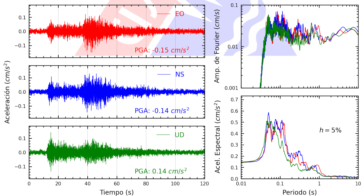
Figura A.28: Registros tiempo-historia, espectros de Fourier y de respuesta en las direcciones EO, NS y vertical de la estación CENEP. Sismo de Huancavelica, Huancavelica - Huancavelica del 2023-10-03, 02:40:16 (Hora local)
