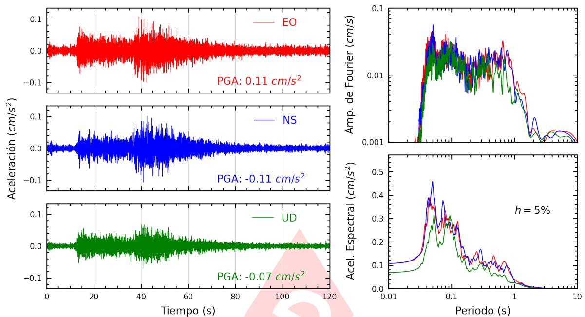
Figura A.33: Registros tiempo-historia, espectros de Fourier y de respuesta en las direcciones EO, NS y vertical de la estación BORJA. Sismo de Huancavelica, Huancavelica - Huancavelica del 2023-10-03, 02:40:16 (Hora local)
