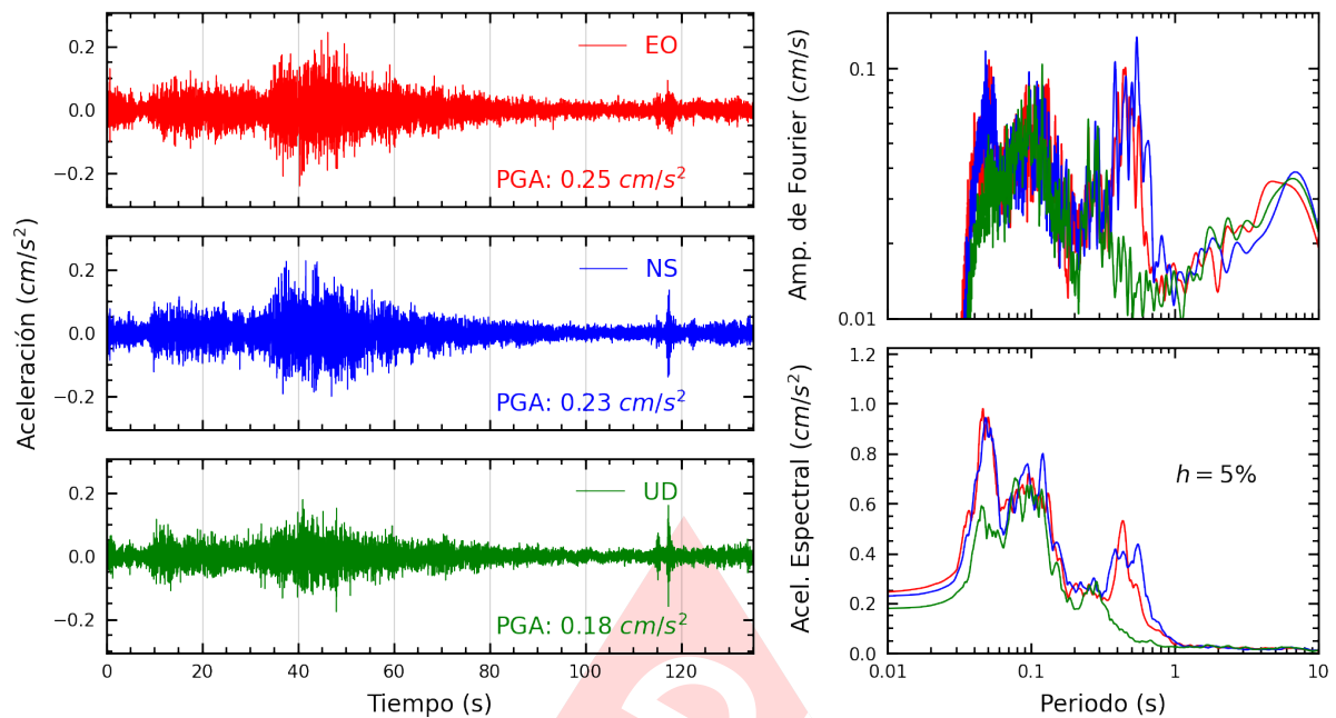
Figura A.15: Registros tiempo-historia, espectros de Fourier y de respuesta en las direcciones EO, NS y vertical de la estación OLIVO. Sismo de Huancavelica, Huancavelica - Huancavelica del 2023-10-03, 02:40:16 (Hora local)
