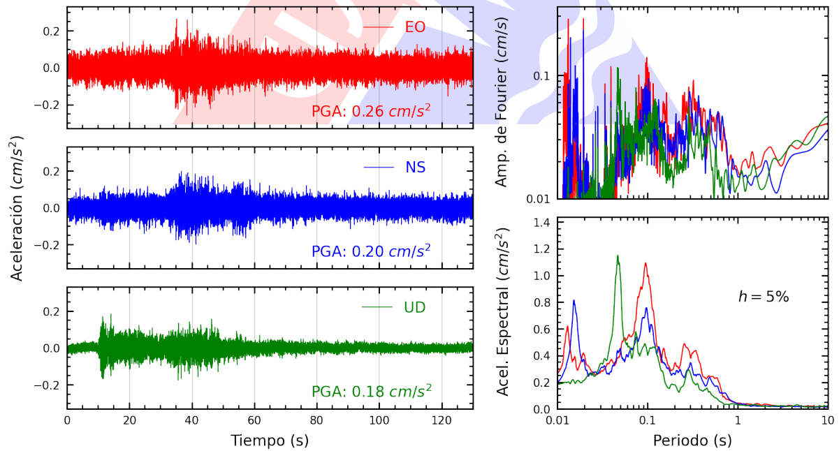
Figura A.12: Registros tiempo-historia, espectros de Fourier y de respuesta en las direcciones EO, NS y vertical de la estación USILP. Sismo de Huancavelica, Huancavelica - Huancavelica del 2023-10-03, 02:40:16 (Hora local)
