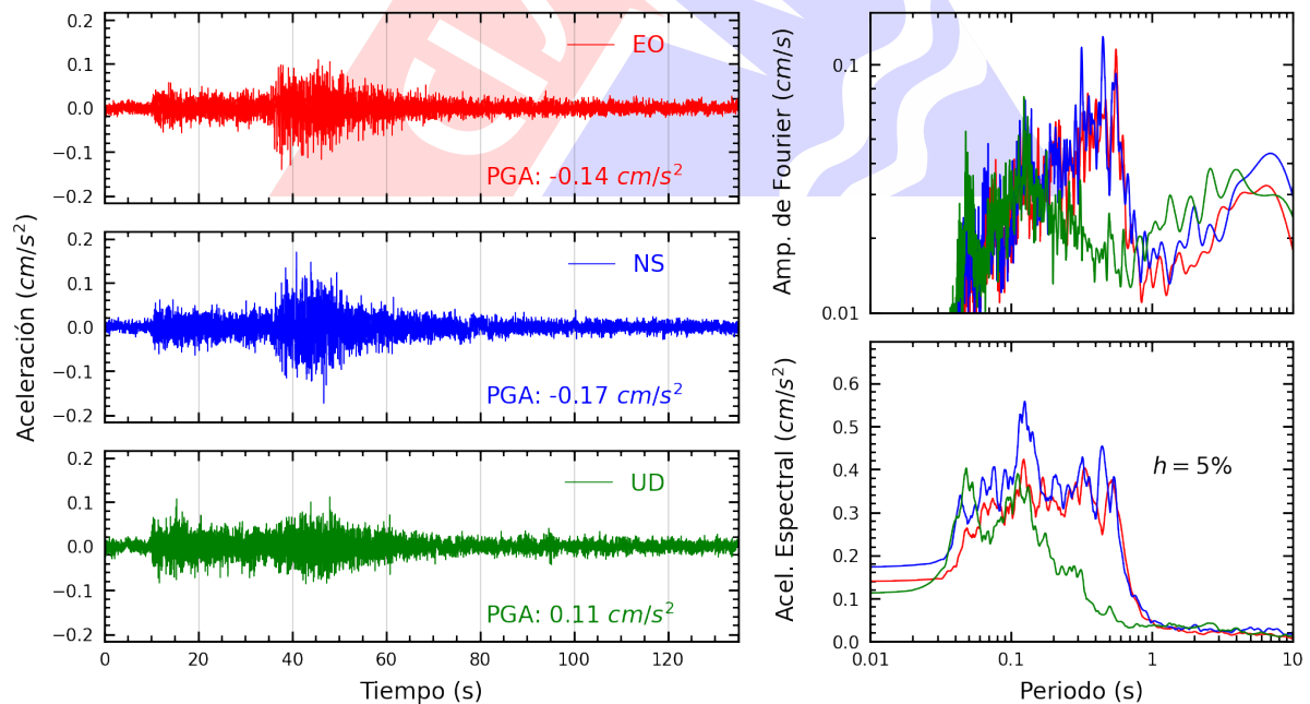
Figura A.26: Registros tiempo-historia, espectros de Fourier y de respuesta en las direcciones EO, NS y vertical de la estación VHAYA. Sismo de Huancavelica, Huancavelica - Huancavelica del 2023-10-03, 02:40:16 (Hora local)
