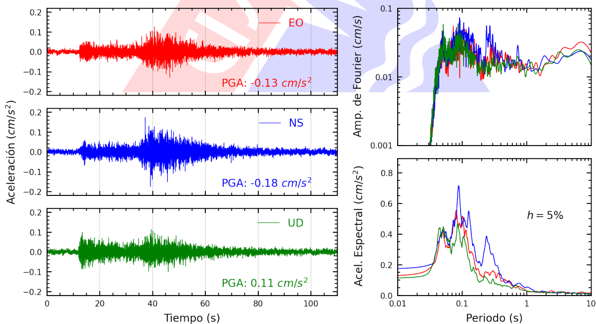
Figura A.24: Registros tiempo-historia, espectros de Fourier y de respuesta en las direcciones EO, NS y vertical de la estación SERVI. Sismo de Huancavelica, Huancavelica - Huancavelica del 2023-10-03, 02:40:16 (Hora local)
