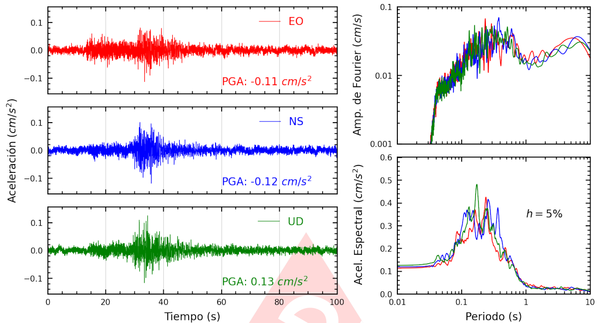
Figura A.31: Registros tiempo-historia, espectros de Fourier y de respuesta en las direcciones EO, NS y vertical de la estación UNSCH. Sismo de Huancavelica, Huancavelica - Huancavelica del 2023-10-03, 02:40:16 (Hora local)
