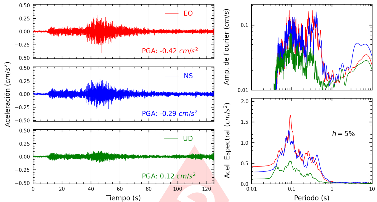
Figura A.5: Registros tiempo-historia, espectros de Fourier y de respuesta en las direcciones EO, NS y vertical de la estación DEFEN. Sismo de Huancavelica, Huancavelica - Huancavelica del 2023-10-03, 02:40:16 (Hora local)
