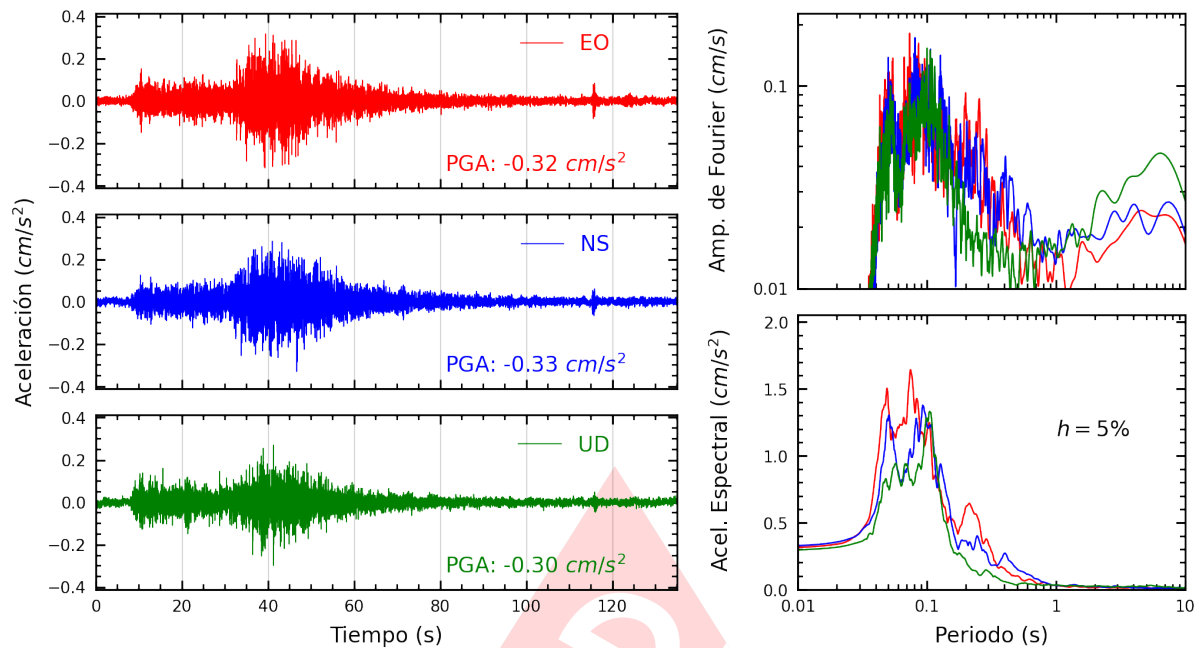
Figura A.9: Registros tiempo-historia, espectros de Fourier y de respuesta en las direcciones EO, NS y vertical de la estación INDEP. Sismo de Huancavelica, Huancavelica - Huancavelica del 2023-10-03, 02:40:16 (Hora local)
