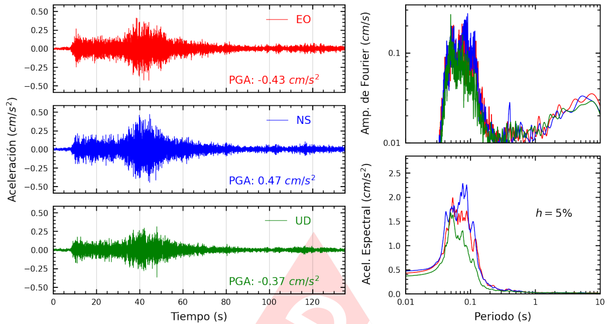
Figura A.3: Registros tiempo-historia, espectros de Fourier y de respuesta en las direcciones EO, NS y vertical de la estación JOSEO. Sismo de Huancavelica, Huancavelica - Huancavelica del 2023-10-03, 02:40:16 (Hora local)
