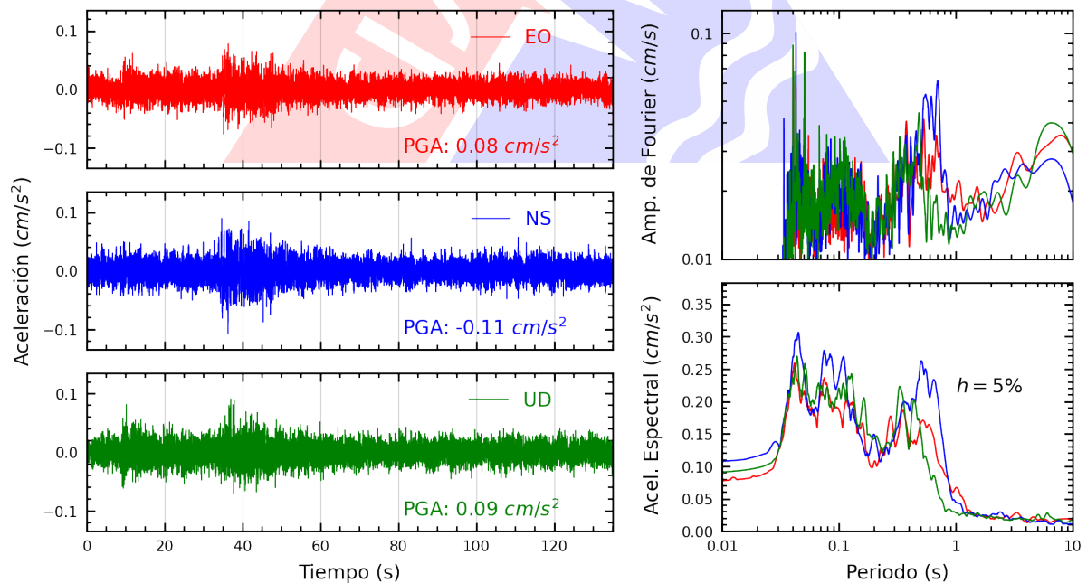
Figura A.32: Registros tiempo-historia, espectros de Fourier y de respuesta en las direcciones EO, NS y vertical de la estación BONDY. Sismo de Huancavelica, Huancavelica - Huancavelica del 2023-10-03, 02:40:16 (Hora local)
