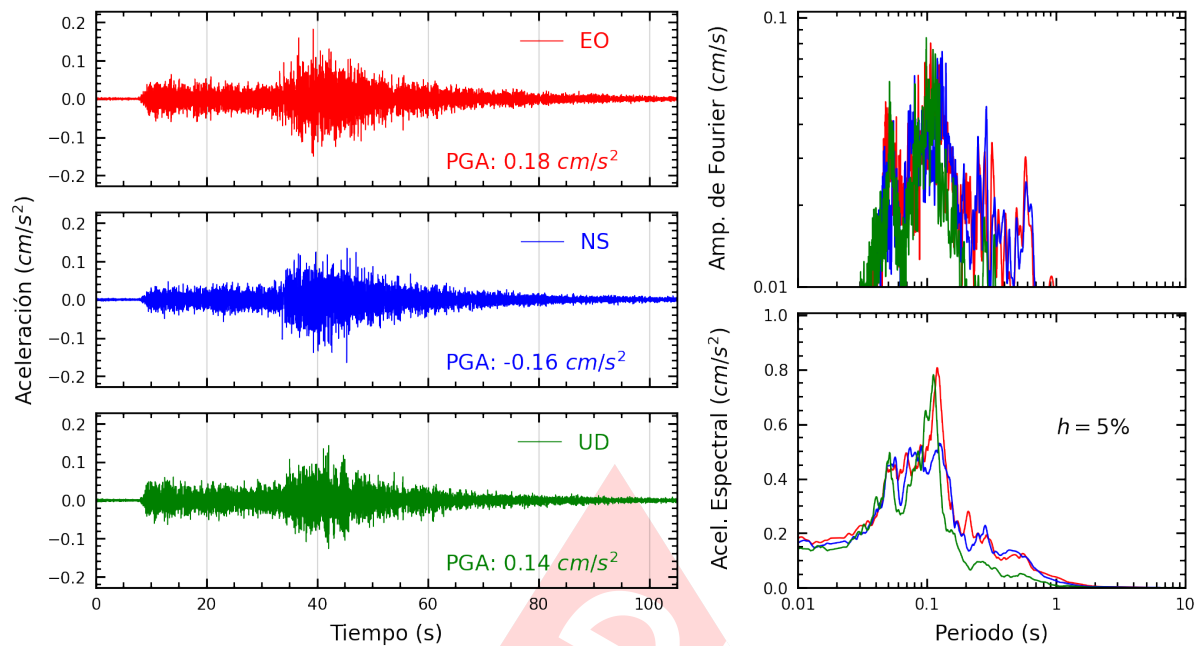
Figura A.21: Registros tiempo-historia, espectros de Fourier y de respuesta en las direcciones EO, NS y vertical de la estación JALV2. Sismo de Huancavelica, Huancavelica - Huancavelica del 2023-10-03, 02:40:16 (Hora local)
