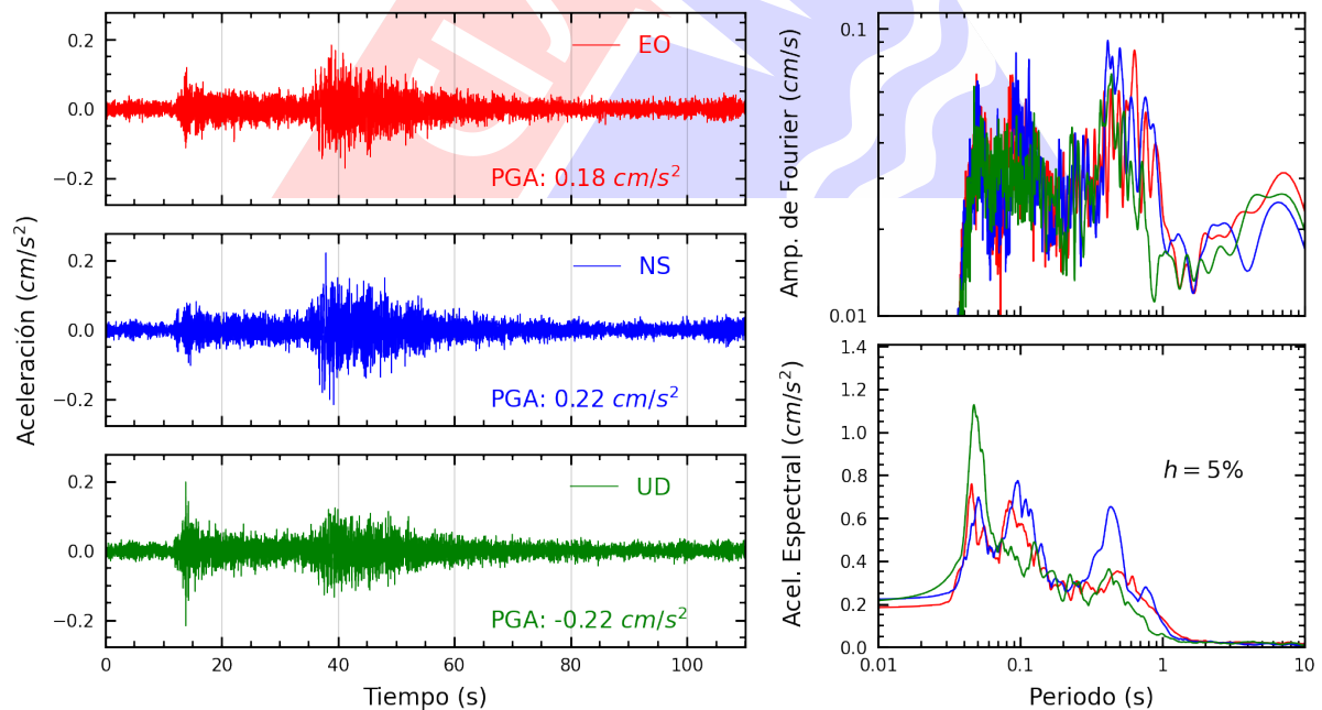
Figura A.18: Registros tiempo-historia, espectros de Fourier y de respuesta en las direcciones EO, NS y vertical de la estación IMCA. Sismo de Huancavelica, Huancavelica - Huancavelica del 2023-10-03, 02:40:16 (Hora local)
