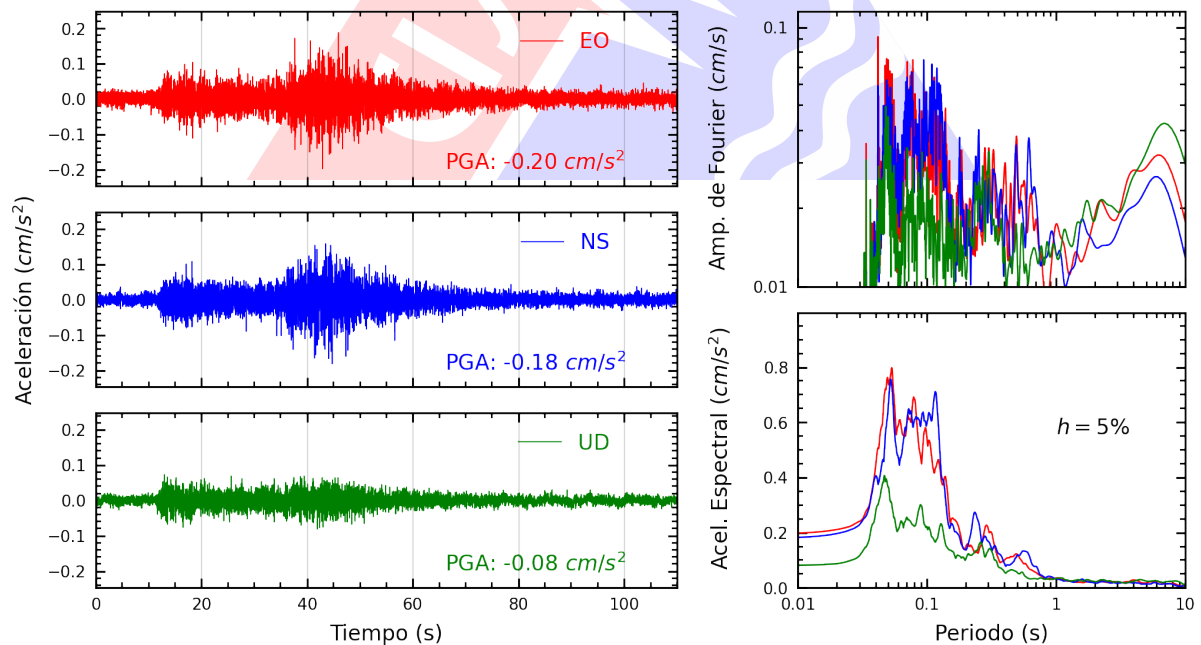
Figura A.20: Registros tiempo-historia, espectros de Fourier y de respuesta en las direcciones EO, NS y vertical de la estación UPCVI. Sismo de Huancavelica, Huancavelica - Huancavelica del 2023-10-03, 02:40:16 (Hora local)
