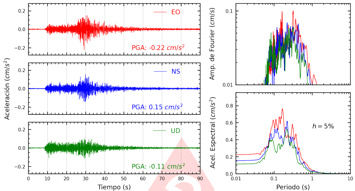
Figura A.17: Registros tiempo-historia, espectros de Fourier y de respuesta en las direcciones EO, NS y vertical de la estación SCAYA. Sismo de Huancavelica, Huancavelica - Huancavelica del 2023-10-03, 02:40:16 (Hora local)
