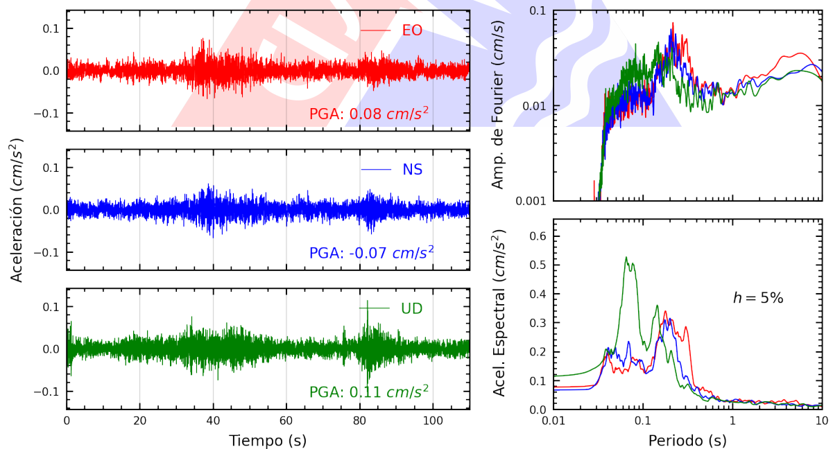
Figura A.28: Registros tiempo-historia, espectros de Fourier y de respuesta en las direcciones EO, NS y vertical de la estación DSMI. Sismo de Barranca, Barranca - Lima del 2023-10-17, 01:53:04 (Hora local)
