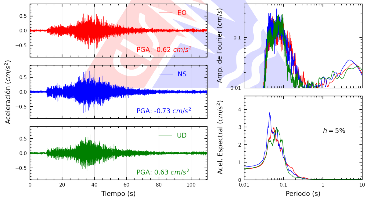
Figura A.2: Registros tiempo-historia, espectros de Fourier y de respuesta en las direcciones EO, NS y vertical de la estación SROSA. Sismo de Barranca, Barranca - Lima del 2023-10-17, 01:53:04 (Hora local)
