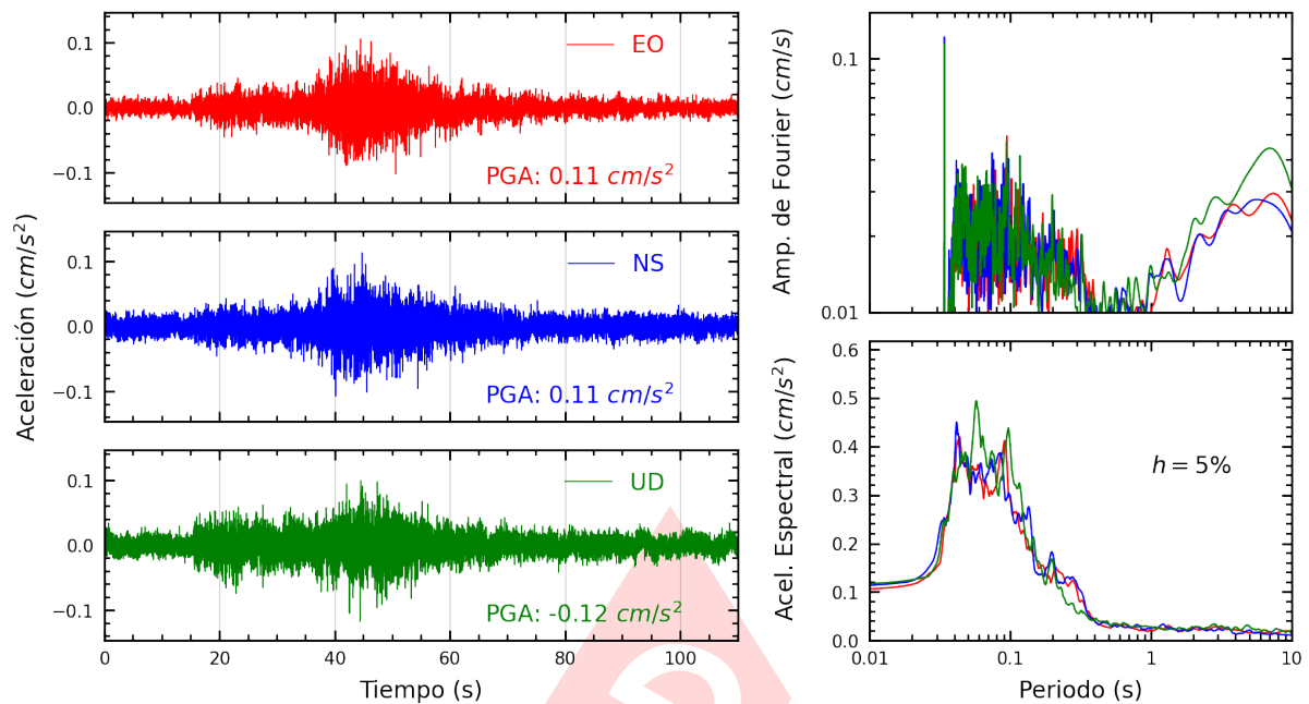
Figura A.27: Registros tiempo-historia, espectros de Fourier y de respuesta en las direcciones EO, NS y vertical de la estación USMP. Sismo de Barranca, Barranca - Lima del 2023-10-17, 01:53:04 (Hora local)
