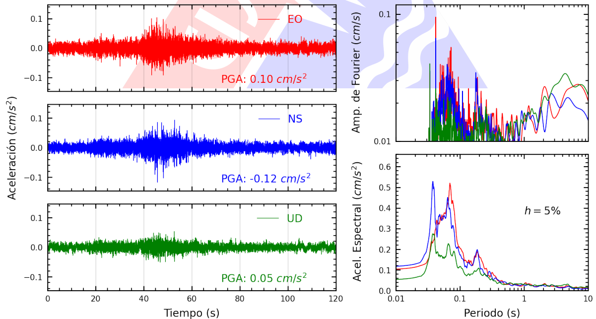
Figura A.26: Registros tiempo-historia, espectros de Fourier y de respuesta en las direcciones EO, NS y vertical de la estación UPCVI. Sismo de Barranca, Barranca - Lima del 2023-10-17, 01:53:04 (Hora local)
