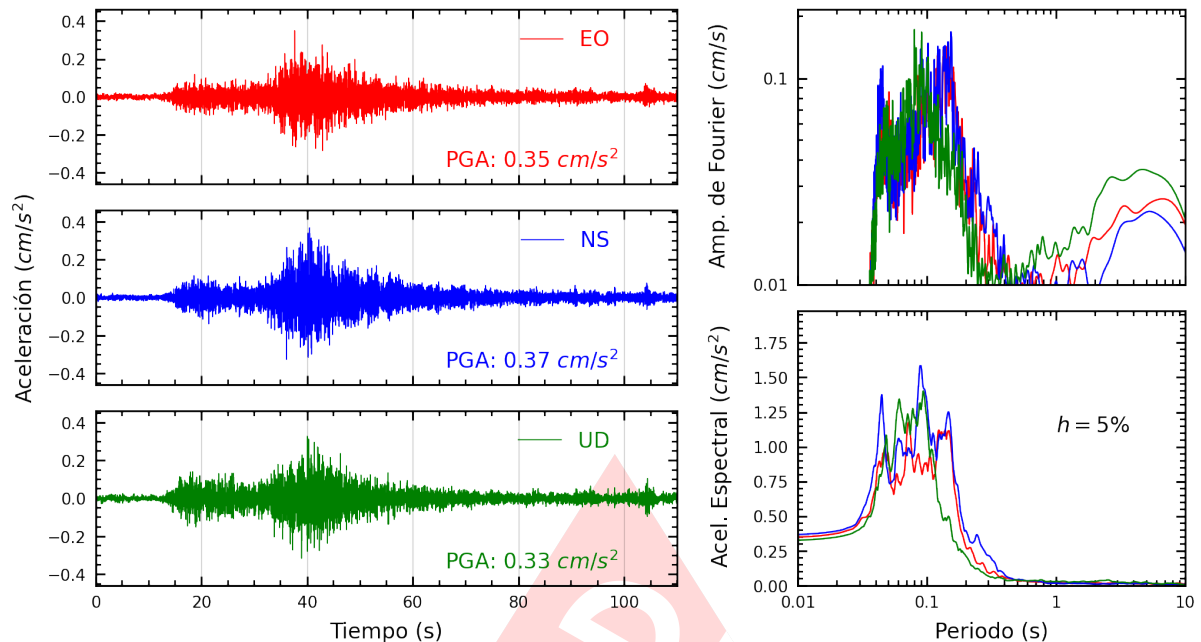
Figura A.9: Registros tiempo-historia, espectros de Fourier y de respuesta en las direcciones EO, NS y vertical de la estación CARAB. Sismo de Barranca, Barranca - Lima del 2023-10-17, 01:53:04 (Hora local)
