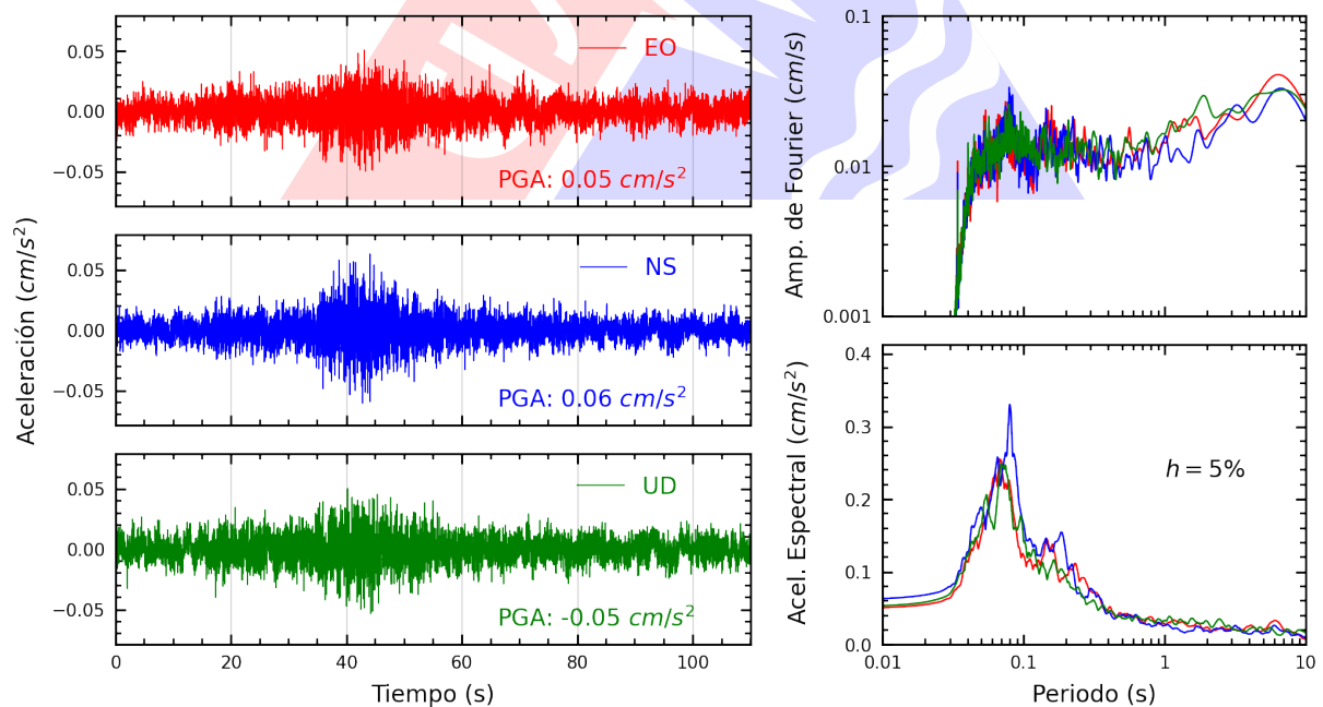
Figura A.34: Registros tiempo-historia, espectros de Fourier y de respuesta en las direcciones EO, NS y vertical de la estación UNMSM. Sismo de Barranca, Barranca - Lima del 2023-10-17, 01:53:04 (Hora local)
