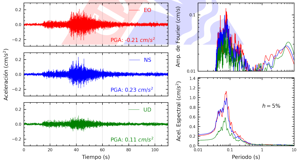
Figura A.12: Registros tiempo-historia, espectros de Fourier y de respuesta en las direcciones EO, NS y vertical de la estación FICPE. Sismo de Barranca, Barranca - Lima del 2023-10-17, 01:53:04 (Hora local)
