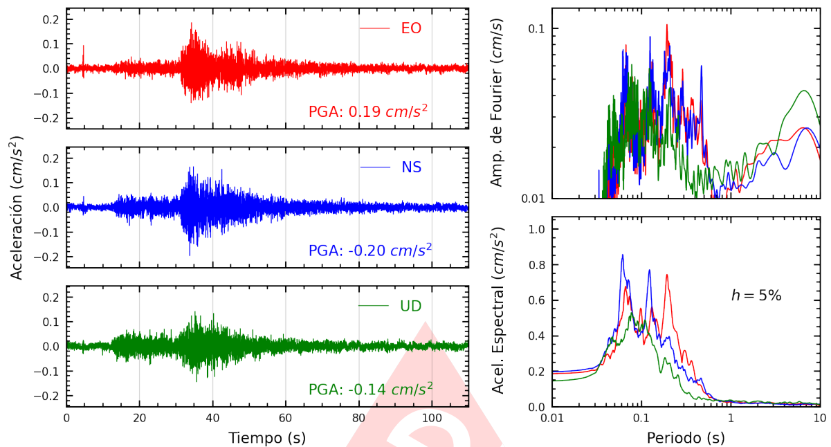
Figura A.15: Registros tiempo-historia, espectros de Fourier y de respuesta en las direcciones EO, NS y vertical de la estación VHAYA. Sismo de Barranca, Barranca - Lima del 2023-10-17, 01:53:04 (Hora local)
