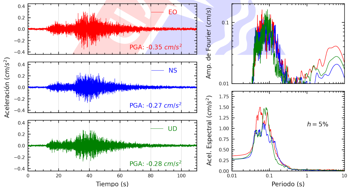
Figura A.10: Registros tiempo-historia, espectros de Fourier y de respuesta en las direcciones EO, NS y vertical de la estación AMORE. Sismo de Barranca, Barranca - Lima del 2023-10-17, 01:53:04 (Hora local)
