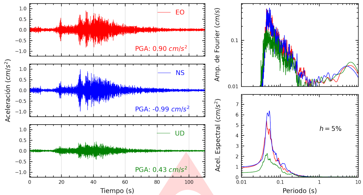
Figura A.1: Registros tiempo-historia, espectros de Fourier y de respuesta en las direcciones EO, NS y vertical de la estación USP. Sismo de Barranca, Barranca - Lima del 2023-10-17, 01:53:04 (Hora local)
