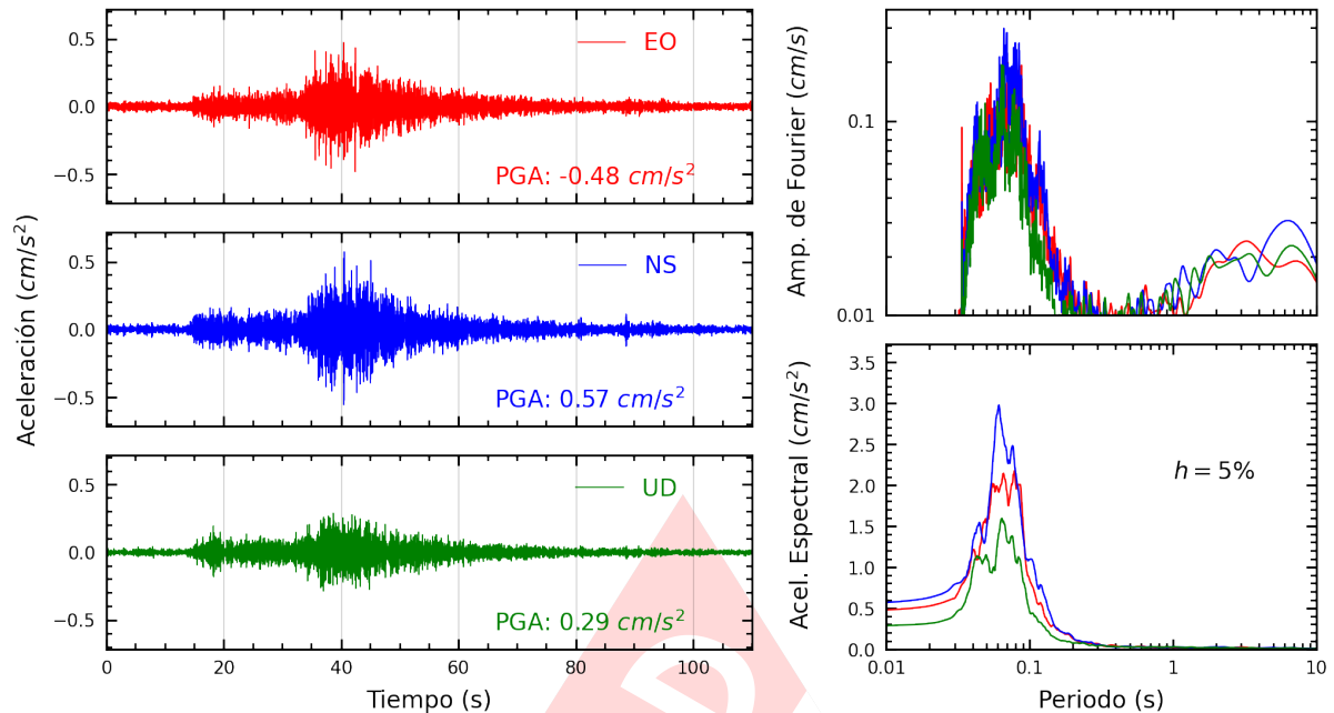
Figura A.5: Registros tiempo-historia, espectros de Fourier y de respuesta en las direcciones EO, NS y vertical de la estación JOSEO. Sismo de Barranca, Barranca - Lima del 2023-10-17, 01:53:04 (Hora local)
