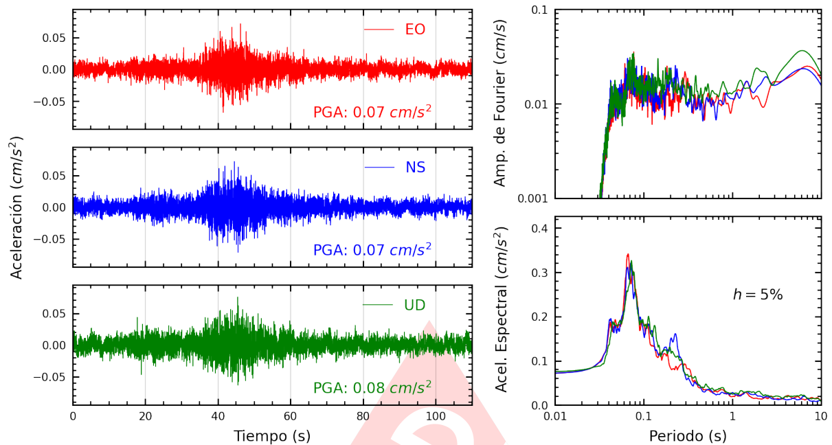
Figura A.33: Registros tiempo-historia, espectros de Fourier y de respuesta en las direcciones EO, NS y vertical de la estación UNFV. Sismo de Barranca, Barranca - Lima del 2023-10-17, 01:53:04 (Hora local)
