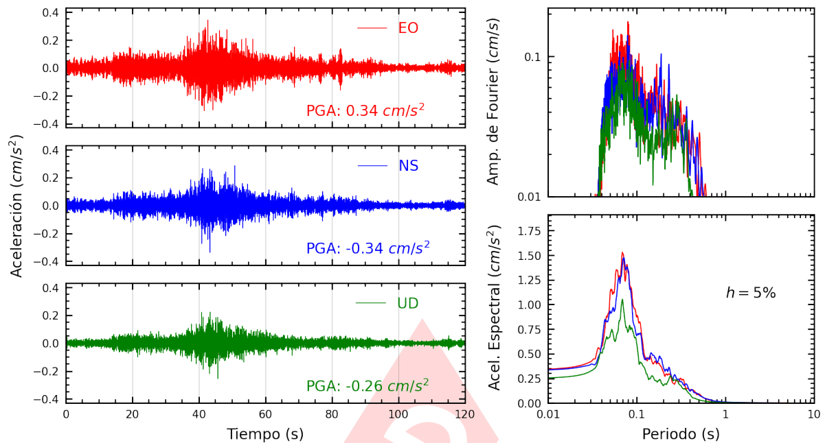
Figura A.11: Registros tiempo-historia, espectros de Fourier y de respuesta en las direcciones EO, NS y vertical de la estación UNTEL. Sismo de Barranca, Barranca - Lima del 2023-10-17, 01:53:04 (Hora local)
