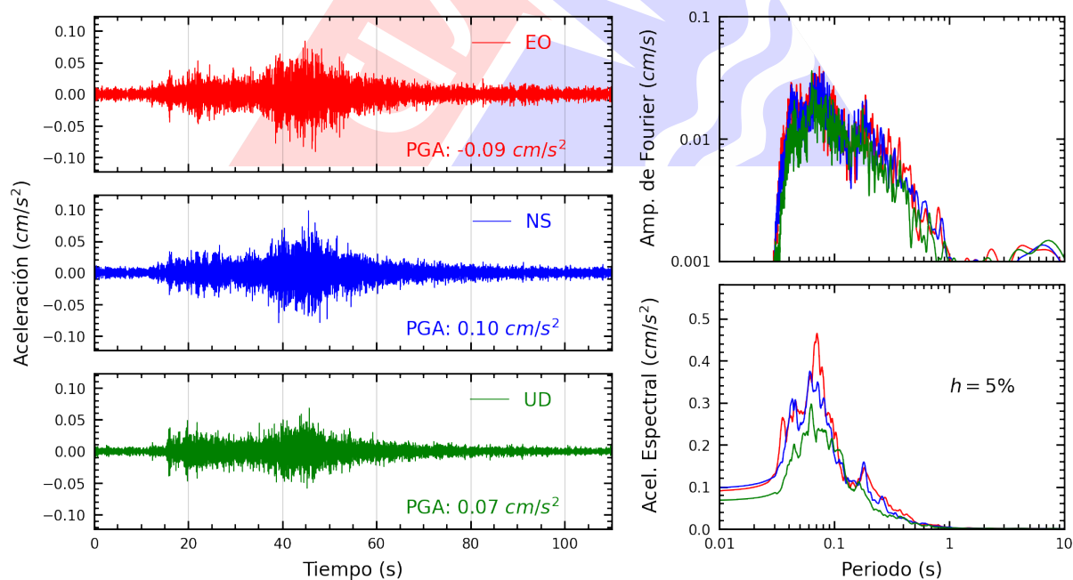
Figura A.30: Registros tiempo-historia, espectros de Fourier y de respuesta en las direcciones EO, NS y vertical de la estación BORJA. Sismo de Barranca, Barranca - Lima del 2023-10-17, 01:53:04 (Hora local)
