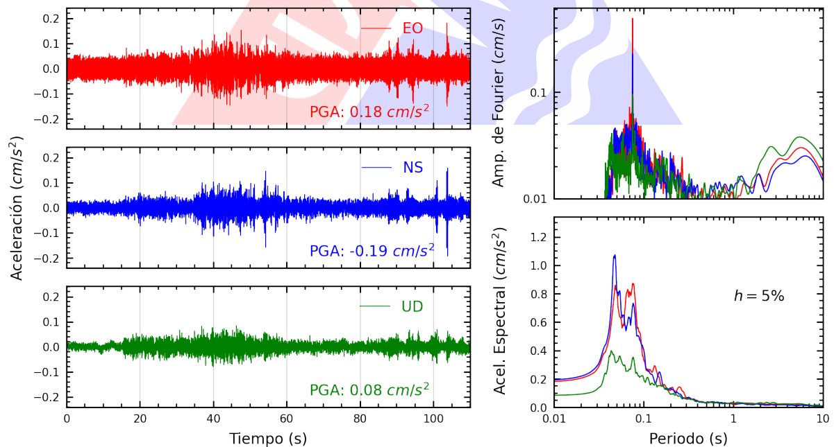
Figura A.16: Registros tiempo-historia, espectros de Fourier y de respuesta en las direcciones EO, NS y vertical de la estación UPCSM. Sismo de Barranca, Barranca - Lima del 2023-10-17, 01:53:04 (Hora local)
