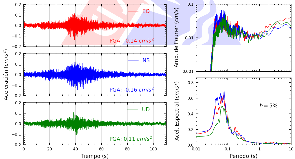
Figura A.18: Registros tiempo-historia, espectros de Fourier y de respuesta en las direcciones EO, NS y vertical de la estación COMAS. Sismo de Barranca, Barranca - Lima del 2023-10-17, 01:53:04 (Hora local)
