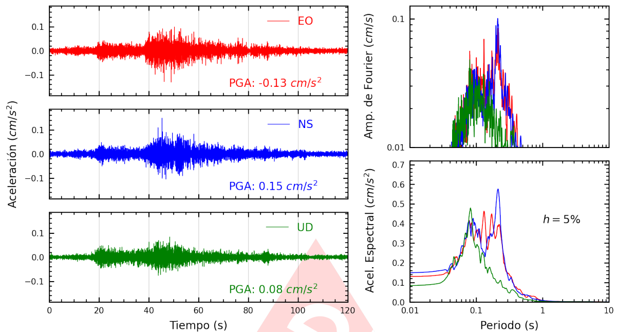
Figura A.21: Registros tiempo-historia, espectros de Fourier y de respuesta en las direcciones EO, NS y vertical de la estación SCCHO. Sismo de Barranca, Barranca - Lima del 2023-10-17, 01:53:04 (Hora local)
