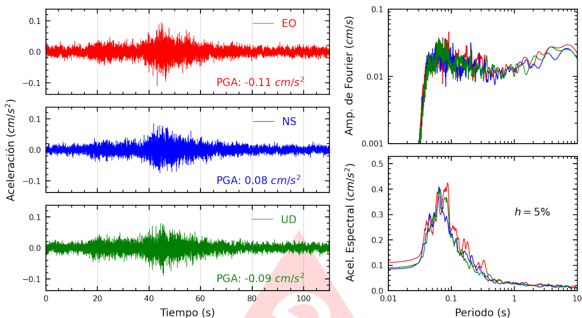
Figura A.29: Registros tiempo-historia, espectros de Fourier y de respuesta en las direcciones EO, NS y vertical de la estación IMCA. Sismo de Barranca, Barranca - Lima del 2023-10-17, 01:53:04 (Hora local)
