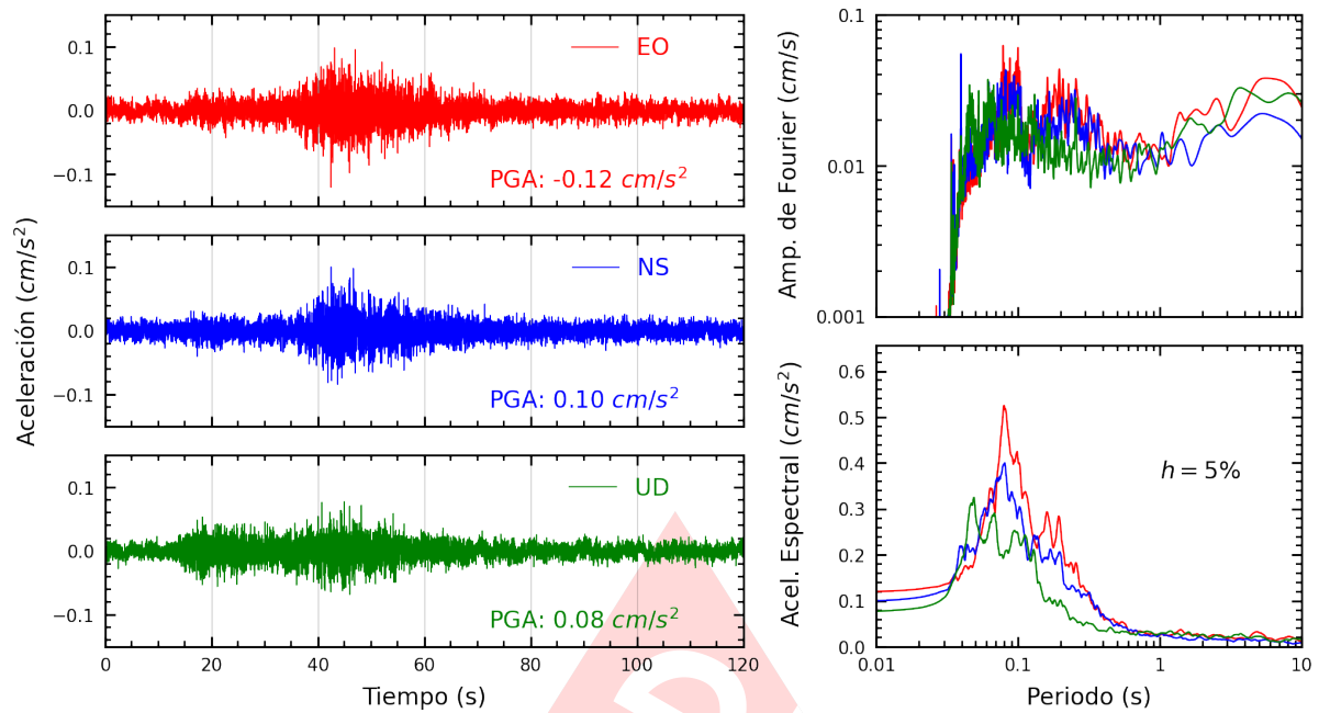
Figura A.25: Registros tiempo-historia, espectros de Fourier y de respuesta en las direcciones EO, NS y vertical de la estación USILP. Sismo de Barranca, Barranca - Lima del 2023-10-17, 01:53:04 (Hora local)
