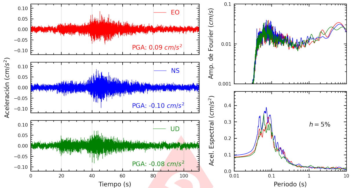
Figura A.31: Registros tiempo-historia, espectros de Fourier y de respuesta en las direcciones EO, NS y vertical de la estación SERVI. Sismo de Barranca, Barranca - Lima del 2023-10-17, 01:53:04 (Hora local)
