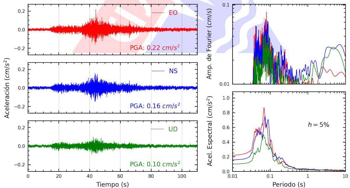
Figura A.14: Registros tiempo-historia, espectros de Fourier y de respuesta en las direcciones EO, NS y vertical de la estación CEPRE. Sismo de Barranca, Barranca - Lima del 2023-10-17, 01:53:04 (Hora local)
