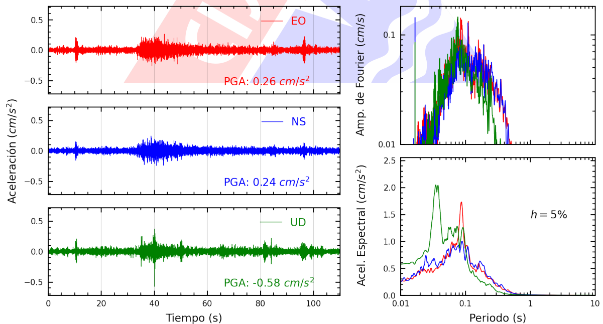
Figura A.4: Registros tiempo-historia, espectros de Fourier y de respuesta en las direcciones EO, NS y vertical de la estación SCOLI. Sismo de Barranca, Barranca - Lima del 2023-10-17, 01:53:04 (Hora local)
