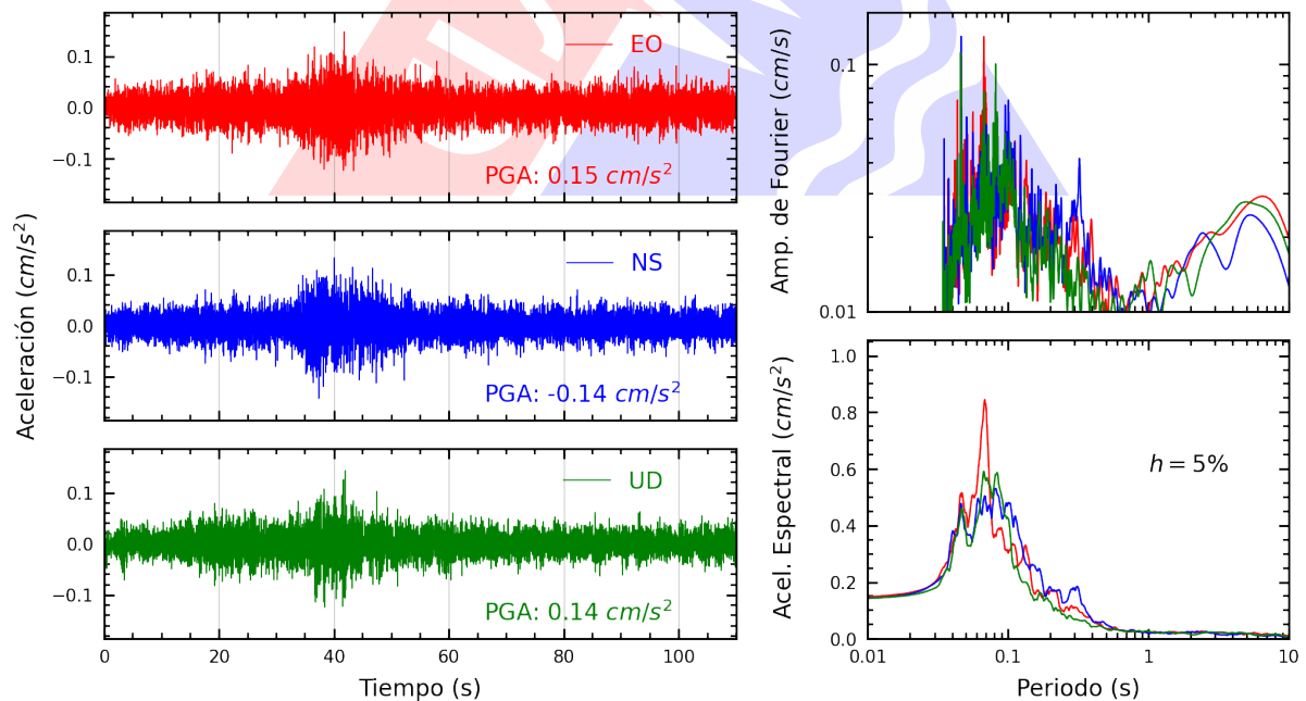
Figura A.22: Registros tiempo-historia, espectros de Fourier y de respuesta en las direcciones EO, NS y vertical de la estación MADRE. Sismo de Barranca, Barranca - Lima del 2023-10-17, 01:53:04 (Hora local)
