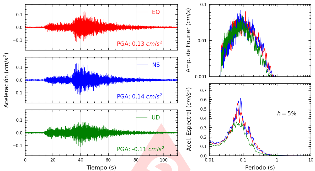
Figura A.23: Registros tiempo-historia, espectros de Fourier y de respuesta en las direcciones EO, NS y vertical de la estación JALV2. Sismo de Barranca, Barranca - Lima del 2023-10-17, 01:53:04 (Hora local)
