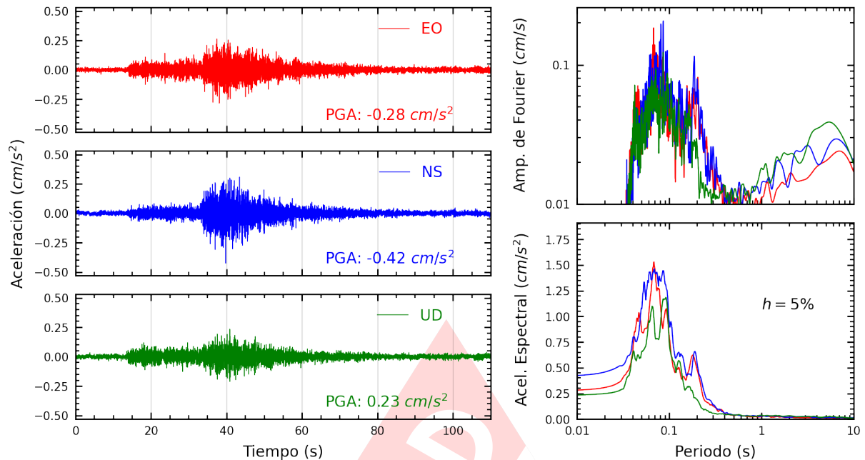
Figura A.7: Registros tiempo-historia, espectros de Fourier y de respuesta en las direcciones EO, NS y vertical de la estación INDEP. Sismo de Barranca, Barranca - Lima del 2023-10-17, 01:53:04 (Hora local)
