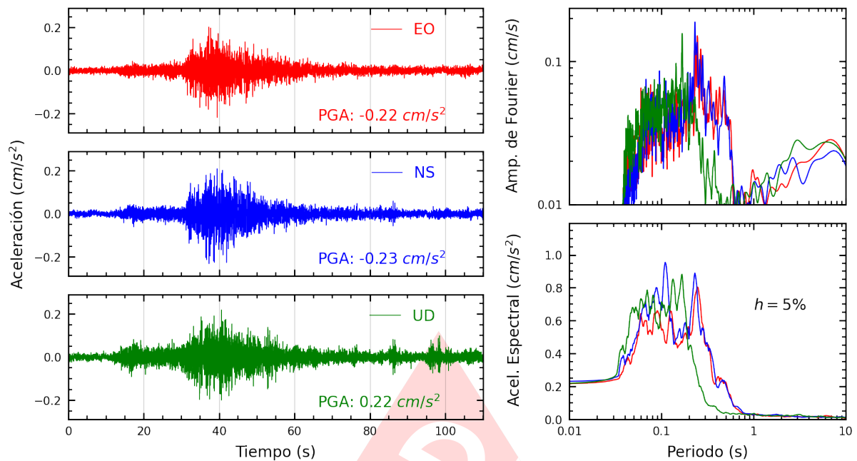
Figura A.13: Registros tiempo-historia, espectros de Fourier y de respuesta en las direcciones EO, NS y vertical de la estación MDPP. Sismo de Barranca, Barranca - Lima del 2023-10-17, 01:53:04 (Hora local)
