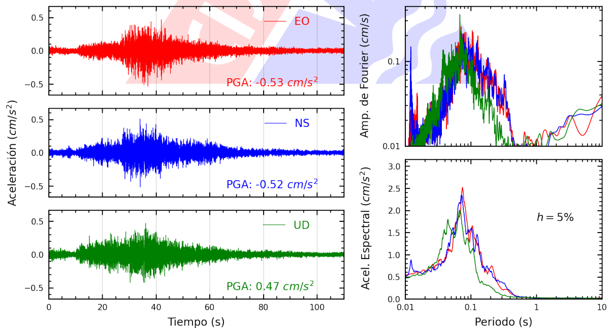
Figura A.6: Registros tiempo-historia, espectros de Fourier y de respuesta en las direcciones EO, NS y vertical de la estación ANCON. Sismo de Barranca, Barranca - Lima del 2023-10-17, 01:53:04 (Hora local)
