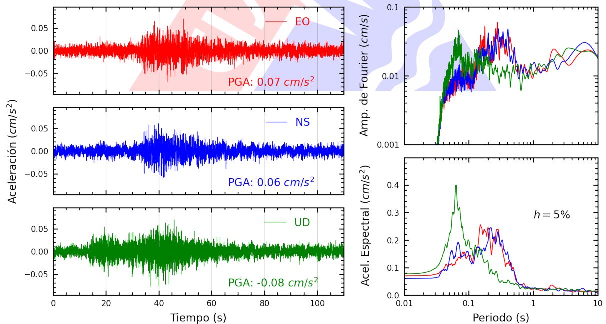
Figura A.32: Registros tiempo-historia, espectros de Fourier y de respuesta en las direcciones EO, NS y vertical de la estación ACAPU. Sismo de Barranca, Barranca - Lima del 2023-10-17, 01:53:04 (Hora local)
