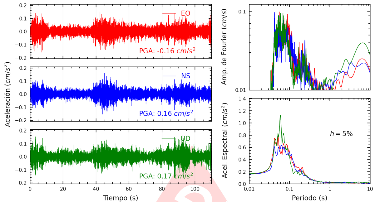
Figura A.17: Registros tiempo-historia, espectros de Fourier y de respuesta en las direcciones EO, NS y vertical de la estación URPE. Sismo de Barranca, Barranca - Lima del 2023-10-17, 01:53:04 (Hora local)
