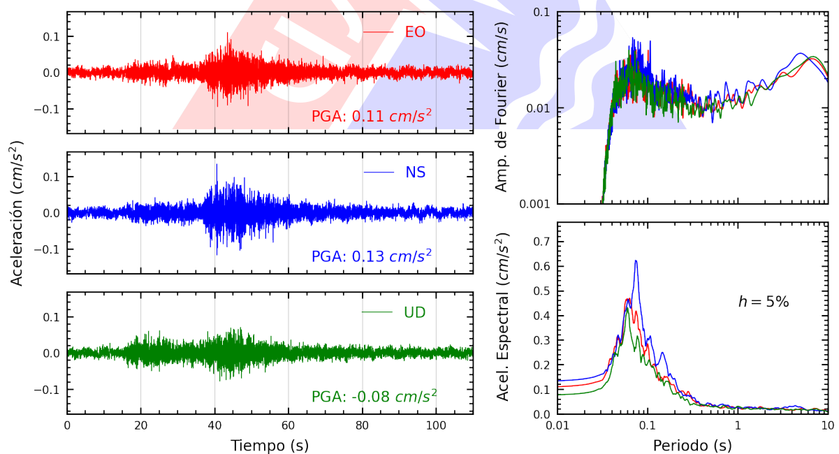
Figura A.24: Registros tiempo-historia, espectros de Fourier y de respuesta en las direcciones EO, NS y vertical de la estación CENEP. Sismo de Barranca, Barranca - Lima del 2023-10-17, 01:53:04 (Hora local)
