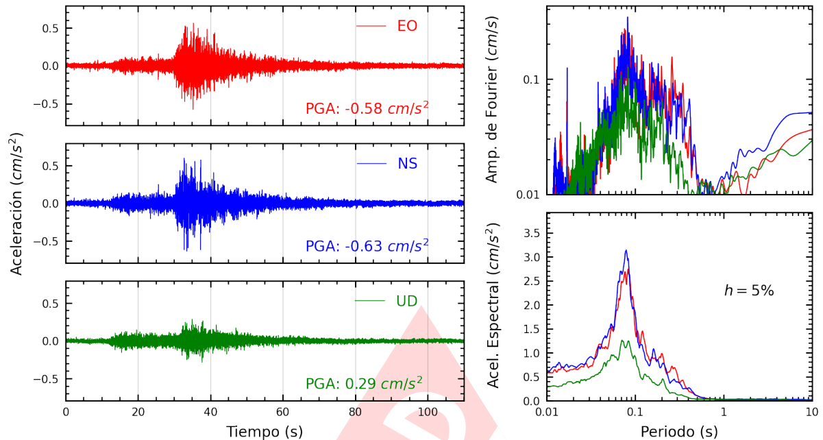
Figura A.3: Registros tiempo-historia, espectros de Fourier y de respuesta en las direcciones EO, NS y vertical de la estación DEFEN. Sismo de Barranca, Barranca - Lima del 2023-10-17, 01:53:04 (Hora local)
