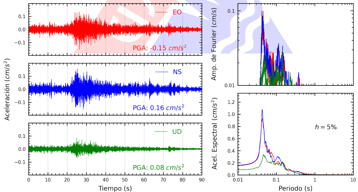
Figura A.20: Registros tiempo-historia, espectros de Fourier y de respuesta en las direcciones EO, NS y vertical de la estación SCTRU. Sismo de Barranca, Barranca - Lima del 2023-10-17, 01:53:04 (Hora local)
