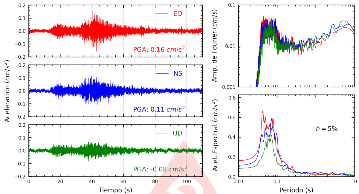
Figura A.19: Registros tiempo-historia, espectros de Fourier y de respuesta en las direcciones EO, NS y vertical de la estación UCSS. Sismo de Barranca, Barranca - Lima del 2023-10-17, 01:53:04 (Hora local)
