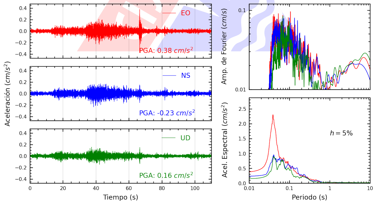
Figura A.8: Registros tiempo-historia, espectros de Fourier y de respuesta en las direcciones EO, NS y vertical de la estación OLIVO. Sismo de Barranca, Barranca - Lima del 2023-10-17, 01:53:04 (Hora local)
