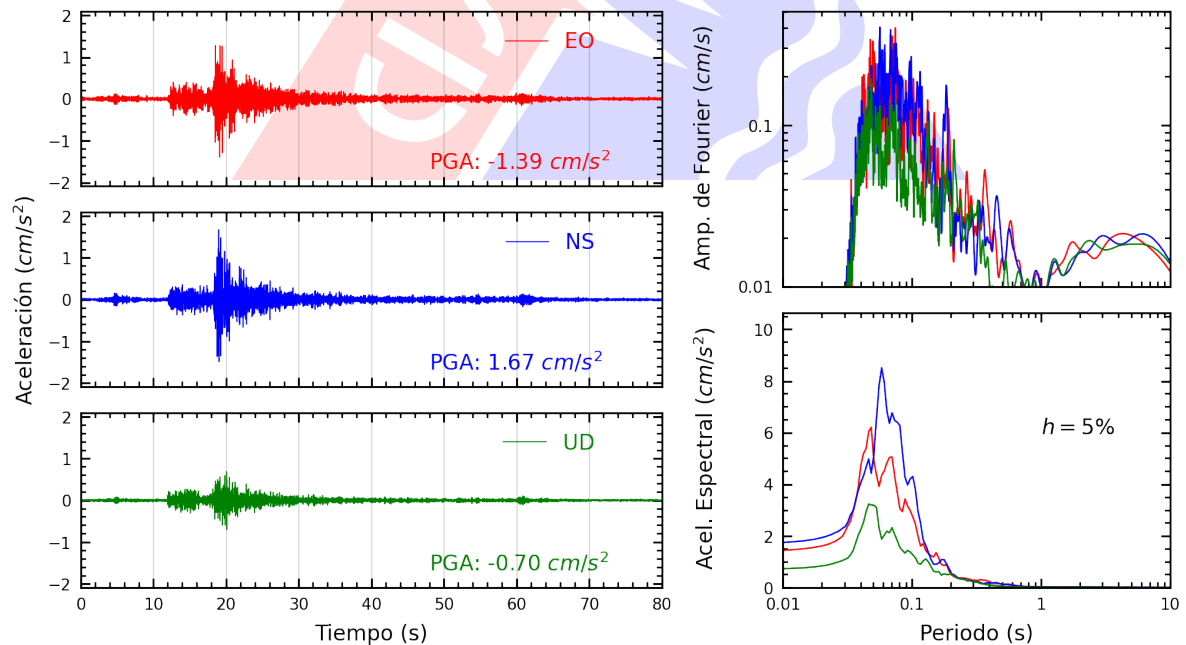
Figura A.20: Registros tiempo-historia, espectros de Fourier y de respuesta en las direcciones EO, NS y vertical de la estación UPCVI. Sismo de Chilca, Cañete - Lima del 2023-11-01, 07:49:31 (Hora local)
