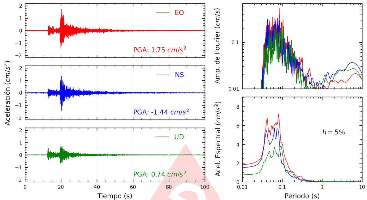
Figura A.17: Registros tiempo-historia, espectros de Fourier y de respuesta en las direcciones EO, NS y vertical de la estación CEPRE. Sismo de Chilca, Cañete - Lima del 2023-11-01, 07:49:31 (Hora local)
