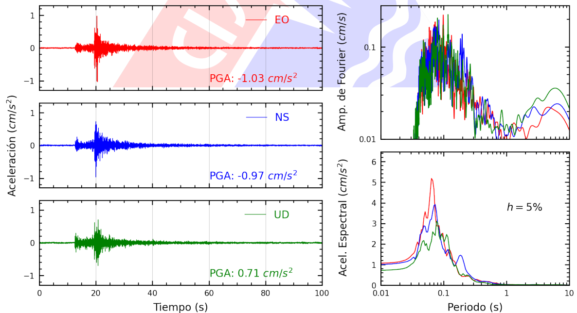
Figura A.32: Registros tiempo-historia, espectros de Fourier y de respuesta en las direcciones EO, NS y vertical de la estación UNFV. Sismo de Chilca, Cañete - Lima del 2023-11-01, 07:49:31 (Hora local)
