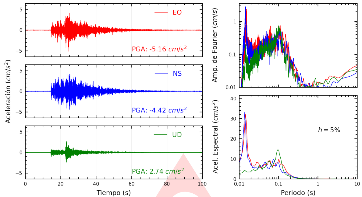
Figura A.1: Registros tiempo-historia, espectros de Fourier y de respuesta en las direcciones EO, NS y vertical de la estación AMORE. Sismo de Chilca, Cañete - Lima del 2023-11-01, 07:49:31 (Hora local)
