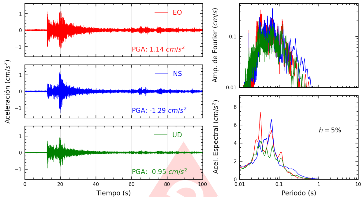
Figura A.29: Registros tiempo-historia, espectros de Fourier y de respuesta en las direcciones EO, NS y vertical de la estación BORJA. Sismo de Chilca, Cañete - Lima del 2023-11-01, 07:49:31 (Hora local)
