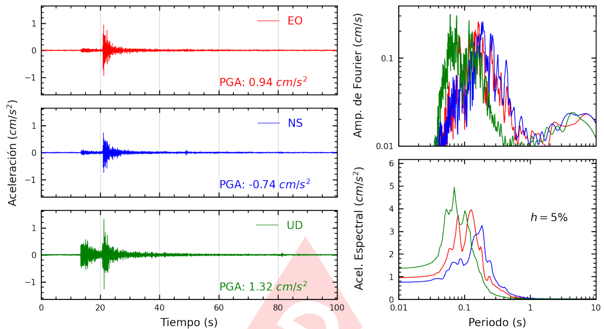
Figura A.27: Registros tiempo-historia, espectros de Fourier y de respuesta en las direcciones EO, NS y vertical de la estación ACAPU. Sismo de Chilca, Cañete - Lima del 2023-11-01, 07:49:31 (Hora local)
