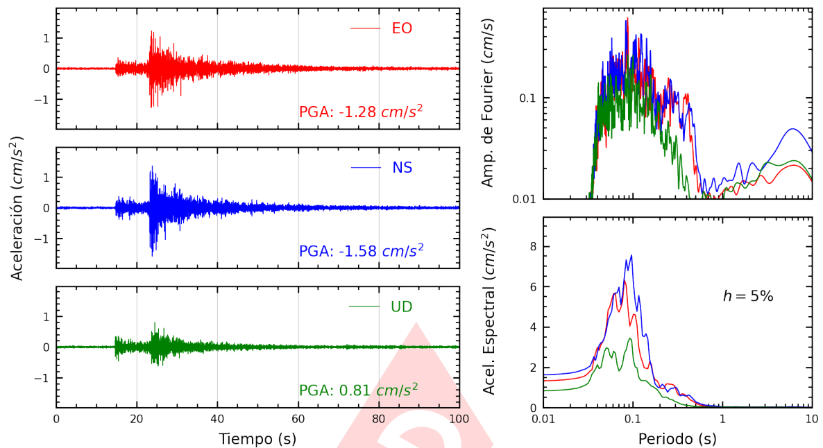
Figura A.21: Registros tiempo-historia, espectros de Fourier y de respuesta en las direcciones EO, NS y vertical de la estación DEFEN. Sismo de Chilca, Cañete - Lima del 2023-11-01, 07:49:31 (Hora local)
