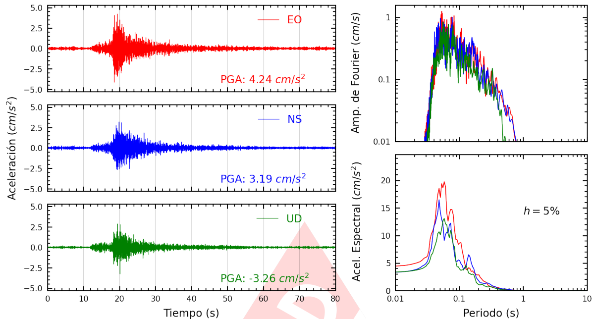
Figura A.3: Registros tiempo-historia, espectros de Fourier y de respuesta en las direcciones EO, NS y vertical de la estación UNTEL. Sismo de Chilca, Cañete - Lima del 2023-11-01, 07:49:31 (Hora local)
