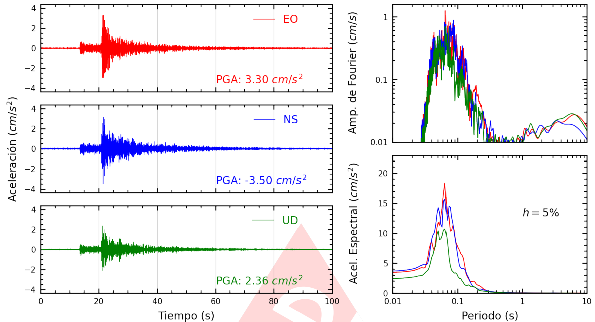
Figura A.5: Registros tiempo-historia, espectros de Fourier y de respuesta en las direcciones EO, NS y vertical de la estación JOSEO. Sismo de Chilca, Cañete - Lima del 2023-11-01, 07:49:31 (Hora local)
