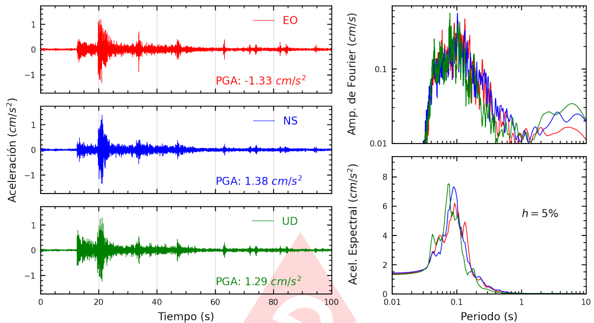
Figura A.25: Registros tiempo-historia, espectros de Fourier y de respuesta en las direcciones EO, NS y vertical de la estación PRADO. Sismo de Chilca, Cañete - Lima del 2023-11-01, 07:49:31 (Hora local)
