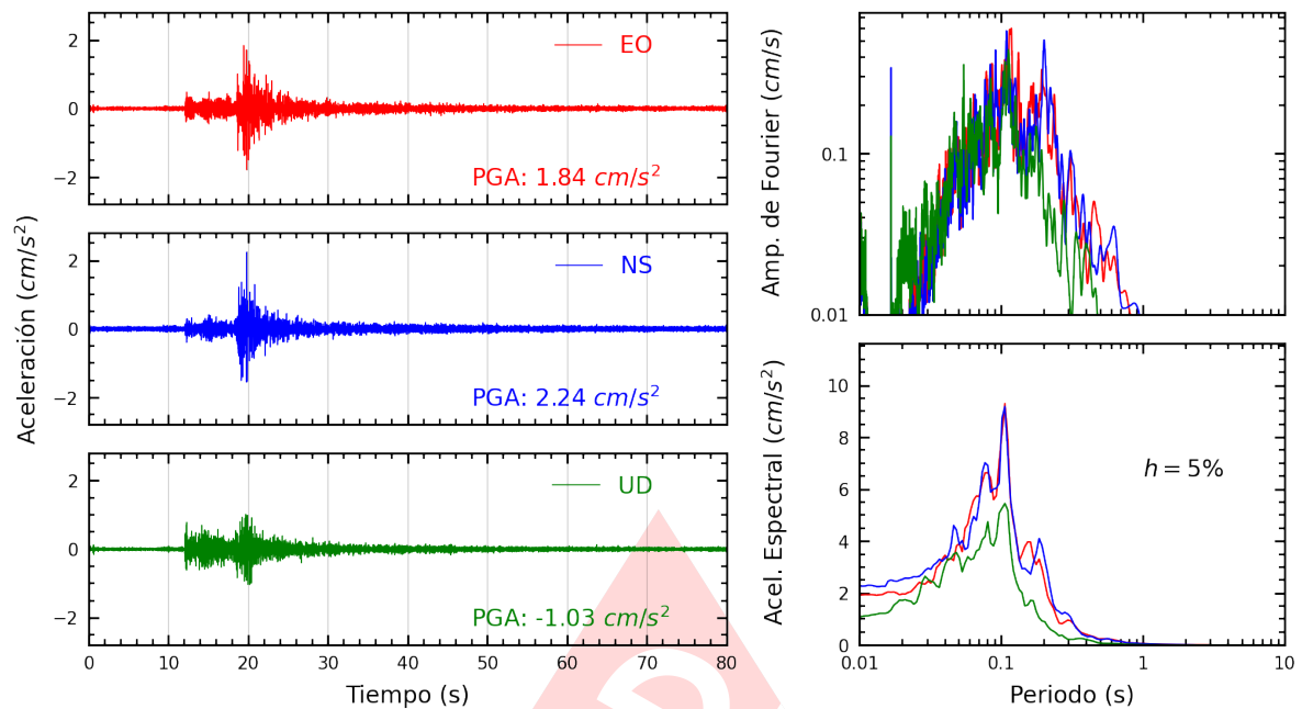
Figura A.13: Registros tiempo-historia, espectros de Fourier y de respuesta en las direcciones EO, NS y vertical de la estación SCCHO. Sismo de Chilca, Cañete - Lima del 2023-11-01, 07:49:31 (Hora local)
