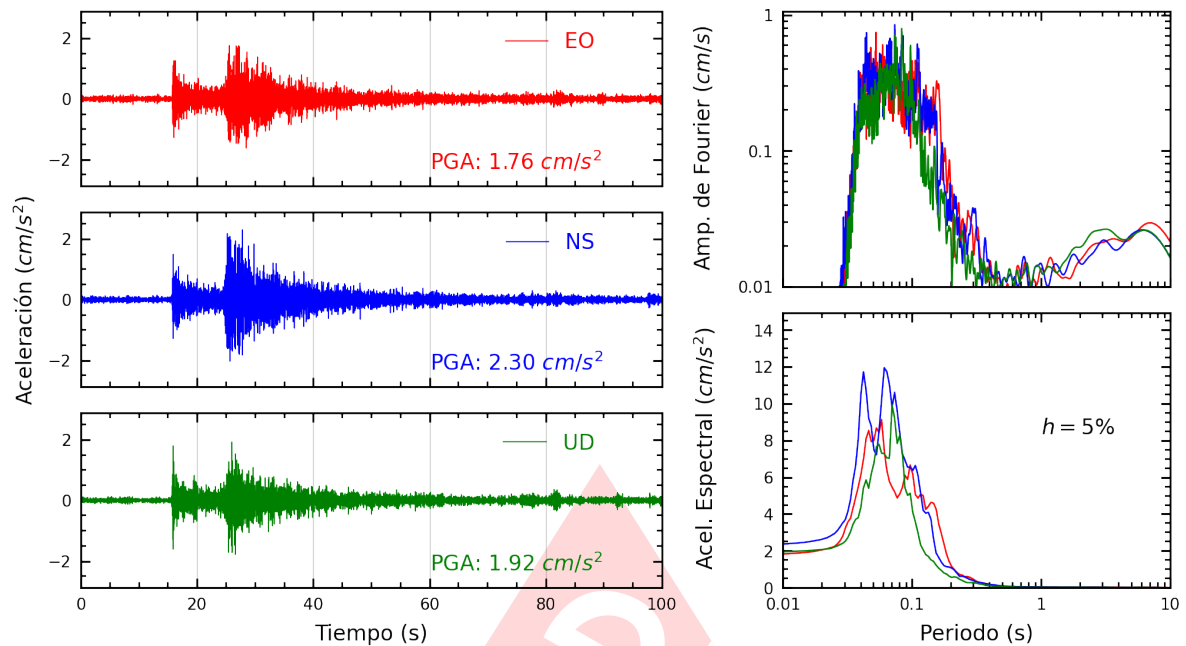
Figura A.11: Registros tiempo-historia, espectros de Fourier y de respuesta en las direcciones EO, NS y vertical de la estación SROSA. Sismo de Chilca, Cañete - Lima del 2023-11-01, 07:49:31 (Hora local)
