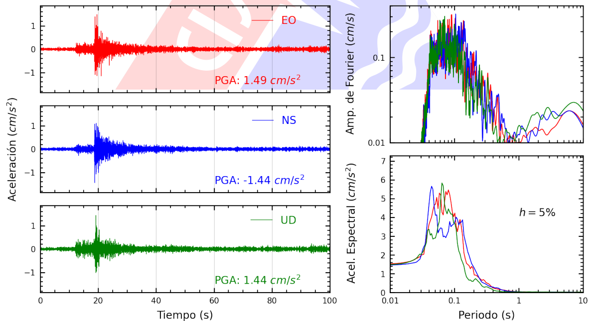
Figura A.22: Registros tiempo-historia, espectros de Fourier y de respuesta en las direcciones EO, NS y vertical de la estación URPPE. Sismo de Chilca, Cañete - Lima del 2023-11-01, 07:49:31 (Hora local)
