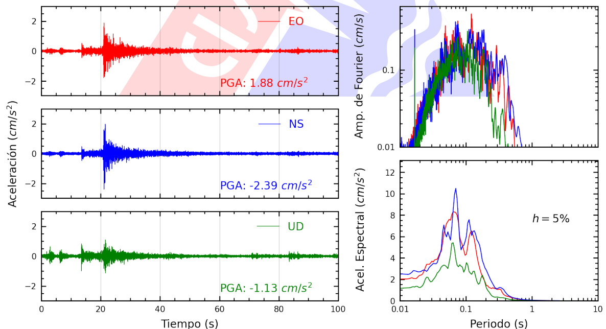
Figura A.10: Registros tiempo-historia, espectros de Fourier y de respuesta en las direcciones EO, NS y vertical de la estación SCOLI. Sismo de Chilca, Cañete - Lima del 2023-11-01, 07:49:31 (Hora local)
