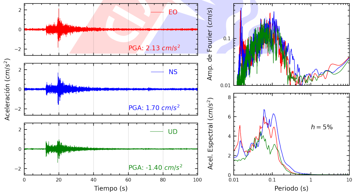
Figura A.14: Registros tiempo-historia, espectros de Fourier y de respuesta en las direcciones EO, NS y vertical de la estación CENEP. Sismo de Chilca, Cañete - Lima del 2023-11-01, 07:49:31 (Hora local)
