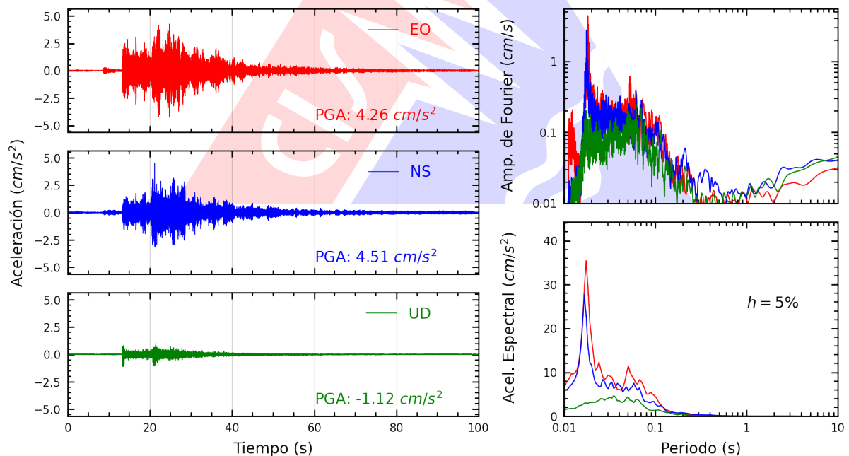
Figura A.2: Registros tiempo-historia, espectros de Fourier y de respuesta en las direcciones EO, NS y vertical de la estación UCSS. Sismo de Chilca, Cañete - Lima del 2023-11-01, 07:49:31 (Hora local)
