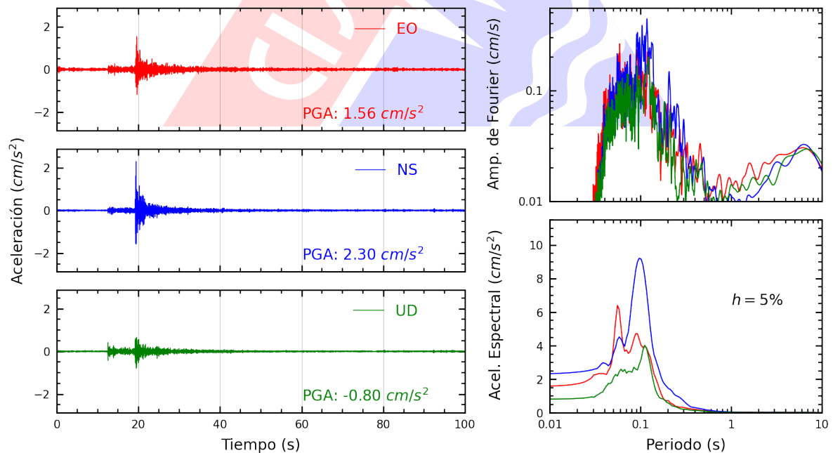
Figura A.12: Registros tiempo-historia, espectros de Fourier y de respuesta en las direcciones EO, NS y vertical de la estación INICT. Sismo de Chilca, Cañete - Lima del 2023-11-01, 07:49:31 (Hora local)
