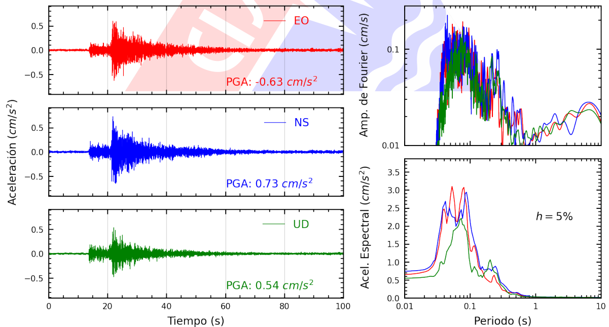
Figura A.36: Registros tiempo-historia, espectros de Fourier y de respuesta en las direcciones EO, NS y vertical de la estación COMAS. Sismo de Chilca, Cañete - Lima del 2023-11-01, 07:49:31 (Hora local)
