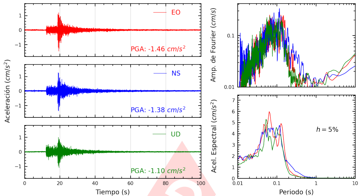
Figura A.23: Registros tiempo-historia, espectros de Fourier y de respuesta en las direcciones EO, NS y vertical de la estación SERVI. Sismo de Chilca, Cañete - Lima del 2023-11-01, 07:49:31 (Hora local)
