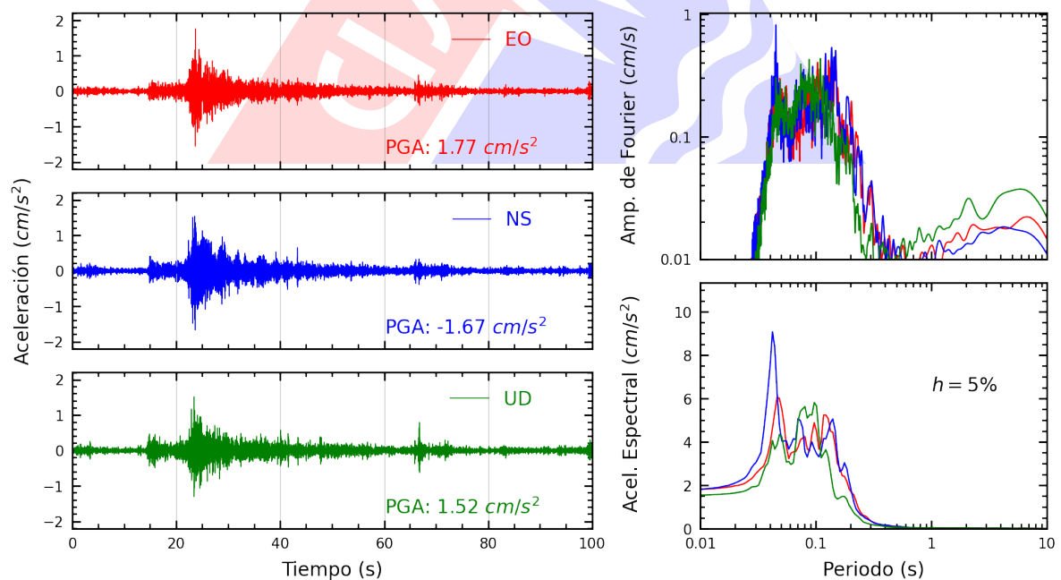
Figura A.16: Registros tiempo-historia, espectros de Fourier y de respuesta en las direcciones EO, NS y vertical de la estación CARAB. Sismo de Chilca, Cañete - Lima del 2023-11-01, 07:49:31 (Hora local)
