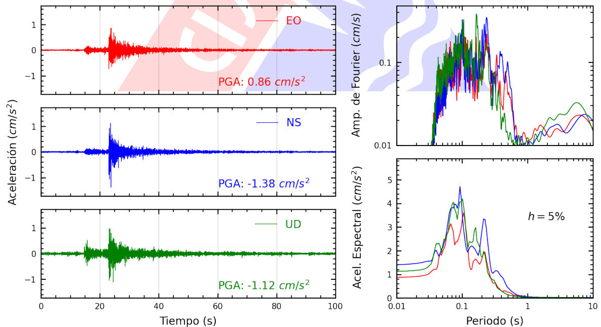
Figura A.26: Registros tiempo-historia, espectros de Fourier y de respuesta en las direcciones EO, NS y vertical de la estación MDPP. Sismo de Chilca, Cañete - Lima del 2023-11-01, 07:49:31 (Hora local)
