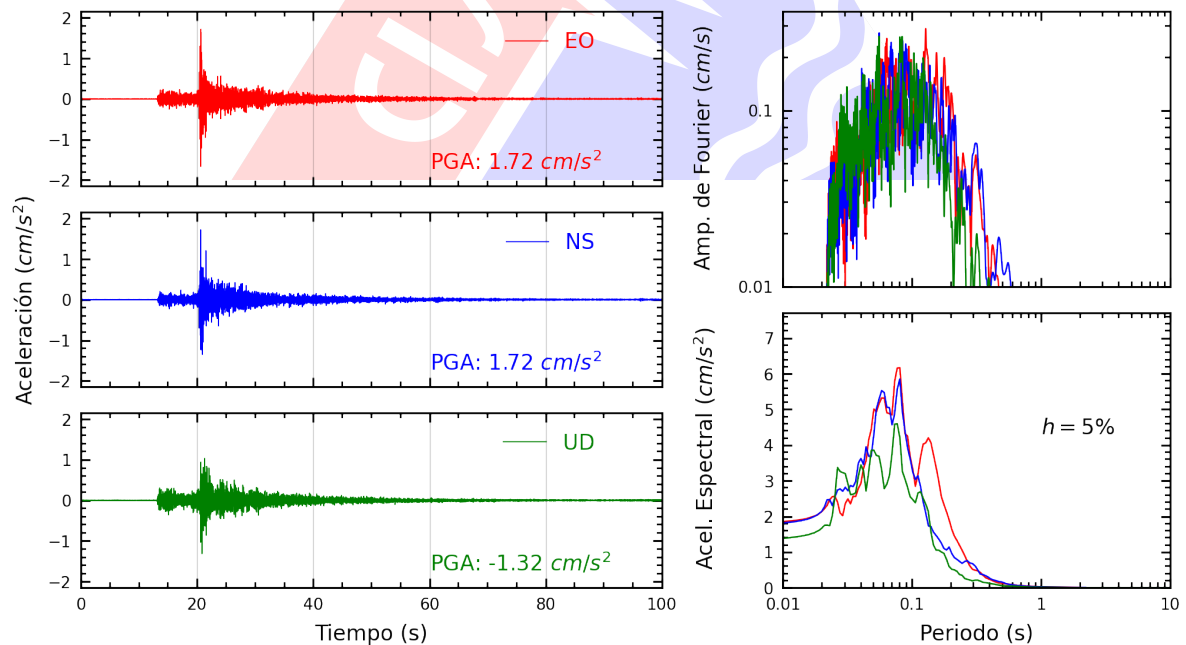
Figura A.18: Registros tiempo-historia, espectros de Fourier y de respuesta en las direcciones EO, NS y vertical de la estación JALV2. Sismo de Chilca, Cañete - Lima del 2023-11-01, 07:49:31 (Hora local)
