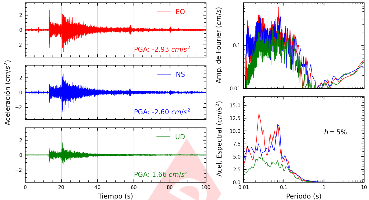
Figura A.7: Registros tiempo-historia, espectros de Fourier y de respuesta en las direcciones EO, NS y vertical de la estación FICPE. Sismo de Chilca, Cañete - Lima del 2023-11-01, 07:49:31 (Hora local)
