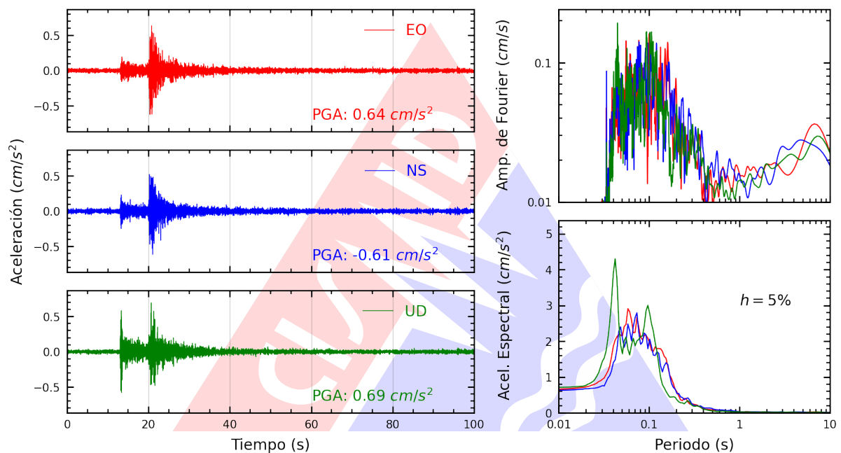
Figura A.37: Registros tiempo-historia, espectros de Fourier y de respuesta en las direcciones EO, NS y vertical de la estación BONDY. Sismo de Chilca, Cañete - Lima del 2023-11-01, 07:49:31 (Hora local)
