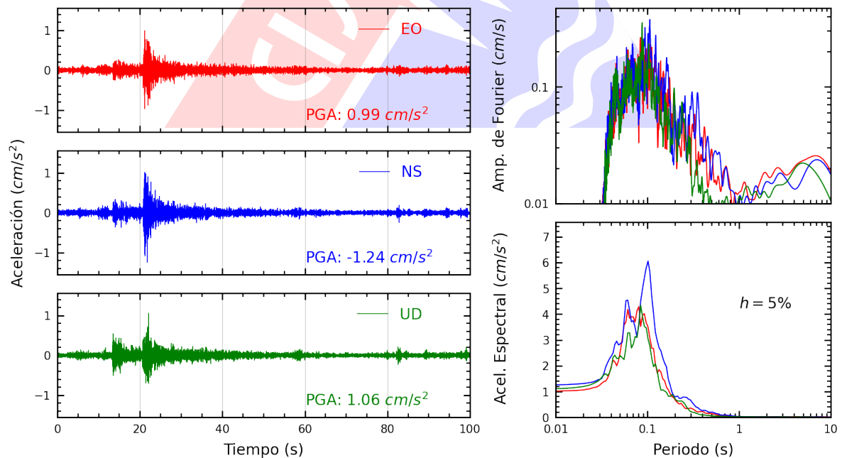
Figura A.30: Registros tiempo-historia, espectros de Fourier y de respuesta en las direcciones EO, NS y vertical de la estación MADRE. Sismo de Chilca, Cañete - Lima del 2023-11-01, 07:49:31 (Hora local)
