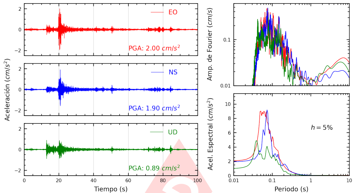
Figura A.15: Registros tiempo-historia, espectros de Fourier y de respuesta en las direcciones EO, NS y vertical de la estación UPCSM. Sismo de Chilca, Cañete - Lima del 2023-11-01, 07:49:31 (Hora local)
