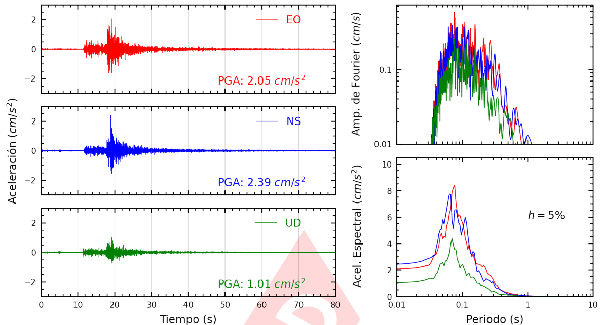
Figura A.9: Registros tiempo-historia, espectros de Fourier y de respuesta en las direcciones EO, NS y vertical de la estación BRISA. Sismo de Chilca, Cañete - Lima del 2023-11-01, 07:49:31 (Hora local)
