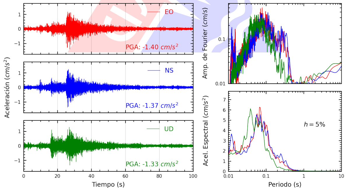
Figura A.24: Registros tiempo-historia, espectros de Fourier y de respuesta en las direcciones EO, NS y vertical de la estación ANCON. Sismo de Chilca, Cañete - Lima del 2023-11-01, 07:49:31 (Hora local)
