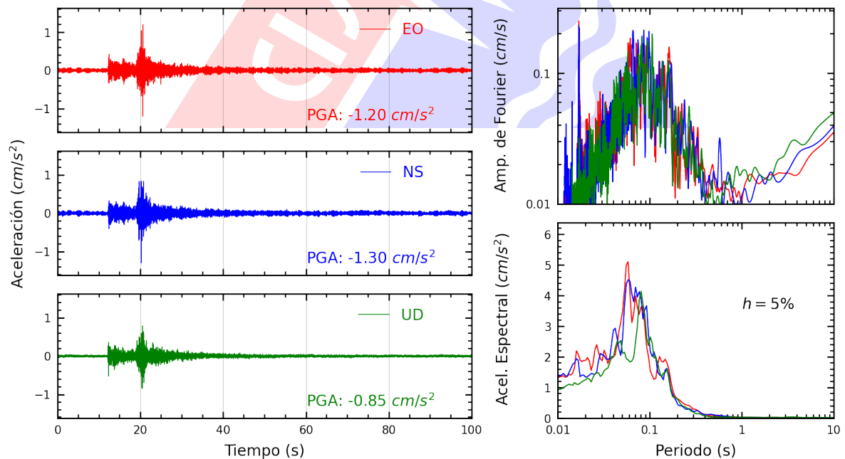
Figura A.28: Registros tiempo-historia, espectros de Fourier y de respuesta en las direcciones EO, NS y vertical de la estación UNMSM. Sismo de Chilca, Cañete - Lima del 2023-11-01, 07:49:31 (Hora local)
