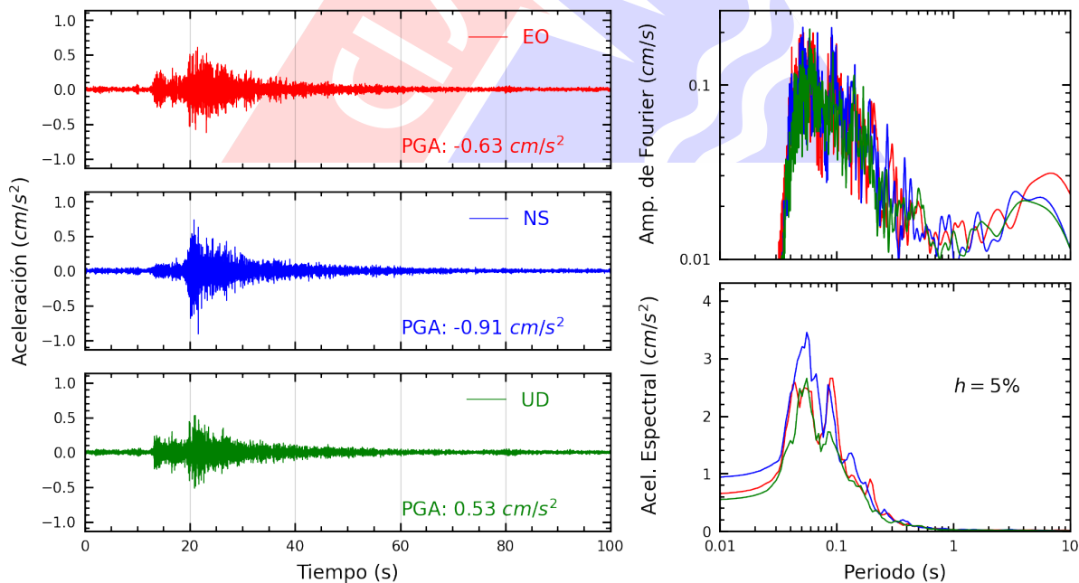
Figura A.34: Registros tiempo-historia, espectros de Fourier y de respuesta en las direcciones EO, NS y vertical de la estación IMCA. Sismo de Chilca, Cañete - Lima del 2023-11-01, 07:49:31 (Hora local)
