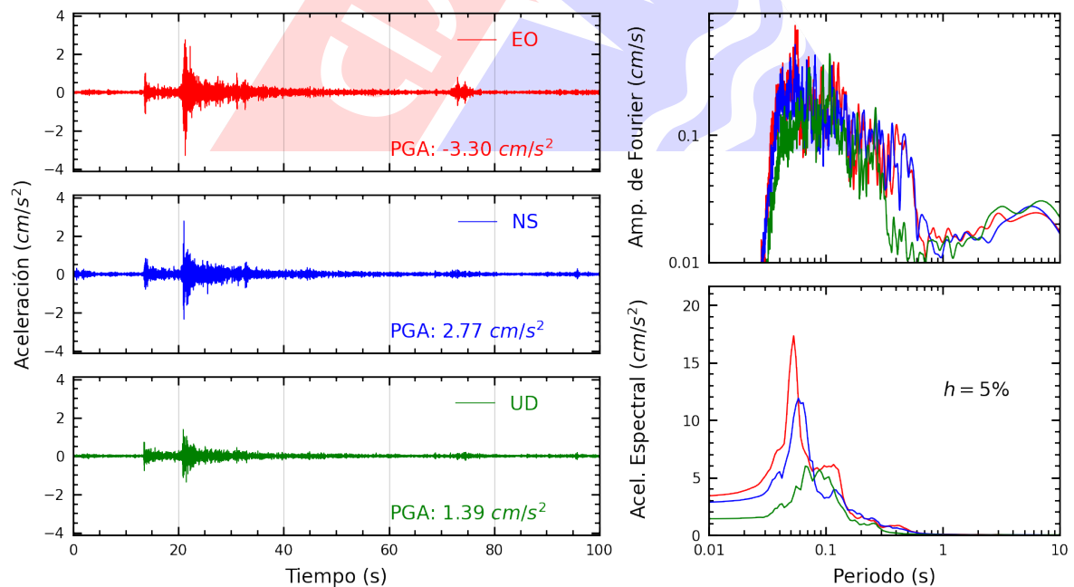
Figura A.6: Registros tiempo-historia, espectros de Fourier y de respuesta en las direcciones EO, NS y vertical de la estación OLIVO. Sismo de Chilca, Cañete - Lima del 2023-11-01, 07:49:31 (Hora local)
