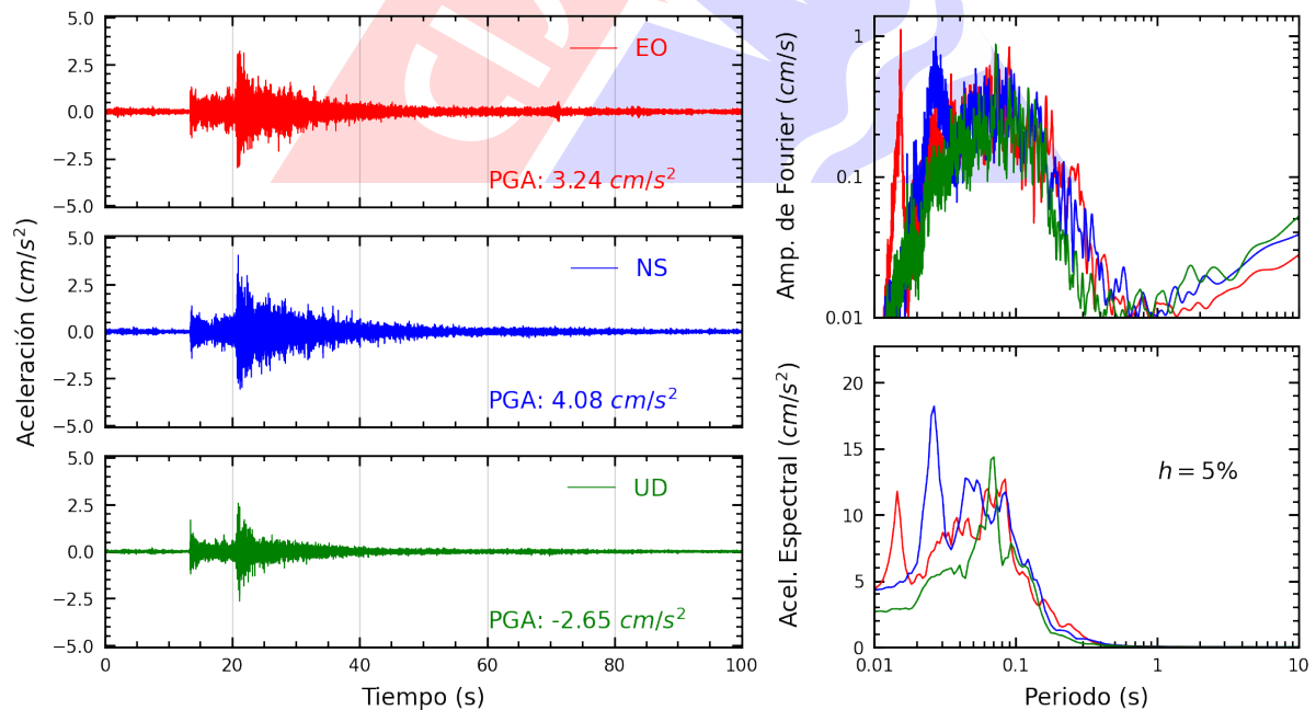
Figura A.4: Registros tiempo-historia, espectros de Fourier y de respuesta en las direcciones EO, NS y vertical de la estación INDEP. Sismo de Chilca, Cañete - Lima del 2023-11-01, 07:49:31 (Hora local)
