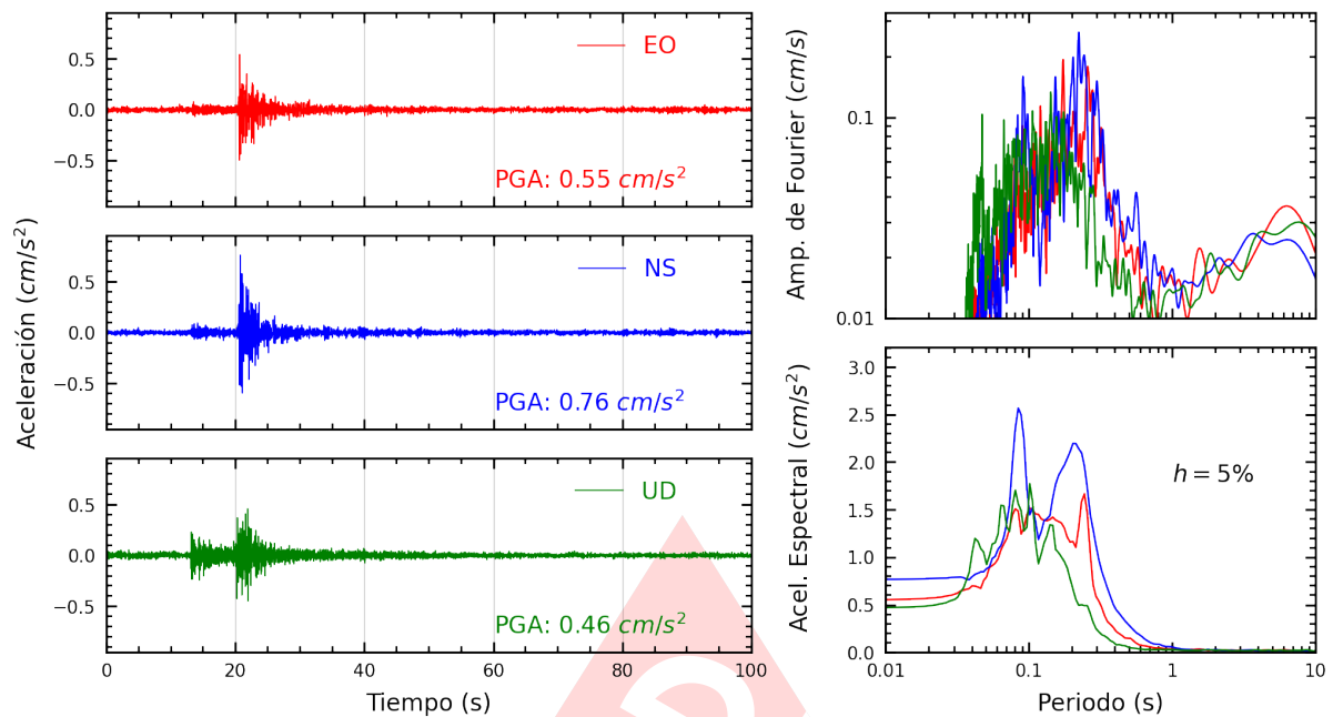
Figura A.35: Registros tiempo-historia, espectros de Fourier y de respuesta en las direcciones EO, NS y vertical de la estación DSMI. Sismo de Chilca, Cañete - Lima del 2023-11-01, 07:49:31 (Hora local)
