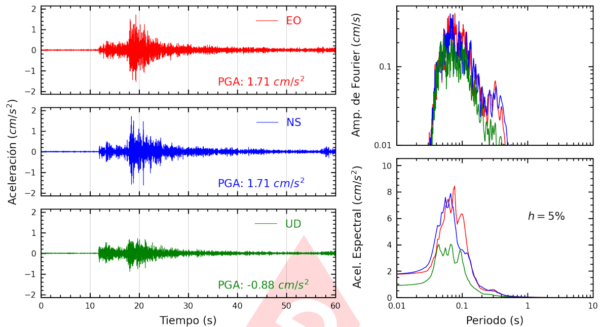
Figura A.19: Registros tiempo-historia, espectros de Fourier y de respuesta en las direcciones EO, NS y vertical de la estación PACHA. Sismo de Chilca, Cañete - Lima del 2023-11-01, 07:49:31 (Hora local)
