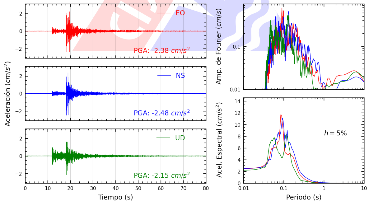
Figura A.8: Registros tiempo-historia, espectros de Fourier y de respuesta en las direcciones EO, NS y vertical de la estación USILP. Sismo de Chilca, Cañete - Lima del 2023-11-01, 07:49:31 (Hora local)
