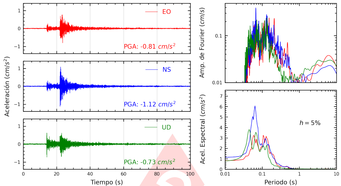
Figura A.31: Registros tiempo-historia, espectros de Fourier y de respuesta en las direcciones EO, NS y vertical de la estación VHAYA. Sismo de Chilca, Cañete - Lima del 2023-11-01, 07:49:31 (Hora local)
