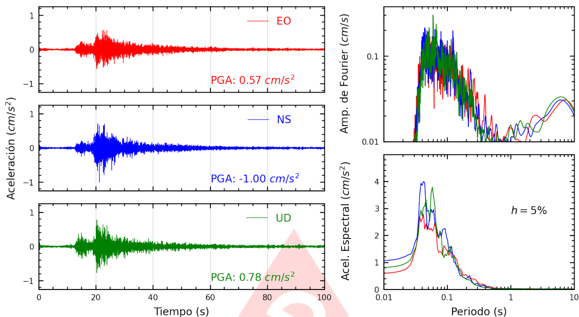
Figura A.33: Registros tiempo-historia, espectros de Fourier y de respuesta en las direcciones EO, NS y vertical de la estación USMP. Sismo de Chilca, Cañete - Lima del 2023-11-01, 07:49:31 (Hora local)
