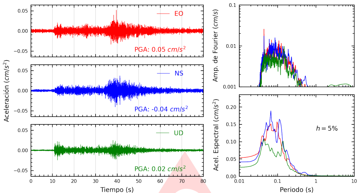
Figura A.1: Registros tiempo-historia, espectros de Fourier y de respuesta en las direcciones EO, NS y vertical de la estación UNSA. Sismo de Chivay, Caylloma - Arequipa del 2023-11-16, 17:07:54 (Hora local)
