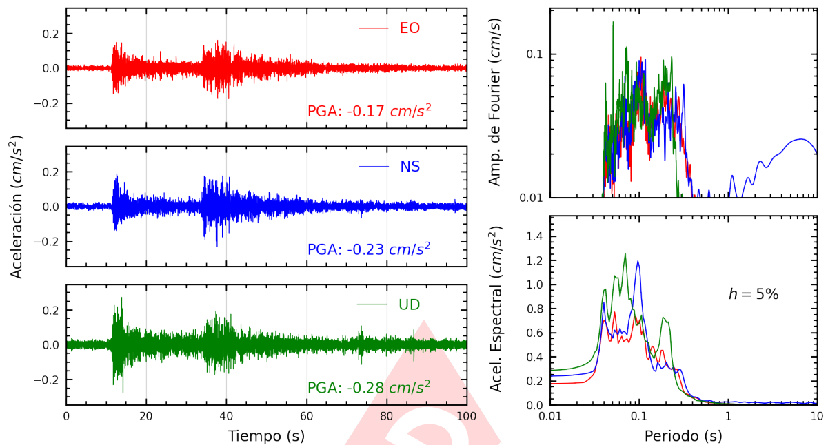
Figura A.5: Registros tiempo-historia, espectros de Fourier y de respuesta en las direcciones EO, NS y vertical de la estación SCTAC. Sismo de La Capilla, General Sanchez Cerro - Moquegua del 2023-11-28, 00:04:25 (Hora local)
