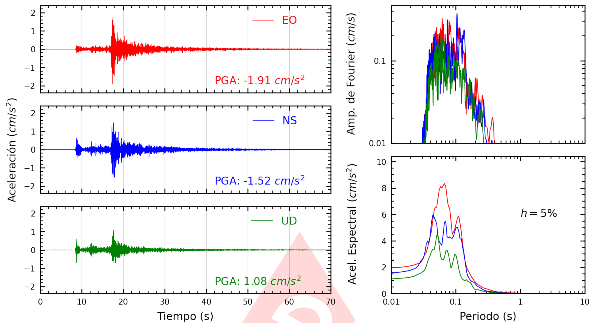
Figura A.3: Registros tiempo-historia, espectros de Fourier y de respuesta en las direcciones EO, NS y vertical de la estación UNSA. Sismo de La Capilla, General Sanchez Cerro - Moquegua del 2023-11-28, 00:04:25 (Hora local)
