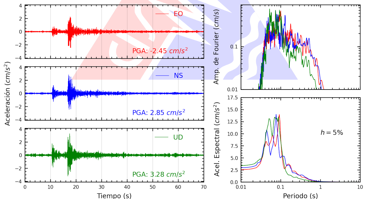
Figura A.2: Registros tiempo-historia, espectros de Fourier y de respuesta en las direcciones EO, NS y vertical de la estación SCAR2. Sismo de La Capilla, General Sanchez Cerro - Moquegua del 2023-11-28, 00:04:25 (Hora local)
