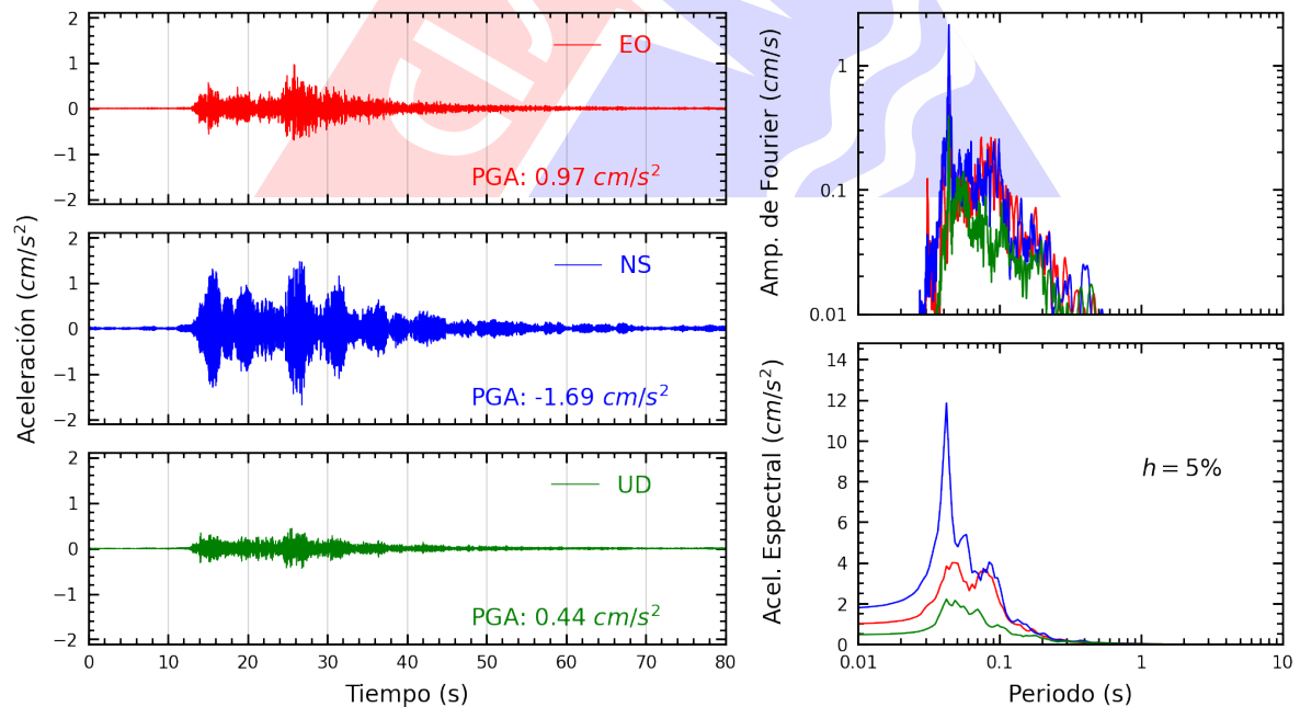
Figura A.4: Registros tiempo-historia, espectros de Fourier y de respuesta en las direcciones EO, NS y vertical de la estación UNAM. Sismo de La Capilla, General Sanchez Cerro - Moquegua del 2023-11-28, 00:04:25 (Hora local)
