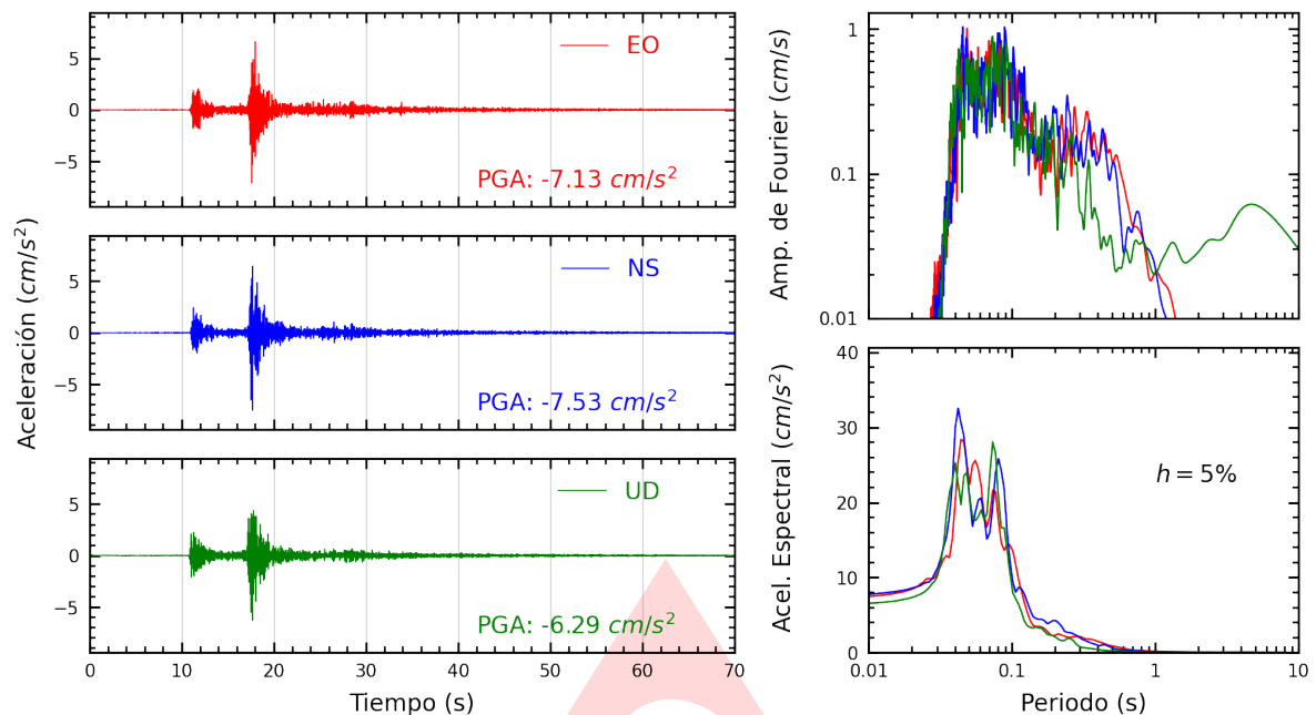
Figura A.1: Registros tiempo-historia, espectros de Fourier y de respuesta en las direcciones EO, NS y vertical de la estación SCARQ. Sismo de La Capilla, General Sanchez Cerro - Moquegua del 2023-11-28, 00:04:25 (Hora local)
