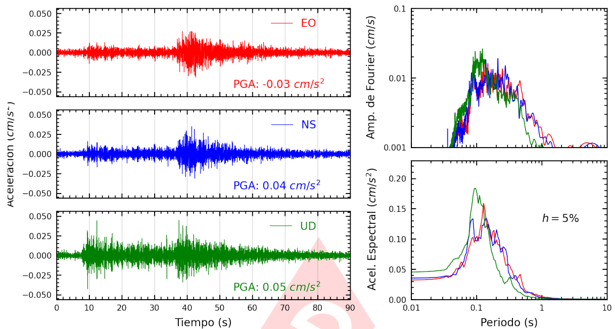
Figura A.3: Registros tiempo-historia, espectros de Fourier y de respuesta en las direcciones EO, NS y vertical de la estación UNIA. Sismo de Huancabamba, Oxapampa - Pasco del 2023-12-08, 07:17:16 (Hora local)
