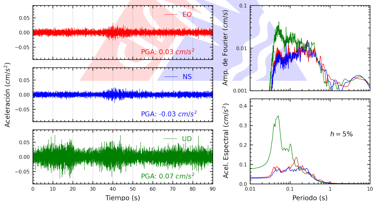
Figura A.2: Registros tiempo-historia, espectros de Fourier y de respuesta en las direcciones EO, NS y vertical de la estación SCPUC. Sismo de Huancabamba, Oxapampa - Pasco del 2023-12-08, 07:17:16 (Hora local)
