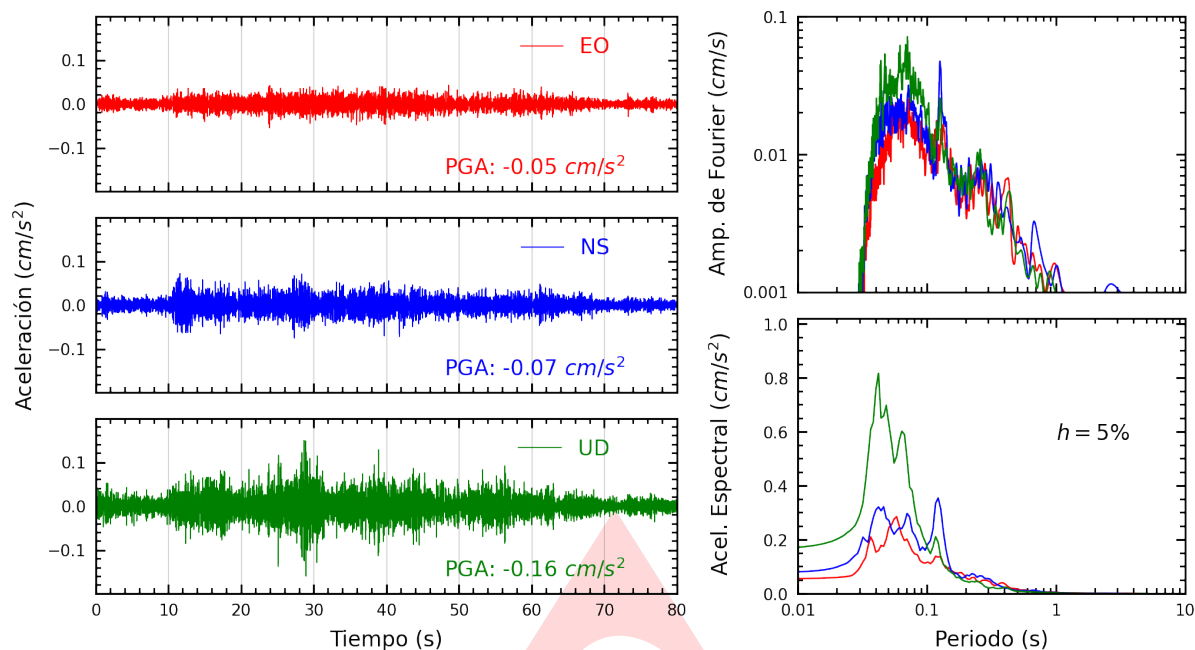
Figura A.1: Registros tiempo-historia, espectros de Fourier y de respuesta en las direcciones EO, NS y vertical de la estación SCHYO. Sismo de Huancabamba, Oxapampa - Pasco del 2023-12-08, 07:17:16 (Hora local)
