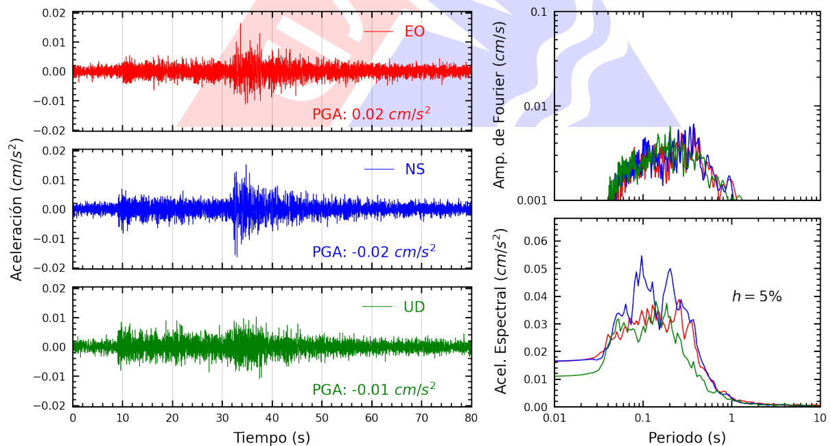
Figura A.4: Registros tiempo-historia, espectros de Fourier y de respuesta en las direcciones EO, NS y vertical de la estación UNCP. Sismo de Huancabamba, Oxapampa - Pasco del 2023-12-08, 07:17:16 (Hora local)
