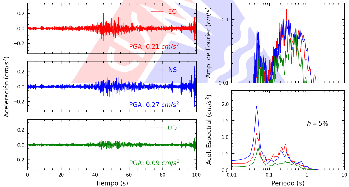
Figura A.2: Registros tiempo-historia, espectros de Fourier y de respuesta en las direcciones EO, NS y vertical de la estación BRISA. Sismo de Pisco, Pisco - Ica del 2023-12-10, 02:35:12 (Hora local)
