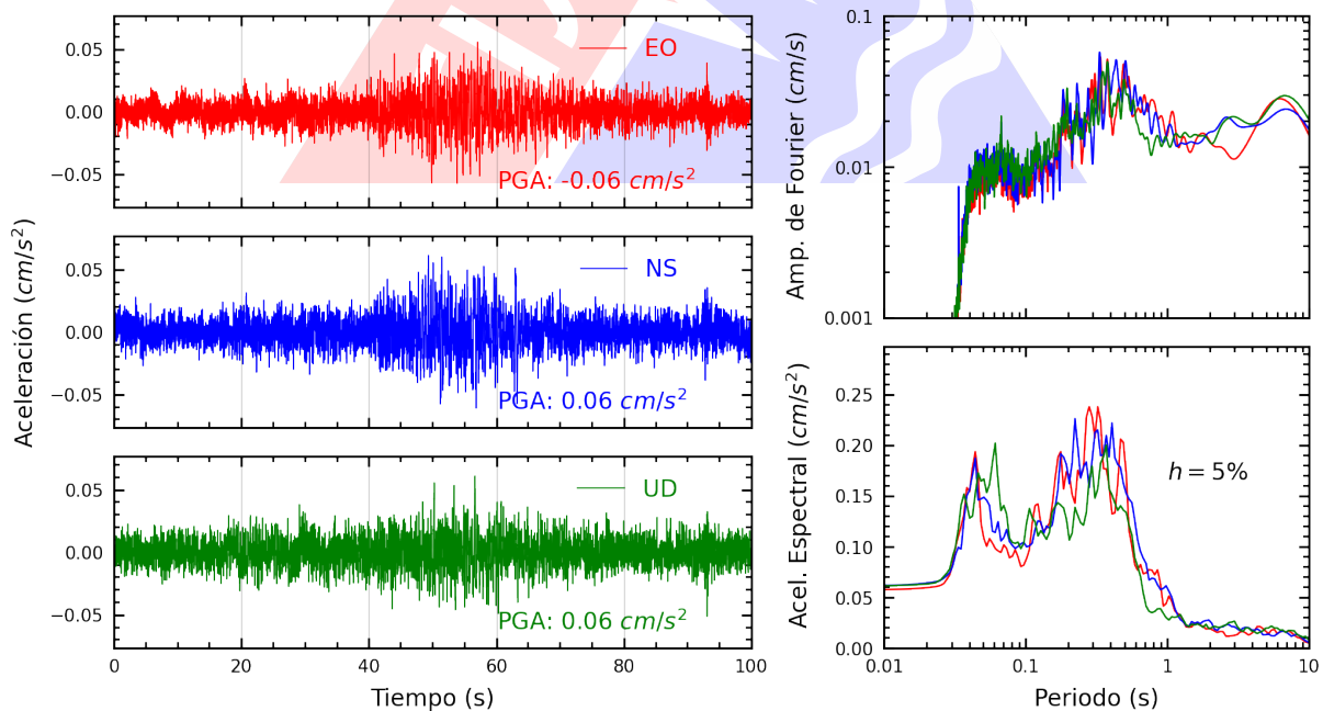
Figura A.10: Registros tiempo-historia, espectros de Fourier y de respuesta en las direcciones EO, NS y vertical de la estación UNFV. Sismo de Pisco, Pisco - Ica del 2023-12-10, 02:35:12 (Hora local)
