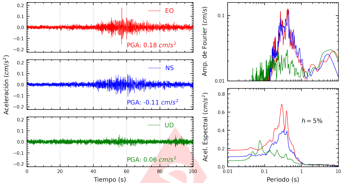
Figura A.5: Registros tiempo-historia, espectros de Fourier y de respuesta en las direcciones EO, NS y vertical de la estación ACAPU. Sismo de Pisco, Pisco - Ica del 2023-12-10, 02:35:12 (Hora local)
