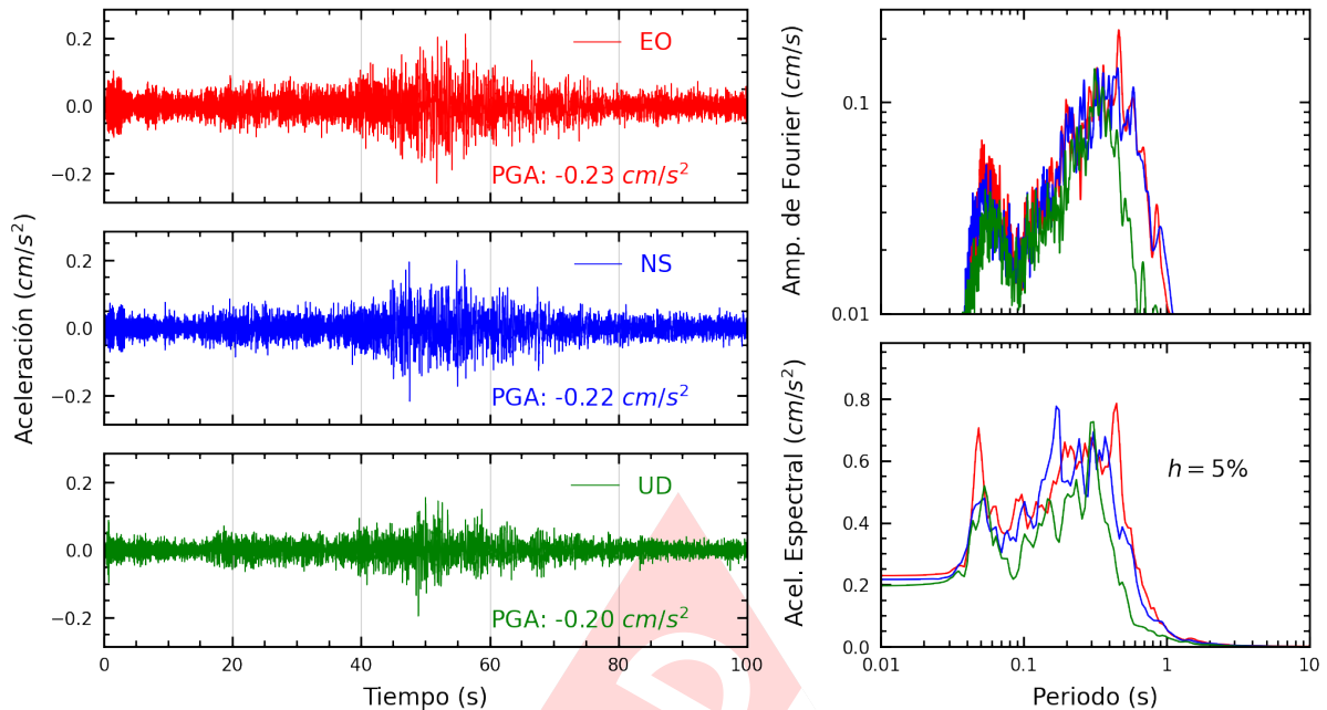
Figura A.3: Registros tiempo-historia, espectros de Fourier y de respuesta en las direcciones EO, NS y vertical de la estación UNTEL. Sismo de Pisco, Pisco - Ica del 2023-12-10, 02:35:12 (Hora local)
