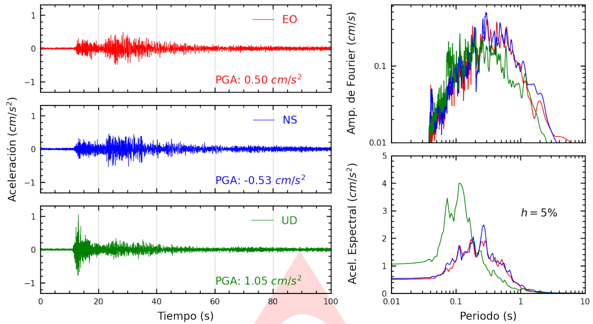
Figura A.1: Registros tiempo-historia, espectros de Fourier y de respuesta en las direcciones EO, NS y vertical de la estación UNICA. Sismo de Pisco, Pisco - Ica del 2023-12-10, 02:35:12 (Hora local)
