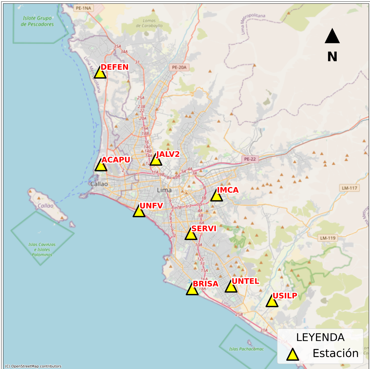
Figura 3: Mapa de ubicación de la(s) estación(es) acelerográfica(s) en Lima Metropolitana correspondiente(s) al Sismo de Pisco, Pisco - Ica del 10 de diciembre de 2023 a las 02:35:12 (hora local)
