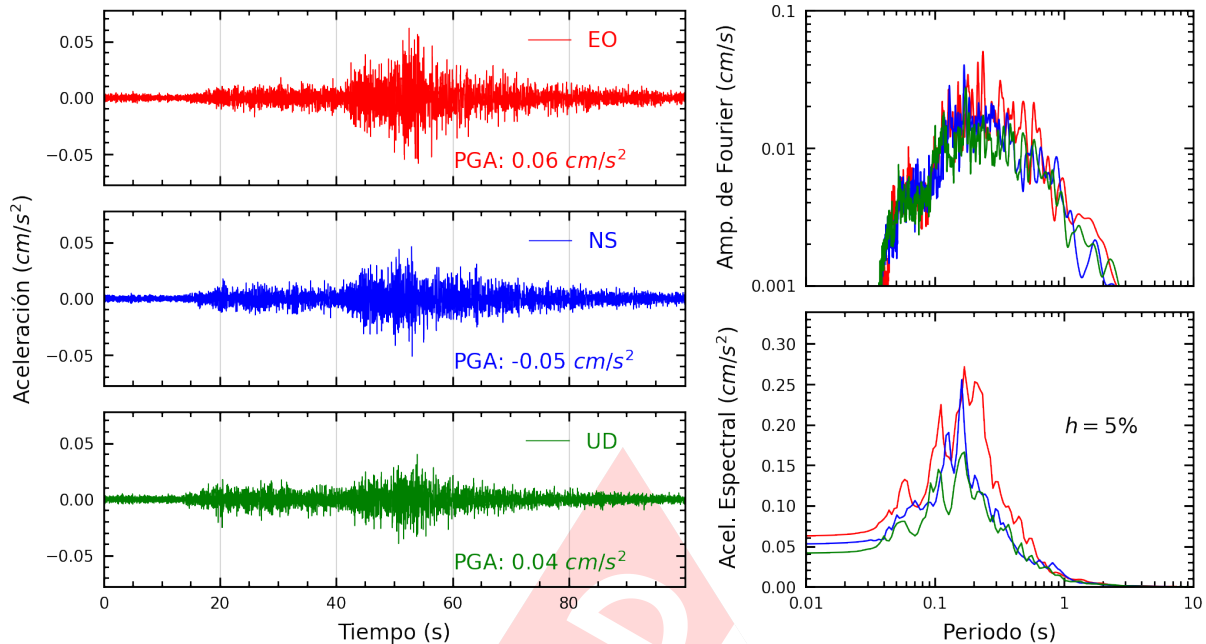
Figura A.9: Registros tiempo-historia, espectros de Fourier y de respuesta en las direcciones EO, NS y vertical de la estación JALV2. Sismo de Pisco, Pisco - Ica del 2023-12-10, 02:35:12 (Hora local)
