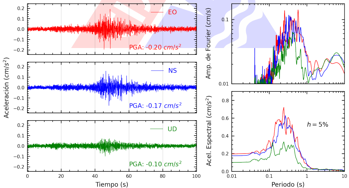
Figura A.4: Registros tiempo-historia, espectros de Fourier y de respuesta en las direcciones EO, NS y vertical de la estación USILP. Sismo de Pisco, Pisco - Ica del 2023-12-10, 02:35:12 (Hora local)
