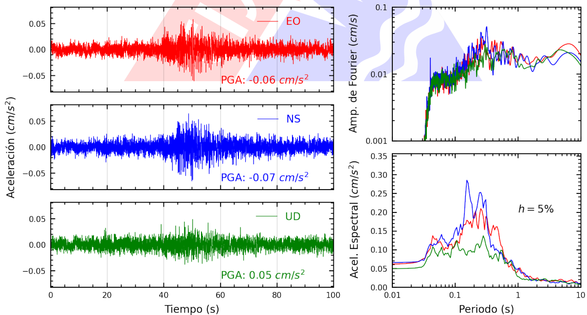
Figura A.8: Registros tiempo-historia, espectros de Fourier y de respuesta en las direcciones EO, NS y vertical de la estación SERVI. Sismo de Pisco, Pisco - Ica del 2023-12-10, 02:35:12 (Hora local)
