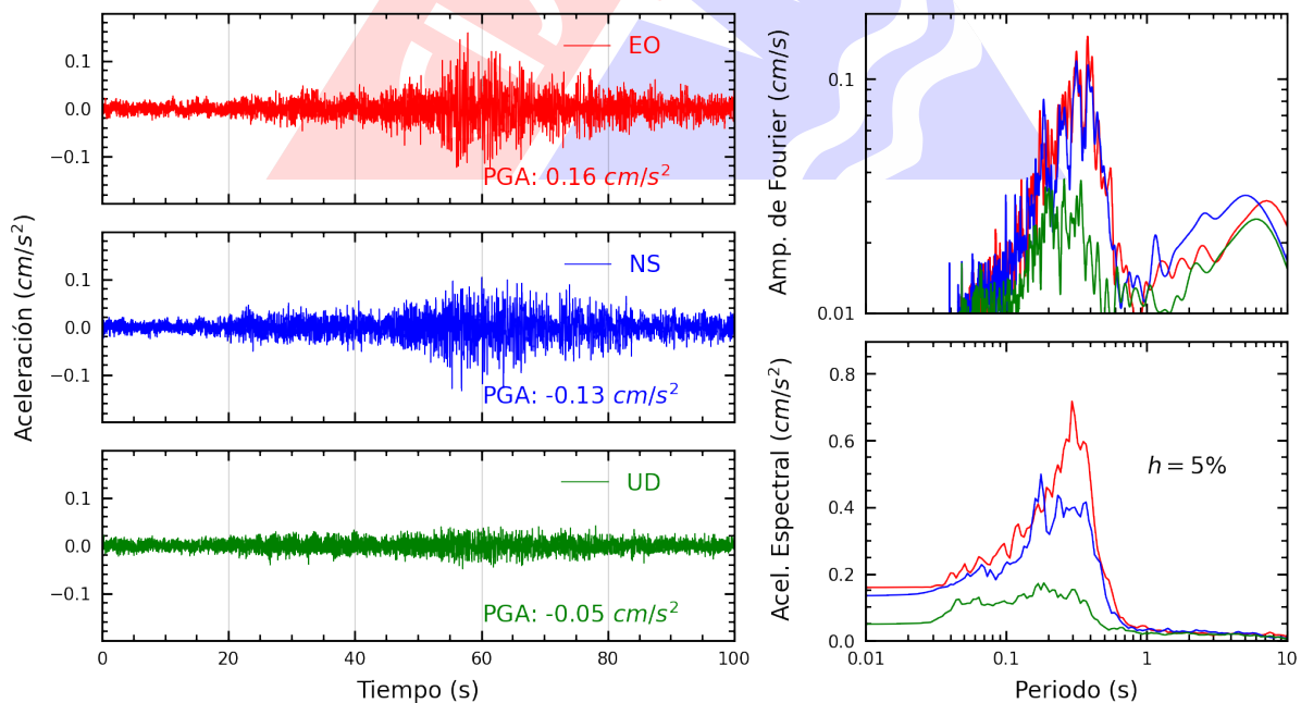
Figura A.6: Registros tiempo-historia, espectros de Fourier y de respuesta en las direcciones EO, NS y vertical de la estación DEFEN. Sismo de Pisco, Pisco - Ica del 2023-12-10, 02:35:12 (Hora local)
