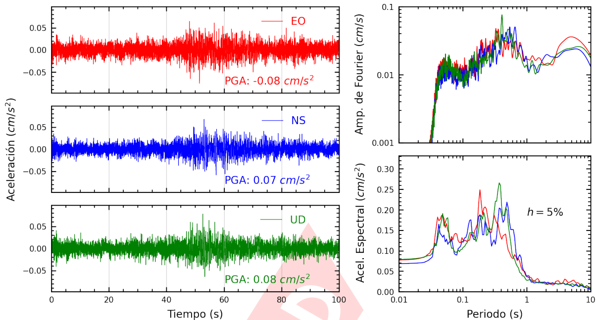
Figura A.7: Registros tiempo-historia, espectros de Fourier y de respuesta en las direcciones EO, NS y vertical de la estación IMCA. Sismo de Pisco, Pisco - Ica del 2023-12-10, 02:35:12 (Hora local)
