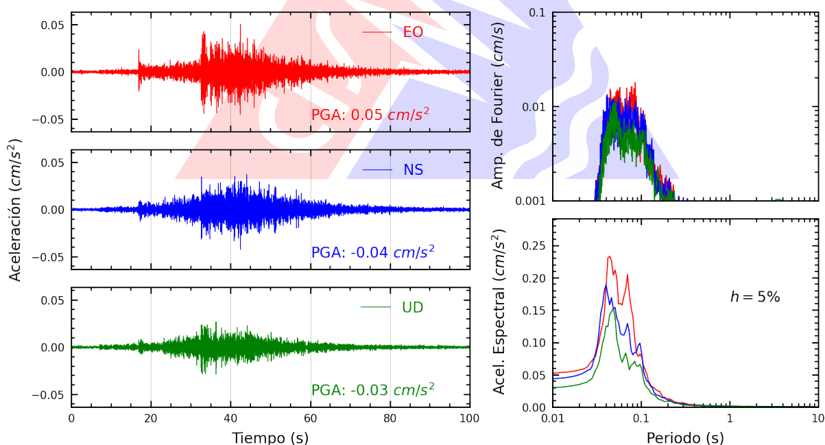
Figura A.2: Registros tiempo-historia, espectros de Fourier y de respuesta en las direcciones EO, NS y vertical de la estación UNSA. Sismo de La Capilla, General Sanchez Cerro - Moquegua del 2023-12-13, 20:53:58 (Hora local)
