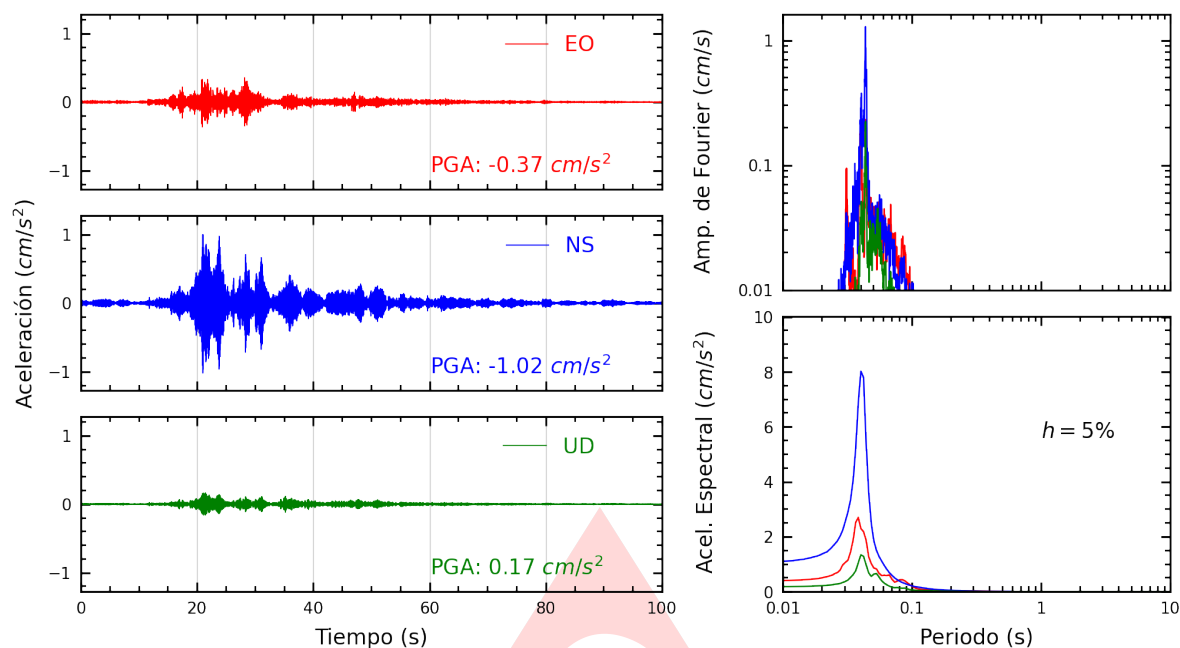
Figura A.1: Registros tiempo-historia, espectros de Fourier y de respuesta en las direcciones EO, NS y vertical de la estación UNAM. Sismo de La Capilla, General Sanchez Cerro - Moquegua del 2023-12-13, 20:53:58 (Hora local)
