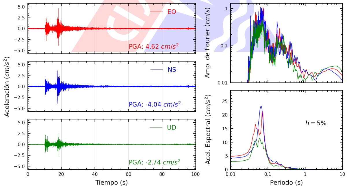
Figura A.16: Registros tiempo-historia, espectros de Fourier y de respuesta en las direcciones EO, NS y vertical de la estación UPCVI. Sismo de Provincia Constitucional del Callao , Callao - Lima del 2024-01-04, 12:42:39 (Hora local)
