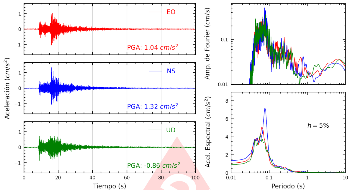
Figura A.35: Registros tiempo-historia, espectros de Fourier y de respuesta en las direcciones EO, NS y vertical de la estación UNMSM. Sismo de Provincia Constitucional del Callao , Callao - Lima del 2024-01-04, 12:42:39 (Hora local)
