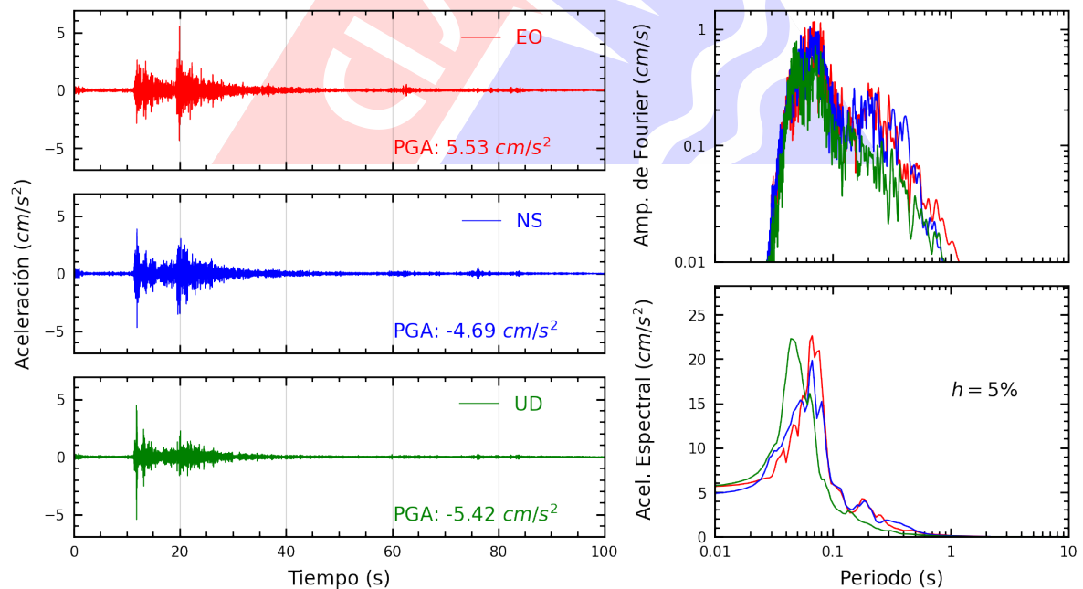
Figura A.14: Registros tiempo-historia, espectros de Fourier y de respuesta en las direcciones EO, NS y vertical de la estación PACHA. Sismo de Provincia Constitucional del Callao , Callao - Lima del 2024-01-04, 12:42:39 (Hora local)
