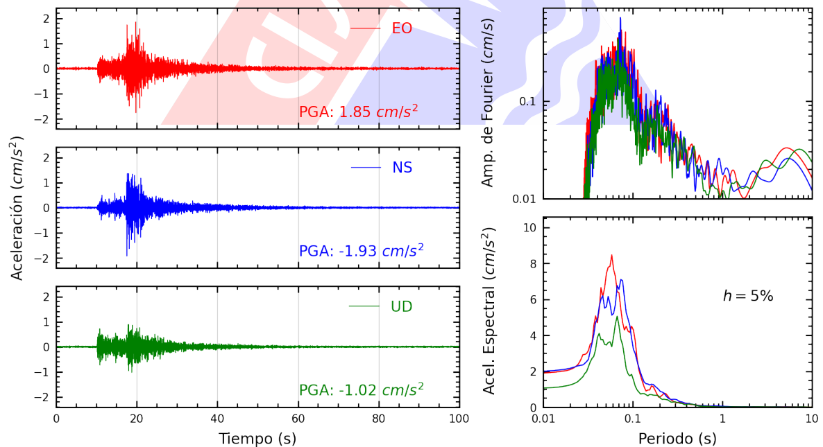
Figura A.32: Registros tiempo-historia, espectros de Fourier y de respuesta en las direcciones EO, NS y vertical de la estación INICT. Sismo de Provincia Constitucional del Callao , Callao - Lima del 2024-01-04, 12:42:39 (Hora local)
