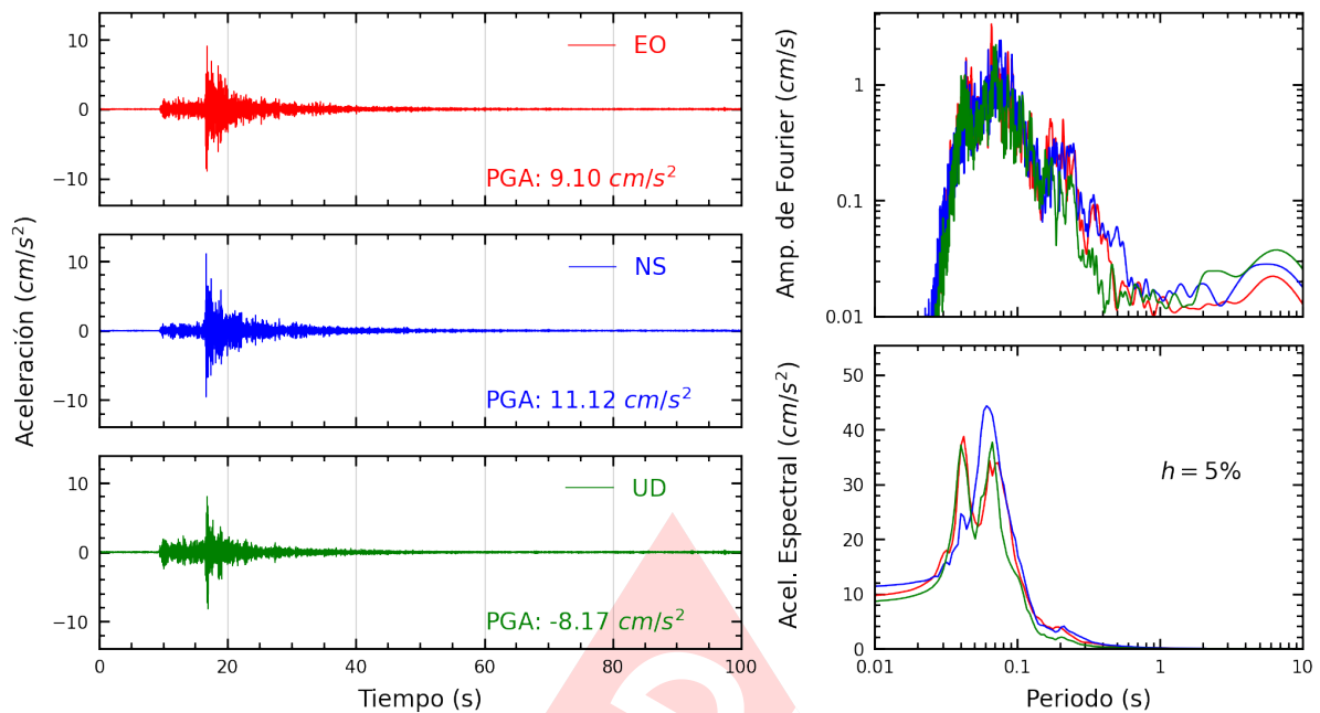
Figura A.5: Registros tiempo-historia, espectros de Fourier y de respuesta en las direcciones EO, NS y vertical de la estación INDEP. Sismo de Provincia Constitucional del Callao , Callao - Lima del 2024-01-04, 12:42:39 (Hora local)
