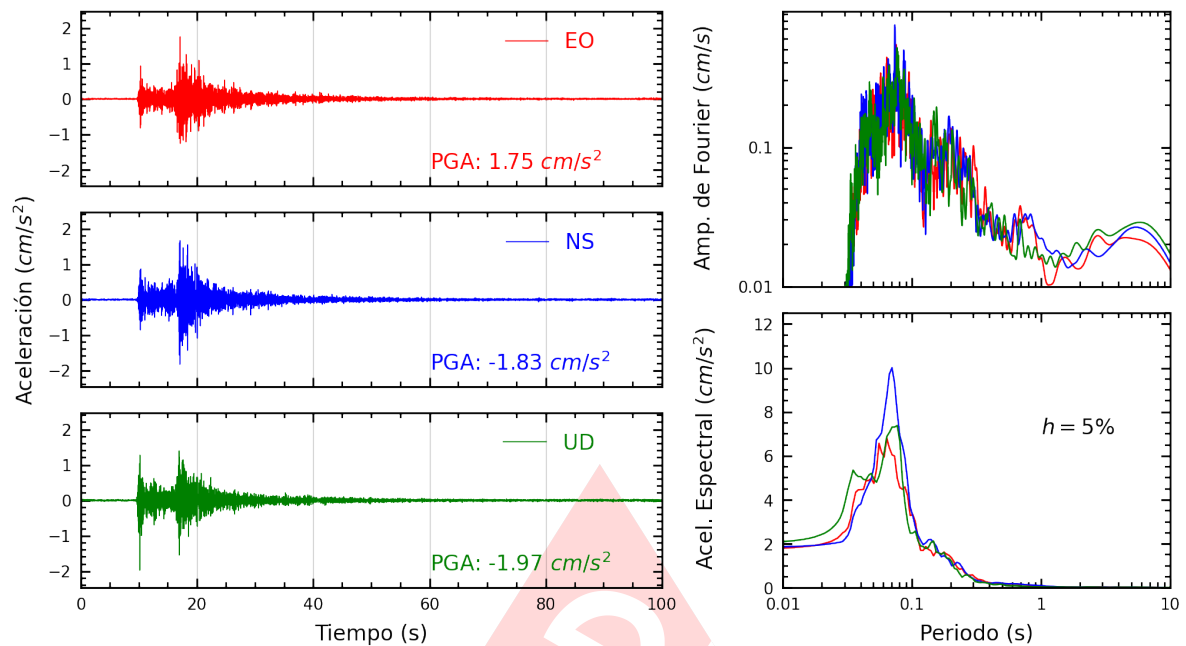
Figura A.31: Registros tiempo-historia, espectros de Fourier y de respuesta en las direcciones EO, NS y vertical de la estación UNFV. Sismo de Provincia Constitucional del Callao , Callao - Lima del 2024-01-04, 12:42:39 (Hora local)
