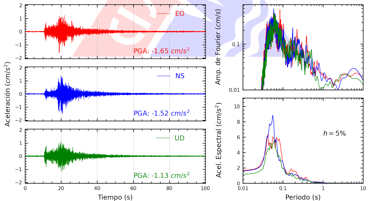
Figura A.34: Registros tiempo-historia, espectros de Fourier y de respuesta en las direcciones EO, NS y vertical de la estación IMCA. Sismo de Provincia Constitucional del Callao , Callao - Lima del 2024-01-04, 12:42:39 (Hora local)
