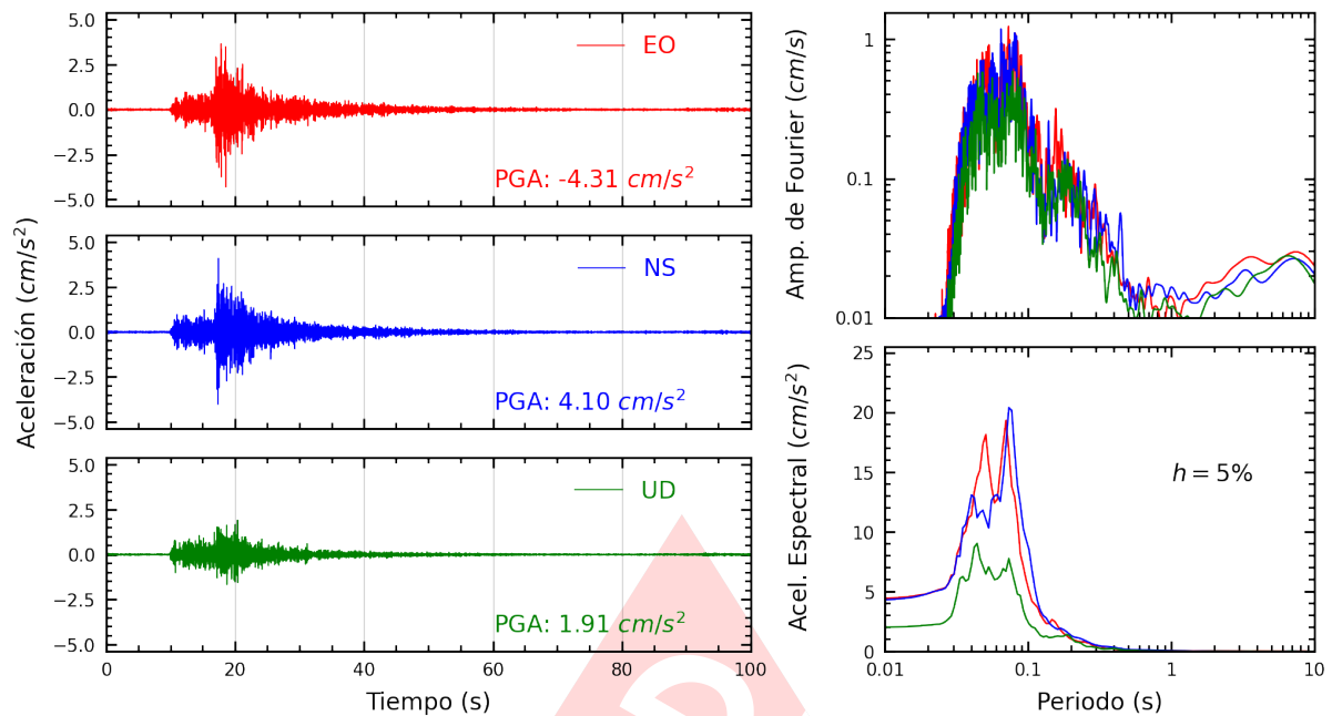
Figura A.17: Registros tiempo-historia, espectros de Fourier y de respuesta en las direcciones EO, NS y vertical de la estación FICPE. Sismo de Provincia Constitucional del Callao , Callao - Lima del 2024-01-04, 12:42:39 (Hora local)
