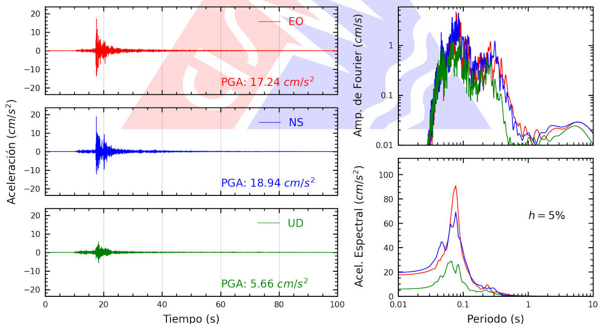
Figura A.2: Registros tiempo-historia, espectros de Fourier y de respuesta en las direcciones EO, NS y vertical de la estación DEFEN. Sismo de Provincia Constitucional del Callao , Callao - Lima del 2024-01-04, 12:42:39 (Hora local)
