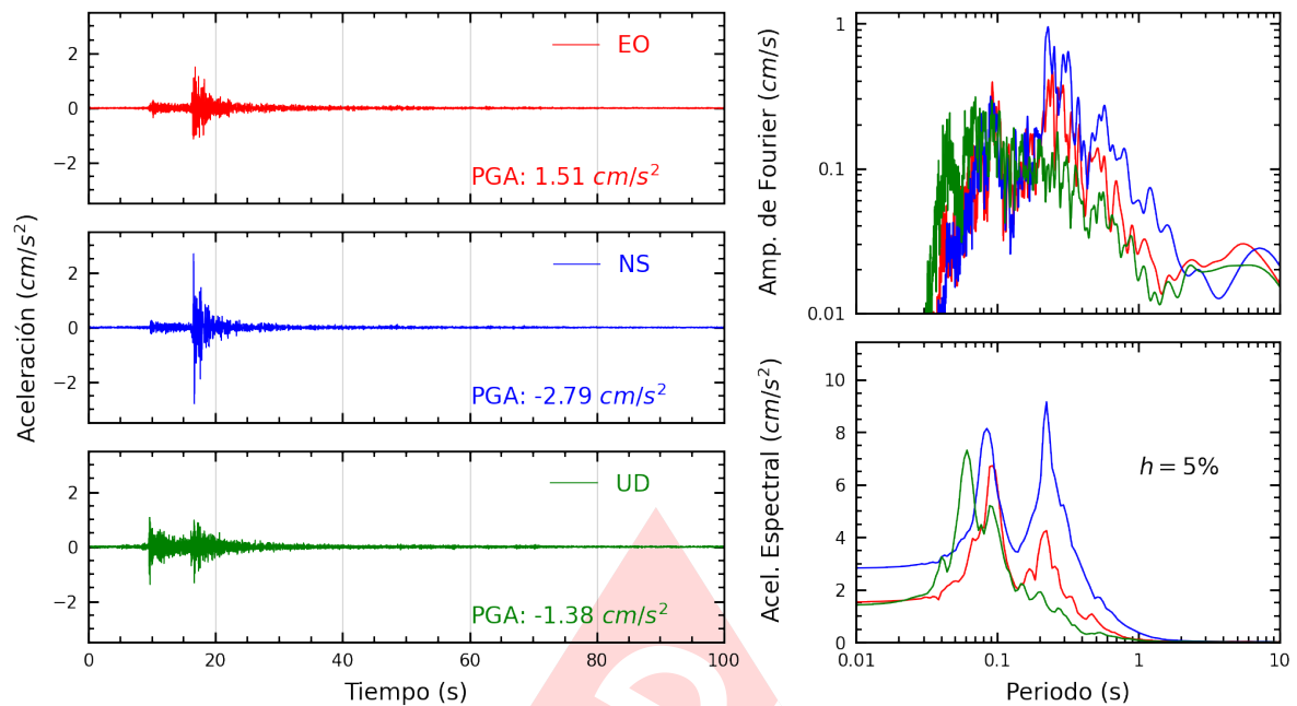
Figura A.25: Registros tiempo-historia, espectros de Fourier y de respuesta en las direcciones EO, NS y vertical de la estación DSML. Sismo de Provincia Constitucional del Callao , Callao - Lima del 2024-01-04, 12:42:39 (Hora local)
