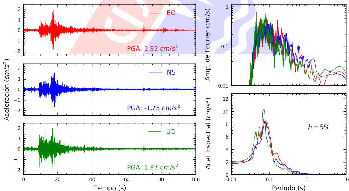
Figura A.30: Registros tiempo-historia, espectros de Fourier y de respuesta en las direcciones EO, NS y vertical de la estación PRADO. Sismo de Provincia Constitucional del Callao , Callao - Lima del 2024-01-04, 12:42:39 (Hora local)
