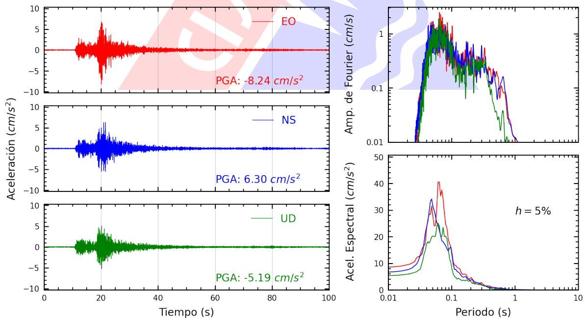
Figura A.8: Registros tiempo-historia, espectros de Fourier y de respuesta en las direcciones EO, NS y vertical de la estación UNTEL. Sismo de Provincia Constitucional del Callao , Callao - Lima del 2024-01-04, 12:42:39 (Hora local)
