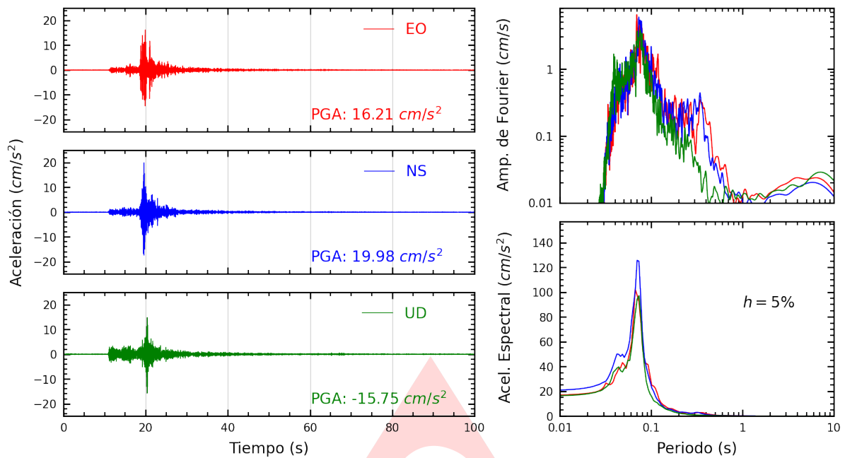
Figura A.1: Registros tiempo-historia, espectros de Fourier y de respuesta en las direcciones EO, NS y vertical de la estación ANCON. Sismo de Provincia Constitucional del Callao , Callao - Lima del 2024-01-04, 12:42:39 (Hora local)
