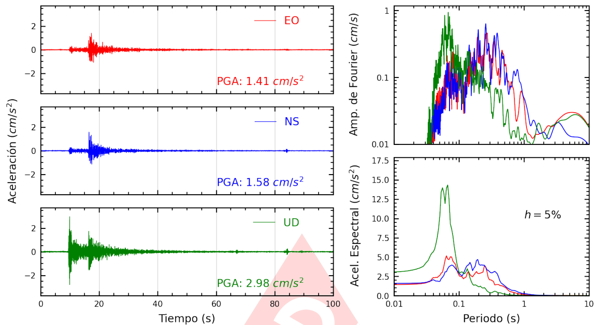
Figura A.23: Registros tiempo-historia, espectros de Fourier y de respuesta en las direcciones EO, NS y vertical de la estación ACAPU. Sismo de Provincia Constitucional del Callao , Callao - Lima del 2024-01-04, 12:42:39 (Hora local)
