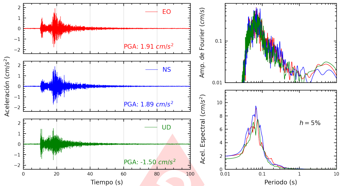
Figura A.33: Registros tiempo-historia, espectros de Fourier y de respuesta en las direcciones EO, NS y vertical de la estación SERVI. Sismo de Provincia Constitucional del Callao , Callao - Lima del 2024-01-04, 12:42:39 (Hora local)
