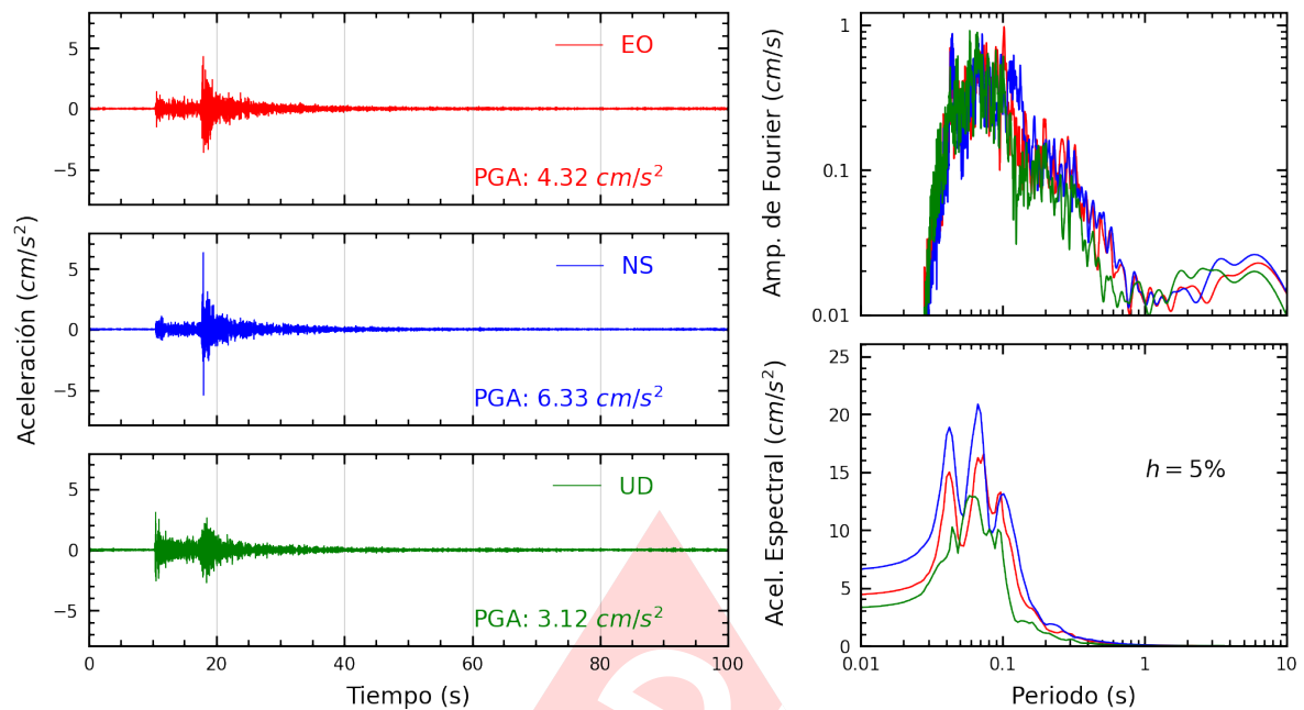
Figura A.11: Registros tiempo-historia, espectros de Fourier y de respuesta en las direcciones EO, NS y vertical de la estación URPE. Sismo de Provincia Constitucional del Callao , Callao - Lima del 2024-01-04, 12:42:39 (Hora local)
