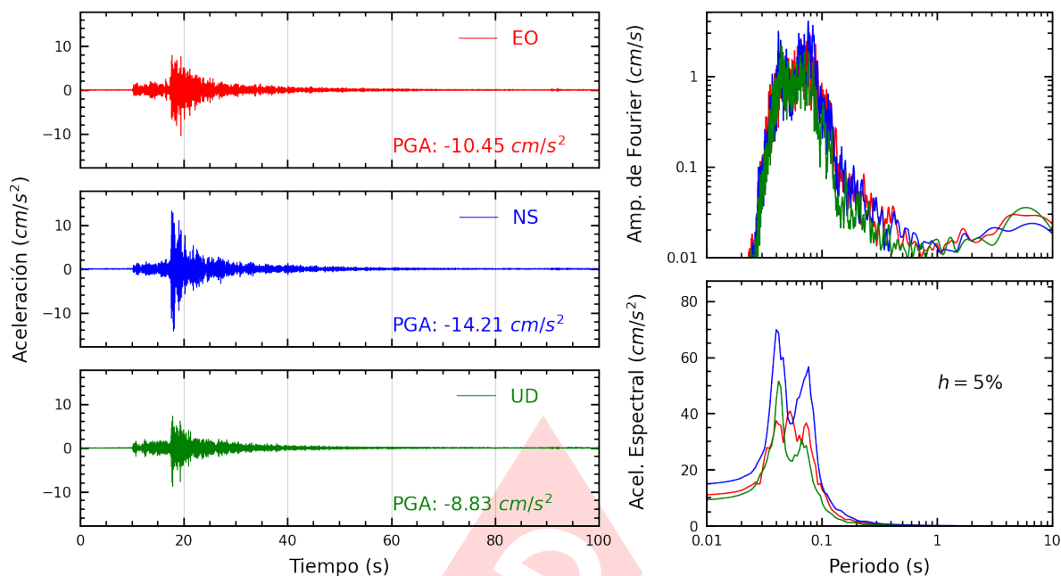
Figura A.3: Registros tiempo-historia, espectros de Fourier y de respuesta en las direcciones EO, NS y vertical de la estación JOSEO. Sismo de Provincia Constitucional del Callao , Callao - Lima del 2024-01-04, 12:42:39 (Hora local)
