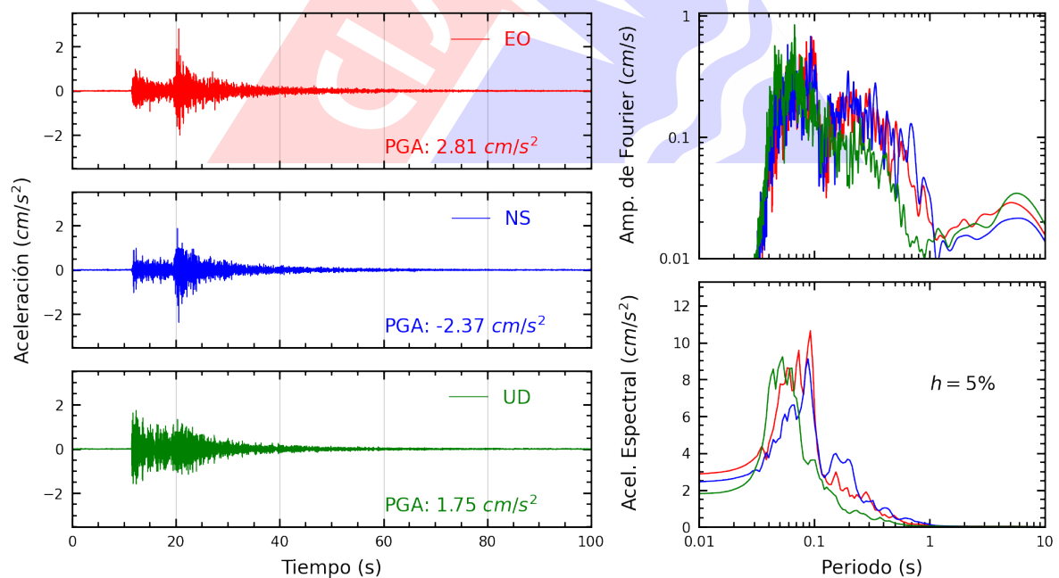
Figura A.24: Registros tiempo-historia, espectros de Fourier y de respuesta en las direcciones EO, NS y vertical de la estación USILP. Sismo de Provincia Constitucional del Callao , Callao - Lima del 2024-01-04, 12:42:39 (Hora local)
