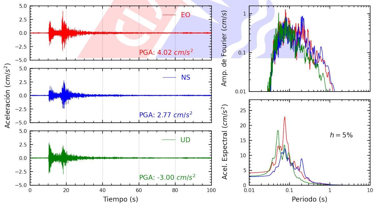
Figura A.18: Registros tiempo-historia, espectros de Fourier y de respuesta en las direcciones EO, NS y vertical de la estación SCCHO. Sismo de Provincia Constitucional del Callao , Callao - Lima del 2024-01-04, 12:42:39 (Hora local)
