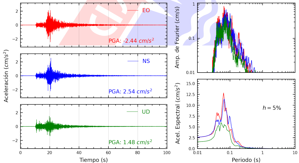
Figura A.26: Registros tiempo-historia, espectros de Fourier y de respuesta en las direcciones EO, NS y vertical de la estación ATARJ. Sismo de Provincia Constitucional del Callao , Callao - Lima del 2024-01-04, 12:42:39 (Hora local)
