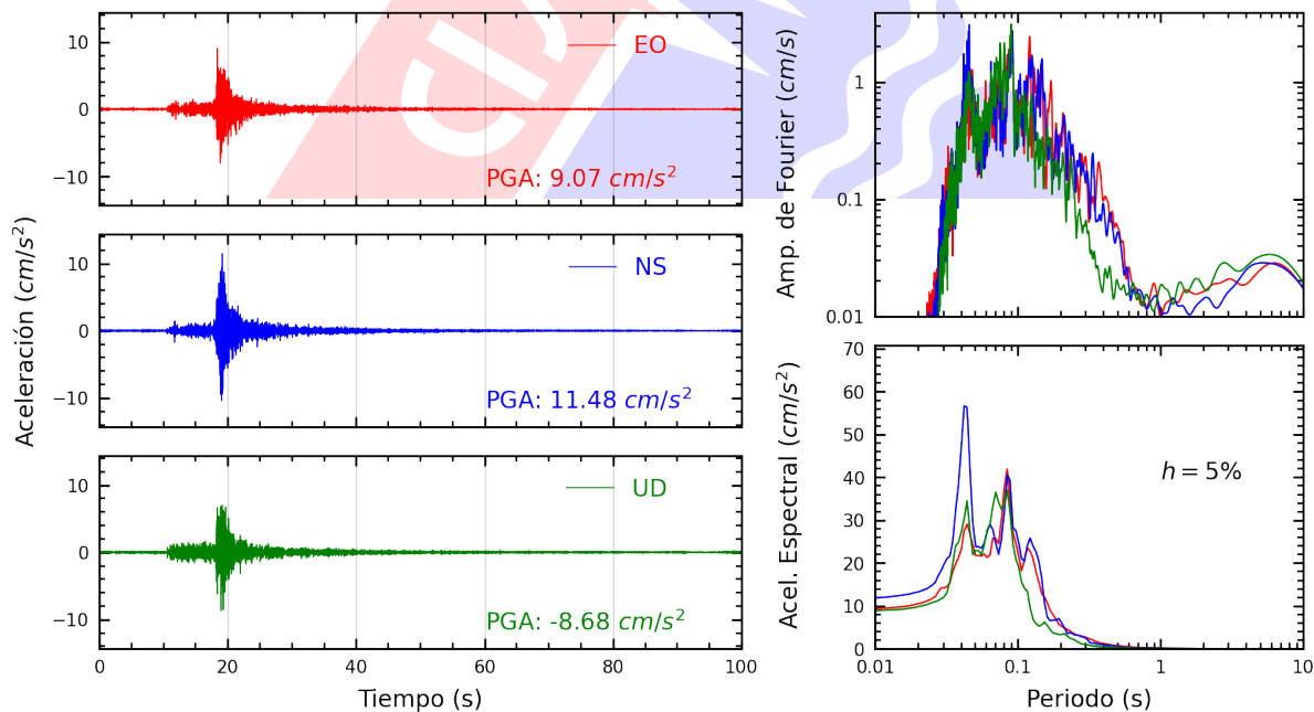
Figura A.4: Registros tiempo-historia, espectros de Fourier y de respuesta en las direcciones EO, NS y vertical de la estación CARAB. Sismo de Provincia Constitucional del Callao , Callao - Lima del 2024-01-04, 12:42:39 (Hora local)
