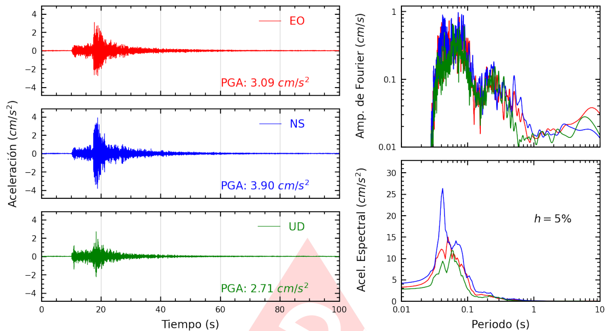
Figura A.19: Registros tiempo-historia, espectros de Fourier y de respuesta en las direcciones EO, NS y vertical de la estación COMAS. Sismo de Provincia Constitucional del Callao , Callao - Lima del 2024-01-04, 12:42:39 (Hora local)
