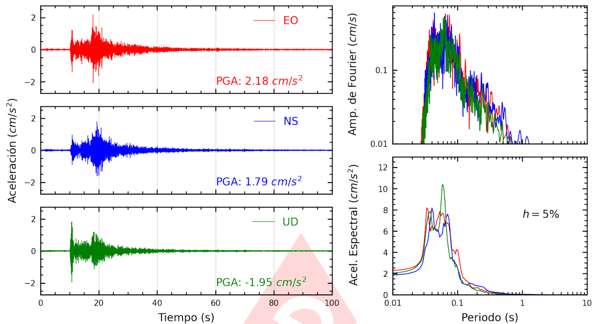
Figura A.27: Registros tiempo-historia, espectros de Fourier y de respuesta en las direcciones EO, NS y vertical de la estación BORJA. Sismo de Provincia Constitucional del Callao , Callao - Lima del 2024-01-04, 12:42:39 (Hora local)
