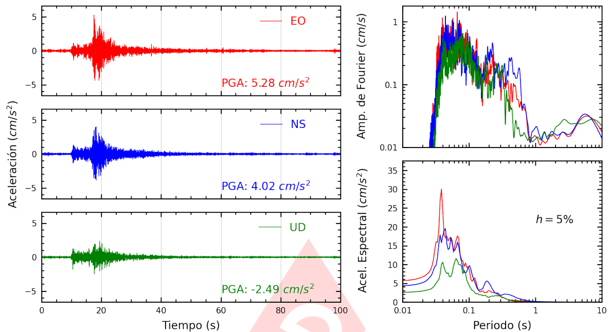
Figura A.15: Registros tiempo-historia, espectros de Fourier y de respuesta en las direcciones EO, NS y vertical de la estación OLIVO. Sismo de Provincia Constitucional del Callao , Callao - Lima del 2024-01-04, 12:42:39 (Hora local)
