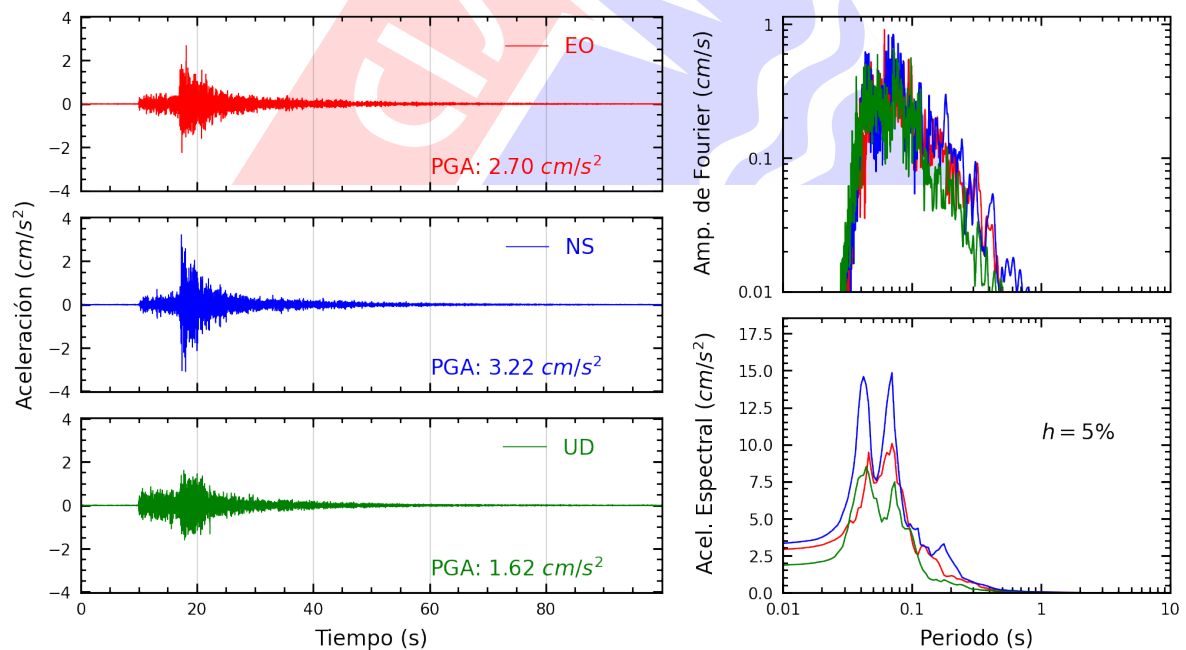
Figura A.22: Registros tiempo-historia, espectros de Fourier y de respuesta en las direcciones EO, NS y vertical de la estación JALV2. Sismo de Provincia Constitucional del Callao , Callao - Lima del 2024-01-04, 12:42:39 (Hora local)
