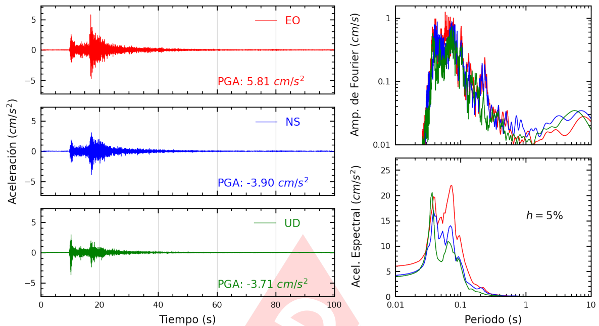
Figura A.13: Registros tiempo-historia, espectros de Fourier y de respuesta en las direcciones EO, NS y vertical de la estación CEPRE. Sismo de Provincia Constitucional del Callao , Callao - Lima del 2024-01-04, 12:42:39 (Hora local)
