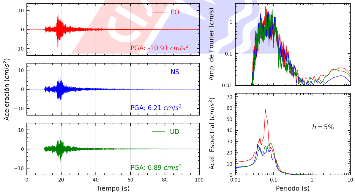
Figura A.6: Registros tiempo-historia, espectros de Fourier y de respuesta en las direcciones EO, NS y vertical de la estación AMORE. Sismo de Provincia Constitucional del Callao , Callao - Lima del 2024-01-04, 12:42:39 (Hora local)
