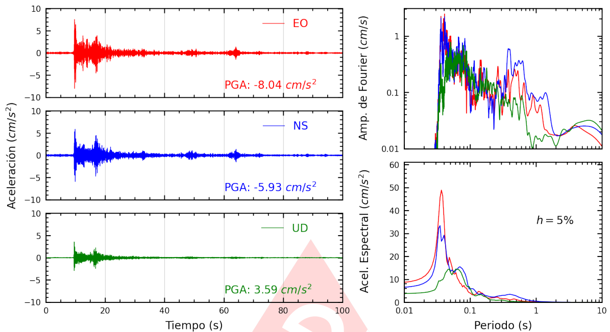
Figura A.9: Registros tiempo-historia, espectros de Fourier y de respuesta en las direcciones EO, NS y vertical de la estación DHNPE. Sismo de Provincia Constitucional del Callao , Callao - Lima del 2024-01-04, 12:42:39 (Hora local)
