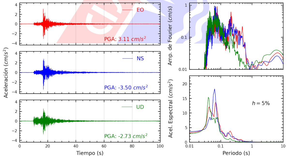
Figura A.20: Registros tiempo-historia, espectros de Fourier y de respuesta en las direcciones EO, NS y vertical de la estación VHAYA. Sismo de Provincia Constitucional del Callao , Callao - Lima del 2024-01-04, 12:42:39 (Hora local)
