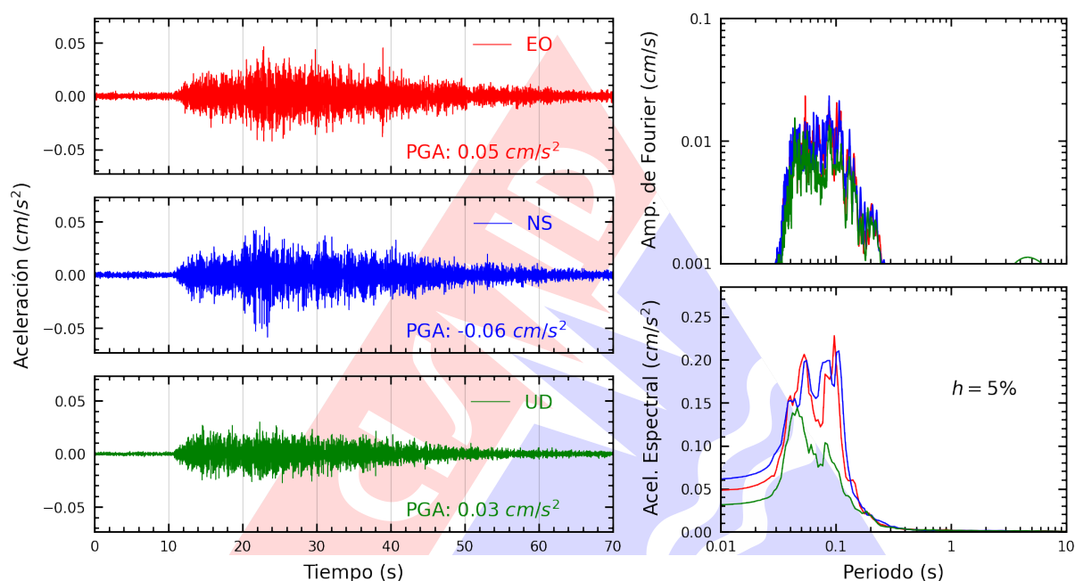
Figura A.3: Registros tiempo-historia, espectros de Fourier y de respuesta en las direcciones EO, NS y vertical de la estación UNSA. Sismo de Arequipa, Arequipa - Arequipa del 2024-01-11, 15:38:52 (Hora local)
