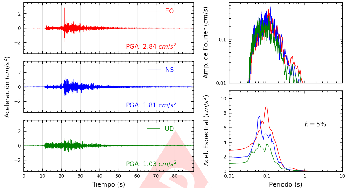
Figura A.7: Registros tiempo-historia, espectros de Fourier y de respuesta en las direcciones EO, NS y vertical de la estación SERV2. Sismo de Chosica, Lima - Lima del 2024-01-29, 17:04:56 (Hora local)
