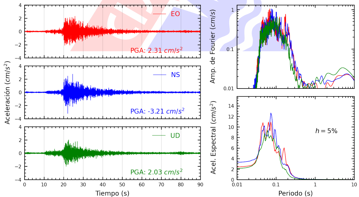
Figura A.6: Registros tiempo-historia, espectros de Fourier y de respuesta en las direcciones EO, NS y vertical de la estación INDEP. Sismo de Chosica, Lima - Lima del 2024-01-29, 17:04:56 (Hora local)
