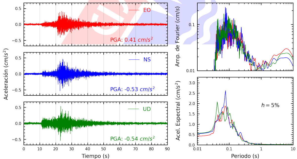
Figura A.38: Registros tiempo-historia, espectros de Fourier y de respuesta en las direcciones EO, NS y vertical de la estación BONDY. Sismo de Chosica, Lima - Lima del 2024-01-29, 17:04:56 (Hora local)
