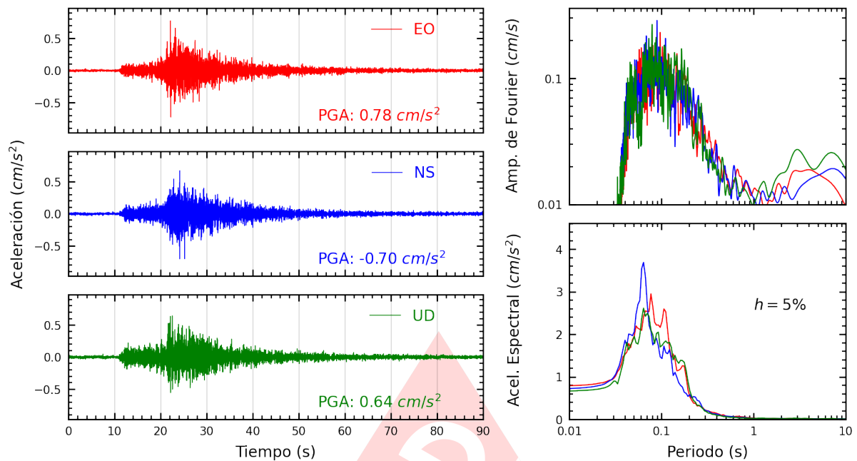
Figura A.35: Registros tiempo-historia, espectros de Fourier y de respuesta en las direcciones EO, NS y vertical de la estación UNFV. Sismo de Chosica, Lima - Lima del 2024-01-29, 17:04:56 (Hora local)
