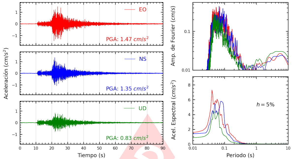
Figura A.23: Registros tiempo-historia, espectros de Fourier y de respuesta en las direcciones EO, NS y vertical de la estación UCSS. Sismo de Chosica, Lima - Lima del 2024-01-29, 17:04:56 (Hora local)
