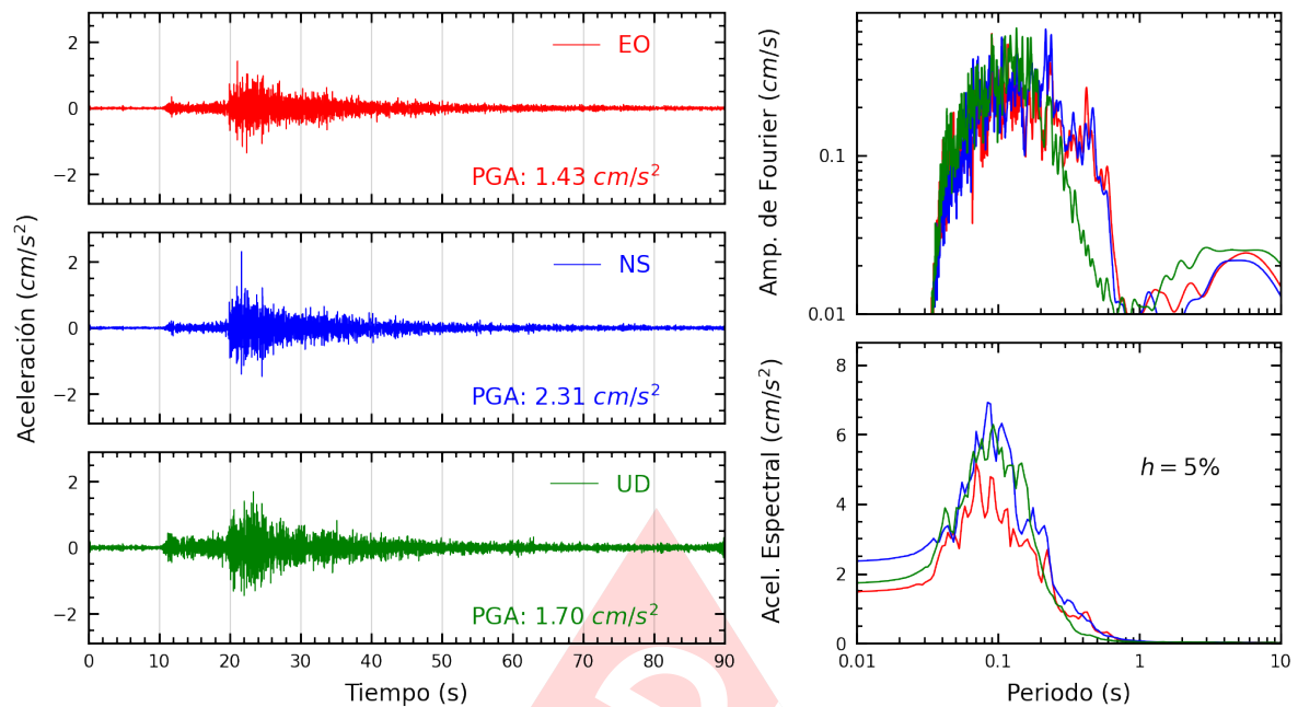
Figura A.11: Registros tiempo-historia, espectros de Fourier y de respuesta en las direcciones EO, NS y vertical de la estación MDPP. Sismo de Chosica, Lima - Lima del 2024-01-29, 17:04:56 (Hora local)
