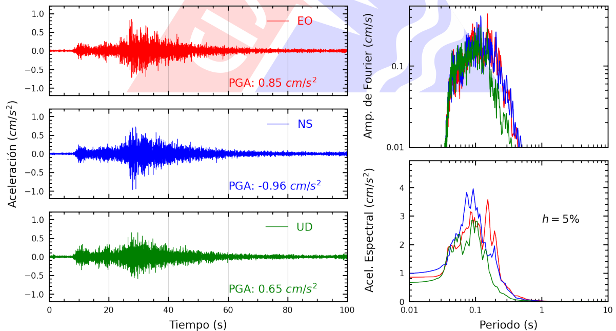
Figura A.32: Registros tiempo-historia, espectros de Fourier y de respuesta en las direcciones EO, NS y vertical de la estación ASIA. Sismo de Chosica, Lima - Lima del 2024-01-29, 17:04:56 (Hora local)
