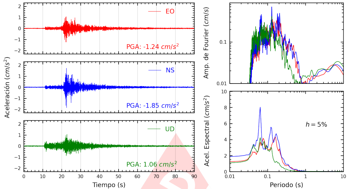
Figura A.15: Registros tiempo-historia, espectros de Fourier y de respuesta en las direcciones EO, NS y vertical de la estación VHAYA. Sismo de Chosica, Lima - Lima del 2024-01-29, 17:04:56 (Hora local)
