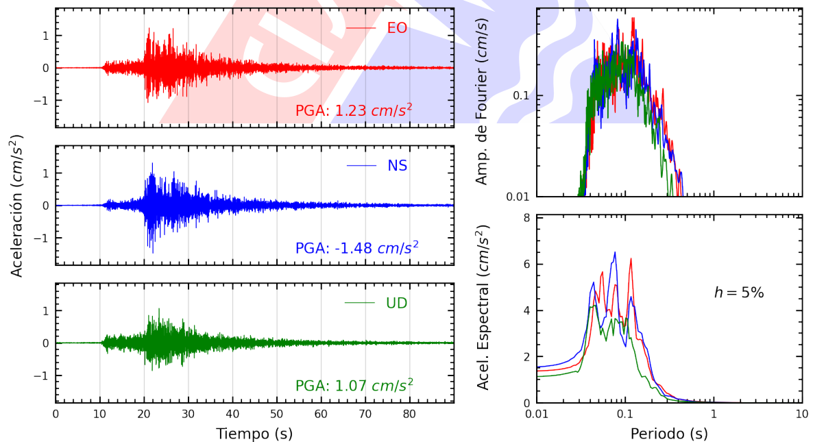
Figura A.22: Registros tiempo-historia, espectros de Fourier y de respuesta en las direcciones EO, NS y vertical de la estación JALV2. Sismo de Chosica, Lima - Lima del 2024-01-29, 17:04:56 (Hora local)
