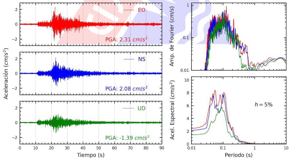
Figura A.12: Registros tiempo-historia, espectros de Fourier y de respuesta en las direcciones EO, NS y vertical de la estación OLIVO. Sismo de Chosica, Lima - Lima del 2024-01-29, 17:04:56 (Hora local)
