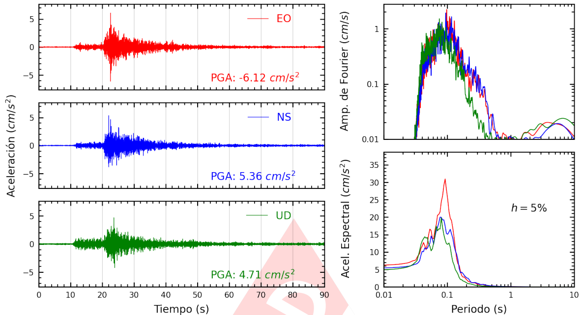
Figura A.3: Registros tiempo-historia, espectros de Fourier y de respuesta en las direcciones EO, NS y vertical de la estación ANCON. Sismo de Chosica, Lima - Lima del 2024-01-29, 17:04:56 (Hora local)
