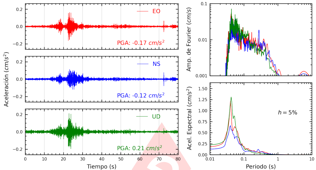
Figura A.39: Registros tiempo-historia, espectros de Fourier y de respuesta en las direcciones EO, NS y vertical de la estación UNIA. Sismo de Chosica, Lima - Lima del 2024-01-29, 17:04:56 (Hora local)
