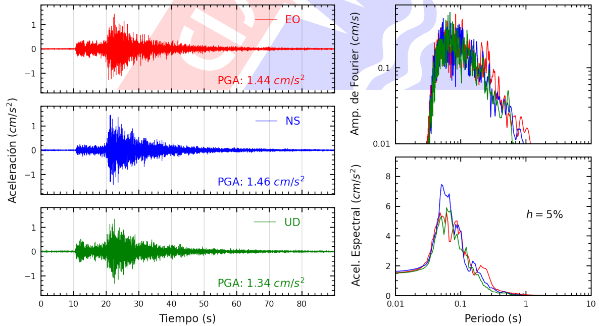
Figura A.24: Registros tiempo-historia, espectros de Fourier y de respuesta en las direcciones EO, NS y vertical de la estación IMCA2. Sismo de Chosica, Lima - Lima del 2024-01-29, 17:04:56 (Hora local)
