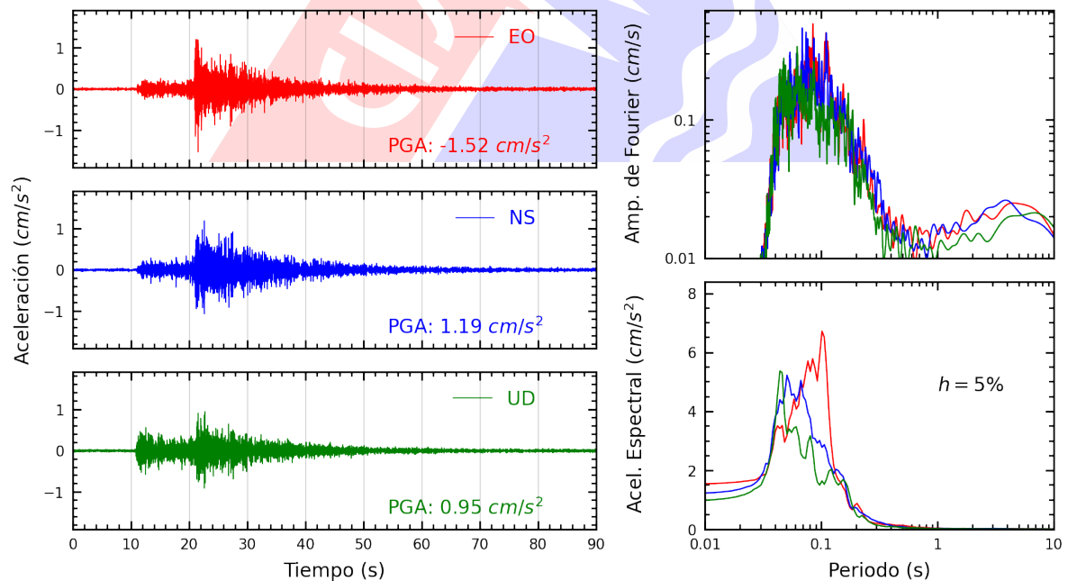
Figura A.20: Registros tiempo-historia, espectros de Fourier y de respuesta en las direcciones EO, NS y vertical de la estación CENEP. Sismo de Chosica, Lima - Lima del 2024-01-29, 17:04:56 (Hora local)
