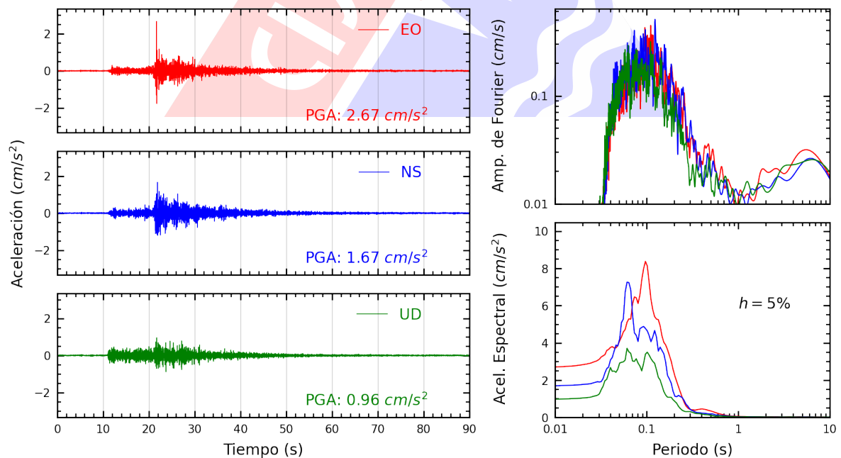
Figura A.8: Registros tiempo-historia, espectros de Fourier y de respuesta en las direcciones EO, NS y vertical de la estación SERVI. Sismo de Chosica, Lima - Lima del 2024-01-29, 17:04:56 (Hora local)
