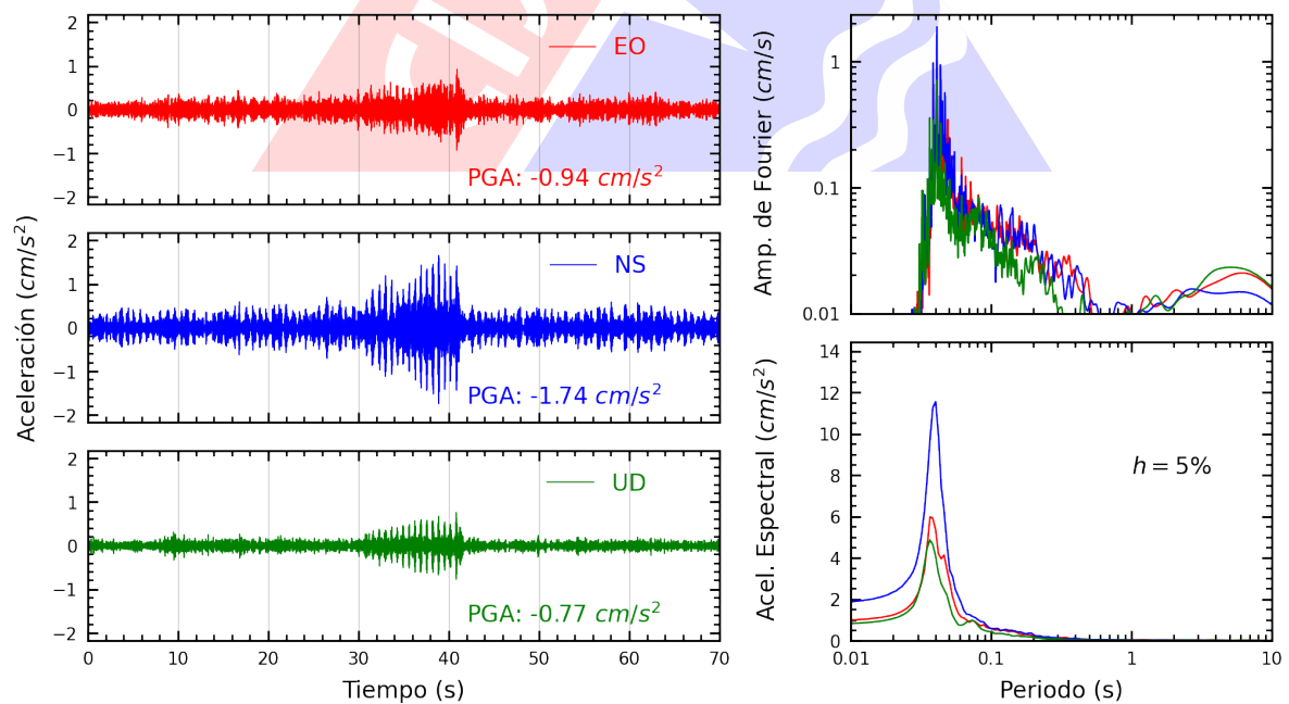
Figura A.16: Registros tiempo-historia, espectros de Fourier y de respuesta en las direcciones EO, NS y vertical de la estación USP. Sismo de Chosica, Lima - Lima del 2024-01-29, 17:04:56 (Hora local)
