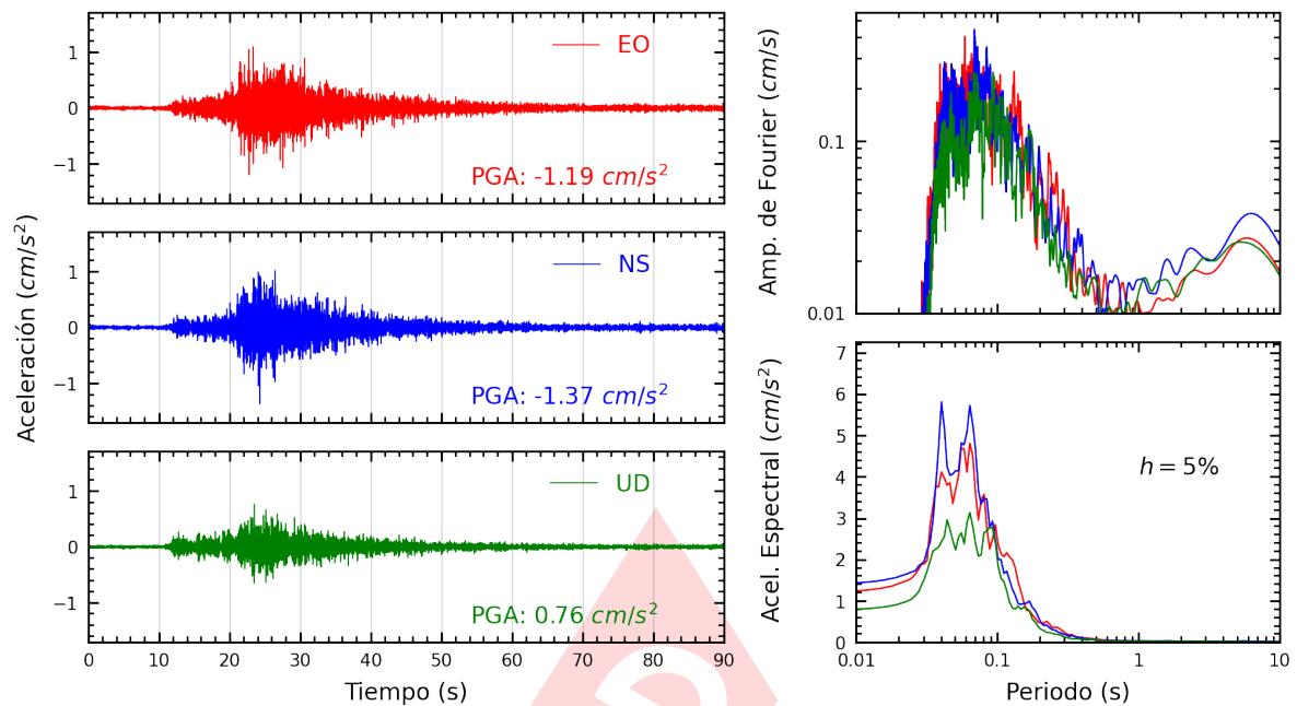
Figura A.29: Registros tiempo-historia, espectros de Fourier y de respuesta en las direcciones EO, NS y vertical de la estación CEPRE. Sismo de Chosica, Lima - Lima del 2024-01-29, 17:04:56 (Hora local)
