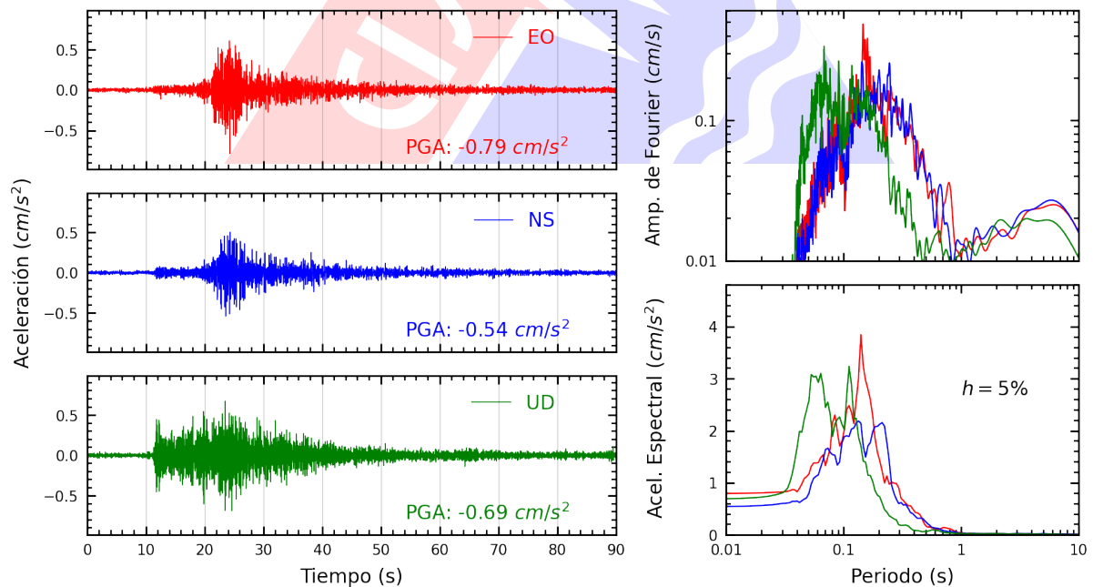
Figura A.34: Registros tiempo-historia, espectros de Fourier y de respuesta en las direcciones EO, NS y vertical de la estación ACAPU. Sismo de Chosica, Lima - Lima del 2024-01-29, 17:04:56 (Hora local)
