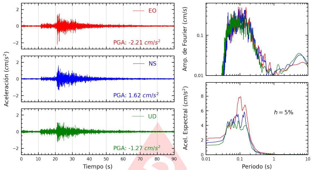
Figura A.13: Registros tiempo-historia, espectros de Fourier y de respuesta en las direcciones EO, NS y vertical de la estación URPE. Sismo de Chosica, Lima - Lima del 2024-01-29, 17:04:56 (Hora local)
