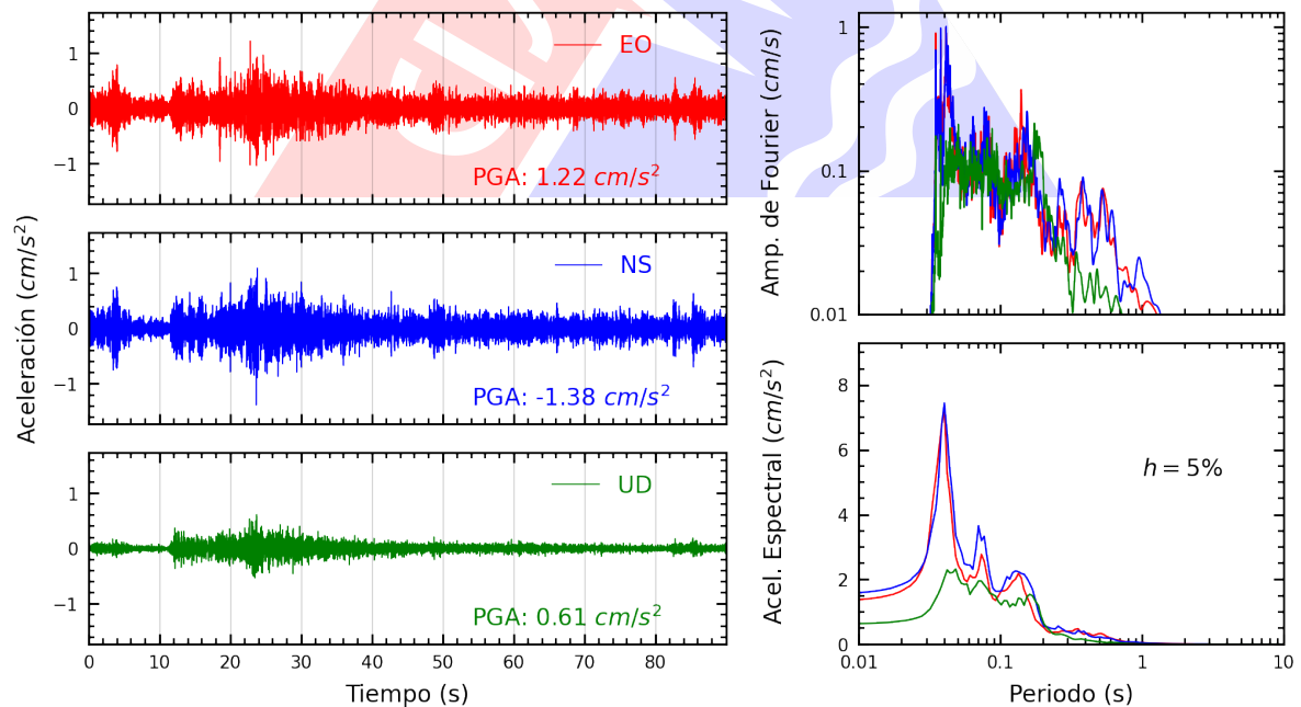
Figura A.28: Registros tiempo-historia, espectros de Fourier y de respuesta en las direcciones EO, NS y vertical de la estación DHN2. Sismo de Chosica, Lima - Lima del 2024-01-29, 17:04:56 (Hora local)
