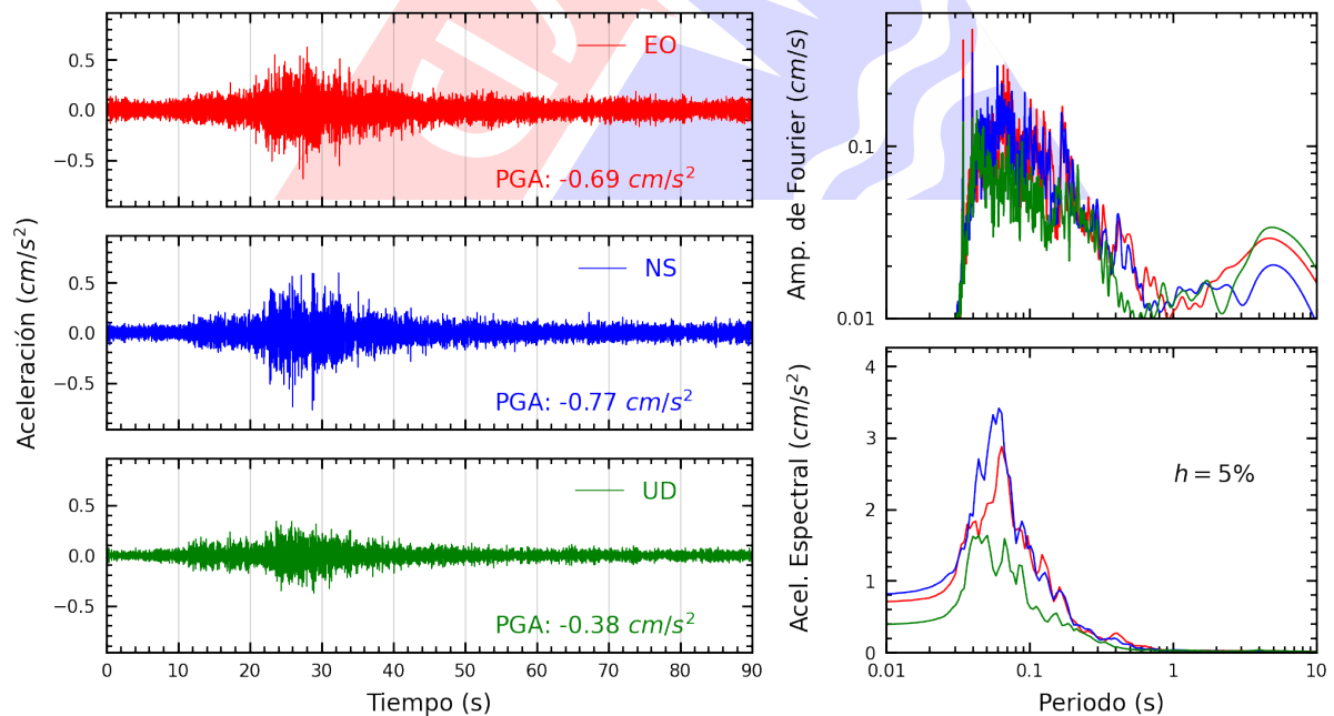
Figura A.36: Registros tiempo-historia, espectros de Fourier y de respuesta en las direcciones EO, NS y vertical de la estación UPCVI. Sismo de Chosica, Lima - Lima del 2024-01-29, 17:04:56 (Hora local)
