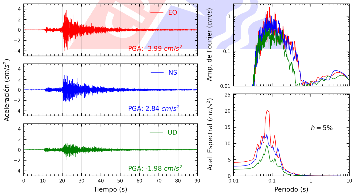
Figura A.4: Registros tiempo-historia, espectros de Fourier y de respuesta en las direcciones EO, NS y vertical de la estación DEFEN. Sismo de Chosica, Lima - Lima del 2024-01-29, 17:04:56 (Hora local)
