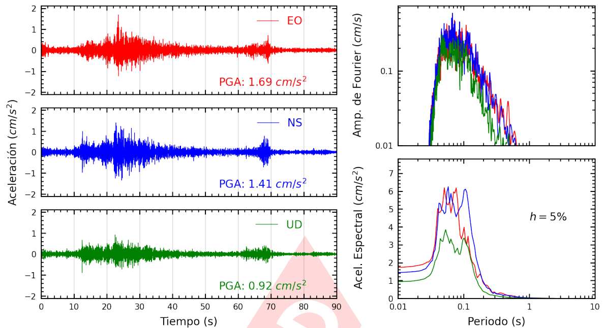
Figura A.17: Registros tiempo-historia, espectros de Fourier y de respuesta en las direcciones EO, NS y vertical de la estación PACHA. Sismo de Chosica, Lima - Lima del 2024-01-29, 17:04:56 (Hora local)
