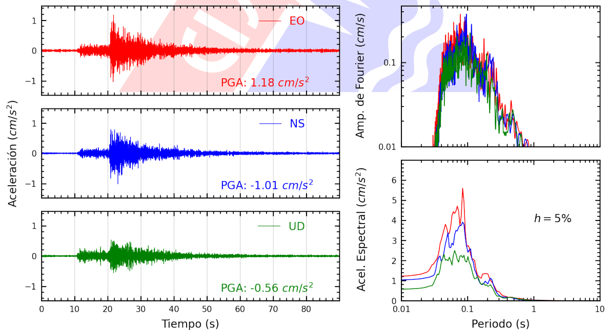
Figura A.30: Registros tiempo-historia, espectros de Fourier y de respuesta en las direcciones EO, NS y vertical de la estación INIC2. Sismo de Chosica, Lima - Lima del 2024-01-29, 17:04:56 (Hora local)
