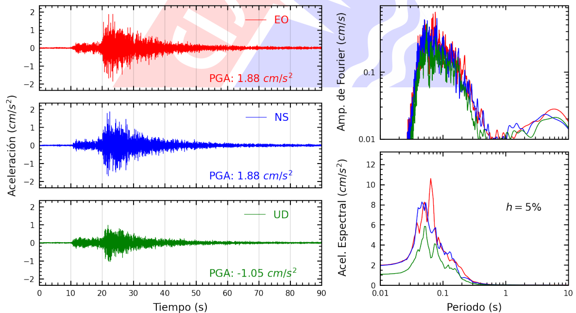
Figura A.14: Registros tiempo-historia, espectros de Fourier y de respuesta en las direcciones EO, NS y vertical de la estación FICPE. Sismo de Chosica, Lima - Lima del 2024-01-29, 17:04:56 (Hora local)
