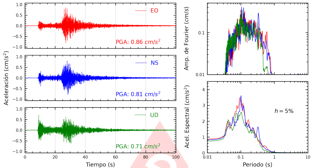
Figura A.33: Registros tiempo-historia, espectros de Fourier y de respuesta en las direcciones EO, NS y vertical de la estación CARAL. Sismo de Chosica, Lima - Lima del 2024-01-29, 17:04:56 (Hora local)
