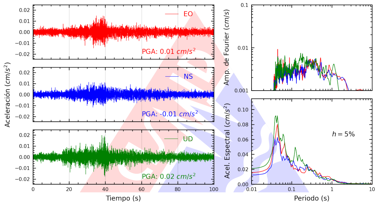
Figura A.41: Registros tiempo-historia, espectros de Fourier y de respuesta en las direcciones EO, NS y vertical de la estación UNCP. Sismo de Chosica, Lima - Lima del 2024-01-29, 17:04:56 (Hora local)
