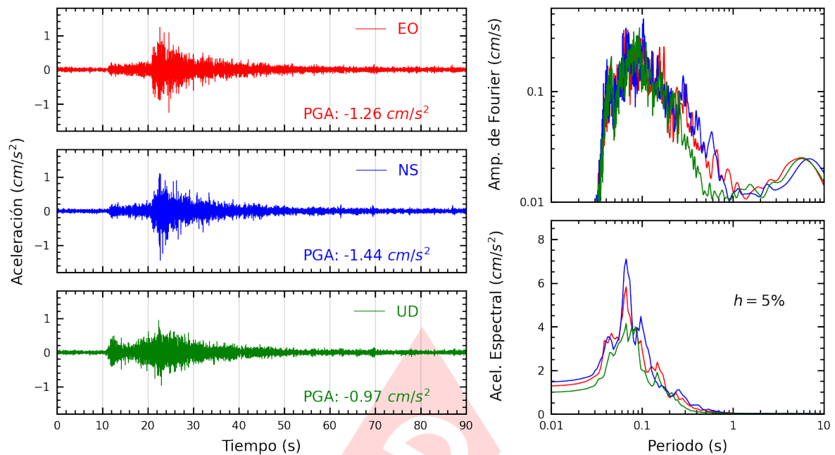
Figura A.25: Registros tiempo-historia, espectros de Fourier y de respuesta en las direcciones EO, NS y vertical de la estación MADRE. Sismo de Chosica, Lima - Lima del 2024-01-29, 17:04:56 (Hora local)
