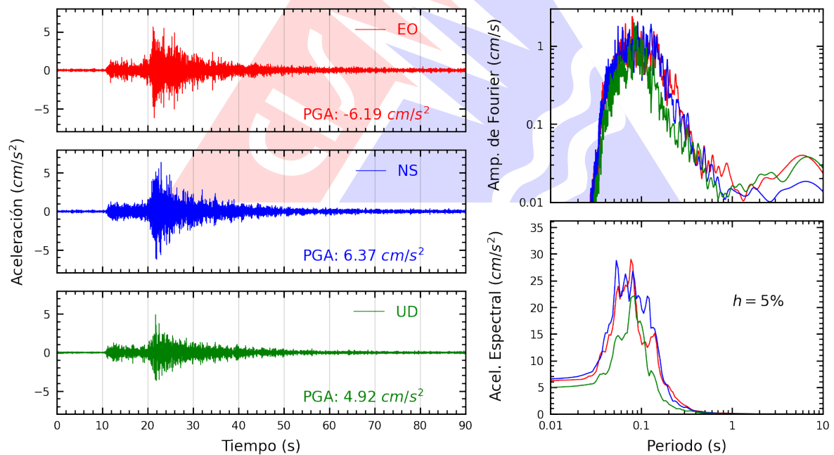
Figura A.2: Registros tiempo-historia, espectros de Fourier y de respuesta en las direcciones EO, NS y vertical de la estación USILM. Sismo de Chosica, Lima - Lima del 2024-01-29, 17:04:56 (Hora local)
