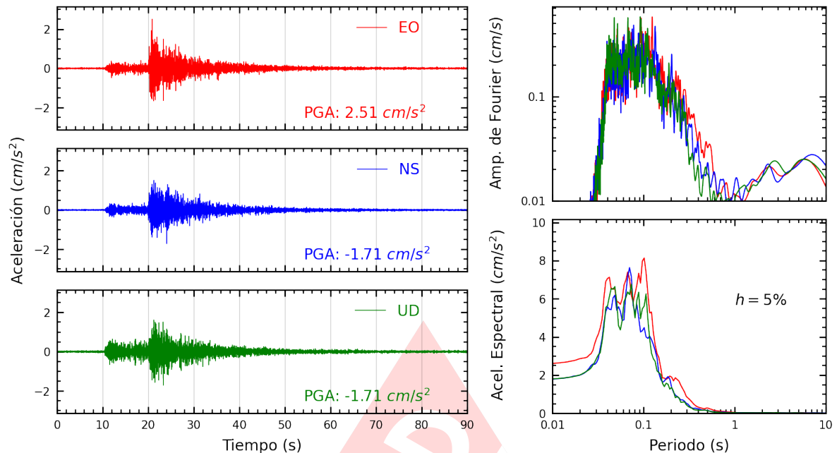
Figura A.9: Registros tiempo-historia, espectros de Fourier y de respuesta en las direcciones EO, NS y vertical de la estación USMP. Sismo de Chosica, Lima - Lima del 2024-01-29, 17:04:56 (Hora local)
