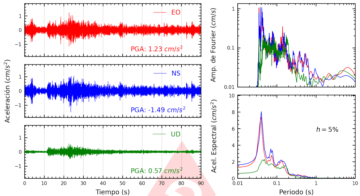
Figura A.21: Registros tiempo-historia, espectros de Fourier y de respuesta en las direcciones EO, NS y vertical de la estación DHNPE. Sismo de Chosica, Lima - Lima del 2024-01-29, 17:04:56 (Hora local)
