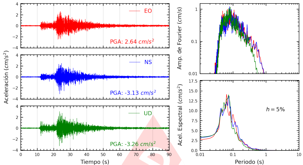
Figura A.5: Registros tiempo-historia, espectros de Fourier y de respuesta en las direcciones EO, NS y vertical de la estación UNTEL. Sismo de Chosica, Lima - Lima del 2024-01-29, 17:04:56 (Hora local)
