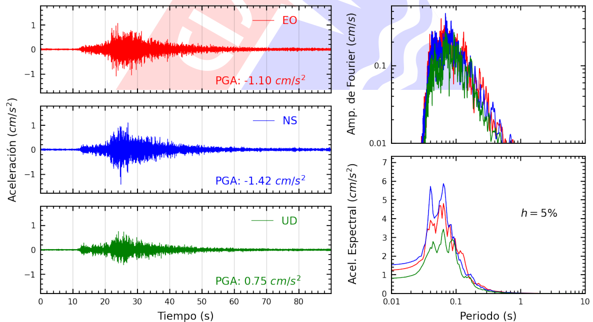
Figura A.26: Registros tiempo-historia, espectros de Fourier y de respuesta en las direcciones EO, NS y vertical de la estación CEPR2. Sismo de Chosica, Lima - Lima del 2024-01-29, 17:04:56 (Hora local)
