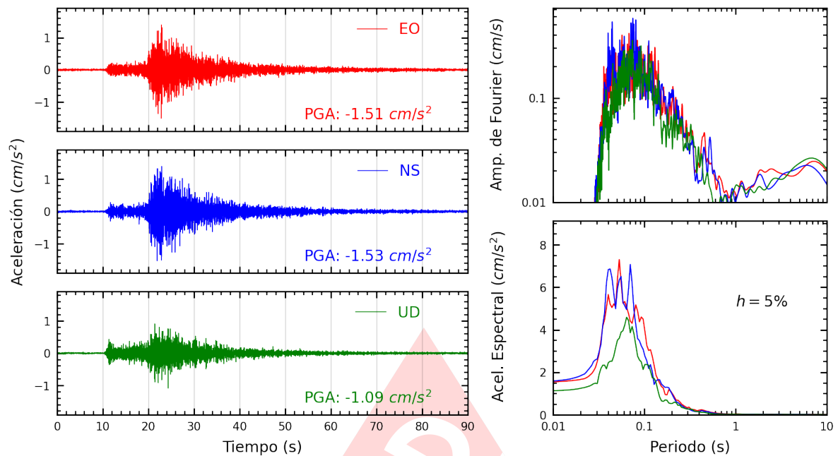
Figura A.19: Registros tiempo-historia, espectros de Fourier y de respuesta en las direcciones EO, NS y vertical de la estación COMAS. Sismo de Chosica, Lima - Lima del 2024-01-29, 17:04:56 (Hora local)
