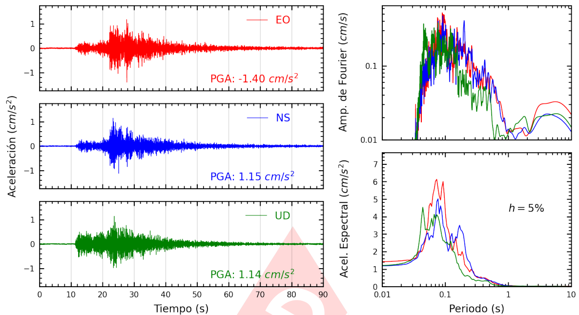
Figura A.27: Registros tiempo-historia, espectros de Fourier y de respuesta en las direcciones EO, NS y vertical de la estación USILP. Sismo de Chosica, Lima - Lima del 2024-01-29, 17:04:56 (Hora local)
