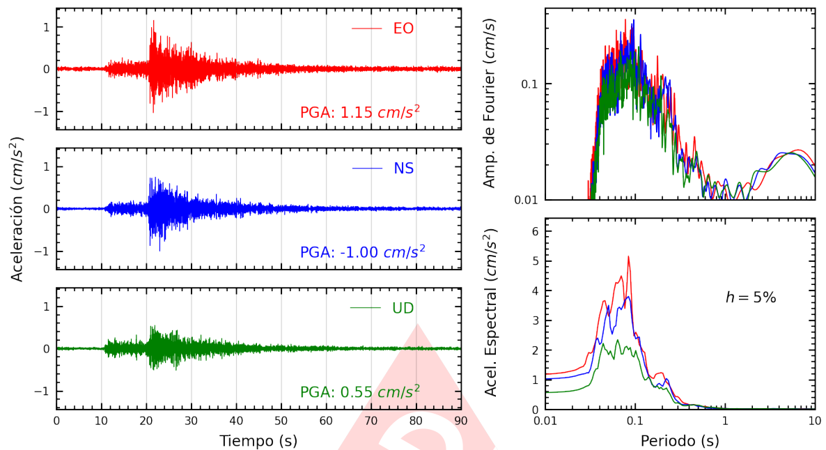
Figura A.31: Registros tiempo-historia, espectros de Fourier y de respuesta en las direcciones EO, NS y vertical de la estación INICT. Sismo de Chosica, Lima - Lima del 2024-01-29, 17:04:56 (Hora local)
