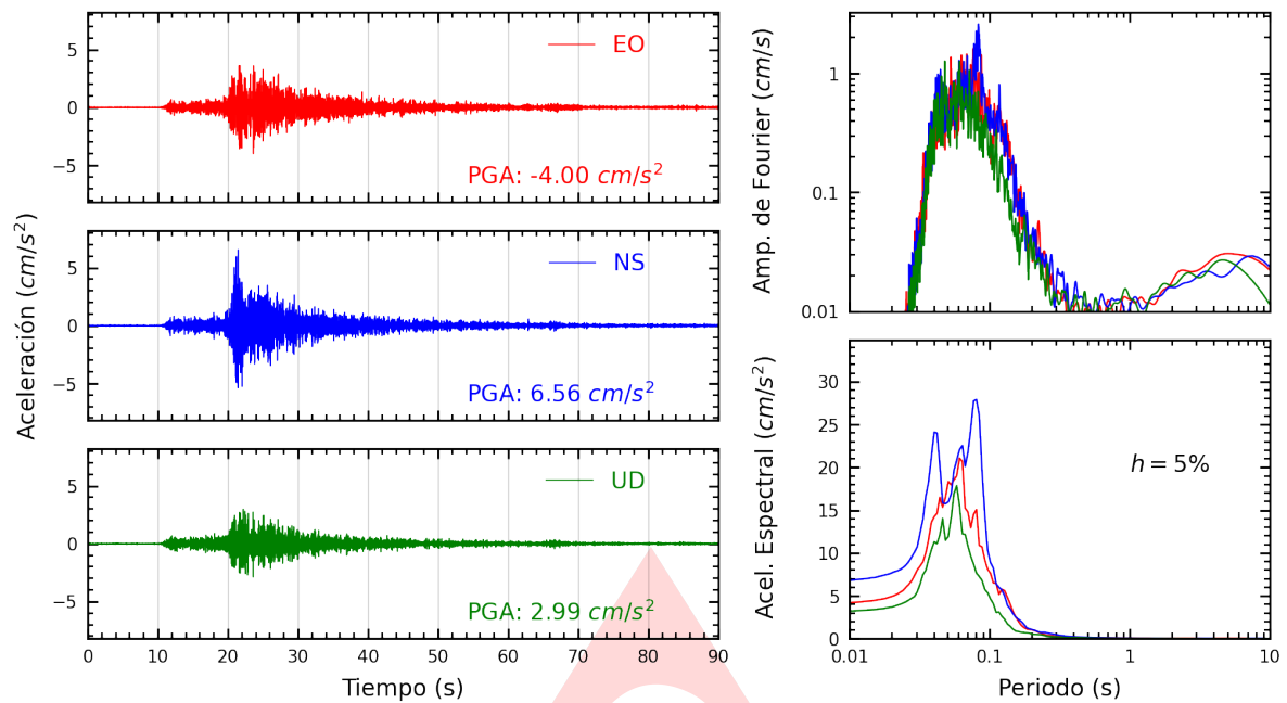
Figura A.1: Registros tiempo-historia, espectros de Fourier y de respuesta en las direcciones EO, NS y vertical de la estación JOSEO. Sismo de Chosica, Lima - Lima del 2024-01-29, 17:04:56 (Hora local)
