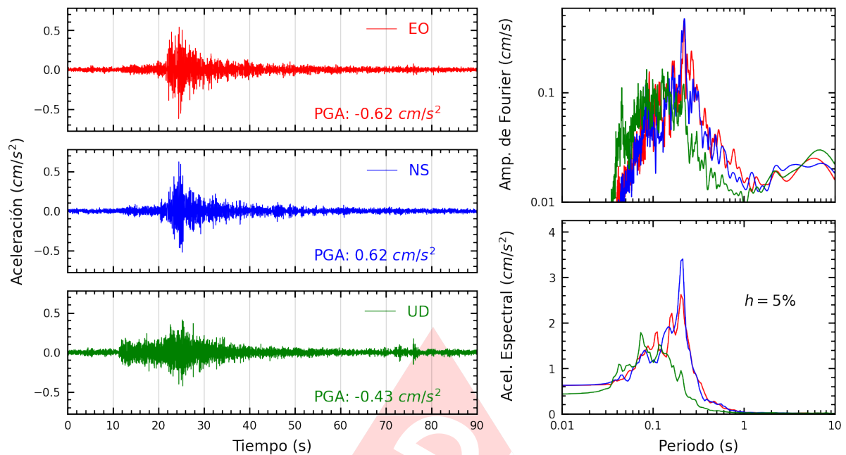
Figura A.37: Registros tiempo-historia, espectros de Fourier y de respuesta en las direcciones EO, NS y vertical de la estación DSML. Sismo de Chosica, Lima - Lima del 2024-01-29, 17:04:56 (Hora local)
