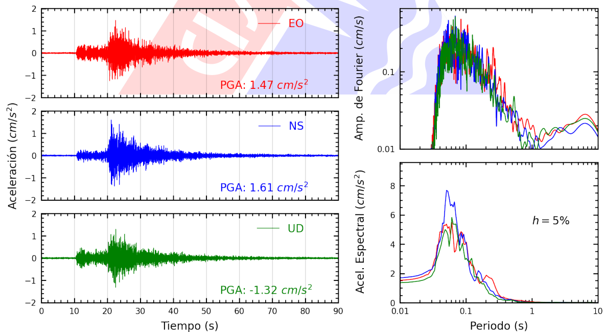
Figura A.18: Registros tiempo-historia, espectros de Fourier y de respuesta en las direcciones EO, NS y vertical de la estación IMCA. Sismo de Chosica, Lima - Lima del 2024-01-29, 17:04:56 (Hora local)
