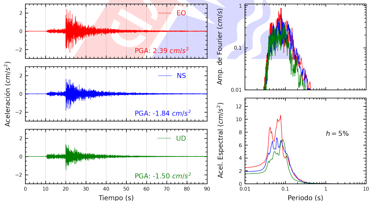
Figura A.10: Registros tiempo-historia, espectros de Fourier y de respuesta en las direcciones EO, NS y vertical de la estación ATARJ. Sismo de Chosica, Lima - Lima del 2024-01-29, 17:04:56 (Hora local)
