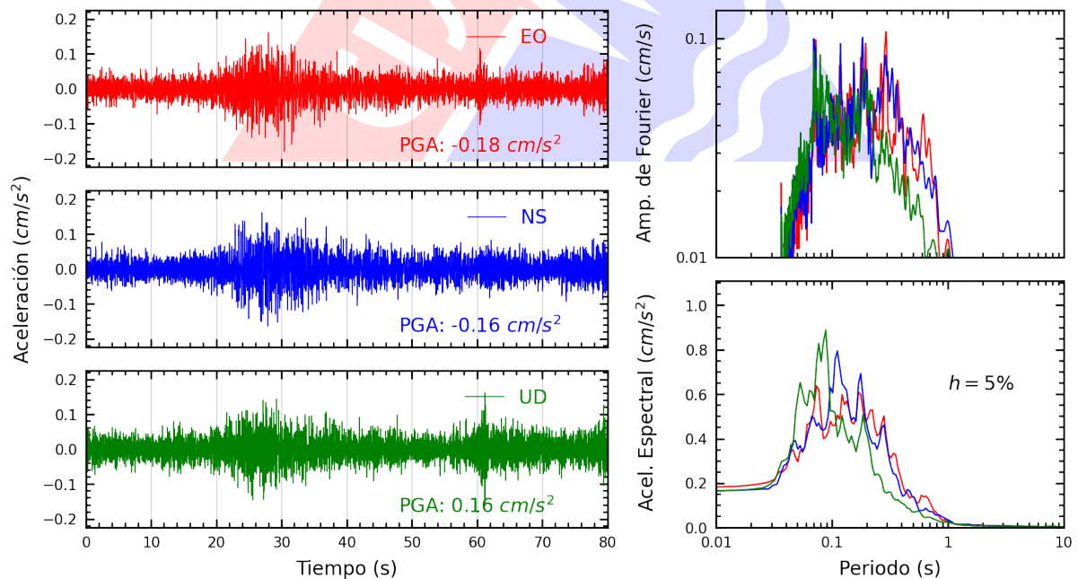
Figura A.40: Registros tiempo-historia, espectros de Fourier y de respuesta en las direcciones EO, NS y vertical de la estación UNICA. Sismo de Chosica, Lima - Lima del 2024-01-29, 17:04:56 (Hora local)
