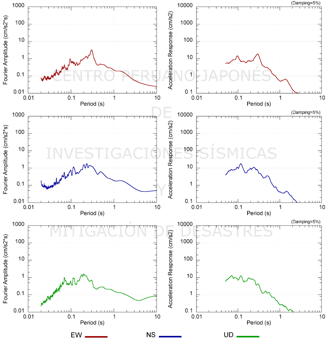
Espectros de amplitudes de Fourier y espectros de respuesta de aceleración absoluta (5% de amortiguamiento) en las direcciones EW, NS y vertical de la estación TAC004. Sismo de Iquique – Chile del 05 de Abril de 2018 08:12:12 (hora local de Chile)
