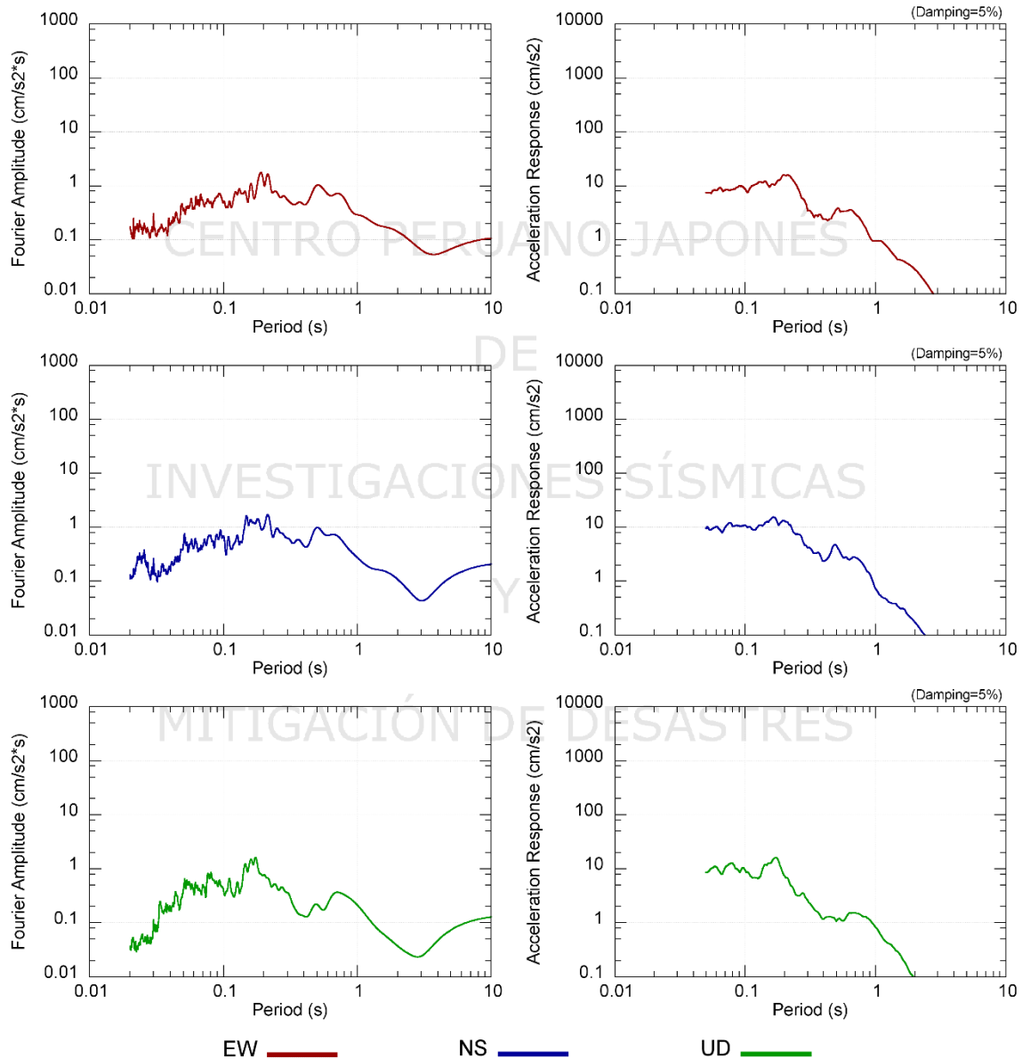
Espectros de amplitudes de Fourier y espectros de respuesta de aceleración absoluta (5% de amortiguamiento) en las direcciones EW, NS y vertical de la estación AQP003. Sismo de Iquique – Chile del 05 de Abril de 2018 08:12:12 (hora local de Chile)
