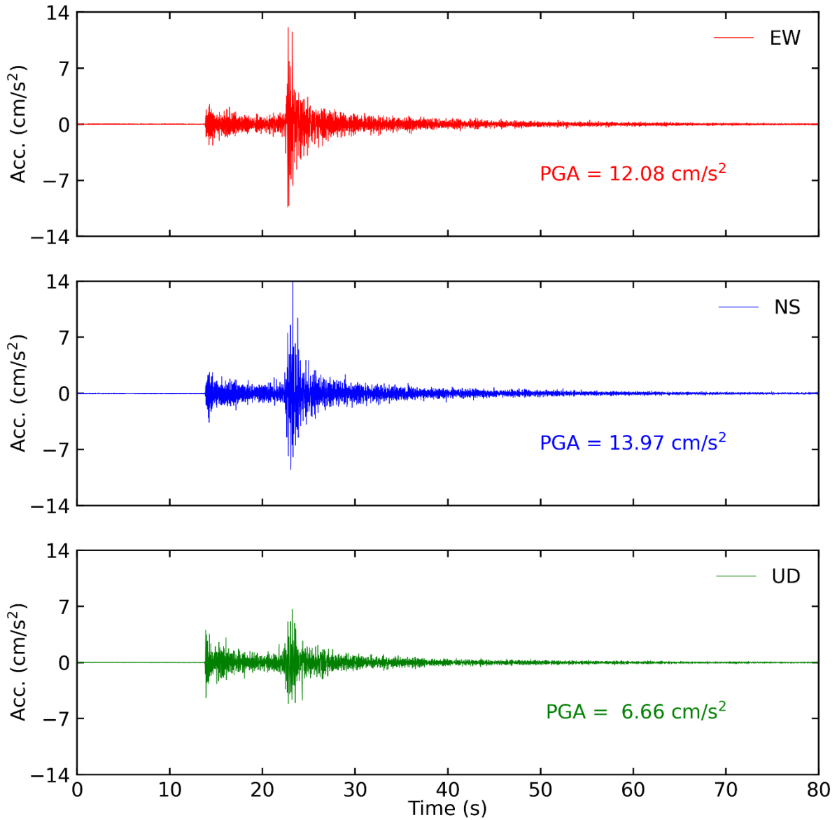
Tiempo historia en las tres direcciones (EW, NS y vertical) de la estación LIM019. Sismo de Callao-Callao del 25 de agosto del 2021 02:15:08 (hora local)
