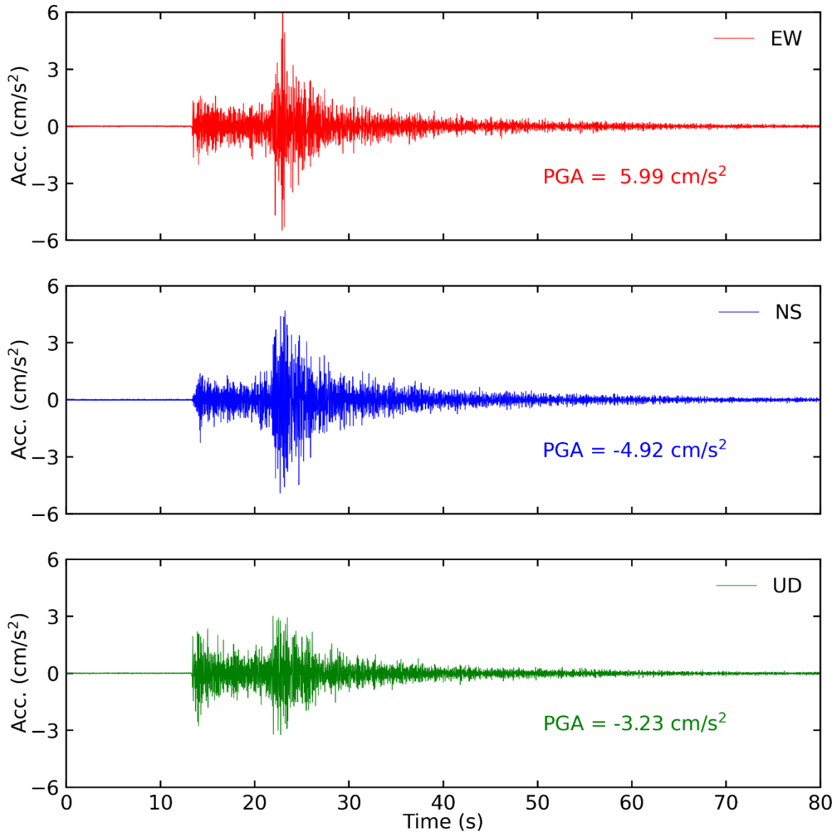
Tiempo historia en las tres direcciones (EW, NS y vertical) de la estación LIM026. Sismo de Callao-Callao del 25 de agosto del 2021 02:15:08 (hora local)
