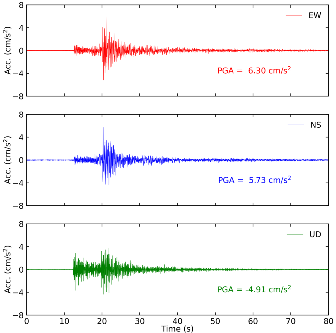
Tiempo historia en las tres direcciones (EW, NS y vertical) de la estación CAL005. Sismo de Callao-Callao del 25 de agosto del 2021 02:15:08 (hora local)
