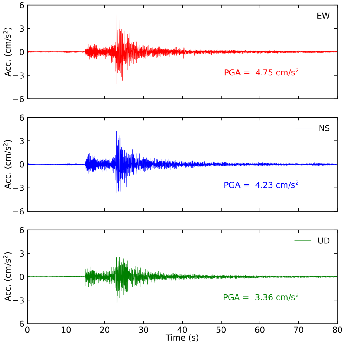
Tiempo historia en las tres direcciones (EW, NS y vertical) de la estación LIM013. Sismo de Callao-Callao del 25 de agosto del 2021 02:15:08 (hora local)
