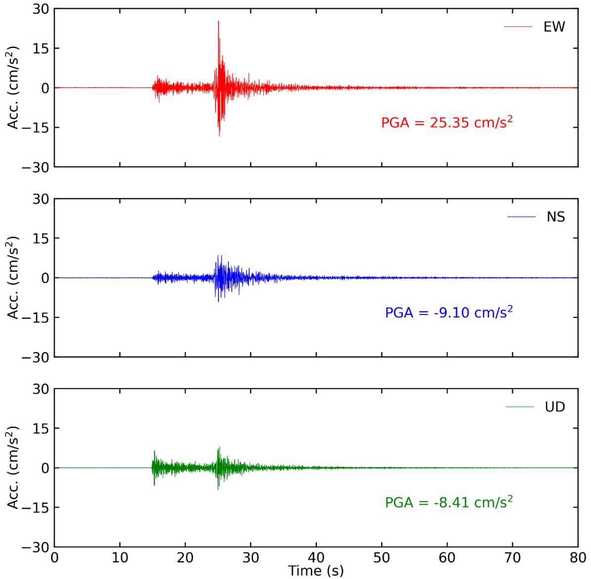
Tiempo historia en las tres direcciones (EW, NS y vertical) de la estación LIM030. Sismo de Callao-Callao del 25 de agosto del 2021 02:15:08 (hora local)
