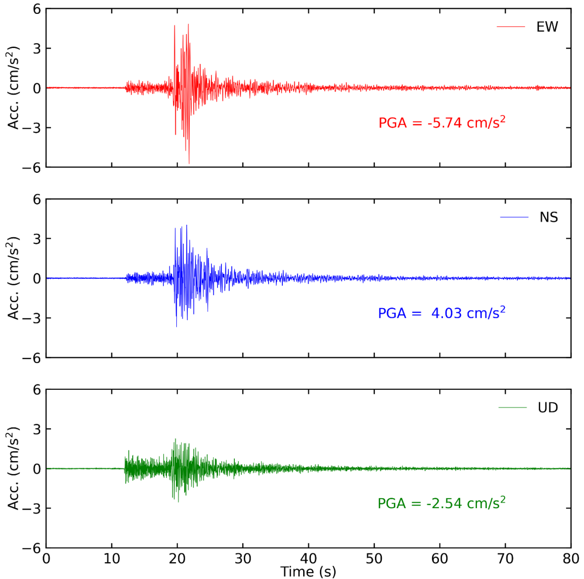
Tiempo historia en las tres direcciones (EW, NS y vertical) de la estación CAL003. Sismo de Callao-Callao del 25 de agosto del 2021 02:15:08 (hora local)
