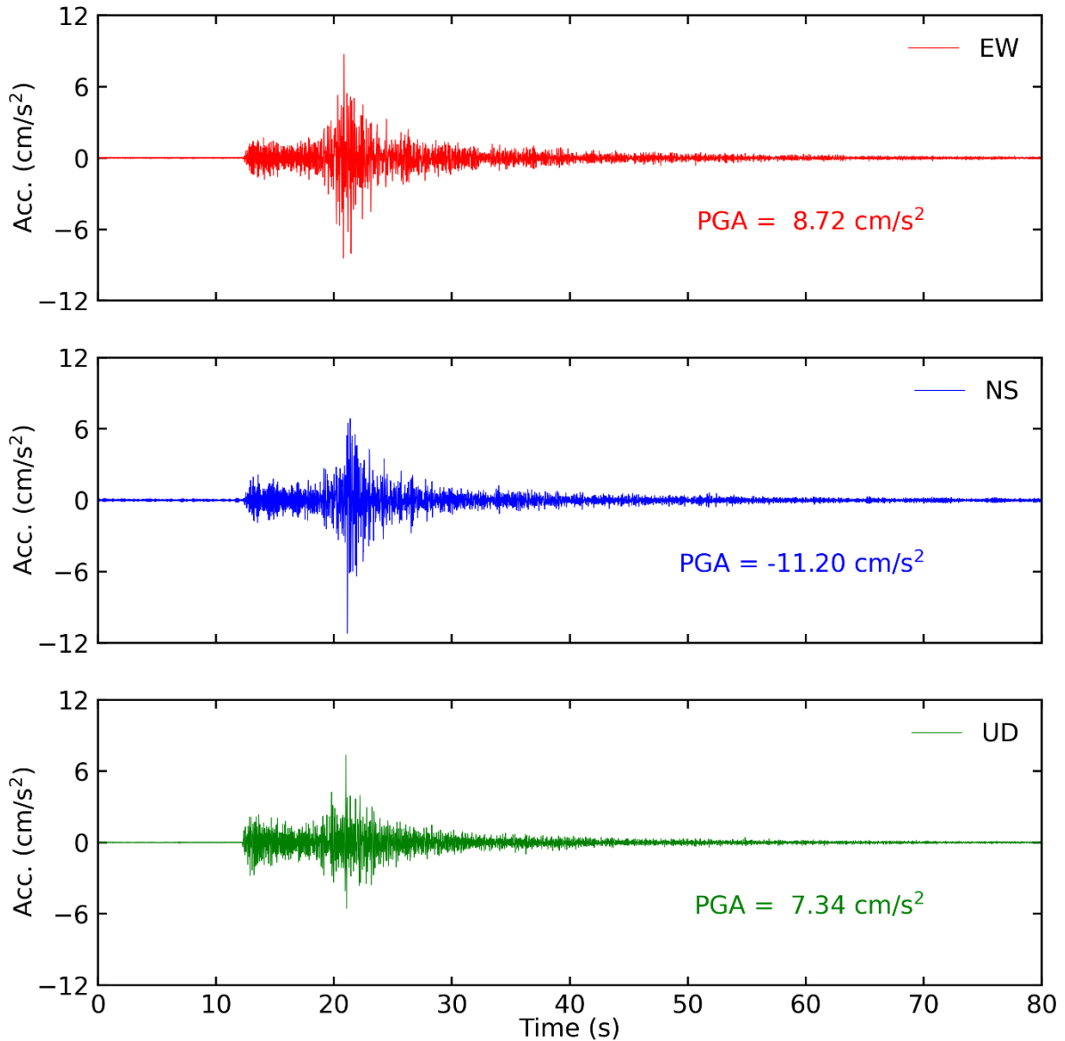
Tiempo historia en las tres direcciones (EW, NS y vertical) de la estación LIM029. Sismo de Callao-Callao del 25 de agosto del 2021 02:15:08 (hora local)
