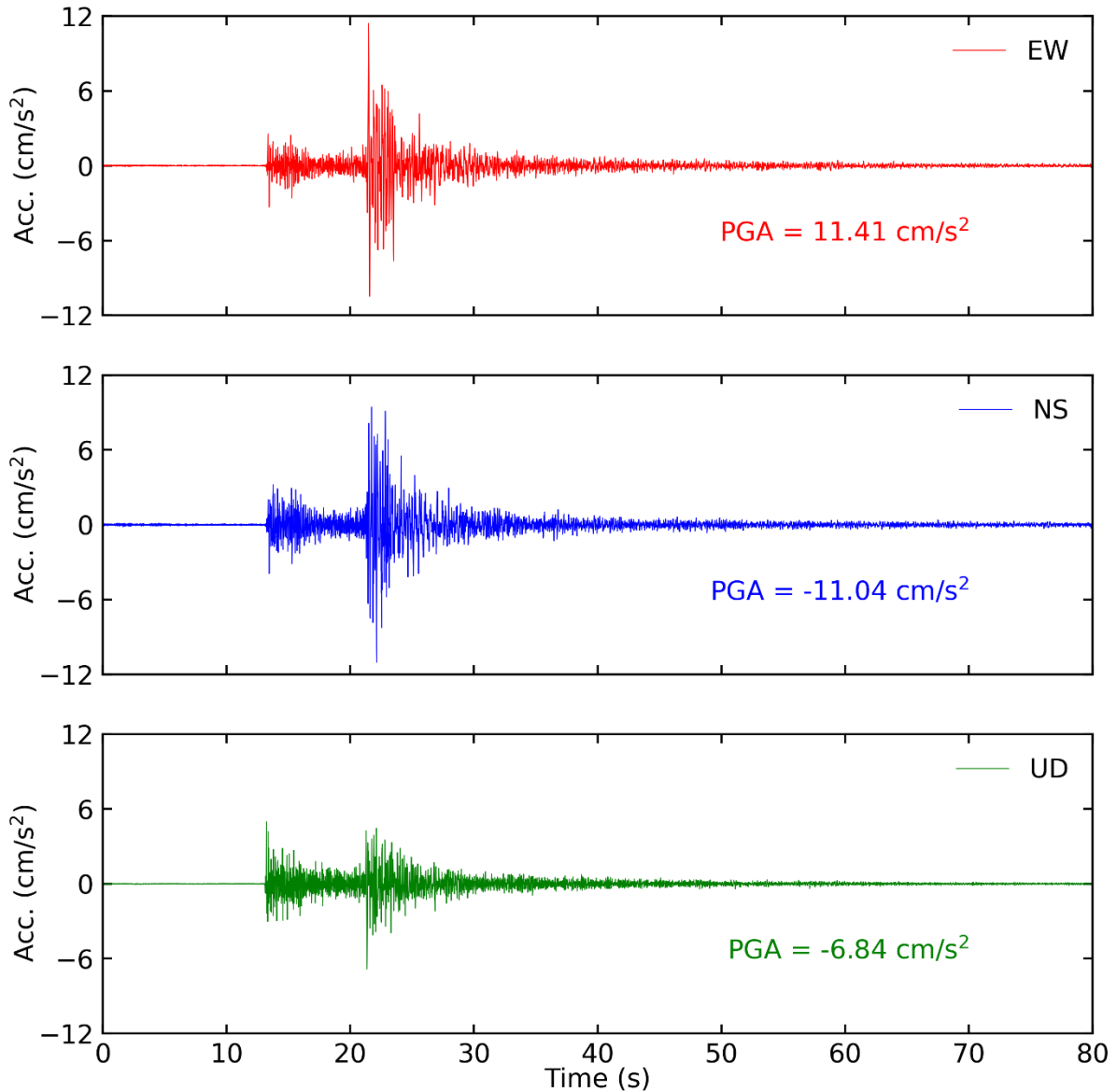
Tiempo historia en las tres direcciones (EW, NS y vertical) de la estación CAL006. Sismo de Callao-Callao del 25 de agosto del 2021 02:15:08 (hora local)
