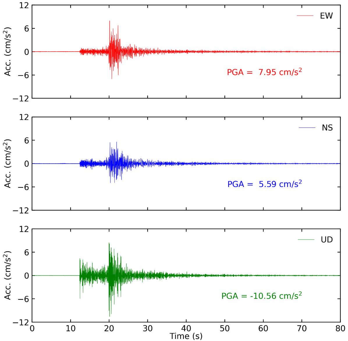
Tiempo historia en las tres direcciones (EW, NS y vertical) de la estación CAL004. Sismo de Callao-Callao del 25 de agosto del 2021 02:15:08 (hora local)
