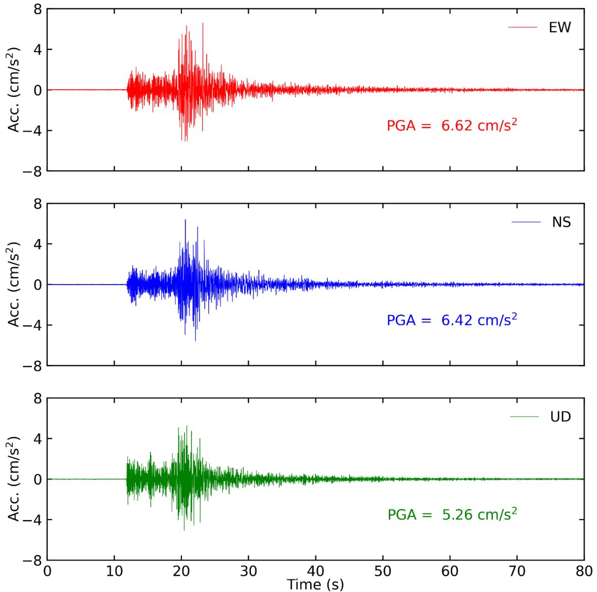
Tiempo historia en las tres direcciones (EW, NS y vertical) de la estación CAL002. Sismo de Callao-Callao del 25 de agosto del 2021 02:15:08 (hora local)
