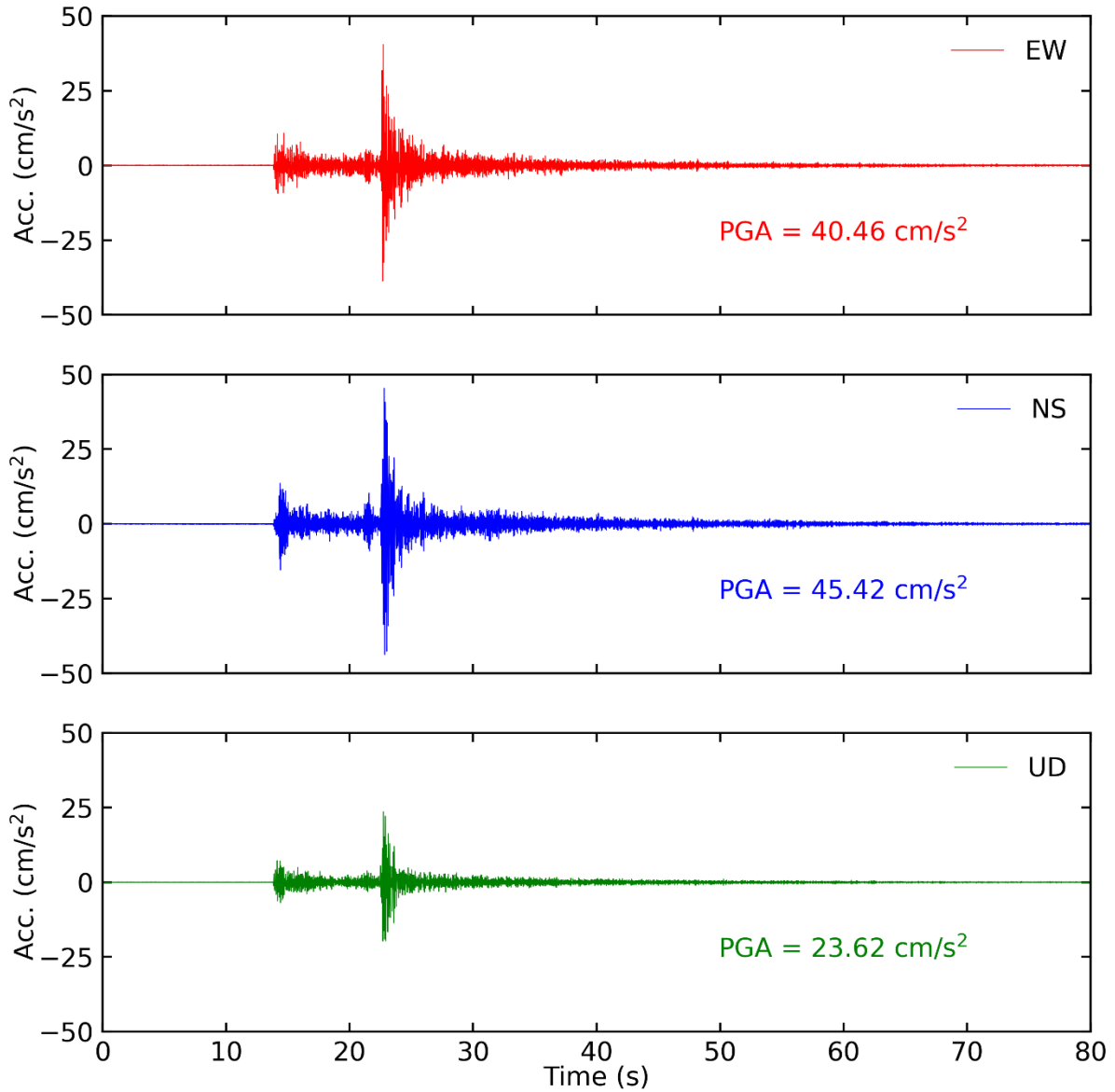
Tiempo historia en las tres direcciones (EW, NS y vertical) de la estación LIM031. Sismo de Callao-Callao del 25 de agosto del 2021 02:15:08 (hora local)
