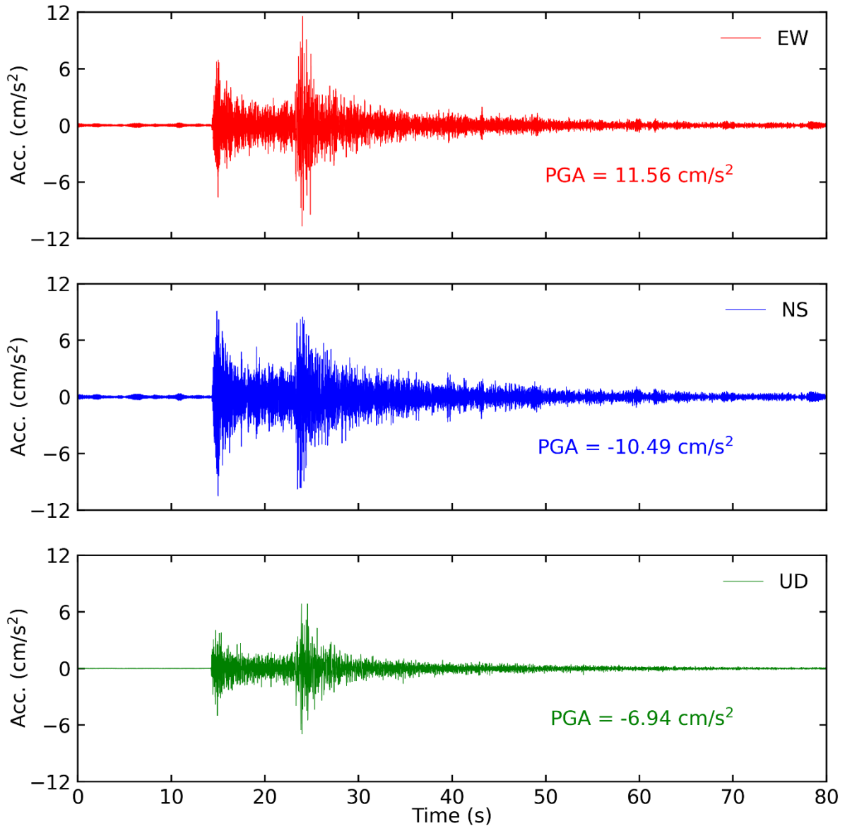
Tiempo historia en las tres direcciones (EW, NS y vertical) de la estación LIM010. Sismo de Callao-Callao del 25 de agosto del 2021 02:15:08 (hora local)
