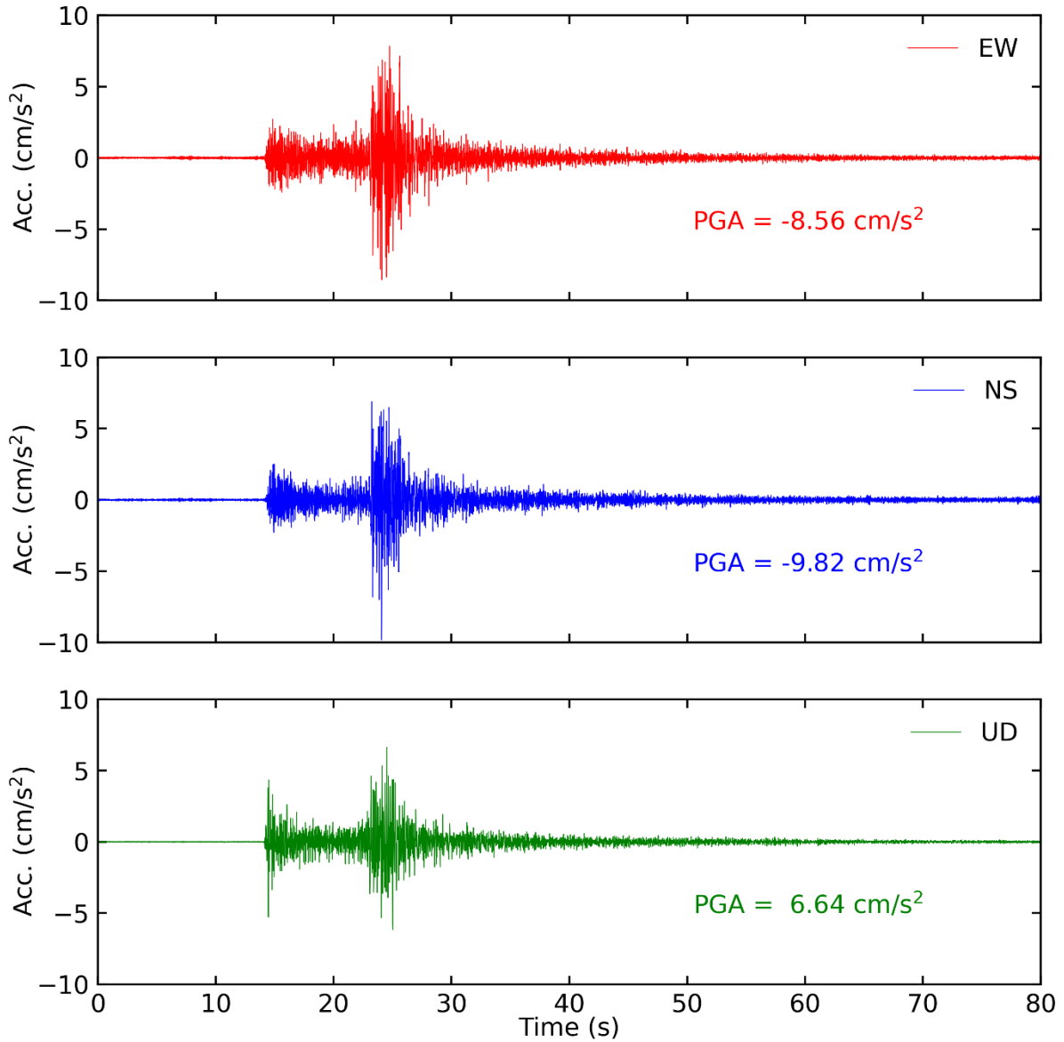
Tiempo historia en las tres direcciones (EW, NS y vertical) de la estación LIM016. Sismo de Callao-Callao del 25 de agosto del 2021 02:15:08 (hora local)
