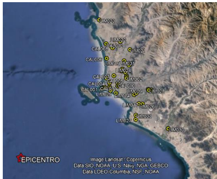
Figura N° 1. Ubicación del epicentro y estaciones acelerográficas.
