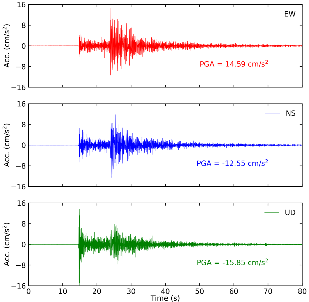
Tiempo historia en las tres direcciones (EW, NS y vertical) de la estación LIM023. Sismo de Callao-Callao del 25 de agosto del 2021 02:15:08 (hora local)
