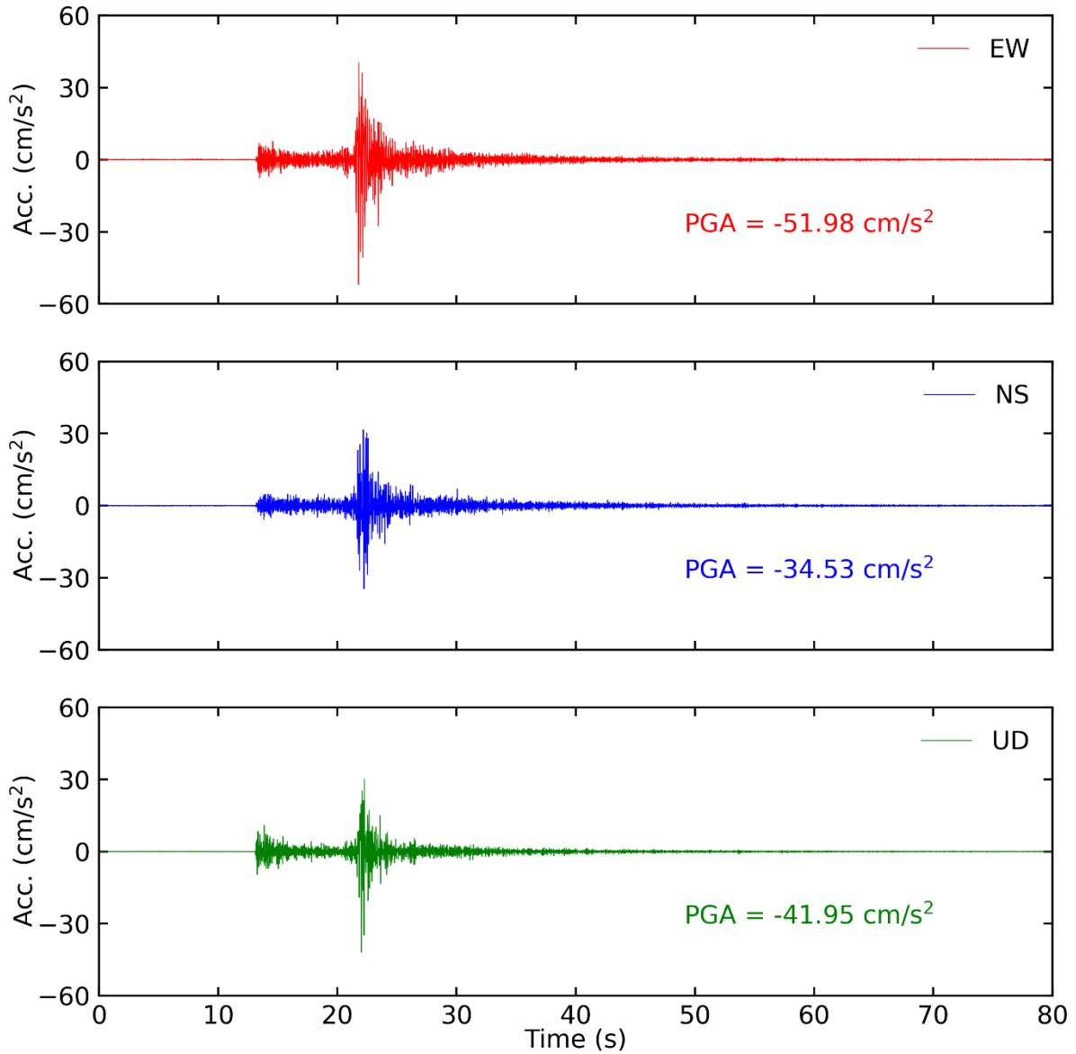
Tiempo historia en las tres direcciones (EW, NS y vertical) de la estación LIM024. Sismo de Callao-Callao del 25 de agosto del 2021 02:15:08 (hora local)
