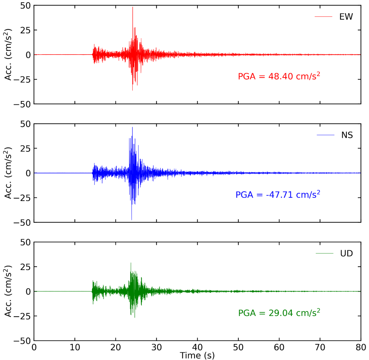
Tiempo historia en las tres direcciones (EW, NS y vertical) de la estación LIM028. Sismo de Callao-Callao del 25 de agosto del 2021 02:15:08 (hora local)
