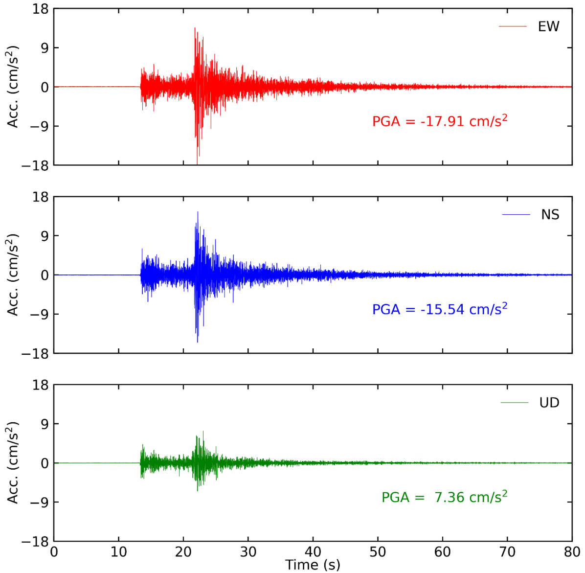
Tiempo historia en las tres direcciones (EW, NS y vertical) de la estación LIM001. Sismo de Callao-Callao del 25 de agosto del 2021 02:15:08 (hora local)
