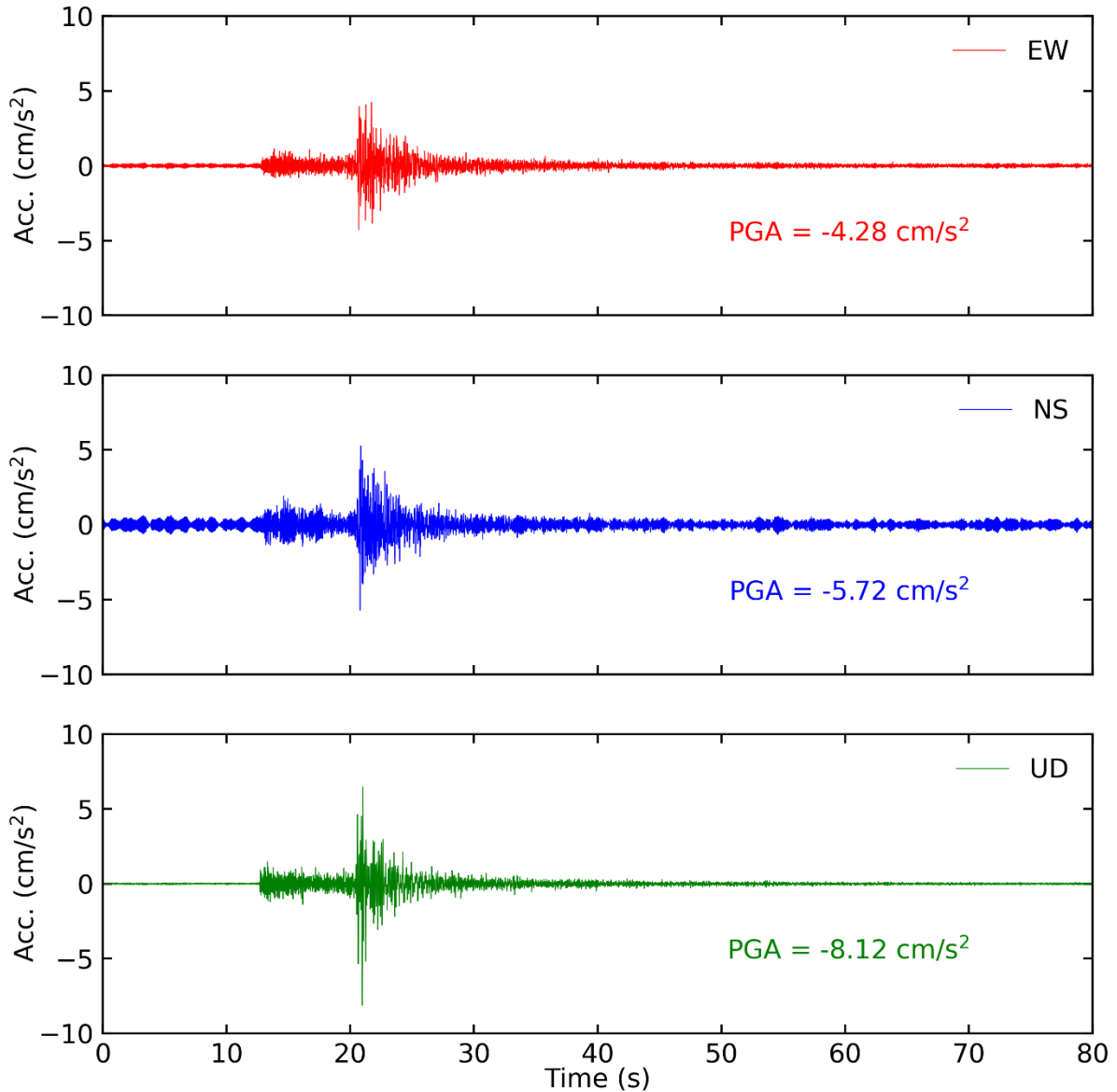
Tiempo historia en las tres direcciones (EW, NS y vertical) de la estación CAL010. Sismo de Callao-Callao del 25 de agosto del 2021 02:15:08 (hora local)
