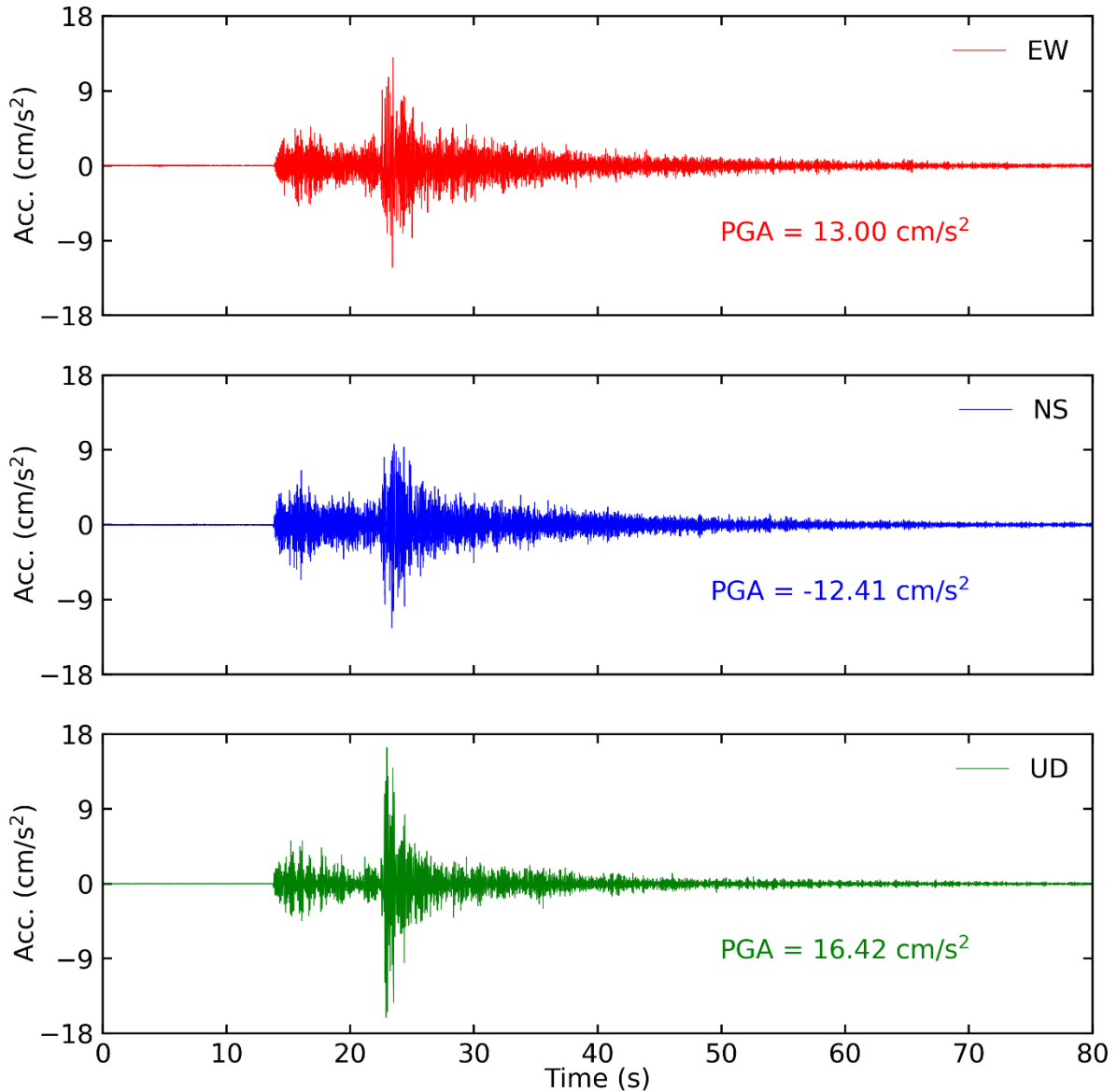
Tiempo historia en las tres direcciones (EW, NS y vertical) de la estación CAL008. Sismo de Callao-Callao del 25 de agosto del 2021 02:15:08 (hora local)
