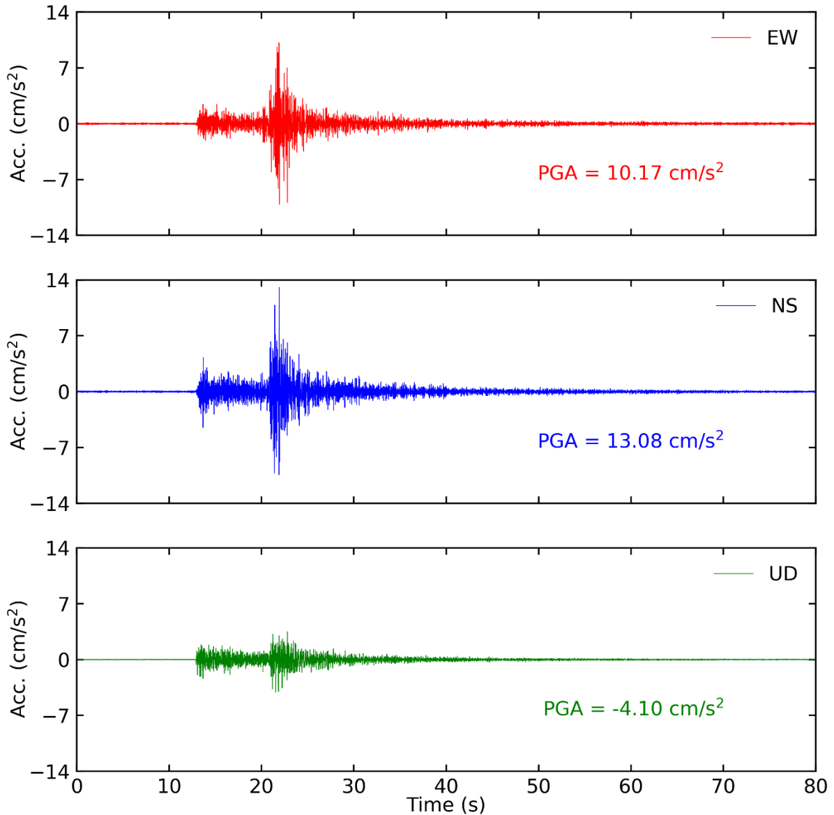
Tiempo historia en las tres direcciones (EW, NS y vertical) de la estación LIM027. Sismo de Callao-Callao del 25 de agosto del 2021 02:15:08 (hora local)
