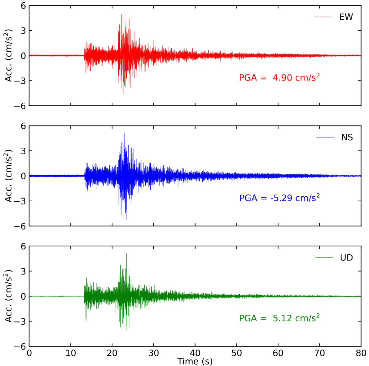
Tiempo historia en las tres direcciones (EW, NS y vertical) de la estación LIM014. Sismo de Callao-Callao del 25 de agosto del 2021 02:15:08 (hora local)
