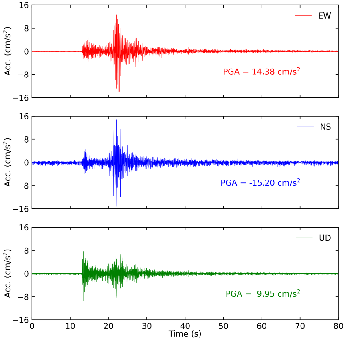
Tiempo historia en las tres direcciones (EW, NS y vertical) de la estación LIM033. Sismo de Callao-Callao del 25 de agosto del 2021 02:15:08 (hora local)
