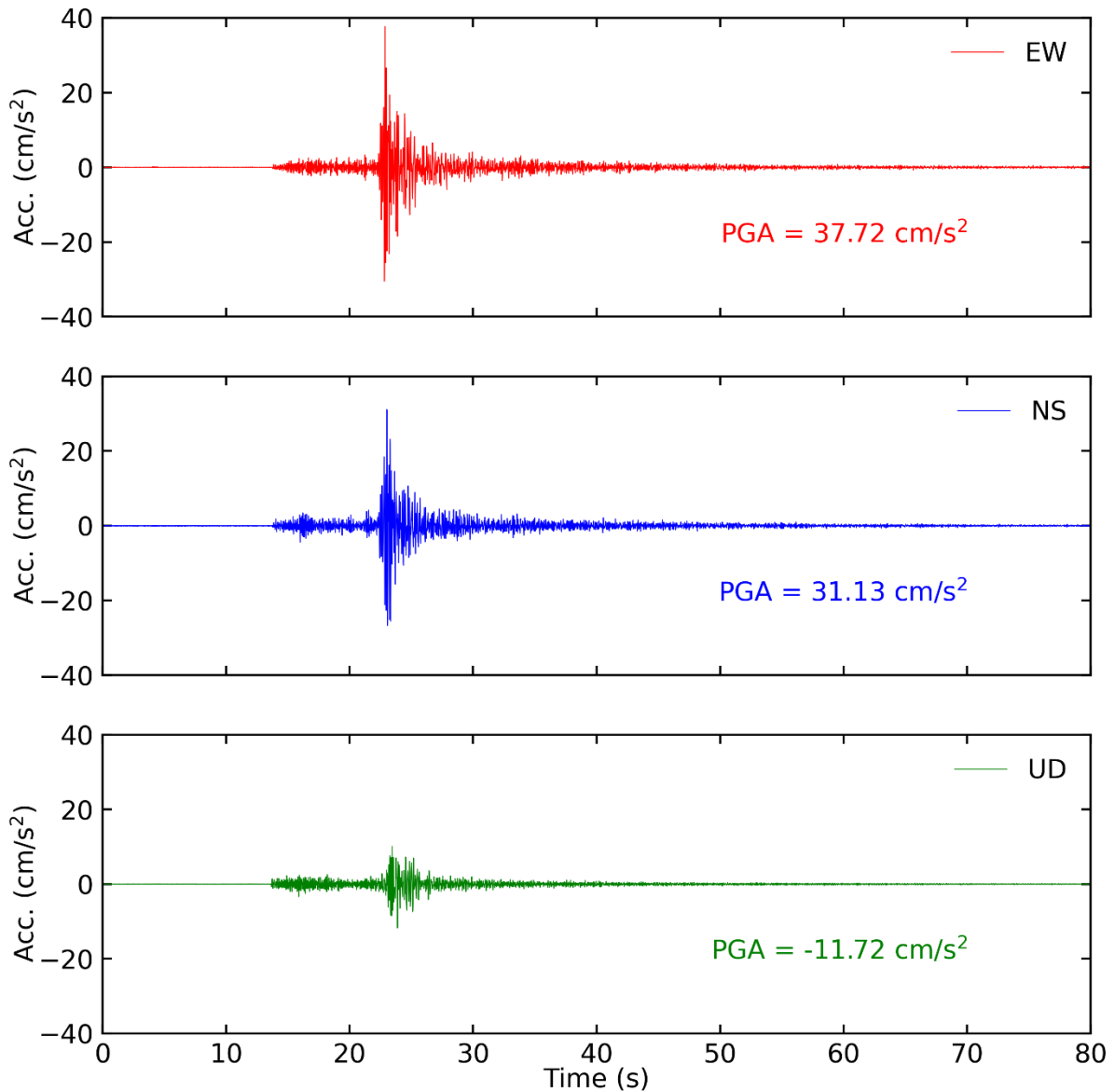
Tiempo historia en las tres direcciones (EW, NS y vertical) de la estación CAL012. Sismo de Callao-Callao del 25 de agosto del 2021 02:15:08 (hora local)
