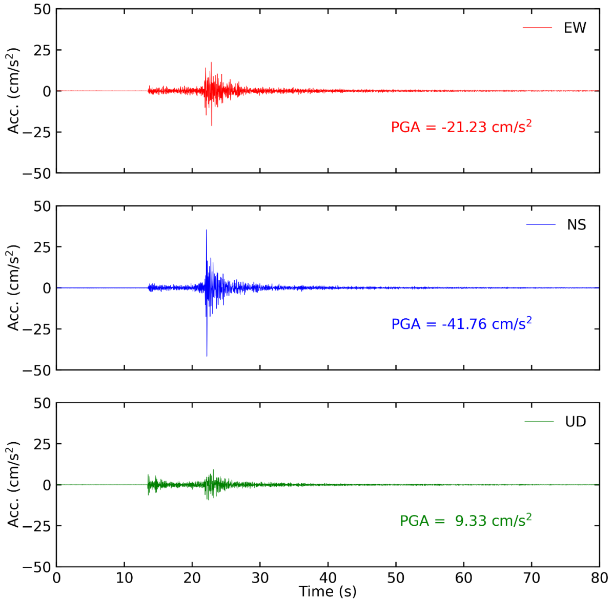
Tiempo historia en las tres direcciones (EW, NS y vertical) de la estación LIM032. Sismo de Callao-Callao del 25 de agosto del 2021 02:15:08 (hora local)
