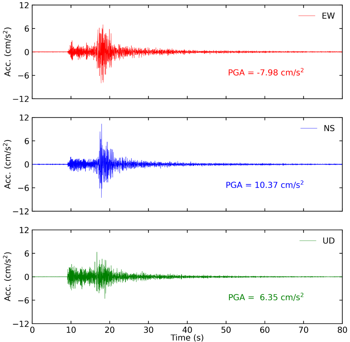
Tiempo historia en las tres direcciones (EW, NS y vertical) de la estación CAL011. Sismo de Callao-Callao del 25 de agosto del 2021 02:15:08 (hora local)
