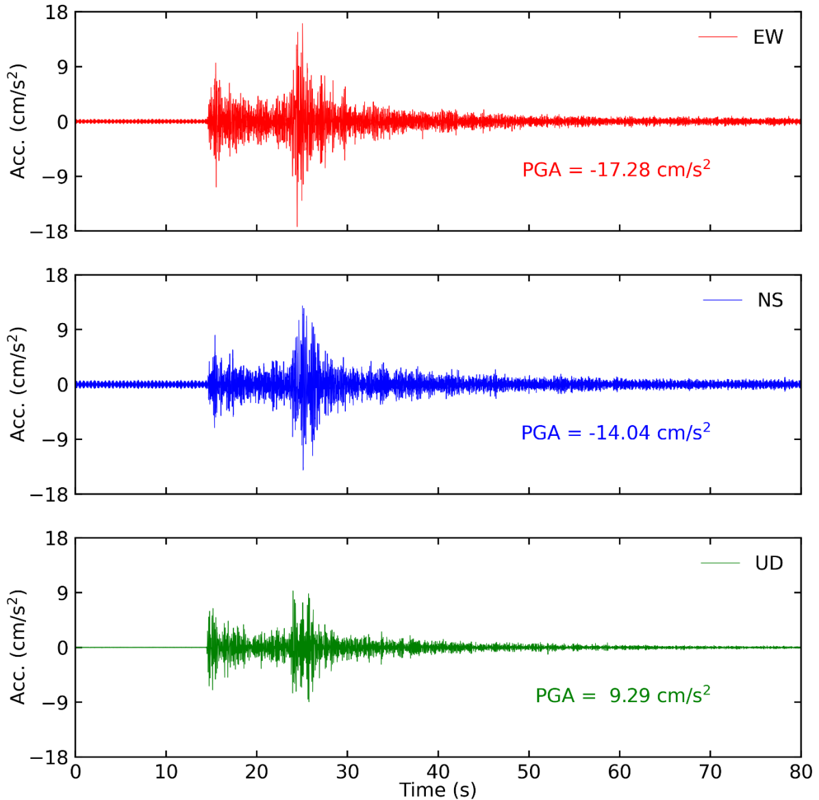
Tiempo historia en las tres direcciones (EW, NS y vertical) de la estación LIM021. Sismo de Callao-Callao del 25 de agosto del 2021 02:15:08 (hora local)
