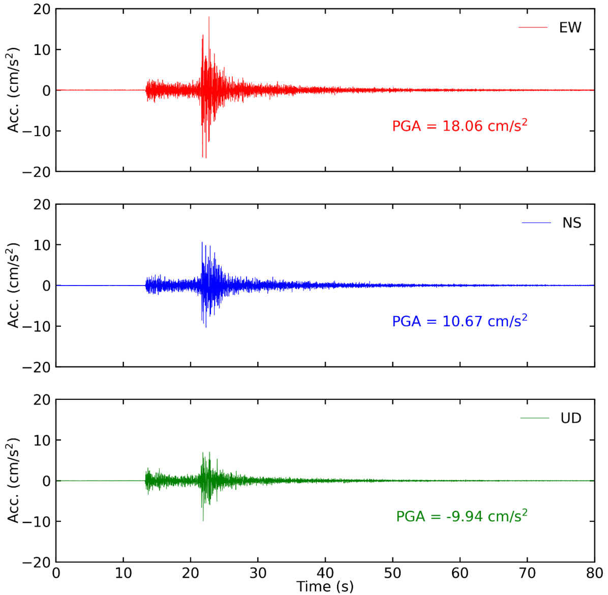
Tiempo historia en las tres direcciones (EW, NS y vertical) de la estación LIM002. Sismo de Callao-Callao del 25 de agosto del 2021 02:15:08 (hora local)
