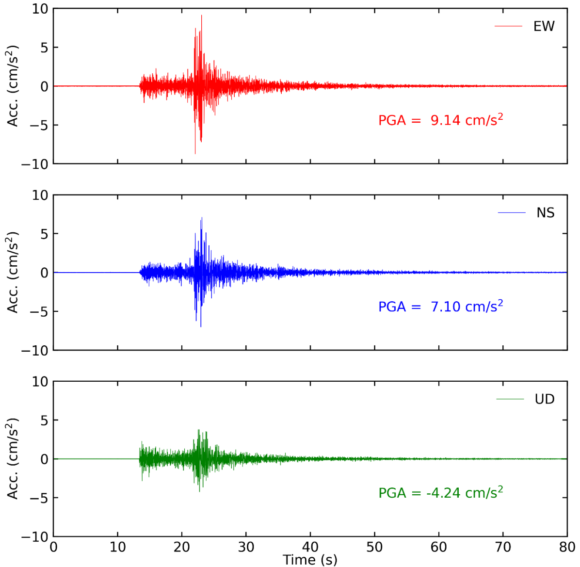
Tiempo historia en las tres direcciones (EW, NS y vertical) de la estación LIM009. Sismo de Callao-Callao del 25 de agosto del 2021 02:15:08 (hora local)
