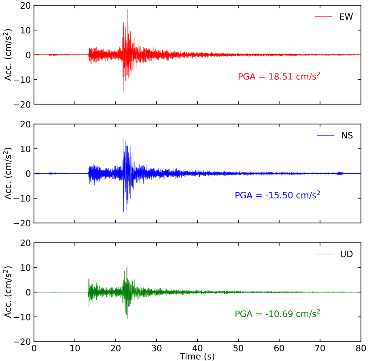
Tiempo historia en las tres direcciones (EW, NS y vertical) de la estación LIM018. Sismo de Callao-Callao del 25 de agosto del 2021 02:15:08 (hora local)
