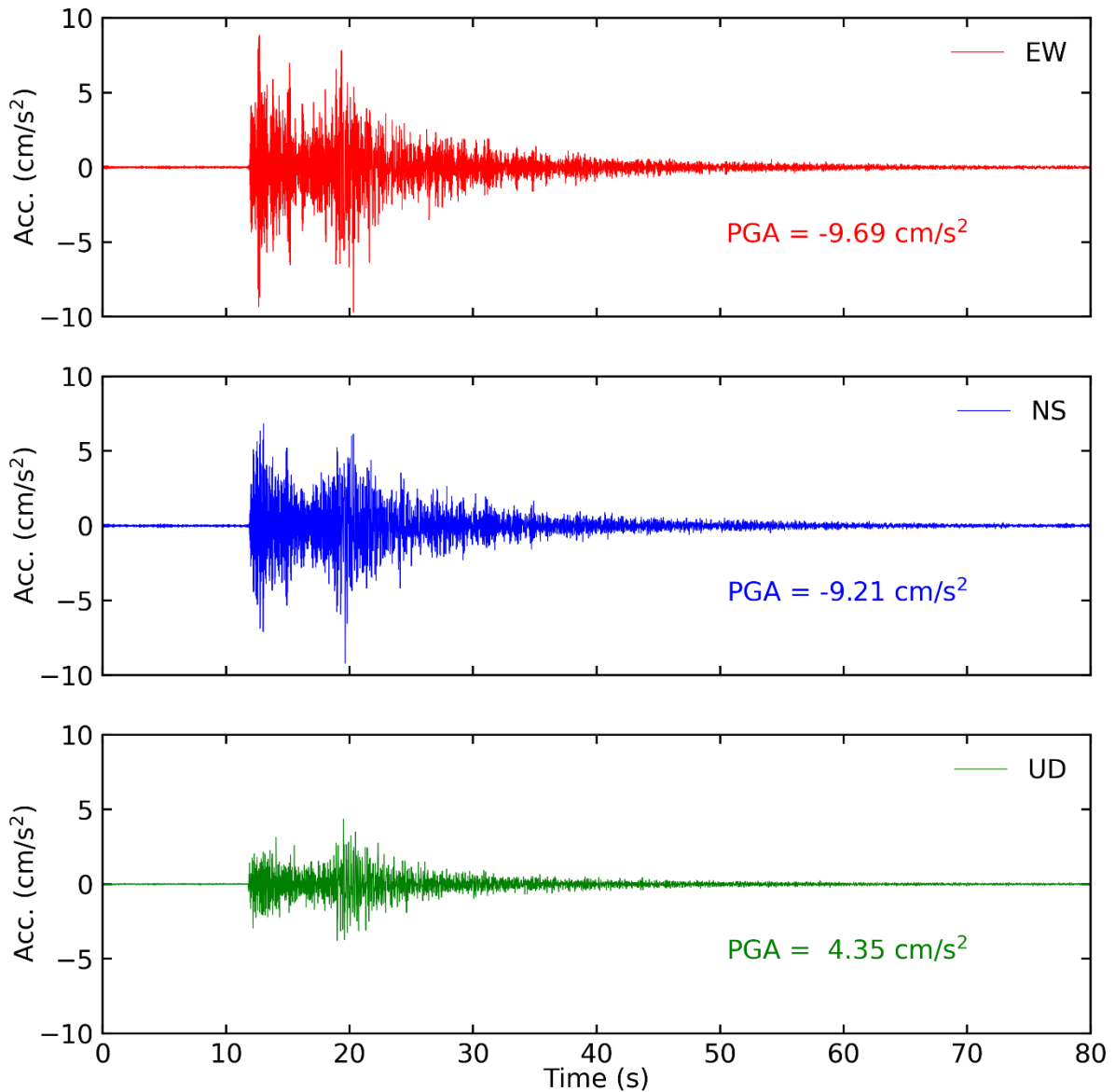
Tiempo historia en las tres direcciones (EW, NS y vertical) de la estación CAL001. Sismo de Callao-Callao del 25 de agosto del 2021 02:15:08 (hora local)
