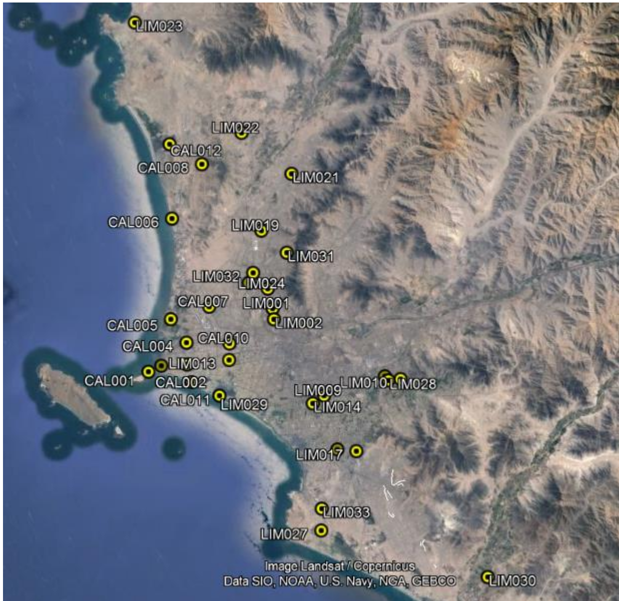
Figura Nº 2 Mapa de ubicación de las estaciones acelerográficas en la ciudad de Lima
