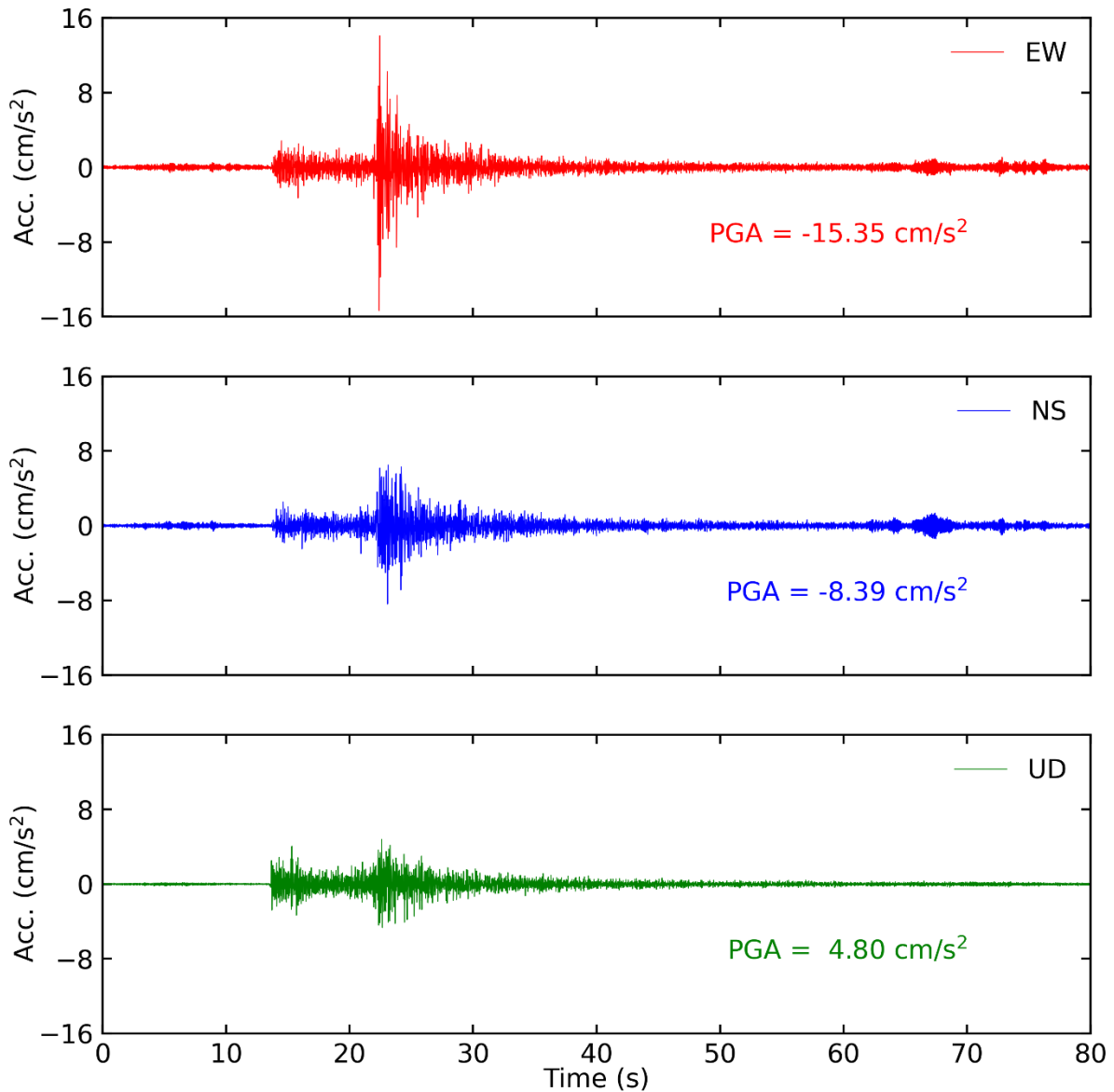
Tiempo historia en las tres direcciones (EW, NS y vertical) de la estación LIM017. Sismo de Callao-Callao del 25 de agosto del 2021 02:15:08 (hora local)
