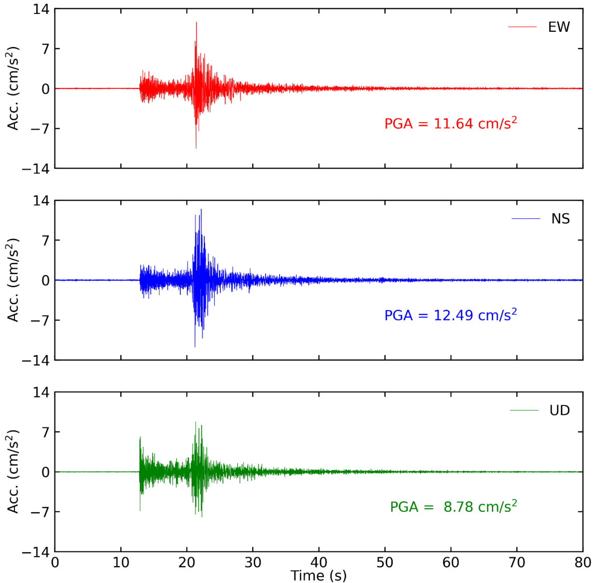
Tiempo historia en las tres direcciones (EW, NS y vertical) de la estación CAL007. Sismo de Callao-Callao del 25 de agosto del 2021 02:15:08 (hora local)
