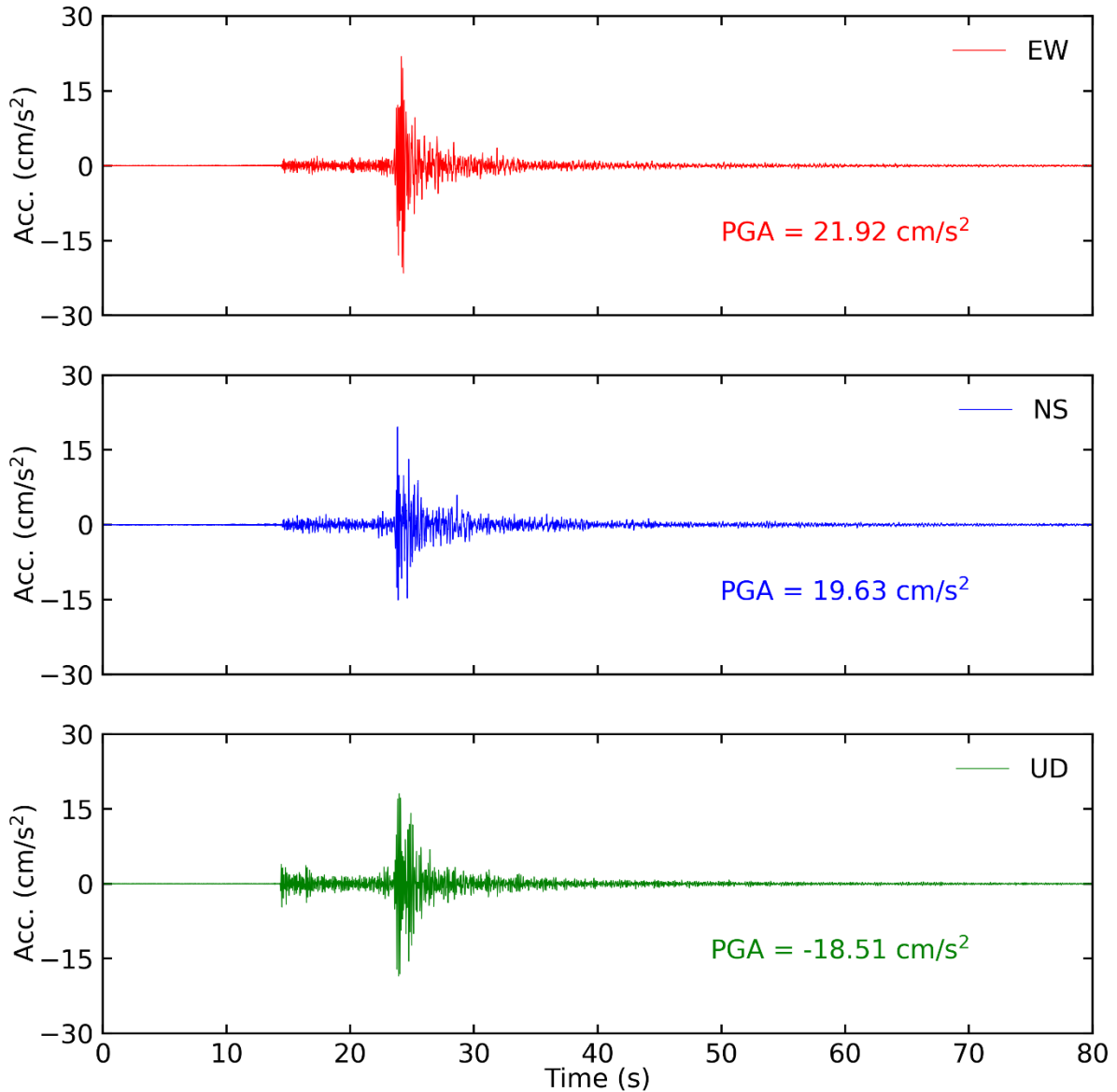
Tiempo historia en las tres direcciones (EW, NS y vertical) de la estación LIM022. Sismo de Callao-Callao del 25 de agosto del 2021 02:15:08 (hora local)
