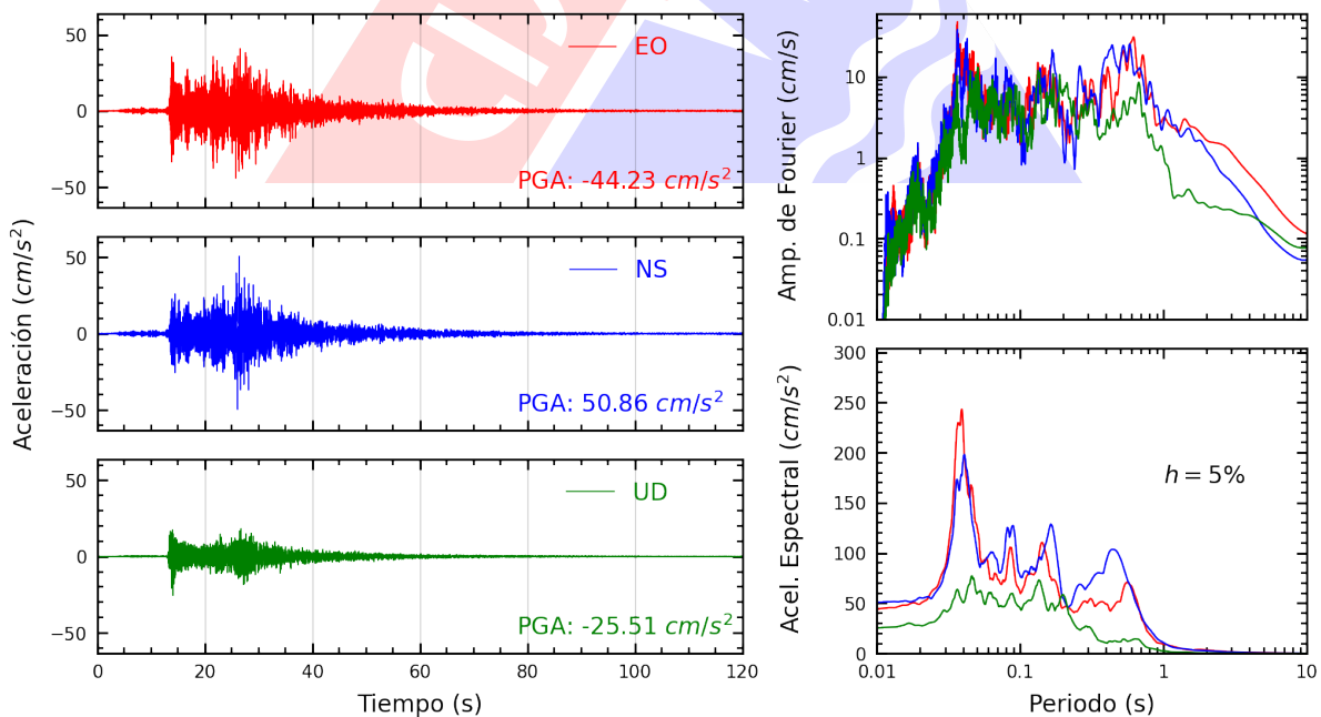
Figura A.24: Registros tiempo-historia, espectros de Fourier y de respuesta en las direcciones EO, NS y UD de la estación CAL001. Sismo de Lima, Lima - Lima de 2022-01-07, 05:27:05 (Hora local)
