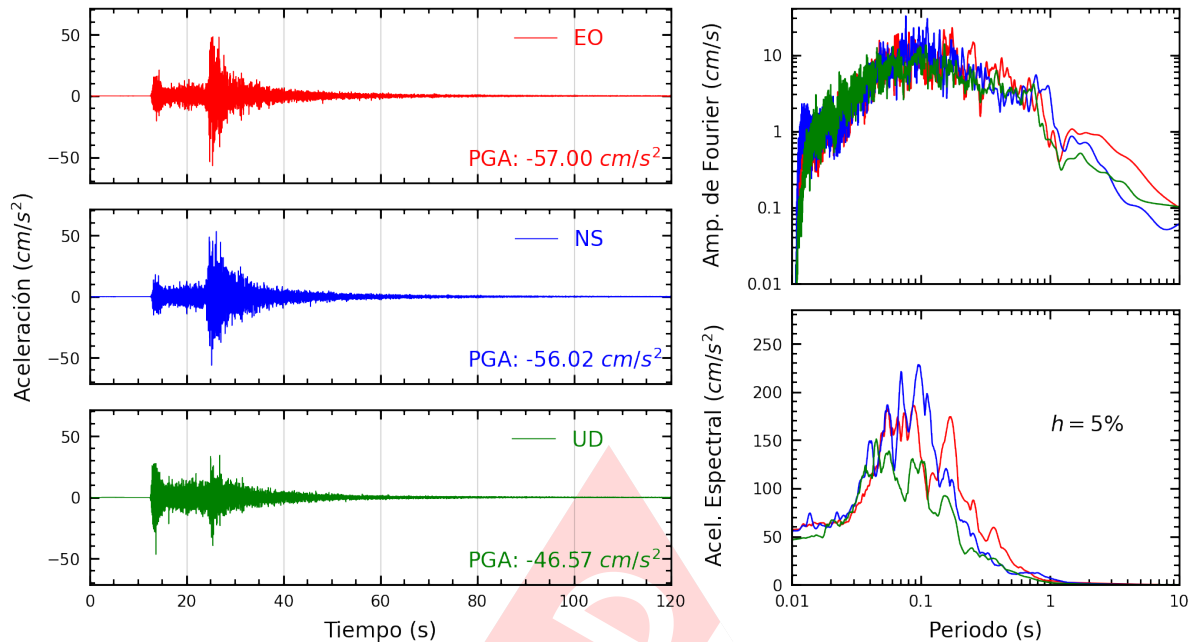
Figura A.19: Registros tiempo-historia, espectros de Fourier y de respuesta en las direcciones EO, NS y UD de la estación LIM026. Sismo de Lima, Lima - Lima de 2022-01-07, 05:27:05 (Hora local)
