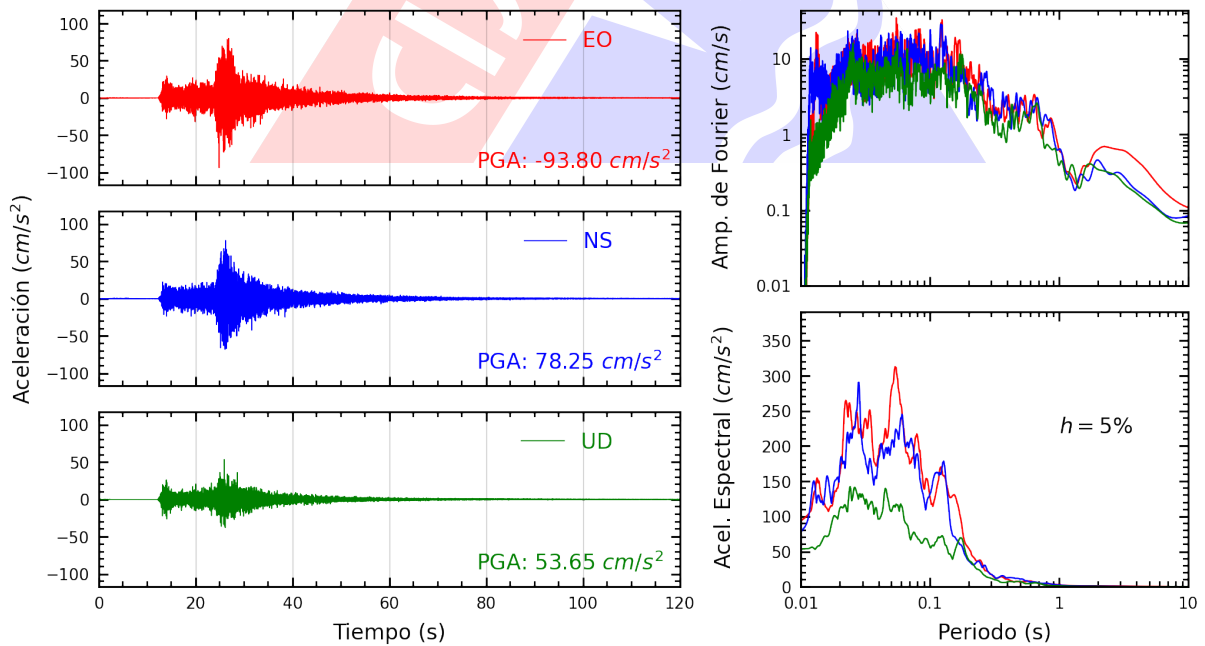
Figura A.12: Registros tiempo-historia, espectros de Fourier y de respuesta en las direcciones EO, NS y UD de la estación LIM002. Sismo de Lima, Lima - Lima de 2022-01-07, 05:27:05 (Hora local)
