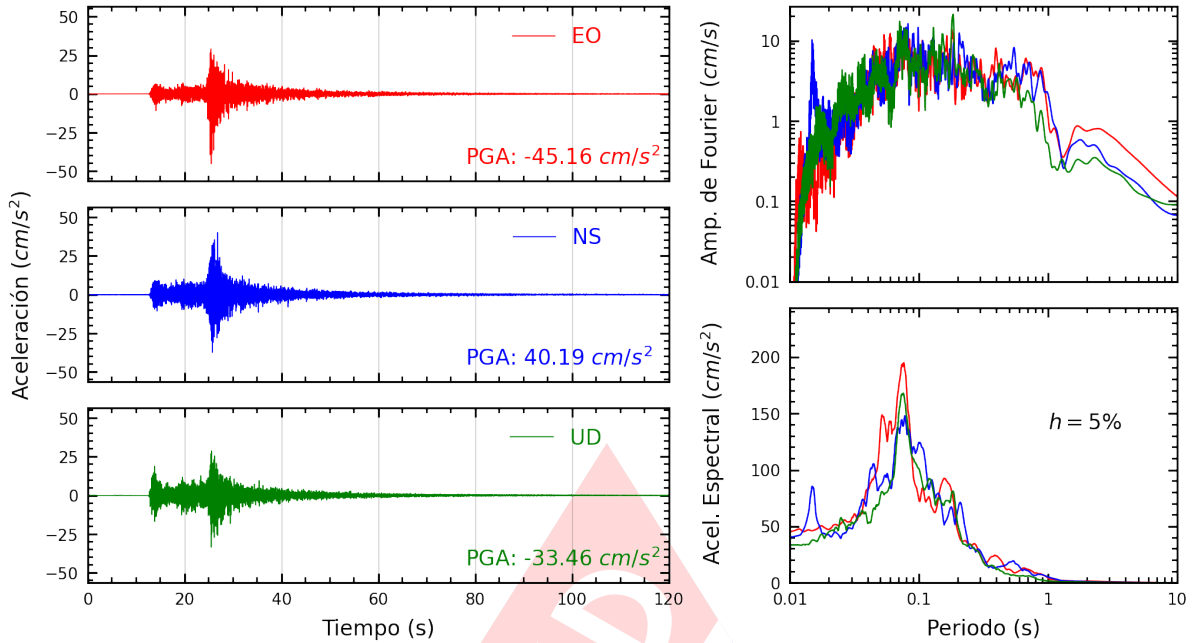
Figura A.27: Registros tiempo-historia, espectros de Fourier y de respuesta en las direcciones EO, NS y UD de la estación LIM012. Sismo de Lima, Lima - Lima de 2022-01-07, 05:27:05 (Hora local)
