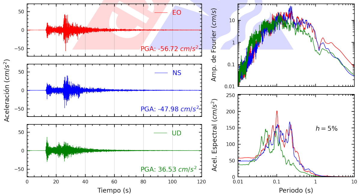
Figura A.20: Registros tiempo-historia, espectros de Fourier y de respuesta en las direcciones EO, NS y UD de la estación LIM033. Sismo de Lima, Lima - Lima de 2022-01-07, 05:27:05 (Hora local)
