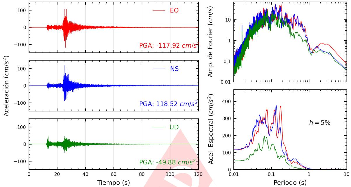
Figura A.9: Registros tiempo-historia, espectros de Fourier y de respuesta en las direcciones EO, NS y UD de la estación LIM032. Sismo de Lima, Lima - Lima de 2022-01-07, 05:27:05 (Hora local)
