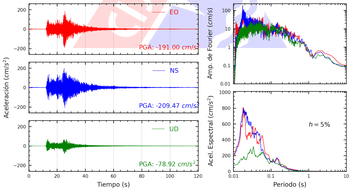
Figura A.4: Registros tiempo-historia, espectros de Fourier y de respuesta en las direcciones EO, NS y UD de la estación LIM010. Sismo de Lima, Lima - Lima de 2022-01-07, 05:27:05 (Hora local)
