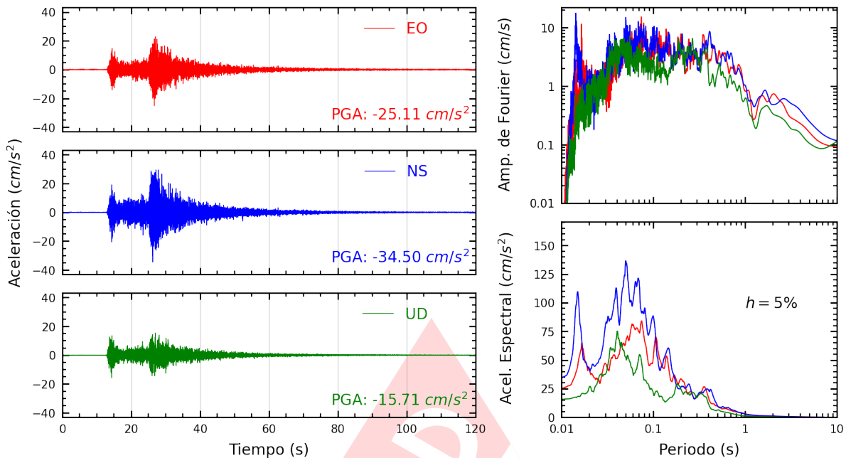
Figura A.29: Registros tiempo-historia, espectros de Fourier y de respuesta en las direcciones EO, NS y UD de la estación LIM027. Sismo de Lima, Lima - Lima de 2022-01-07, 05:27:05 (Hora local)
