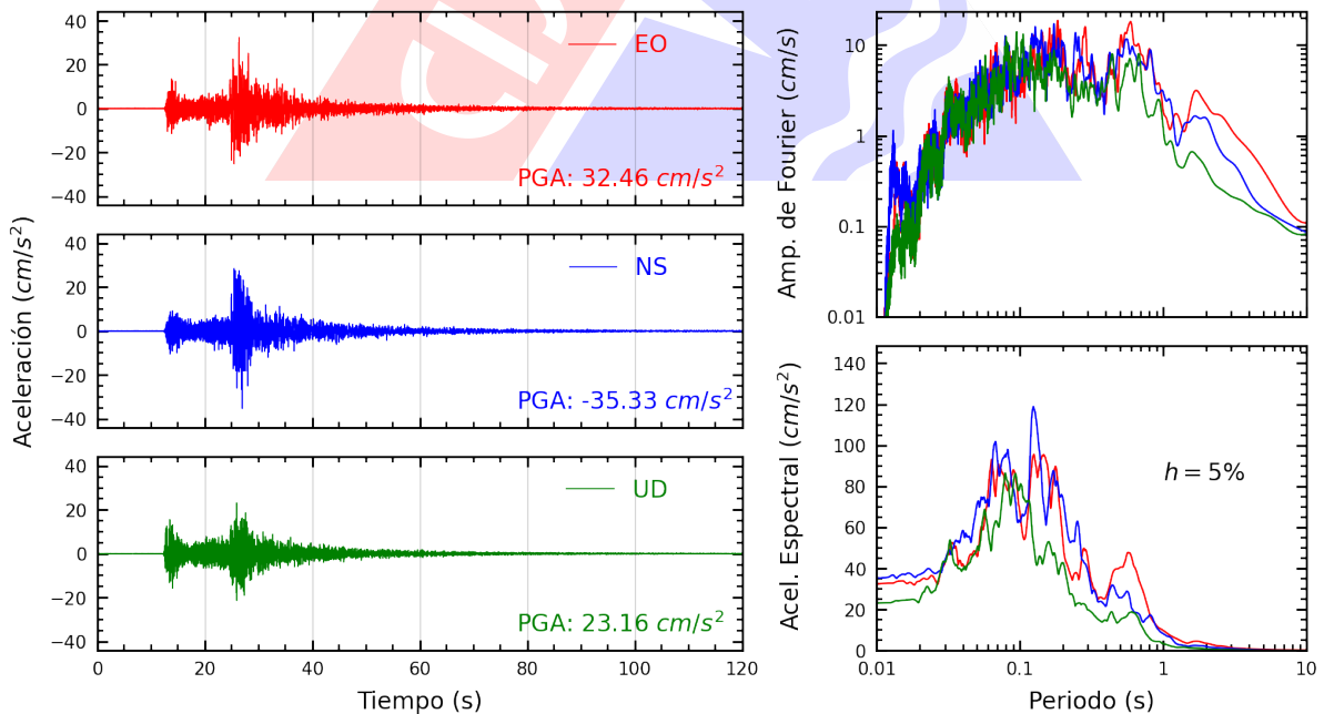
Figura A.28: Registros tiempo-historia, espectros de Fourier y de respuesta en las direcciones EO, NS y UD de la estación CAL002. Sismo de Lima, Lima - Lima de 2022-01-07, 05:27:05 (Hora local)
