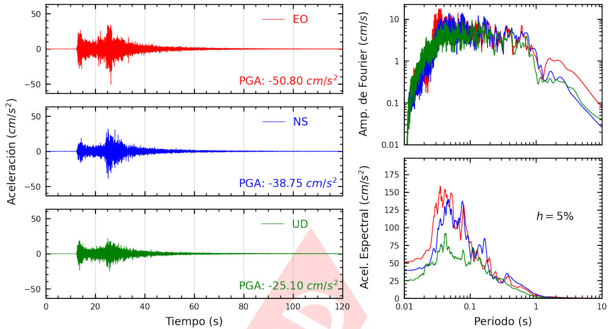
Figura A.25: Registros tiempo-historia, espectros de Fourier y de respuesta en las direcciones EO, NS y UD de la estación LIM009. Sismo de Lima, Lima - Lima de 2022-01-07, 05:27:05 (Hora local)
