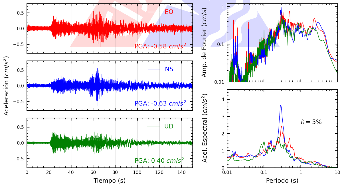
Figura A.32: Registros tiempo-historia, espectros de Fourier y de respuesta en las direcciones EO, NS y UD de la estación AYA001. Sismo de Lima, Lima - Lima de 2022-01-07, 05:27:05 (Hora local)
