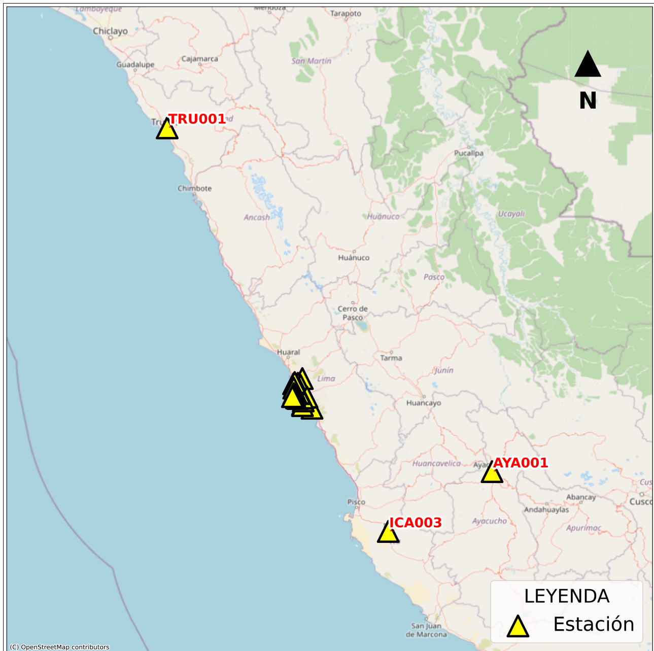
Figura 2: Mapa de ubicación de las estaciones acelerográficas a nivel nacional que registraron el Sismo de Lima, Lima - Lima del 07 de enero de 2022 a las 05:27:05 (hora local)
