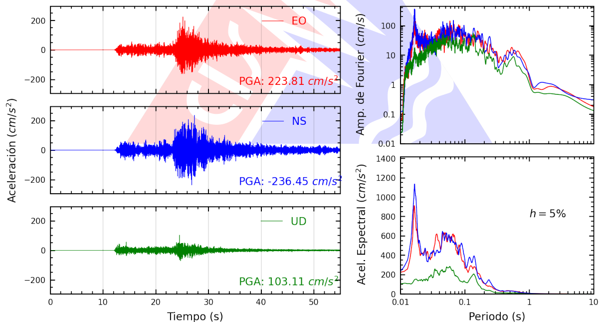
Figura A.2: Registros tiempo-historia, espectros de Fourier y de respuesta en las direcciones EO, NS y UD de la estación LIM034. Sismo de Lima, Lima - Lima de 2022-01-07, 05:27:05 (Hora local)
