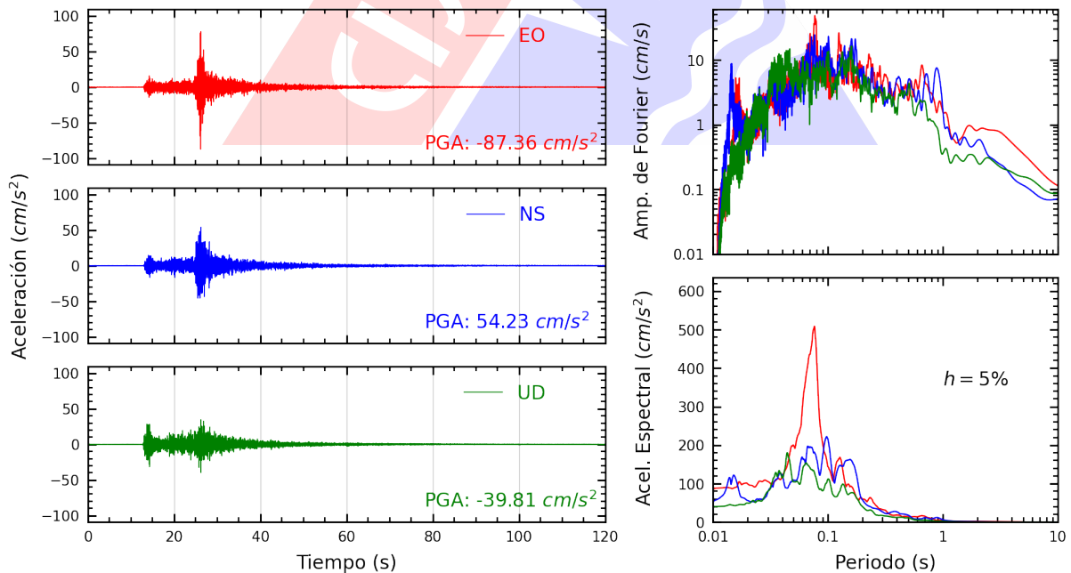
Figura A.14: Registros tiempo-historia, espectros de Fourier y de respuesta en las direcciones EO, NS y UD de la estación LIM029. Sismo de Lima, Lima - Lima de 2022-01-07, 05:27:05 (Hora local)
