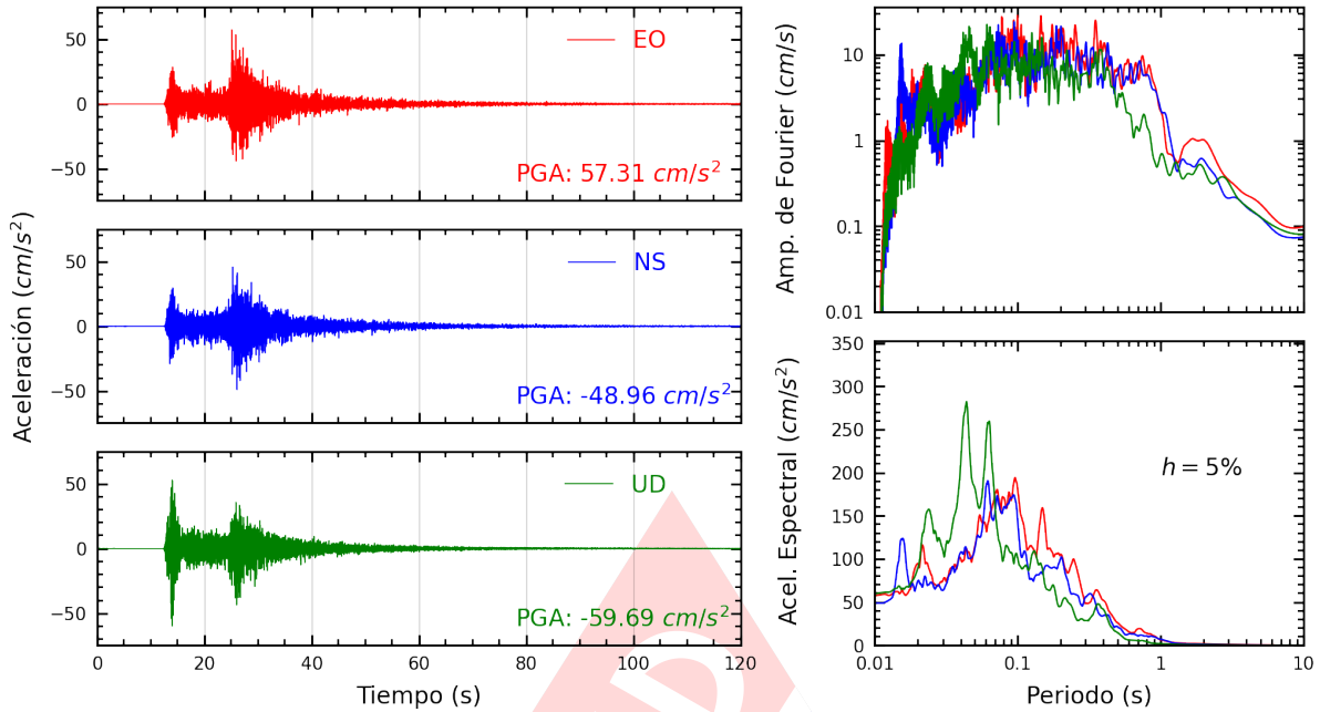
Figura A.17: Registros tiempo-historia, espectros de Fourier y de respuesta en las direcciones EO, NS y UD de la estación LIM030. Sismo de Lima, Lima - Lima de 2022-01-07, 05:27:05 (Hora local)
