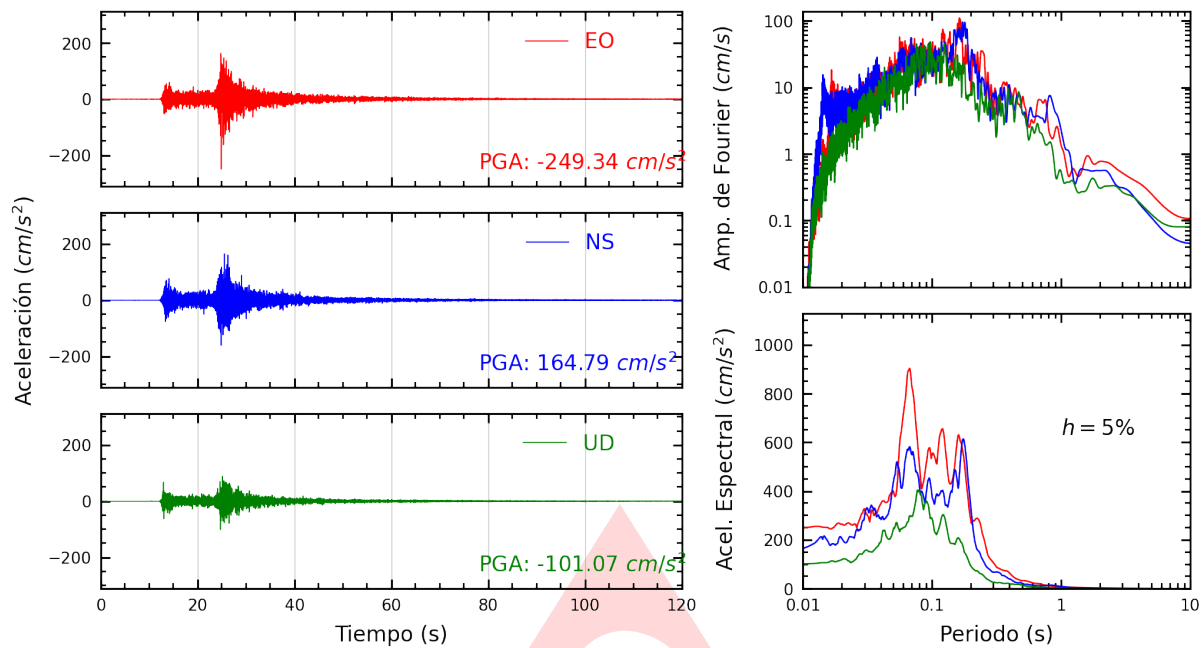
Figura A.1: Registros tiempo-historia, espectros de Fourier y de respuesta en las direcciones EO, NS y UD de la estación LIM028. Sismo de Lima, Lima - Lima de 2022-01-07, 05:27:05 (Hora local)
