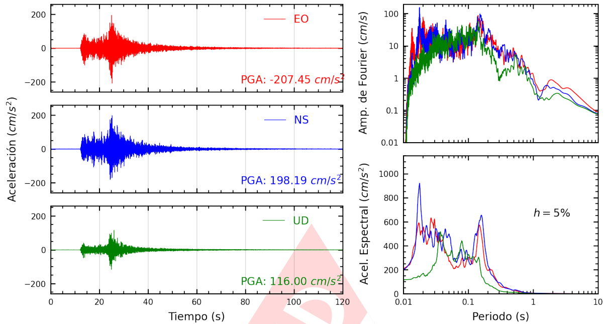
Figura A.5: Registros tiempo-historia, espectros de Fourier y de respuesta en las direcciones EO, NS y UD de la estación LIM021. Sismo de Lima, Lima - Lima de 2022-01-07, 05:27:05 (Hora local)
