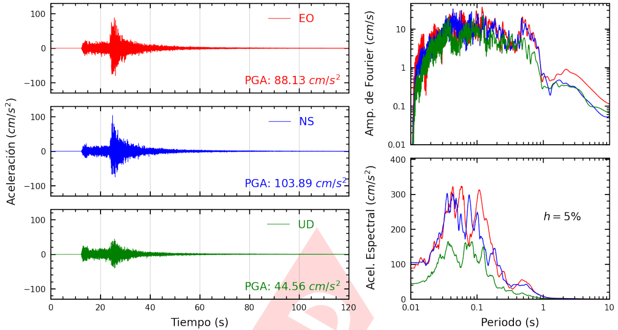
Figura A.11: Registros tiempo-historia, espectros de Fourier y de respuesta en las direcciones EO, NS y UD de la estación LIM019. Sismo de Lima, Lima - Lima de 2022-01-07, 05:27:05 (Hora local)
