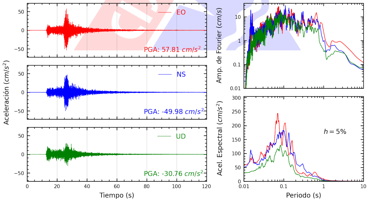
Figura A.18: Registros tiempo-historia, espectros de Fourier y de respuesta en las direcciones EO, NS y UD de la estación CAL007. Sismo de Lima, Lima - Lima de 2022-01-07, 05:27:05 (Hora local)
