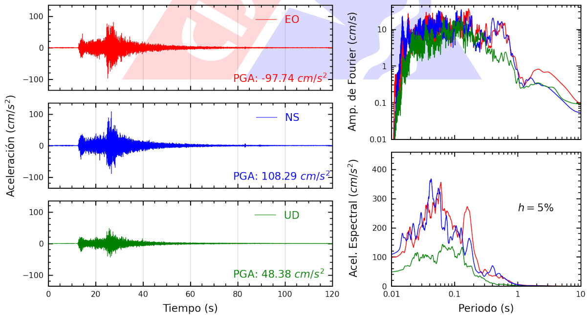
Figura A.10: Registros tiempo-historia, espectros de Fourier y de respuesta en las direcciones EO, NS y UD de la estación LIM018. Sismo de Lima, Lima - Lima de 2022-01-07, 05:27:05 (Hora local)
