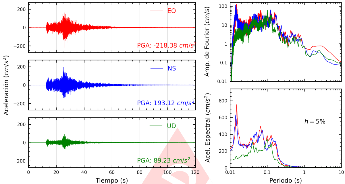
Figura A.3: Registros tiempo-historia, espectros de Fourier y de respuesta en las direcciones EO, NS y UD de la estación CAL008. Sismo de Lima, Lima - Lima de 2022-01-07, 05:27:05 (Hora local)
