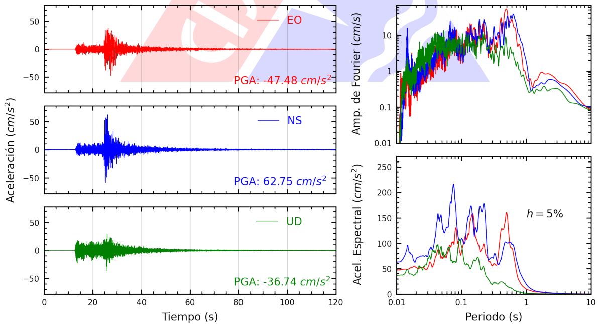
Figura A.16: Registros tiempo-historia, espectros de Fourier y de respuesta en las direcciones EO, NS y UD de la estación CAL006. Sismo de Lima, Lima - Lima de 2022-01-07, 05:27:05 (Hora local)
