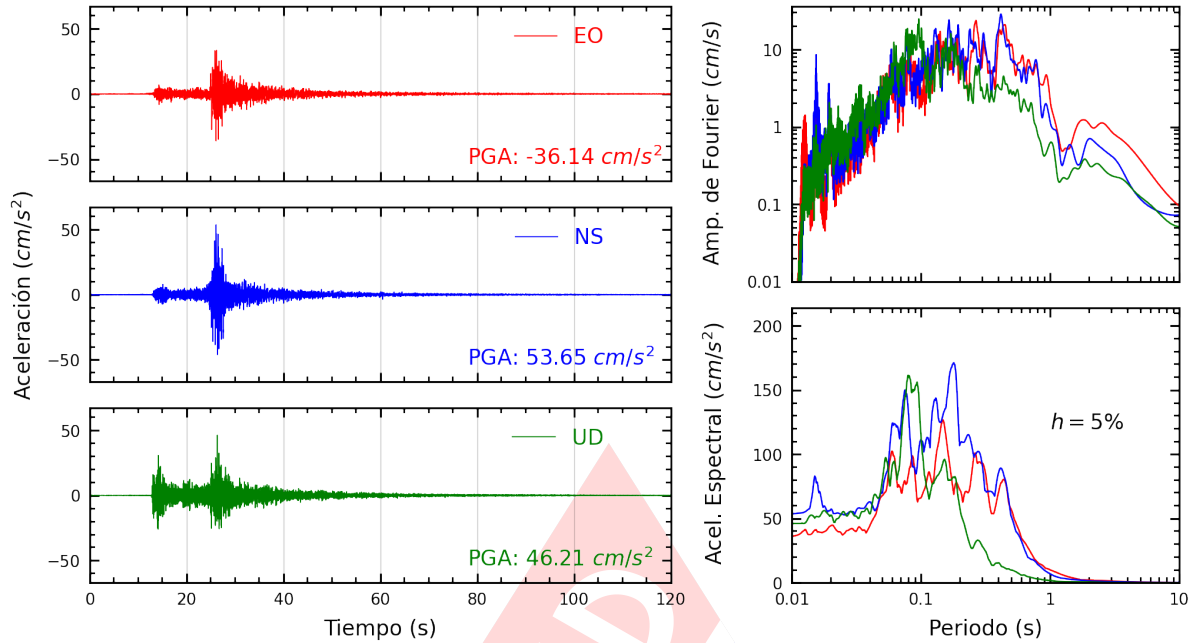
Figura A.21: Registros tiempo-historia, espectros de Fourier y de respuesta en las direcciones EO, NS y UD de la estación CAL004. Sismo de Lima, Lima - Lima de 2022-01-07, 05:27:05 (Hora local)
