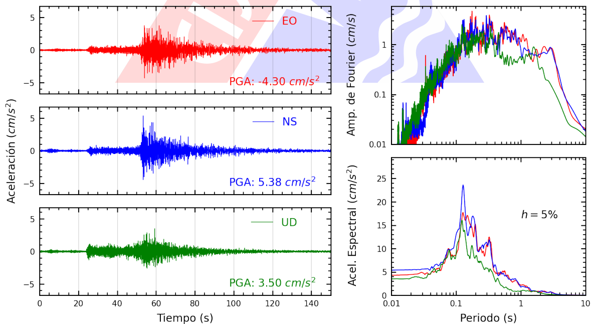
Figura A.30: Registros tiempo-historia, espectros de Fourier y de respuesta en las direcciones EO, NS y UD de la estación ICA003. Sismo de Lima, Lima - Lima de 2022-01-07, 05:27:05 (Hora local)
