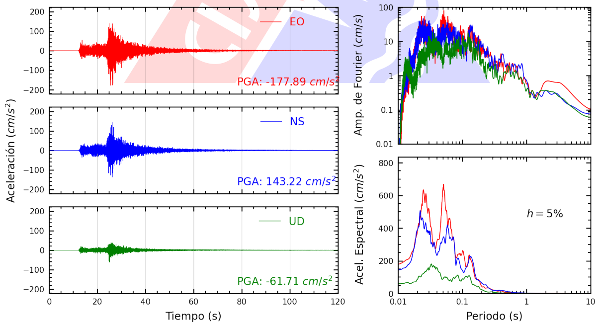
Figura A.8: Registros tiempo-historia, espectros de Fourier y de respuesta en las direcciones EO, NS y UD de la estación LIM001. Sismo de Lima, Lima - Lima de 2022-01-07, 05:27:05 (Hora local)
