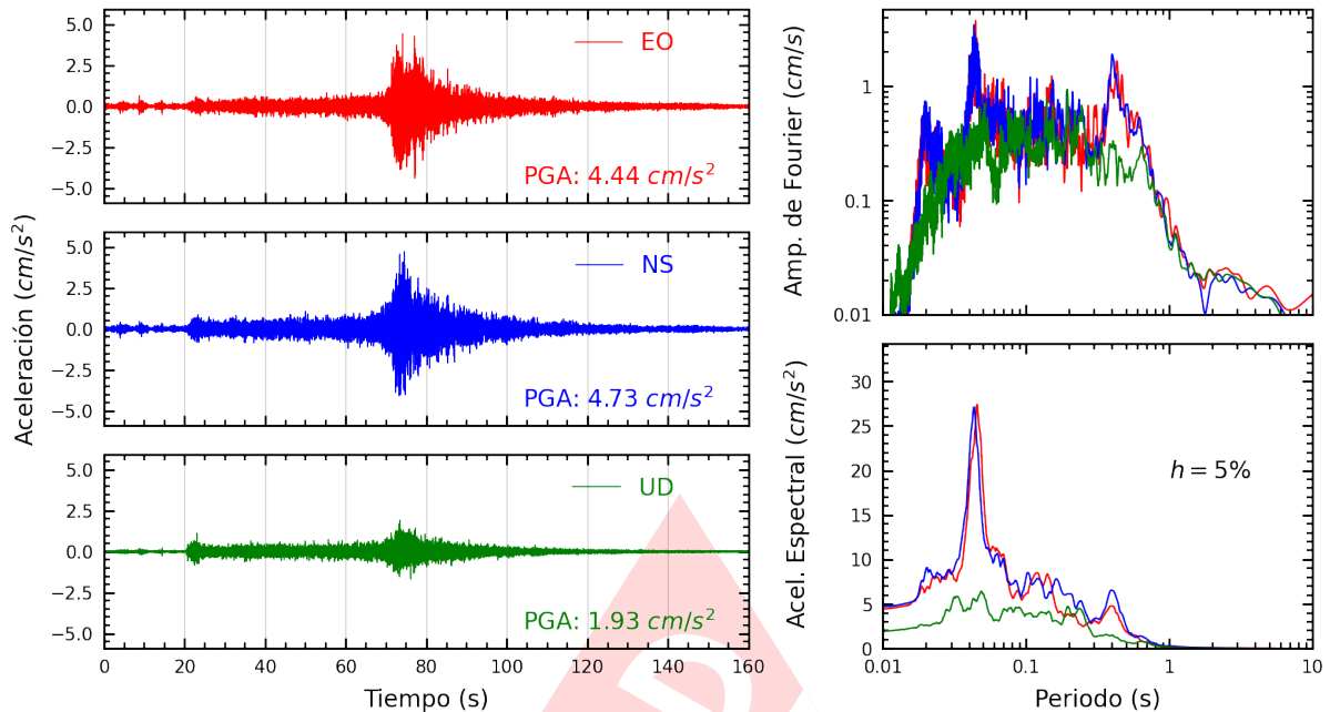
Figura A.31: Registros tiempo-historia, espectros de Fourier y de respuesta en las direcciones EO, NS y UD de la estación TRU001. Sismo de Lima, Lima - Lima de 2022-01-07, 05:27:05 (Hora local)
