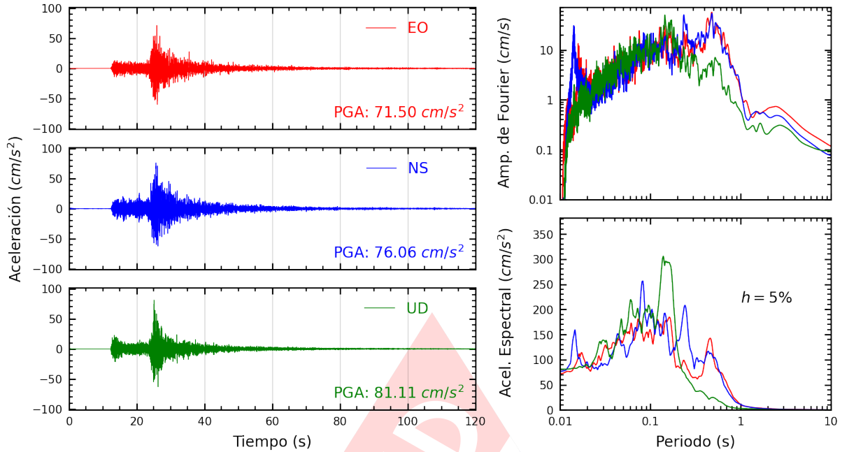
Figura A.15: Registros tiempo-historia, espectros de Fourier y de respuesta en las direcciones EO, NS y UD de la estación LIM022. Sismo de Lima, Lima - Lima de 2022-01-07, 05:27:05 (Hora local)
