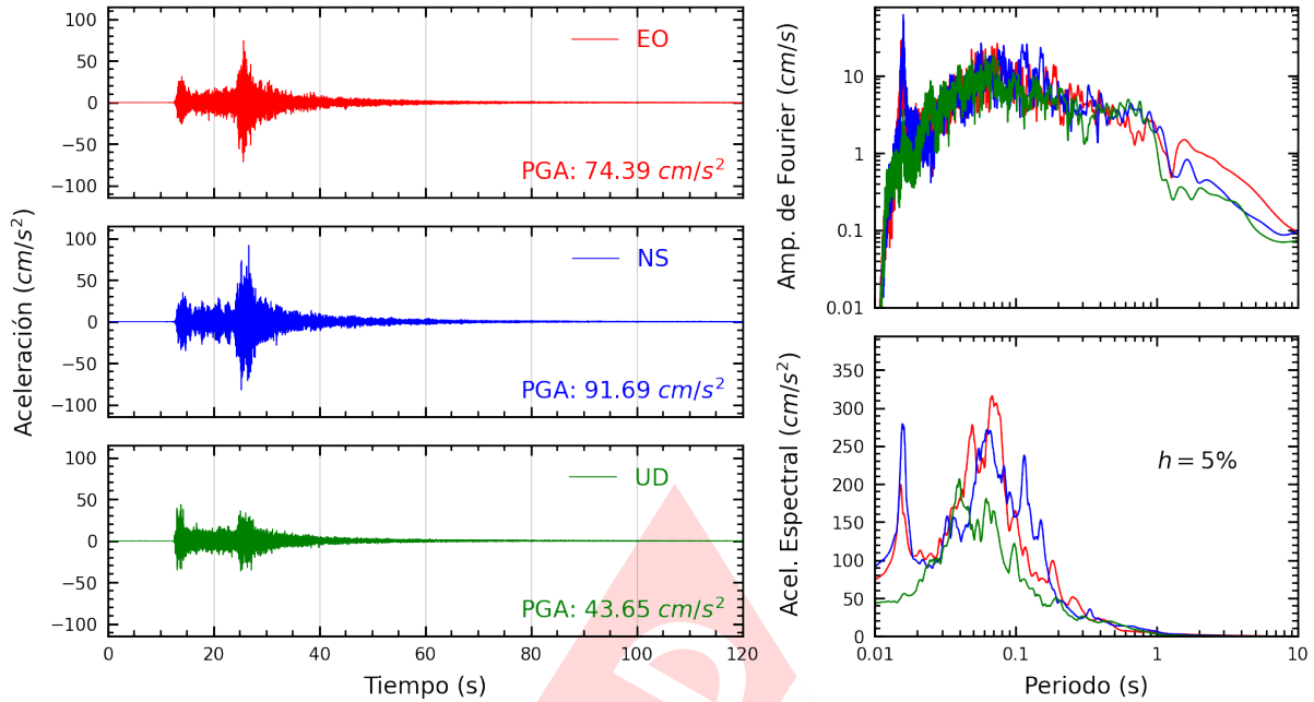
Figura A.13: Registros tiempo-historia, espectros de Fourier y de respuesta en las direcciones EO, NS y UD de la estación LIM014. Sismo de Lima, Lima - Lima de 2022-01-07, 05:27:05 (Hora local)
