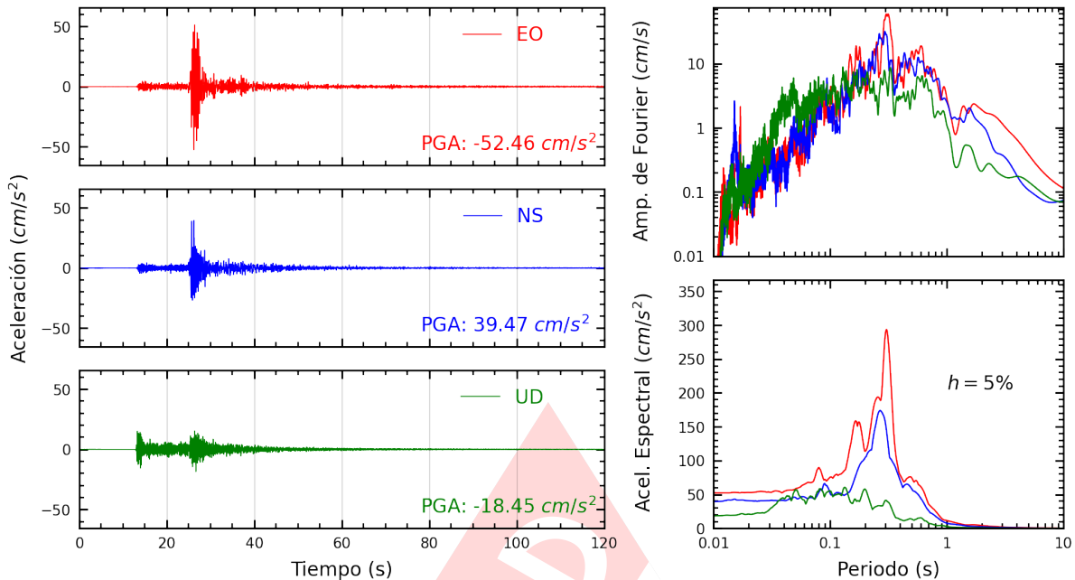
Figura A.23: Registros tiempo-historia, espectros de Fourier y de respuesta en las direcciones EO, NS y UD de la estación CAL003. Sismo de Lima, Lima - Lima de 2022-01-07, 05:27:05 (Hora local)
