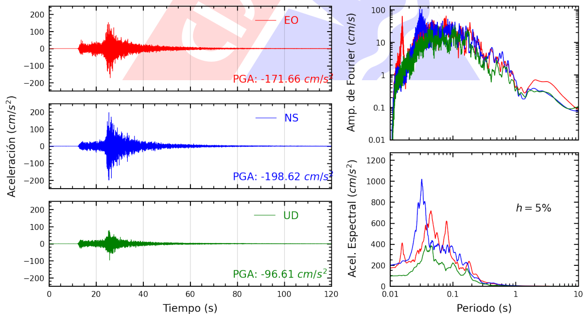
Figura A.6: Registros tiempo-historia, espectros de Fourier y de respuesta en las direcciones EO, NS y UD de la estación LIM024. Sismo de Lima, Lima - Lima de 2022-01-07, 05:27:05 (Hora local)
