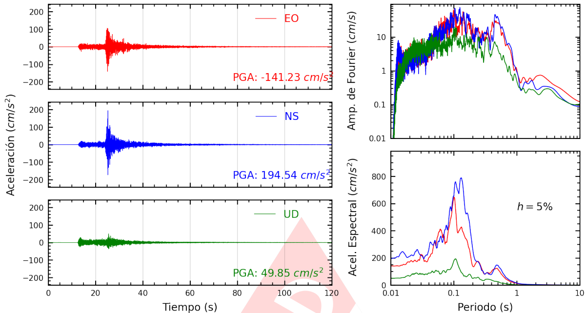
Figura A.7: Registros tiempo-historia, espectros de Fourier y de respuesta en las direcciones EO, NS y UD de la estación CAL012. Sismo de Lima, Lima - Lima de 2022-01-07, 05:27:05 (Hora local)
