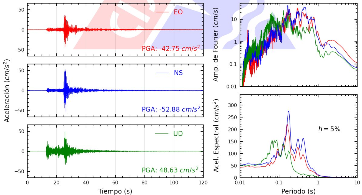
Figura A.22: Registros tiempo-historia, espectros de Fourier y de respuesta en las direcciones EO, NS y UD de la estación CAL005. Sismo de Lima, Lima - Lima de 2022-01-07, 05:27:05 (Hora local)
