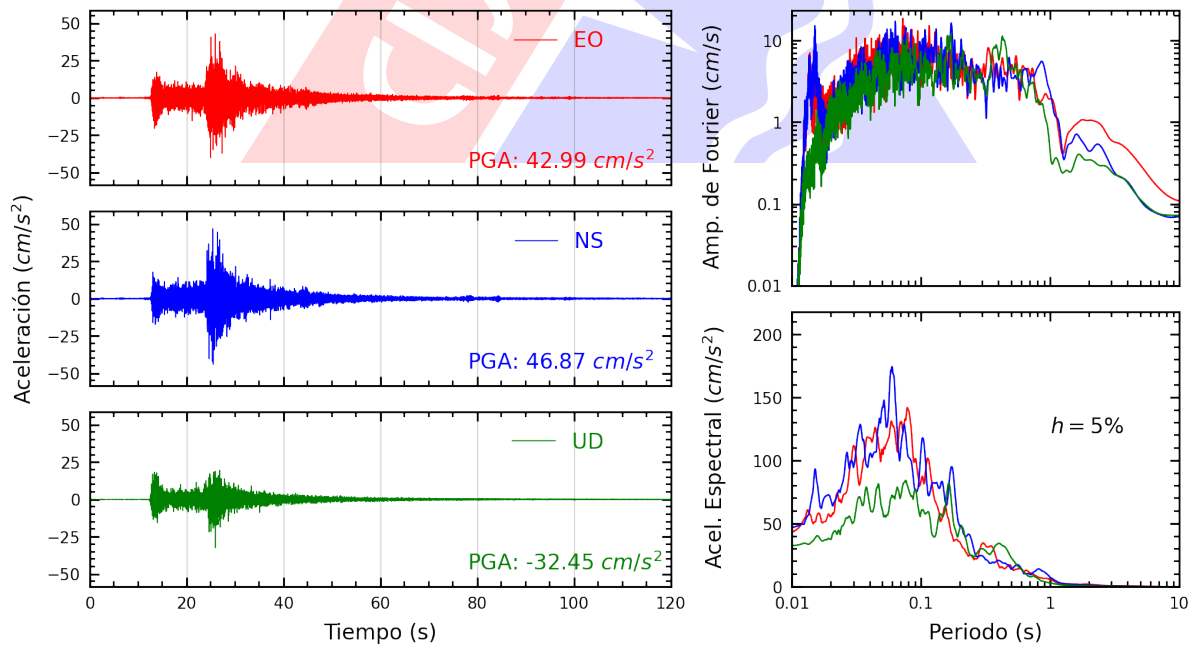
Figura A.26: Registros tiempo-historia, espectros de Fourier y de respuesta en las direcciones EO, NS y UD de la estación LIM015. Sismo de Lima, Lima - Lima de 2022-01-07, 05:27:05 (Hora local)
