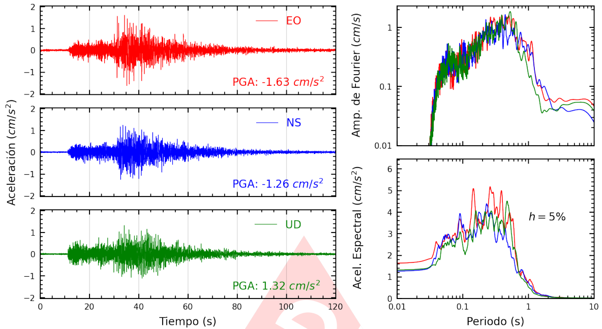
Figura A.29: Registros tiempo-historia, espectros de Fourier y de respuesta en las direcciones EO, NS y vertical de la estación IMCA. Sismo de Huacho, Huaura - Lima de 2022-03-30, 19:11:41 (Hora local)
