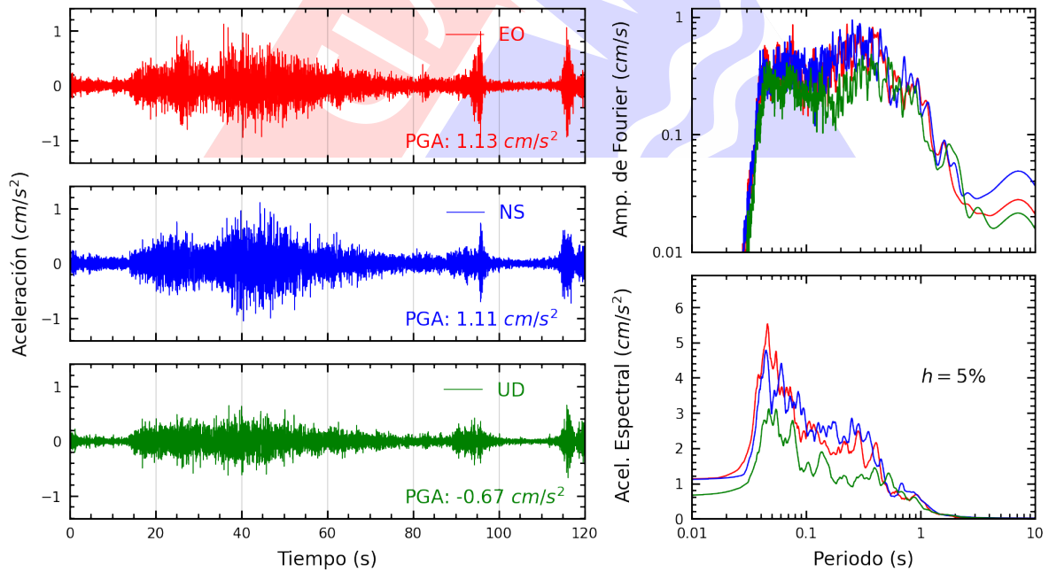
Figura A.38: Registros tiempo-historia, espectros de Fourier y de respuesta en las direcciones EO, NS y vertical de la estación PACHA. Sismo de Huacho, Huaura - Lima de 2022-03-30, 19:11:41 (Hora local)
