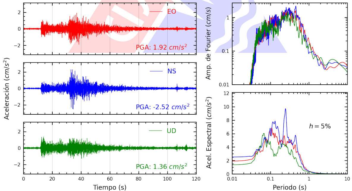
Figura A.20: Registros tiempo-historia, espectros de Fourier y de respuesta en las direcciones EO, NS y vertical de la estación URPE. Sismo de Huacho, Huaura - Lima de 2022-03-30, 19:11:41 (Hora local)
