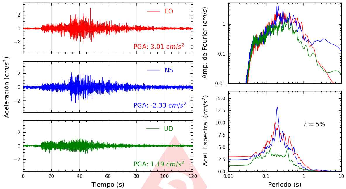
Figura A.19: Registros tiempo-historia, espectros de Fourier y de respuesta en las direcciones EO, NS y vertical de la estación SCCHO. Sismo de Huacho, Huaura - Lima de 2022-03-30, 19:11:41 (Hora local)
