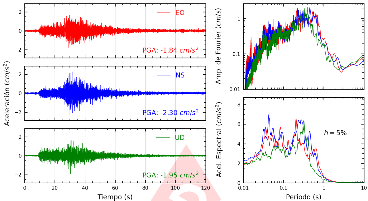
Figura A.23: Registros tiempo-historia, espectros de Fourier y de respuesta en las direcciones EO, NS y vertical de la estación COMAS. Sismo de Huacho, Huaura - Lima de 2022-03-30, 19:11:41 (Hora local)
