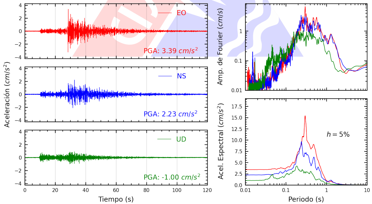
Figura A.16: Registros tiempo-historia, espectros de Fourier y de respuesta en las direcciones EO, NS y vertical de la estación DSMI. Sismo de Huacho, Huaura - Lima de 2022-03-30, 19:11:41 (Hora local)
