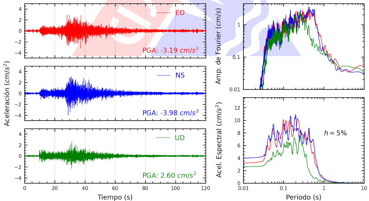
Figura A.12: Registros tiempo-historia, espectros de Fourier y de respuesta en las direcciones EO, NS y vertical de la estación OLIVO. Sismo de Huacho, Huaura - Lima de 2022-03-30, 19:11:41 (Hora local)
