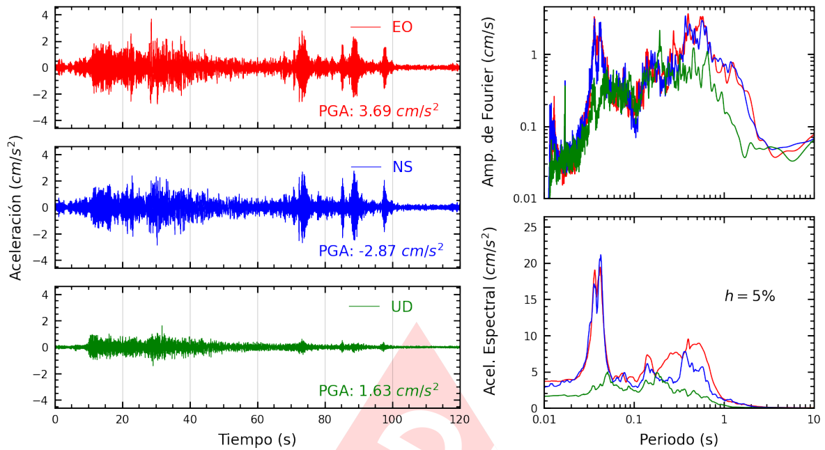
Figura A.15: Registros tiempo-historia, espectros de Fourier y de respuesta en las direcciones EO, NS y vertical de la estación DHNPE. Sismo de Huacho, Huaura - Lima de 2022-03-30, 19:11:41 (Hora local)
