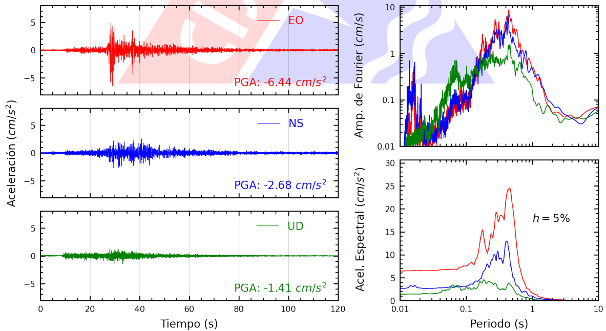
Figura A.4: Registros tiempo-historia, espectros de Fourier y de respuesta en las direcciones EO, NS y vertical de la estación ACAPU. Sismo de Huacho, Huaura - Lima de 2022-03-30, 19:11:41 (Hora local)
