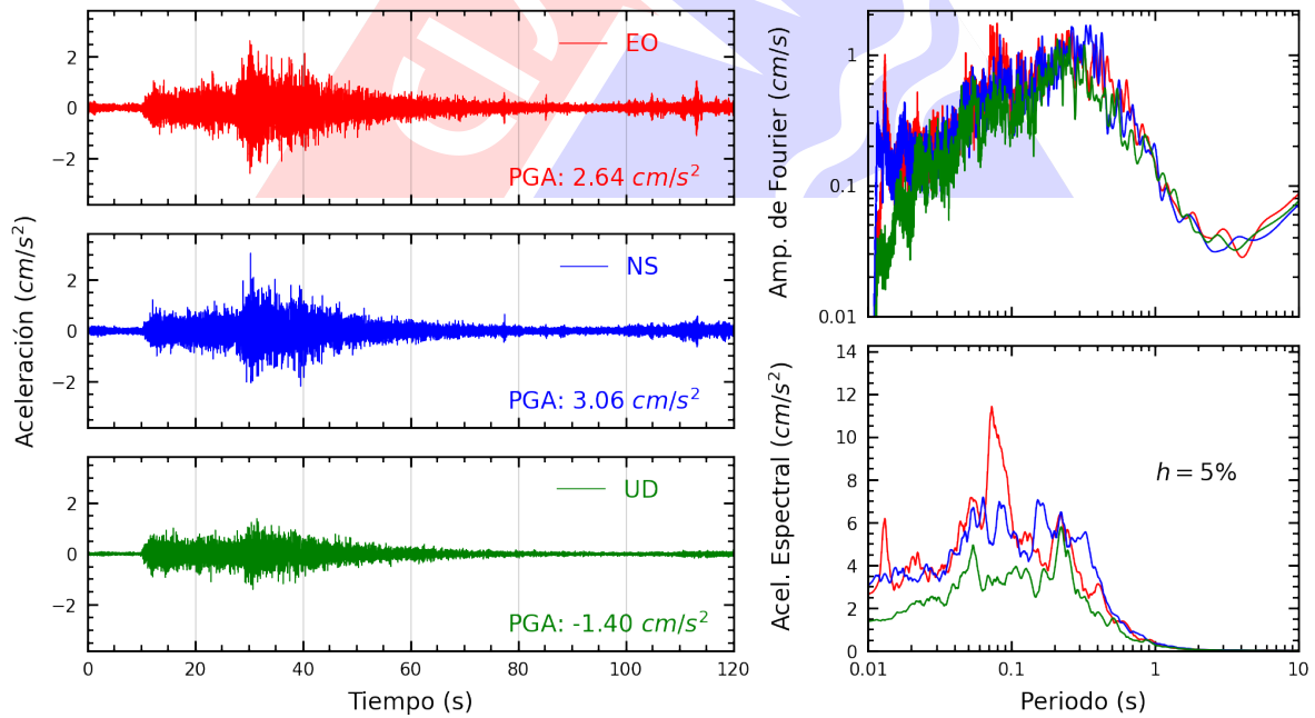
Figura A.18: Registros tiempo-historia, espectros de Fourier y de respuesta en las direcciones EO, NS y vertical de la estación FICPE. Sismo de Huacho, Huaura - Lima de 2022-03-30, 19:11:41 (Hora local)
