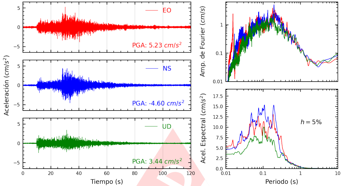
Figura A.5: Registros tiempo-historia, espectros de Fourier y de respuesta en las direcciones EO, NS y vertical de la estación INDEP. Sismo de Huacho, Huaura - Lima de 2022-03-30, 19:11:41 (Hora local)
