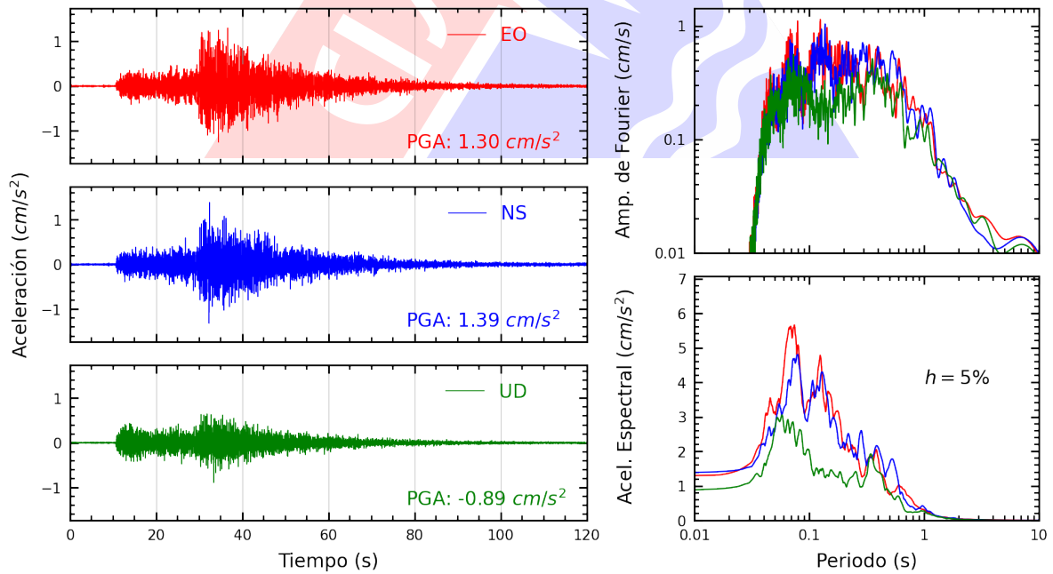
Figura A.36: Registros tiempo-historia, espectros de Fourier y de respuesta en las direcciones EO, NS y vertical de la estación ATARJ. Sismo de Huacho, Huaura - Lima de 2022-03-30, 19:11:41 (Hora local)
