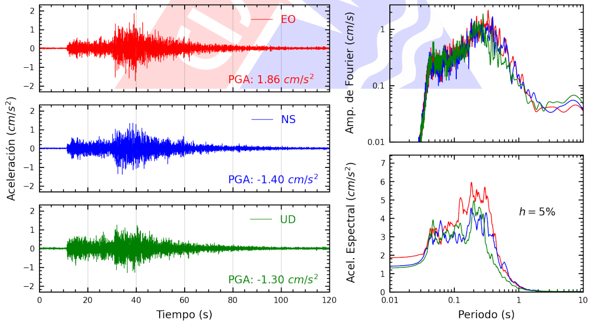
Figura A.26: Registros tiempo-historia, espectros de Fourier y de respuesta en las direcciones EO, NS y vertical de la estación USMP. Sismo de Huacho, Huaura - Lima de 2022-03-30, 19:11:41 (Hora local)
