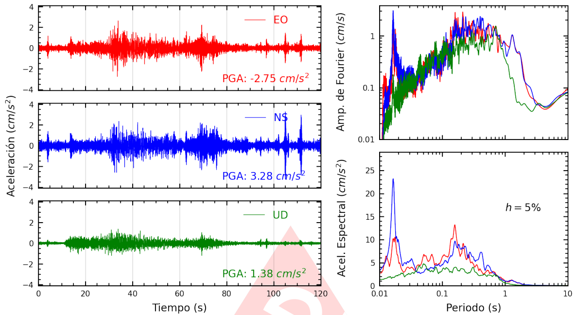
Figura A.17: Registros tiempo-historia, espectros de Fourier y de respuesta en las direcciones EO, NS y vertical de la estación PRADO. Sismo de Huacho, Huaura - Lima de 2022-03-30, 19:11:41 (Hora local)
