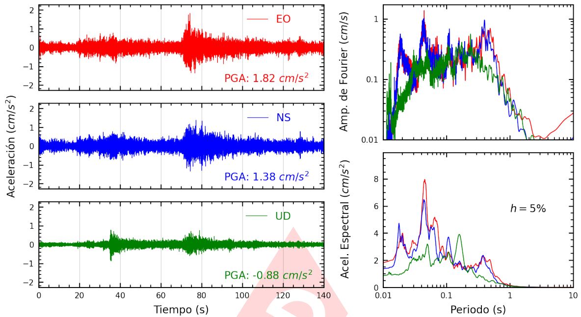
Figura A.27: Registros tiempo-historia, espectros de Fourier y de respuesta en las direcciones EO, NS y vertical de la estación SCTRÚ. Sismo de Huacho, Huaura - Lima de 2022-03-30, 19:11:41 (Hora local)
