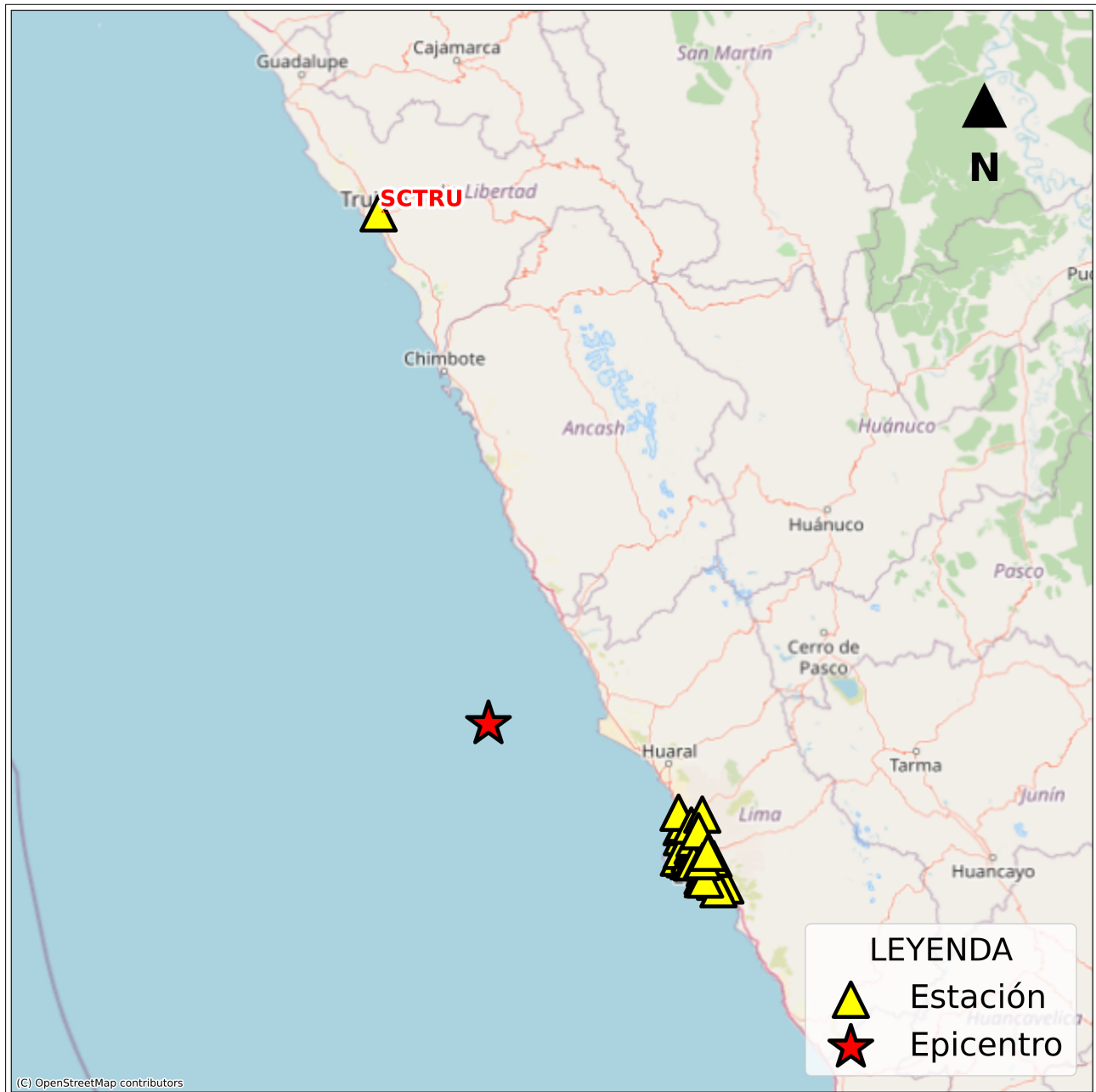
Figura 2: Mapa de ubicación de la(s) estación(es) acelerográfica(s) a nivel nacional correspondiente(s) al Sismo de Huacho, Huaura - Lima del 30 de marzo de 2022 a las 19:11:41 (hora local)
