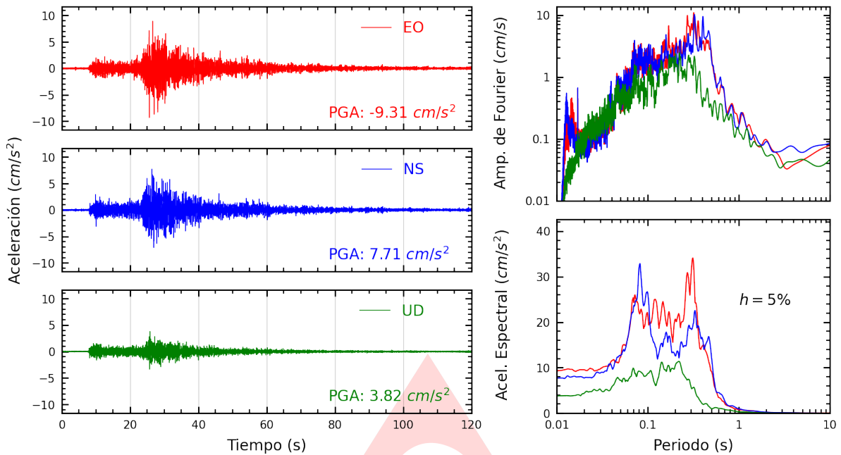
Figura A.1: Registros tiempo-historia, espectros de Fourier y de respuesta en las direcciones EO, NS y vertical de la estación DEFEN. Sismo de Huacho, Huaura - Lima de 2022-03-30, 19:11:41 (Hora local)
