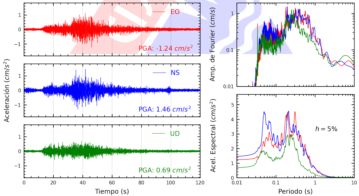
Figura A.32: Registros tiempo-historia, espectros de Fourier y de respuesta en las direcciones EO, NS y vertical de la estación UPCVI. Sismo de Huacho, Huaura - Lima de 2022-03-30, 19:11:41 (Hora local)
