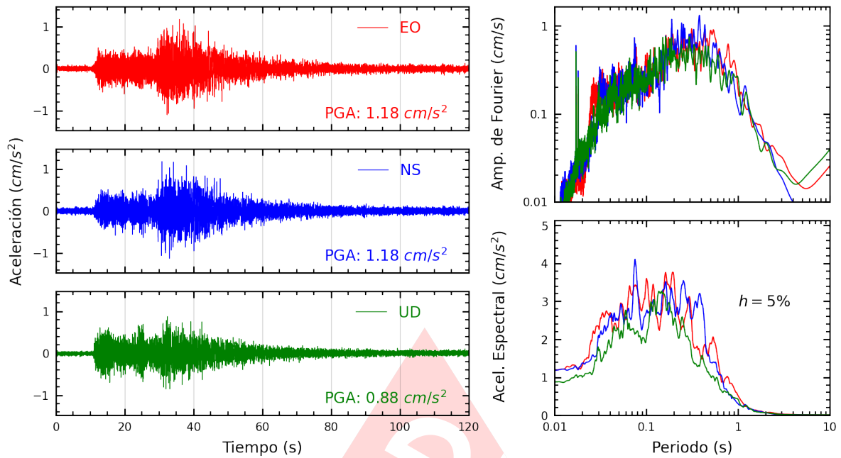
Figura A.37: Registros tiempo-historia, espectros de Fourier y de respuesta en las direcciones EO, NS y vertical de la estación BORJA. Sismo de Huacho, Huaura - Lima de 2022-03-30, 19:11:41 (Hora local)
