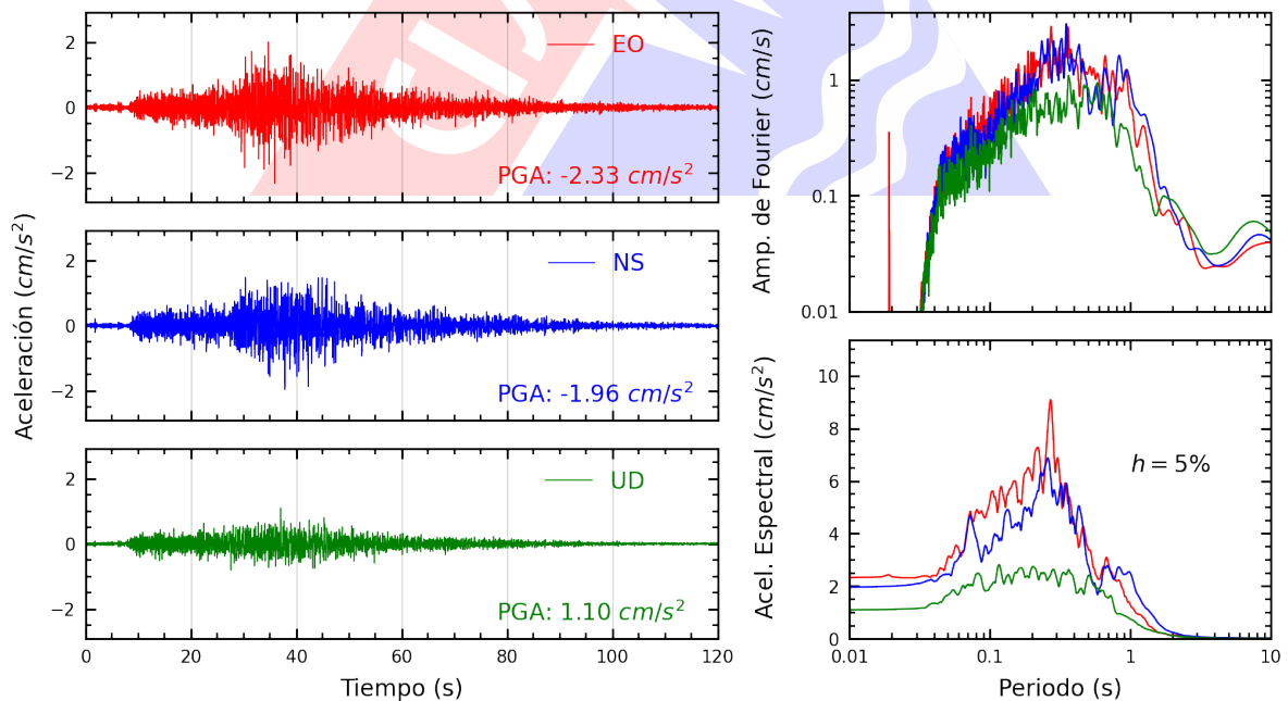
Figura A.22: Registros tiempo-historia, espectros de Fourier y de respuesta en las direcciones EO, NS y vertical de la estación BRISA. Sismo de Huacho, Huaura - Lima de 2022-03-30, 19:11:41 (Hora local)
