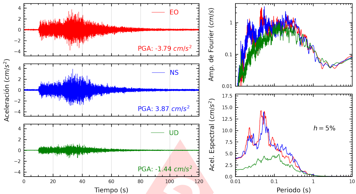
Figura A.13: Registros tiempo-historia, espectros de Fourier y de respuesta en las direcciones EO, NS y vertical de la estación JALVA. Sismo de Huacho, Huaura - Lima de 2022-03-30, 19:11:41 (Hora local)
