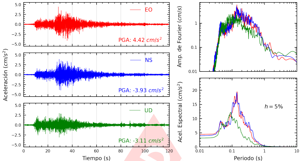
Figura A.9: Registros tiempo-historia, espectros de Fourier y de respuesta en las direcciones EO, NS y vertical de la estación CARAB. Sismo de Huacho, Huaura - Lima de 2022-03-30, 19:11:41 (Hora local)
