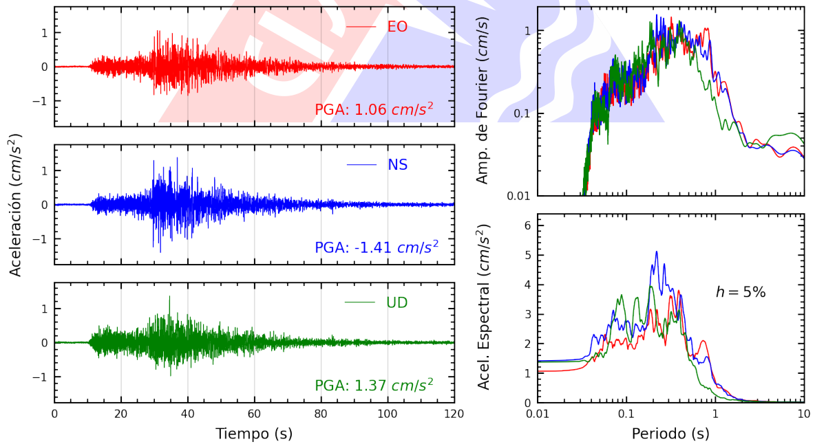
Figura A.34: Registros tiempo-historia, espectros de Fourier y de respuesta en las direcciones EO, NS y vertical de la estación UNFV. Sismo de Huacho, Huaura - Lima de 2022-03-30, 19:11:41 (Hora local)
