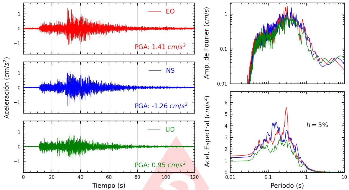
Figura A.33: Registros tiempo-historia, espectros de Fourier y de respuesta en las direcciones EO, NS y vertical de la estación INICT. Sismo de Huacho, Huaura - Lima de 2022-03-30, 19:11:41 (Hora local)
