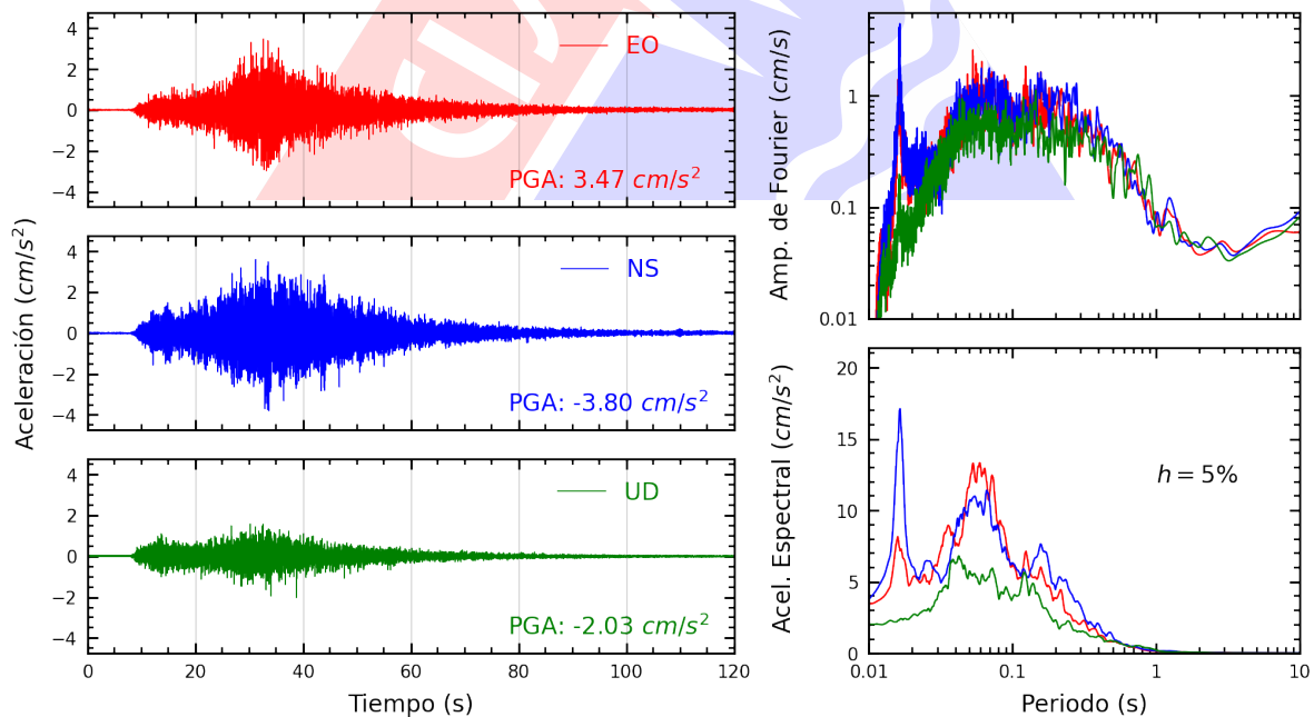
Figura A.14: Registros tiempo-historia, espectros de Fourier y de respuesta en las direcciones EO, NS y vertical de la estación IPEN. Sismo de Huacho, Huaura - Lima de 2022-03-30, 19:11:41 (Hora local)
