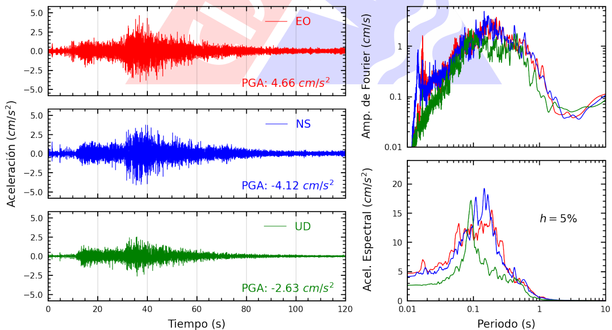
Figura A.8: Registros tiempo-historia, espectros de Fourier y de respuesta en las direcciones EO, NS y vertical de la estación USILM. Sismo de Huacho, Huaura - Lima de 2022-03-30, 19:11:41 (Hora local)
