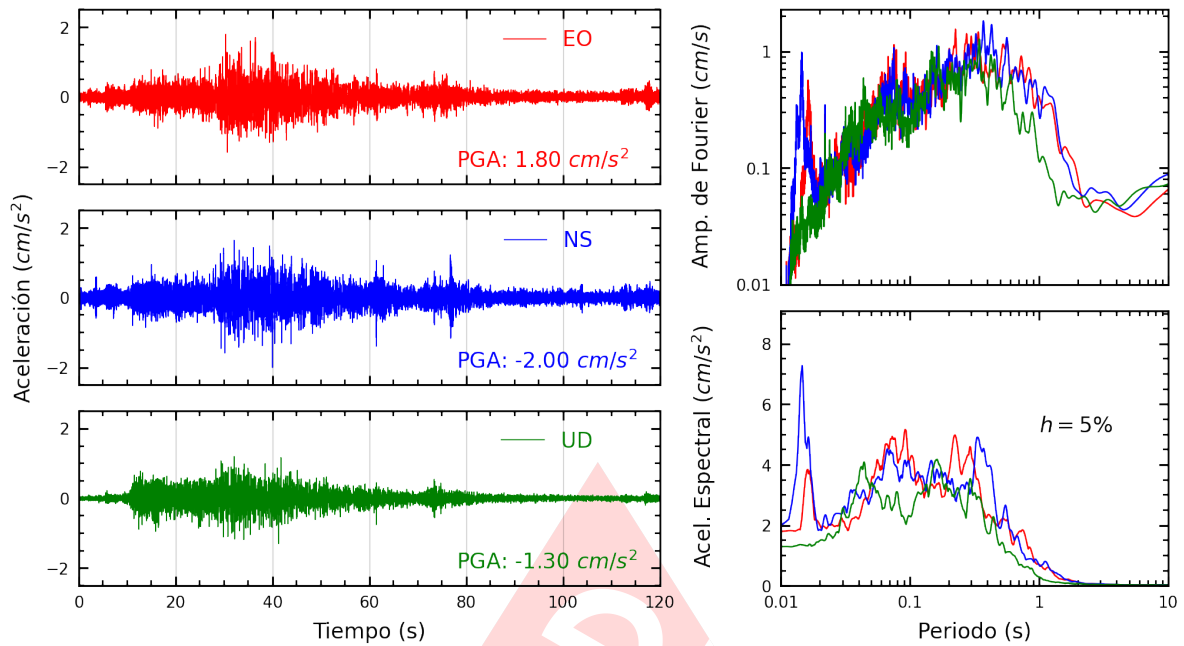
Figura A.25: Registros tiempo-historia, espectros de Fourier y de respuesta en las direcciones EO, NS y vertical de la estación UPCSM. Sismo de Huacho, Huaura - Lima de 2022-03-30, 19:11:41 (Hora local)
