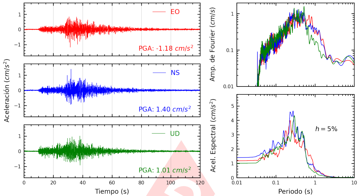
Figura A.35: Registros tiempo-historia, espectros de Fourier y de respuesta en las direcciones EO, NS y vertical de la estación BONDY. Sismo de Huacho, Huaura - Lima de 2022-03-30, 19:11:41 (Hora local)
