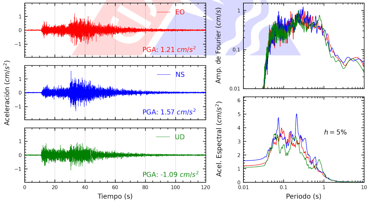
Figura A.30: Registros tiempo-historia, espectros de Fourier y de respuesta en las direcciones EO, NS y vertical de la estación CENEP. Sismo de Huacho, Huaura - Lima de 2022-03-30, 19:11:41 (Hora local)
