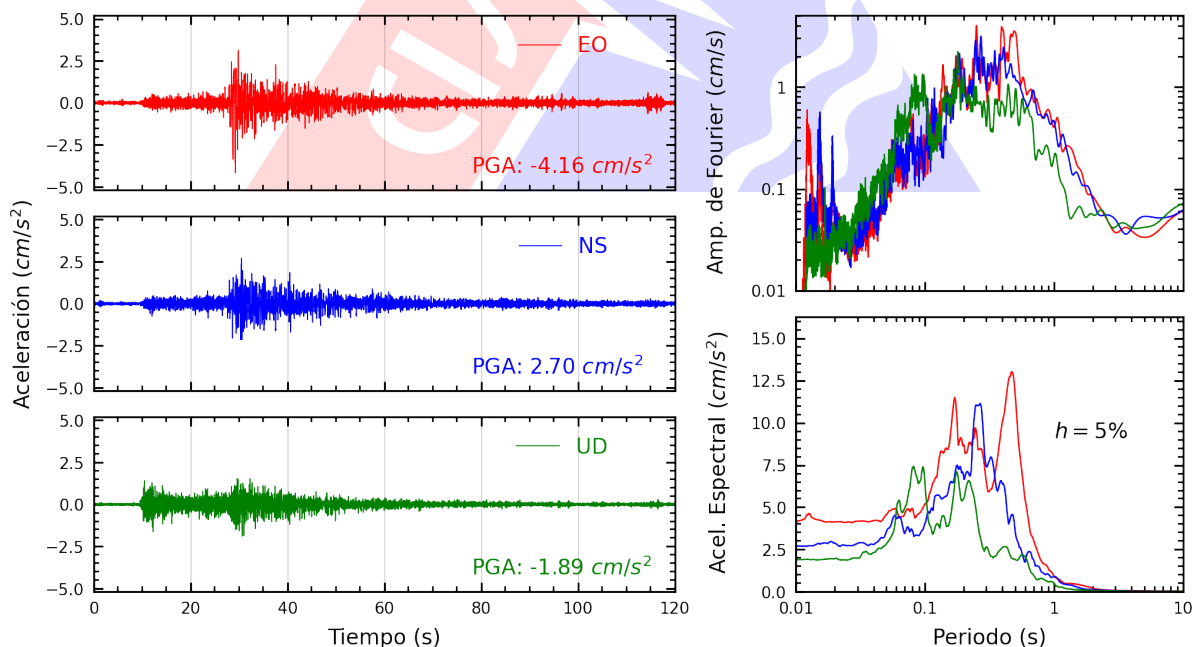
Figura A.10: Registros tiempo-historia, espectros de Fourier y de respuesta en las direcciones EO, NS y vertical de la estación RAMON. Sismo de Huacho, Huaura - Lima de 2022-03-30, 19:11:41 (Hora local)
