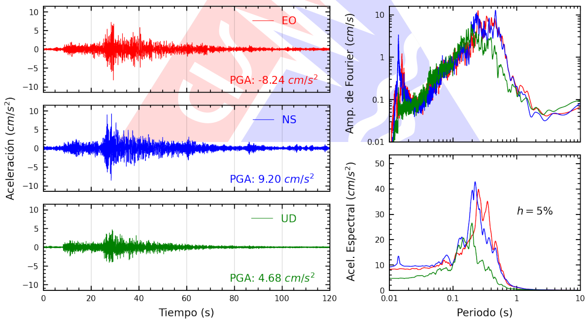
Figura A.2: Registros tiempo-historia, espectros de Fourier y de respuesta en las direcciones EO, NS y vertical de la estación MDPP. Sismo de Huacho, Huaura - Lima de 2022-03-30, 19:11:41 (Hora local)
