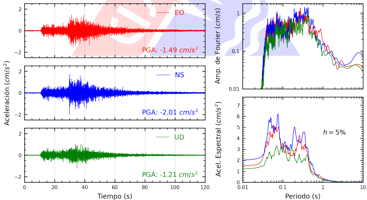
Figura A.24: Registros tiempo-historia, espectros de Fourier y de respuesta en las direcciones EO, NS y vertical de la estación CEPRE. Sismo de Huacho, Huaura - Lima de 2022-03-30, 19:11:41 (Hora local)
