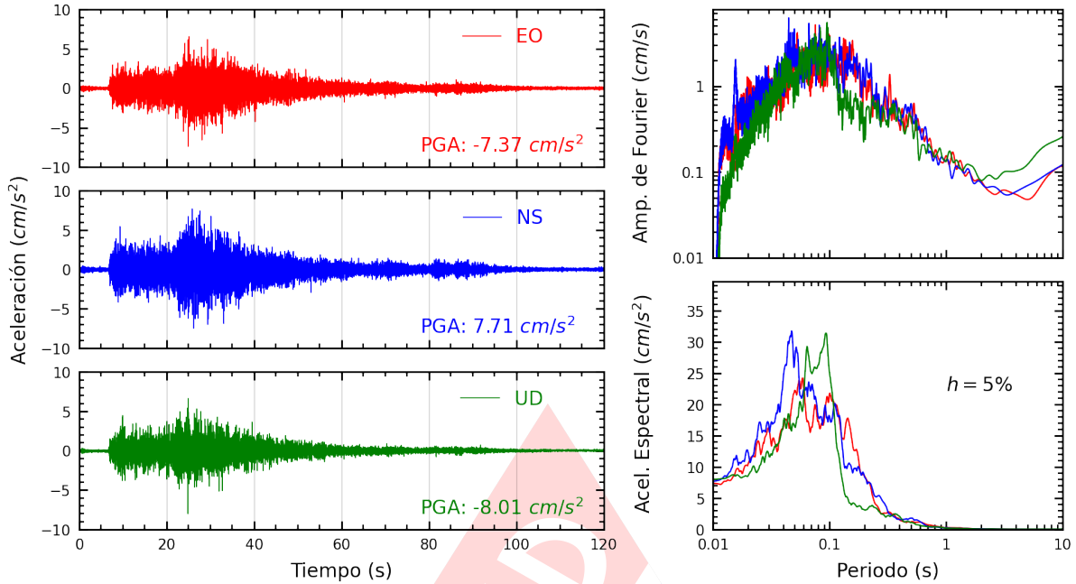
Figura A.3: Registros tiempo-historia, espectros de Fourier y de respuesta en las direcciones EO, NS y vertical de la estación SROSA. Sismo de Huacho, Huaura - Lima de 2022-03-30, 19:11:41 (Hora local)
