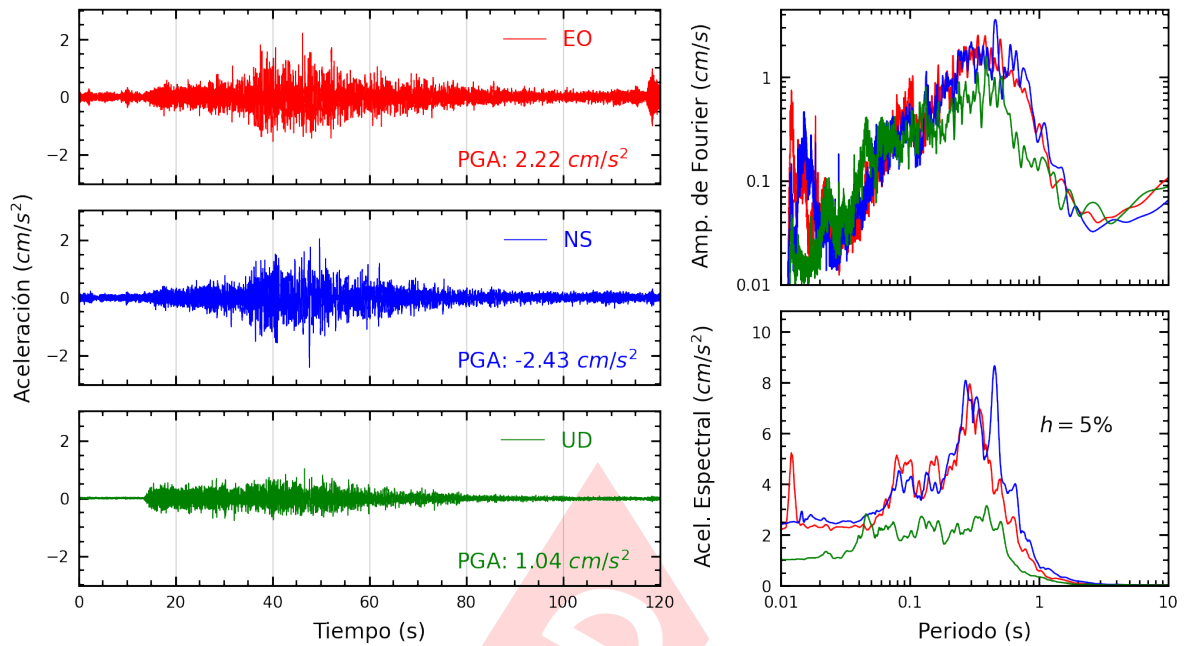
Figura A.21: Registros tiempo-historia, espectros de Fourier y de respuesta en las direcciones EO, NS y vertical de la estación USILP. Sismo de Huacho, Huaura - Lima de 2022-03-30, 19:11:41 (Hora local)
