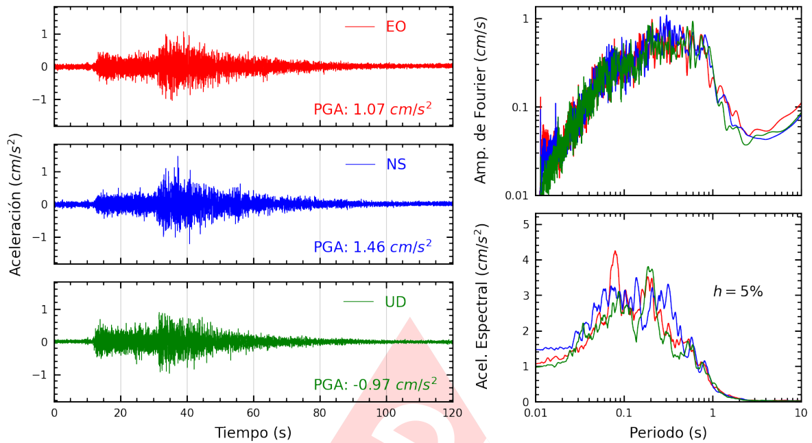
Figura A.31: Registros tiempo-historia, espectros de Fourier y de respuesta en las direcciones EO, NS y vertical de la estación SERVI. Sismo de Huacho, Huaura - Lima de 2022-03-30, 19:11:41 (Hora local)
