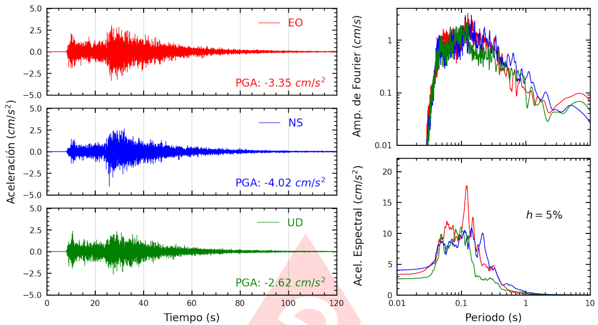
Figura A.11: Registros tiempo-historia, espectros de Fourier y de respuesta en las direcciones EO, NS y vertical de la estación AMORE. Sismo de Huacho, Huaura - Lima de 2022-03-30, 19:11:41 (Hora local)
