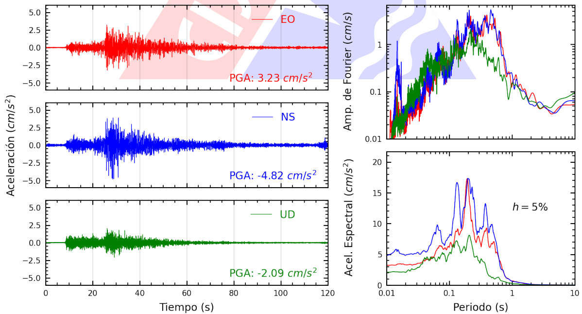
Figura A.6: Registros tiempo-historia, espectros de Fourier y de respuesta en las direcciones EO, NS y vertical de la estación VHAYA. Sismo de Huacho, Huaura - Lima de 2022-03-30, 19:11:41 (Hora local)
