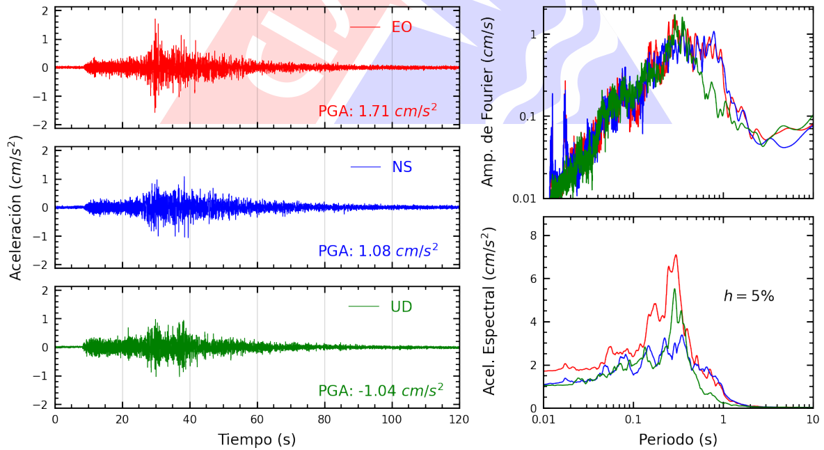
Figura A.28: Registros tiempo-historia, espectros de Fourier y de respuesta en las direcciones EO, NS y vertical de la estación UNMSM. Sismo de Huacho, Huaura - Lima de 2022-03-30, 19:11:41 (Hora local)
