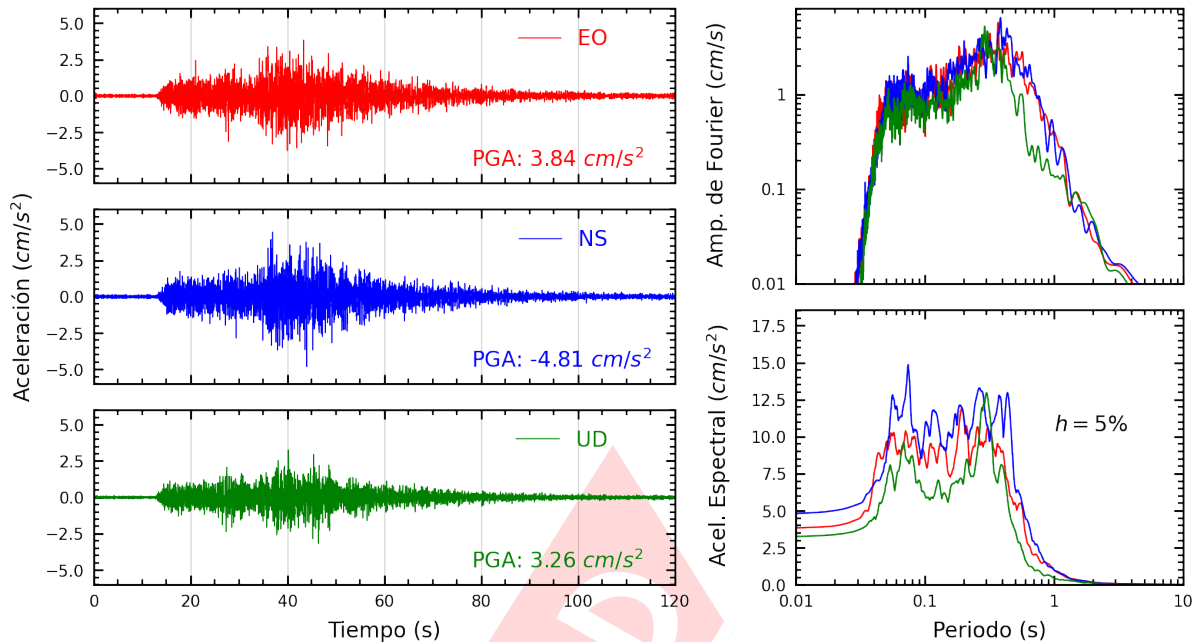
Figura A.7: Registros tiempo-historia, espectros de Fourier y de respuesta en las direcciones EO, NS y vertical de la estación UNTEL. Sismo de Huacho, Huaura - Lima de 2022-03-30, 19:11:41 (Hora local)
