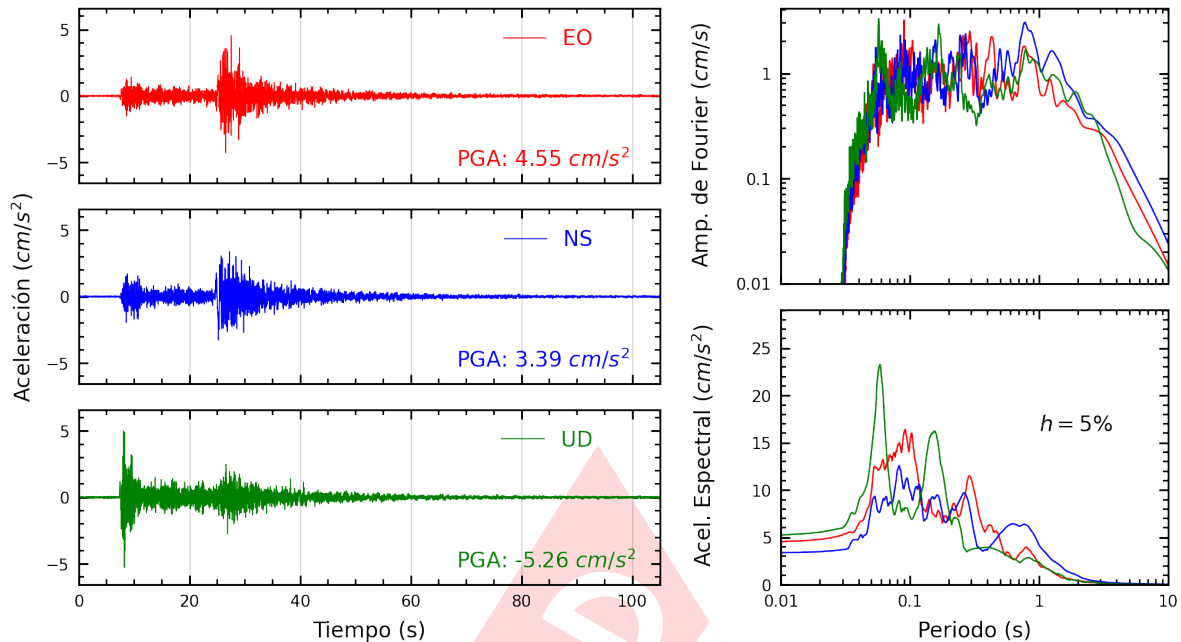
Figura A.3: Registros tiempo-historia, espectros de Fourier y de respuesta en las direcciones EO, NS y vertical de la estación UJBG2. Sismo de Tarata, Tarata - Tacna de 2022-05-24, 07:57:58 (Hora local)
