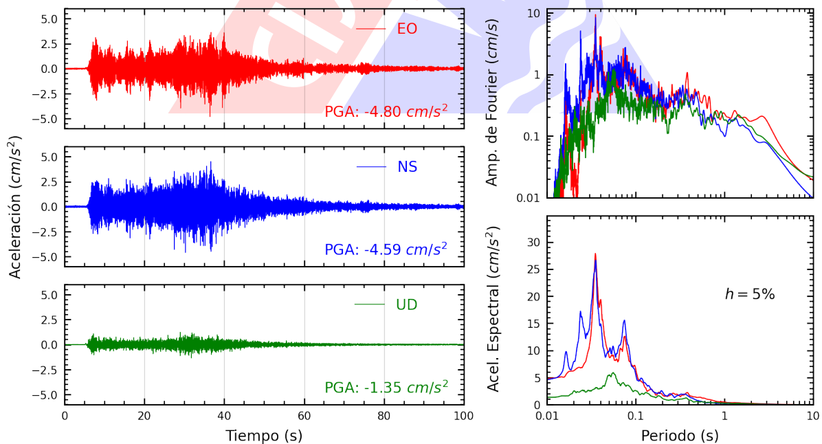
Figura A.4: Registros tiempo-historia, espectros de Fourier y de respuesta en las direcciones EO, NS y vertical de la estación UNAM. Sismo de Tarata, Tarata - Tacna de 2022-05-24, 07:57:58 (Hora local)
