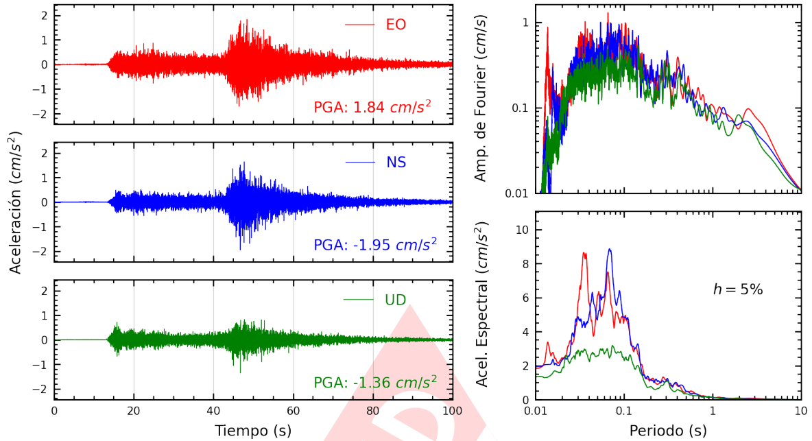
Figura A.7: Registros tiempo-historia, espectros de Fourier y de respuesta en las direcciones EO, NS y vertical de la estación UNSA. Sismo de Tarata, Tarata - Tacna de 2022-05-24, 07:57:58 (Hora local)
