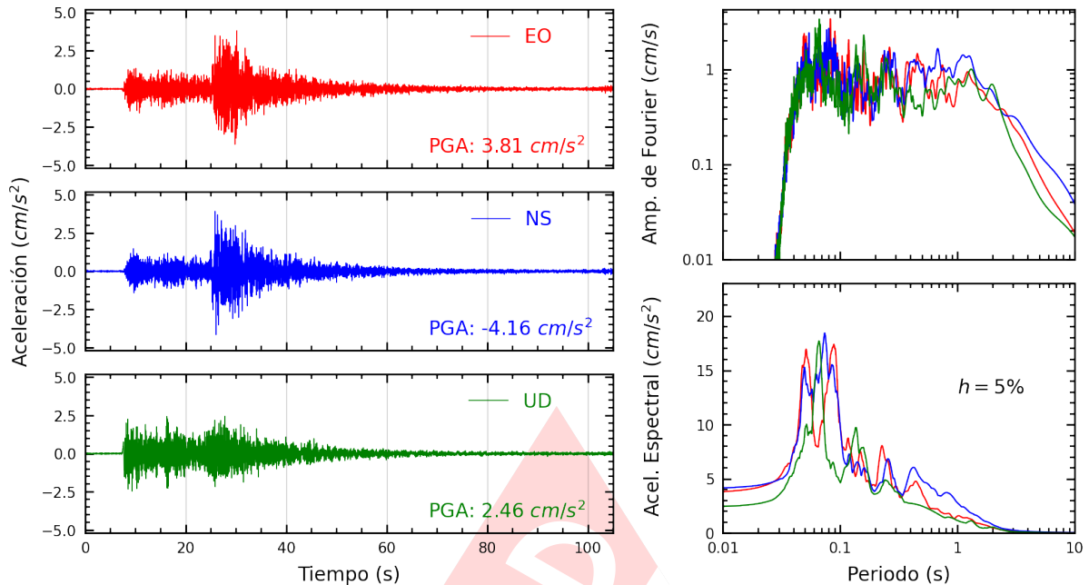
Figura A.5: Registros tiempo-historia, espectros de Fourier y de respuesta en las direcciones EO, NS y vertical de la estación CREY. Sismo de Tarata, Tarata - Tacna de 2022-05-24, 07:57:58 (Hora local)
