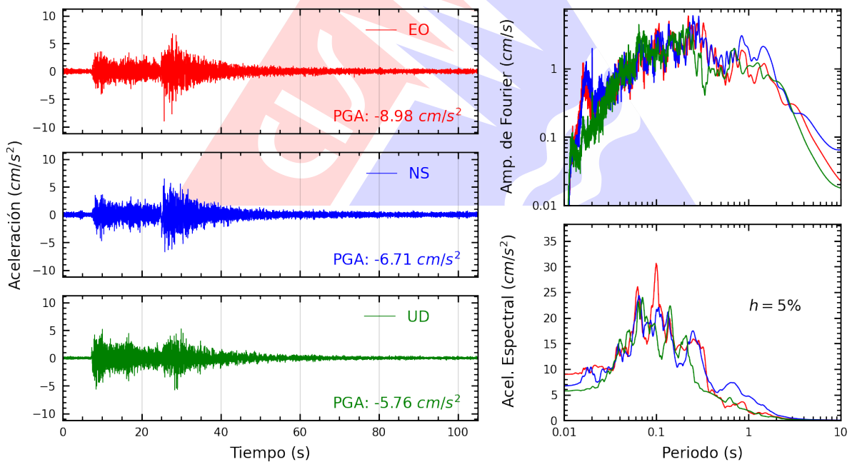
Figura A.2: Registros tiempo-historia, espectros de Fourier y de respuesta en las direcciones EO, NS y vertical de la estación SCTAC. Sismo de Tarata, Tarata - Tacna de 2022-05-24, 07:57:58 (Hora local)
