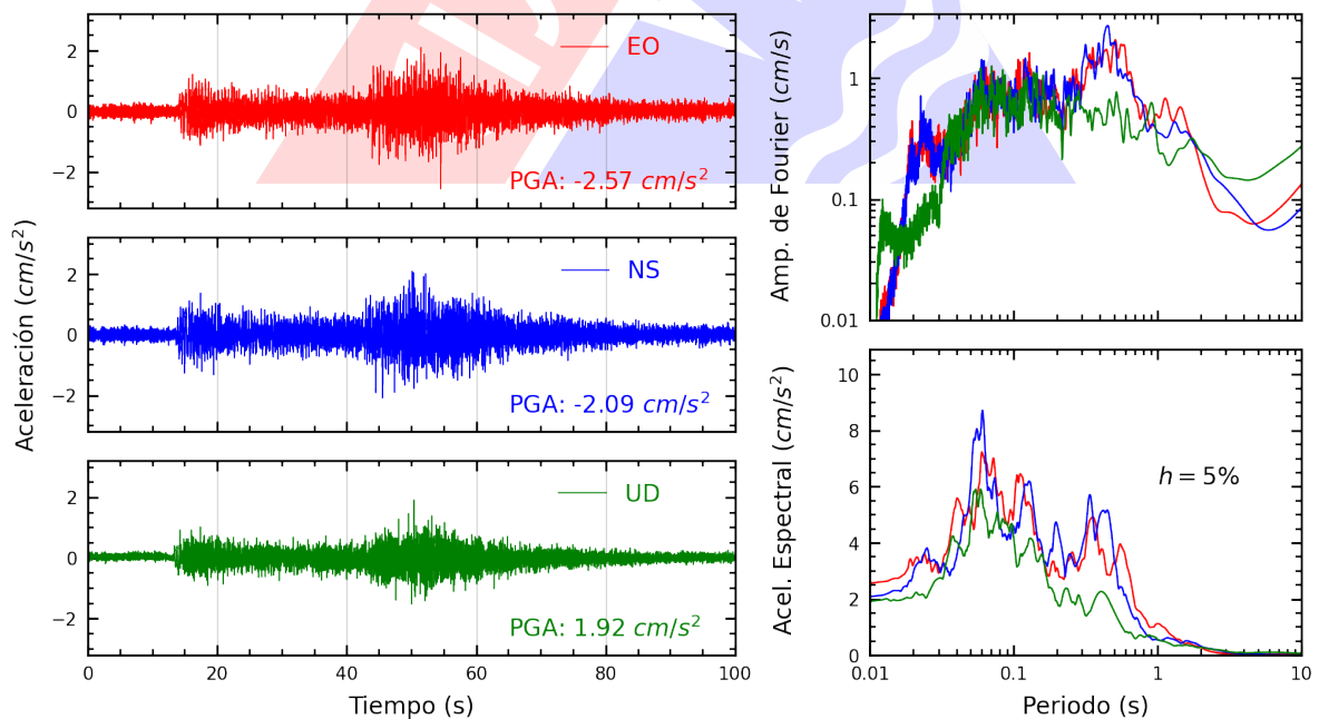
Figura A.6: Registros tiempo-historia, espectros de Fourier y de respuesta en las direcciones EO, NS y vertical de la estación SCARQ. Sismo de Tarata, Tarata - Tacna de 2022-05-24, 07:57:58 (Hora local)
