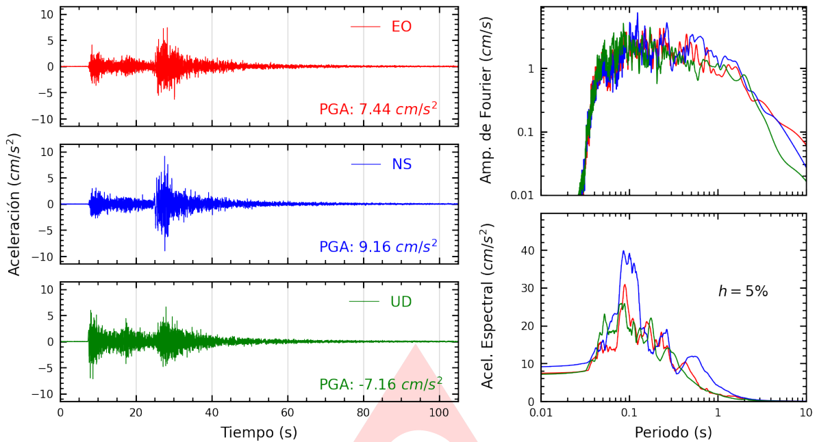
Figura A.1: Registros tiempo-historia, espectros de Fourier y de respuesta en las direcciones EO, NS y vertical de la estación UJBG3. Sismo de Tarata, Tarata - Tacna de 2022-05-24, 07:57:58 (Hora local)
