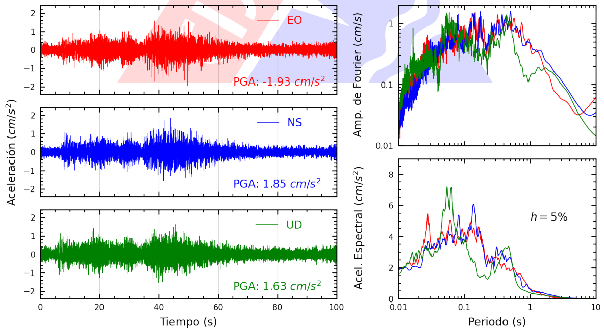
Figura A.8: Registros tiempo-historia, espectros de Fourier y de respuesta en las direcciones EO, NS y vertical de la estación SCAR2. Sismo de Tarata, Tarata - Tacna de 2022-05-24, 07:57:58 (Hora local)
