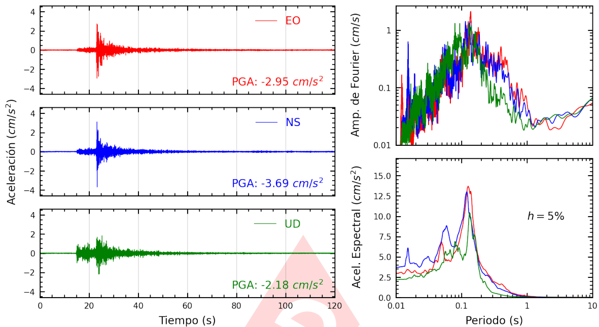
Figura A.15: Registros tiempo-historia, espectros de Fourier y de respuesta en las direcciones EO, NS y vertical de la estación RAMON. Sismo de Ancon, Lima - Lima de 2022-07-29, 23:20:12 (Hora local)
