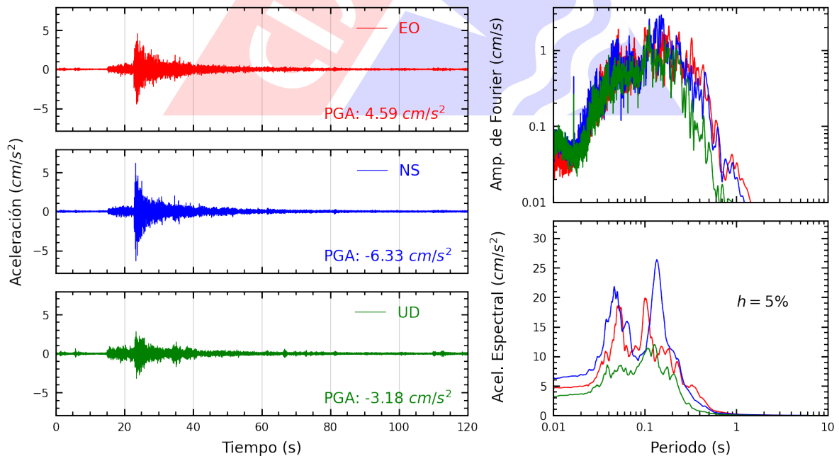
Figura A.10: Registros tiempo-historia, espectros de Fourier y de respuesta en las direcciones EO, NS y vertical de la estación SCOLI. Sismo de Ancon, Lima - Lima de 2022-07-29, 23:20:12 (Hora local)
