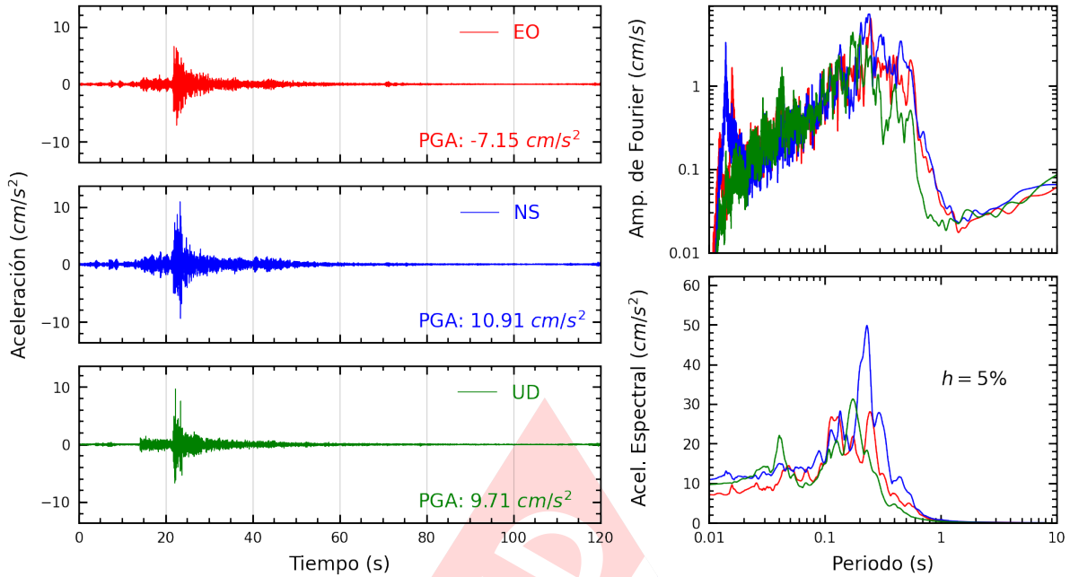
Figura A.5: Registros tiempo-historia, espectros de Fourier y de respuesta en las direcciones EO, NS y vertical de la estación MDPP. Sismo de Ancon, Lima - Lima de 2022-07-29, 23:20:12 (Hora local)
