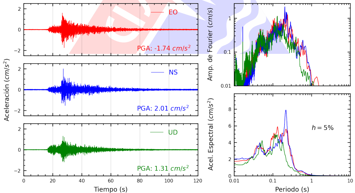
Figura A.24: Registros tiempo-historia, espectros de Fourier y de respuesta en las direcciones EO, NS y vertical de la estación SCCHO. Sismo de Ancon, Lima - Lima de 2022-07-29, 23:20:12 (Hora local)
