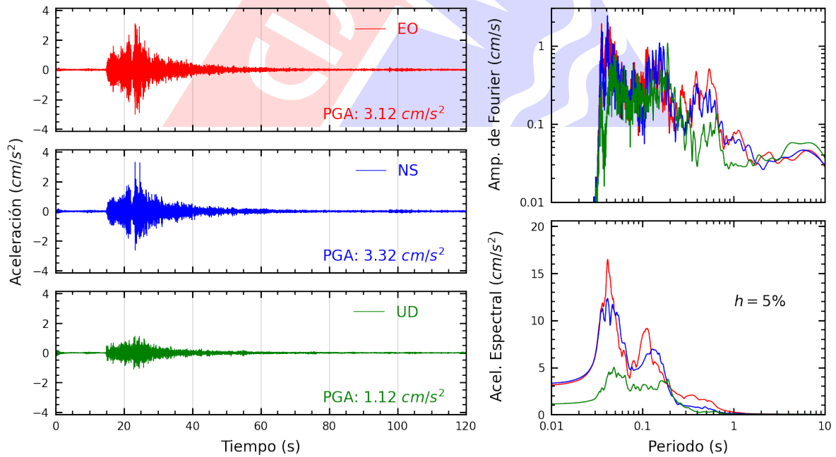
Figura A.18: Registros tiempo-historia, espectros de Fourier y de respuesta en las direcciones EO, NS y vertical de la estación DHNPE. Sismo de Ancon, Lima - Lima de 2022-07-29, 23:20:12 (Hora local)
