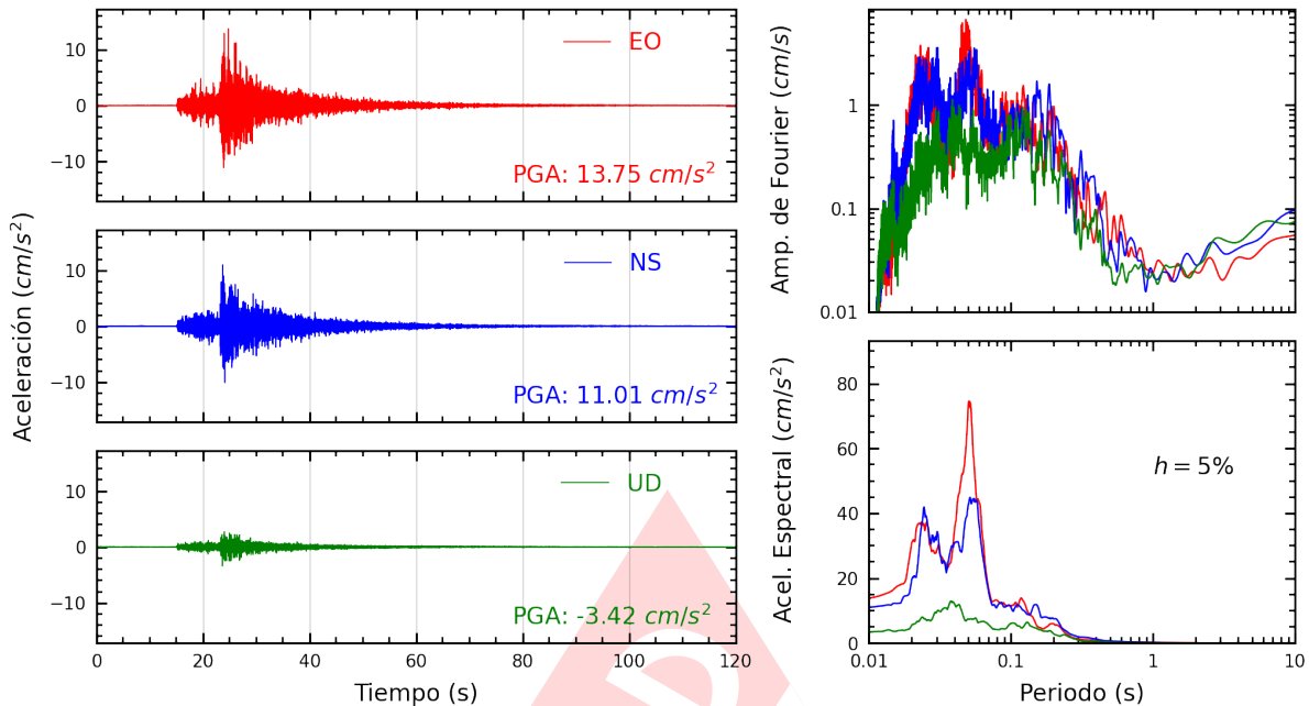
Figura A.3: Registros tiempo-historia, espectros de Fourier y de respuesta en las direcciones EO, NS y vertical de la estación JALVA. Sismo de Ancon, Lima - Lima de 2022-07-29, 23:20:12 (Hora local)
