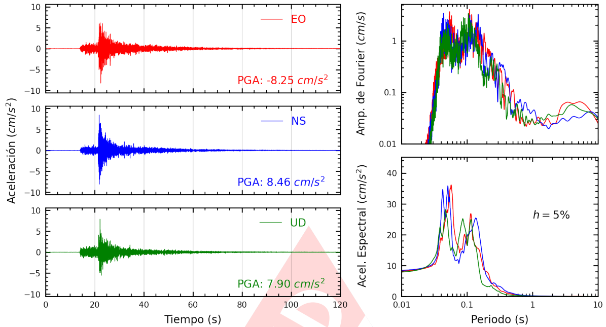
Figura A.7: Registros tiempo-historia, espectros de Fourier y de respuesta en las direcciones EO, NS y vertical de la estación AMORE. Sismo de Ancon, Lima - Lima de 2022-07-29, 23:20:12 (Hora local)
