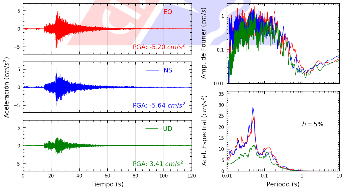
Figura A.12: Registros tiempo-historia, espectros de Fourier y de respuesta en las direcciones EO, NS y vertical de la estación FICPE. Sismo de Ancon, Lima - Lima de 2022-07-29, 23:20:12 (Hora local)
