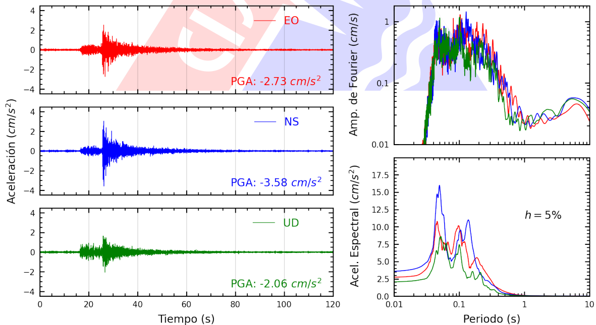
Figura A.16: Registros tiempo-historia, espectros de Fourier y de respuesta en las direcciones EO, NS y vertical de la estación URPE. Sismo de Ancon, Lima - Lima de 2022-07-29, 23:20:12 (Hora local)
