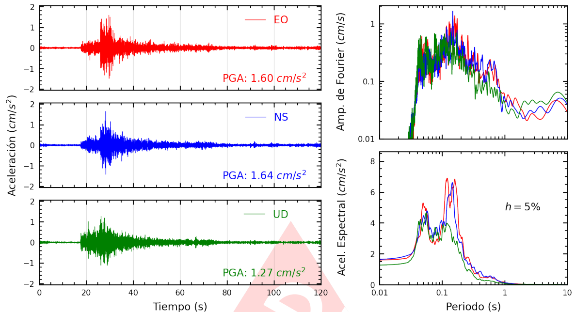
Figura A.29: Registros tiempo-historia, espectros de Fourier y de respuesta en las direcciones EO, NS y vertical de la estación PRADO. Sismo de Ancon, Lima - Lima de 2022-07-29, 23:20:12 (Hora local)
