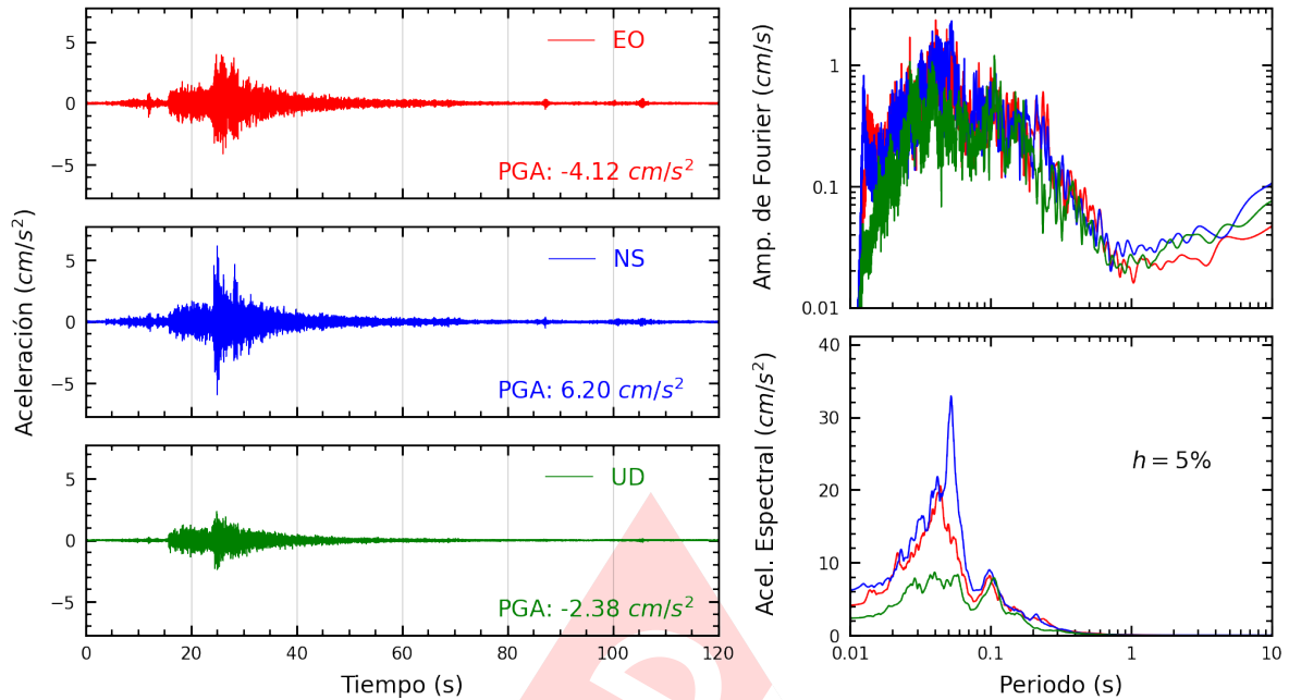
Figura A.11: Registros tiempo-historia, espectros de Fourier y de respuesta en las direcciones EO, NS y vertical de la estación CEPRE. Sismo de Ancon, Lima - Lima de 2022-07-29, 23:20:12 (Hora local)
