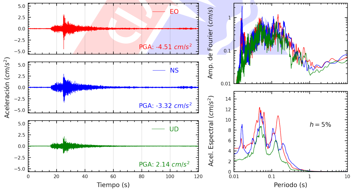
Figura A.14: Registros tiempo-historia, espectros de Fourier y de respuesta en las direcciones EO, NS y vertical de la estación CENEP. Sismo de Ancon, Lima - Lima de 2022-07-29, 23:20:12 (Hora local)
