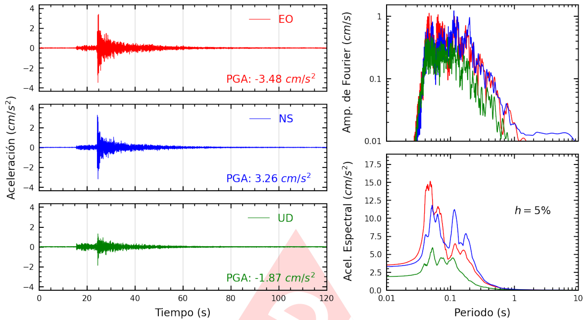
Figura A.17: Registros tiempo-historia, espectros de Fourier y de respuesta en las direcciones EO, NS y vertical de la estación ATARJ. Sismo de Ancon, Lima - Lima de 2022-07-29, 23:20:12 (Hora local)
