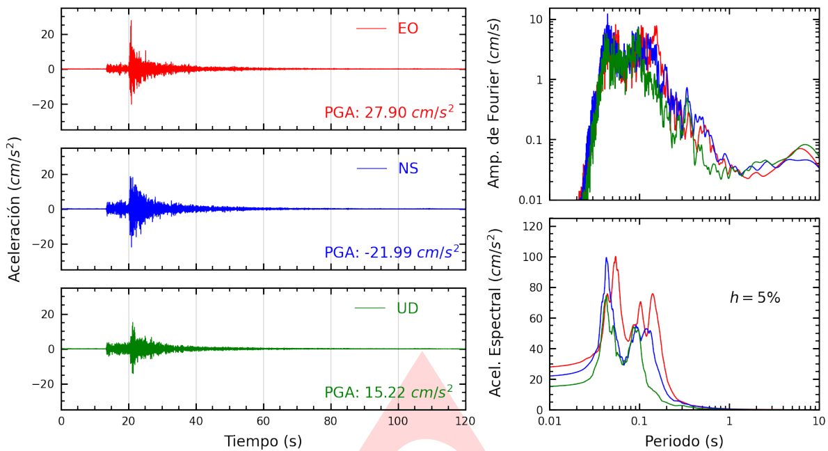
Figura A.1: Registros tiempo-historia, espectros de Fourier y de respuesta en las direcciones EO, NS y vertical de la estación SROSA. Sismo de Ancon, Lima - Lima de 2022-07-29, 23:20:12 (Hora local)
