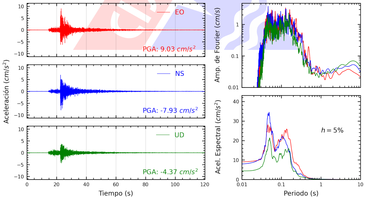
Figura A.6: Registros tiempo-historia, espectros de Fourier y de respuesta en las direcciones EO, NS y vertical de la estación INDEP. Sismo de Ancon, Lima - Lima de 2022-07-29, 23:20:12 (Hora local)
