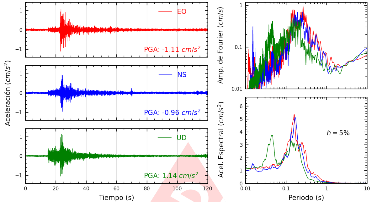
Figura A.31: Registros tiempo-historia, espectros de Fourier y de respuesta en las direcciones EO, NS y vertical de la estación DSML. Sismo de Ancon, Lima - Lima de 2022-07-29, 23:20:12 (Hora local)
