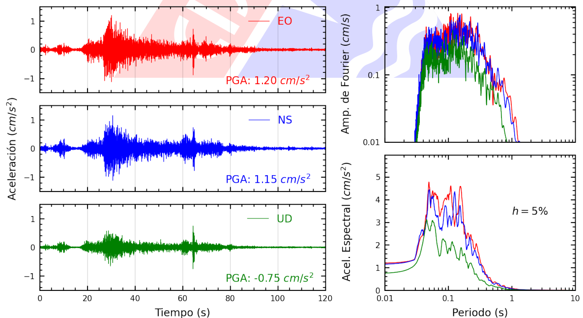
Figura A.30: Registros tiempo-historia, espectros de Fourier y de respuesta en las direcciones EO, NS y vertical de la estación BRISA. Sismo de Ancon, Lima - Lima de 2022-07-29, 23:20:12 (Hora local)
