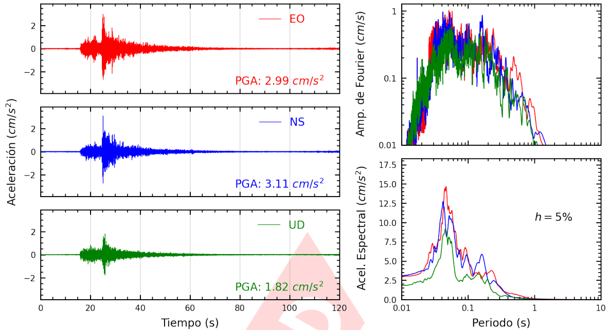
Figura A.19: Registros tiempo-historia, espectros de Fourier y de respuesta en las direcciones EO, NS y vertical de la estación BORJA. Sismo de Ancon, Lima - Lima de 2022-07-29, 23:20:12 (Hora local)
