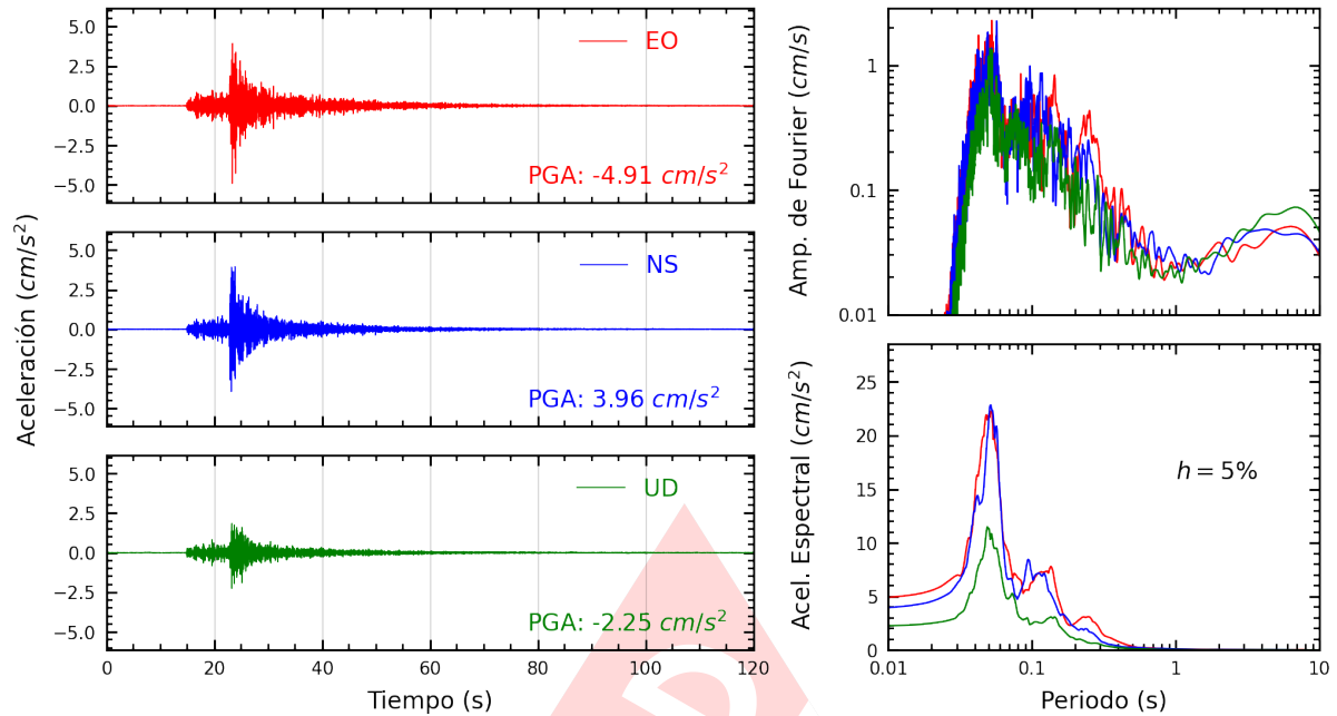
Figura A.13: Registros tiempo-historia, espectros de Fourier y de respuesta en las direcciones EO, NS y vertical de la estación UCSS. Sismo de Ancon, Lima - Lima de 2022-07-29, 23:20:12 (Hora local)
