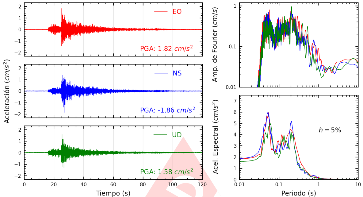
Figura A.27: Registros tiempo-historia, espectros de Fourier y de respuesta en las direcciones EO, NS y vertical de la estación IMCA. Sismo de Ancon, Lima - Lima de 2022-07-29, 23:20:12 (Hora local)
