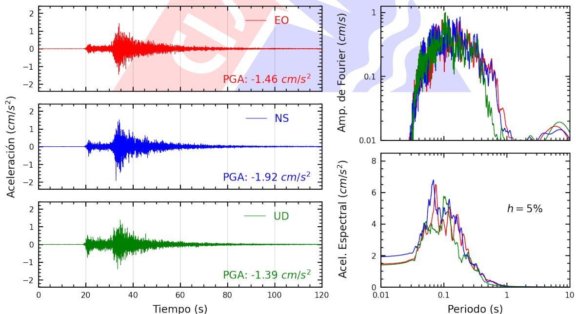
Figura A.26: Registros tiempo-historia, espectros de Fourier y de respuesta en las direcciones EO, NS y vertical de la estación CARAL. Sismo de Ancon, Lima - Lima de 2022-07-29, 23:20:12 (Hora local)
