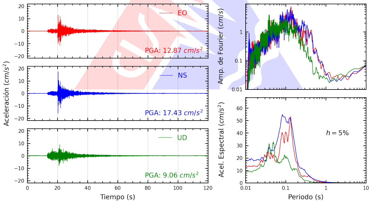
Figura A.2: Registros tiempo-historia, espectros de Fourier y de respuesta en las direcciones EO, NS y vertical de la estación ANCON. Sismo de Ancon, Lima - Lima de 2022-07-29, 23:20:12 (Hora local)
