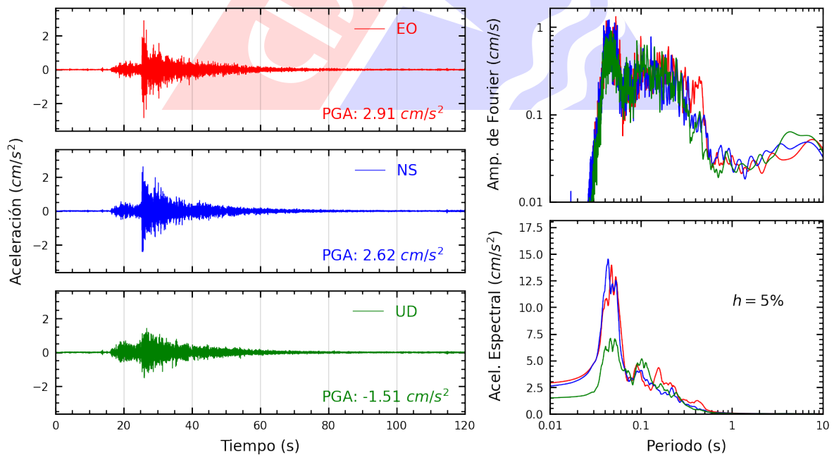
Figura A.20: Registros tiempo-historia, espectros de Fourier y de respuesta en las direcciones EO, NS y vertical de la estación USMP. Sismo de Ancon, Lima - Lima de 2022-07-29, 23:20:12 (Hora local)
