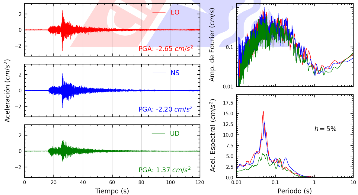
Figura A.22: Registros tiempo-historia, espectros de Fourier y de respuesta en las direcciones EO, NS y vertical de la estación SERVI. Sismo de Ancon, Lima - Lima de 2022-07-29, 23:20:12 (Hora local)
