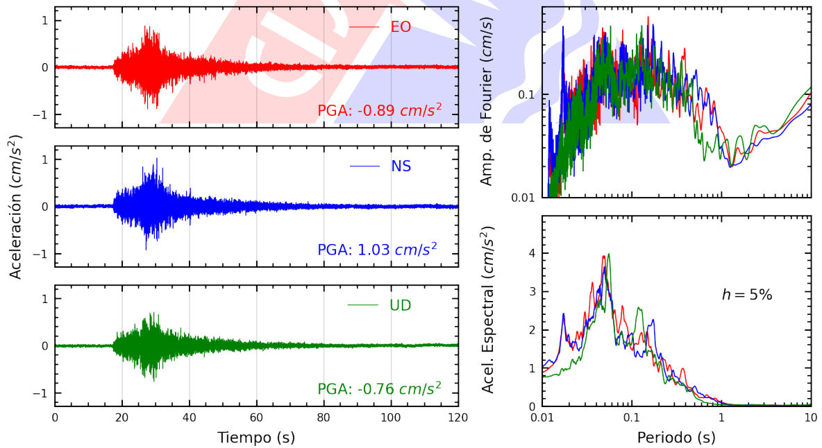
Figura A.34: Registros tiempo-historia, espectros de Fourier y de respuesta en las direcciones EO, NS y vertical de la estación UNMSM. Sismo de Ancon, Lima - Lima de 2022-07-29, 23:20:12 (Hora local)
