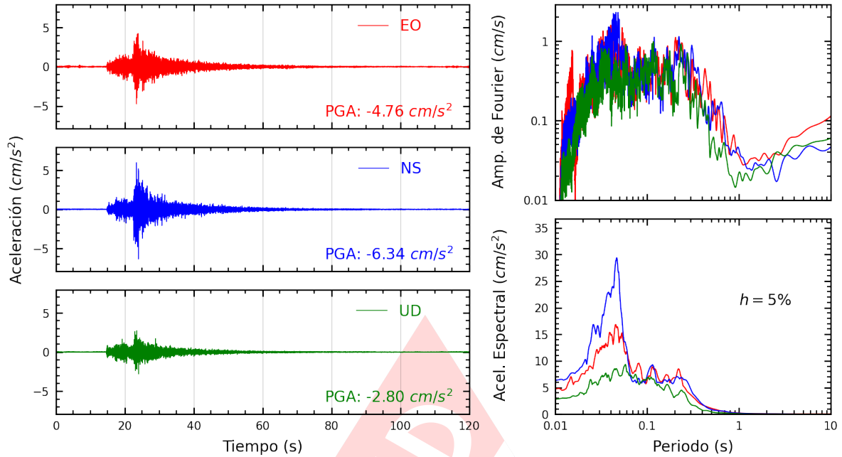
Figura A.9: Registros tiempo-historia, espectros de Fourier y de respuesta en las direcciones EO, NS y vertical de la estación COMAS. Sismo de Ancon, Lima - Lima de 2022-07-29, 23:20:12 (Hora local)
