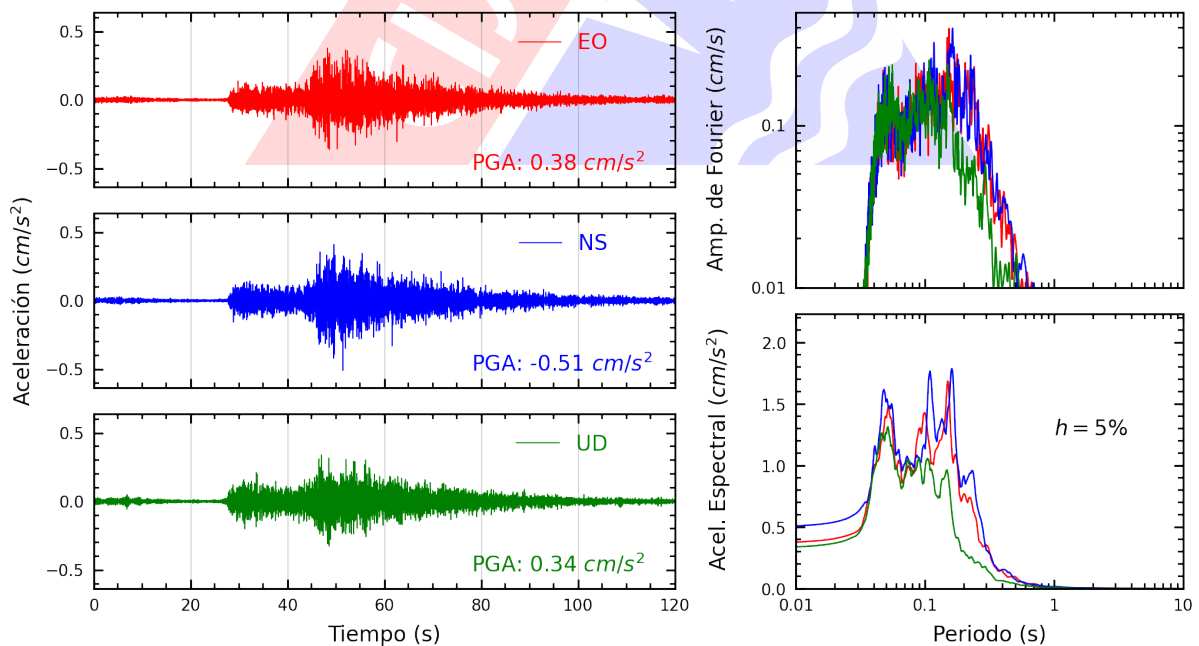
Figura A.36: Registros tiempo-historia, espectros de Fourier y de respuesta en las direcciones EO, NS y vertical de la estación ASIA. Sismo de Ancon, Lima - Lima de 2022-07-29, 23:20:12 (Hora local)
