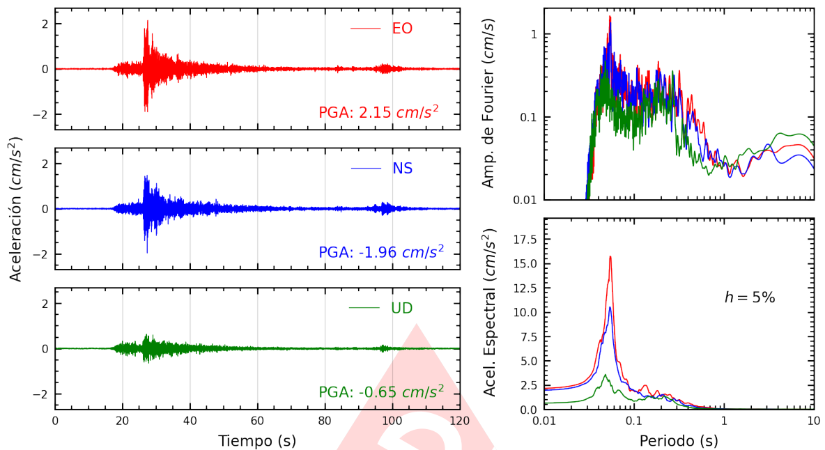
Figura A.23: Registros tiempo-historia, espectros de Fourier y de respuesta en las direcciones EO, NS y vertical de la estación UPCVI. Sismo de Ancon, Lima - Lima de 2022-07-29, 23:20:12 (Hora local)
