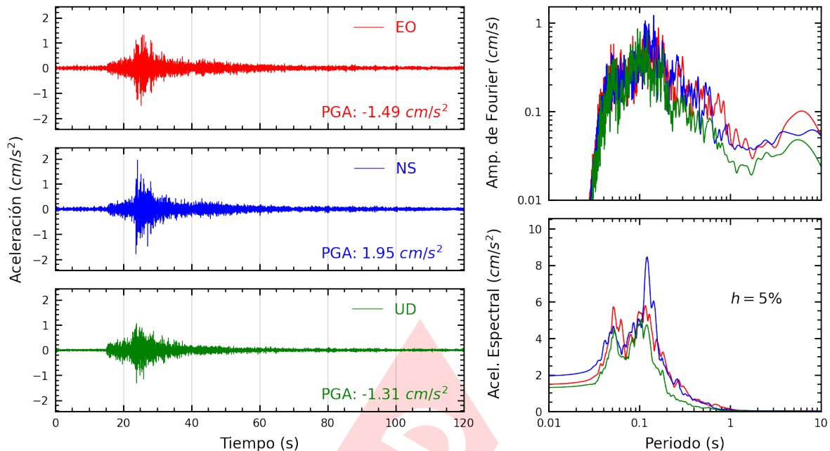
Figura A.25: Registros tiempo-historia, espectros de Fourier y de respuesta en las direcciones EO, NS y vertical de la estación NISTA. Sismo de Ancon, Lima - Lima de 2022-07-29, 23:20:12 (Hora local)
