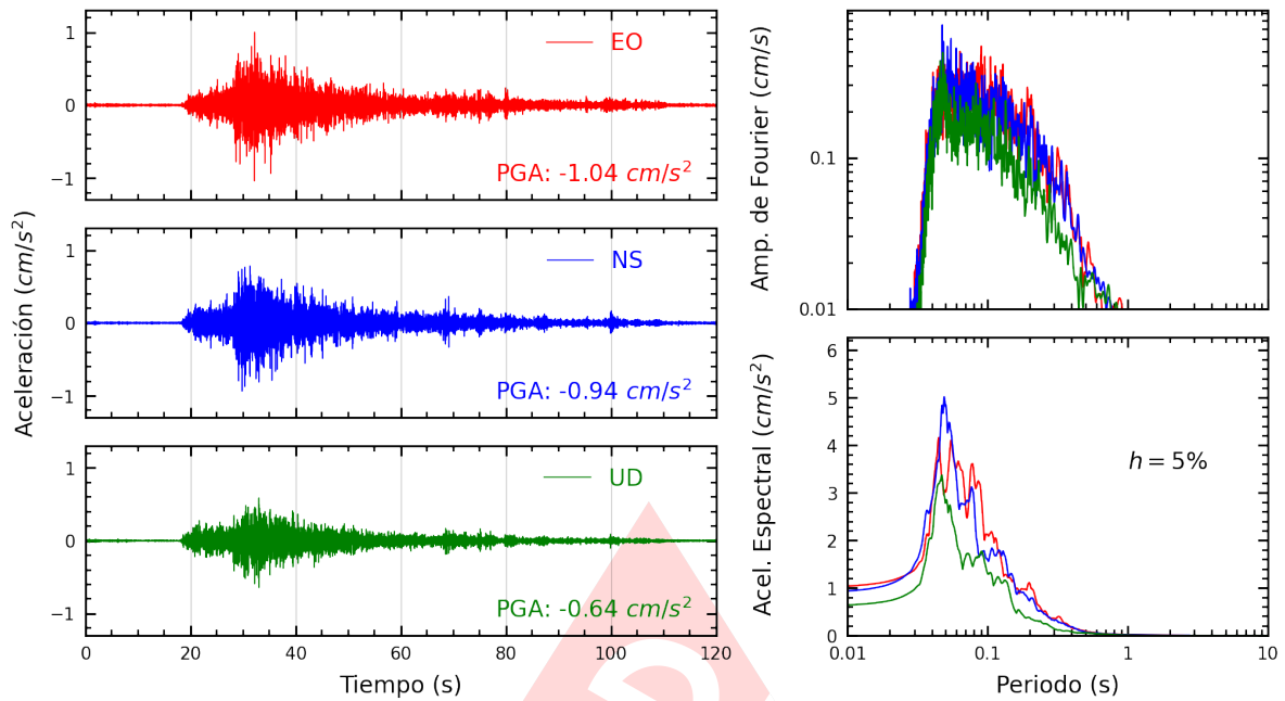
Figura A.33: Registros tiempo-historia, espectros de Fourier y de respuesta en las direcciones EO, NS y vertical de la estación PACHA. Sismo de Ancon, Lima - Lima de 2022-07-29, 23:20:12 (Hora local)
