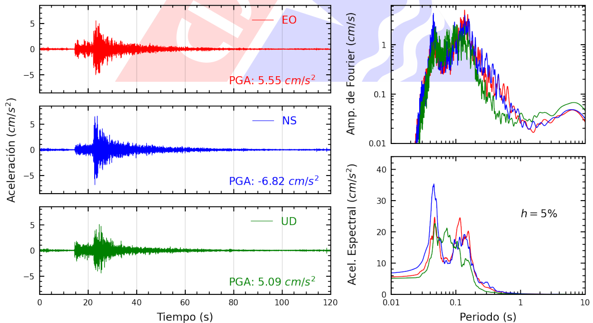
Figura A.8: Registros tiempo-historia, espectros de Fourier y de respuesta en las direcciones EO, NS y vertical de la estación CARAB. Sismo de Ancon, Lima - Lima de 2022-07-29, 23:20:12 (Hora local)
