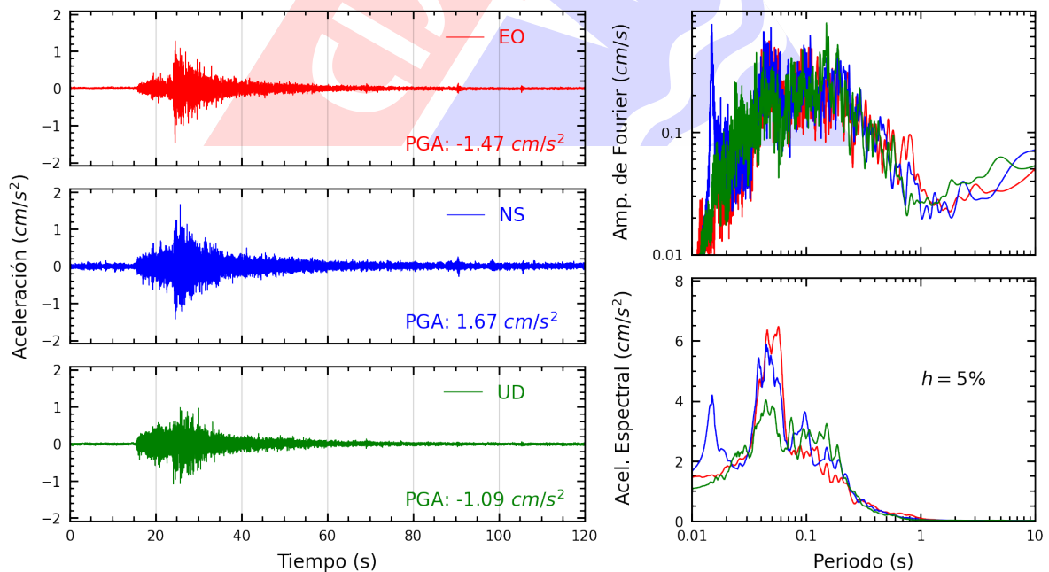
Figura A.28: Registros tiempo-historia, espectros de Fourier y de respuesta en las direcciones EO, NS y vertical de la estación UNFV. Sismo de Ancon, Lima - Lima de 2022-07-29, 23:20:12 (Hora local)
