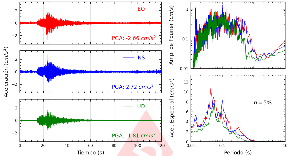
Figura A.21: Registros tiempo-historia, espectros de Fourier y de respuesta en las direcciones EO, NS y vertical de la estación MADRE. Sismo de Ancon, Lima - Lima de 2022-07-29, 23:20:12 (Hora local)
