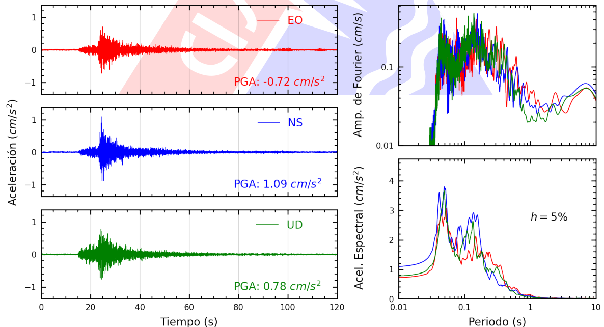
Figura A.32: Registros tiempo-historia, espectros de Fourier y de respuesta en las direcciones EO, NS y vertical de la estación BONDY. Sismo de Ancon, Lima - Lima de 2022-07-29, 23:20:12 (Hora local)
