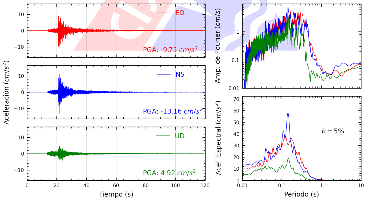
Figura A.4: Registros tiempo-historia, espectros de Fourier y de respuesta en las direcciones EO, NS y vertical de la estación DEFEN. Sismo de Ancon, Lima - Lima de 2022-07-29, 23:20:12 (Hora local)
