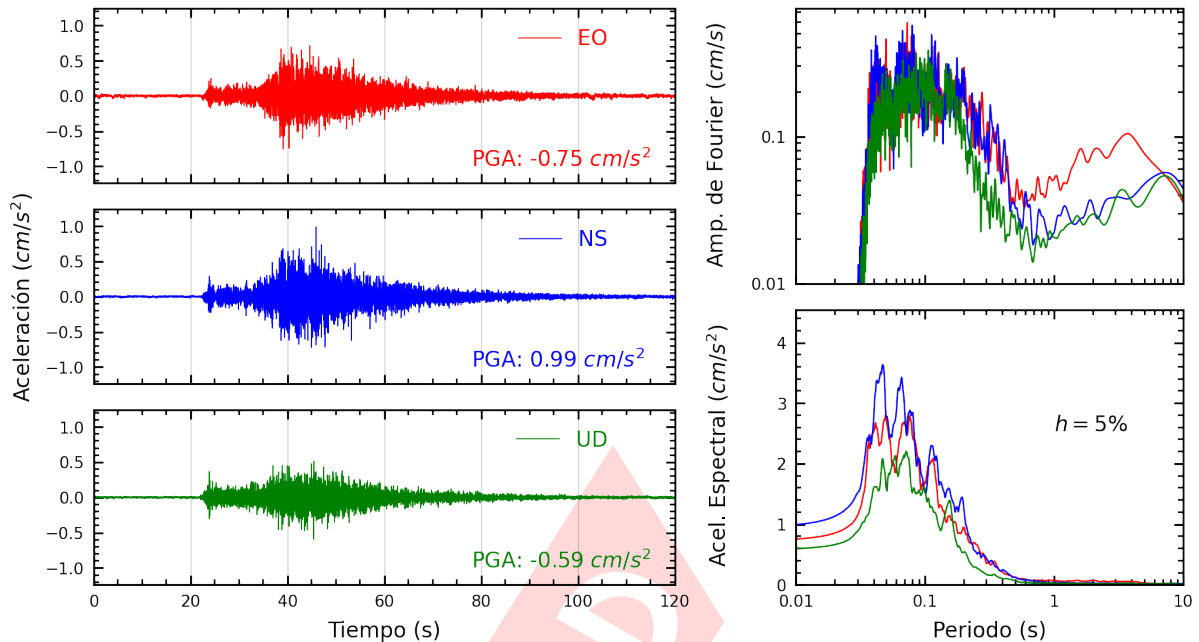
Figura A.35: Registros tiempo-historia, espectros de Fourier y de respuesta en las direcciones EO, NS y vertical de la estación UNAB. Sismo de Ancon, Lima - Lima de 2022-07-29, 23:20:12 (Hora local)
