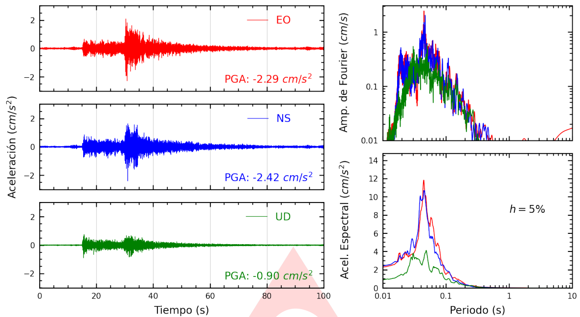
Figura A.1: Registros tiempo-historia, espectros de Fourier y de respuesta en las direcciones EO, NS y vertical de la estación SCTRU. Sismo de Chimbote, Santa - Ancash de 2022-08-20, 02:22:43 (Hora local)
