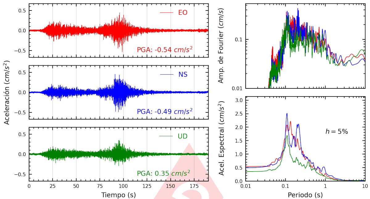
Figura A.31: Registros tiempo-historia, espectros de Fourier y de respuesta en las direcciones EO, NS y vertical de la estación AMORE. Sismo de Atico, Caraveli - Arequipa del 2022-09-08, 16:59:41 (Hora local)
