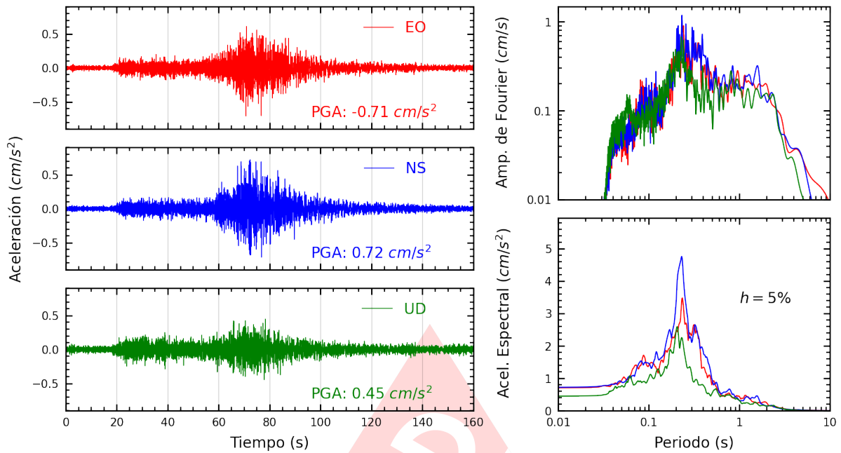
Figura A.25: Registros tiempo-historia, espectros de Fourier y de respuesta en las direcciones EO, NS y vertical de la estación UJBG2. Sismo de Atico, Caraveli - Arequipa del 2022-09-08, 16:59:41 (Hora local)
