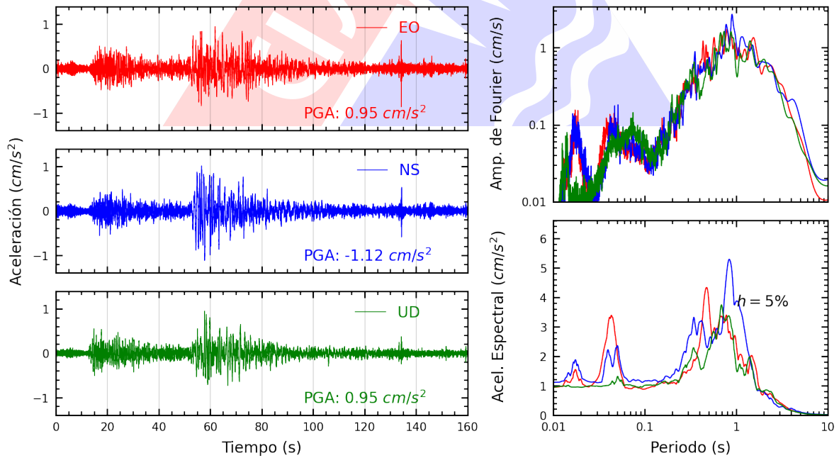
Figura A.16: Registros tiempo-historia, espectros de Fourier y de respuesta en las direcciones EO, NS y vertical de la estación SCAYA. Sismo de Atico, Caraveli - Arequipa del 2022-09-08, 16:59:41 (Hora local)
