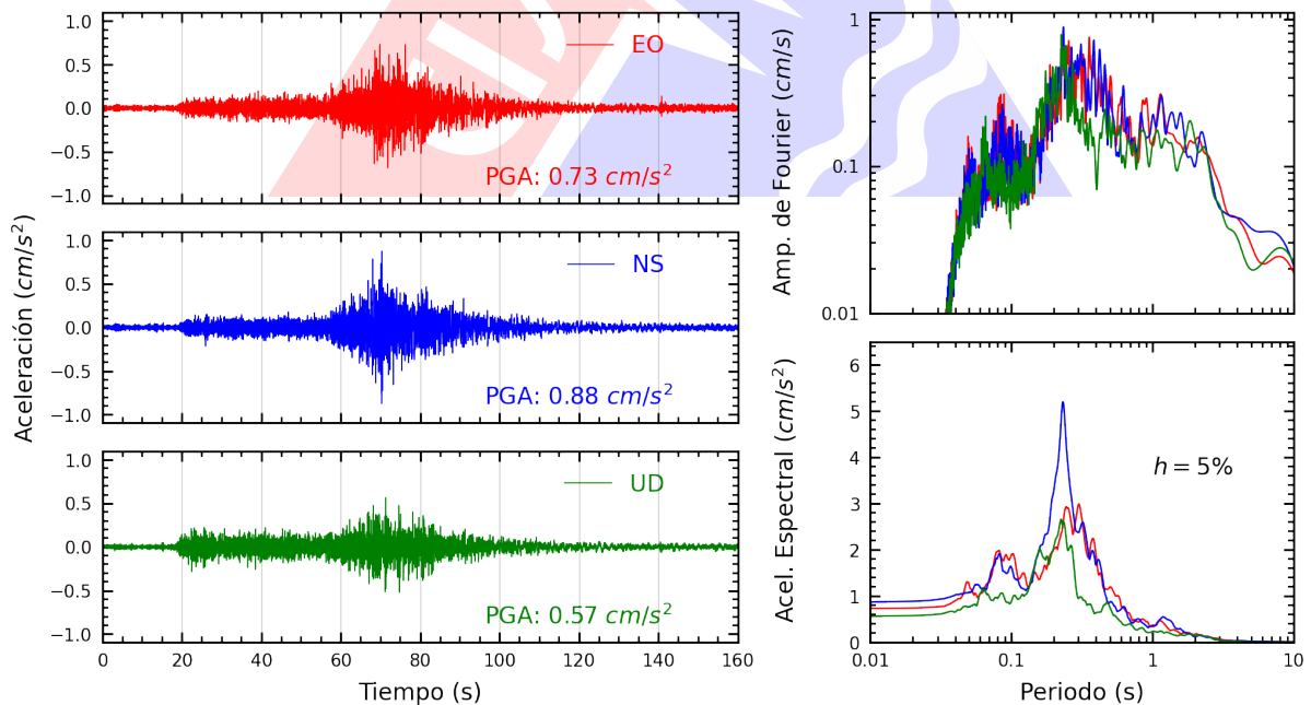
Figura A.22: Registros tiempo-historia, espectros de Fourier y de respuesta en las direcciones EO, NS y vertical de la estación CREY. Sismo de Atico, Caraveli - Arequipa del 2022-09-08, 16:59:41 (Hora local)
