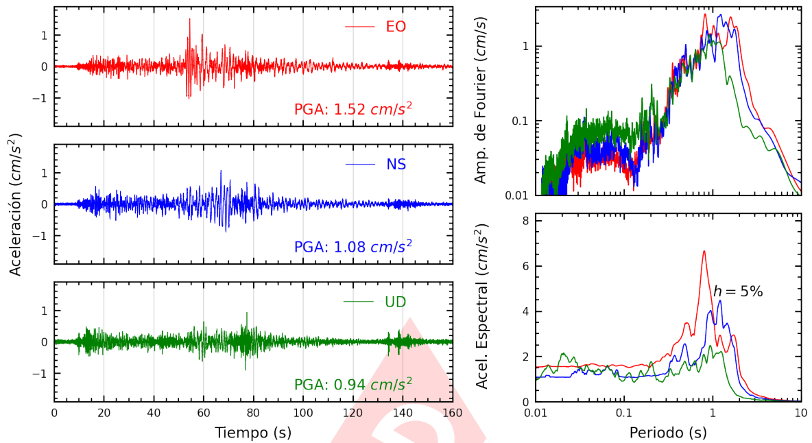
Figura A.11: Registros tiempo-historia, espectros de Fourier y de respuesta en las direcciones EO, NS y vertical de la estación SCCUS. Sismo de Atico, Caraveli - Arequipa del 2022-09-08, 16:59:41 (Hora local)
