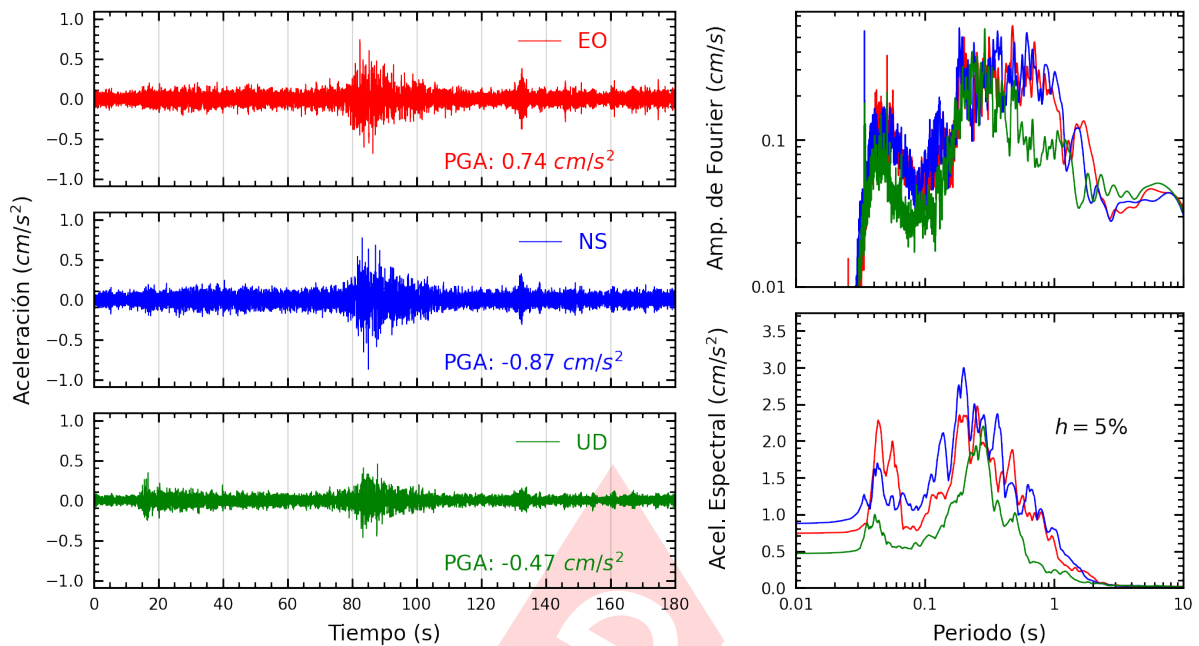
Figura A.23: Registros tiempo-historia, espectros de Fourier y de respuesta en las direcciones EO, NS y vertical de la estación UPCVI. Sismo de Atico, Caraveli - Arequipa del 2022-09-08, 16:59:41 (Hora local)
