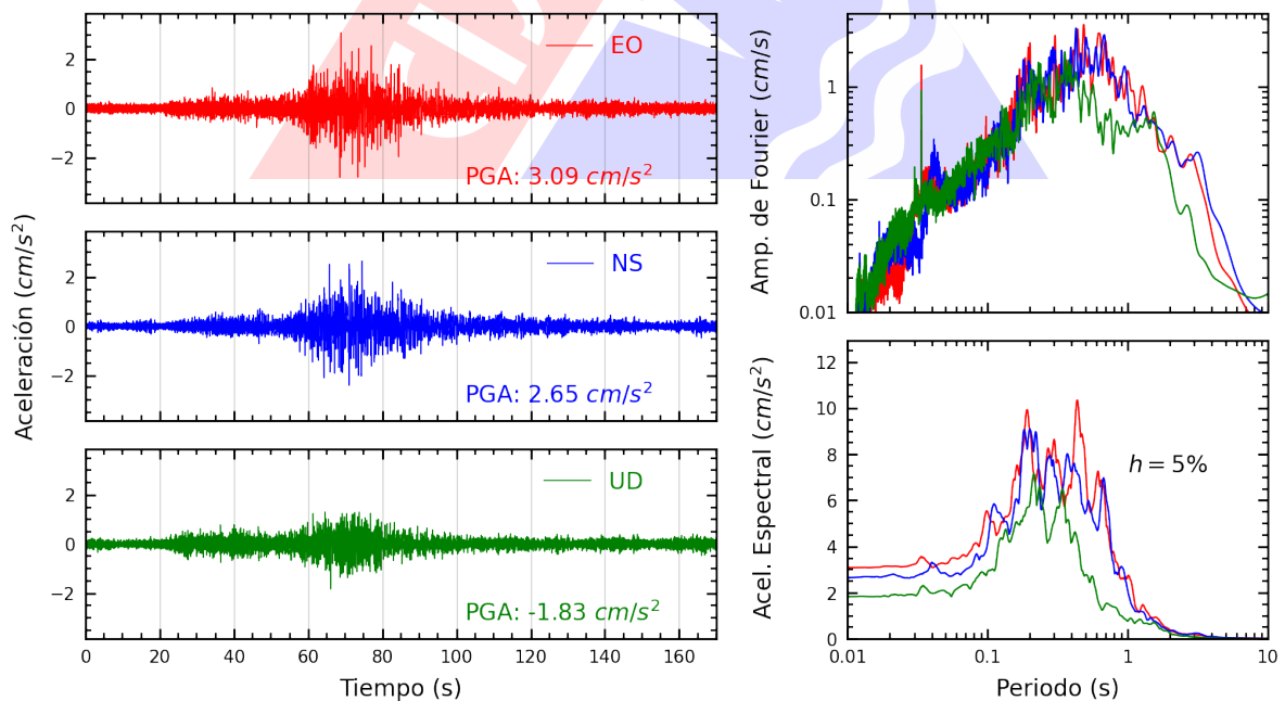
Figura A.4: Registros tiempo-historia, espectros de Fourier y de respuesta en las direcciones EO, NS y vertical de la estación SCICA. Sismo de Atico, Caraveli - Arequipa del 2022-09-08, 16:59:41 (Hora local)
