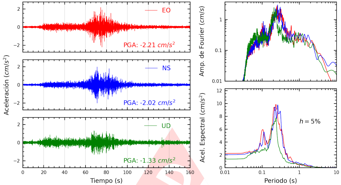
Figura A.5: Registros tiempo-historia, espectros de Fourier y de respuesta en las direcciones EO, NS y vertical de la estación SCTAC. Sismo de Atico, Caraveli - Arequipa del 2022-09-08, 16:59:41 (Hora local)
