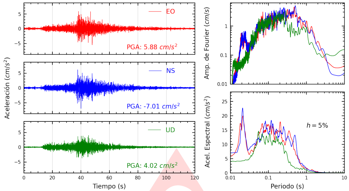
Figura A.1: Registros tiempo-historia, espectros de Fourier y de respuesta en las direcciones EO, NS y vertical de la estación SCARQ. Sismo de Atico, Caraveli - Arequipa del 2022-09-08, 16:59:41 (Hora local)
