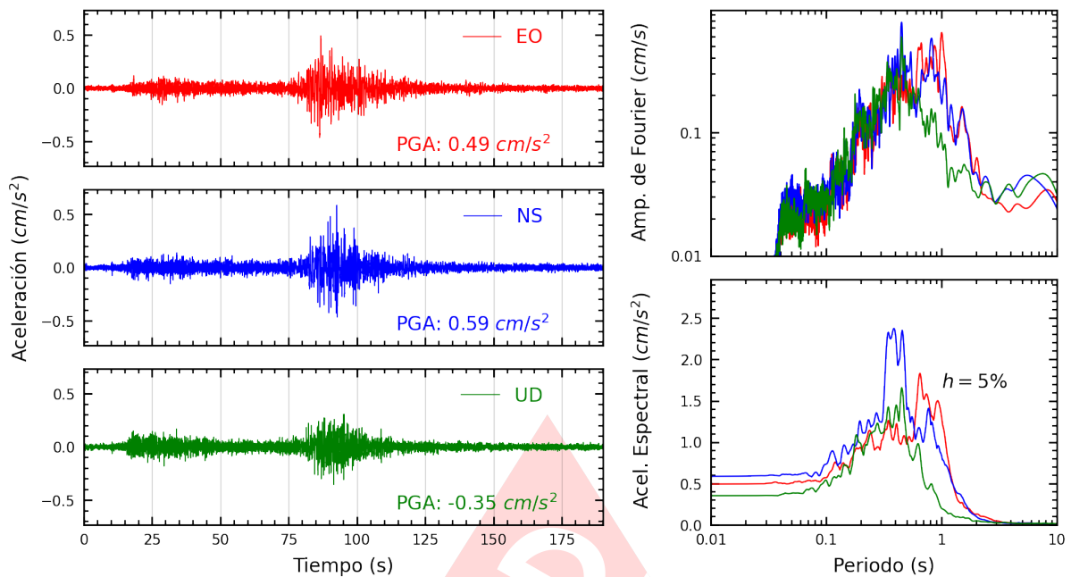
Figura A.29: Registros tiempo-historia, espectros de Fourier y de respuesta en las direcciones EO, NS y vertical de la estación UNFV. Sismo de Atico, Caraveli - Arequipa del 2022-09-08, 16:59:41 (Hora local)
