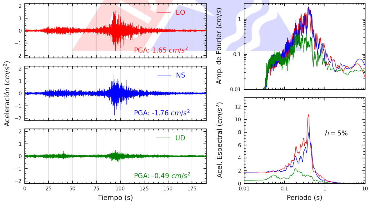
Figura A.8: Registros tiempo-historia, espectros de Fourier y de respuesta en las direcciones EO, NS y vertical de la estación DEFEN. Sismo de Atico, Caraveli - Arequipa del 2022-09-08, 16:59:41 (Hora local)
