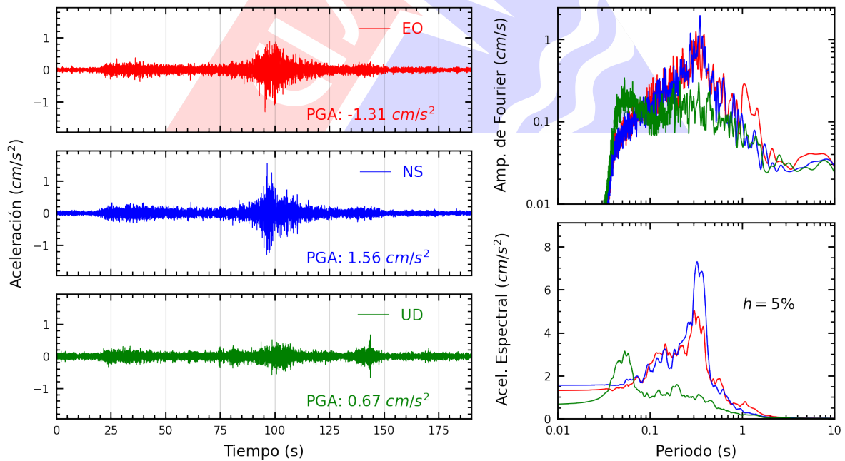
Figura A.10: Registros tiempo-historia, espectros de Fourier y de respuesta en las direcciones EO, NS y vertical de la estación ANCON. Sismo de Atico, Caraveli - Arequipa del 2022-09-08, 16:59:41 (Hora local)
