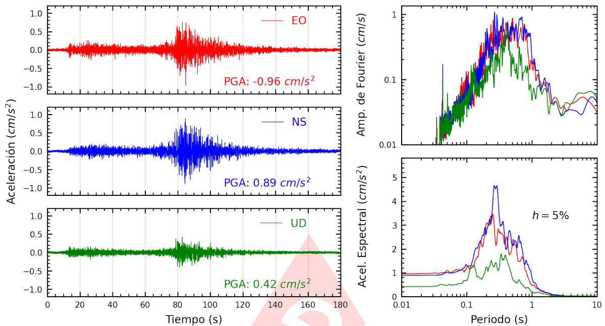
Figura A.19: Registros tiempo-historia, espectros de Fourier y de respuesta en las direcciones EO, NS y vertical de la estación USILP. Sismo de Atico, Caraveli - Arequipa del 2022-09-08, 16:59:41 (Hora local)
