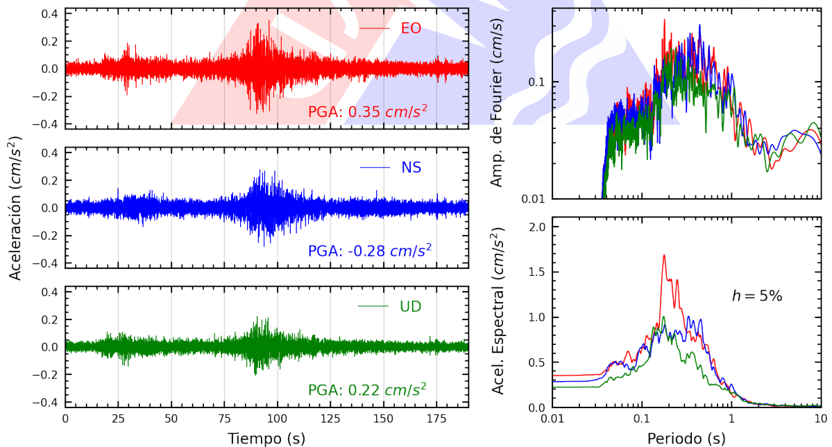
Figura A.36: Registros tiempo-historia, espectros de Fourier y de respuesta en las direcciones EO, NS y vertical de la estación FICPE. Sismo de Atico, Caraveli - Arequipa del 2022-09-08, 16:59:41 (Hora local)
