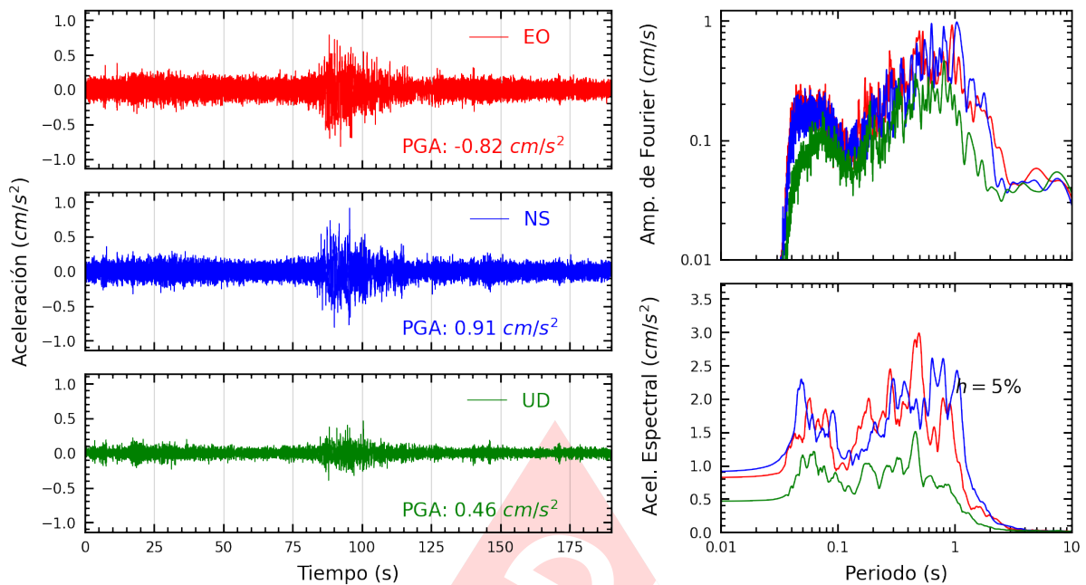
Figura A.21: Registros tiempo-historia, espectros de Fourier y de respuesta en las direcciones EO, NS y vertical de la estación NISTA. Sismo de Atico, Caraveli - Arequipa del 2022-09-08, 16:59:41 (Hora local)
