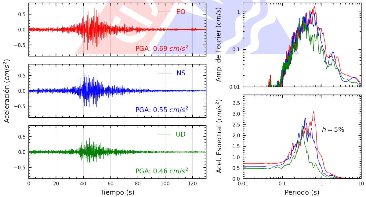
Figura A.26: Registros tiempo-historia, espectros de Fourier y de respuesta en las direcciones EO, NS y vertical de la estación CARAL. Sismo de Atico, Caraveli - Arequipa del 2022-09-08, 16:59:41 (Hora local)
