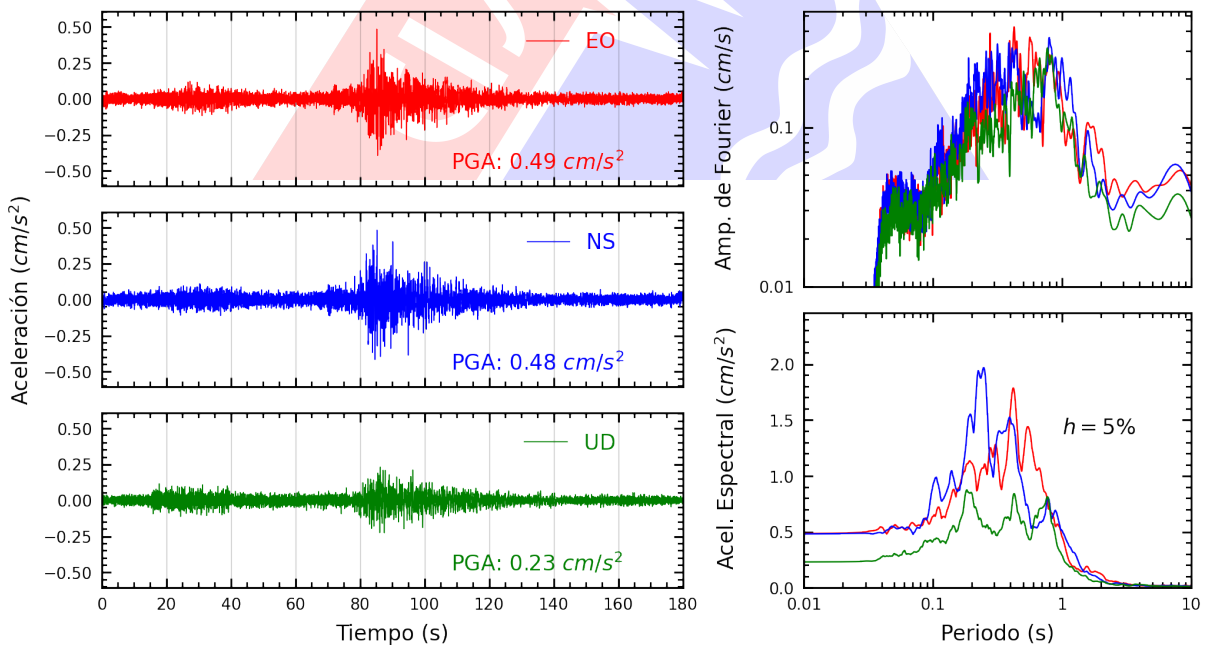
Figura A.32: Registros tiempo-historia, espectros de Fourier y de respuesta en las direcciones EO, NS y vertical de la estación SERVI. Sismo de Atico, Caraveli - Arequipa del 2022-09-08, 16:59:41 (Hora local)
