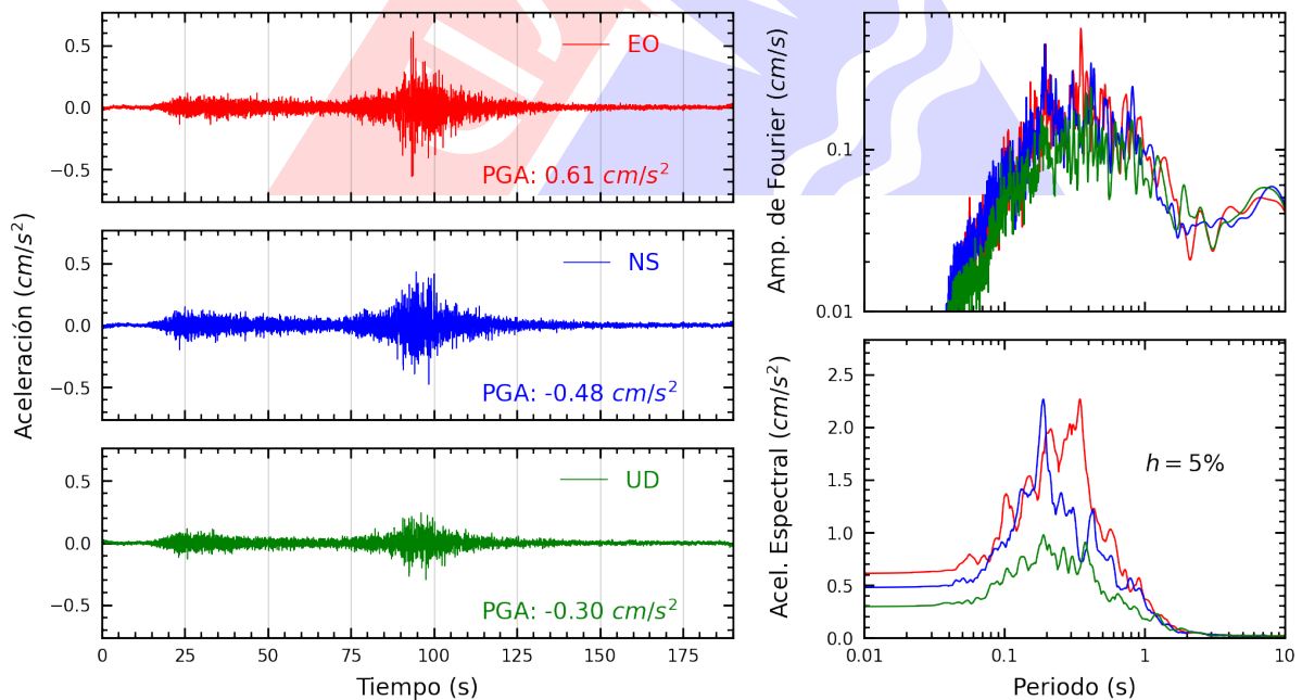
Figura A.28: Registros tiempo-historia, espectros de Fourier y de respuesta en las direcciones EO, NS y vertical de la estación IPEN. Sismo de Atico, Caraveli - Arequipa del 2022-09-08, 16:59:41 (Hora local)
