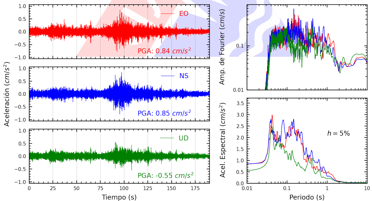
Figura A.24: Registros tiempo-historia, espectros de Fourier y de respuesta en las direcciones EO, NS y vertical de la estación SROSA. Sismo de Atico, Caraveli - Arequipa del 2022-09-08, 16:59:41 (Hora local)
