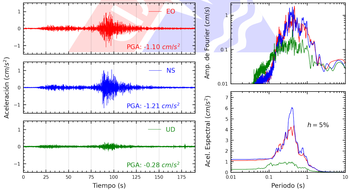
Figura A.14: Registros tiempo-historia, espectros de Fourier y de respuesta en las direcciones EO, NS y vertical de la estación ACAPU. Sismo de Atico, Caraveli - Arequipa del 2022-09-08, 16:59:41 (Hora local)
