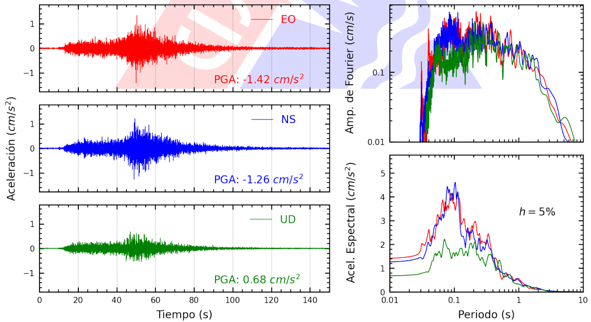
Figura A.12: Registros tiempo-historia, espectros de Fourier y de respuesta en las direcciones EO, NS y vertical de la estación UNAM. Sismo de Atico, Caraveli - Arequipa del 2022-09-08, 16:59:41 (Hora local)
