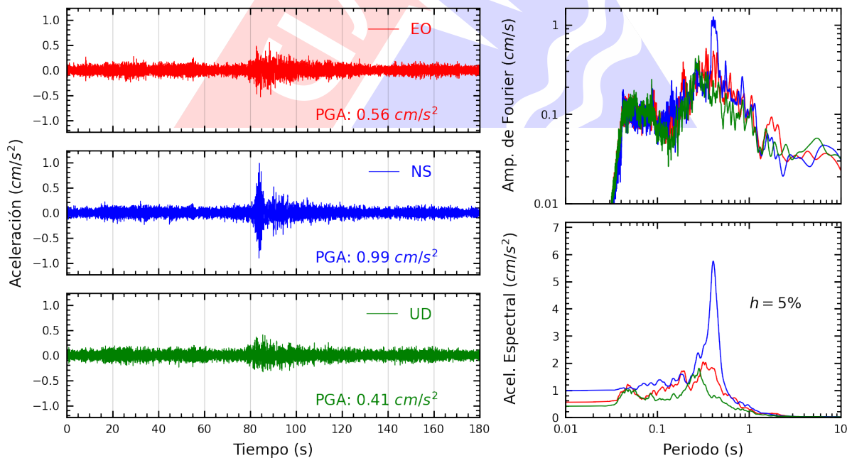
Figura A.18: Registros tiempo-historia, espectros de Fourier y de respuesta en las direcciones EO, NS y vertical de la estación URPPE. Sismo de Atico, Caraveli - Arequipa del 2022-09-08, 16:59:41 (Hora local)
