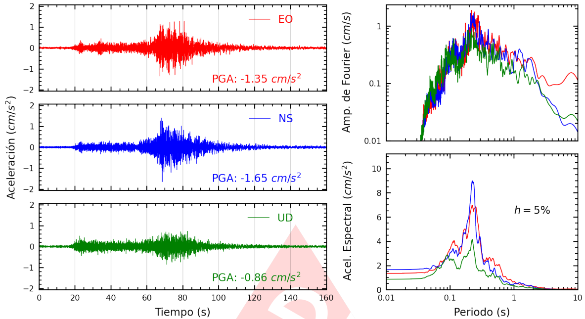
Figura A.9: Registros tiempo-historia, espectros de Fourier y de respuesta en las direcciones EO, NS y vertical de la estación UJBG3. Sismo de Atico, Caraveli - Arequipa del 2022-09-08, 16:59:41 (Hora local)
