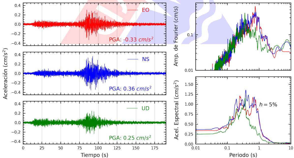
Figura A.34: Registros tiempo-historia, espectros de Fourier y de respuesta en las direcciones EO, NS y vertical de la estación UNMSM. Sismo de Atico, Caraveli - Arequipa del 2022-09-08, 16:59:41 (Hora local)
