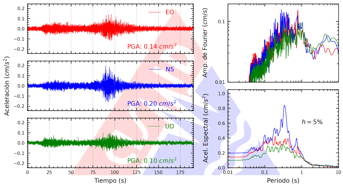
Figura A.37: Registros tiempo-historia, espectros de Fourier y de respuesta en las direcciones EO, NS y vertical de la estación UCSS. Sismo de Atico, Caraveli - Arequipa del 2022-09-08, 16:59:41 (Hora local)
