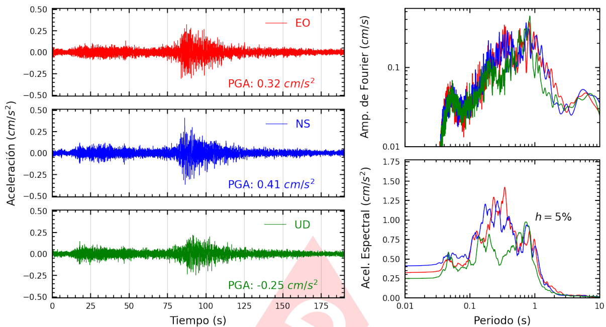
Figura A.33: Registros tiempo-historia, espectros de Fourier y de respuesta en las direcciones EO, NS y vertical de la estación CENEP. Sismo de Atico, Caraveli - Arequipa del 2022-09-08, 16:59:41 (Hora local)
