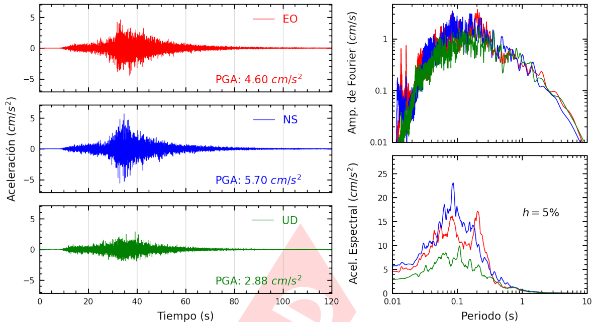
Figura A.3: Registros tiempo-historia, espectros de Fourier y de respuesta en las direcciones EO, NS y vertical de la estación UNSA. Sismo de Atico, Caraveli - Arequipa del 2022-09-08, 16:59:41 (Hora local)
