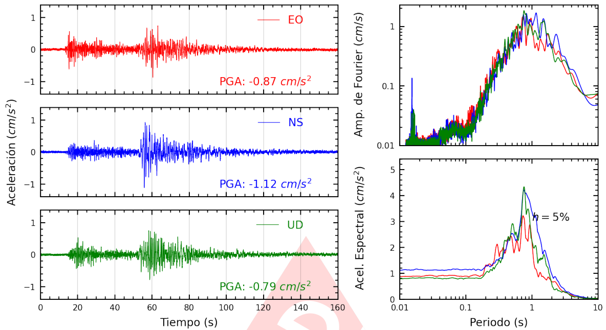
Figura A.15: Registros tiempo-historia, espectros de Fourier y de respuesta en las direcciones EO, NS y vertical de la estación UNSCH. Sismo de Atico, Caraveli - Arequipa del 2022-09-08, 16:59:41 (Hora local)
