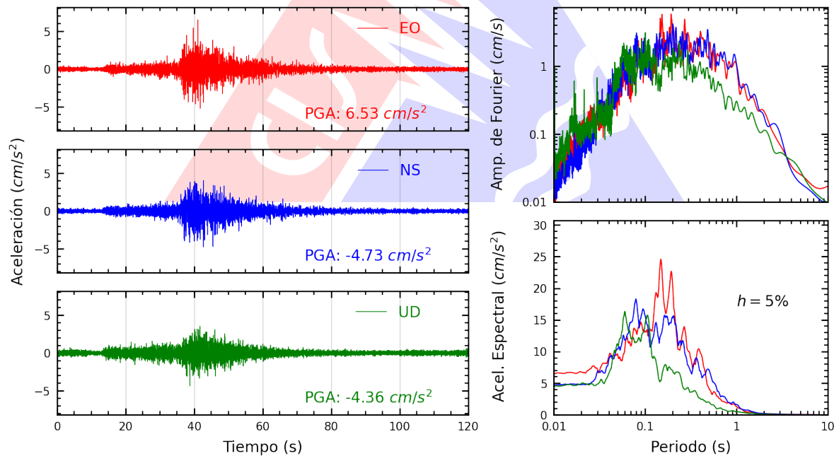
Figura A.2: Registros tiempo-historia, espectros de Fourier y de respuesta en las direcciones EO, NS y vertical de la estación SCAR2. Sismo de Atico, Caraveli - Arequipa del 2022-09-08, 16:59:41 (Hora local)
