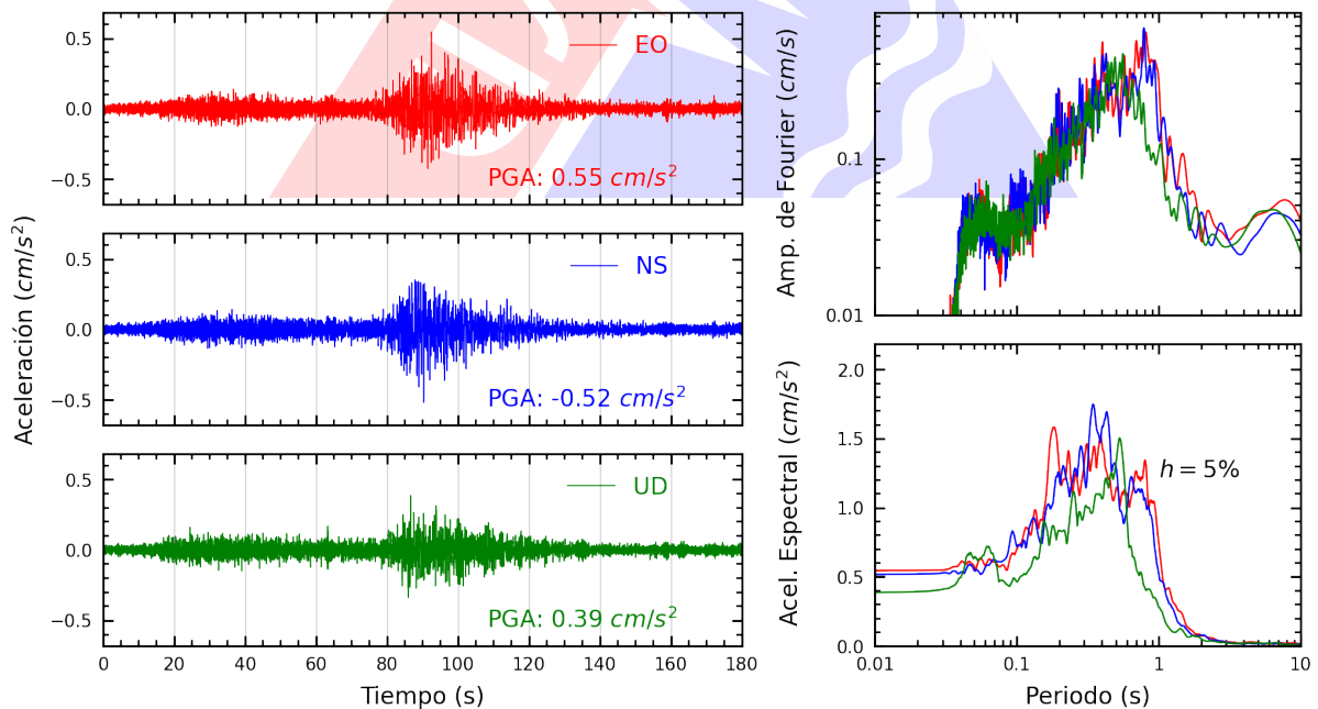
Figura A.30: Registros tiempo-historia, espectros de Fourier y de respuesta en las direcciones EO, NS y vertical de la estación IMCA. Sismo de Atico, Caraveli - Arequipa del 2022-09-08, 16:59:41 (Hora local)
