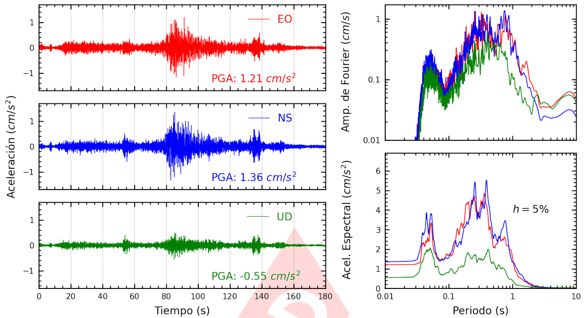
Figura A.13: Registros tiempo-historia, espectros de Fourier y de respuesta en las direcciones EO, NS y vertical de la estación BRISA. Sismo de Atico, Caraveli - Arequipa del 2022-09-08, 16:59:41 (Hora local)
