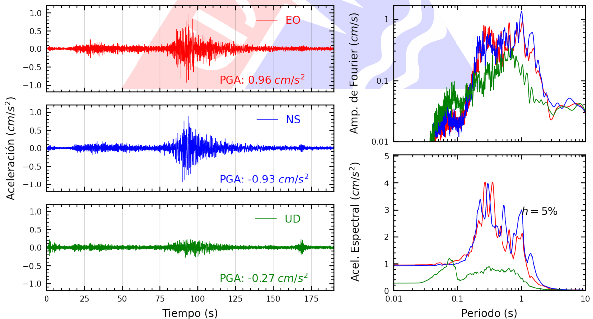
Figura A.20: Registros tiempo-historia, espectros de Fourier y de respuesta en las direcciones EO, NS y vertical de la estación DSMI. Sismo de Atico, Caraveli - Arequipa del 2022-09-08, 16:59:41 (Hora local)
