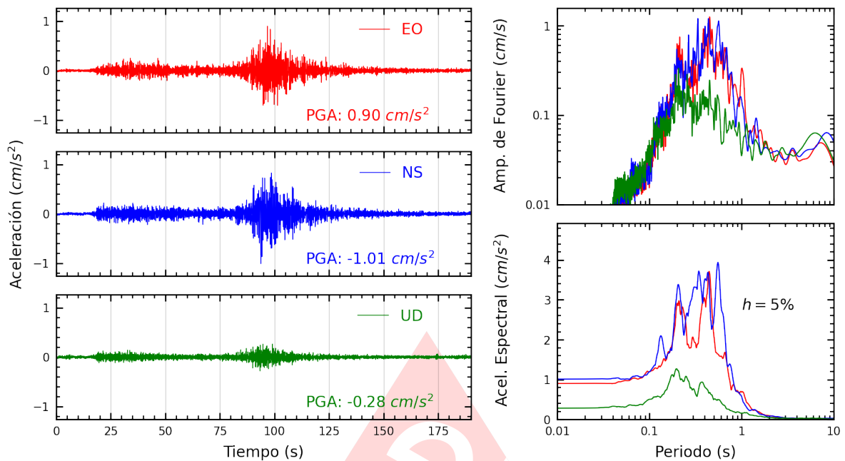
Figura A.17: Registros tiempo-historia, espectros de Fourier y de respuesta en las direcciones EO, NS y vertical de la estación VHAYA. Sismo de Atico, Caraveli - Arequipa del 2022-09-08, 16:59:41 (Hora local)
