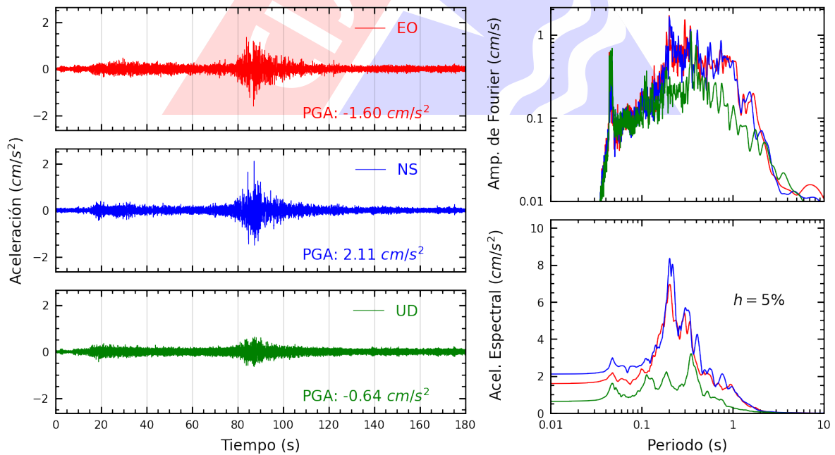
Figura A.6: Registros tiempo-historia, espectros de Fourier y de respuesta en las direcciones EO, NS y vertical de la estación SCCHO. Sismo de Atico, Caraveli - Arequipa del 2022-09-08, 16:59:41 (Hora local)
