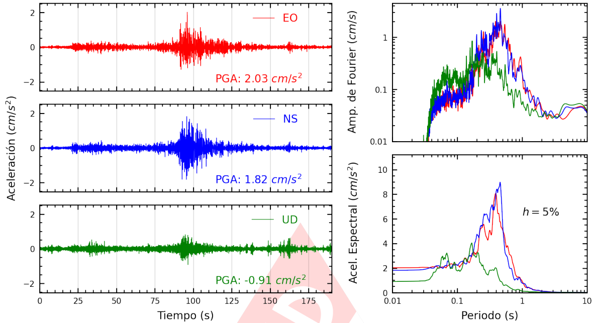
Figura A.7: Registros tiempo-historia, espectros de Fourier y de respuesta en las direcciones EO, NS y vertical de la estación MDPP. Sismo de Atico, Caraveli - Arequipa del 2022-09-08, 16:59:41 (Hora local)
