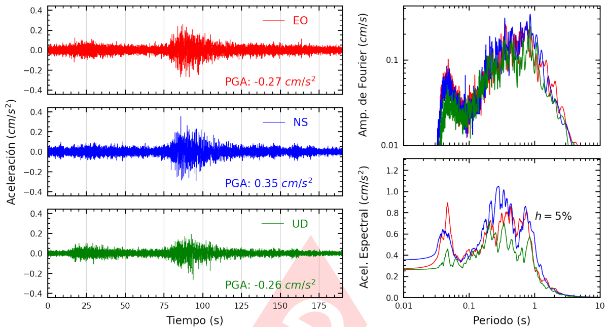
Figura A.35: Registros tiempo-historia, espectros de Fourier y de respuesta en las direcciones EO, NS y vertical de la estación BORJA. Sismo de Atico, Caraveli - Arequipa del 2022-09-08, 16:59:41 (Hora local)
