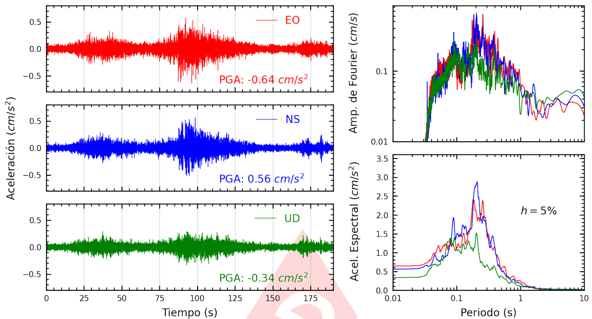
Figura A.27: Registros tiempo-historia, espectros de Fourier y de respuesta en las direcciones EO, NS y vertical de la estación INDEP. Sismo de Atico, Caraveli - Arequipa del 2022-09-08, 16:59:41 (Hora local)
