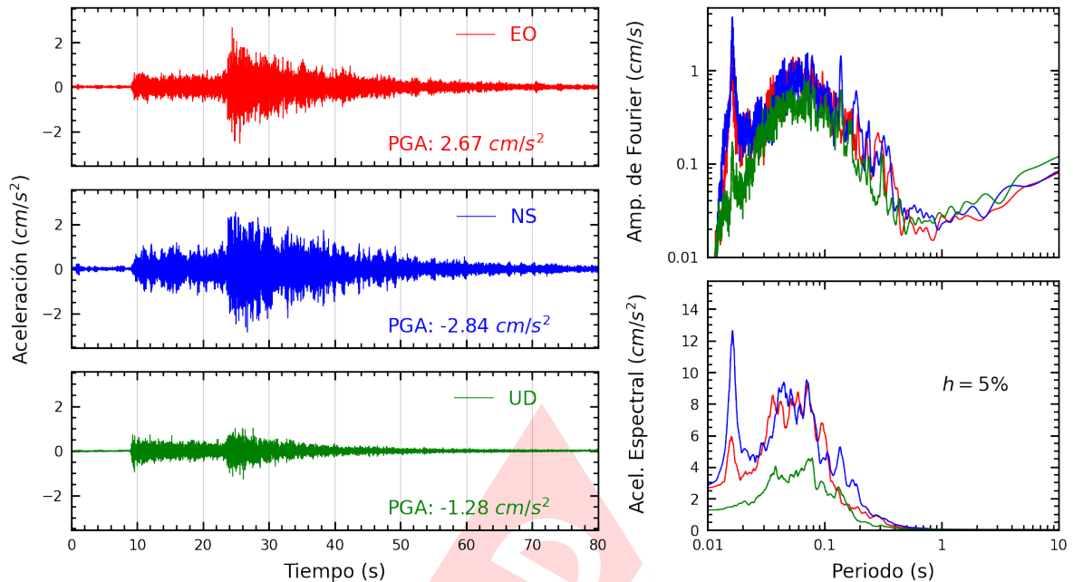
Figura A.5: Registros tiempo-historia, espectros de Fourier y de respuesta en las direcciones EO, NS y vertical de la estación IPEN. Sismo de Canta, Canta - Lima del 2022-09-13, 10:38:29 (Hora local)
