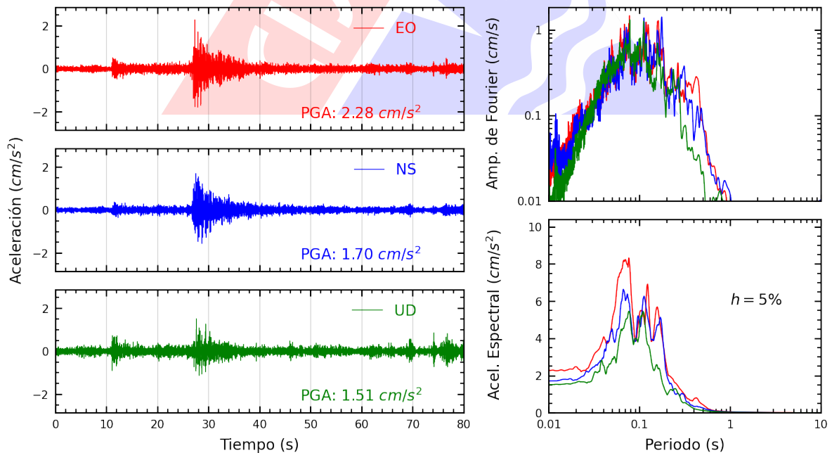
Figura A.8: Registros tiempo-historia, espectros de Fourier y de respuesta en las direcciones EO, NS y vertical de la estación SCOLI. Sismo de Canta, Canta - Lima del 2022-09-13, 10:38:29 (Hora local)
