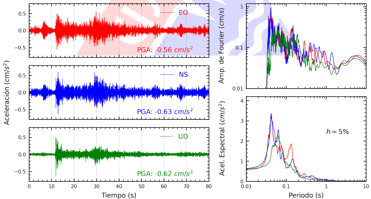
Figura A.32: Registros tiempo-historia, espectros de Fourier y de respuesta en las direcciones EO, NS y vertical de la estación DHNPE. Sismo de Canta, Canta - Lima del 2022-09-13, 10:38:29 (Hora local)
