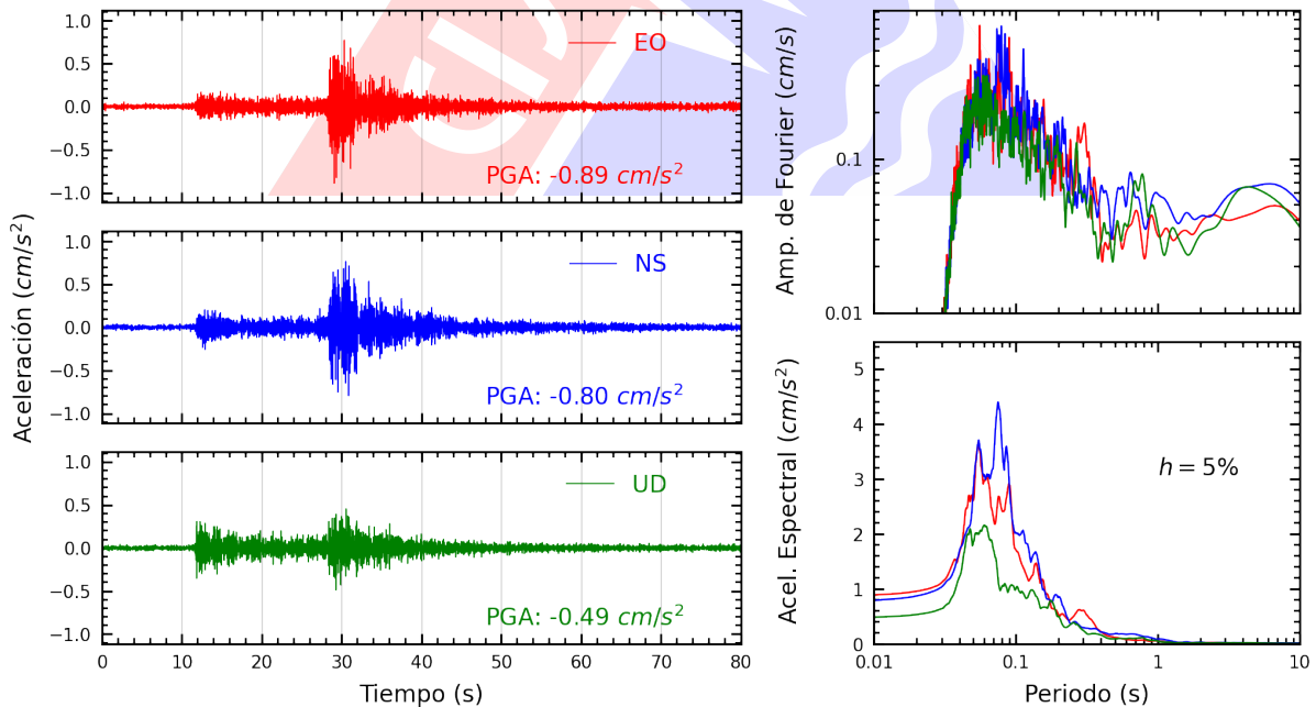
Figura A.26: Registros tiempo-historia, espectros de Fourier y de respuesta en las direcciones EO, NS y vertical de la estación CENEP. Sismo de Canta, Canta - Lima del 2022-09-13, 10:38:29 (Hora local)
