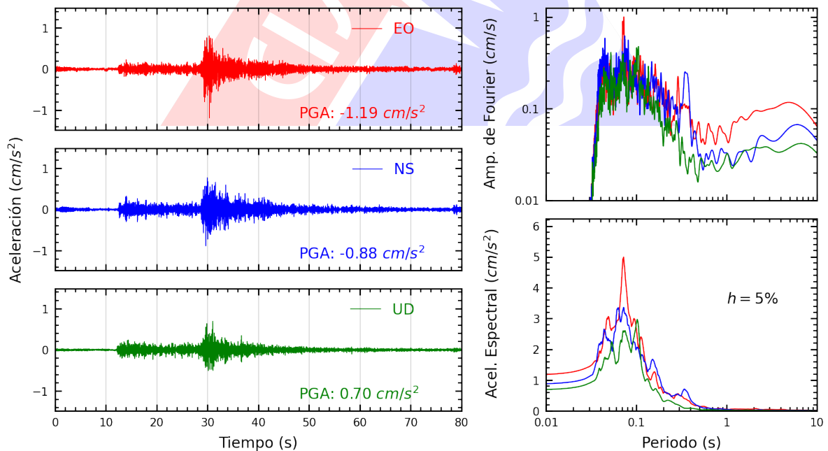
Figura A.18: Registros tiempo-historia, espectros de Fourier y de respuesta en las direcciones EO, NS y vertical de la estación UNAB. Sismo de Canta, Canta - Lima del 2022-09-13, 10:38:29 (Hora local)
