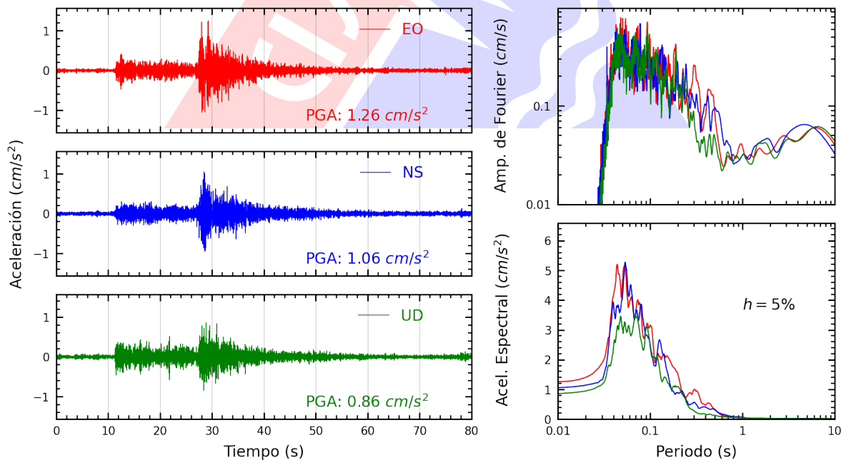
Figura A.16: Registros tiempo-historia, espectros de Fourier y de respuesta en las direcciones EO, NS y vertical de la estación USMP. Sismo de Canta, Canta - Lima del 2022-09-13, 10:38:29 (Hora local)
