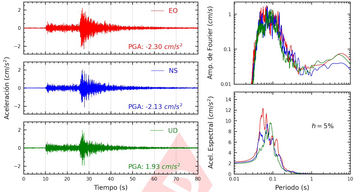
Figura A.7: Registros tiempo-historia, espectros de Fourier y de respuesta en las direcciones EO, NS y vertical de la estación AMORE. Sismo de Canta, Canta - Lima del 2022-09-13, 10:38:29 (Hora local)
