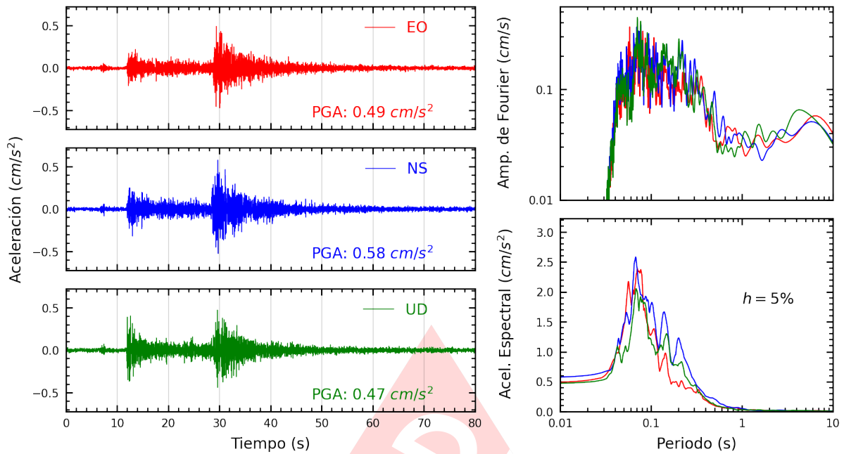
Figura A.33: Registros tiempo-historia, espectros de Fourier y de respuesta en las direcciones EO, NS y vertical de la estación UNFV. Sismo de Canta, Canta - Lima del 2022-09-13, 10:38:29 (Hora local)
