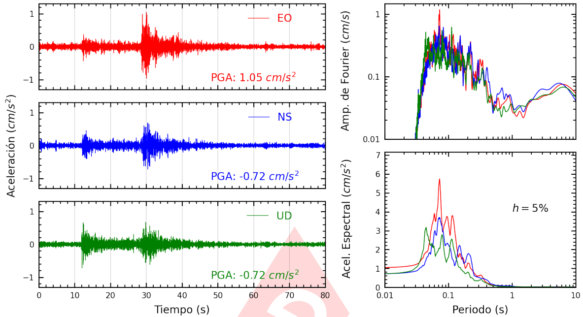
Figura A.25: Registros tiempo-historia, espectros de Fourier y de respuesta en las direcciones EO, NS y vertical de la estación UPCSM. Sismo de Canta, Canta - Lima del 2022-09-13, 10:38:29 (Hora local)
