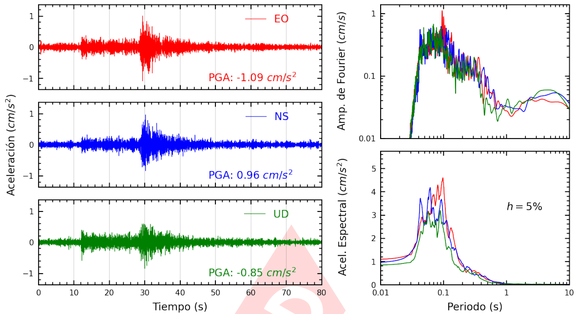
Figura A.21: Registros tiempo-historia, espectros de Fourier y de respuesta en las direcciones EO, NS y vertical de la estación URPE. Sismo de Canta, Canta - Lima del 2022-09-13, 10:38:29 (Hora local)
