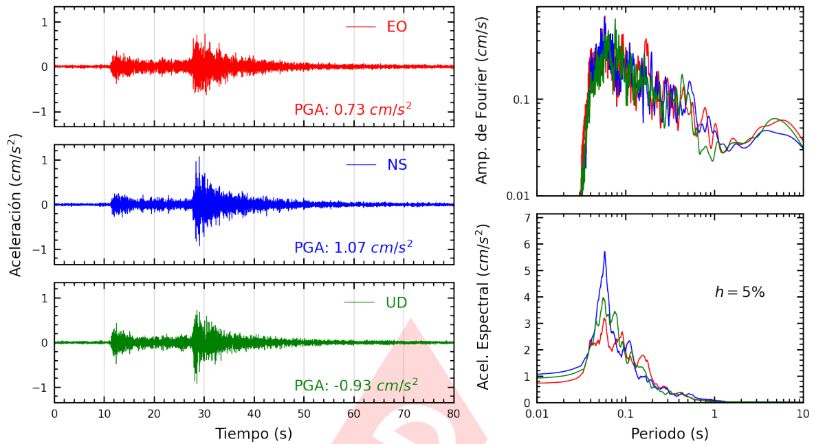
Figura A.23: Registros tiempo-historia, espectros de Fourier y de respuesta en las direcciones EO, NS y vertical de la estación IMCA. Sismo de Canta, Canta - Lima del 2022-09-13, 10:38:29 (Hora local)
