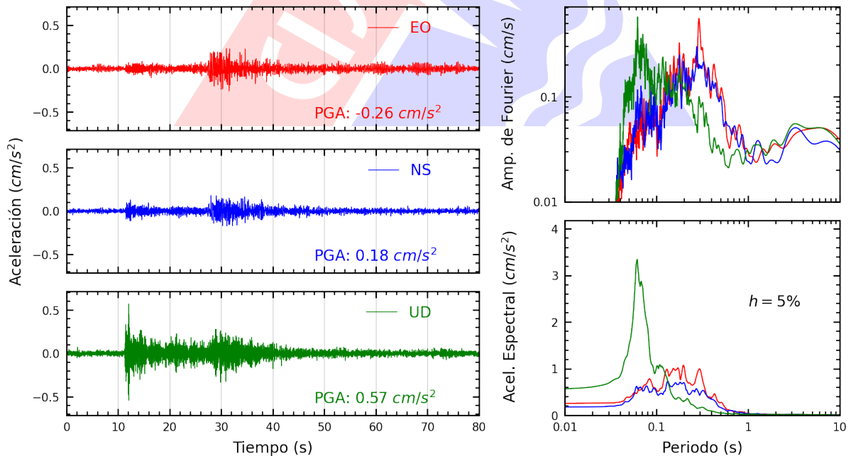
Figura A.34: Registros tiempo-historia, espectros de Fourier y de respuesta en las direcciones EO, NS y vertical de la estación ACAPU. Sismo de Canta, Canta - Lima del 2022-09-13, 10:38:29 (Hora local)
