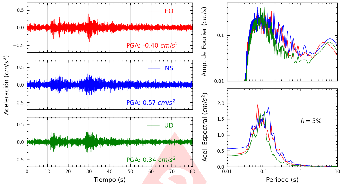
Figura A.35: Registros tiempo-historia, espectros de Fourier y de respuesta en las direcciones EO, NS y vertical de la estación NISTA. Sismo de Canta, Canta - Lima del 2022-09-13, 10:38:29 (Hora local)
