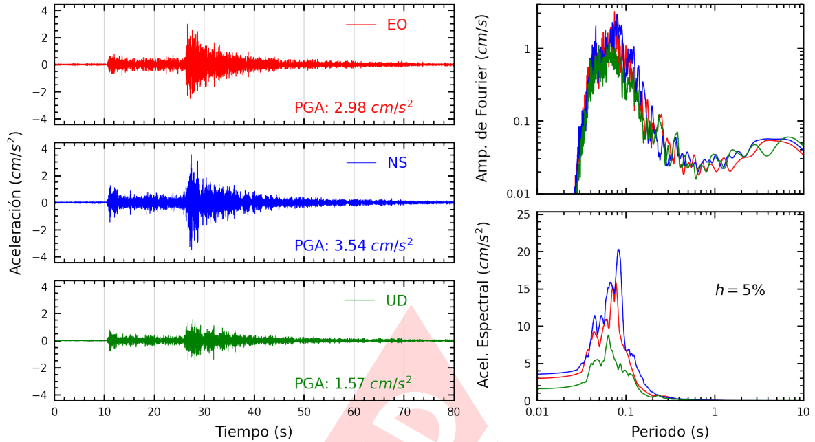
Figura A.3: Registros tiempo-historia, espectros de Fourier y de respuesta en las direcciones EO, NS y vertical de la estación JOSEO. Sismo de Canta, Canta - Lima del 2022-09-13, 10:38:29 (Hora local)
