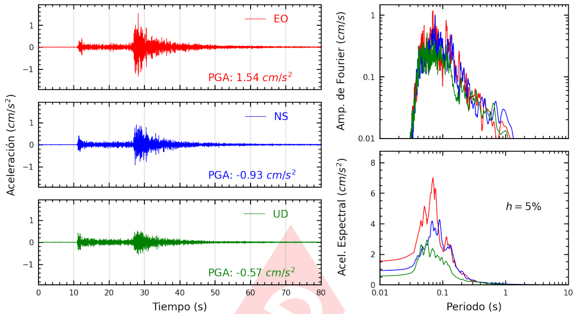
Figura A.13: Registros tiempo-historia, espectros de Fourier y de respuesta en las direcciones EO, NS y vertical de la estación ATARJ. Sismo de Canta, Canta - Lima del 2022-09-13, 10:38:29 (Hora local)
