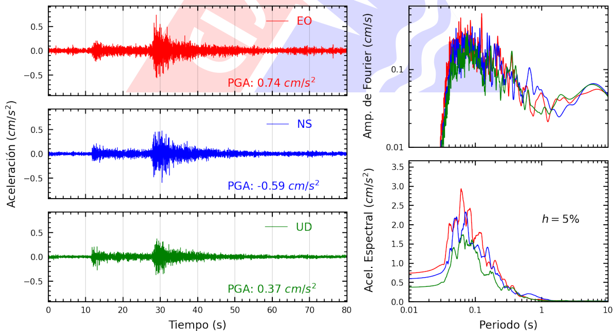
Figura A.30: Registros tiempo-historia, espectros de Fourier y de respuesta en las direcciones EO, NS y vertical de la estación INICT. Sismo de Canta, Canta - Lima del 2022-09-13, 10:38:29 (Hora local)
