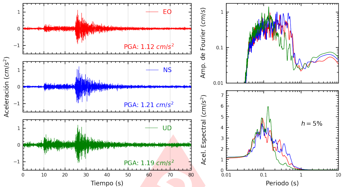
Figura A.17: Registros tiempo-historia, espectros de Fourier y de respuesta en las direcciones EO, NS y vertical de la estación MDPP. Sismo de Canta, Canta - Lima del 2022-09-13, 10:38:29 (Hora local)
