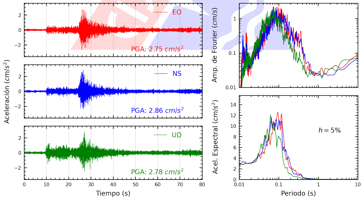
Figura A.4: Registros tiempo-historia, espectros de Fourier y de respuesta en las direcciones EO, NS y vertical de la estación ANCON. Sismo de Canta, Canta - Lima del 2022-09-13, 10:38:29 (Hora local)
