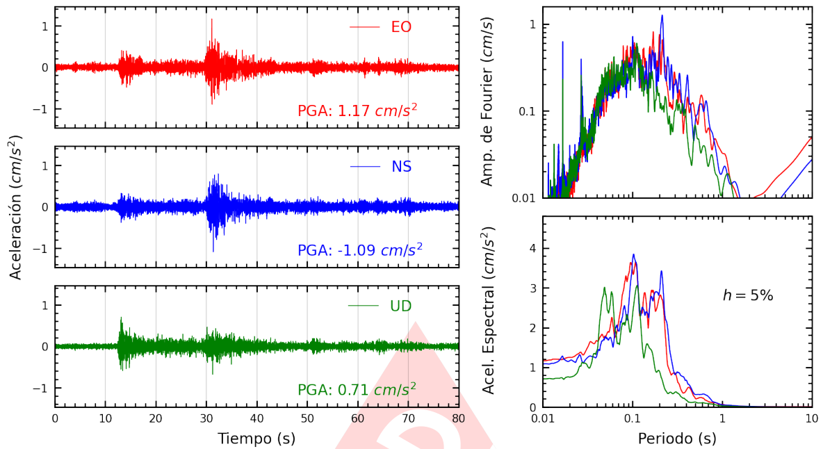
Figura A.19: Registros tiempo-historia, espectros de Fourier y de respuesta en las direcciones EO, NS y vertical de la estación SCCHO. Sismo de Canta, Canta - Lima del 2022-09-13, 10:38:29 (Hora local)
