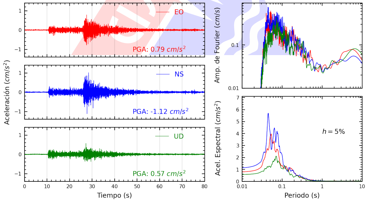
Figura A.20: Registros tiempo-historia, espectros de Fourier y de respuesta en las direcciones EO, NS y vertical de la estación COMAS. Sismo de Canta, Canta - Lima del 2022-09-13, 10:38:29 (Hora local)
