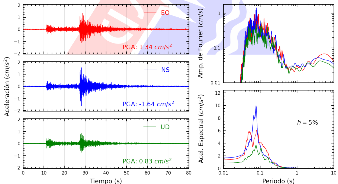
Figura A.12: Registros tiempo-historia, espectros de Fourier y de respuesta en las direcciones EO, NS y vertical de la estación FICPE. Sismo de Canta, Canta - Lima del 2022-09-13, 10:38:29 (Hora local)
