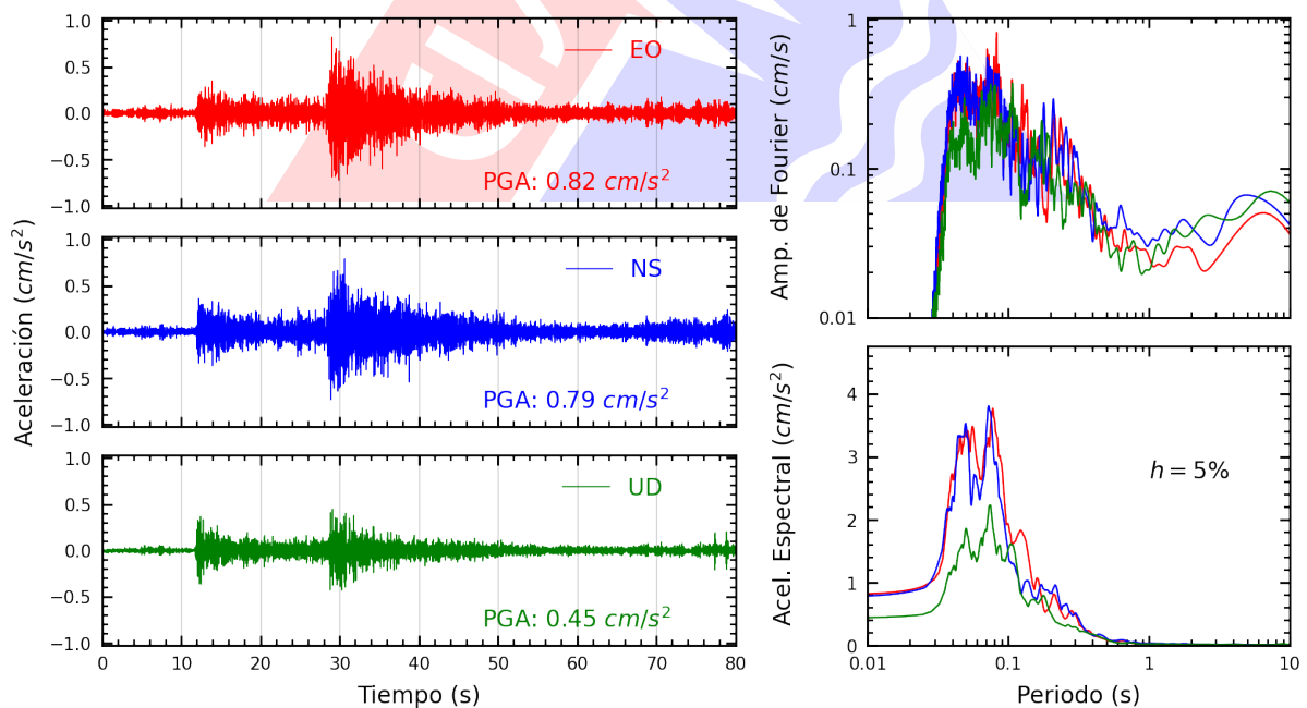
Figura A.28: Registros tiempo-historia, espectros de Fourier y de respuesta en las direcciones EO, NS y vertical de la estación CEPRE. Sismo de Canta, Canta - Lima del 2022-09-13, 10:38:29 (Hora local)
