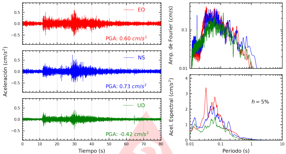
Figura A.31: Registros tiempo-historia, espectros de Fourier y de respuesta en las direcciones EO, NS y vertical de la estación BORJA. Sismo de Canta, Canta - Lima del 2022-09-13, 10:38:29 (Hora local)
