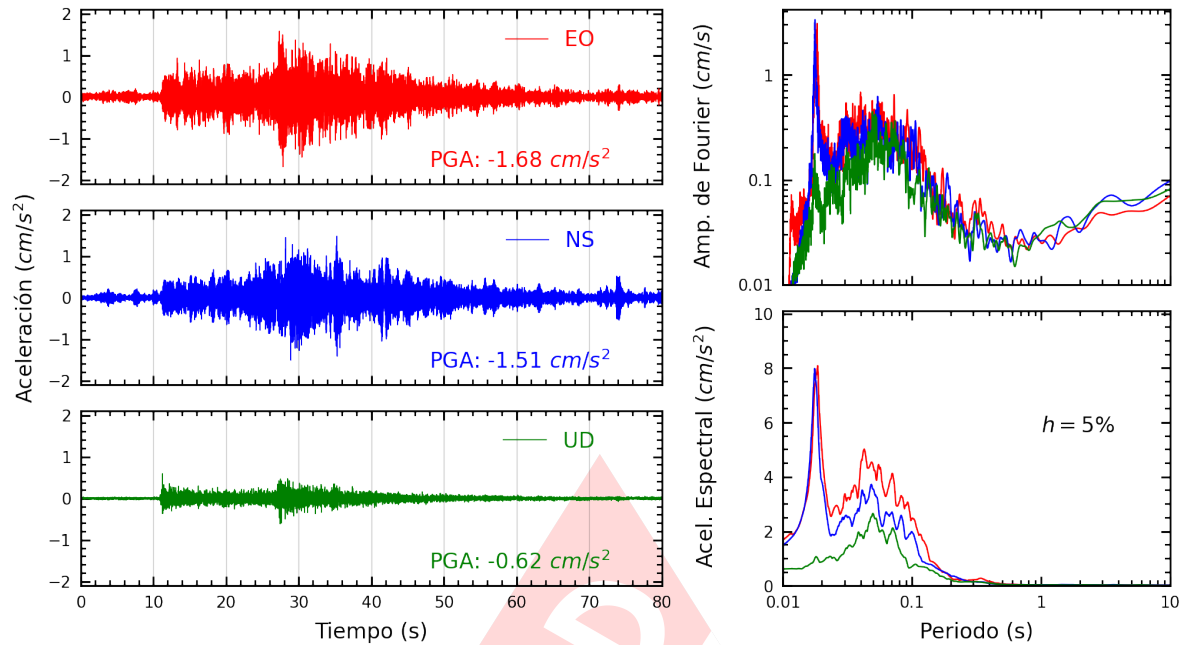
Figura A.11: Registros tiempo-historia, espectros de Fourier y de respuesta en las direcciones EO, NS y vertical de la estación UCSS. Sismo de Canta, Canta - Lima del 2022-09-13, 10:38:29 (Hora local)
