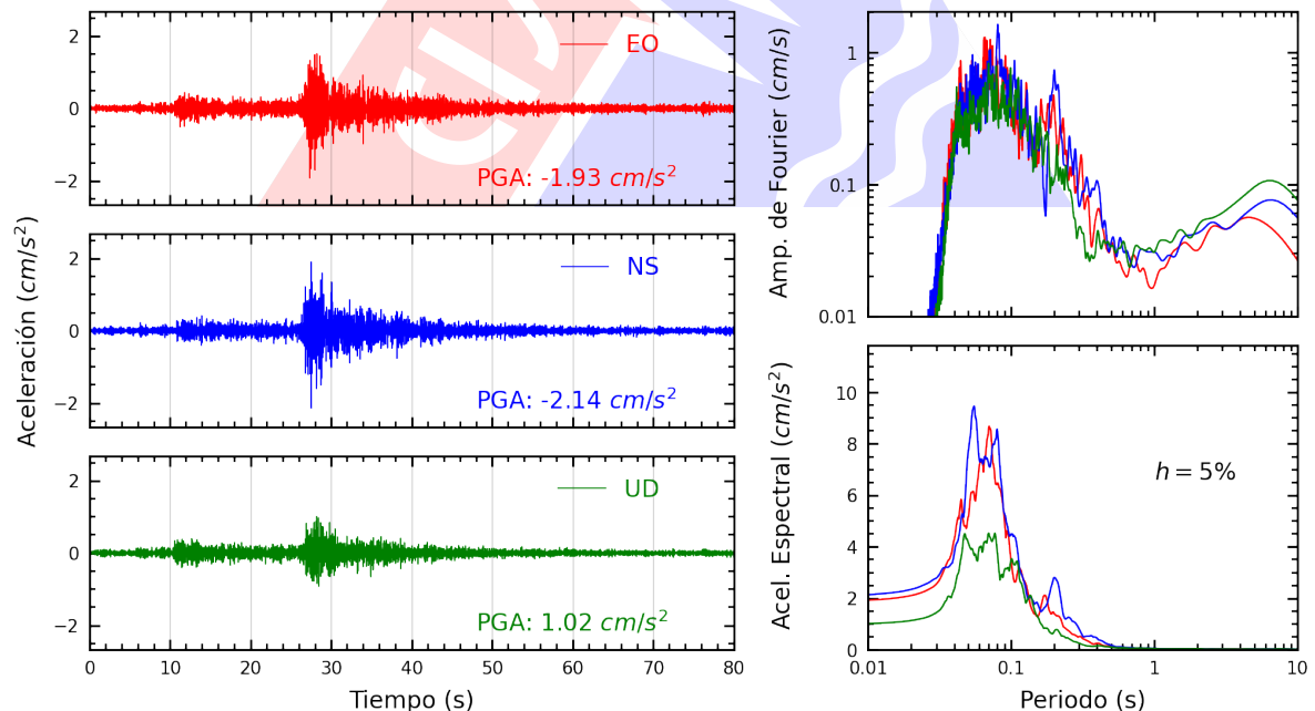
Figura A.10: Registros tiempo-historia, espectros de Fourier y de respuesta en las direcciones EO, NS y vertical de la estación INDEP. Sismo de Canta, Canta - Lima del 2022-09-13, 10:38:29 (Hora local)
