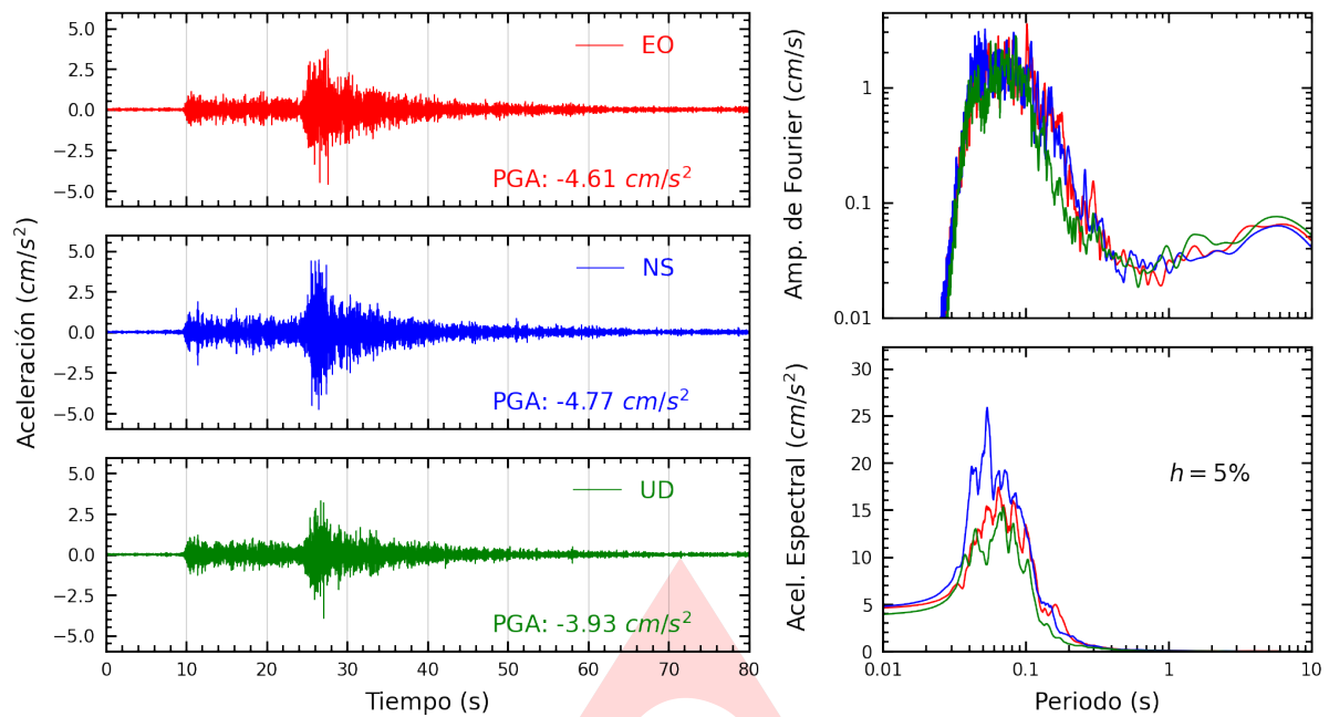
Figura A.1: Registros tiempo-historia, espectros de Fourier y de respuesta en las direcciones EO, NS y vertical de la estación SROSA. Sismo de Canta, Canta - Lima del 2022-09-13, 10:38:29 (Hora local)
