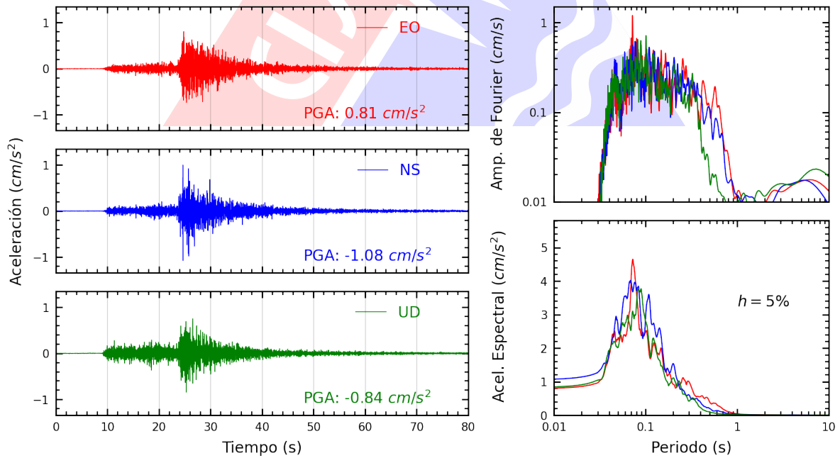
Figura A.22: Registros tiempo-historia, espectros de Fourier y de respuesta en las direcciones EO, NS y vertical de la estación CARAL. Sismo de Canta, Canta - Lima del 2022-09-13, 10:38:29 (Hora local)
