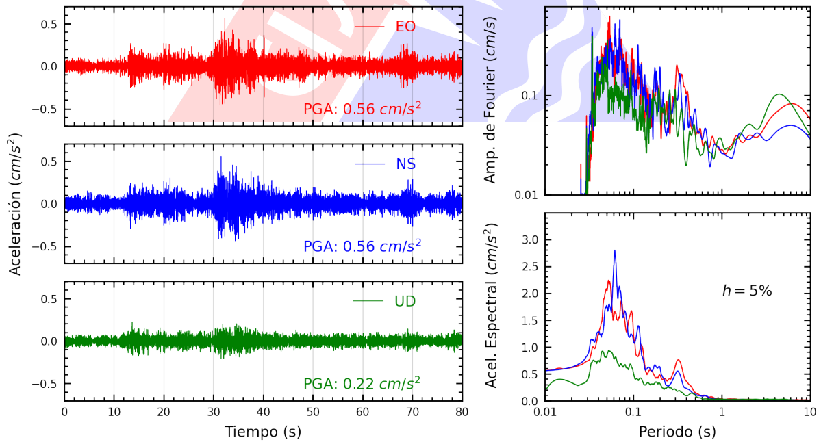
Figura A.36: Registros tiempo-historia, espectros de Fourier y de respuesta en las direcciones EO, NS y vertical de la estación UPCVI. Sismo de Canta, Canta - Lima del 2022-09-13, 10:38:29 (Hora local)
