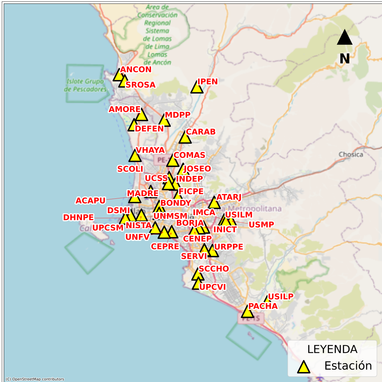
Figura 3: Mapa de ubicación de la(s) estación(es) acelerográfica(s) en Lima Metropolitana correspondiente(s) al Sismo de Canta, Canta - Lima del 13 de setiembre de 2022 a las 10:38:29 (hora local)
