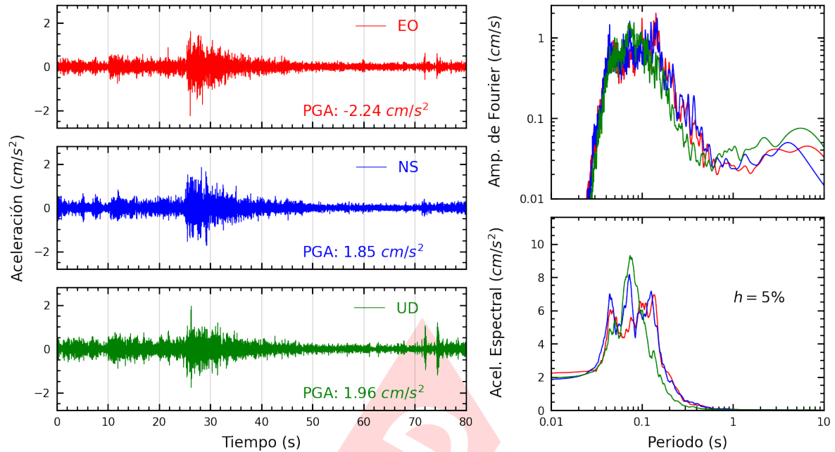
Figura A.9: Registros tiempo-historia, espectros de Fourier y de respuesta en las direcciones EO, NS y vertical de la estación CARAB. Sismo de Canta, Canta - Lima del 2022-09-13, 10:38:29 (Hora local)
