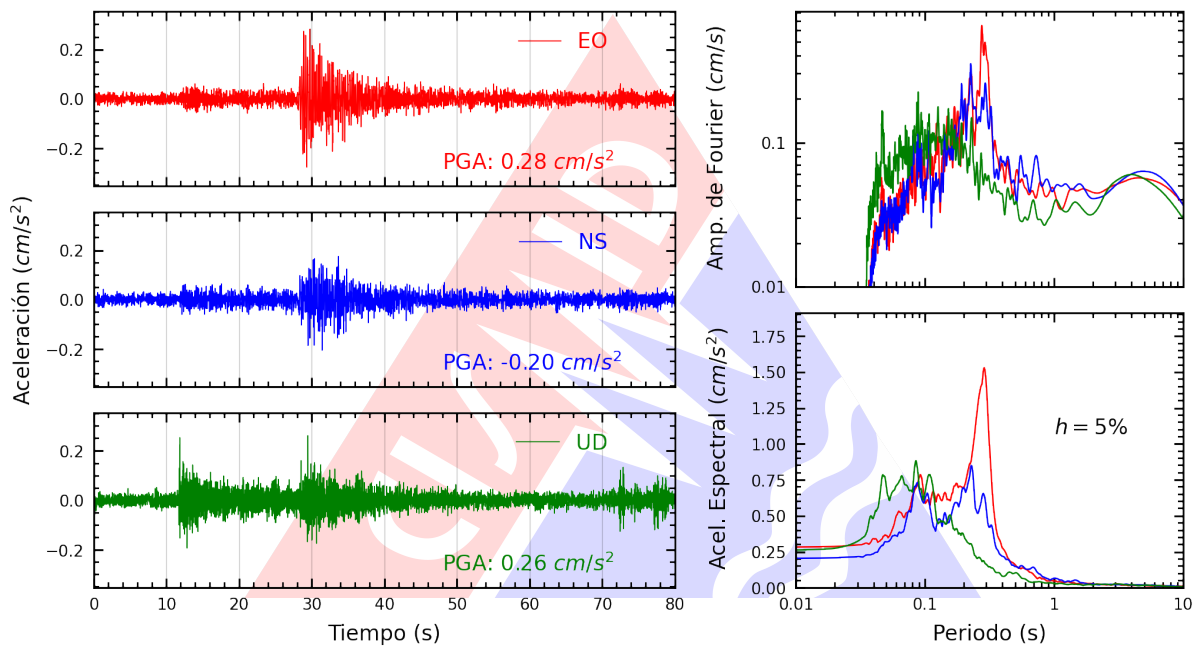
Figura A.39: Registros tiempo-historia, espectros de Fourier y de respuesta en las direcciones EO, NS y vertical de la estación DSMI. Sismo de Canta, Canta - Lima del 2022-09-13, 10:38:29 (Hora local)
