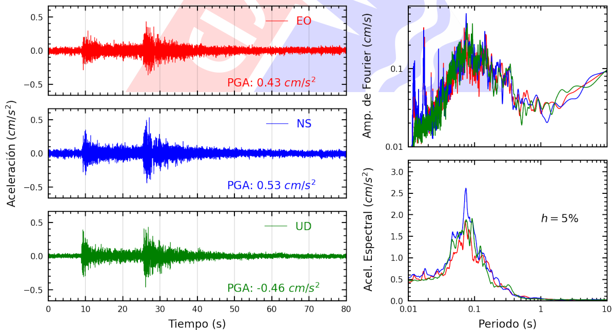
Figura A.38: Registros tiempo-historia, espectros de Fourier y de respuesta en las direcciones EO, NS y vertical de la estación UNMSM. Sismo de Canta, Canta - Lima del 2022-09-13, 10:38:29 (Hora local)
