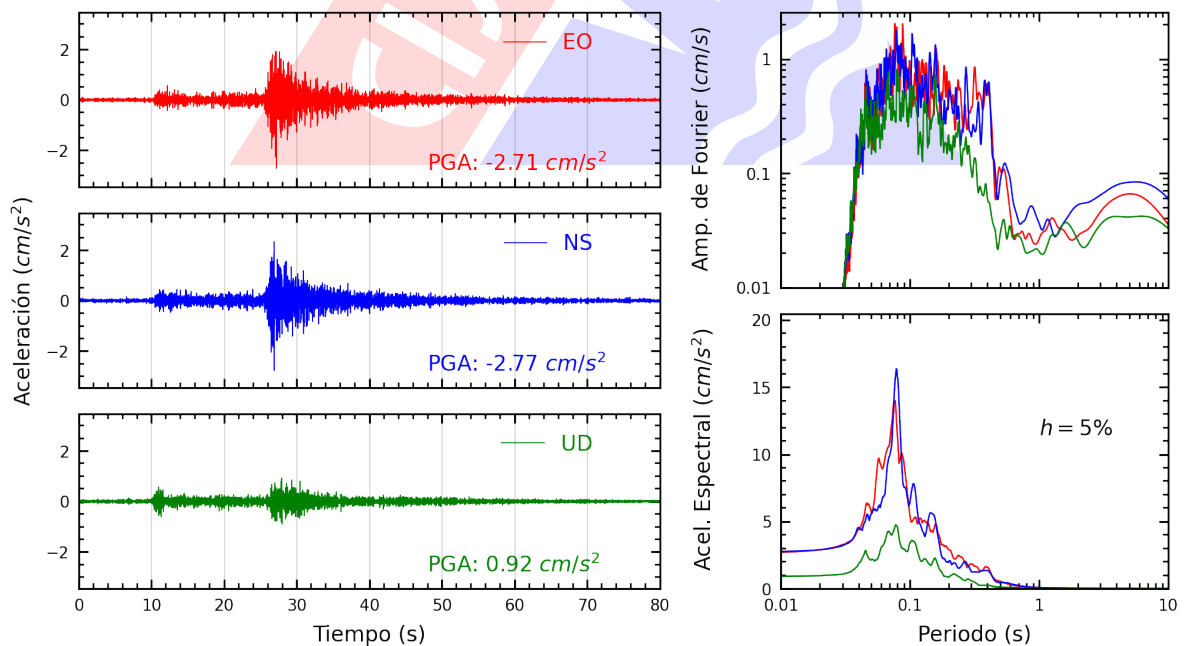
Figura A.6: Registros tiempo-historia, espectros de Fourier y de respuesta en las direcciones EO, NS y vertical de la estación DEFEN. Sismo de Canta, Canta - Lima del 2022-09-13, 10:38:29 (Hora local)
