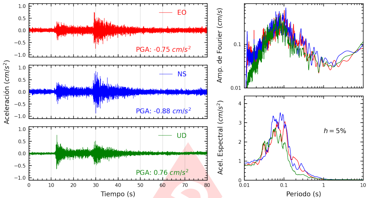
Figura A.27: Registros tiempo-historia, espectros de Fourier y de respuesta en las direcciones EO, NS y vertical de la estación SERVI. Sismo de Canta, Canta - Lima del 2022-09-13, 10:38:29 (Hora local)
