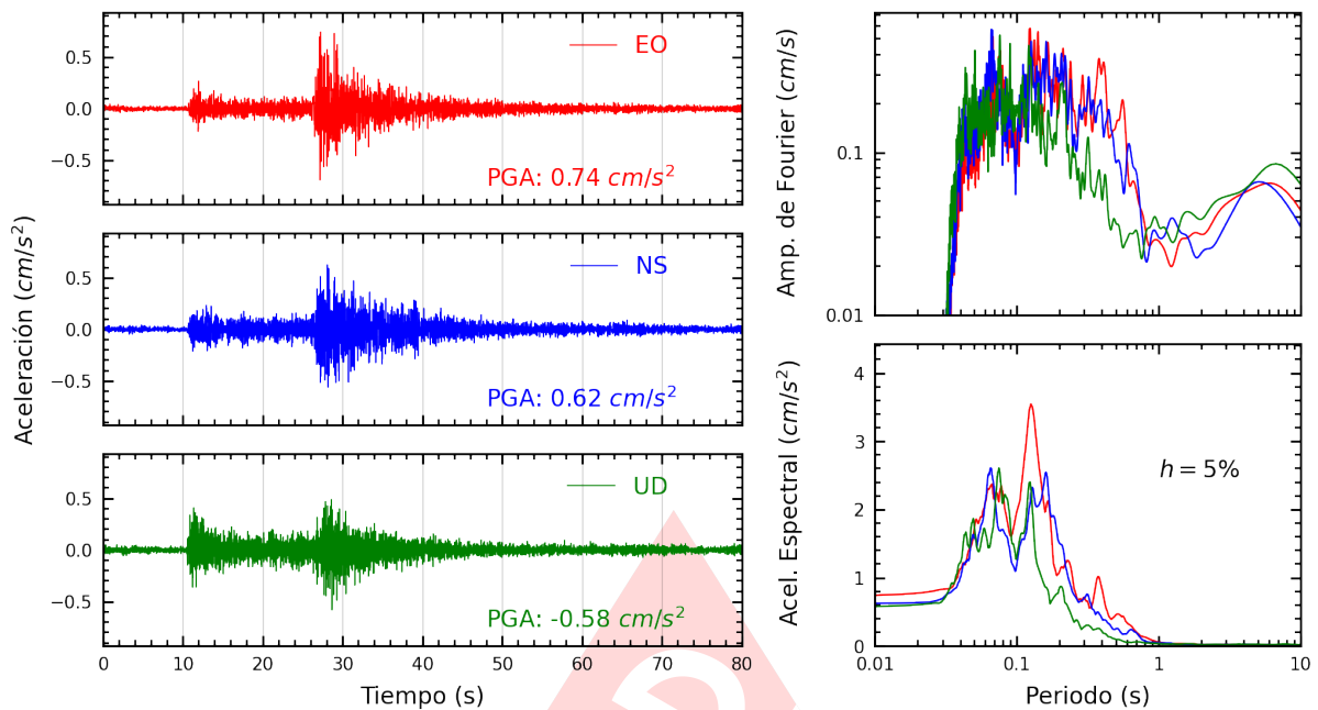
Figura A.29: Registros tiempo-historia, espectros de Fourier y de respuesta en las direcciones EO, NS y vertical de la estación VHAYA. Sismo de Canta, Canta - Lima del 2022-09-13, 10:38:29 (Hora local)
