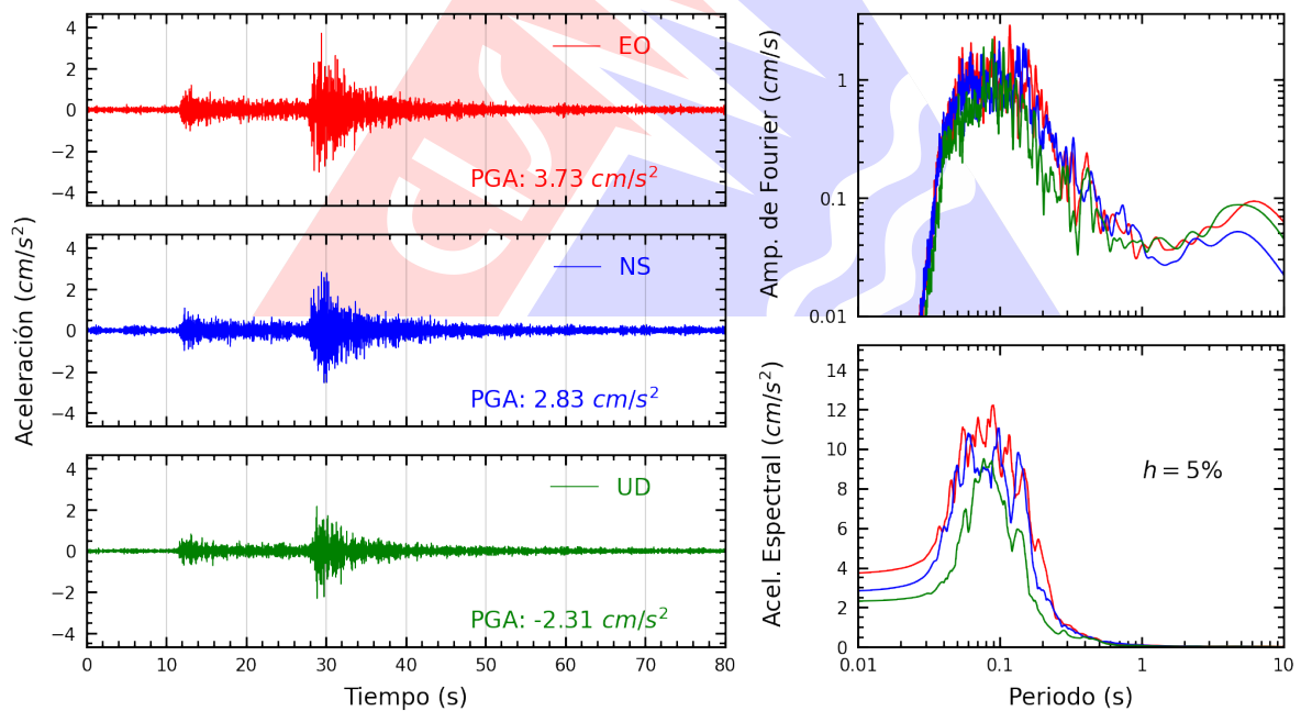
Figura A.2: Registros tiempo-historia, espectros de Fourier y de respuesta en las direcciones EO, NS y vertical de la estación USILM. Sismo de Canta, Canta - Lima del 2022-09-13, 10:38:29 (Hora local)
