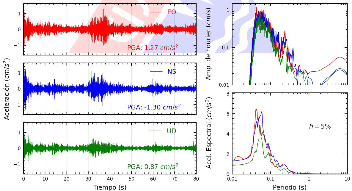
Figura A.14: Registros tiempo-historia, espectros de Fourier y de respuesta en las direcciones EO, NS y vertical de la estación PACHA. Sismo de Canta, Canta - Lima del 2022-09-13, 10:38:29 (Hora local)
