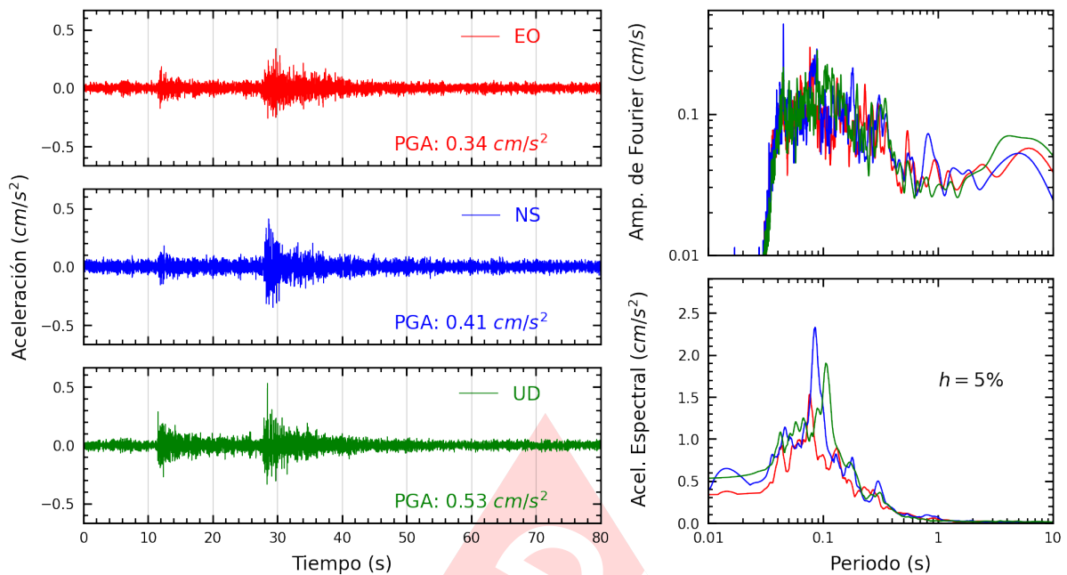
Figura A.37: Registros tiempo-historia, espectros de Fourier y de respuesta en las direcciones EO, NS y vertical de la estación BONDY. Sismo de Canta, Canta - Lima del 2022-09-13, 10:38:29 (Hora local)
