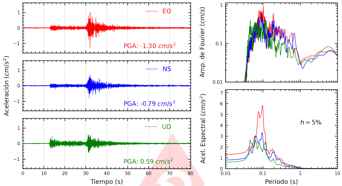
Figura A.15: Registros tiempo-historia, espectros de Fourier y de respuesta en las direcciones EO, NS y vertical de la estación USILP. Sismo de Canta, Canta - Lima del 2022-09-13, 10:38:29 (Hora local)
