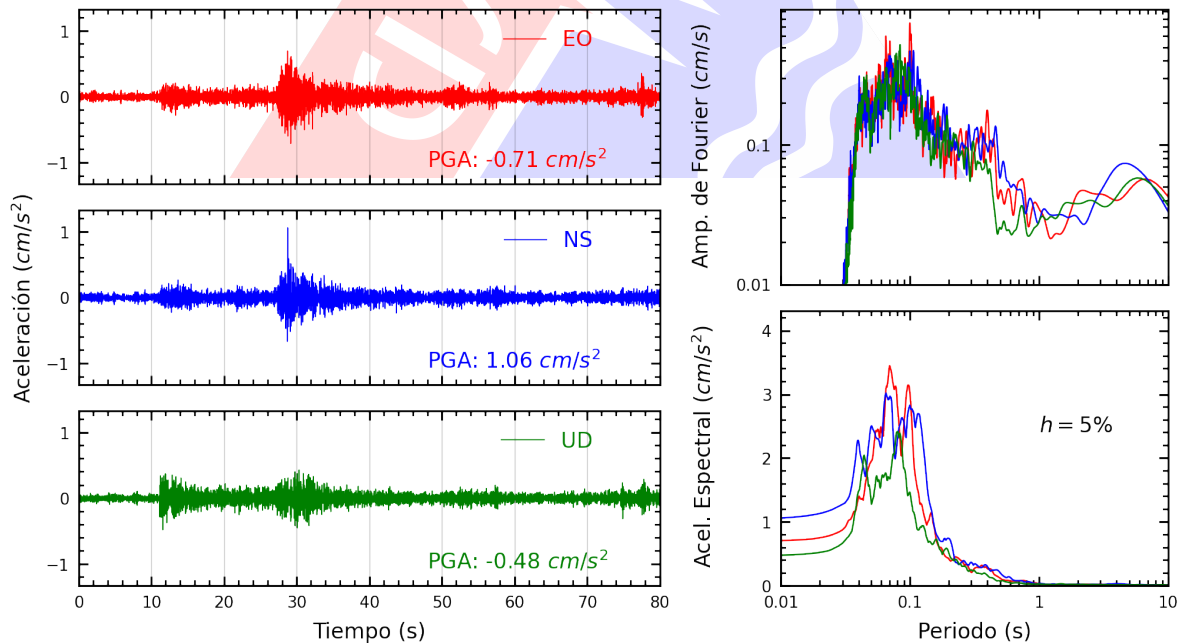
Figura A.24: Registros tiempo-historia, espectros de Fourier y de respuesta en las direcciones EO, NS y vertical de la estación MADRE. Sismo de Canta, Canta - Lima del 2022-09-13, 10:38:29 (Hora local)
