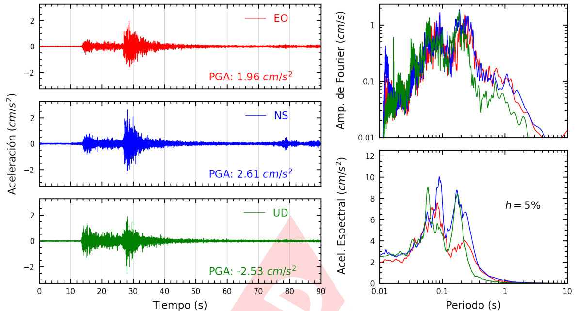
Figura A.3: Registros tiempo-historia, espectros de Fourier y de respuesta en las direcciones EO, NS y vertical de la estación UJBG2. Sismo de Calana, Tacna - Tacna del 2022-09-17, 05:50:45 (Hora local)
