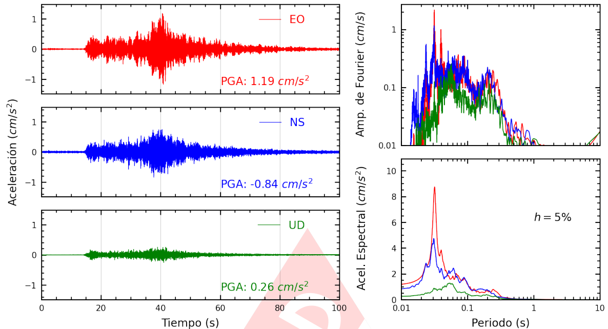
Figura A.5: Registros tiempo-historia, espectros de Fourier y de respuesta en las direcciones EO, NS y vertical de la estación UNAM. Sismo de Calana, Tacna - Tacna del 2022-09-17, 05:50:45 (Hora local)
