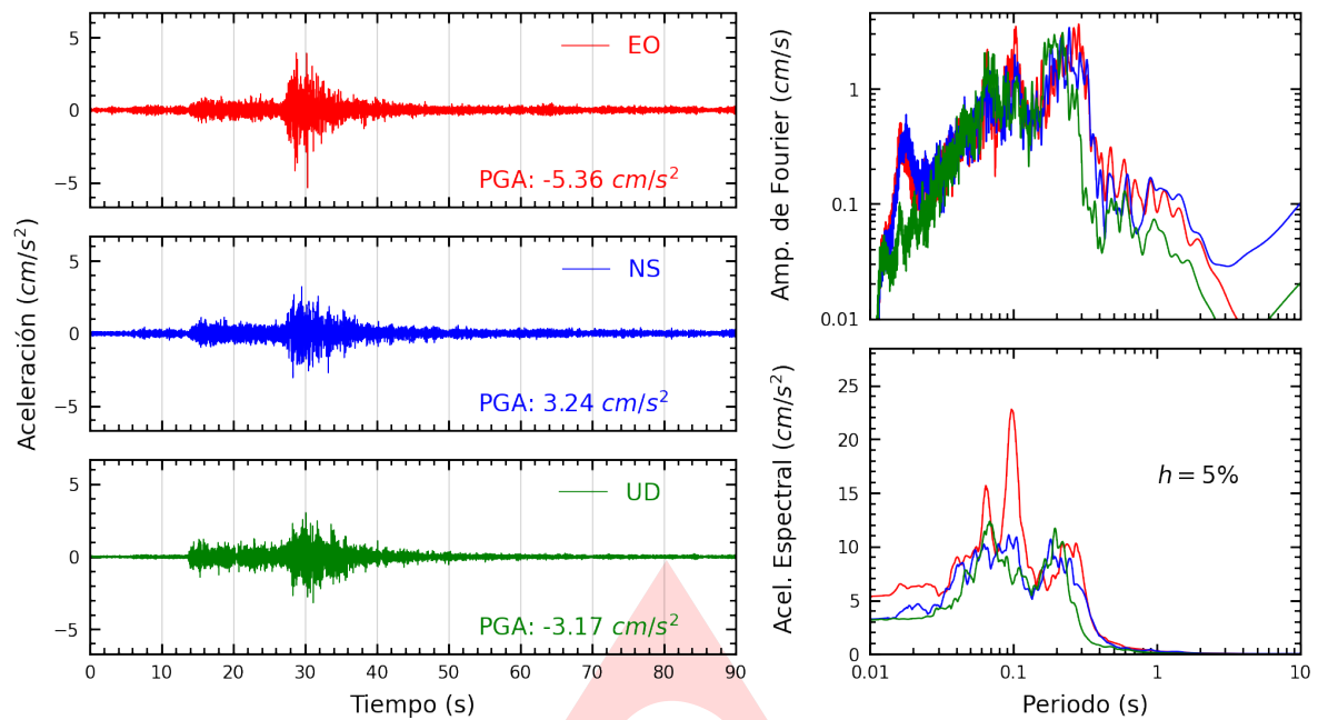
Figura A.1: Registros tiempo-historia, espectros de Fourier y de respuesta en las direcciones EO, NS y vertical de la estación SCTAC. Sismo de Calana, Tacna - Tacna del 2022-09-17, 05:50:45 (Hora local)
