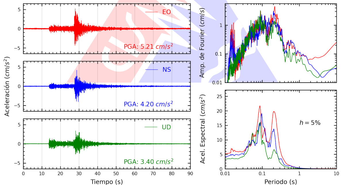
Figura A.2: Registros tiempo-historia, espectros de Fourier y de respuesta en las direcciones EO, NS y vertical de la estación UJBG3. Sismo de Calana, Tacna - Tacna del 2022-09-17, 05:50:45 (Hora local)
