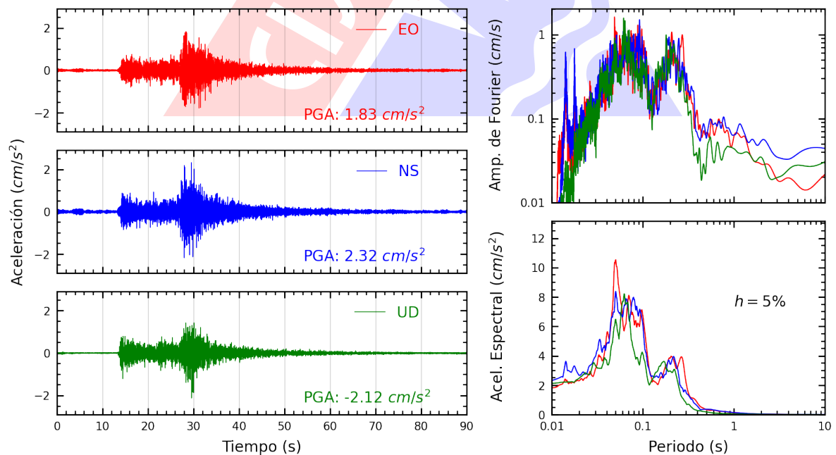
Figura A.4: Registros tiempo-historia, espectros de Fourier y de respuesta en las direcciones EO, NS y vertical de la estación CREY. Sismo de Calana, Tacna - Tacna del 2022-09-17, 05:50:45 (Hora local)
