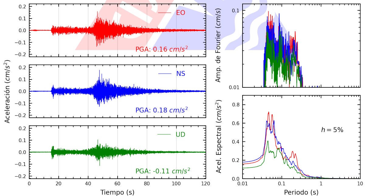
Figura A.6: Registros tiempo-historia, espectros de Fourier y de respuesta en las direcciones EO, NS y vertical de la estación UNSA. Sismo de Calana, Tacna - Tacna del 2022-09-17, 05:50:45 (Hora local)
