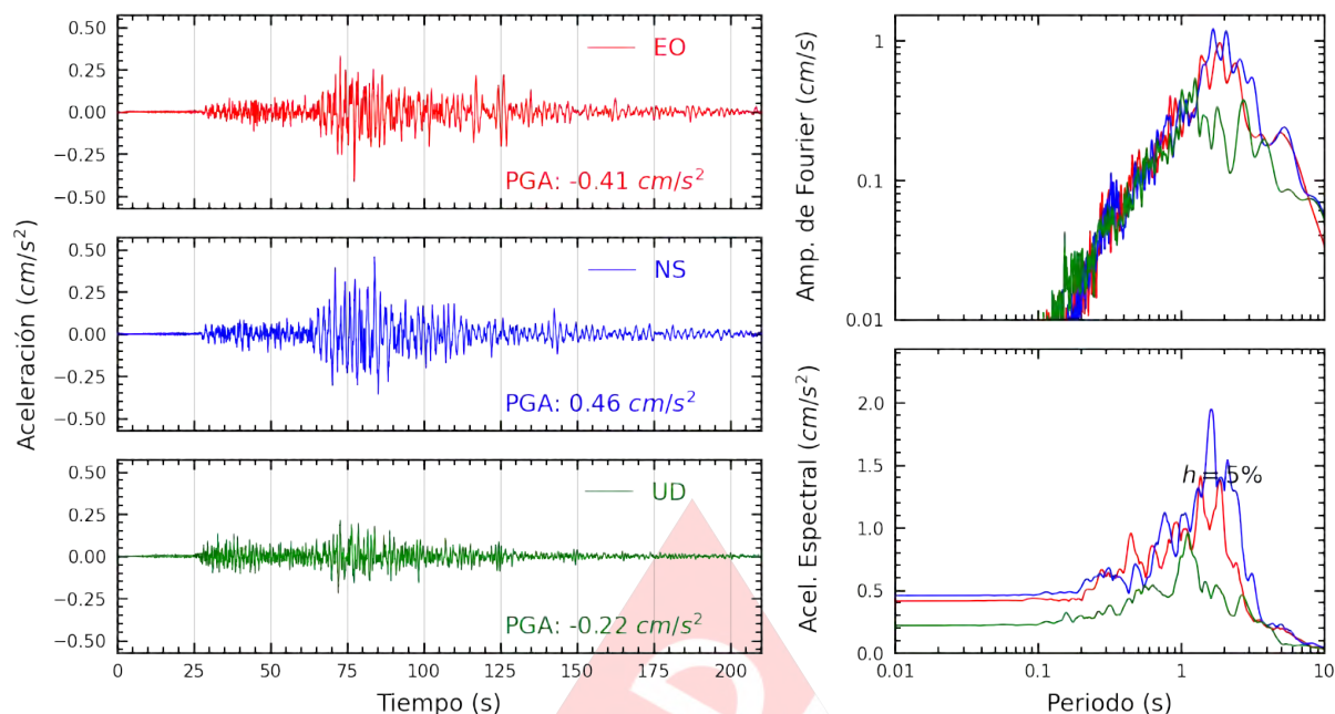
Figura A.31: Registros tiempo-historia, espectros de Fourier y de respuesta en las direcciones EO, NS y vertical de la estación UNCP. Sismo de Ica, Ica - Ica del 2022-10-28, 19:09:46 (Hora local)
