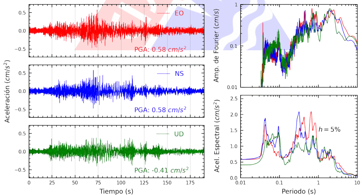
Figura A.28: Registros tiempo-historia, espectros de Fourier y de respuesta en las direcciones EO, NS y vertical de la estación SCAYA. Sismo de Ica, Ica - Ica del 2022-10-28, 19:09:46 (Hora local)
