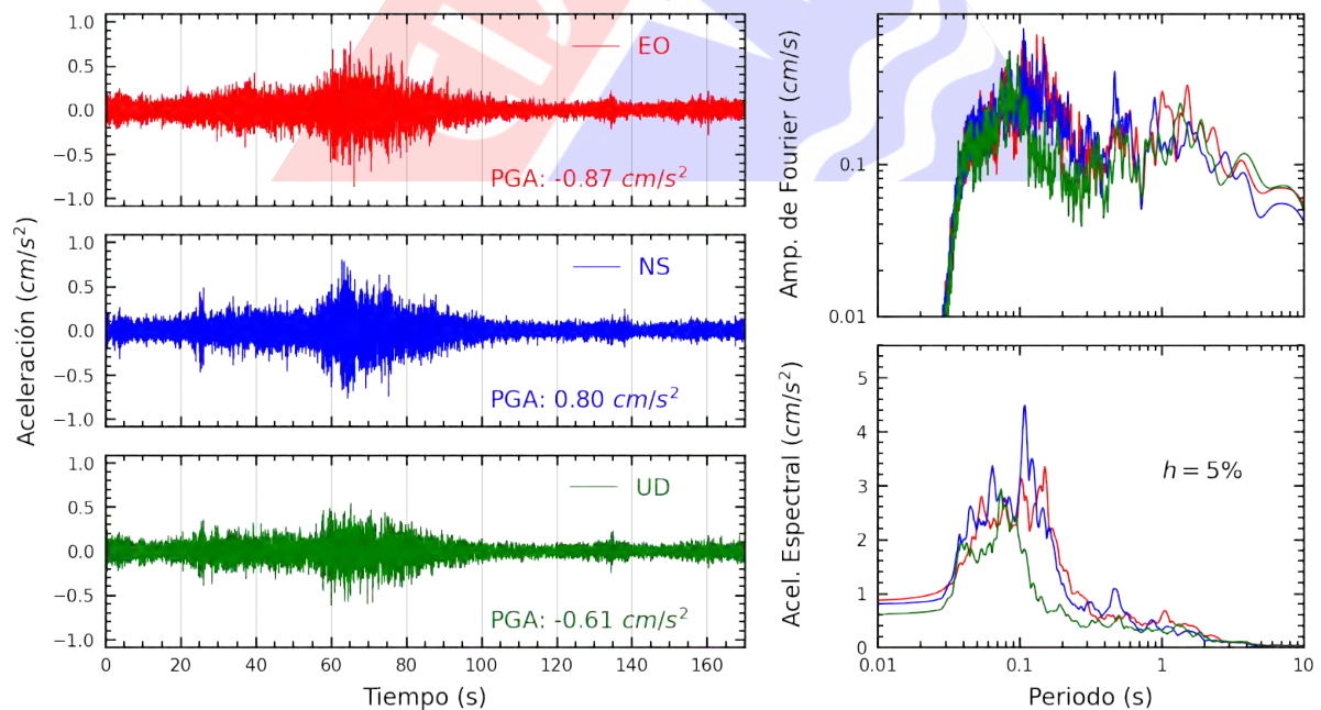
Figura A.20: Registros tiempo-historia, espectros de Fourier y de respuesta en las direcciones EO, NS y vertical de la estación SROSA. Sismo de Ica, Ica - Ica del 2022-10-28, 19:09:46 (Hora local)
