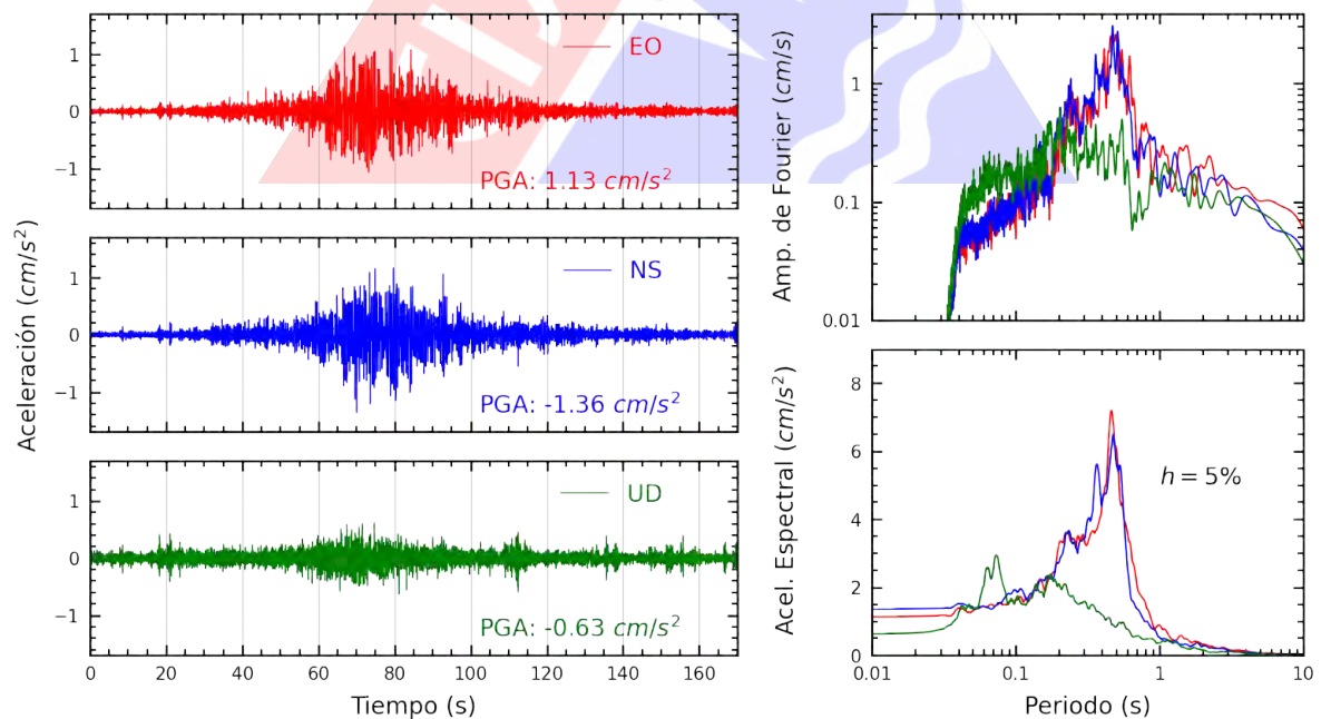
Figura A.10: Registros tiempo-historia, espectros de Fourier y de respuesta en las direcciones EO, NS y vertical de la estación MDPP. Sismo de Ica, Ica - Ica del 2022-10-28, 19:09:46 (Hora local)
