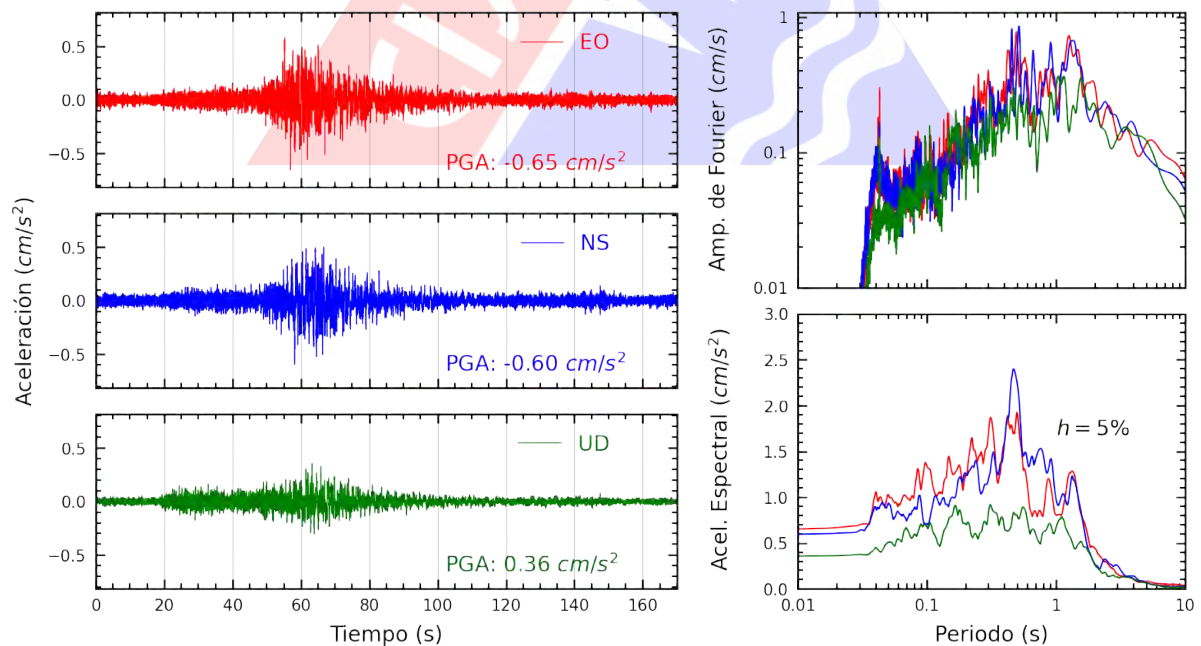
Figura A.26: Registros tiempo-historia, espectros de Fourier y de respuesta en las direcciones EO, NS y vertical de la estación CEPRE. Sismo de Ica, Ica - Ica del 2022-10-28, 19:09:46 (Hora local)
