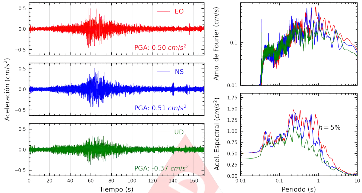
Figura A.29: Registros tiempo-historia, espectros de Fourier y de respuesta en las direcciones EO, NS y vertical de la estación USMP. Sismo de Ica, Ica - Ica del 2022-10-28, 19:09:46 (Hora local)
