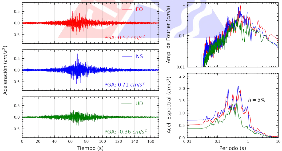
Figura A.24: Registros tiempo-historia, espectros de Fourier y de respuesta en las direcciones EO, NS y vertical de la estación COMAS. Sismo de Ica, Ica - Ica del 2022-10-28, 19:09:46 (Hora local)
