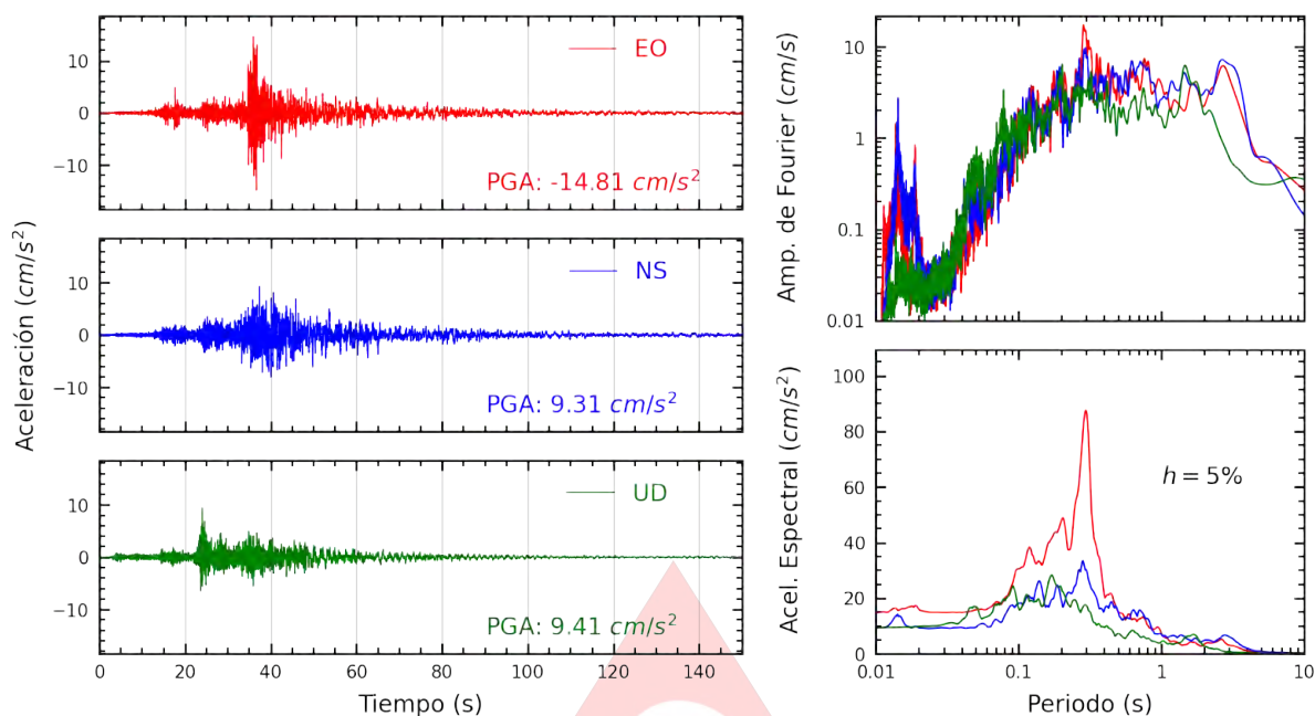
Figura A.1: Registros tiempo-historia, espectros de Fourier y de respuesta en las direcciones EO, NS y vertical de la estación UNICA. Sismo de Ica, Ica - Ica del 2022-10-28, 19:09:46 (Hora local)
