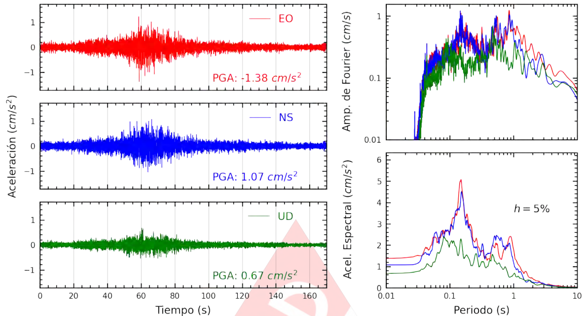
Figura A.9: Registros tiempo-historia, espectros de Fourier y de respuesta en las direcciones EO, NS y vertical de la estación USILM. Sismo de Ica, Ica - Ica del 2022-10-28, 19:09:46 (Hora local)
