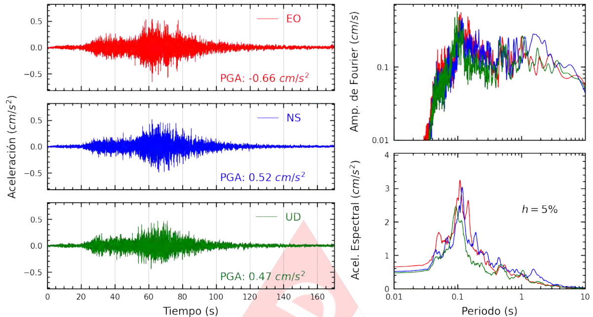
Figura A.25: Registros tiempo-historia, espectros de Fourier y de respuesta en las direcciones EO, NS y vertical de la estación AMORE. Sismo de Ica, Ica - Ica del 2022-10-28, 19:09:46 (Hora local)
