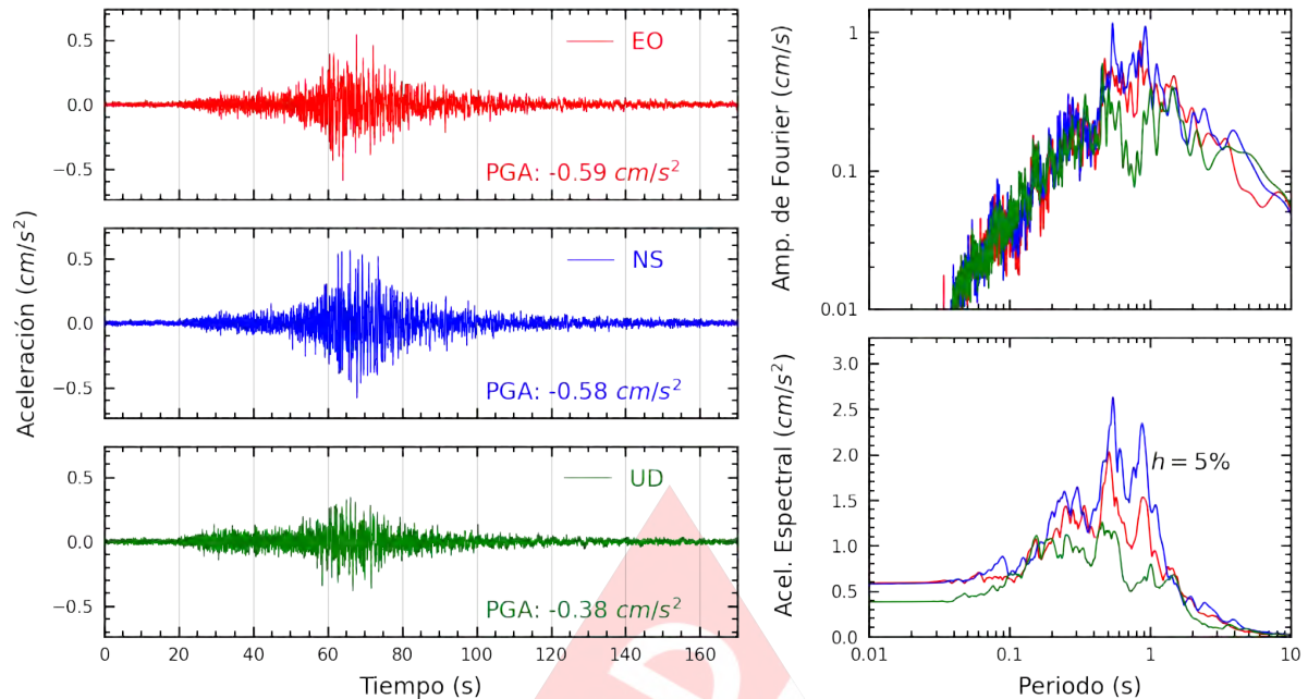
Figura A.27: Registros tiempo-historia, espectros de Fourier y de respuesta en las direcciones EO, NS y vertical de la estación UNMSM. Sismo de Ica, Ica - Ica del 2022-10-28, 19:09:46 (Hora local)
