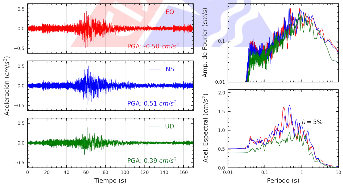
Figura A.30: Registros tiempo-historia, espectros de Fourier y de respuesta en las direcciones EO, NS y vertical de la estación BORJA. Sismo de Ica, Ica - Ica del 2022-10-28, 19:09:46 (Hora local)
