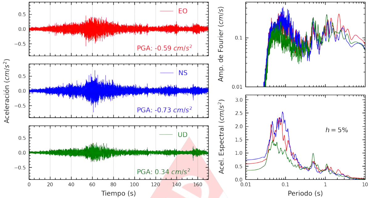
Figura A.23: Registros tiempo-historia, espectros de Fourier y de respuesta en las direcciones EO, NS y vertical de la estación JOSEO. Sismo de Ica, Ica - Ica del 2022-10-28, 19:09:46 (Hora local)
