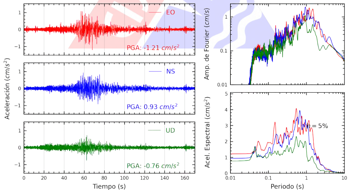
Figura A.12: Registros tiempo-historia, espectros de Fourier y de respuesta en las direcciones EO, NS y vertical de la estación PRADO. Sismo de Ica, Ica - Ica del 2022-10-28, 19:09:46 (Hora local)
