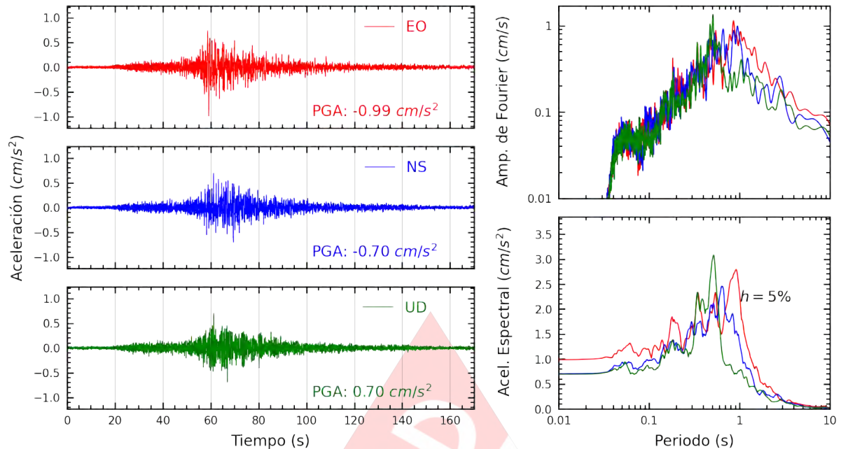
Figura A.15: Registros tiempo-historia, espectros de Fourier y de respuesta en las direcciones EO, NS y vertical de la estación IMCA. Sismo de Ica, Ica - Ica del 2022-10-28, 19:09:46 (Hora local)
