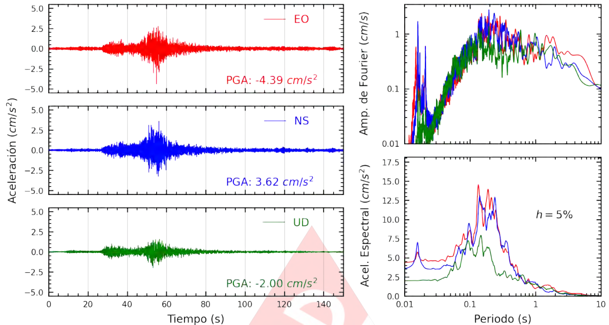
Figura A.3: Registros tiempo-historia, espectros de Fourier y de respuesta en las direcciones EO, NS y vertical de la estación ASIA. Sismo de Ica, Ica - Ica del 2022-10-28, 19:09:46 (Hora local)
