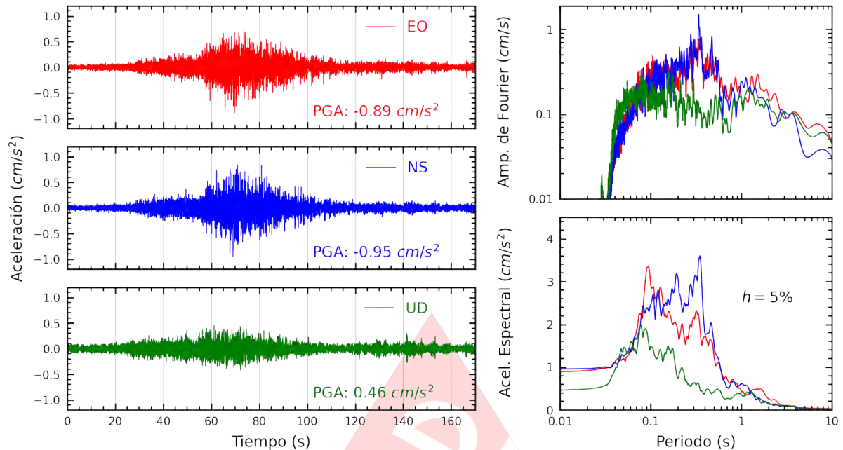
Figura A.17: Registros tiempo-historia, espectros de Fourier y de respuesta en las direcciones EO, NS y vertical de la estación ANCON. Sismo de Ica, Ica - Ica del 2022-10-28, 19:09:46 (Hora local)
