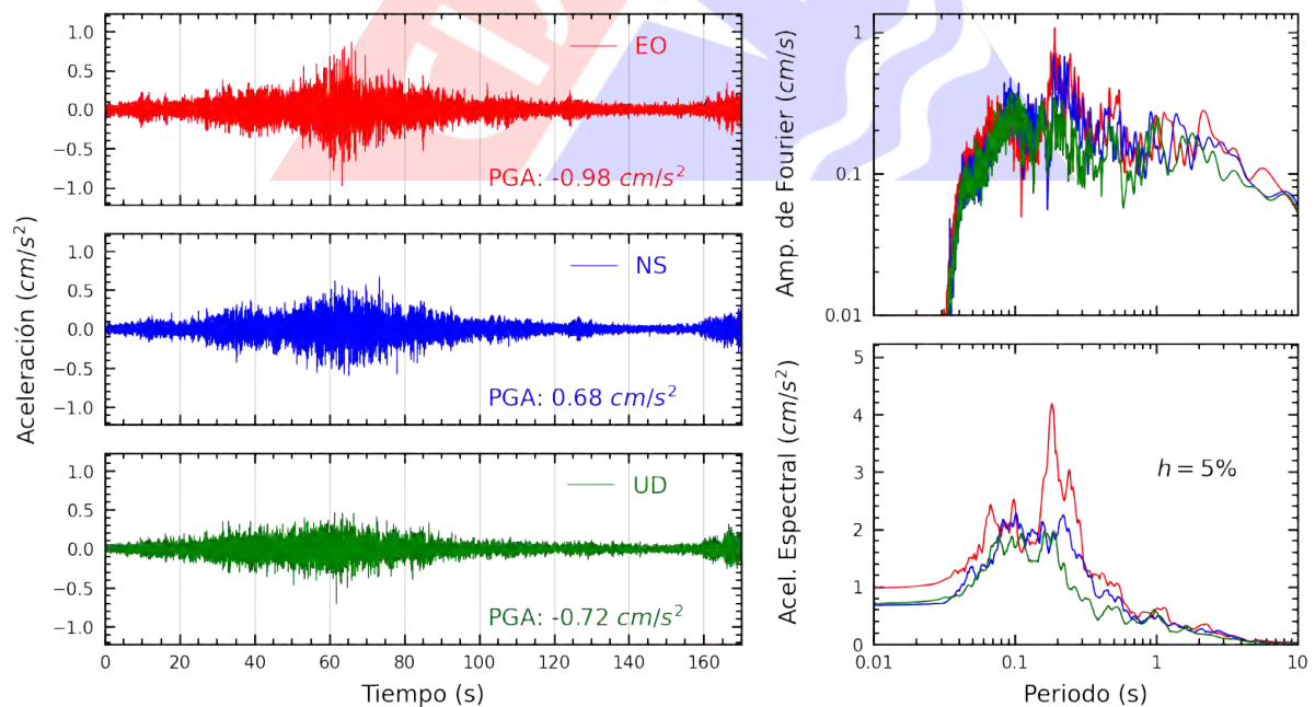
Figura A.16: Registros tiempo-historia, espectros de Fourier y de respuesta en las direcciones EO, NS y vertical de la estación INDEP. Sismo de Ica, Ica - Ica del 2022-10-28, 19:09:46 (Hora local)
