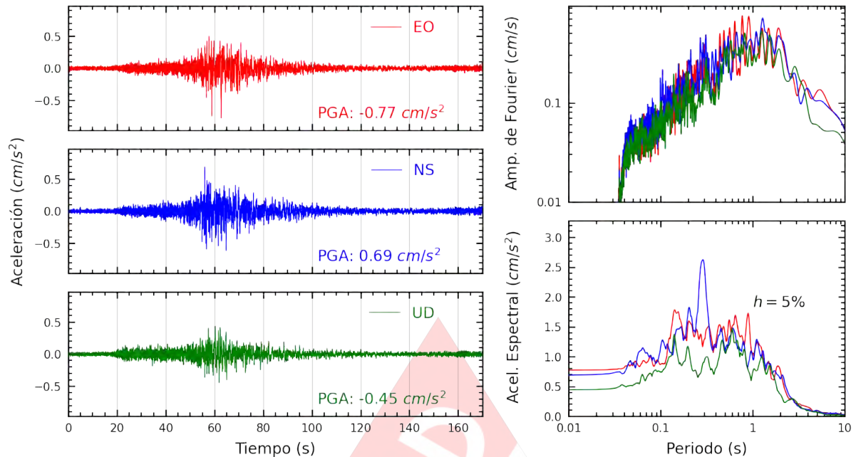
Figura A.21: Registros tiempo-historia, espectros de Fourier y de respuesta en las direcciones EO, NS y vertical de la estación SERVI. Sismo de Ica, Ica - Ica del 2022-10-28, 19:09:46 (Hora local)
