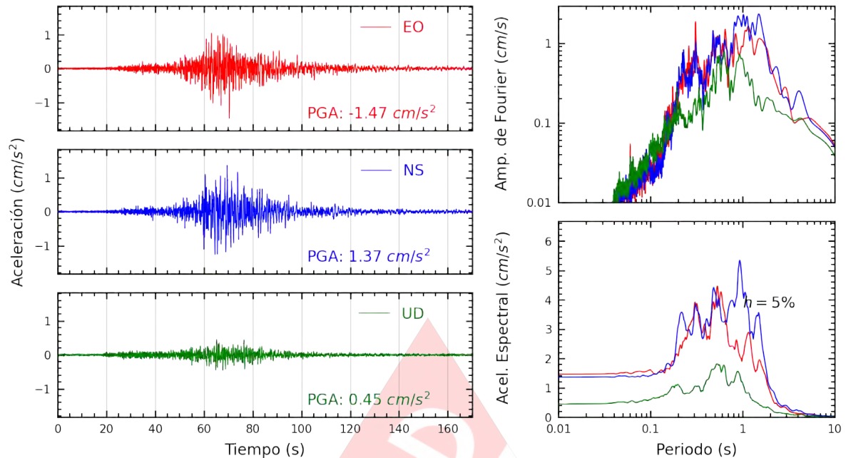
Figura A.7: Registros tiempo-historia, espectros de Fourier y de respuesta en las direcciones EO, NS y vertical de la estación DSML. Sismo de Ica, Ica - Ica del 2022-10-28, 19:09:46 (Hora local)
