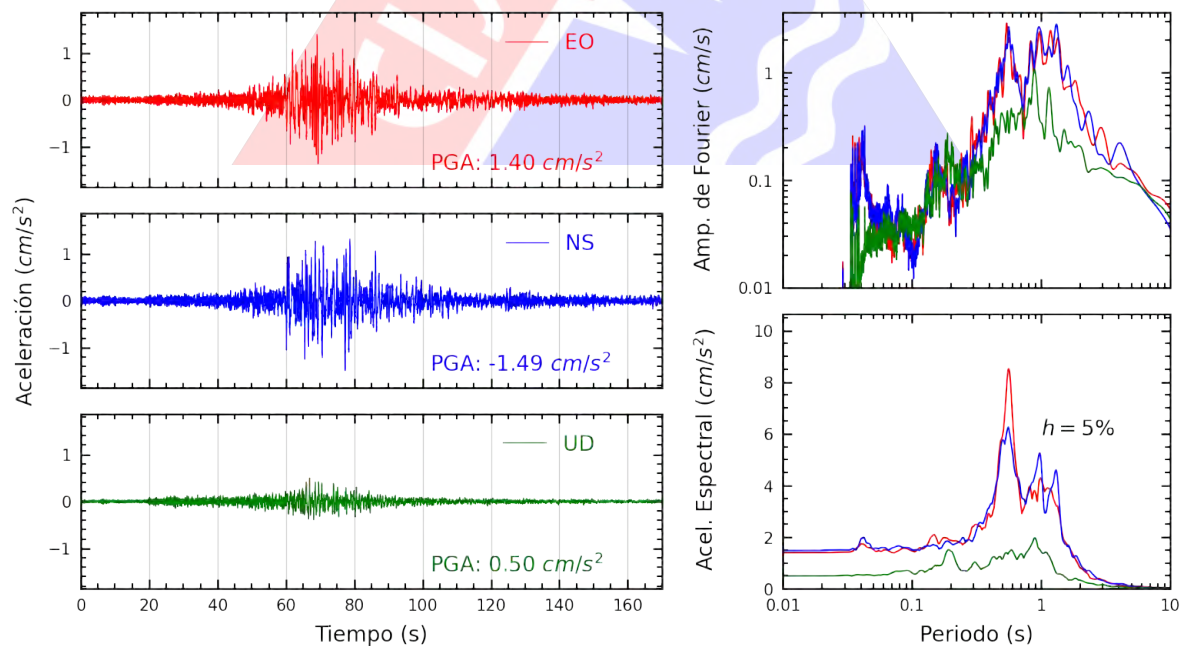
Figura A.6: Registros tiempo-historia, espectros de Fourier y de respuesta en las direcciones EO, NS y vertical de la estación DHNPE. Sismo de Ica, Ica - Ica del 2022-10-28, 19:09:46 (Hora local)
