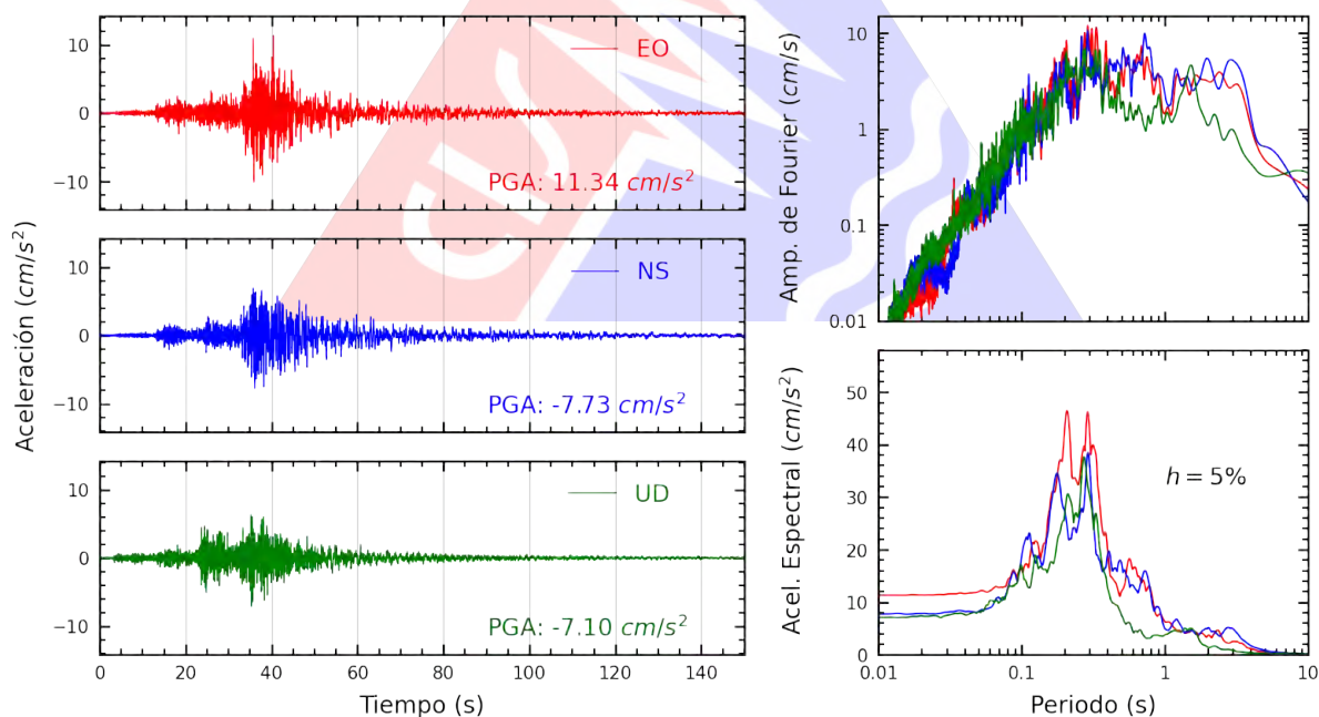
Figura A.2: Registros tiempo-historia, espectros de Fourier y de respuesta en las direcciones EO, NS y vertical de la estación SCICA. Sismo de Ica, Ica - Ica del 2022-10-28, 19:09:46 (Hora local)
