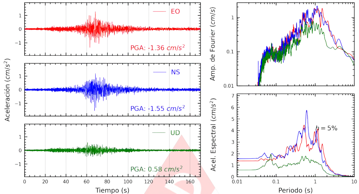
Figura A.5: Registros tiempo-historia, espectros de Fourier y de respuesta en las direcciones EO, NS y vertical de la estación NISTA. Sismo de Ica, Ica - Ica del 2022-10-28, 19:09:46 (Hora local)
