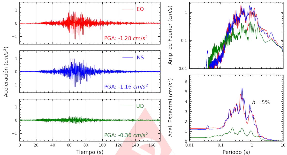
Figura A.11: Registros tiempo-historia, espectros de Fourier y de respuesta en las direcciones EO, NS y vertical de la estación ACAPU. Sismo de Ica, Ica - Ica del 2022-10-28, 19:09:46 (Hora local)
