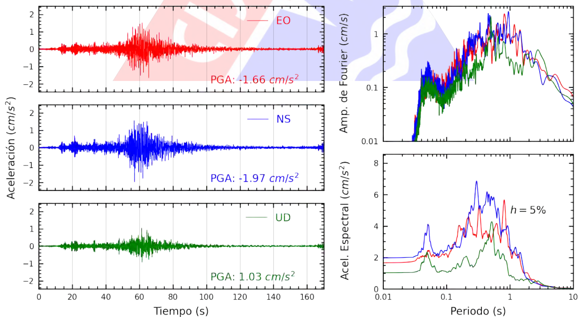
Figura A.4: Registros tiempo-historia, espectros de Fourier y de respuesta en las direcciones EO, NS y vertical de la estación BRISA. Sismo de Ica, Ica - Ica del 2022-10-28, 19:09:46 (Hora local)
