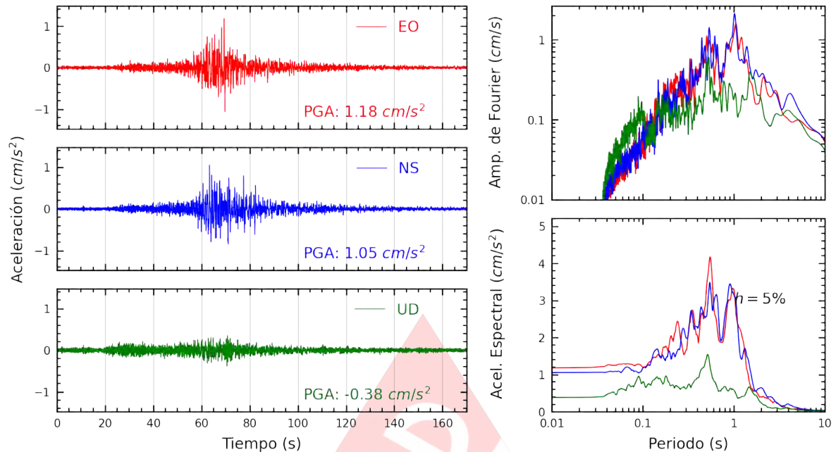
Figura A.13: Registros tiempo-historia, espectros de Fourier y de respuesta en las direcciones EO, NS y vertical de la estación RAMON. Sismo de Ica, Ica - Ica del 2022-10-28, 19:09:46 (Hora local)
