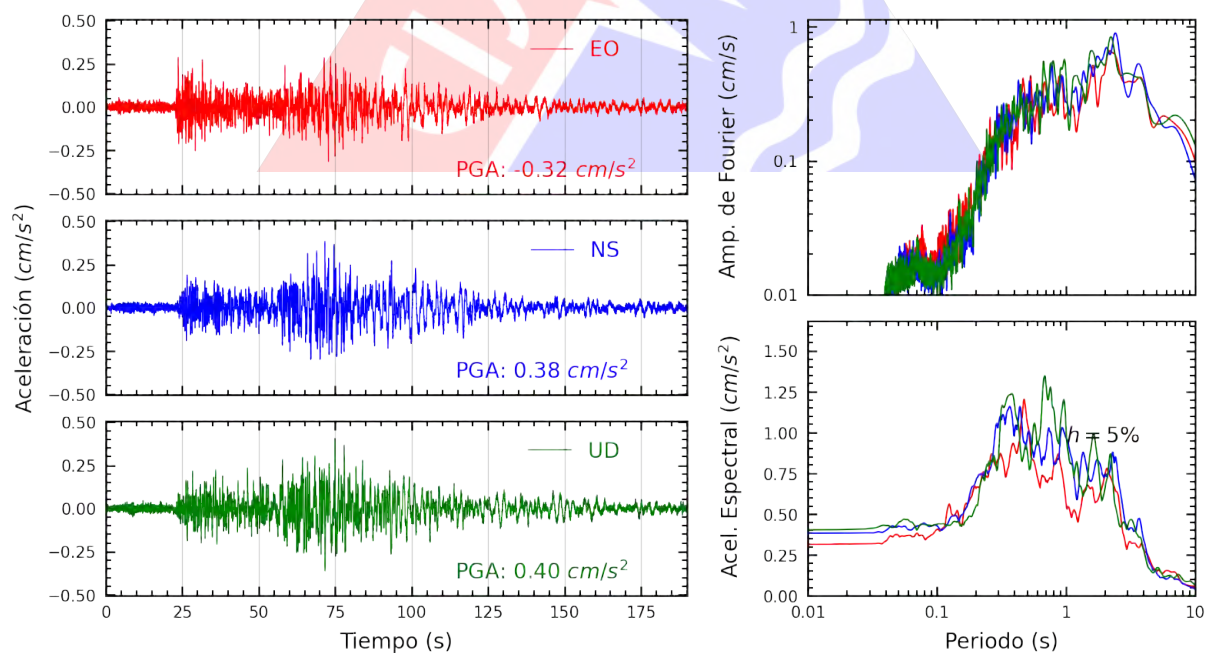
Figura A.32: Registros tiempo-historia, espectros de Fourier y de respuesta en las direcciones EO, NS y vertical de la estación UNSCH. Sismo de Ica, Ica - Ica del 2022-10-28, 19:09:46 (Hora local)
