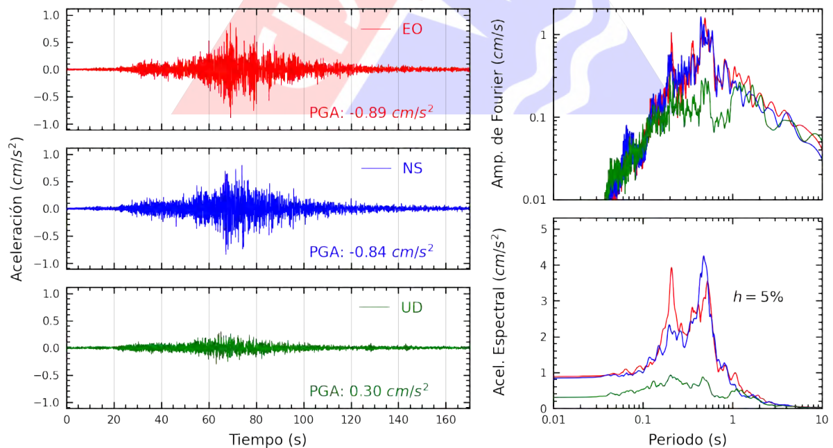
Figura A.18: Registros tiempo-historia, espectros de Fourier y de respuesta en las direcciones EO, NS y vertical de la estación VHAYA. Sismo de Ica, Ica - Ica del 2022-10-28, 19:09:46 (Hora local)
