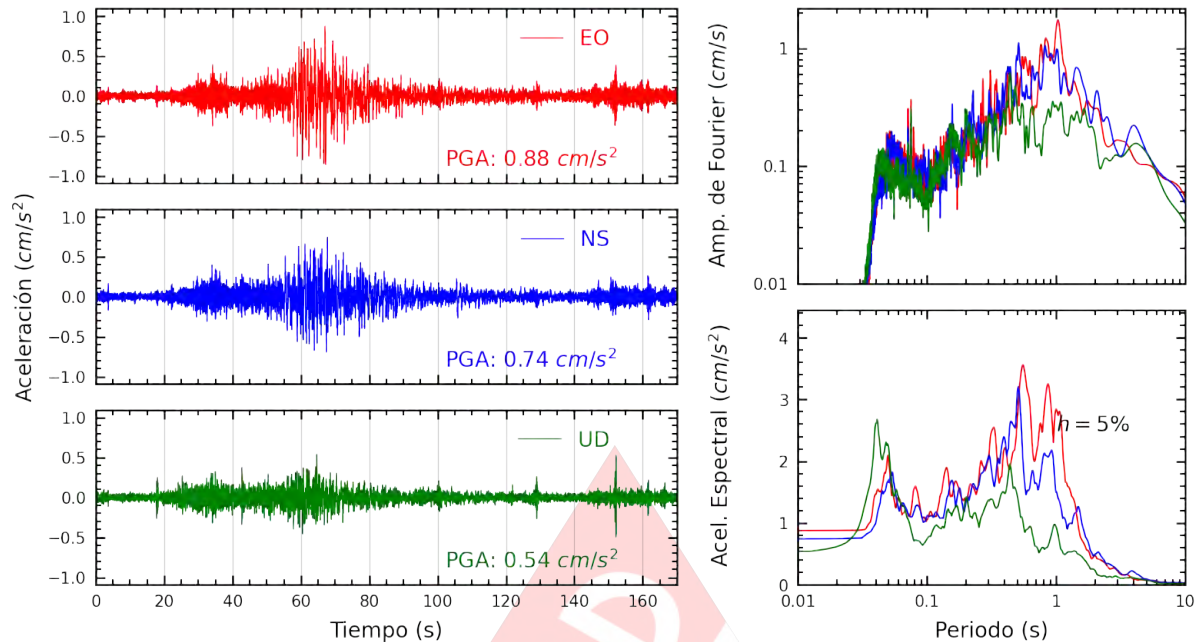
Figura A.19: Registros tiempo-historia, espectros de Fourier y de respuesta en las direcciones EO, NS y vertical de la estación UPCSM. Sismo de Ica, Ica - Ica del 2022-10-28, 19:09:46 (Hora local)
