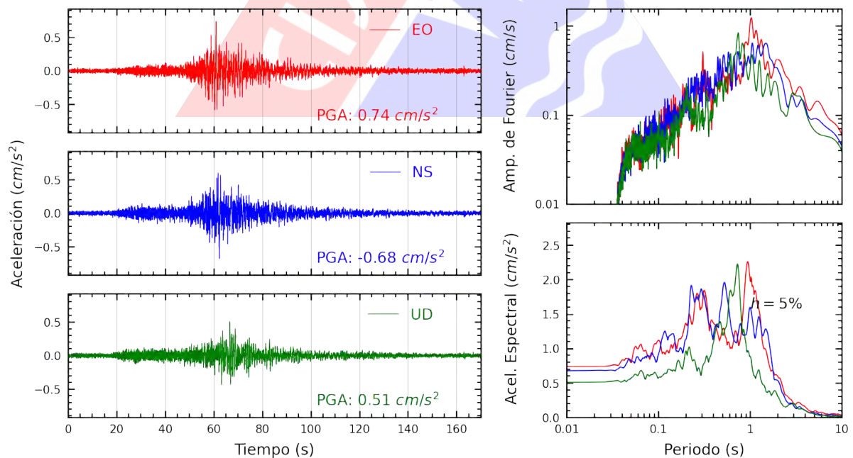
Figura A.22: Registros tiempo-historia, espectros de Fourier y de respuesta en las direcciones EO, NS y vertical de la estación CENEP. Sismo de Ica, Ica - Ica del 2022-10-28, 19:09:46 (Hora local)
