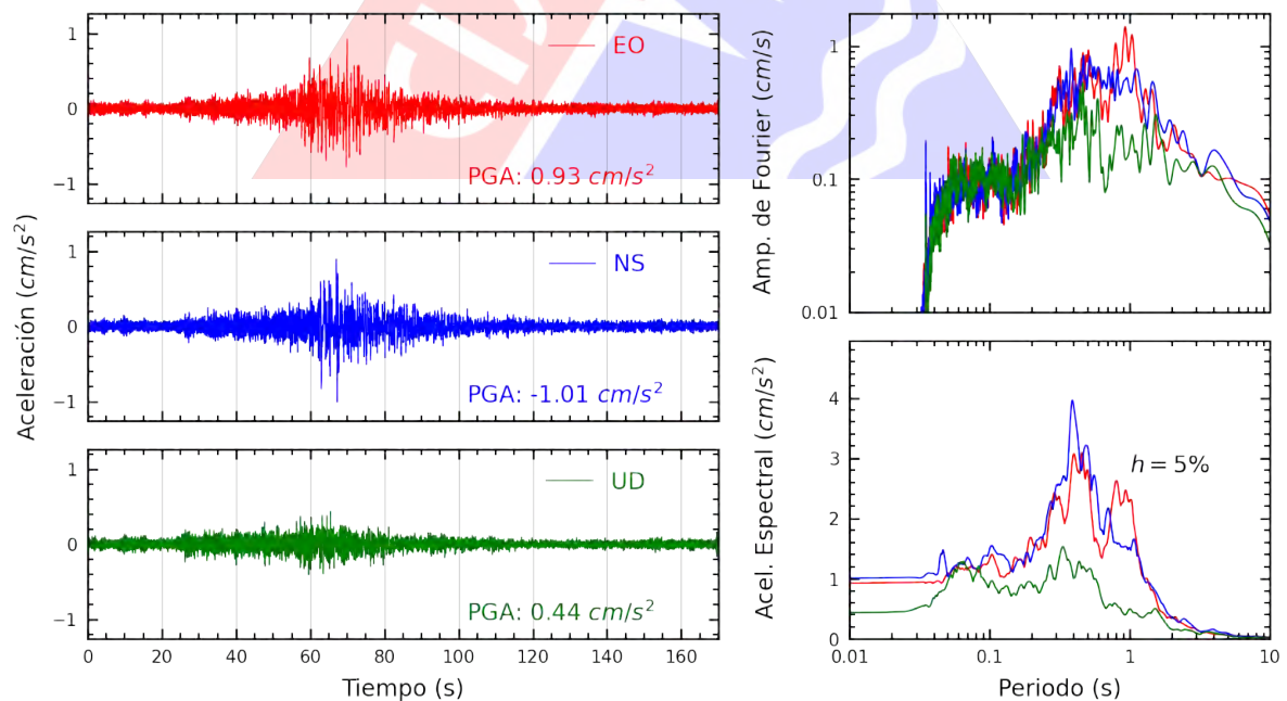
Figura A.14: Registros tiempo-historia, espectros de Fourier y de respuesta en las direcciones EO, NS y vertical de la estación MADRE. Sismo de Ica, Ica - Ica del 2022-10-28, 19:09:46 (Hora local)
