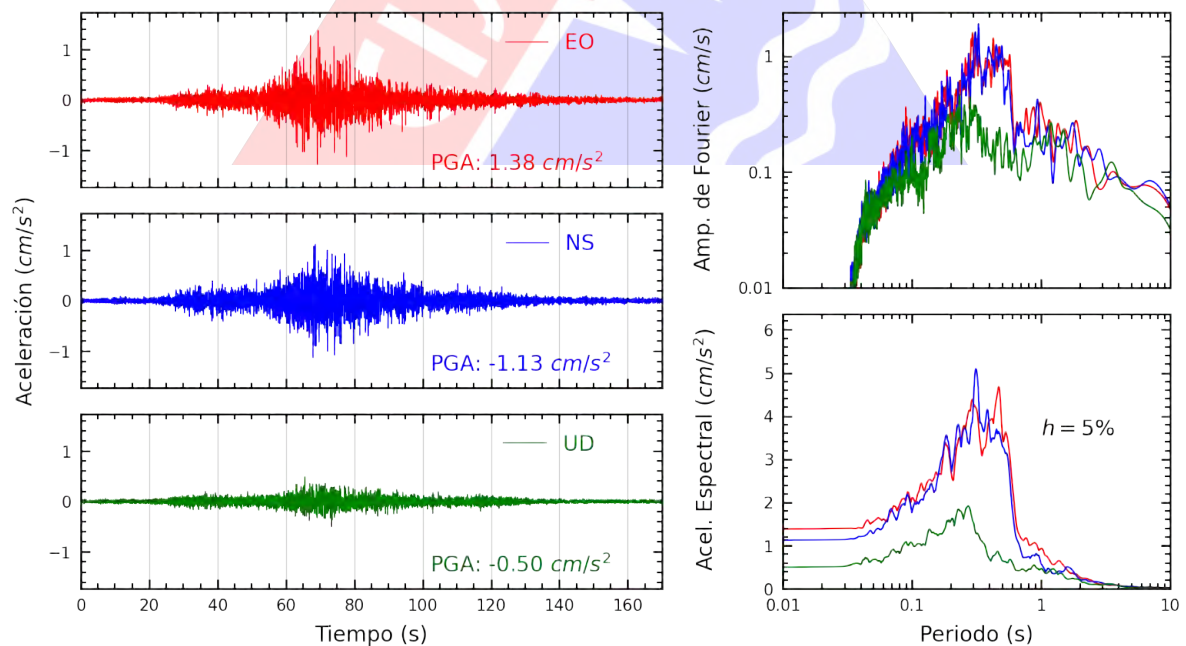
Figura A.8: Registros tiempo-historia, espectros de Fourier y de respuesta en las direcciones EO, NS y vertical de la estación DEFEN. Sismo de Ica, Ica - Ica del 2022-10-28, 19:09:46 (Hora local)
