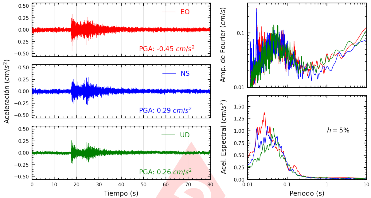
Figura A.21: Registros tiempo-historia, espectros de Fourier y de respuesta en las direcciones EO, NS y vertical de la estación UNMSM. Sismo de Provincia Constitucional del Callao , Callao - Lima del 2022-11-05, 05:26:06 (Hora local)
