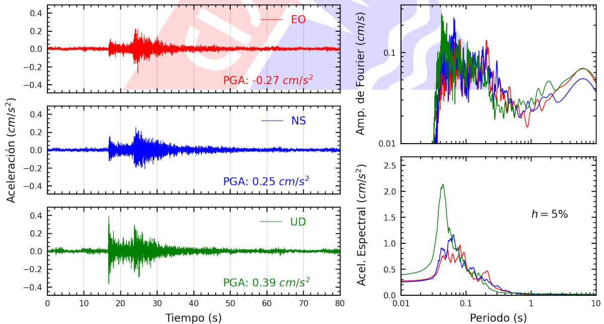
Figura A.26: Registros tiempo-historia, espectros de Fourier y de respuesta en las direcciones EO, NS y vertical de la estación VHAYA. Sismo de Provincia Constitucional del Callao , Callao - Lima del 2022-11-05, 05:26:06 (Hora local)
