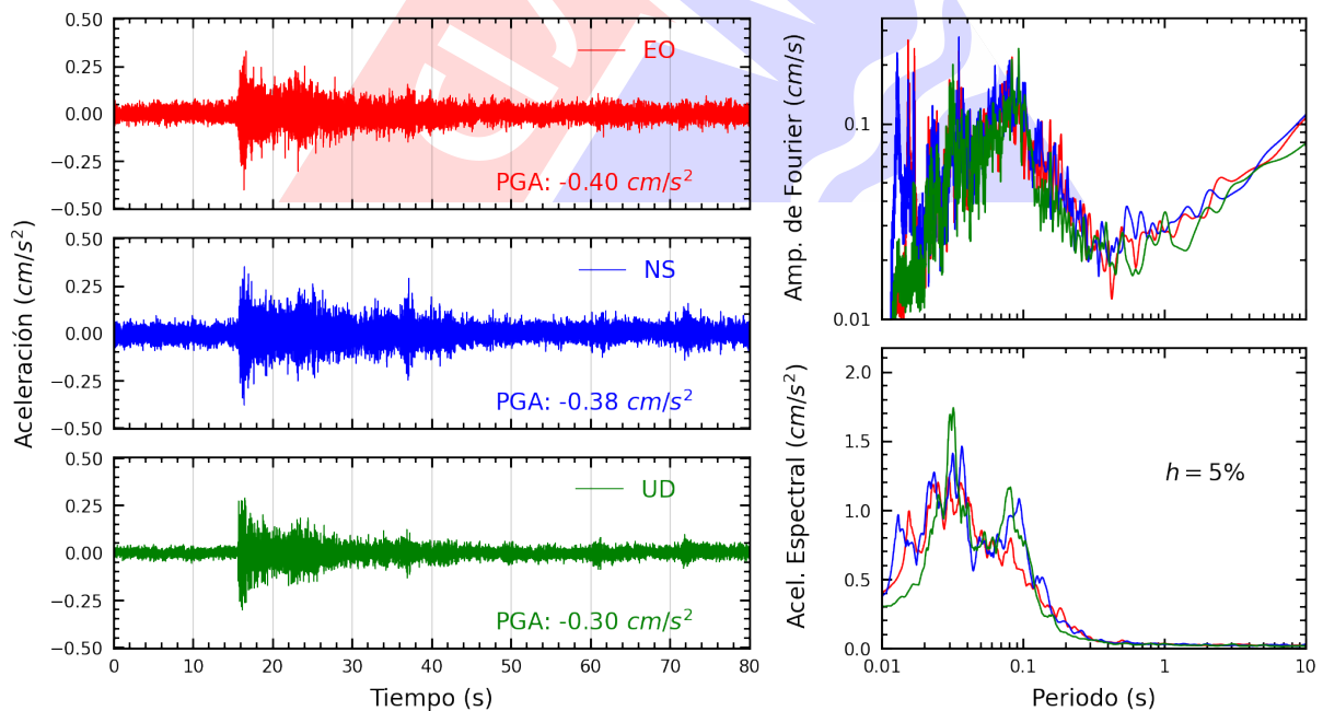
Figura A.24: Registros tiempo-historia, espectros de Fourier y de respuesta en las direcciones EO, NS y vertical de la estación NISTA. Sismo de Provincia Constitucional del Callao , Callao - Lima del 2022-11-05, 05:26:06 (Hora local)
