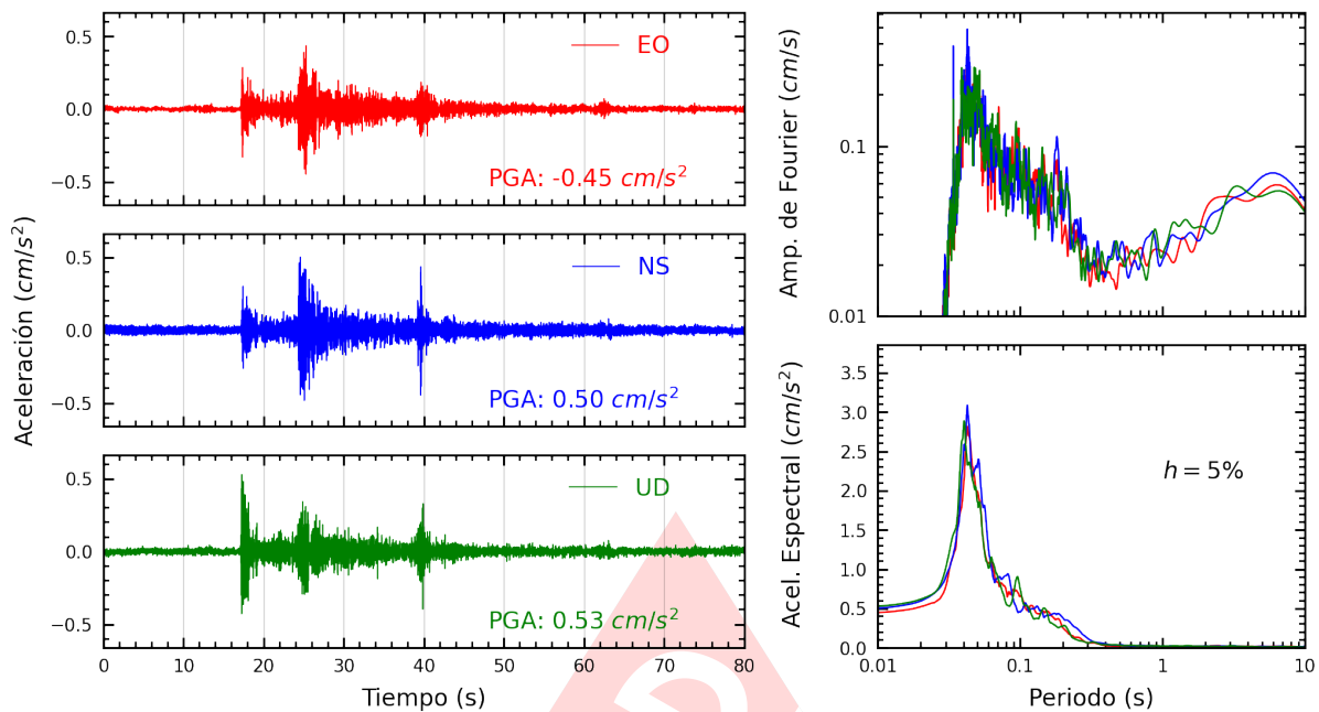
Figura A.19: Registros tiempo-historia, espectros de Fourier y de respuesta en las direcciones EO, NS y vertical de la estación USMP. Sismo de Provincia Constitucional del Callao , Callao - Lima del 2022-11-05, 05:26:06 (Hora local)
