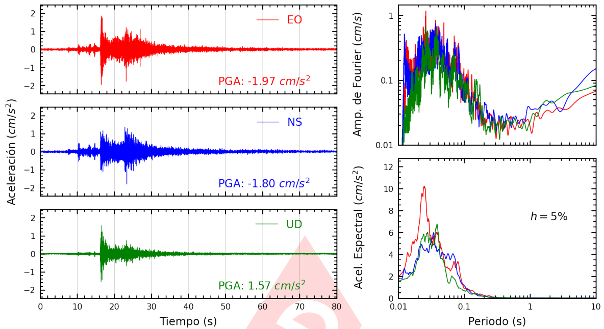
Figura A.7: Registros tiempo-historia, espectros de Fourier y de respuesta en las direcciones EO, NS y vertical de la estación CEPRE. Sismo de Provincia Constitucional del Callao , Callao - Lima del 2022-11-05, 05:26:06 (Hora local)
