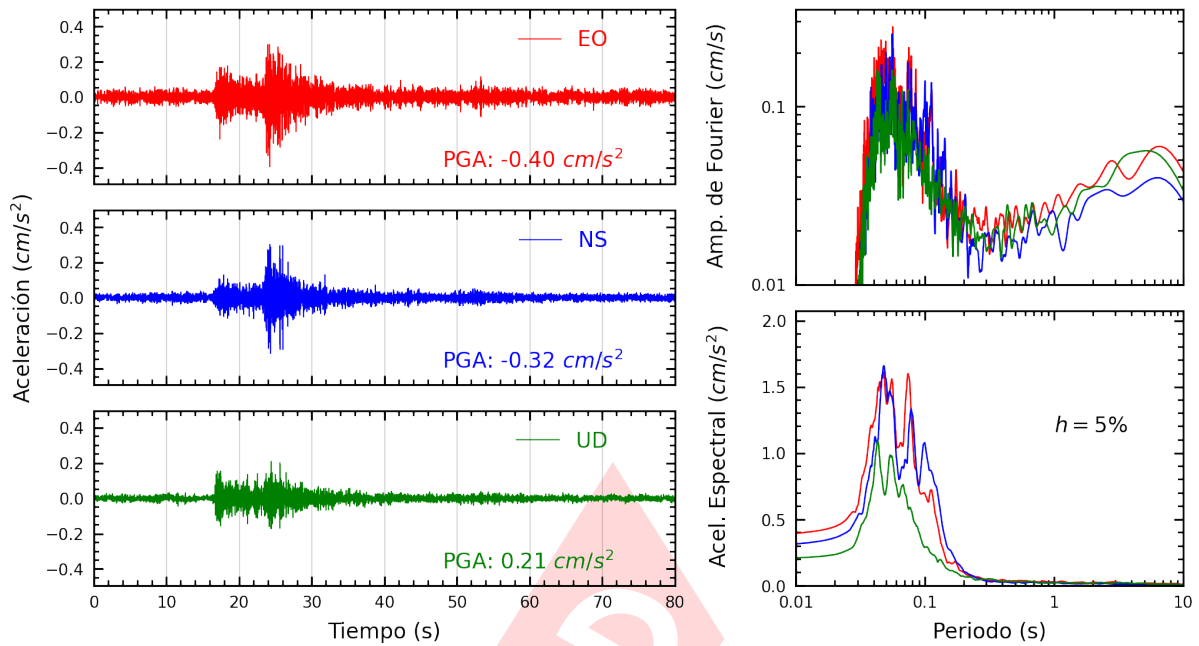
Figura A.25: Registros tiempo-historia, espectros de Fourier y de respuesta en las direcciones EO, NS y vertical de la estación INICT. Sismo de Provincia Constitucional del Callao , Callao - Lima del 2022-11-05, 05:26:06 (Hora local)
