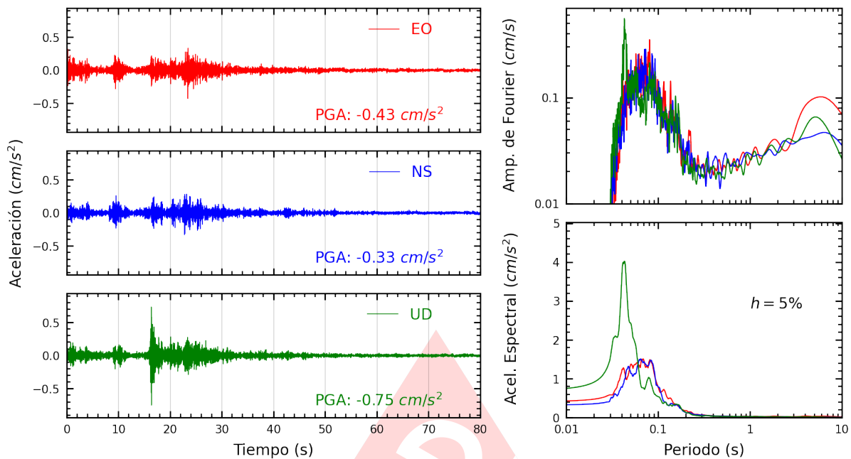
Figura A.15: Registros tiempo-historia, espectros de Fourier y de respuesta en las direcciones EO, NS y vertical de la estación UPCSM. Sismo de Provincia Constitucional del Callao , Callao - Lima del 2022-11-05, 05:26:06 (Hora local)
