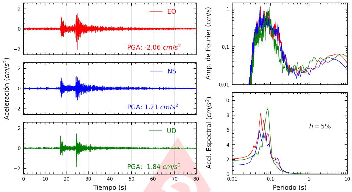
Figura A.5: Registros tiempo-historia, espectros de Fourier y de respuesta en las direcciones EO, NS y vertical de la estación USILM. Sismo de Provincia Constitucional del Callao , Callao - Lima del 2022-11-05, 05:26:06 (Hora local)
