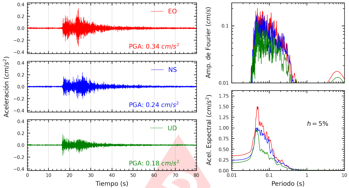
Figura A.29: Registros tiempo-historia, espectros de Fourier y de respuesta en las direcciones EO, NS y vertical de la estación BRISA. Sismo de Provincia Constitucional del Callao , Callao - Lima del 2022-11-05, 05:26:06 (Hora local)
