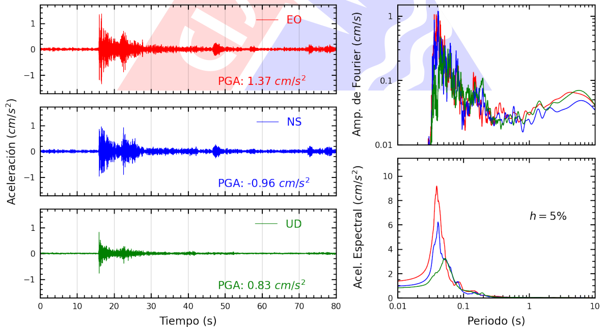
Figura A.8: Registros tiempo-historia, espectros de Fourier y de respuesta en las direcciones EO, NS y vertical de la estación DHNPE. Sismo de Provincia Constitucional del Callao , Callao - Lima del 2022-11-05, 05:26:06 (Hora local)
