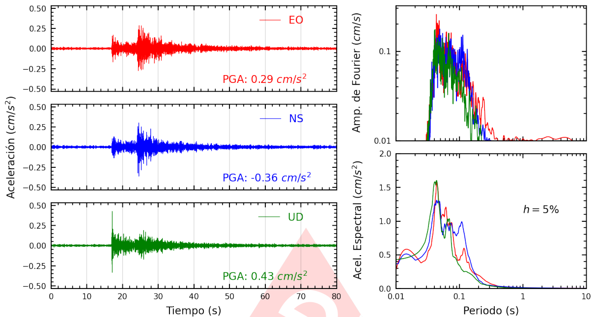
Figura A.23: Registros tiempo-historia, espectros de Fourier y de respuesta en las direcciones EO, NS y vertical de la estación ATARJ. Sismo de Provincia Constitucional del Callao , Callao - Lima del 2022-11-05, 05:26:06 (Hora local)
