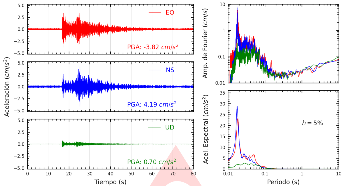
Figura A.1: Registros tiempo-historia, espectros de Fourier y de respuesta en las direcciones EO, NS y vertical de la estación UCSS. Sismo de Provincia Constitucional del Callao , Callao - Lima del 2022-11-05, 05:26:06 (Hora local)
