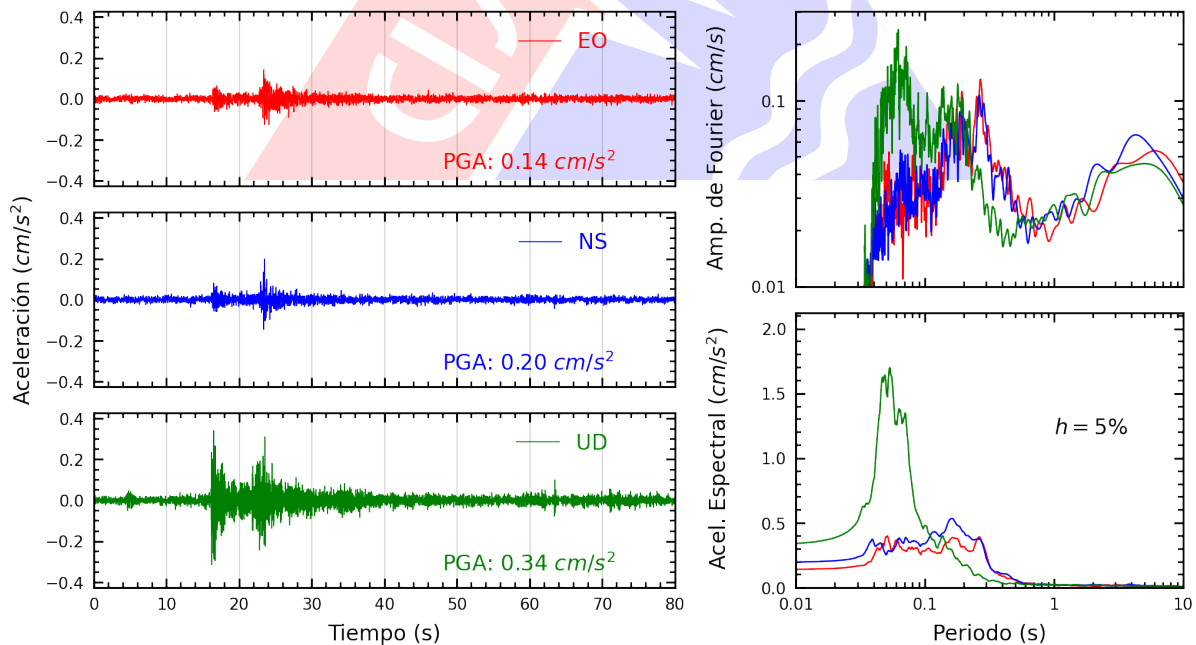
Figura A.28: Registros tiempo-historia, espectros de Fourier y de respuesta en las direcciones EO, NS y vertical de la estación ACAPU. Sismo de Provincia Constitucional del Callao , Callao - Lima del 2022-11-05, 05:26:06 (Hora local)
