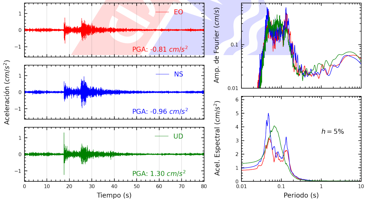
Figura A.10: Registros tiempo-historia, espectros de Fourier y de respuesta en las direcciones EO, NS y vertical de la estación CARAB. Sismo de Provincia Constitucional del Callao , Callao - Lima del 2022-11-05, 05:26:06 (Hora local)
