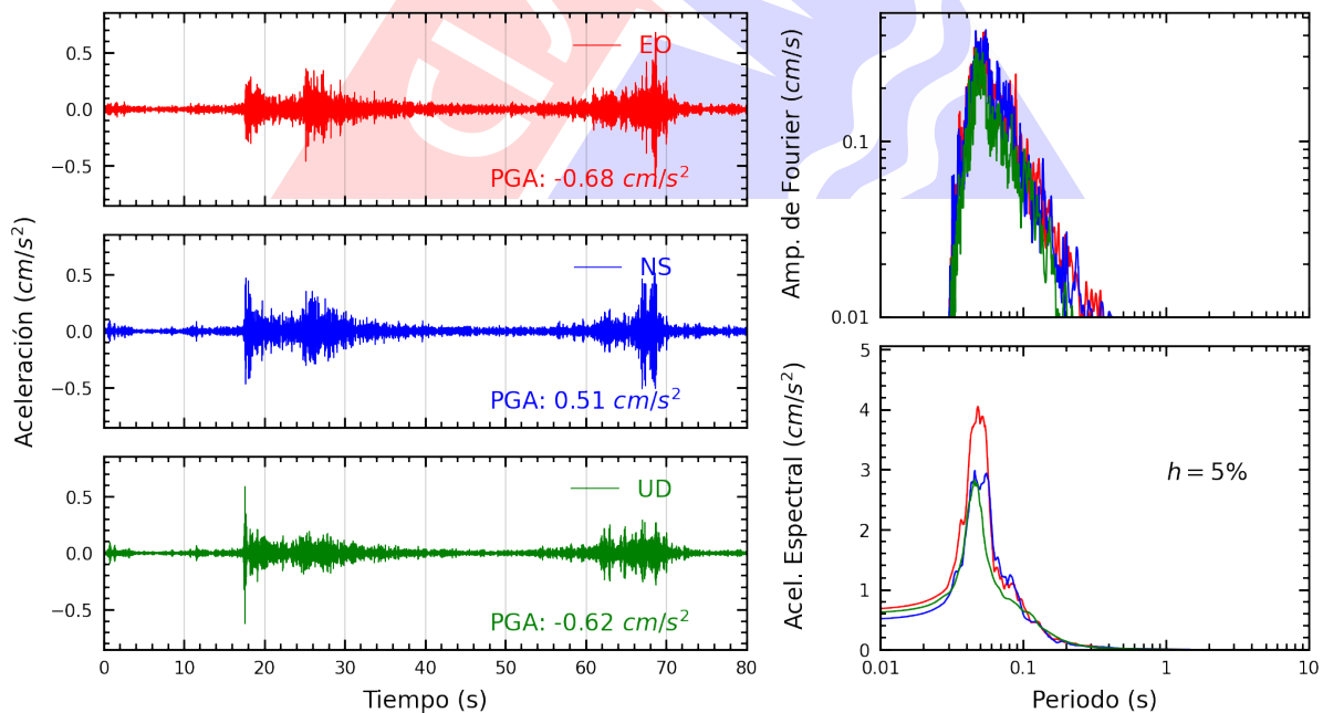
Figura A.16: Registros tiempo-historia, espectros de Fourier y de respuesta en las direcciones EO, NS y vertical de la estación PACHA. Sismo de Provincia Constitucional del Callao , Callao - Lima del 2022-11-05, 05:26:06 (Hora local)
