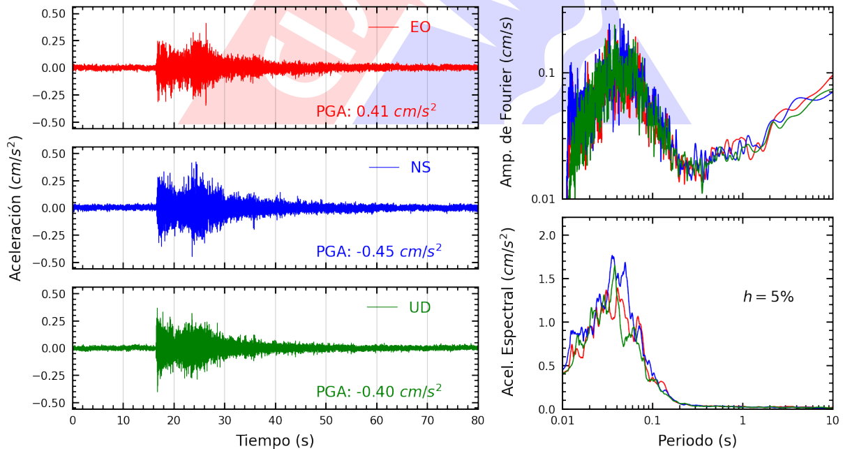
Figura A.22: Registros tiempo-historia, espectros de Fourier y de respuesta en las direcciones EO, NS y vertical de la estación SERVI. Sismo de Provincia Constitucional del Callao , Callao - Lima del 2022-11-05, 05:26:06 (Hora local)
