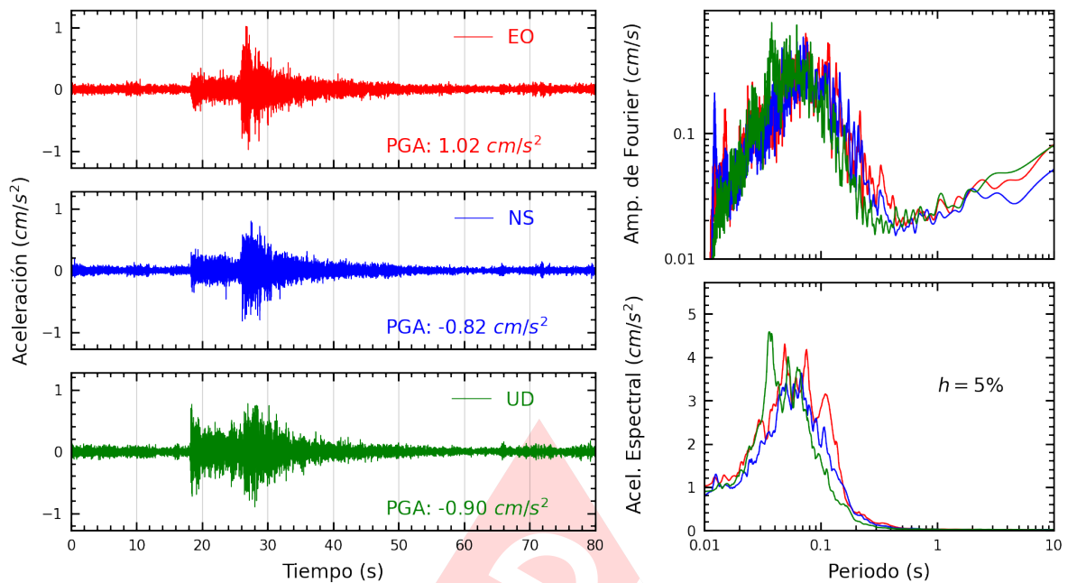
Figura A.11: Registros tiempo-historia, espectros de Fourier y de respuesta en las direcciones EO, NS y vertical de la estación ANCON. Sismo de Provincia Constitucional del Callao , Callao - Lima del 2022-11-05, 05:26:06 (Hora local)
