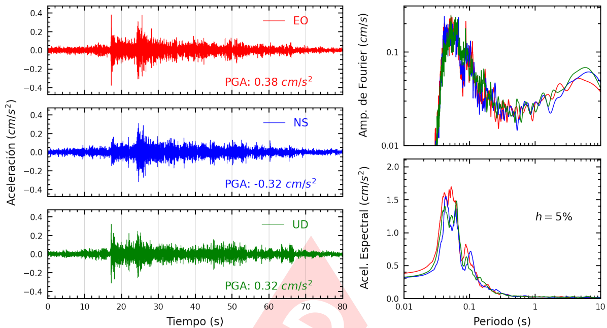
Figura A.27: Registros tiempo-historia, espectros de Fourier y de respuesta en las direcciones EO, NS y vertical de la estación IMCA. Sismo de Provincia Constitucional del Callao , Callao - Lima del 2022-11-05, 05:26:06 (Hora local)
