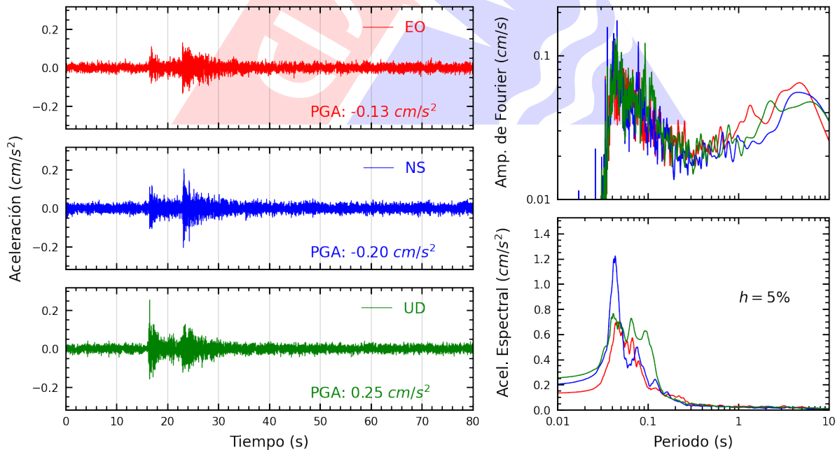
Figura A.32: Registros tiempo-historia, espectros de Fourier y de respuesta en las direcciones EO, NS y vertical de la estación BONDY. Sismo de Provincia Constitucional del Callao , Callao - Lima del 2022-11-05, 05:26:06 (Hora local)
