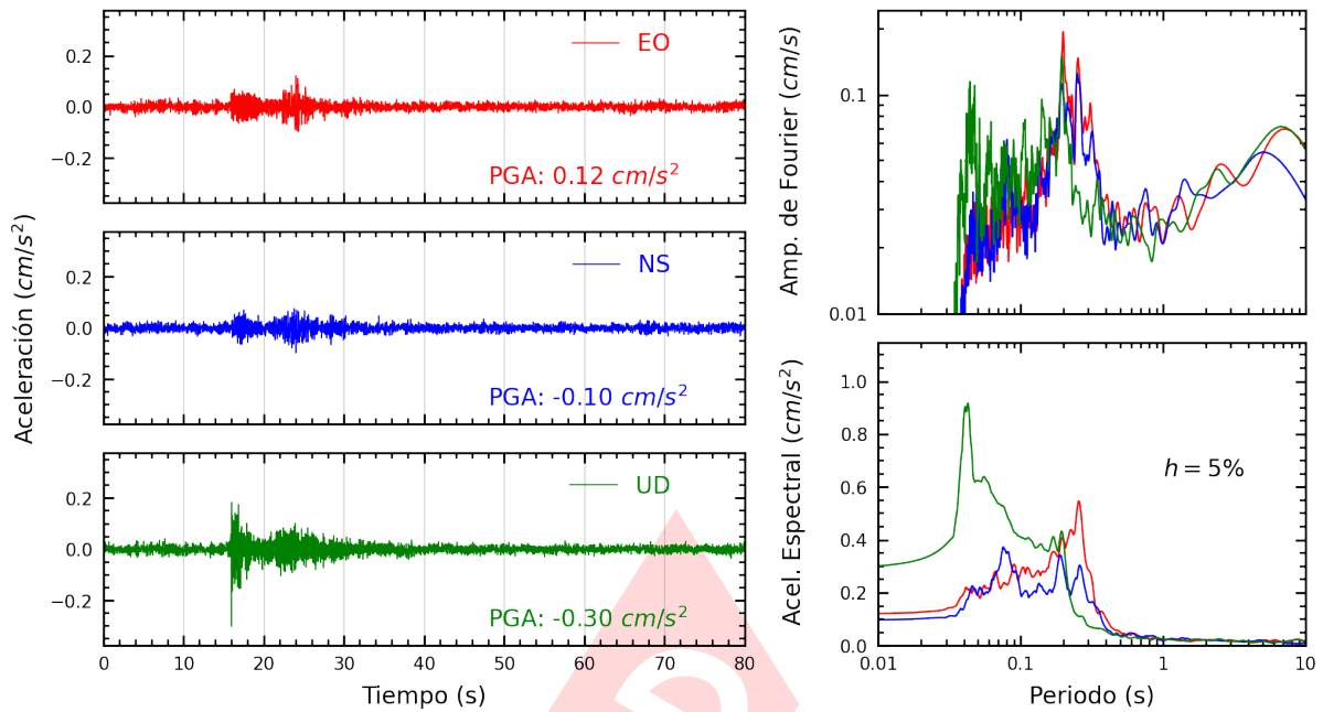
Figura A.31: Registros tiempo-historia, espectros de Fourier y de respuesta en las direcciones EO, NS y vertical de la estación DSMI. Sismo de Provincia Constitucional del Callao , Callao - Lima del 2022-11-05, 05:26:06 (Hora local)
