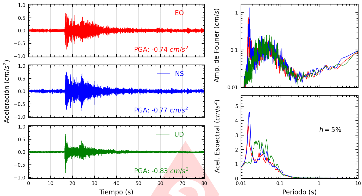
Figura A.13: Registros tiempo-historia, espectros de Fourier y de respuesta en las direcciones EO, NS y vertical de la estación CENEP. Sismo de Provincia Constitucional del Callao , Callao - Lima del 2022-11-05, 05:26:06 (Hora local)
