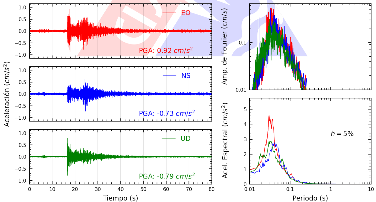
Figura A.12: Registros tiempo-historia, espectros de Fourier y de respuesta en las direcciones EO, NS y vertical de la estación BORJA. Sismo de Provincia Constitucional del Callao , Callao - Lima del 2022-11-05, 05:26:06 (Hora local)
