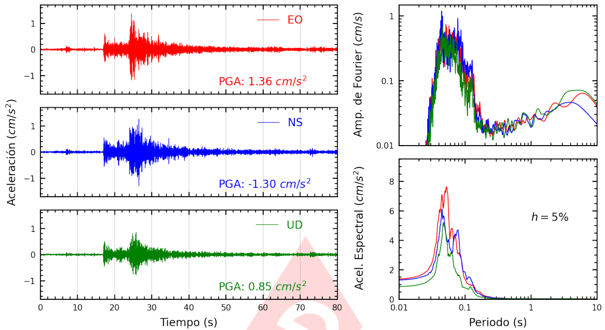
Figura A.9: Registros tiempo-historia, espectros de Fourier y de respuesta en las direcciones EO, NS y vertical de la estación JOSEO. Sismo de Provincia Constitucional del Callao , Callao - Lima del 2022-11-05, 05:26:06 (Hora local)
