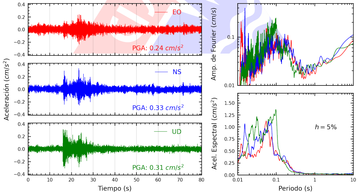
Figura A.30: Registros tiempo-historia, espectros de Fourier y de respuesta en las direcciones EO, NS y vertical de la estación RAMON. Sismo de Provincia Constitucional del Callao , Callao - Lima del 2022-11-05, 05:26:06 (Hora local)
