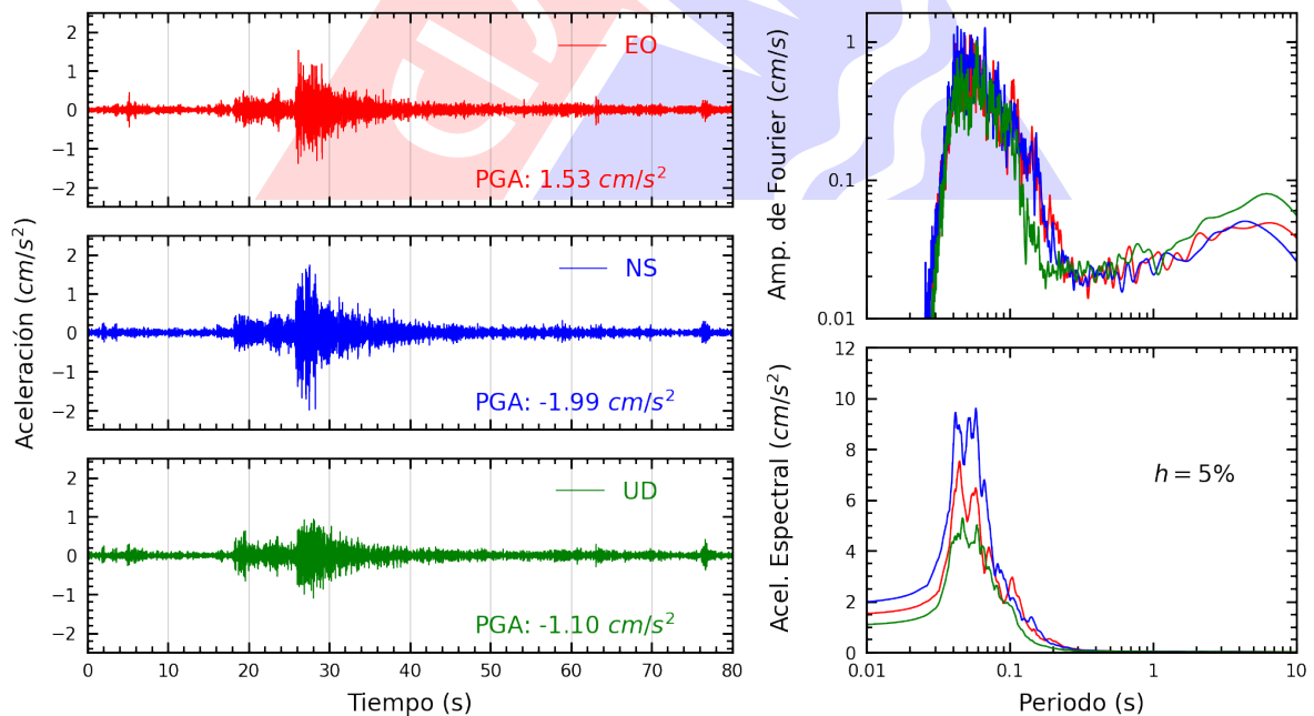
Figura A.6: Registros tiempo-historia, espectros de Fourier y de respuesta en las direcciones EO, NS y vertical de la estación SROSA. Sismo de Provincia Constitucional del Callao , Callao - Lima del 2022-11-05, 05:26:06 (Hora local)
