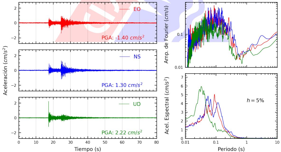
Figura A.4: Registros tiempo-historia, espectros de Fourier y de respuesta en las direcciones EO, NS y vertical de la estación DEFEN. Sismo de Provincia Constitucional del Callao , Callao - Lima del 2022-11-05, 05:26:06 (Hora local)
