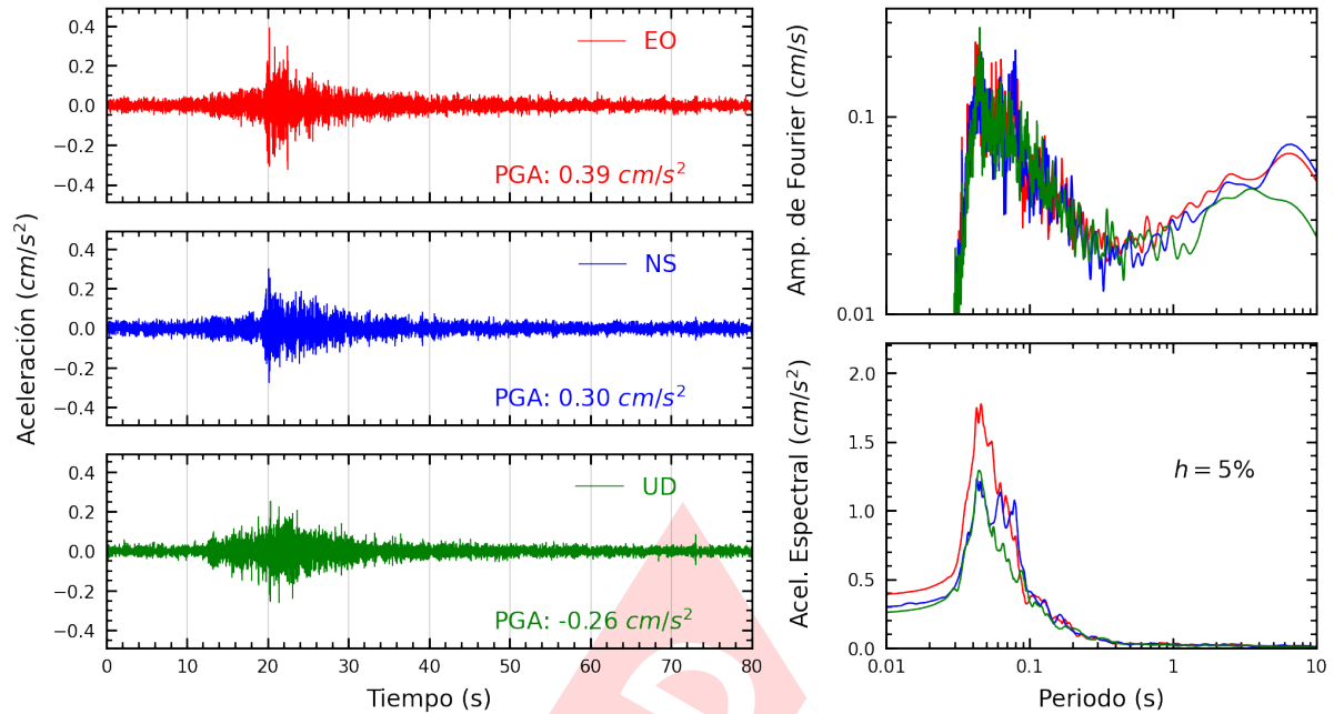
Figura A.27: Registros tiempo-historia, espectros de Fourier y de respuesta en las direcciones EO, NS y vertical de la estación BONDY. Sismo de Ancon, Lima - Lima del 2022-11-10, 07:42:29 (Hora local)
