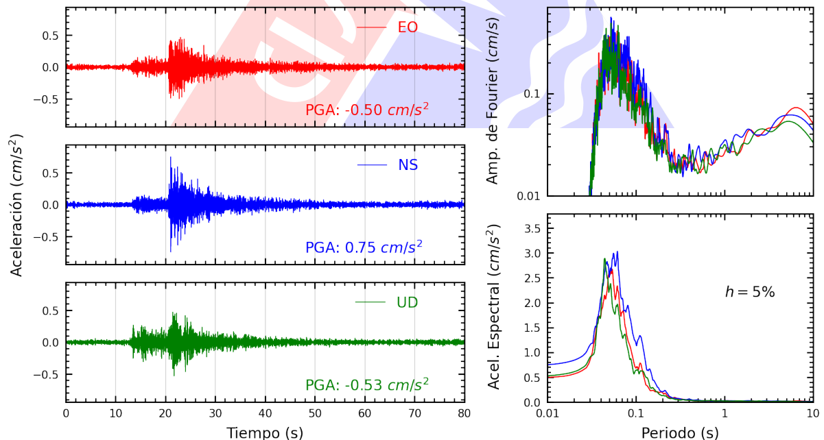
Figura A.18: Registros tiempo-historia, espectros de Fourier y de respuesta en las direcciones EO, NS y vertical de la estación CENEP. Sismo de Ancon, Lima - Lima del 2022-11-10, 07:42:29 (Hora local)
