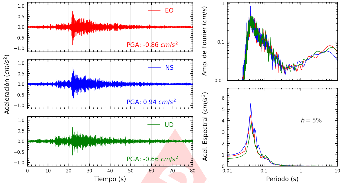
Figura A.17: Registros tiempo-historia, espectros de Fourier y de respuesta en las direcciones EO, NS y vertical de la estación USMP. Sismo de Ancon, Lima - Lima del 2022-11-10, 07:42:29 (Hora local)
