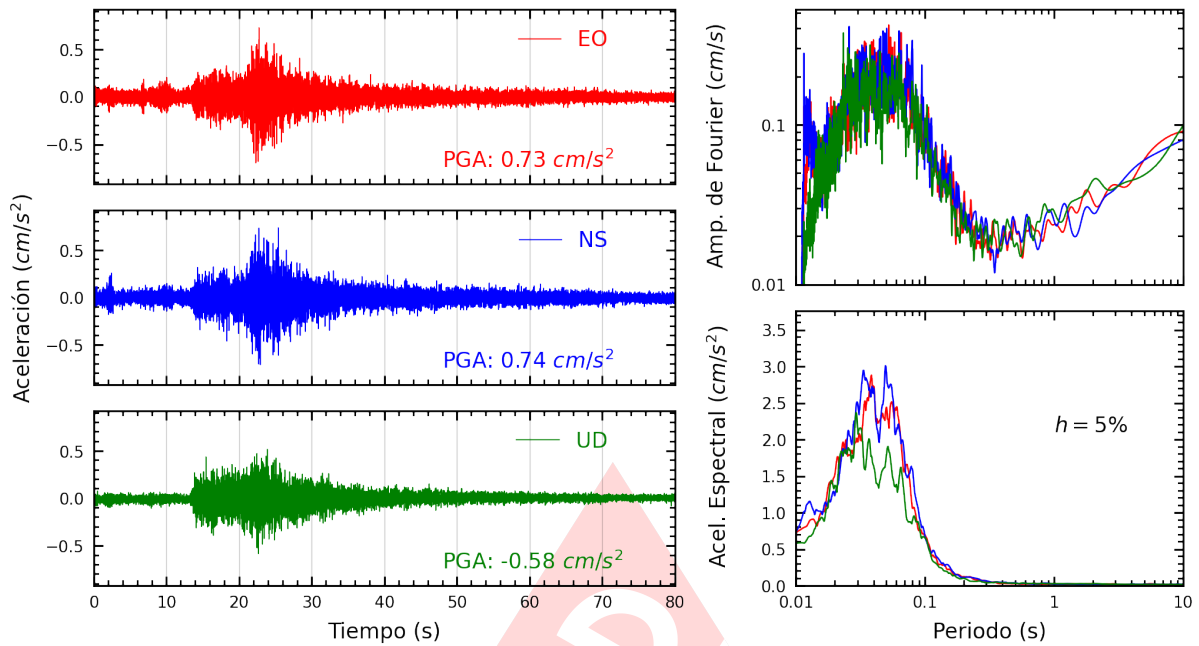
Figura A.19: Registros tiempo-historia, espectros de Fourier y de respuesta en las direcciones EO, NS y vertical de la estación SERVI. Sismo de Ancon, Lima - Lima del 2022-11-10, 07:42:29 (Hora local)
