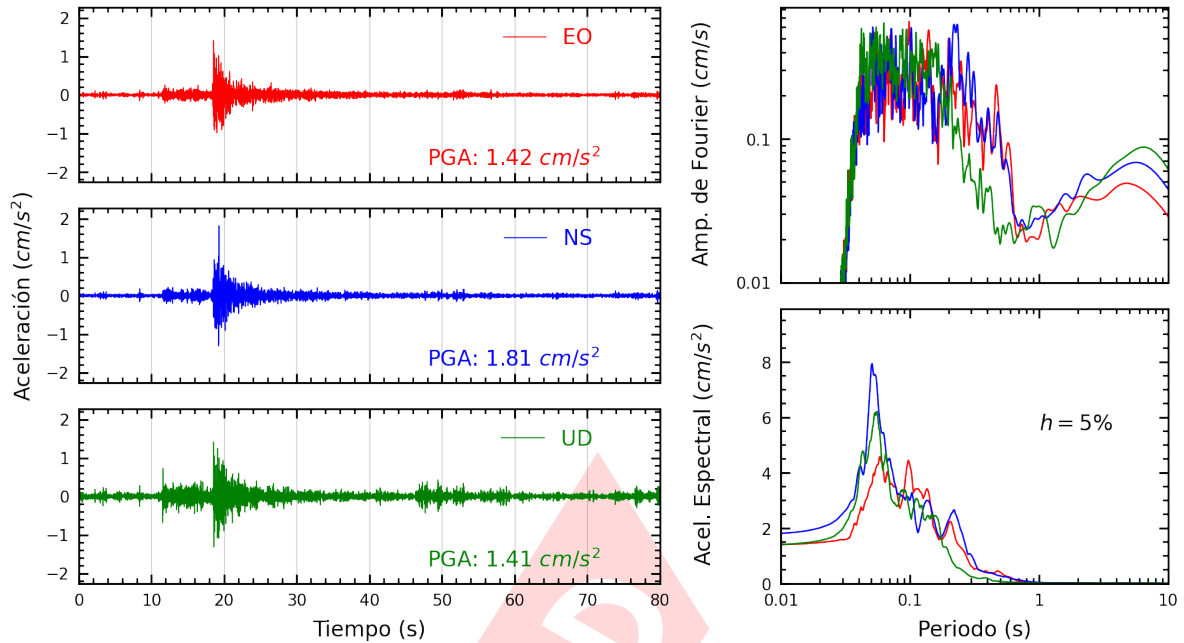
Figura A.9: Registros tiempo-historia, espectros de Fourier y de respuesta en las direcciones EO, NS y vertical de la estación MDPP. Sismo de Ancon, Lima - Lima del 2022-11-10, 07:42:29 (Hora local)
