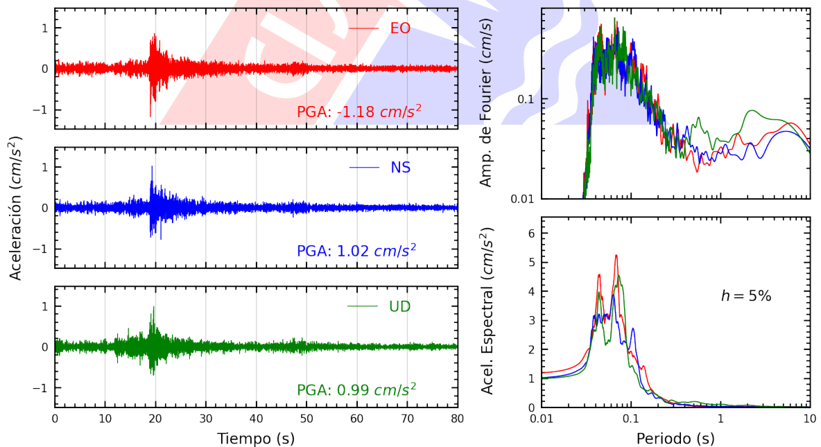
Figura A.14: Registros tiempo-historia, espectros de Fourier y de respuesta en las direcciones EO, NS y vertical de la estación MADRE. Sismo de Ancon, Lima - Lima del 2022-11-10, 07:42:29 (Hora local)
