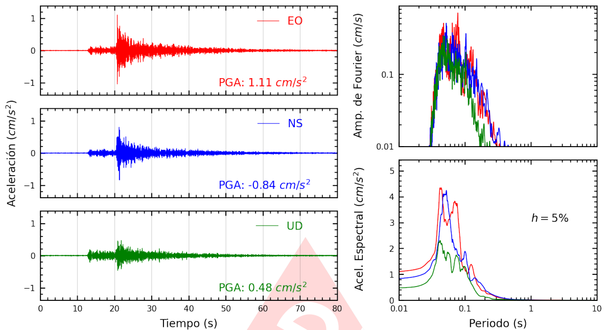
Figura A.15: Registros tiempo-historia, espectros de Fourier y de respuesta en las direcciones EO, NS y vertical de la estación ATARJ. Sismo de Ancon, Lima - Lima del 2022-11-10, 07:42:29 (Hora local)
