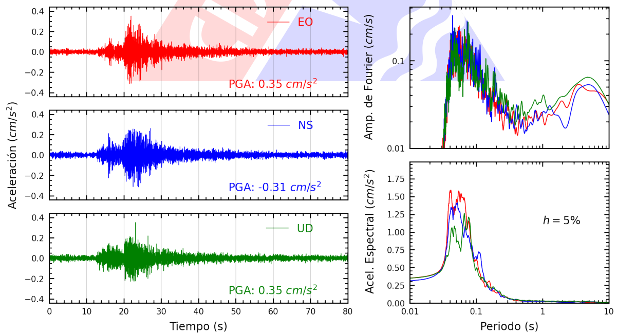
Figura A.28: Registros tiempo-historia, espectros de Fourier y de respuesta en las direcciones EO, NS y vertical de la estación UNFV. Sismo de Ancon, Lima - Lima del 2022-11-10, 07:42:29 (Hora local)
