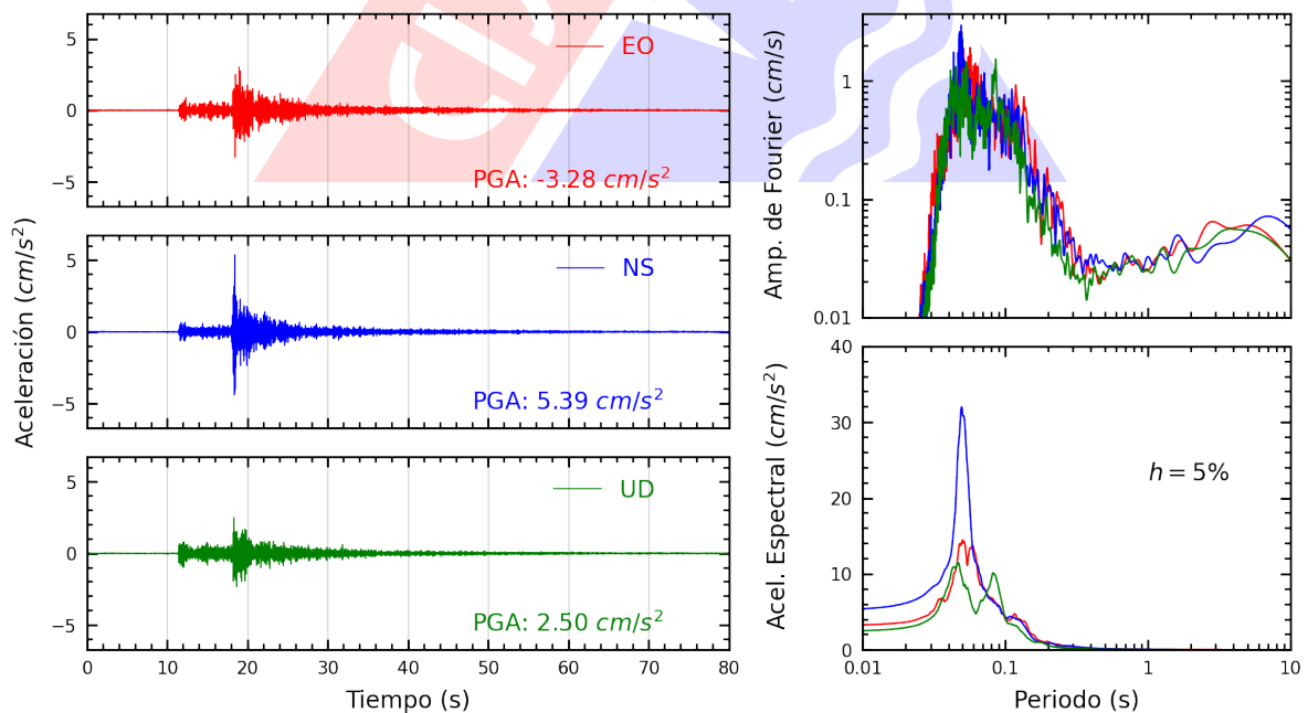
Figura A.4: Registros tiempo-historia, espectros de Fourier y de respuesta en las direcciones EO, NS y vertical de la estación AMORE. Sismo de Ancon, Lima - Lima del 2022-11-10, 07:42:29 (Hora local)
