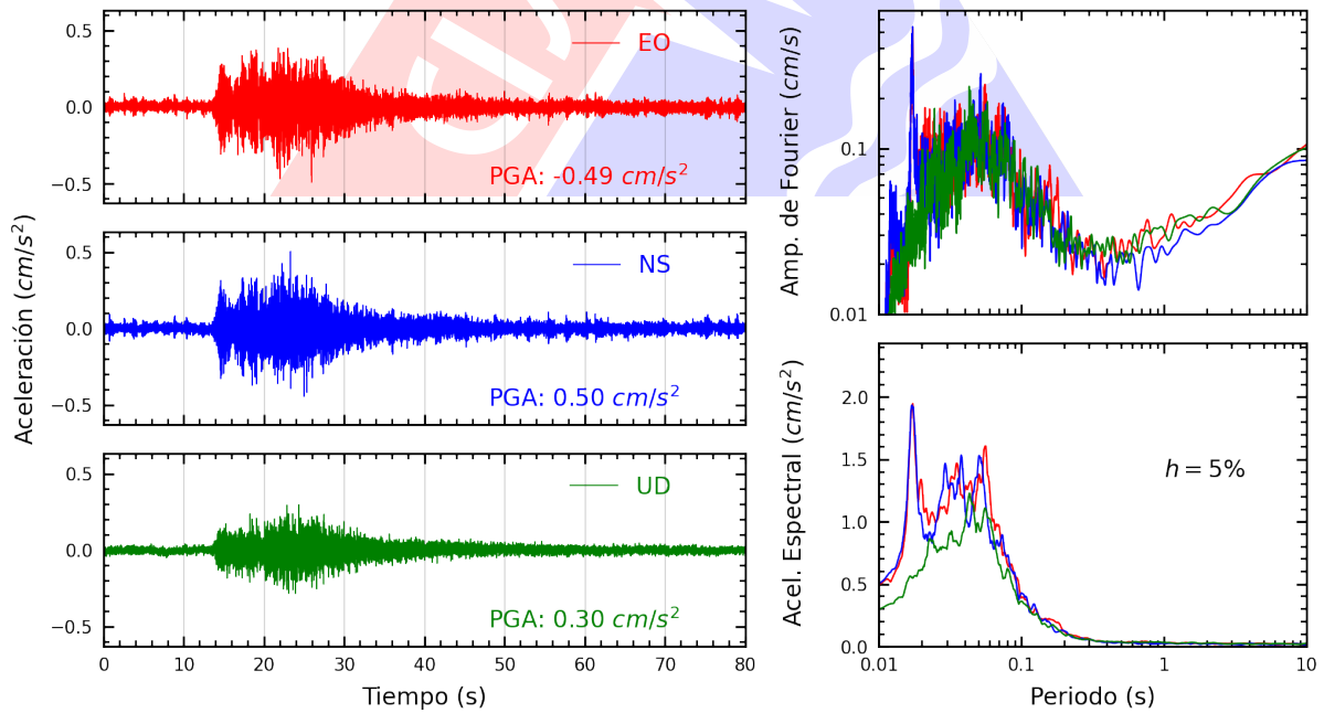
Figura A.22: Registros tiempo-historia, espectros de Fourier y de respuesta en las direcciones EO, NS y vertical de la estación UNMSM. Sismo de Ancon, Lima - Lima del 2022-11-10, 07:42:29 (Hora local)
