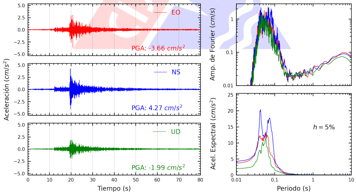
Figura A.6: Registros tiempo-historia, espectros de Fourier y de respuesta en las direcciones EO, NS y vertical de la estación JOSEO. Sismo de Ancon, Lima - Lima del 2022-11-10, 07:42:29 (Hora local)
