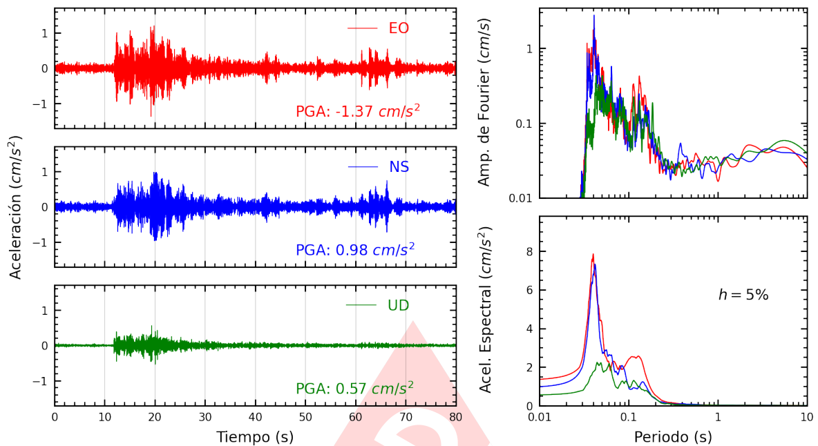
Figura A.13: Registros tiempo-historia, espectros de Fourier y de respuesta en las direcciones EO, NS y vertical de la estación DHNPE. Sismo de Ancon, Lima - Lima del 2022-11-10, 07:42:29 (Hora local)
