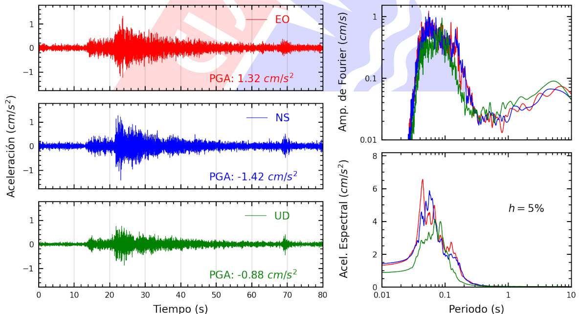
Figura A.12: Registros tiempo-historia, espectros de Fourier y de respuesta en las direcciones EO, NS y vertical de la estación USILM. Sismo de Ancon, Lima - Lima del 2022-11-10, 07:42:29 (Hora local)
