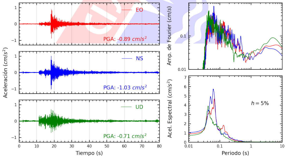
Figura A.16: Registros tiempo-historia, espectros de Fourier y de respuesta en las direcciones EO, NS y vertical de la estación VHAYA. Sismo de Ancon, Lima - Lima del 2022-11-10, 07:42:29 (Hora local)
