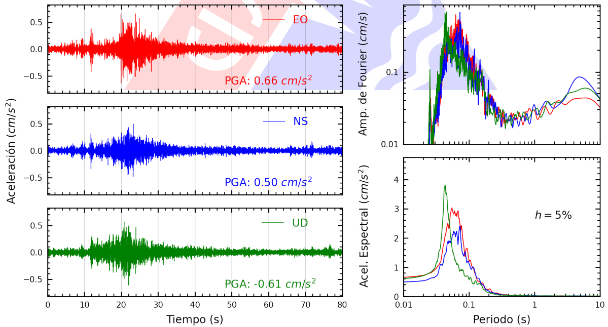
Figura A.20: Registros tiempo-historia, espectros de Fourier y de respuesta en las direcciones EO, NS y vertical de la estación UPCSM. Sismo de Ancon, Lima - Lima del 2022-11-10, 07:42:29 (Hora local)
