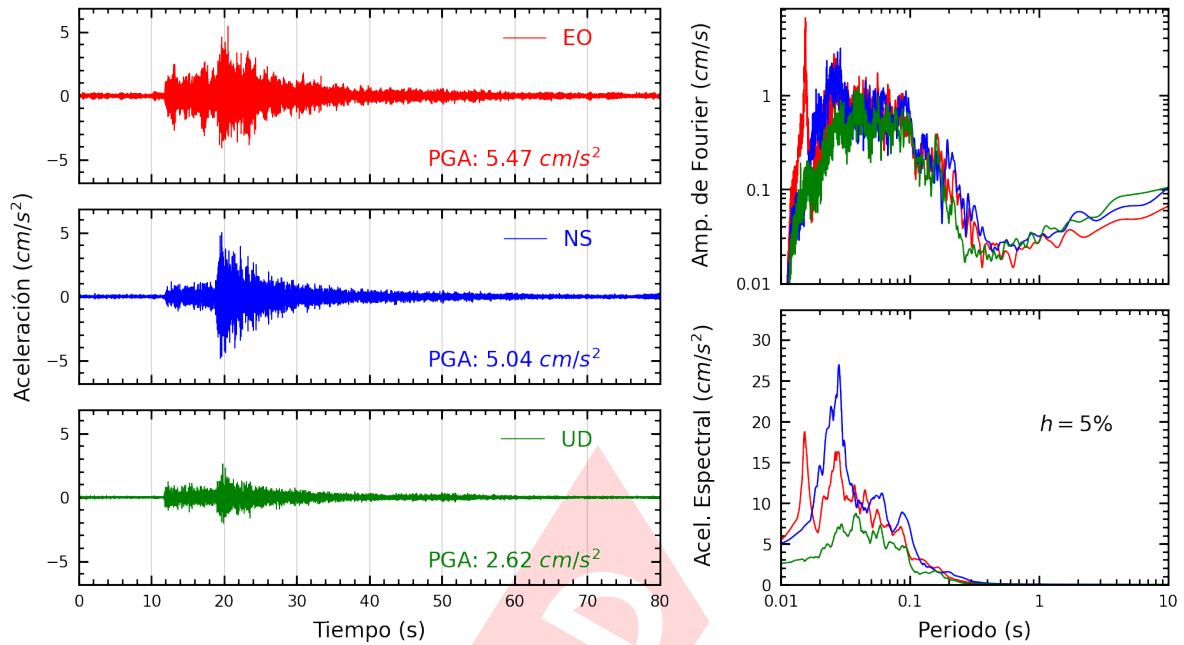
Figura A.3: Registros tiempo-historia, espectros de Fourier y de respuesta en las direcciones EO, NS y vertical de la estación INDEP. Sismo de Ancon, Lima - Lima del 2022-11-10, 07:42:29 (Hora local)
