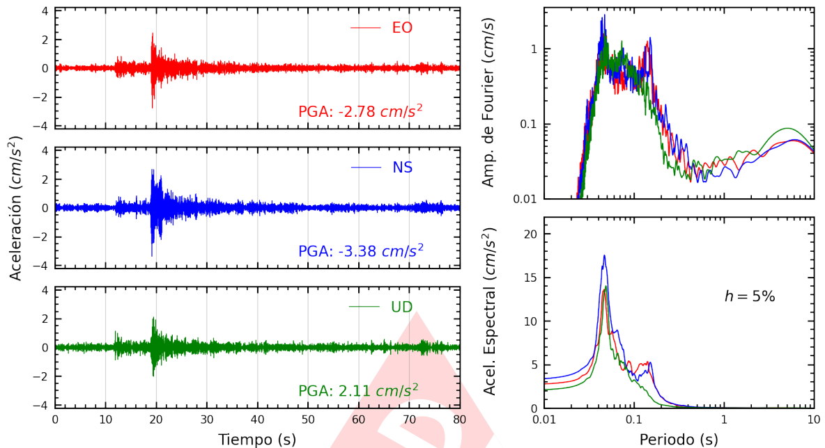
Figura A.7: Registros tiempo-historia, espectros de Fourier y de respuesta en las direcciones EO, NS y vertical de la estación CARAB. Sismo de Ancon, Lima - Lima del 2022-11-10, 07:42:29 (Hora local)
