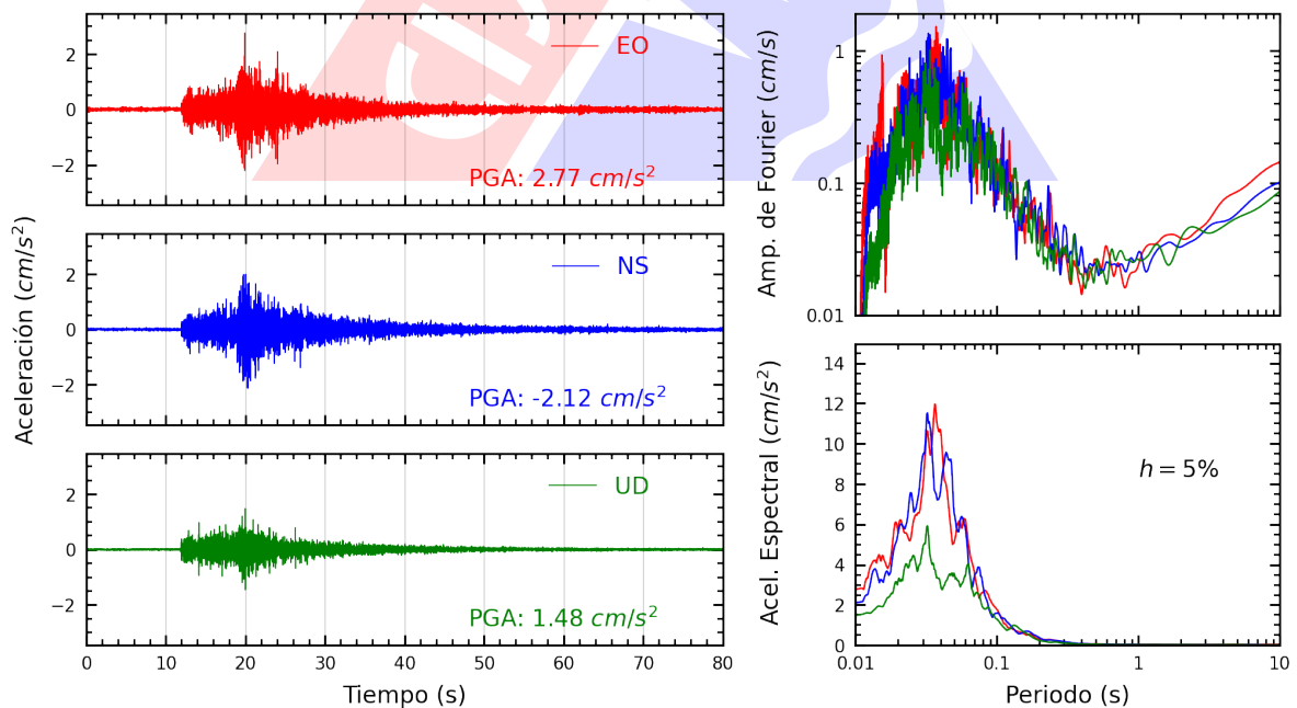
Figura A.8: Registros tiempo-historia, espectros de Fourier y de respuesta en las direcciones EO, NS y vertical de la estación COMAS. Sismo de Ancon, Lima - Lima del 2022-11-10, 07:42:29 (Hora local)
