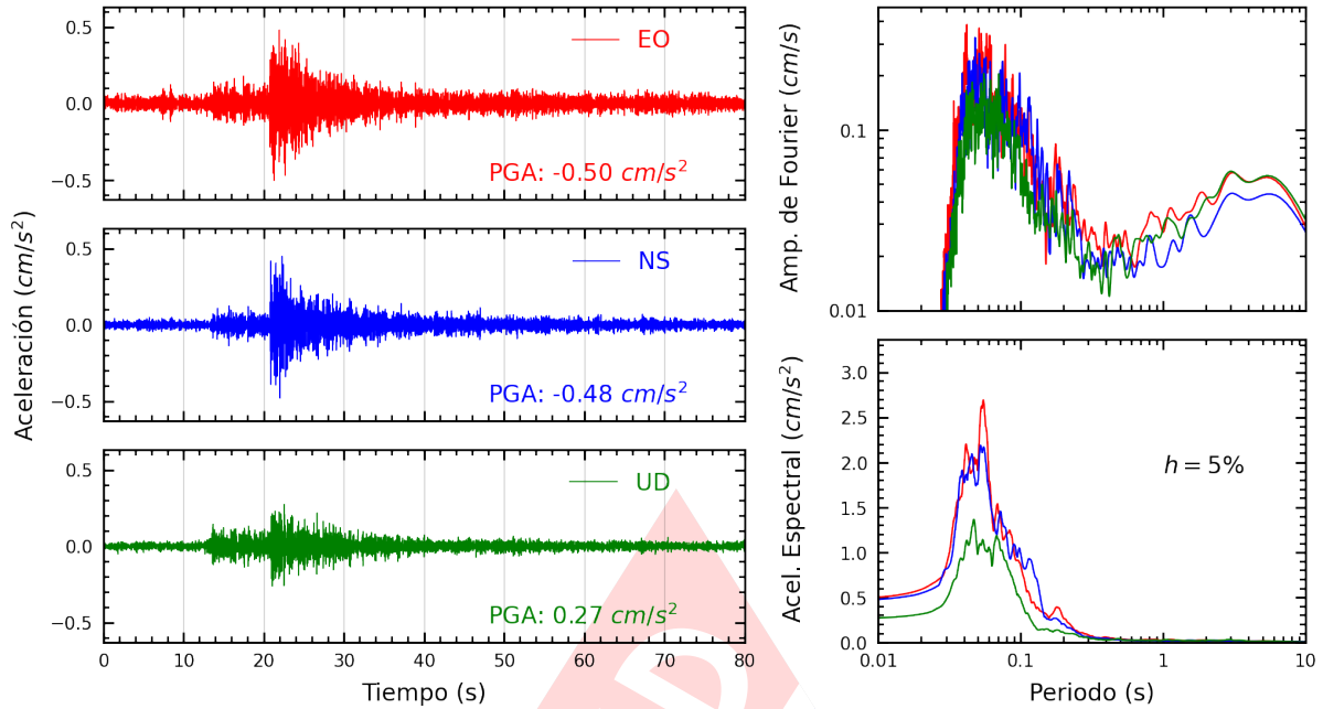
Figura A.23: Registros tiempo-historia, espectros de Fourier y de respuesta en las direcciones EO, NS y vertical de la estación INICT. Sismo de Ancon, Lima - Lima del 2022-11-10, 07:42:29 (Hora local)
