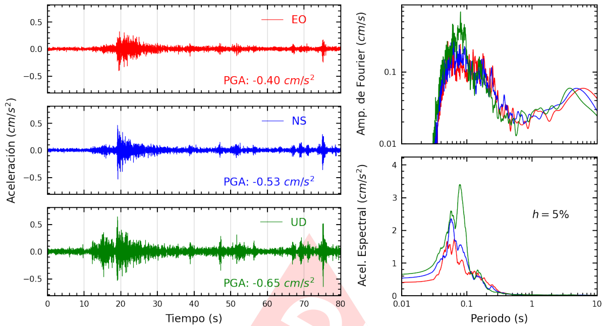
Figura A.21: Registros tiempo-historia, espectros de Fourier y de respuesta en las direcciones EO, NS y vertical de la estación RAMON. Sismo de Ancon, Lima - Lima del 2022-11-10, 07:42:29 (Hora local)
