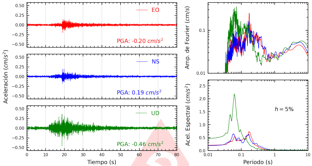
Figura A.25: Registros tiempo-historia, espectros de Fourier y de respuesta en las direcciones EO, NS y vertical de la estación ACAPU. Sismo de Ancon, Lima - Lima del 2022-11-10, 07:42:29 (Hora local)
