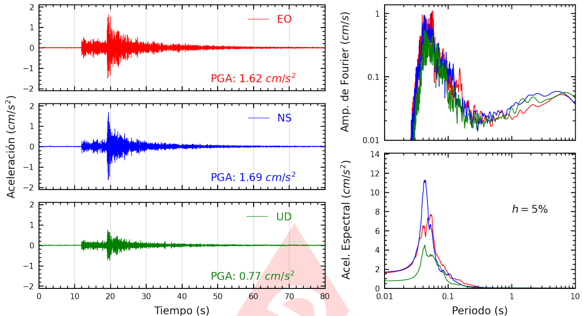
Figura A.11: Registros tiempo-historia, espectros de Fourier y de respuesta en las direcciones EO, NS y vertical de la estación UCSS. Sismo de Ancon, Lima - Lima del 2022-11-10, 07:42:29 (Hora local)
