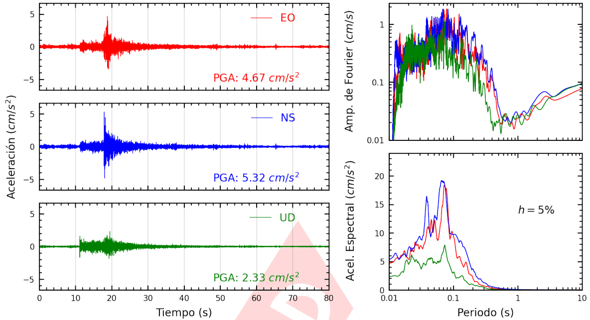
Figura A.5: Registros tiempo-historia, espectros de Fourier y de respuesta en las direcciones EO, NS y vertical de la estación DEFEN. Sismo de Ancon, Lima - Lima del 2022-11-10, 07:42:29 (Hora local)
