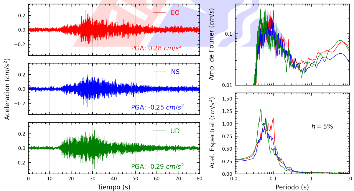
Figura A.30: Registros tiempo-historia, espectros de Fourier y de respuesta en las direcciones EO, NS y vertical de la estación USILP. Sismo de Ancon, Lima - Lima del 2022-11-10, 07:42:29 (Hora local)
