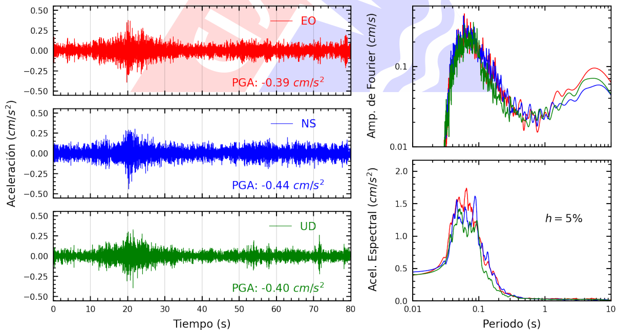
Figura A.26: Registros tiempo-historia, espectros de Fourier y de respuesta en las direcciones EO, NS y vertical de la estación NISTA. Sismo de Ancon, Lima - Lima del 2022-11-10, 07:42:29 (Hora local)
