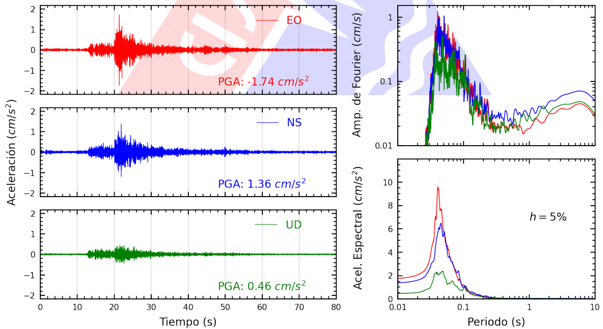
Figura A.10: Registros tiempo-historia, espectros de Fourier y de respuesta en las direcciones EO, NS y vertical de la estación CEPRE. Sismo de Ancon, Lima - Lima del 2022-11-10, 07:42:29 (Hora local)
