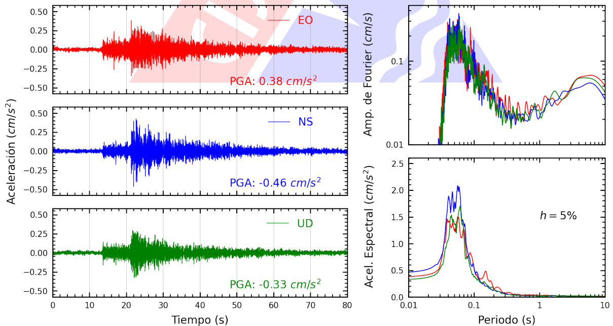
Figura A.24: Registros tiempo-historia, espectros de Fourier y de respuesta en las direcciones EO, NS y vertical de la estación IMCA. Sismo de Ancon, Lima - Lima del 2022-11-10, 07:42:29 (Hora local)
