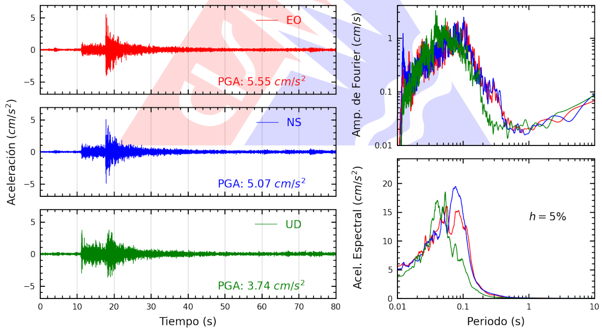
Figura A.2: Registros tiempo-historia, espectros de Fourier y de respuesta en las direcciones EO, NS y vertical de la estación ANCON. Sismo de Ancon, Lima - Lima del 2022-11-10, 07:42:29 (Hora local)
