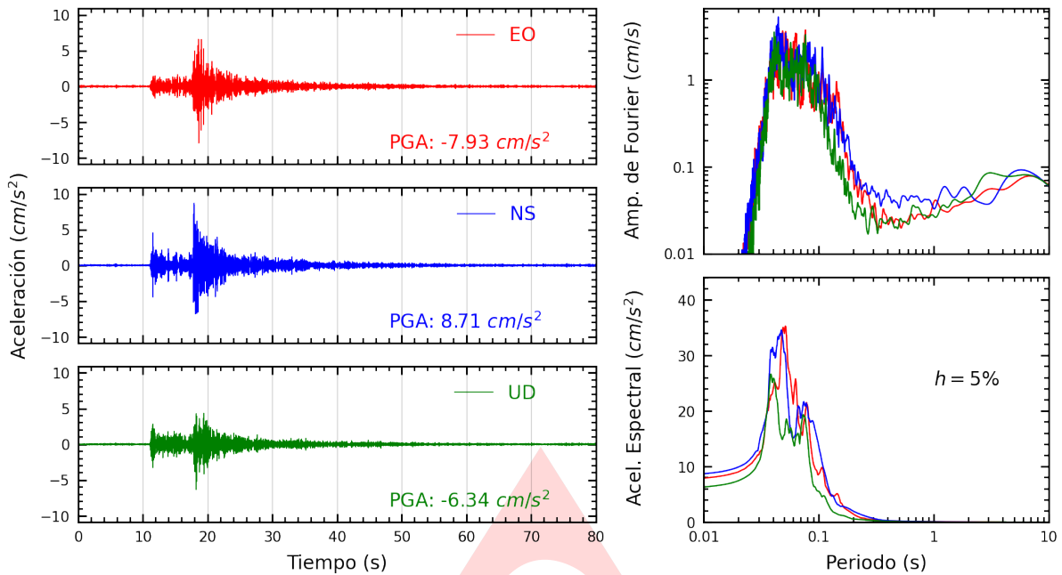
Figura A.1: Registros tiempo-historia, espectros de Fourier y de respuesta en las direcciones EO, NS y vertical de la estación SROSA. Sismo de Ancon, Lima - Lima del 2022-11-10, 07:42:29 (Hora local)
