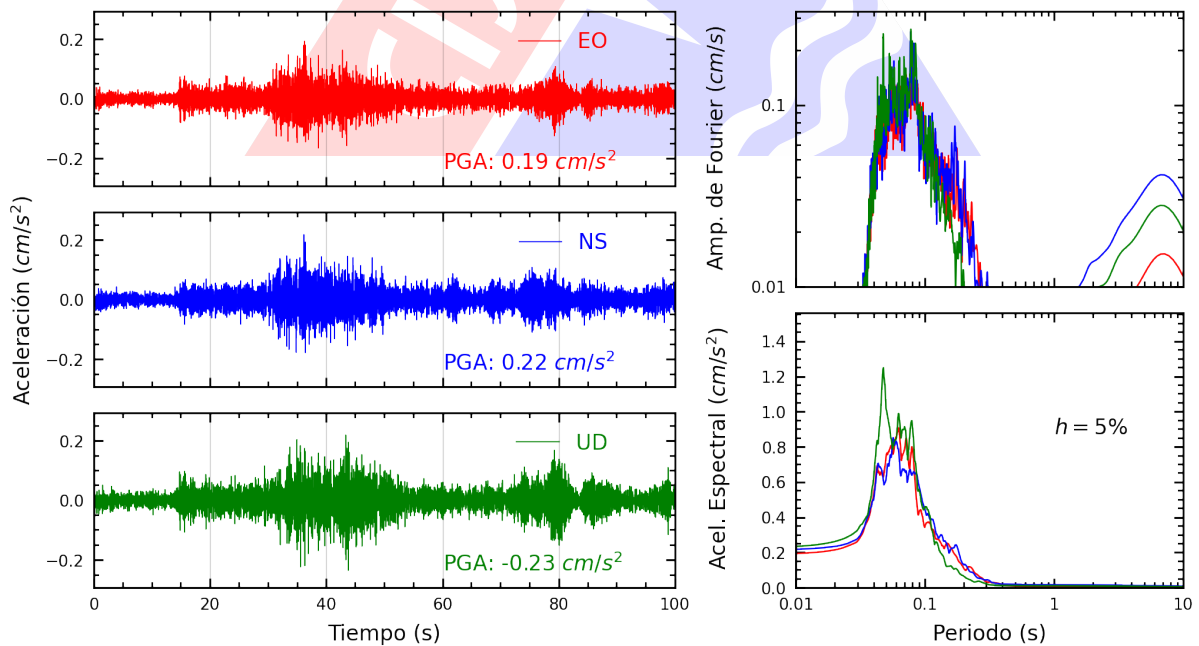
Figura A.32: Registros tiempo-historia, espectros de Fourier y de respuesta en las direcciones EO, NS y vertical de la estación ASIA. Sismo de Ancon, Lima - Lima del 2022-11-10, 07:42:29 (Hora local)
