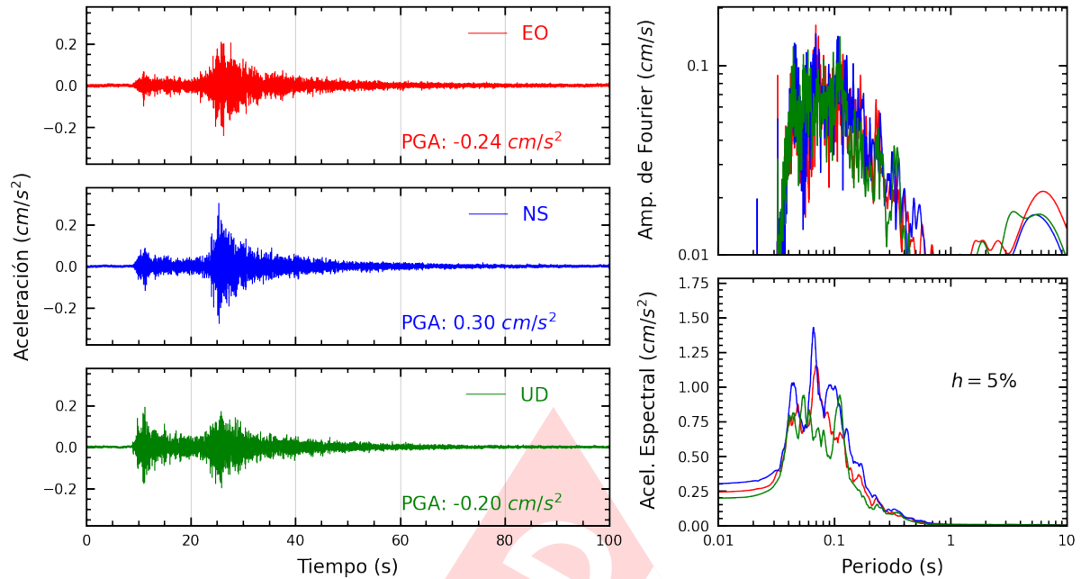
Figura A.29: Registros tiempo-historia, espectros de Fourier y de respuesta en las direcciones EO, NS y vertical de la estación CARAL. Sismo de Ancon, Lima - Lima del 2022-11-10, 07:42:29 (Hora local)
