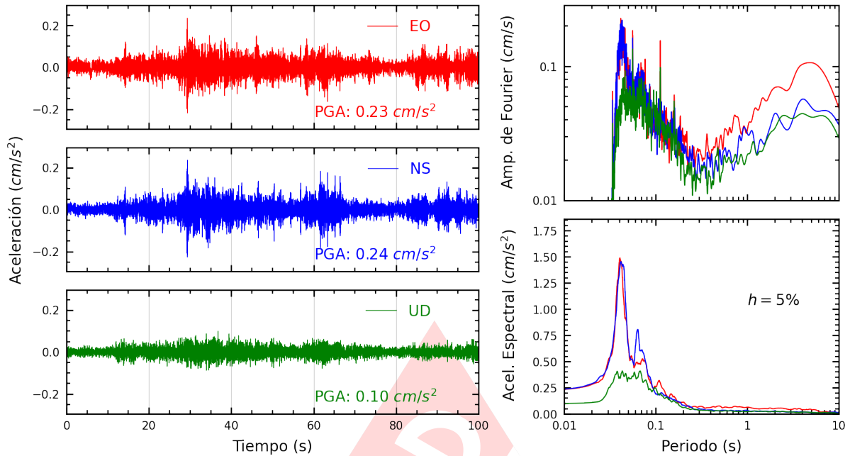
Figura A.31: Registros tiempo-historia, espectros de Fourier y de respuesta en las direcciones EO, NS y vertical de la estación UNAB. Sismo de Ancon, Lima - Lima del 2022-11-10, 07:42:29 (Hora local)
