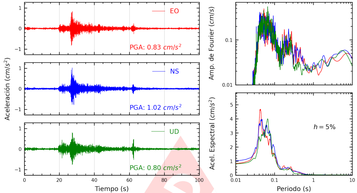
Figura A.25: Registros tiempo-historia, espectros de Fourier y de respuesta en las direcciones EO, NS y vertical de la estación USMP. Sismo de Lima, Lima - Lima del 2022-11-24, 05:56:59 (Hora local)
