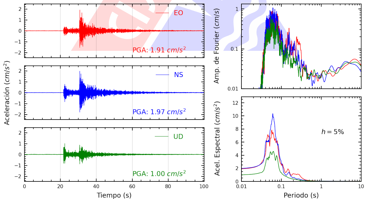
Figura A.12: Registros tiempo-historia, espectros de Fourier y de respuesta en las direcciones EO, NS y vertical de la estación IPEN. Sismo de Lima, Lima - Lima del 2022-11-24, 05:56:59 (Hora local)
