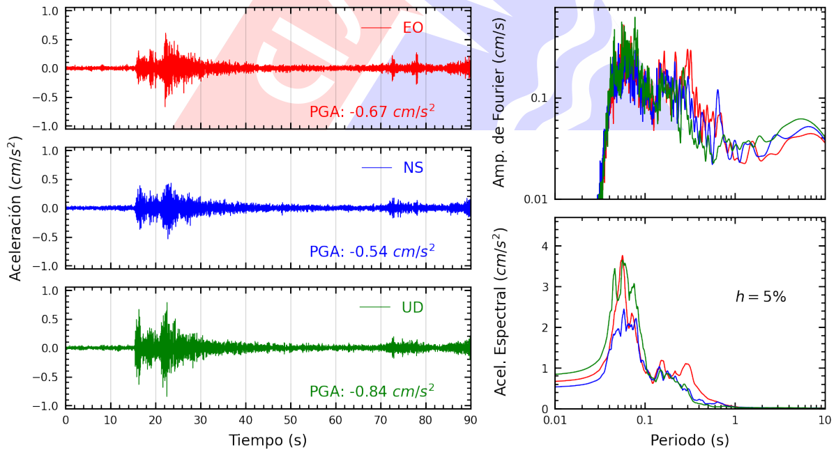
Figura A.30: Registros tiempo-historia, espectros de Fourier y de respuesta en las direcciones EO, NS y vertical de la estación PRADO. Sismo de Lima, Lima - Lima del 2022-11-24, 05:56:59 (Hora local)
