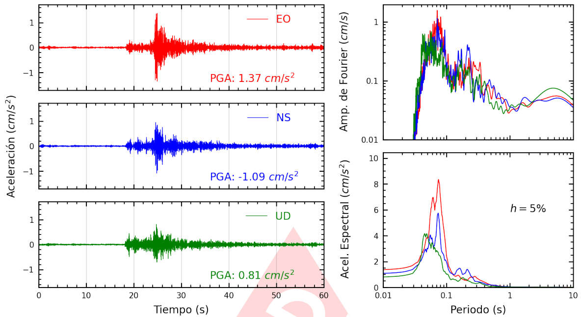
Figura A.17: Registros tiempo-historia, espectros de Fourier y de respuesta en las direcciones EO, NS y vertical de la estación UPCSM. Sismo de Lima, Lima - Lima del 2022-11-24, 05:56:59 (Hora local)
