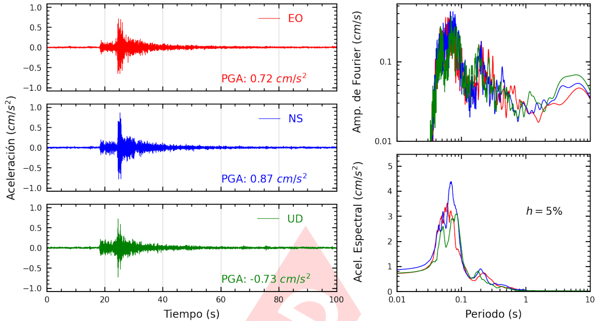
Figura A.29: Registros tiempo-historia, espectros de Fourier y de respuesta en las direcciones EO, NS y vertical de la estación UNFV. Sismo de Lima, Lima - Lima del 2022-11-24, 05:56:59 (Hora local)
