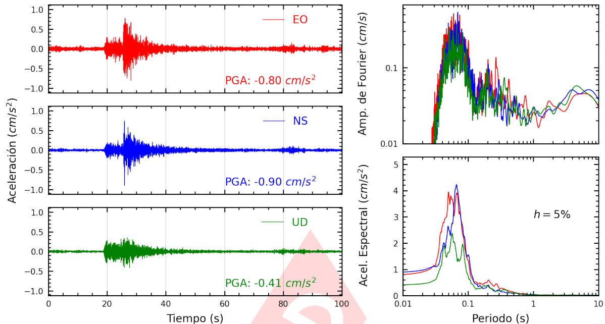
Figura A.27: Registros tiempo-historia, espectros de Fourier y de respuesta en las direcciones EO, NS y vertical de la estación INICT. Sismo de Lima, Lima - Lima del 2022-11-24, 05:56:59 (Hora local)
