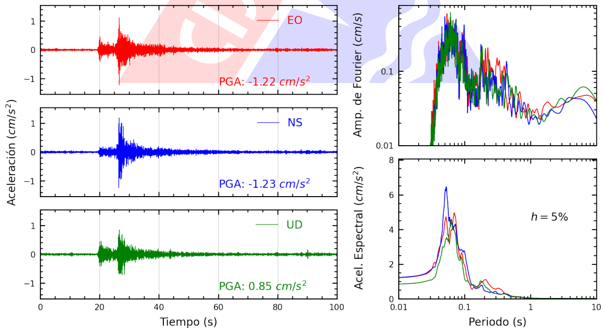
Figura A.20: Registros tiempo-historia, espectros de Fourier y de respuesta en las direcciones EO, NS y vertical de la estación IMCA. Sismo de Lima, Lima - Lima del 2022-11-24, 05:56:59 (Hora local)
