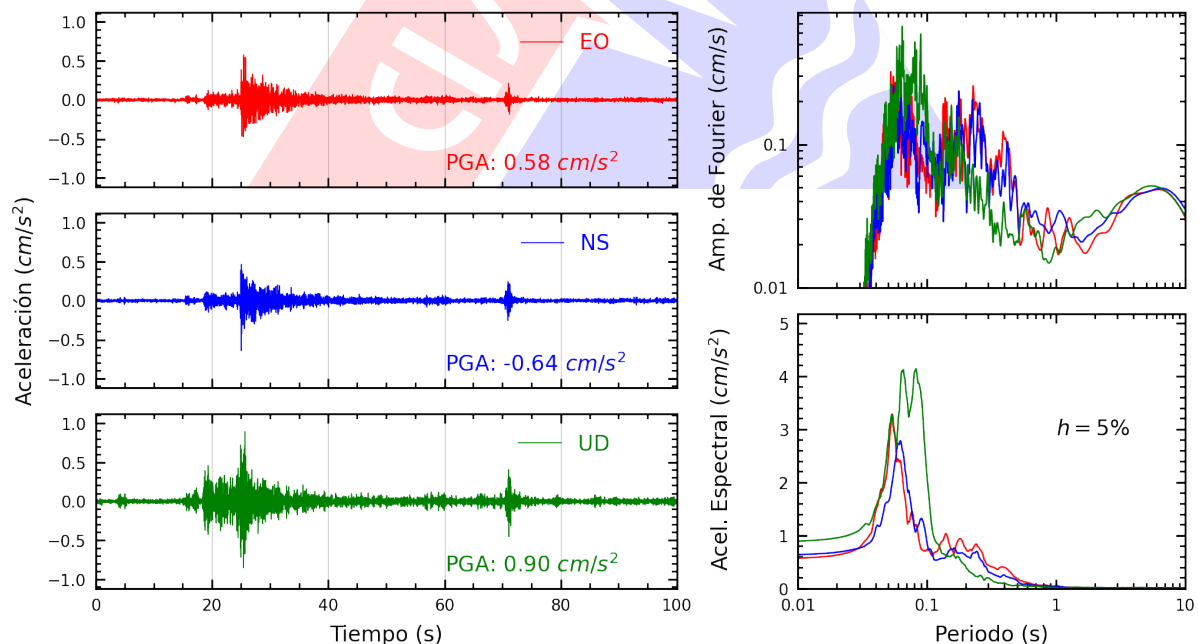
Figura A.28: Registros tiempo-historia, espectros de Fourier y de respuesta en las direcciones EO, NS y vertical de la estación RAMON. Sismo de Lima, Lima - Lima del 2022-11-24, 05:56:59 (Hora local)
