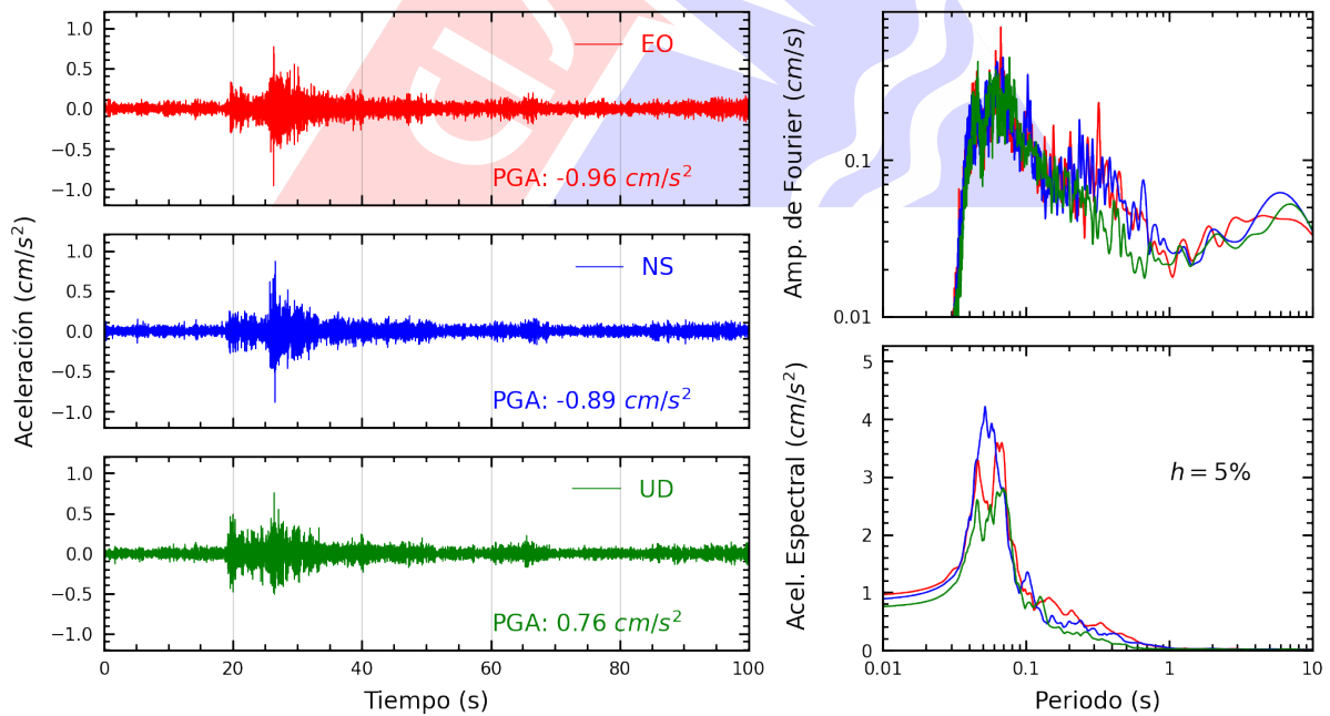
Figura A.26: Registros tiempo-historia, espectros de Fourier y de respuesta en las direcciones EO, NS y vertical de la estación MADRE. Sismo de Lima, Lima - Lima del 2022-11-24, 05:56:59 (Hora local)
