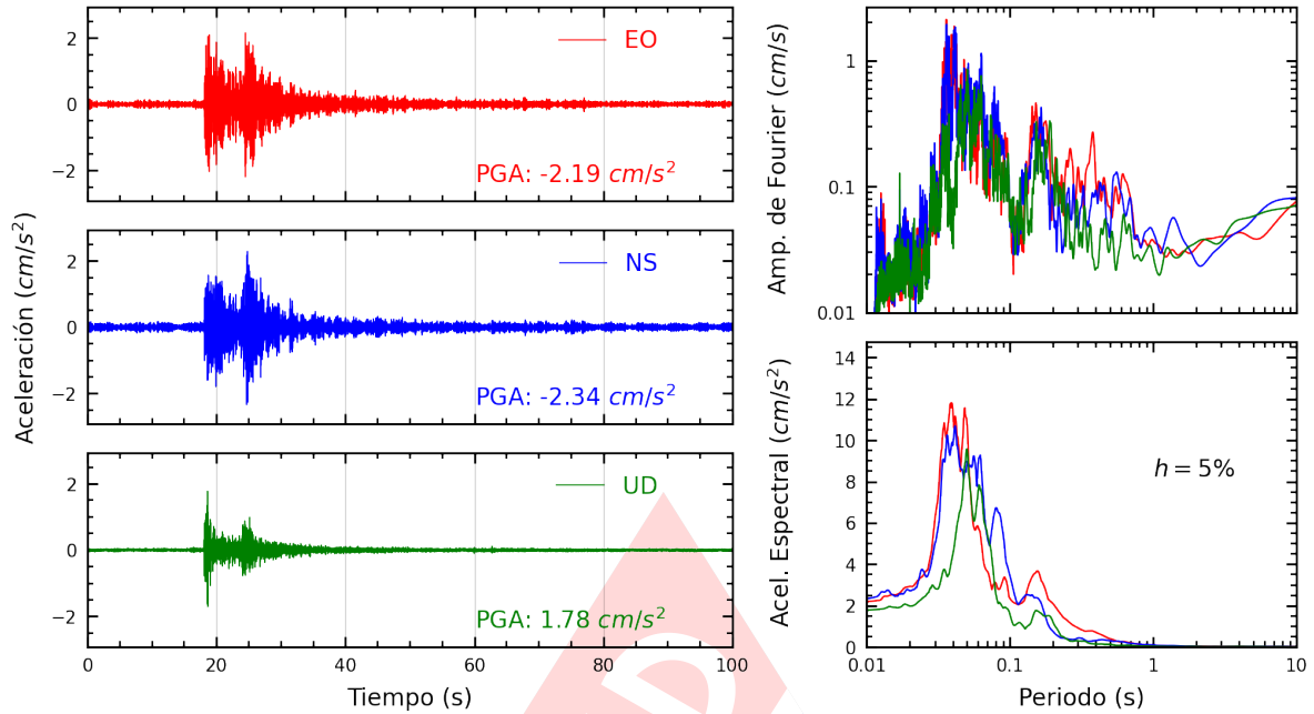
Figura A.9: Registros tiempo-historia, espectros de Fourier y de respuesta en las direcciones EO, NS y vertical de la estación DHNPE. Sismo de Lima, Lima - Lima del 2022-11-24, 05:56:59 (Hora local)
