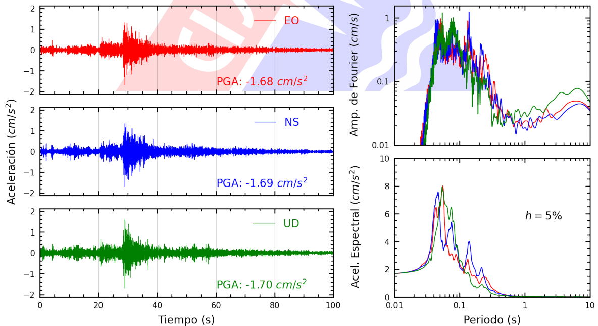
Figura A.14: Registros tiempo-historia, espectros de Fourier y de respuesta en las direcciones EO, NS y vertical de la estación CARAB. Sismo de Lima, Lima - Lima del 2022-11-24, 05:56:59 (Hora local)
