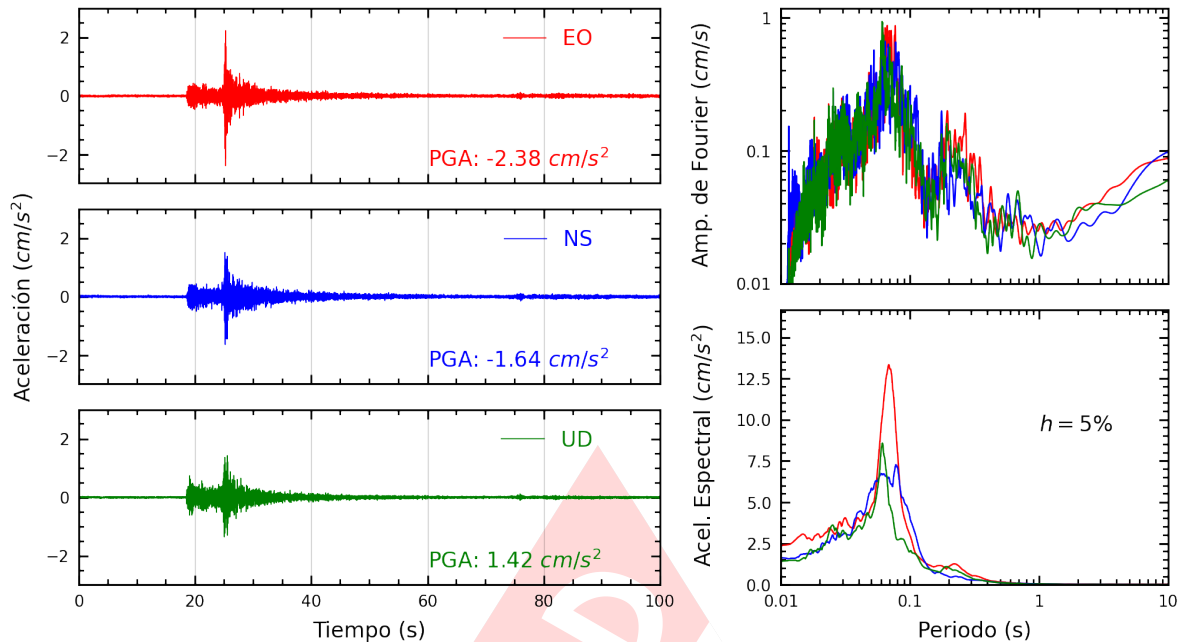
Figura A.7: Registros tiempo-historia, espectros de Fourier y de respuesta en las direcciones EO, NS y vertical de la estación SERVI. Sismo de Lima, Lima - Lima del 2022-11-24, 05:56:59 (Hora local)
