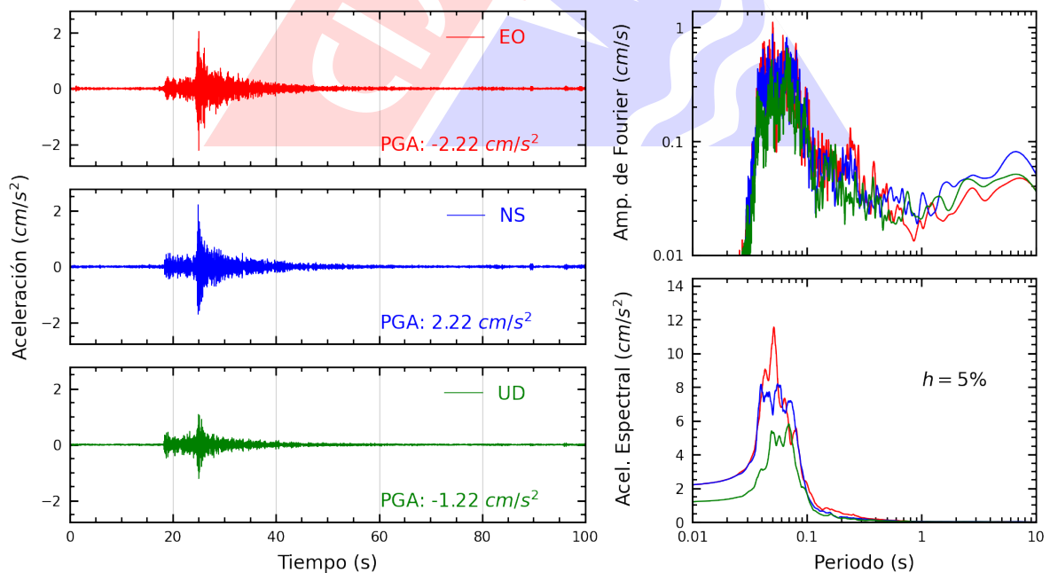
Figura A.10: Registros tiempo-historia, espectros de Fourier y de respuesta en las direcciones EO, NS y vertical de la estación CEPRE. Sismo de Lima, Lima - Lima del 2022-11-24, 05:56:59 (Hora local)
