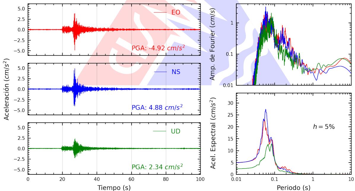
Figura A.2: Registros tiempo-historia, espectros de Fourier y de respuesta en las direcciones EO, NS y vertical de la estación USILM. Sismo de Lima, Lima - Lima del 2022-11-24, 05:56:59 (Hora local)
