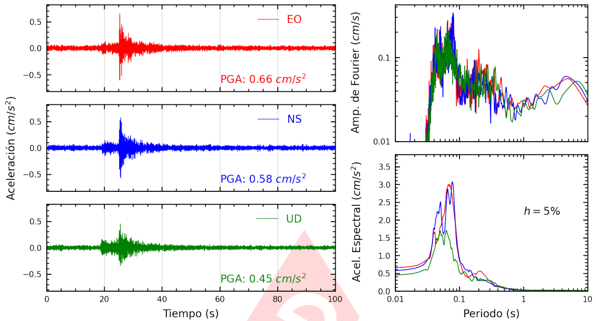
Figura A.33: Registros tiempo-historia, espectros de Fourier y de respuesta en las direcciones EO, NS y vertical de la estación BONDY. Sismo de Lima, Lima - Lima del 2022-11-24, 05:56:59 (Hora local)
