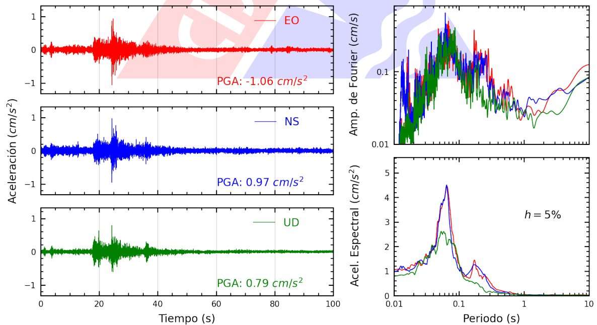
Figura A.24: Registros tiempo-historia, espectros de Fourier y de respuesta en las direcciones EO, NS y vertical de la estación NISTA. Sismo de Lima, Lima - Lima del 2022-11-24, 05:56:59 (Hora local)
