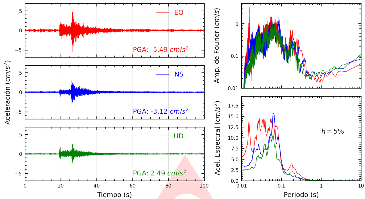
Figura A.1: Registros tiempo-historia, espectros de Fourier y de respuesta en las direcciones EO, NS y vertical de la estación INDEP. Sismo de Lima, Lima - Lima del 2022-11-24, 05:56:59 (Hora local)
