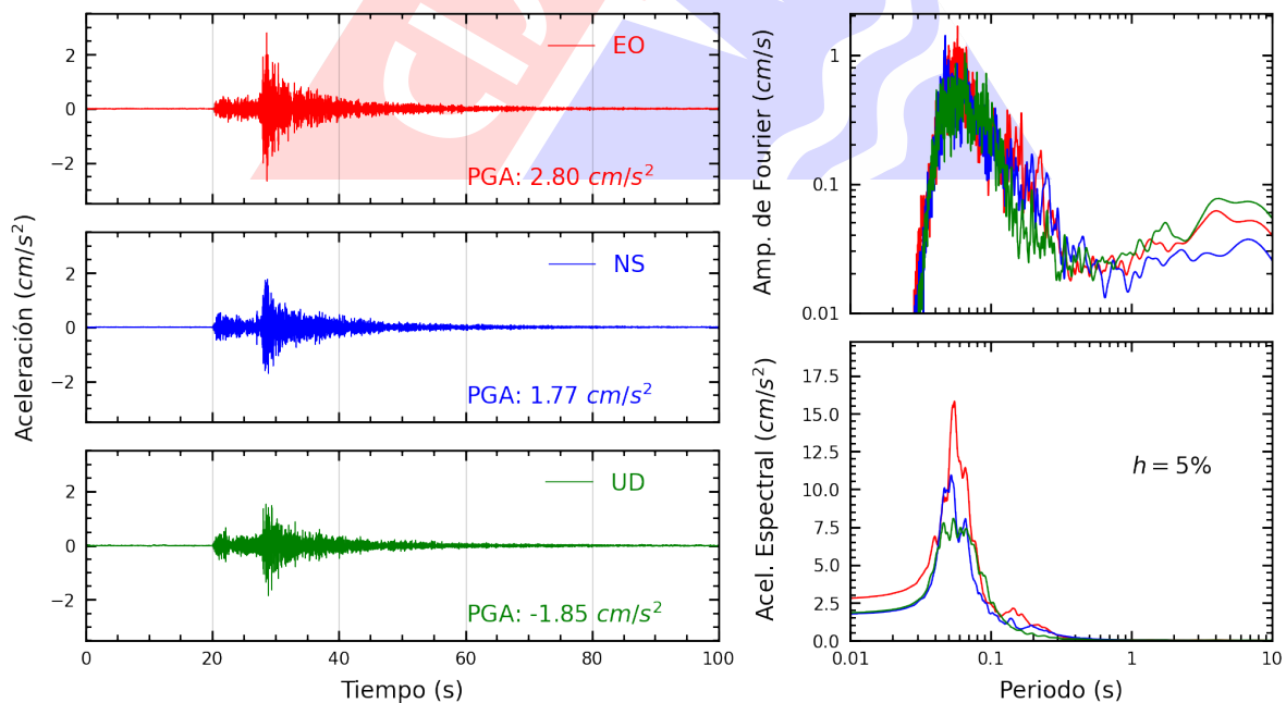
Figura A.4: Registros tiempo-historia, espectros de Fourier y de respuesta en las direcciones EO, NS y vertical de la estación AMORE. Sismo de Lima, Lima - Lima del 2022-11-24, 05:56:59 (Hora local)
