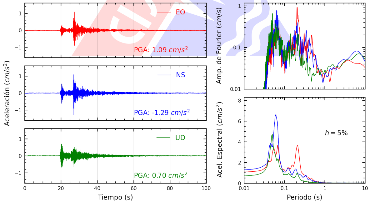
Figura A.18: Registros tiempo-historia, espectros de Fourier y de respuesta en las direcciones EO, NS y vertical de la estación VHAYA. Sismo de Lima, Lima - Lima del 2022-11-24, 05:56:59 (Hora local)
