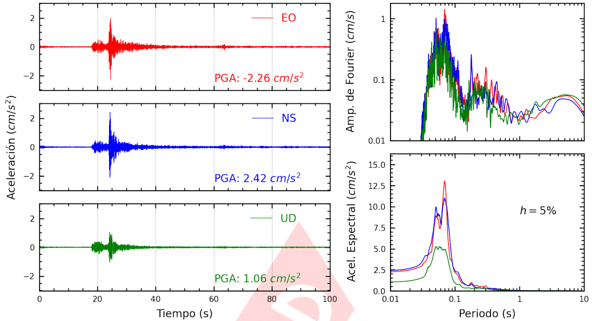
Figura A.5: Registros tiempo-historia, espectros de Fourier y de respuesta en las direcciones EO, NS y vertical de la estación UPCVI. Sismo de Lima, Lima - Lima del 2022-11-24, 05:56:59 (Hora local)
