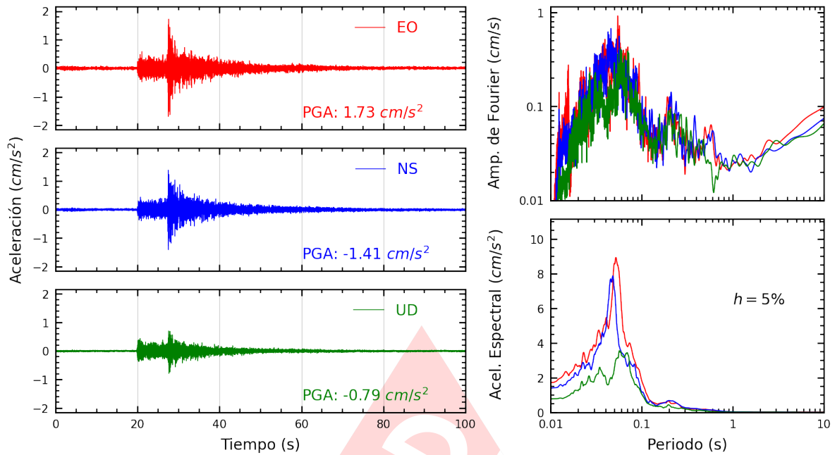
Figura A.13: Registros tiempo-historia, espectros de Fourier y de respuesta en las direcciones EO, NS y vertical de la estación COMAS. Sismo de Lima, Lima - Lima del 2022-11-24, 05:56:59 (Hora local)
