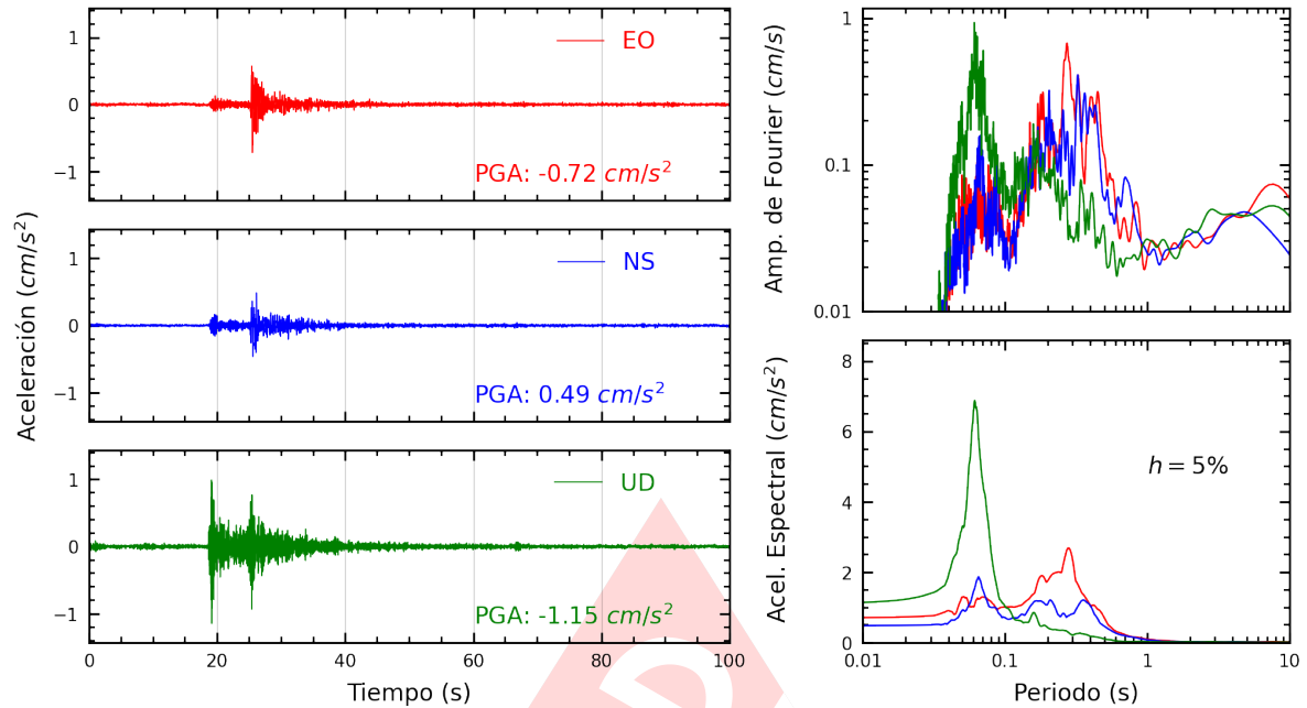
Figura A.23: Registros tiempo-historia, espectros de Fourier y de respuesta en las direcciones EO, NS y vertical de la estación ACAPU. Sismo de Lima, Lima - Lima del 2022-11-24, 05:56:59 (Hora local)
