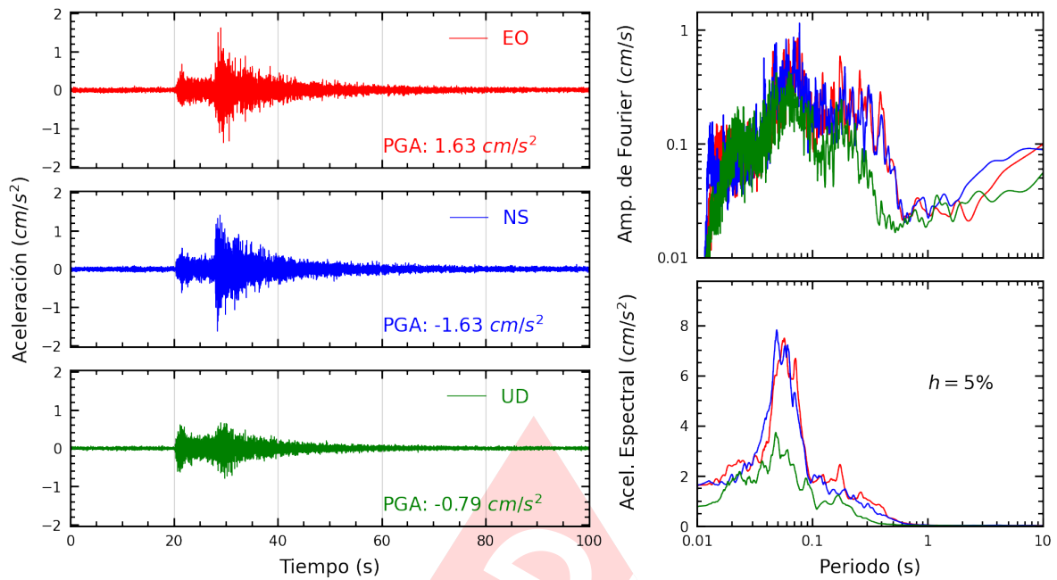
Figura A.15: Registros tiempo-historia, espectros de Fourier y de respuesta en las direcciones EO, NS y vertical de la estación DEFEN. Sismo de Lima, Lima - Lima del 2022-11-24, 05:56:59 (Hora local)
