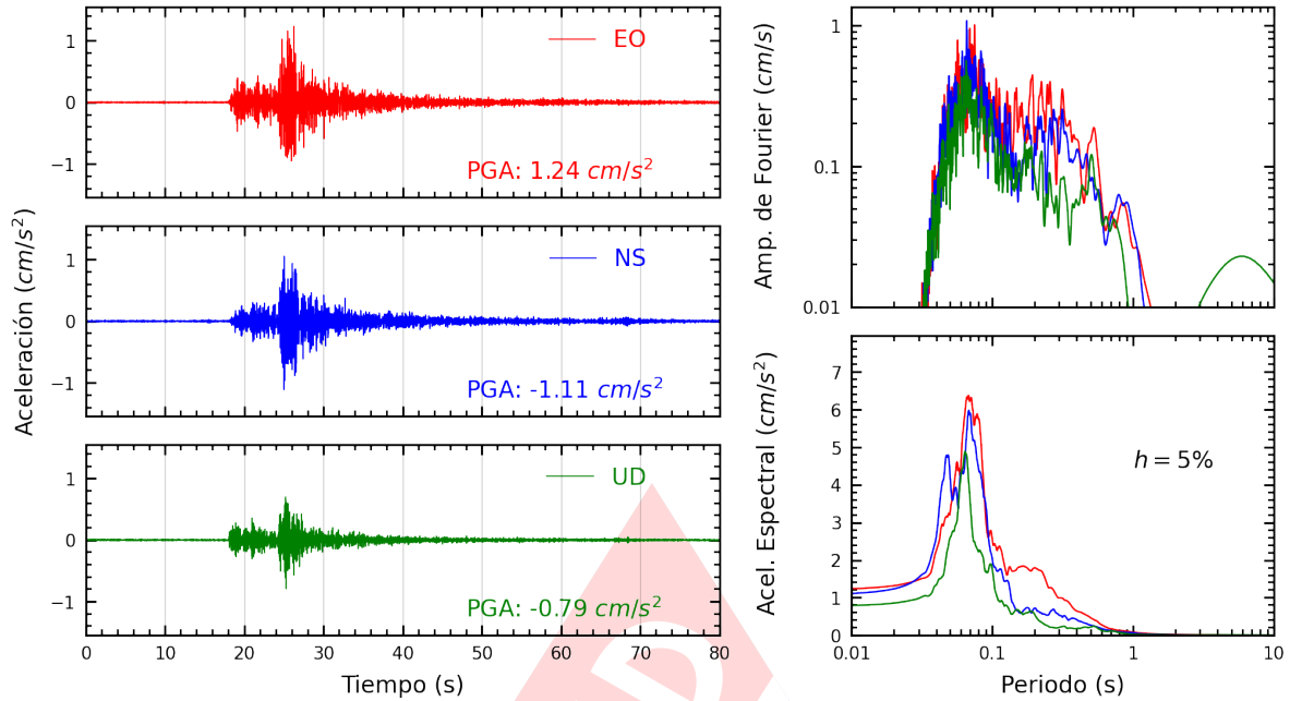
Figura A.19: Registros tiempo-historia, espectros de Fourier y de respuesta en las direcciones EO, NS y vertical de la estación BRISA. Sismo de Lima, Lima - Lima del 2022-11-24, 05:56:59 (Hora local)
