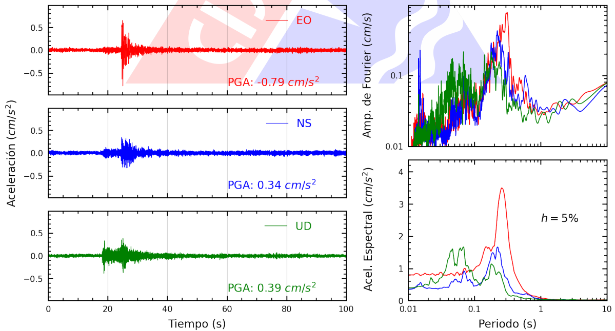
Figura A.32: Registros tiempo-historia, espectros de Fourier y de respuesta en las direcciones EO, NS y vertical de la estación DSMI. Sismo de Lima, Lima - Lima del 2022-11-24, 05:56:59 (Hora local)
