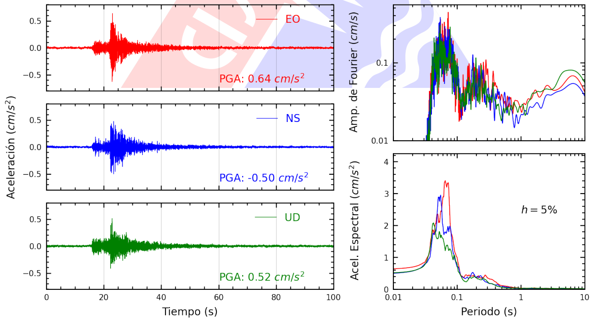
Figura A.34: Registros tiempo-historia, espectros de Fourier y de respuesta en las direcciones EO, NS y vertical de la estación UNMSM. Sismo de Lima, Lima - Lima del 2022-11-24, 05:56:59 (Hora local)
