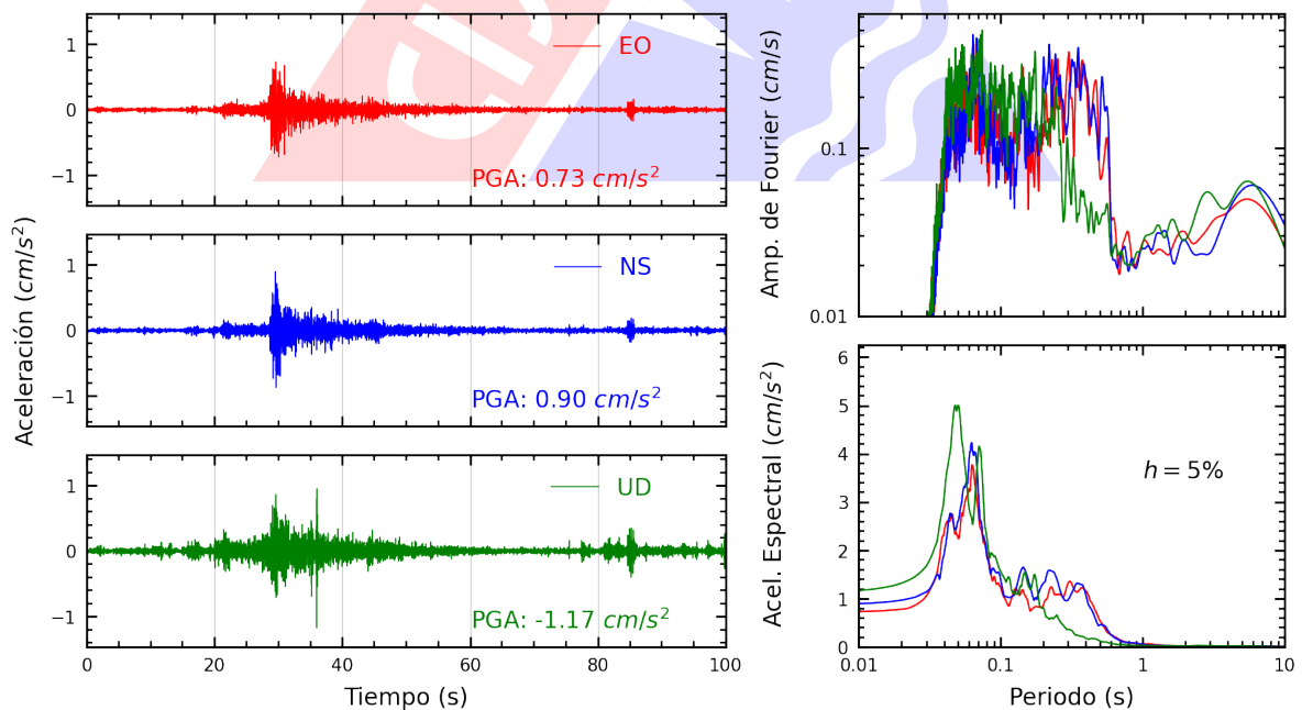
Figura A.22: Registros tiempo-historia, espectros de Fourier y de respuesta en las direcciones EO, NS y vertical de la estación MDPP. Sismo de Lima, Lima - Lima del 2022-11-24, 05:56:59 (Hora local)
