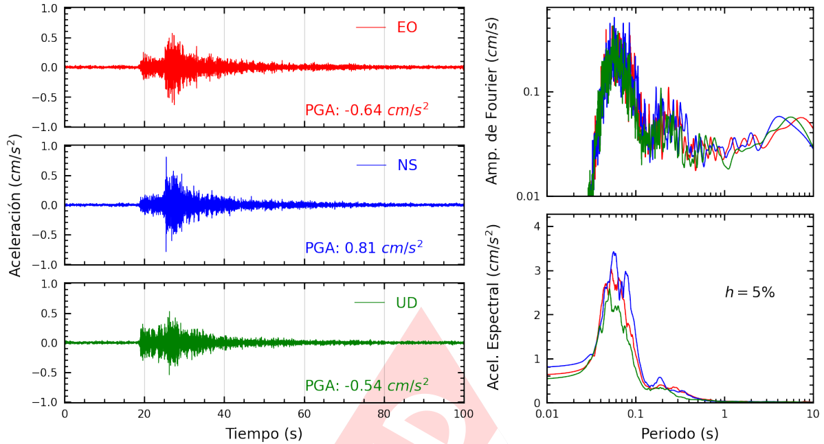
Figura A.31: Registros tiempo-historia, espectros de Fourier y de respuesta en las direcciones EO, NS y vertical de la estación CENEP. Sismo de Lima, Lima - Lima del 2022-11-24, 05:56:59 (Hora local)
