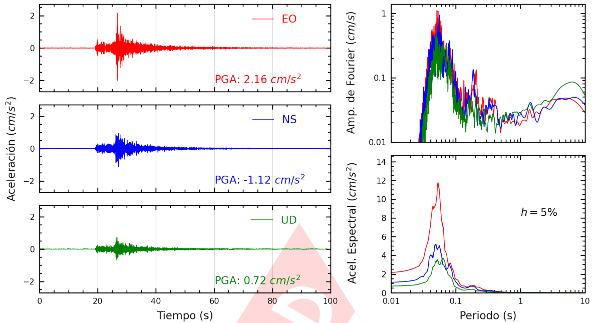
Figura A.11: Registros tiempo-historia, espectros de Fourier y de respuesta en las direcciones EO, NS y vertical de la estación UCSS. Sismo de Lima, Lima - Lima del 2022-11-24, 05:56:59 (Hora local)
