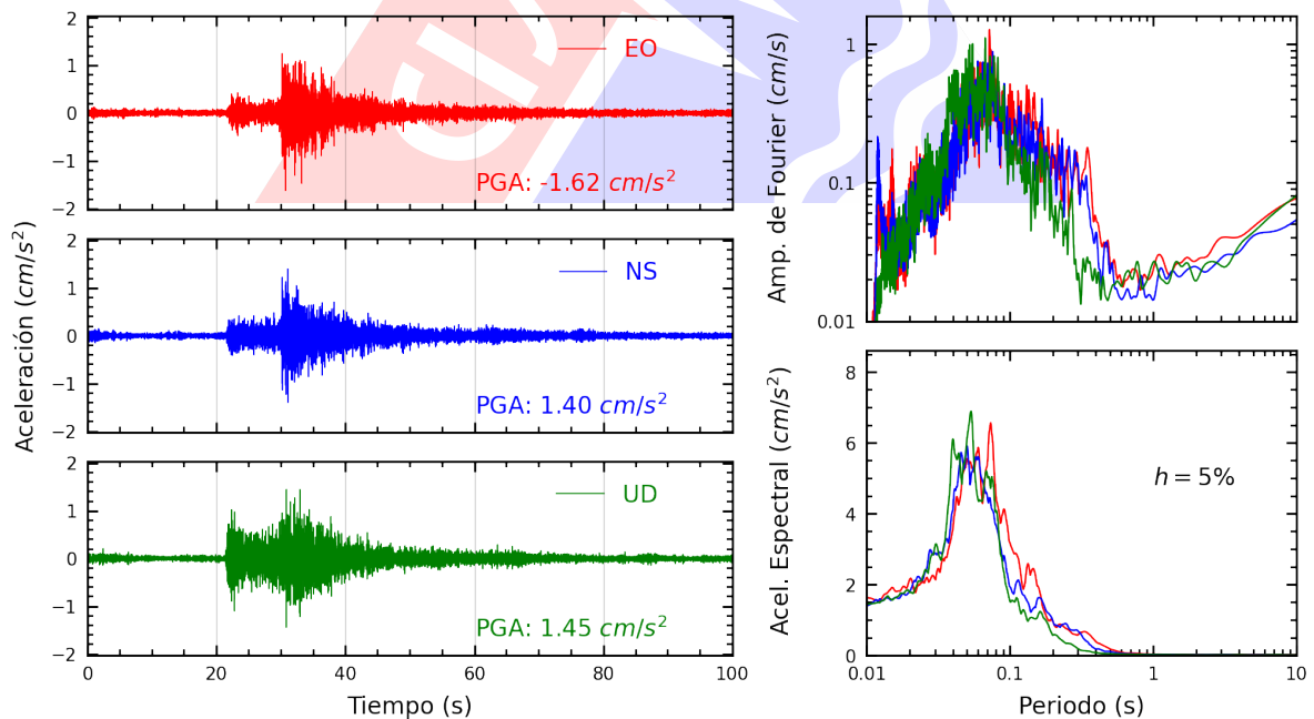
Figura A.16: Registros tiempo-historia, espectros de Fourier y de respuesta en las direcciones EO, NS y vertical de la estación ANCON. Sismo de Lima, Lima - Lima del 2022-11-24, 05:56:59 (Hora local)
