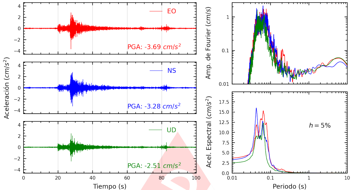
Figura A.3: Registros tiempo-historia, espectros de Fourier y de respuesta en las direcciones EO, NS y vertical de la estación JOSEO. Sismo de Lima, Lima - Lima del 2022-11-24, 05:56:59 (Hora local)
