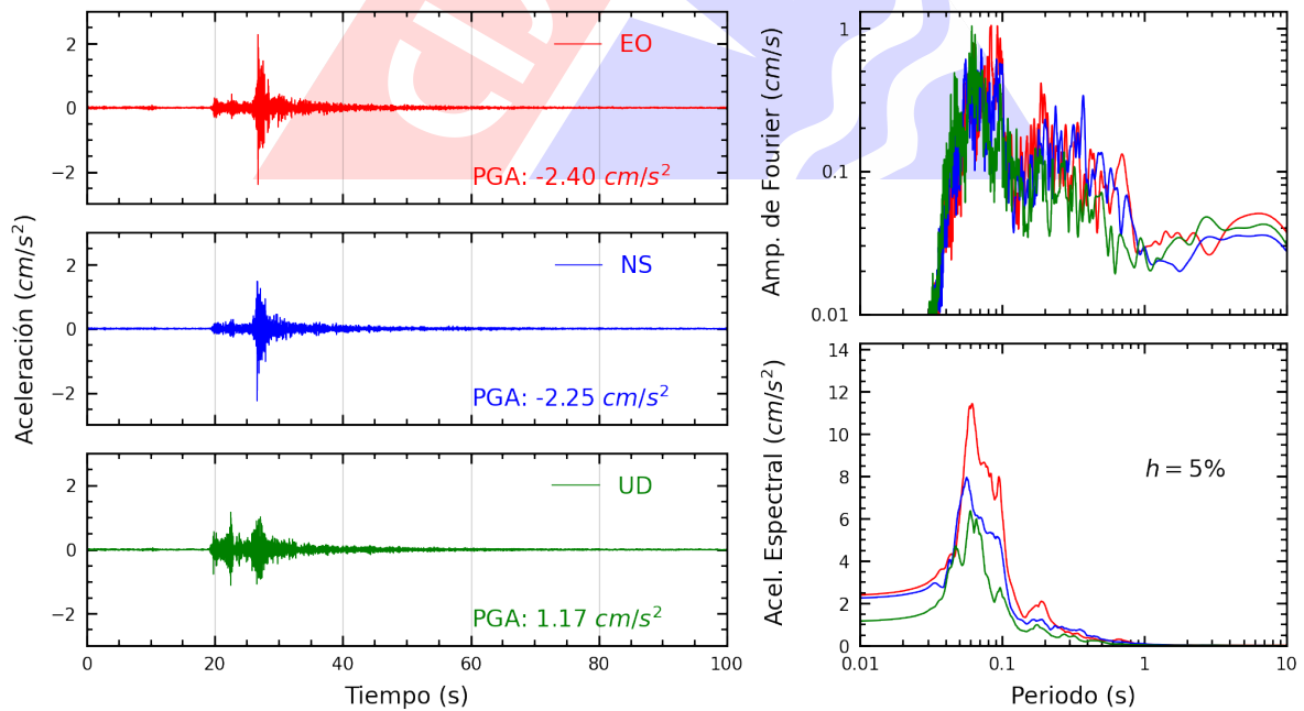
Figura A.6: Registros tiempo-historia, espectros de Fourier y de respuesta en las direcciones EO, NS y vertical de la estación USILP. Sismo de Lima, Lima - Lima del 2022-11-24, 05:56:59 (Hora local)
