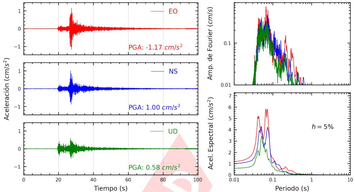
Figura A.21: Registros tiempo-historia, espectros de Fourier y de respuesta en las direcciones EO, NS y vertical de la estación ATARJ. Sismo de Lima, Lima - Lima del 2022-11-24, 05:56:59 (Hora local)
