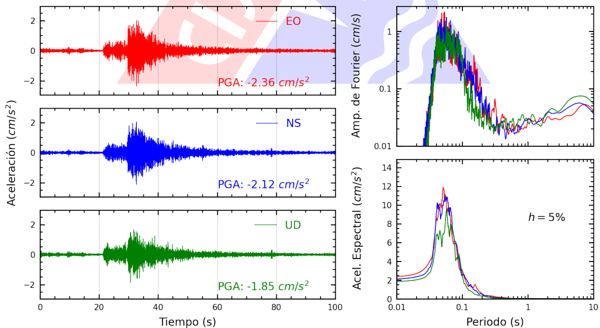
Figura A.8: Registros tiempo-historia, espectros de Fourier y de respuesta en las direcciones EO, NS y vertical de la estación SROSA. Sismo de Lima, Lima - Lima del 2022-11-24, 05:56:59 (Hora local)
