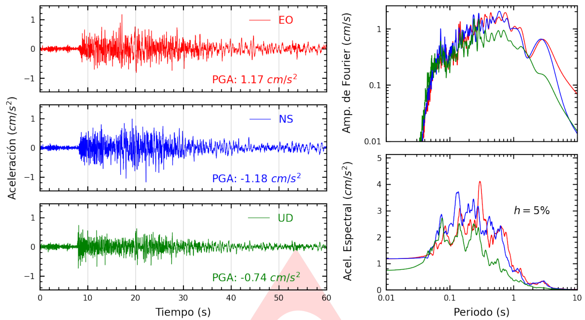
Figura A.1: Registros tiempo-historia, espectros de Fourier y de respuesta en las direcciones EO, NS y vertical de la estación UNAJ. Sismo de Santa Lucia, Lampa - Puno del 2021-08-27, 16:00:15 (Hora local)
