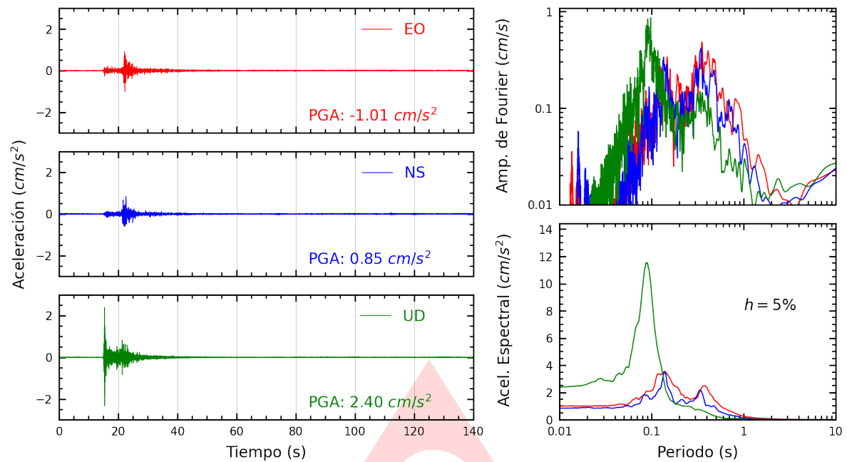
Figura A.1: Registros tiempo-historia, espectros de Fourier y de respuesta en las direcciones EO, NS y vertical de la estación UNIPE. Sismo de Sullana, Sullana - Piura del 2022-12-02, 03:19:25 (Hora local)
