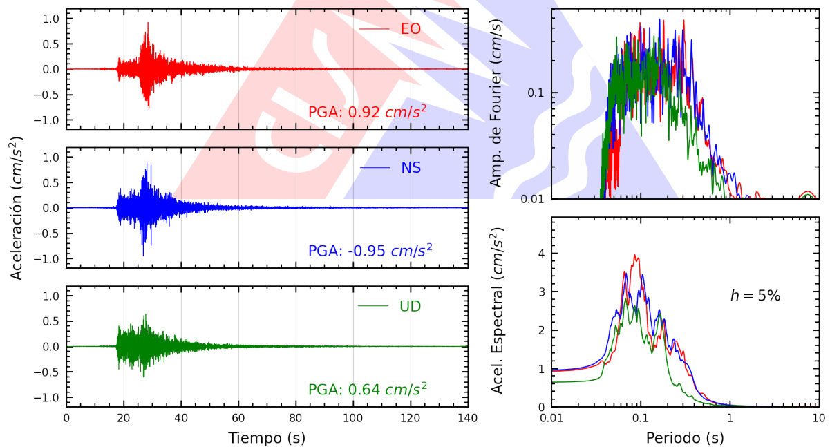
Figura A.2: Registros tiempo-historia, espectros de Fourier y de respuesta en las direcciones EO, NS y vertical de la estación UPAOP. Sismo de Sullana, Sullana - Piura del 2022-12-02, 03:19:25 (Hora local)
