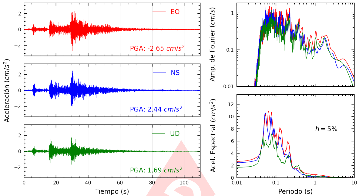
Figura A.31: Registros tiempo-historia, espectros de Fourier y de respuesta en las direcciones EO, NS y vertical de la estación PACHA. Sismo de Canta, Canta - Lima del 2022-12-15, 04:31:16 (Hora local)
