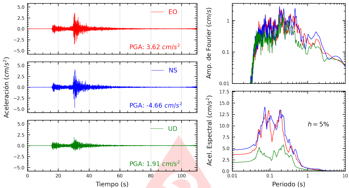
Figura A.15: Registros tiempo-historia, espectros de Fourier y de respuesta en las direcciones EO, NS y vertical de la estación UPCVI. Sismo de Canta, Canta - Lima del 2022-12-15, 04:31:16 (Hora local)
