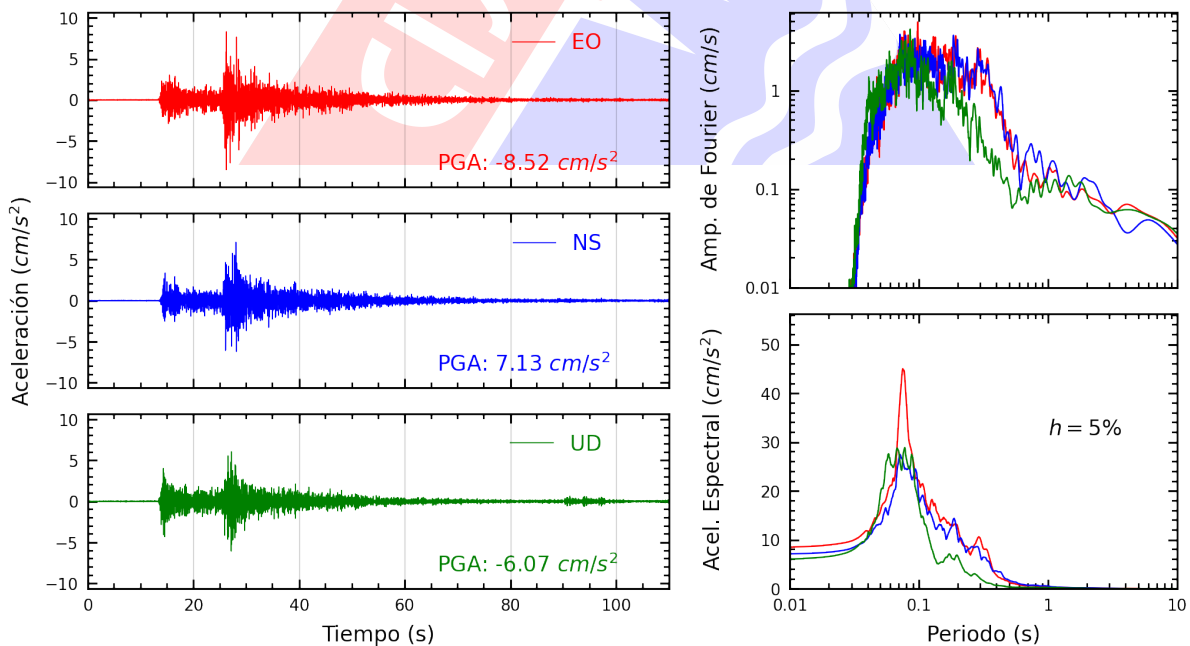
Figura A.6: Registros tiempo-historia, espectros de Fourier y de respuesta en las direcciones EO, NS y vertical de la estación ANCON. Sismo de Canta, Canta - Lima del 2022-12-15, 04:31:16 (Hora local)
