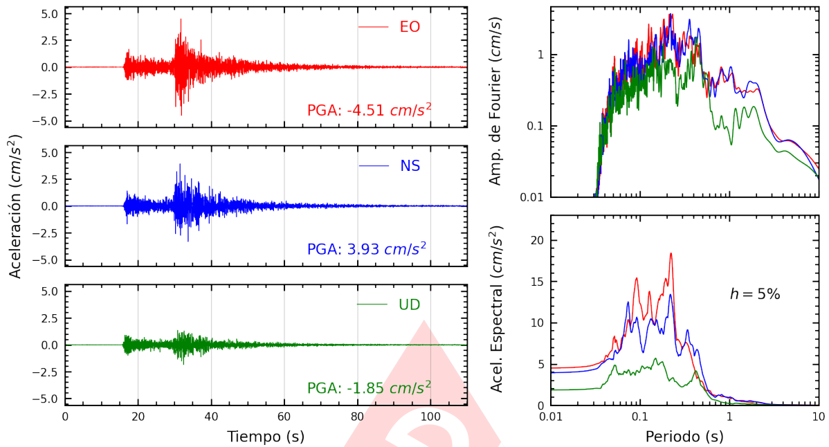
Figura A.17: Registros tiempo-historia, espectros de Fourier y de respuesta en las direcciones EO, NS y vertical de la estación BRISA. Sismo de Canta, Canta - Lima del 2022-12-15, 04:31:16 (Hora local)
