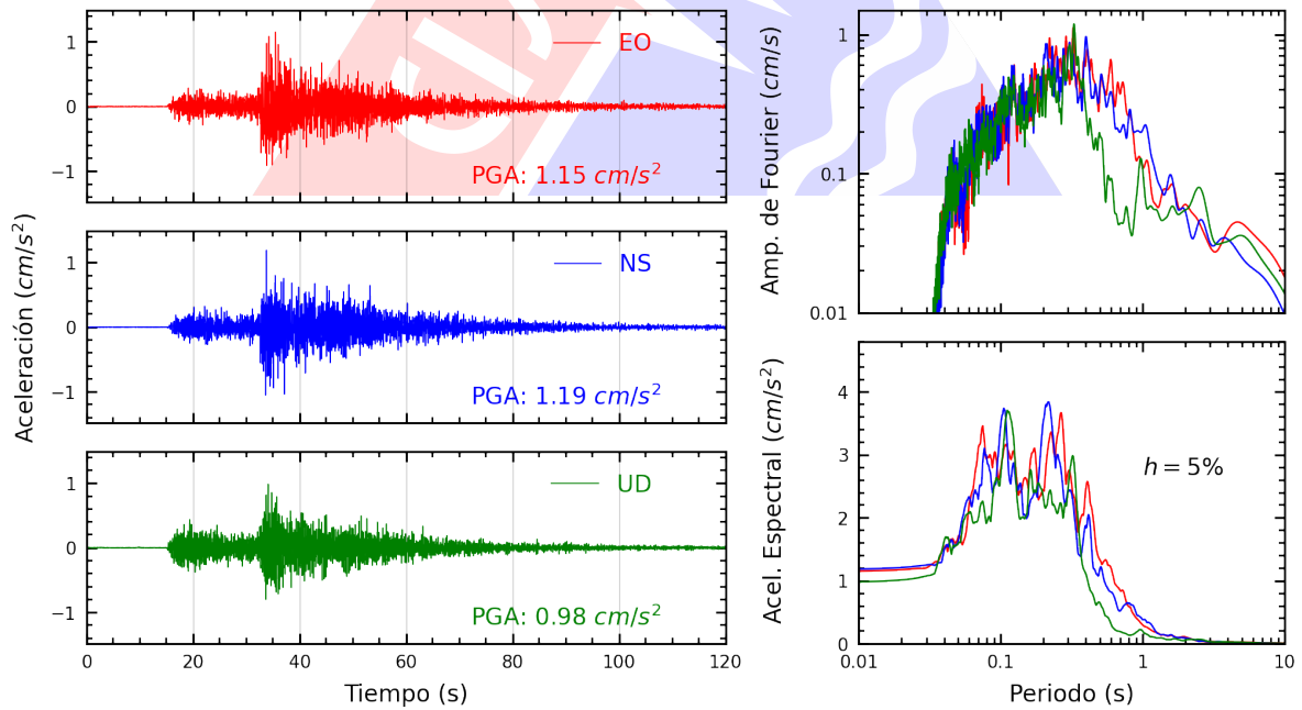
Figura A.34: Registros tiempo-historia, espectros de Fourier y de respuesta en las direcciones EO, NS y vertical de la estación CARAL. Sismo de Canta, Canta - Lima del 2022-12-15, 04:31:16 (Hora local)
