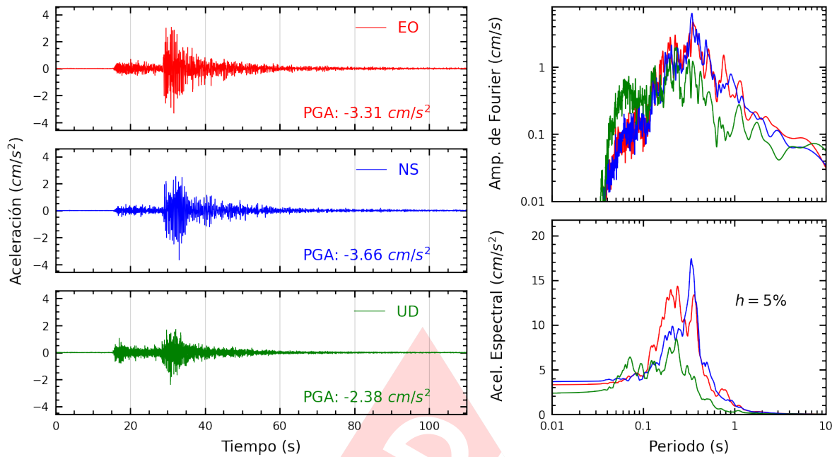
Figura A.25: Registros tiempo-historia, espectros de Fourier y de respuesta en las direcciones EO, NS y vertical de la estación ACAPU. Sismo de Canta, Canta - Lima del 2022-12-15, 04:31:16 (Hora local)
