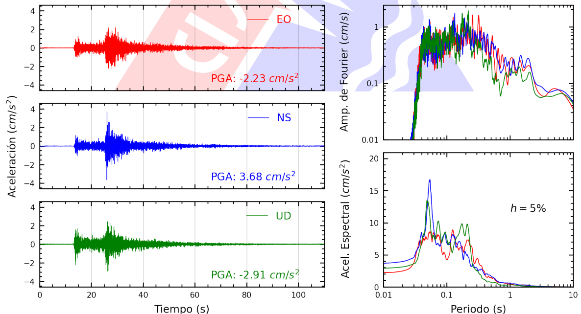
Figura A.24: Registros tiempo-historia, espectros de Fourier y de respuesta en las direcciones EO, NS y vertical de la estación USMP. Sismo de Canta, Canta - Lima del 2022-12-15, 04:31:16 (Hora local)
