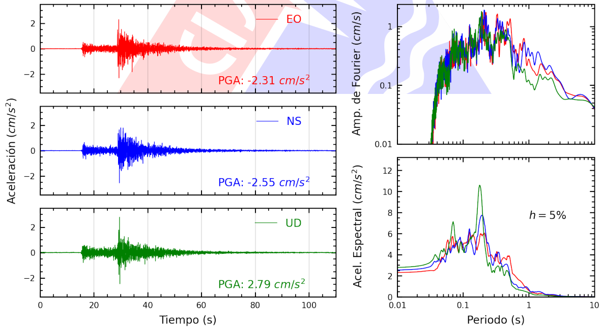
Figura A.30: Registros tiempo-historia, espectros de Fourier y de respuesta en las direcciones EO, NS y vertical de la estación UNFV. Sismo de Canta, Canta - Lima del 2022-12-15, 04:31:16 (Hora local)
