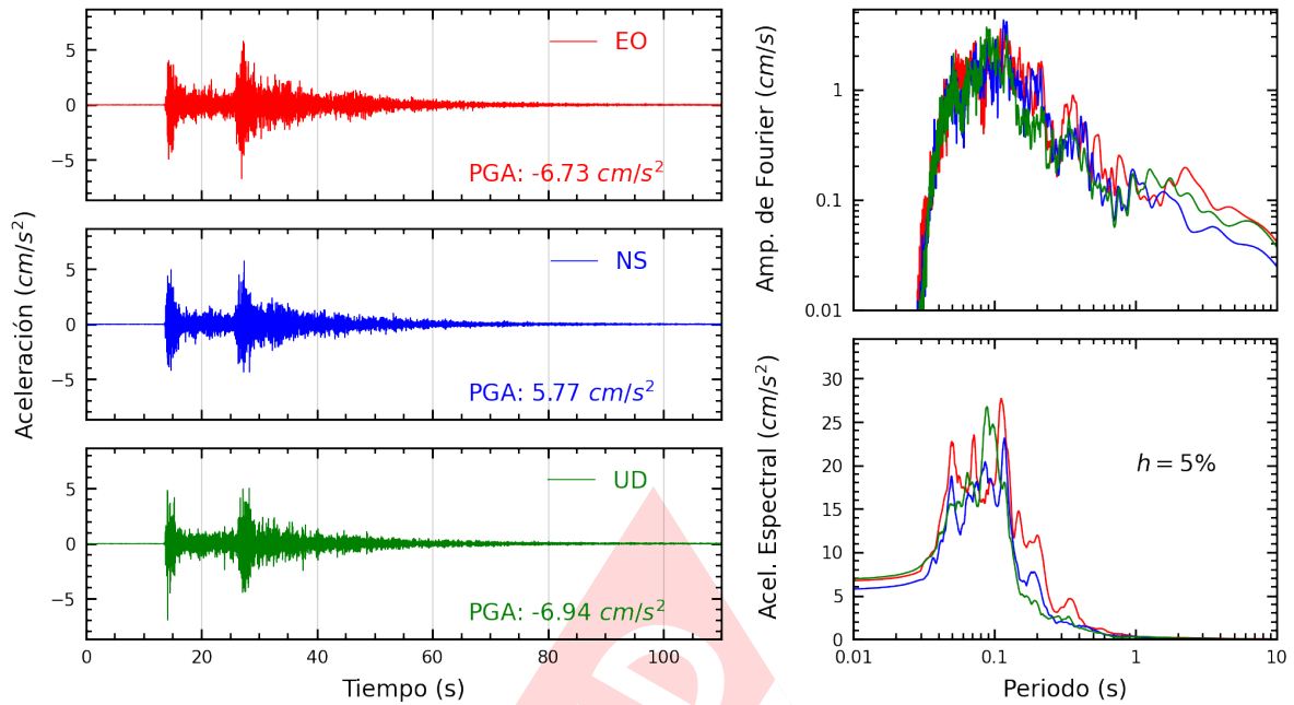
Figura A.7: Registros tiempo-historia, espectros de Fourier y de respuesta en las direcciones EO, NS y vertical de la estación AMORE. Sismo de Canta, Canta - Lima del 2022-12-15, 04:31:16 (Hora local)
