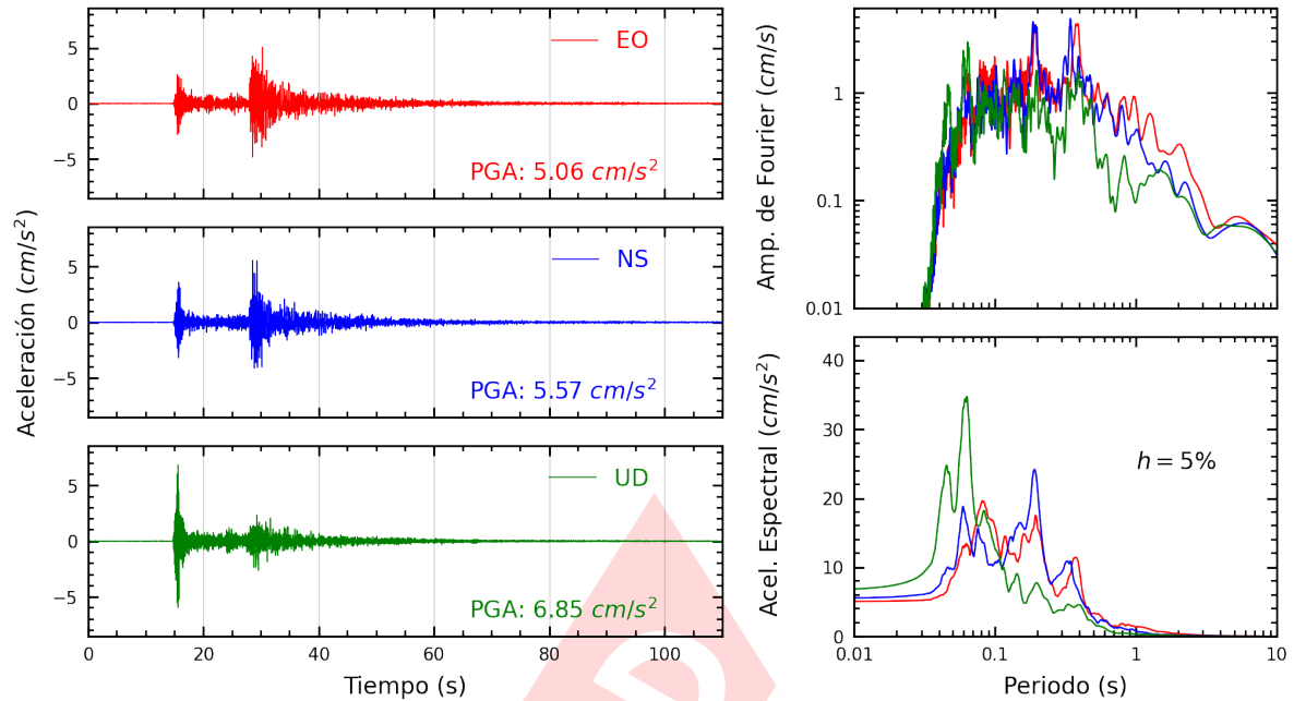
Figura A.9: Registros tiempo-historia, espectros de Fourier y de respuesta en las direcciones EO, NS y vertical de la estación USILP. Sismo de Canta, Canta - Lima del 2022-12-15, 04:31:16 (Hora local)
