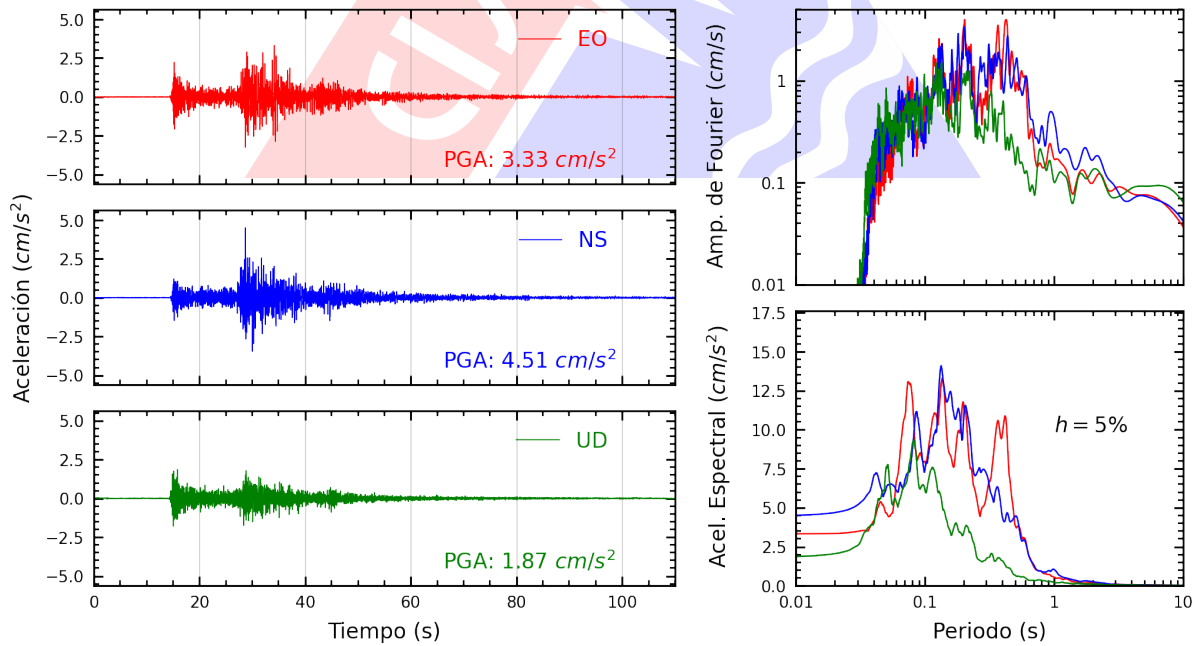
Figura A.18: Registros tiempo-historia, espectros de Fourier y de respuesta en las direcciones EO, NS y vertical de la estación VHAYA. Sismo de Canta, Canta - Lima del 2022-12-15, 04:31:16 (Hora local)
