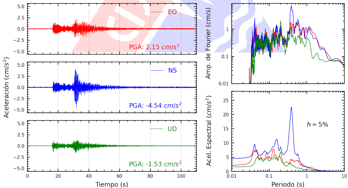
Figura A.16: Registros tiempo-historia, espectros de Fourier y de respuesta en las direcciones EO, NS y vertical de la estación DHNPE. Sismo de Canta, Canta - Lima del 2022-12-15, 04:31:16 (Hora local)
