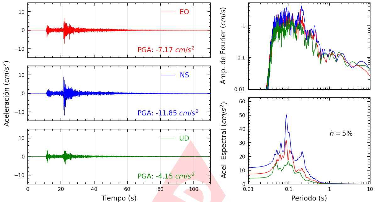
Figura A.3: Registros tiempo-historia, espectros de Fourier y de respuesta en las direcciones EO, NS y vertical de la estación IPEN. Sismo de Canta, Canta - Lima del 2022-12-15, 04:31:16 (Hora local)
