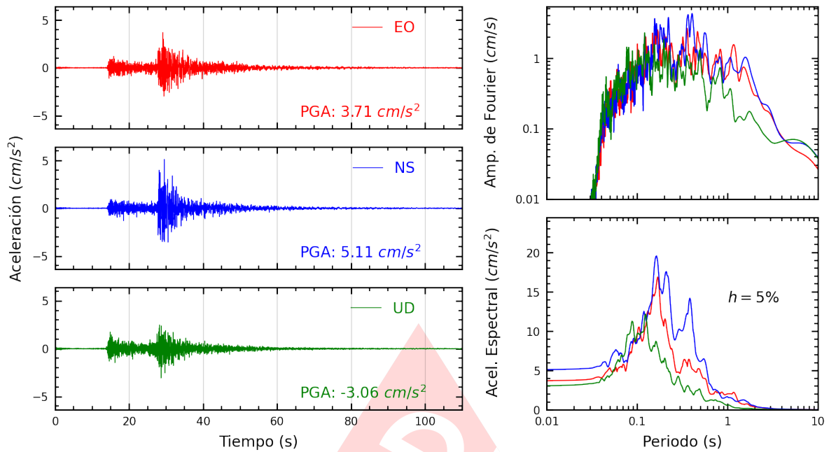
Figura A.13: Registros tiempo-historia, espectros de Fourier y de respuesta en las direcciones EO, NS y vertical de la estación PRADO. Sismo de Canta, Canta - Lima del 2022-12-15, 04:31:16 (Hora local)
