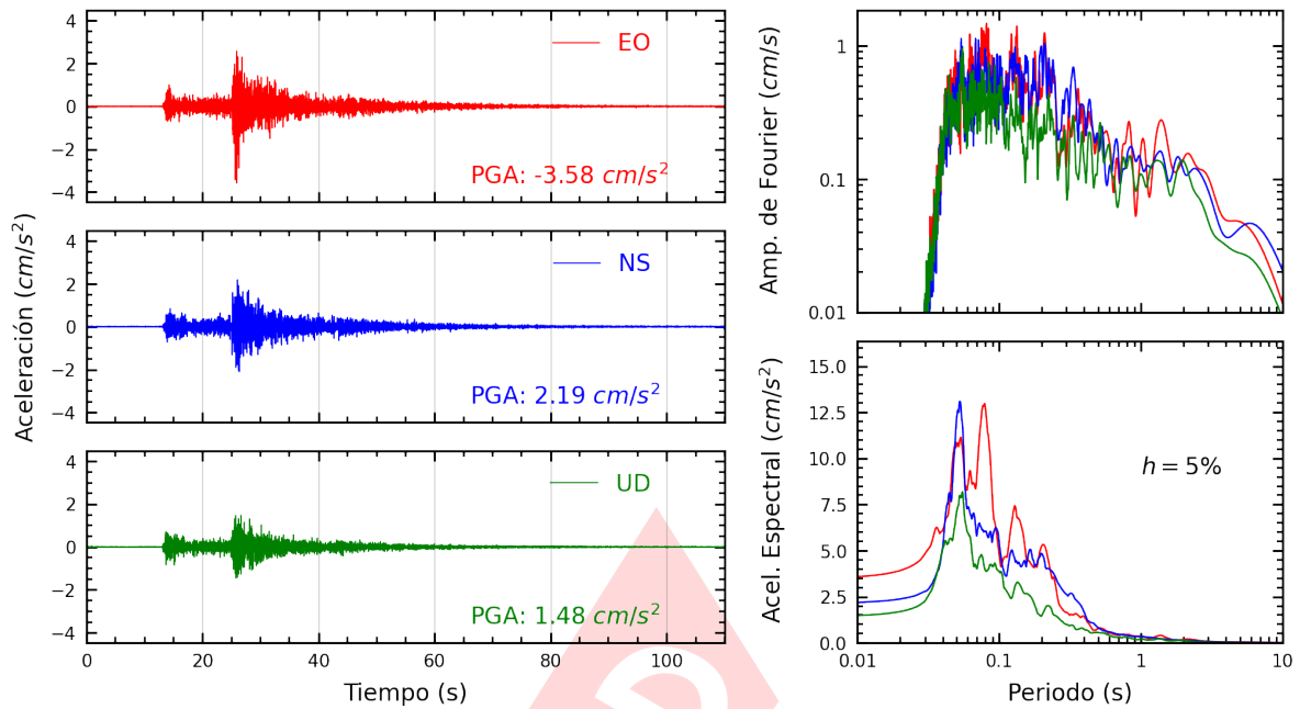
Figura A.27: Registros tiempo-historia, espectros de Fourier y de respuesta en las direcciones EO, NS y vertical de la estación ATARJ. Sismo de Canta, Canta - Lima del 2022-12-15, 04:31:16 (Hora local)
