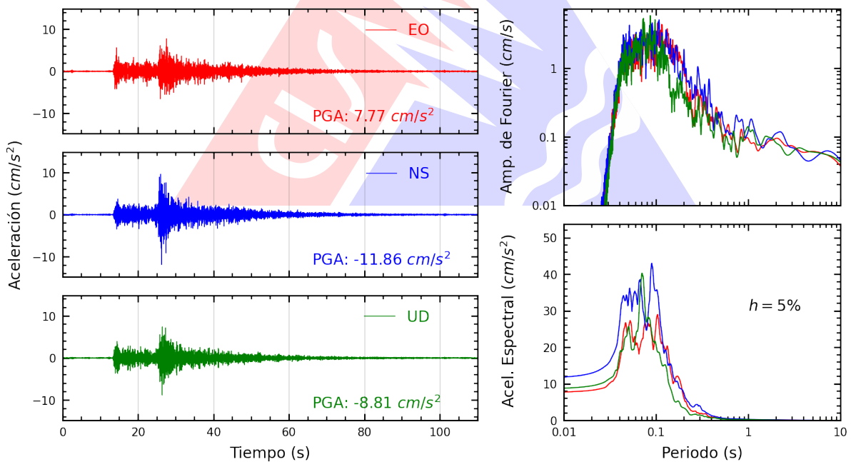
Figura A.2: Registros tiempo-historia, espectros de Fourier y de respuesta en las direcciones EO, NS y vertical de la estación SROSA. Sismo de Canta, Canta - Lima del 2022-12-15, 04:31:16 (Hora local)
