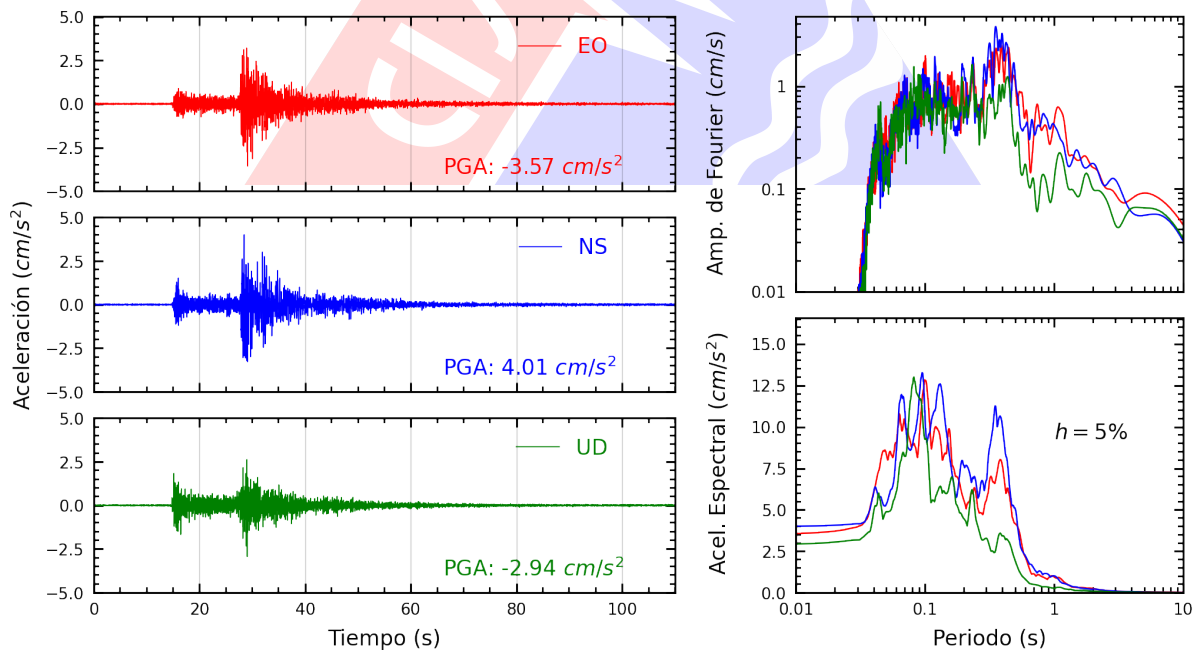
Figura A.22: Registros tiempo-historia, espectros de Fourier y de respuesta en las direcciones EO, NS y vertical de la estación MADRE. Sismo de Canta, Canta - Lima del 2022-12-15, 04:31:16 (Hora local)
