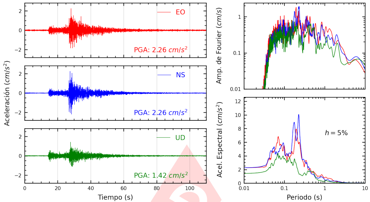
Figura A.33: Registros tiempo-historia, espectros de Fourier y de respuesta en las direcciones EO, NS y vertical de la estación INICT. Sismo de Canta, Canta - Lima del 2022-12-15, 04:31:16 (Hora local)
