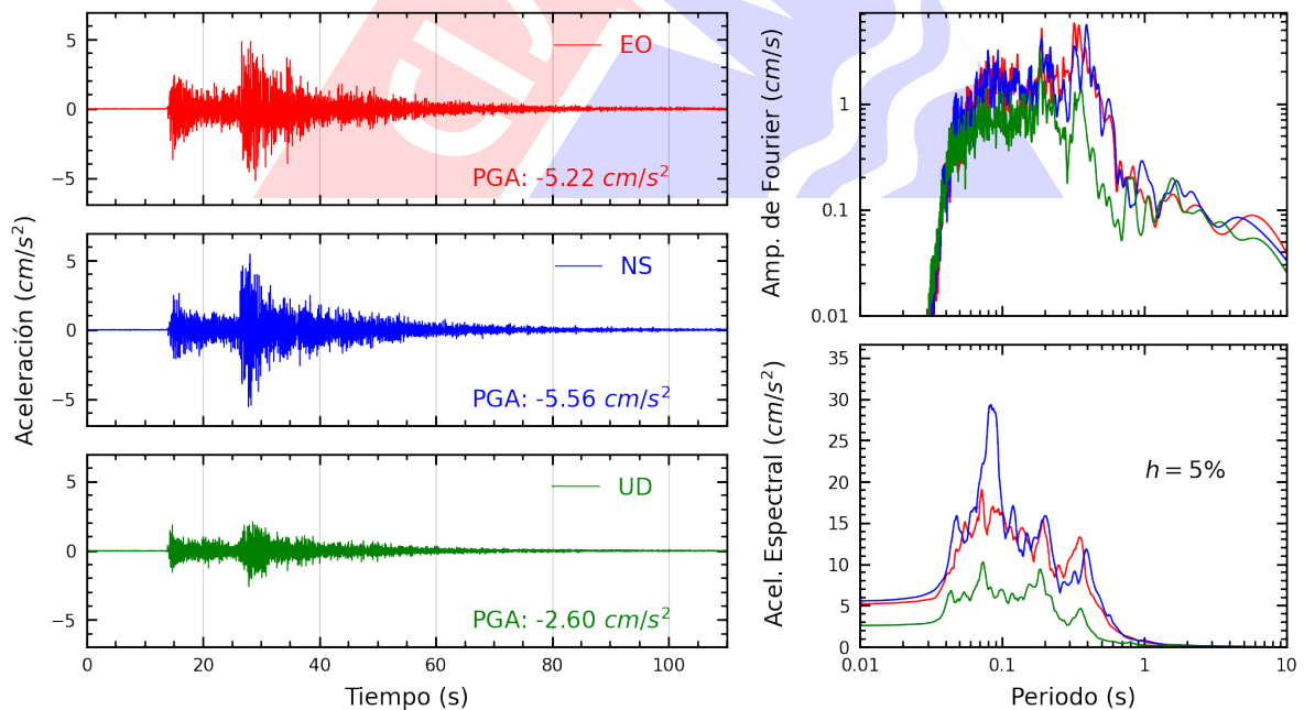
Figura A.12: Registros tiempo-historia, espectros de Fourier y de respuesta en las direcciones EO, NS y vertical de la estación DEFEN. Sismo de Canta, Canta - Lima del 2022-12-15, 04:31:16 (Hora local)
