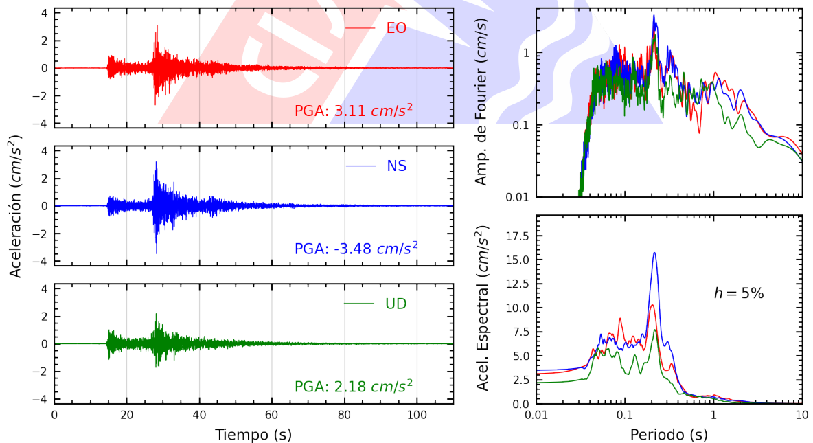
Figura A.28: Registros tiempo-historia, espectros de Fourier y de respuesta en las direcciones EO, NS y vertical de la estación CENEP. Sismo de Canta, Canta - Lima del 2022-12-15, 04:31:16 (Hora local)
