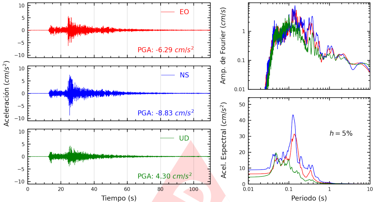
Figura A.5: Registros tiempo-historia, espectros de Fourier y de respuesta en las direcciones EO, NS y vertical de la estación CARAB. Sismo de Canta, Canta - Lima del 2022-12-15, 04:31:16 (Hora local)
