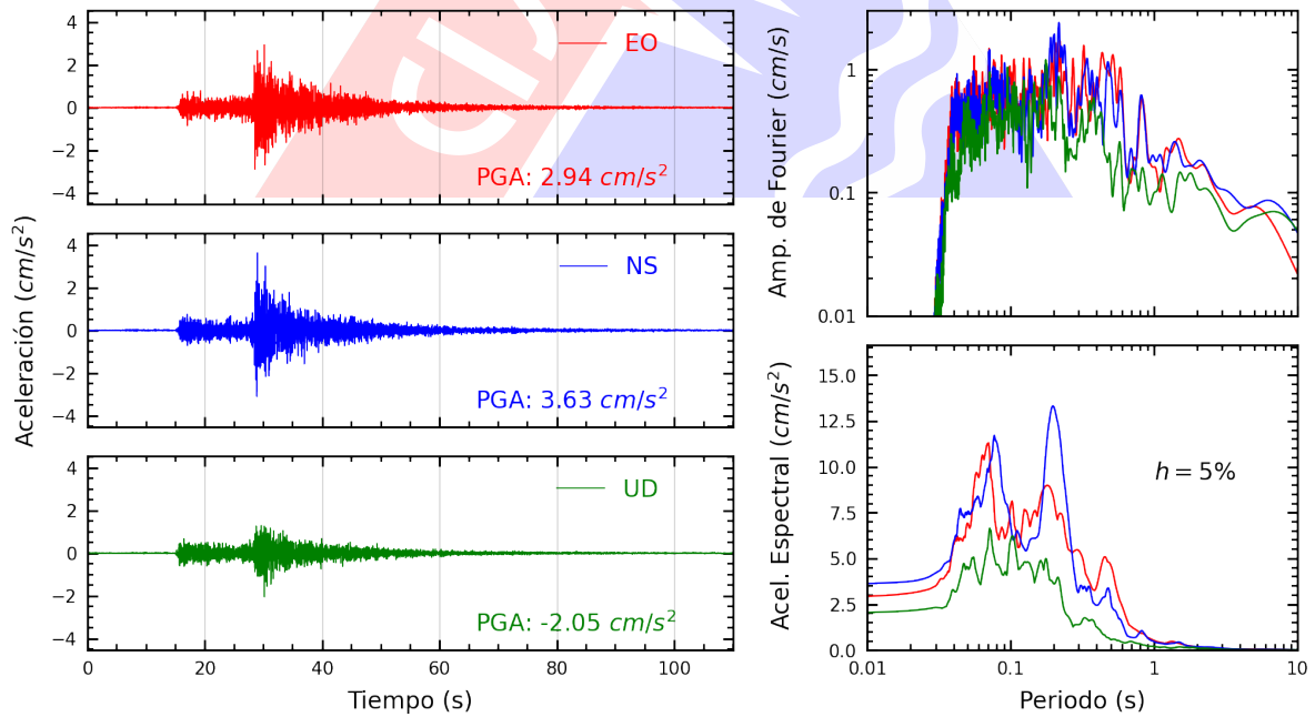
Figura A.26: Registros tiempo-historia, espectros de Fourier y de respuesta en las direcciones EO, NS y vertical de la estación CEPRE. Sismo de Canta, Canta - Lima del 2022-12-15, 04:31:16 (Hora local)
