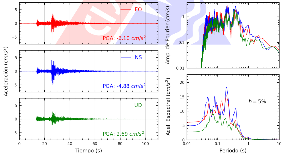
Figura A.10: Registros tiempo-historia, espectros de Fourier y de respuesta en las direcciones EO, NS y vertical de la estación COMAS. Sismo de Canta, Canta - Lima del 2022-12-15, 04:31:16 (Hora local)
