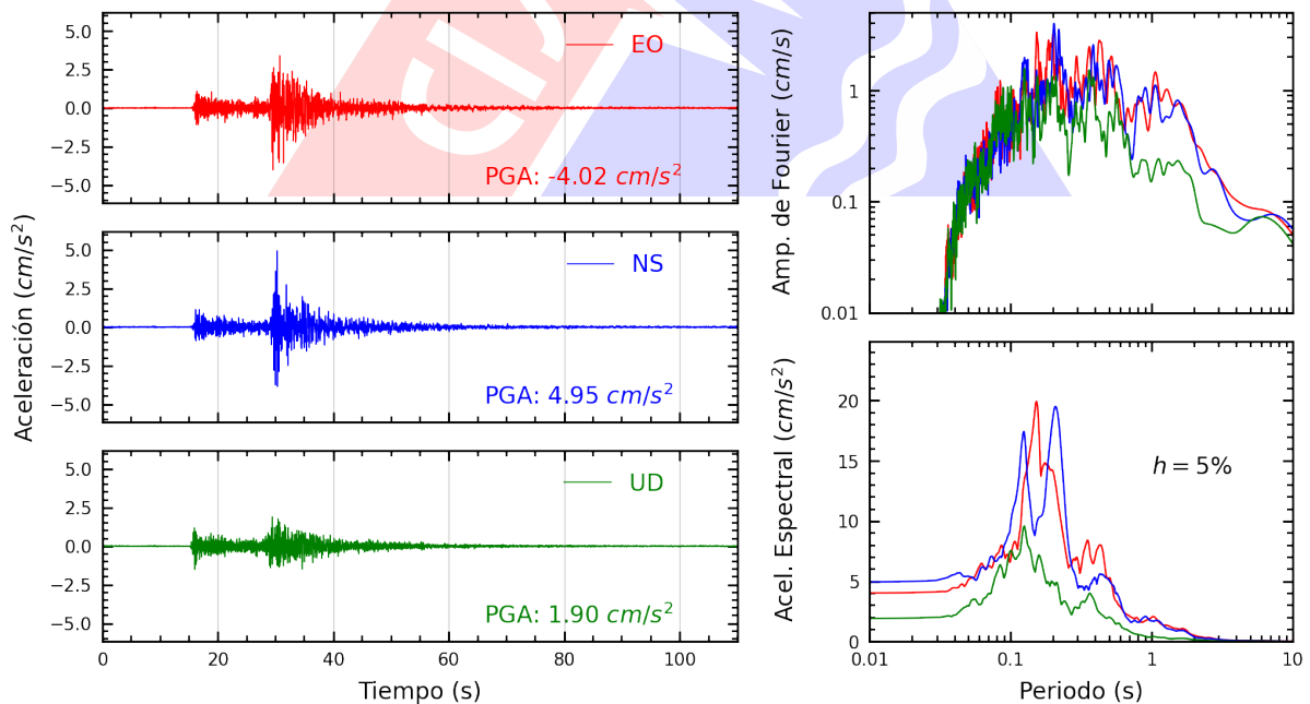
Figura A.14: Registros tiempo-historia, espectros de Fourier y de respuesta en las direcciones EO, NS y vertical de la estación NISTA. Sismo de Canta, Canta - Lima del 2022-12-15, 04:31:16 (Hora local)
