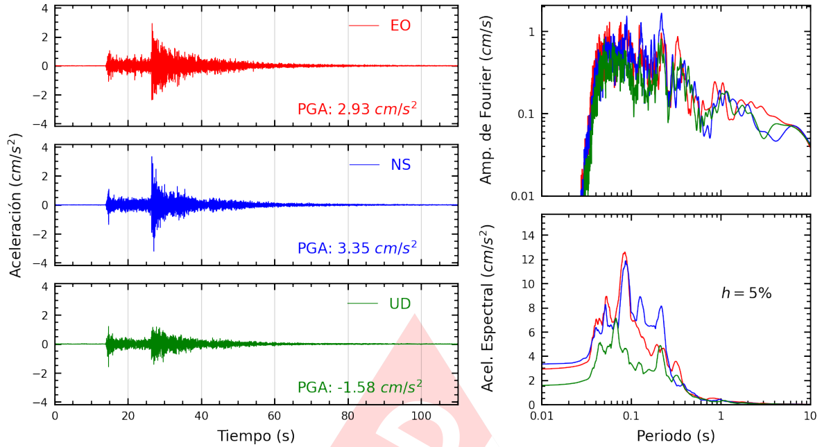
Figura A.29: Registros tiempo-historia, espectros de Fourier y de respuesta en las direcciones EO, NS y vertical de la estación UCSS. Sismo de Canta, Canta - Lima del 2022-12-15, 04:31:16 (Hora local)
