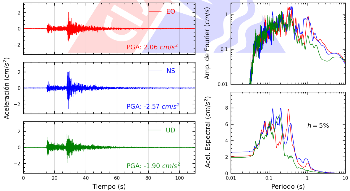
Figura A.32: Registros tiempo-historia, espectros de Fourier y de respuesta en las direcciones EO, NS y vertical de la estación BONDY. Sismo de Canta, Canta - Lima del 2022-12-15, 04:31:16 (Hora local)
