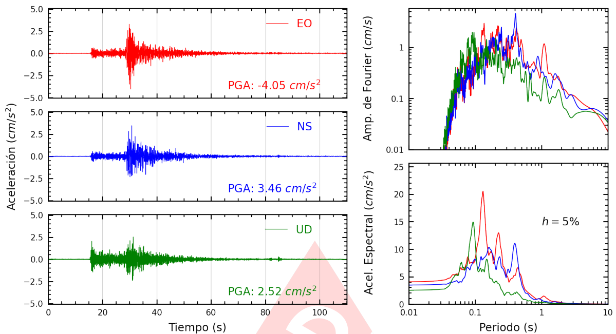
Figura A.21: Registros tiempo-historia, espectros de Fourier y de respuesta en las direcciones EO, NS y vertical de la estación RAMON. Sismo de Canta, Canta - Lima del 2022-12-15, 04:31:16 (Hora local)
