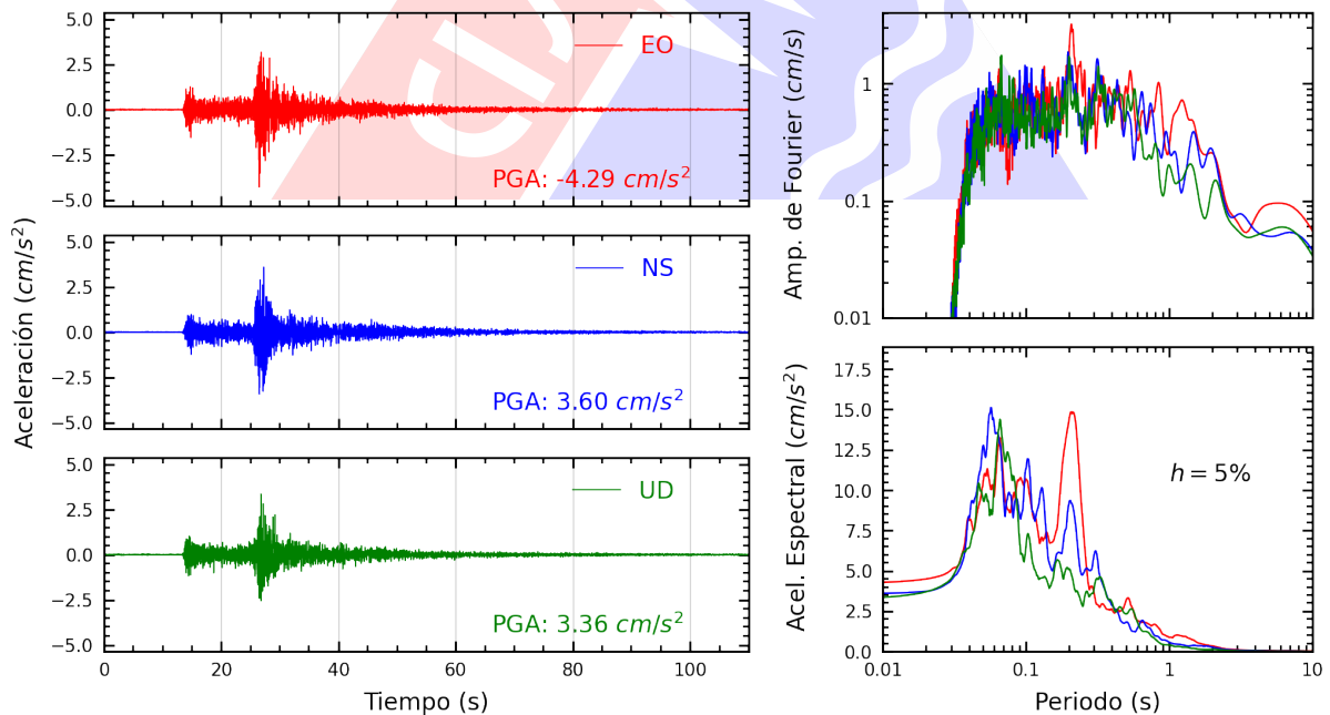
Figura A.20: Registros tiempo-historia, espectros de Fourier y de respuesta en las direcciones EO, NS y vertical de la estación IMCA. Sismo de Canta, Canta - Lima del 2022-12-15, 04:31:16 (Hora local)
