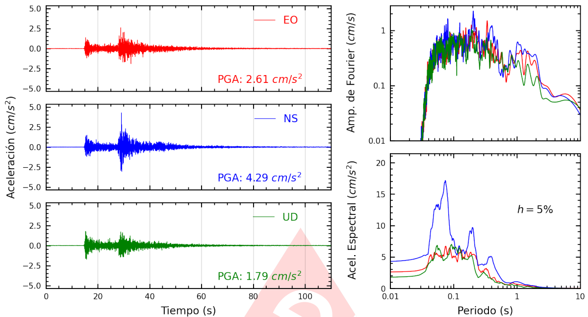
Figura A.19: Registros tiempo-historia, espectros de Fourier y de respuesta en las direcciones EO, NS y vertical de la estación SERVI. Sismo de Canta, Canta - Lima del 2022-12-15, 04:31:16 (Hora local)
