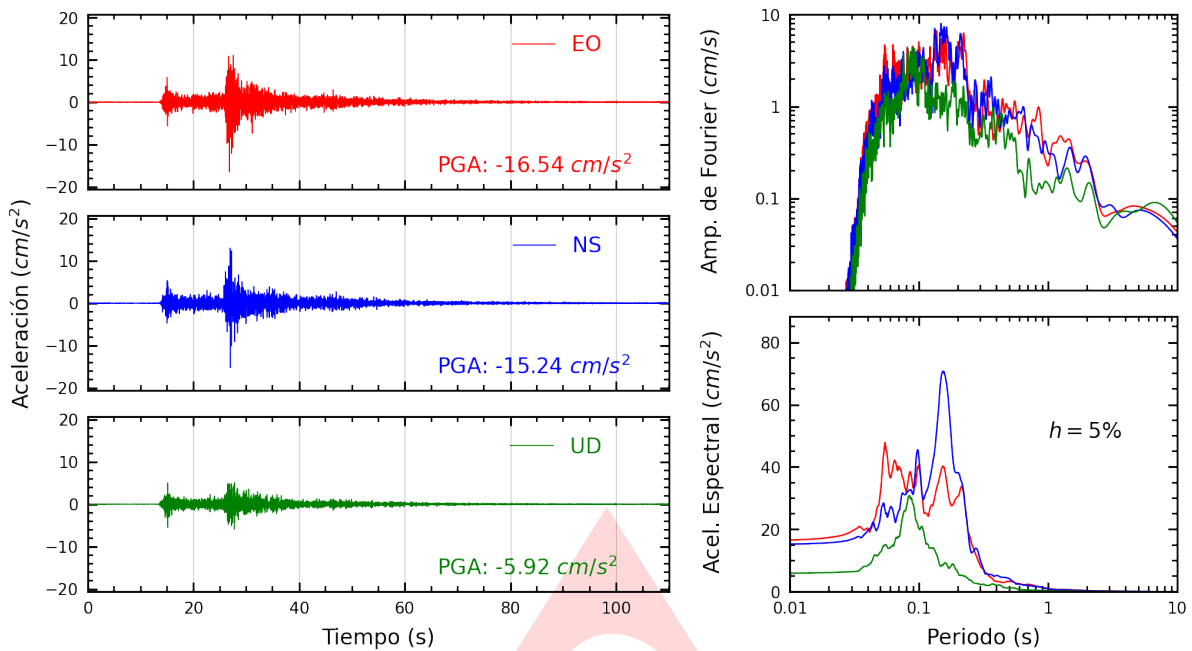
Figura A.1: Registros tiempo-historia, espectros de Fourier y de respuesta en las direcciones EO, NS y vertical de la estación USILM. Sismo de Canta, Canta - Lima del 2022-12-15, 04:31:16 (Hora local)
