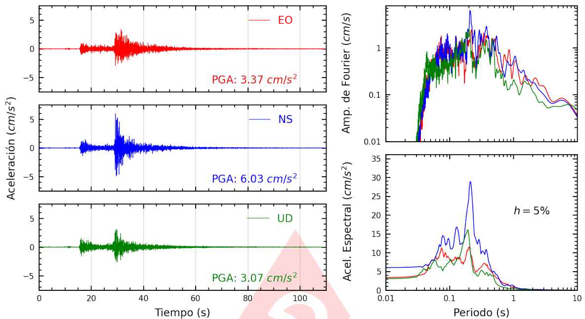
Figura A.11: Registros tiempo-historia, espectros de Fourier y de respuesta en las direcciones EO, NS y vertical de la estación UPCSM. Sismo de Canta, Canta - Lima del 2022-12-15, 04:31:16 (Hora local)
