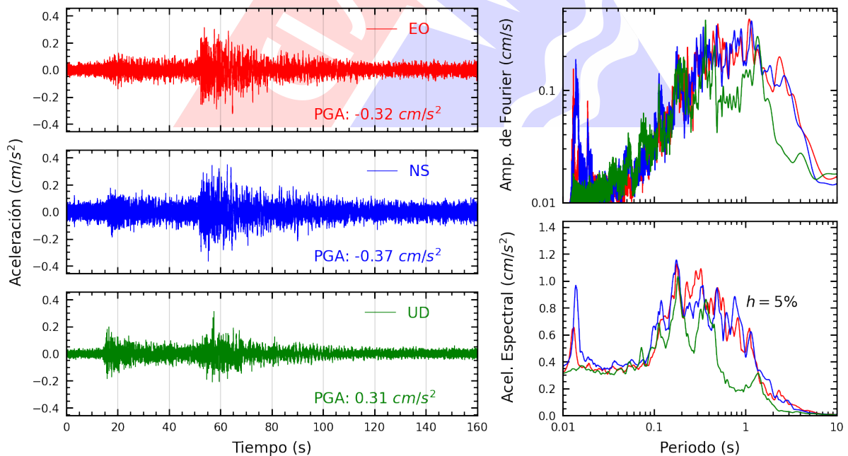
Figura A.36: Registros tiempo-historia, espectros de Fourier y de respuesta en las direcciones EO, NS y vertical de la estación UNICA. Sismo de Canta, Canta - Lima del 2022-12-15, 04:31:16 (Hora local)
