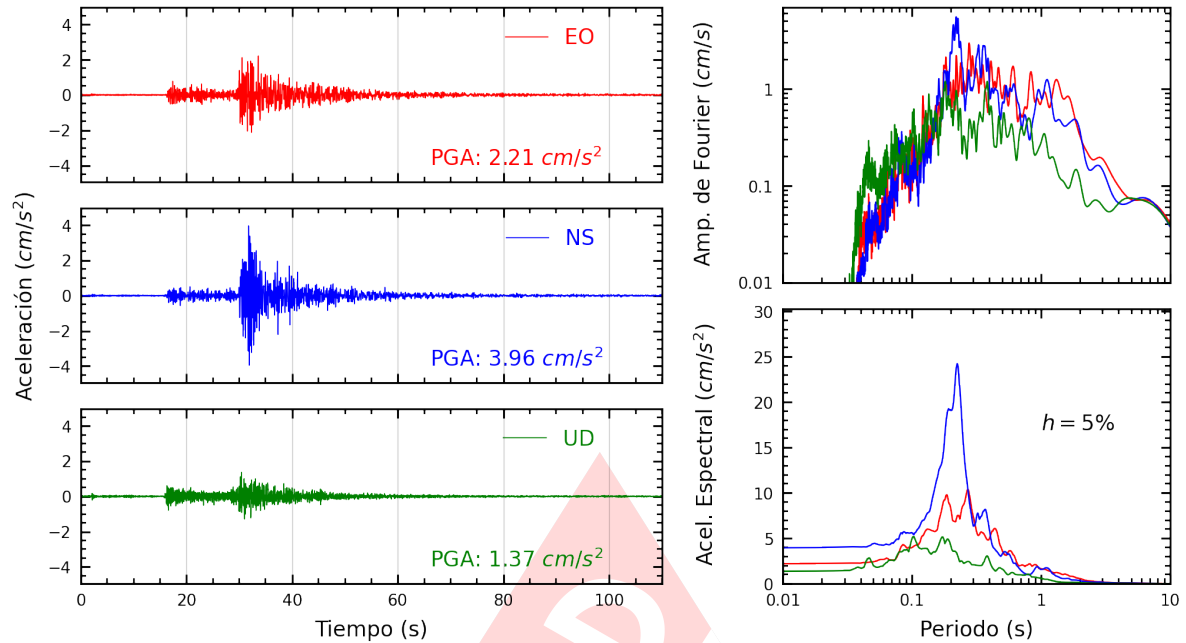
Figura A.23: Registros tiempo-historia, espectros de Fourier y de respuesta en las direcciones EO, NS y vertical de la estación DSML. Sismo de Canta, Canta - Lima del 2022-12-15, 04:31:16 (Hora local)
