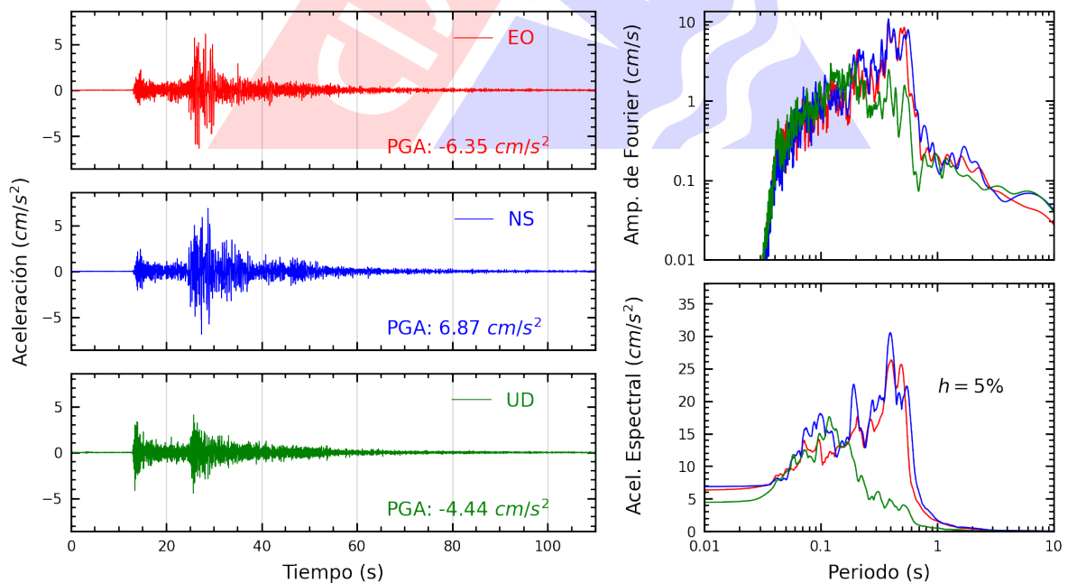
Figura A.8: Registros tiempo-historia, espectros de Fourier y de respuesta en las direcciones EO, NS y vertical de la estación MDPP. Sismo de Canta, Canta - Lima del 2022-12-15, 04:31:16 (Hora local)
