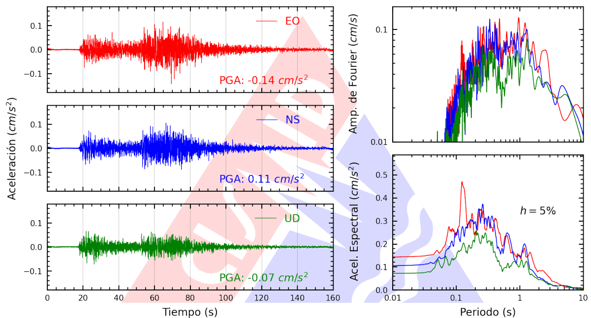
Figura A.37: Registros tiempo-historia, espectros de Fourier y de respuesta en las direcciones EO, NS y vertical de la estación YUNGA. Sismo de Canta, Canta - Lima del 2022-12-15, 04:31:16 (Hora local)
