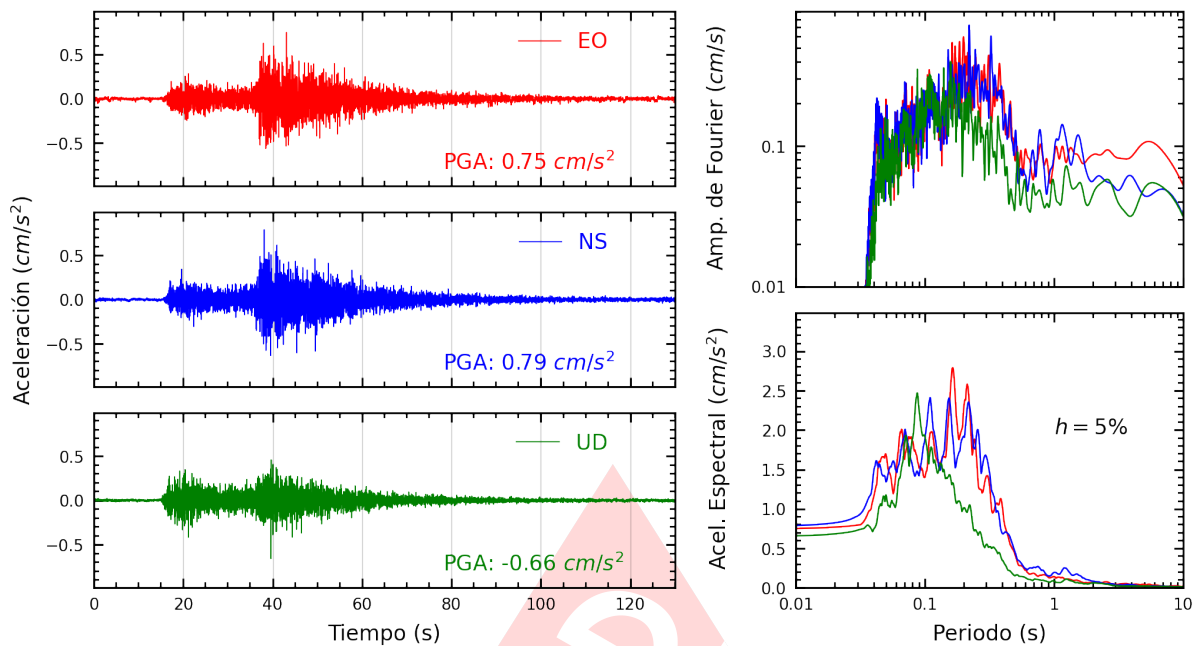
Figura A.35: Registros tiempo-historia, espectros de Fourier y de respuesta en las direcciones EO, NS y vertical de la estación UNAB. Sismo de Canta, Canta - Lima del 2022-12-15, 04:31:16 (Hora local)
