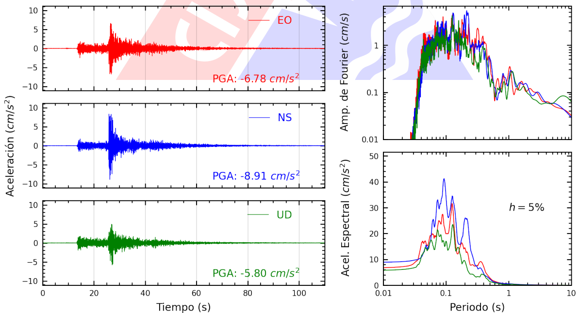
Figura A.4: Registros tiempo-historia, espectros de Fourier y de respuesta en las direcciones EO, NS y vertical de la estación INDEP. Sismo de Canta, Canta - Lima del 2022-12-15, 04:31:16 (Hora local)
