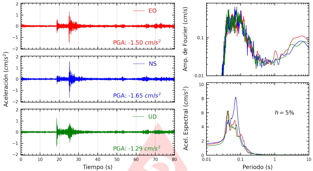
Figura A.11: Registros tiempo-historia, espectros de Fourier y de respuesta en las direcciones EO, NS y vertical de la estación MADRE. Sismo de Provincia Constitucional del Callao , Callao - Lima del 2022-12-22, 12:08:17 (Hora local)
