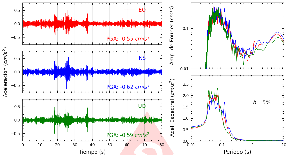
Figura A.25: Registros tiempo-historia, espectros de Fourier y de respuesta en las direcciones EO, NS y vertical de la estación NISTA. Sismo de Provincia Constitucional del Callao , Callao - Lima del 2022-12-22, 12:08:17 (Hora local)
