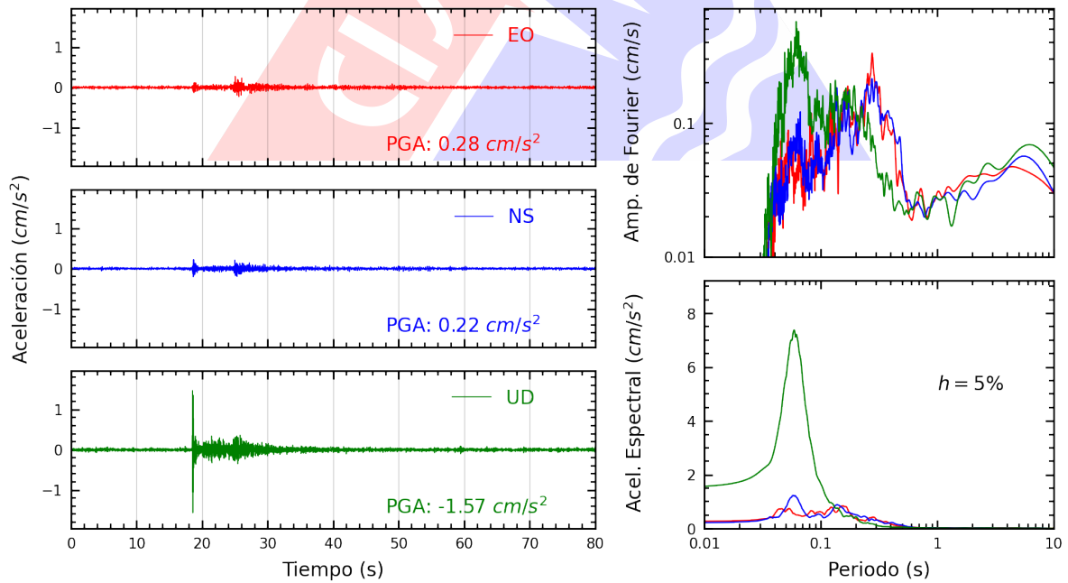
Figura A.12: Registros tiempo-historia, espectros de Fourier y de respuesta en las direcciones EO, NS y vertical de la estación ACAPU. Sismo de Provincia Constitucional del Callao , Callao - Lima del 2022-12-22, 12:08:17 (Hora local)
