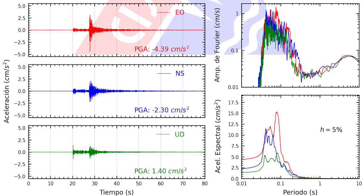
Figura A.4: Registros tiempo-historia, espectros de Fourier y de respuesta en las direcciones EO, NS y vertical de la estación IPEN. Sismo de Provincia Constitucional del Callao , Callao - Lima del 2022-12-22, 12:08:17 (Hora local)
