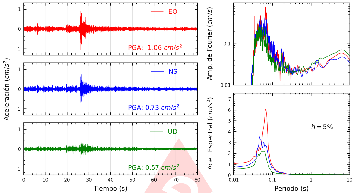
Figura A.19: Registros tiempo-historia, espectros de Fourier y de respuesta en las direcciones EO, NS y vertical de la estación UPCVI. Sismo de Provincia Constitucional del Callao , Callao - Lima del 2022-12-22, 12:08:17 (Hora local)
