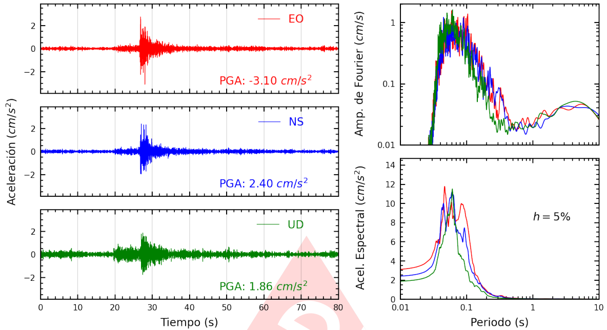
Figura A.5: Registros tiempo-historia, espectros de Fourier y de respuesta en las direcciones EO, NS y vertical de la estación ANCON. Sismo de Provincia Constitucional del Callao , Callao - Lima del 2022-12-22, 12:08:17 (Hora local)
