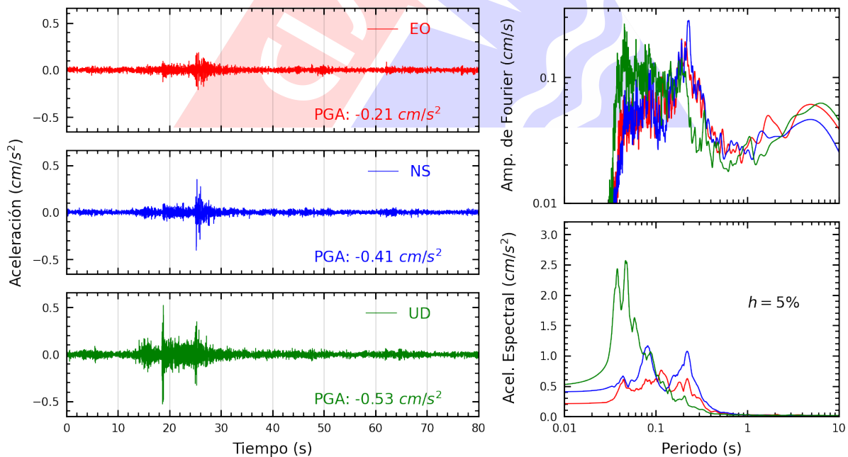
Figura A.28: Registros tiempo-historia, espectros de Fourier y de respuesta en las direcciones EO, NS y vertical de la estación DSMI. Sismo de Provincia Constitucional del Callao , Callao - Lima del 2022-12-22, 12:08:17 (Hora local)
