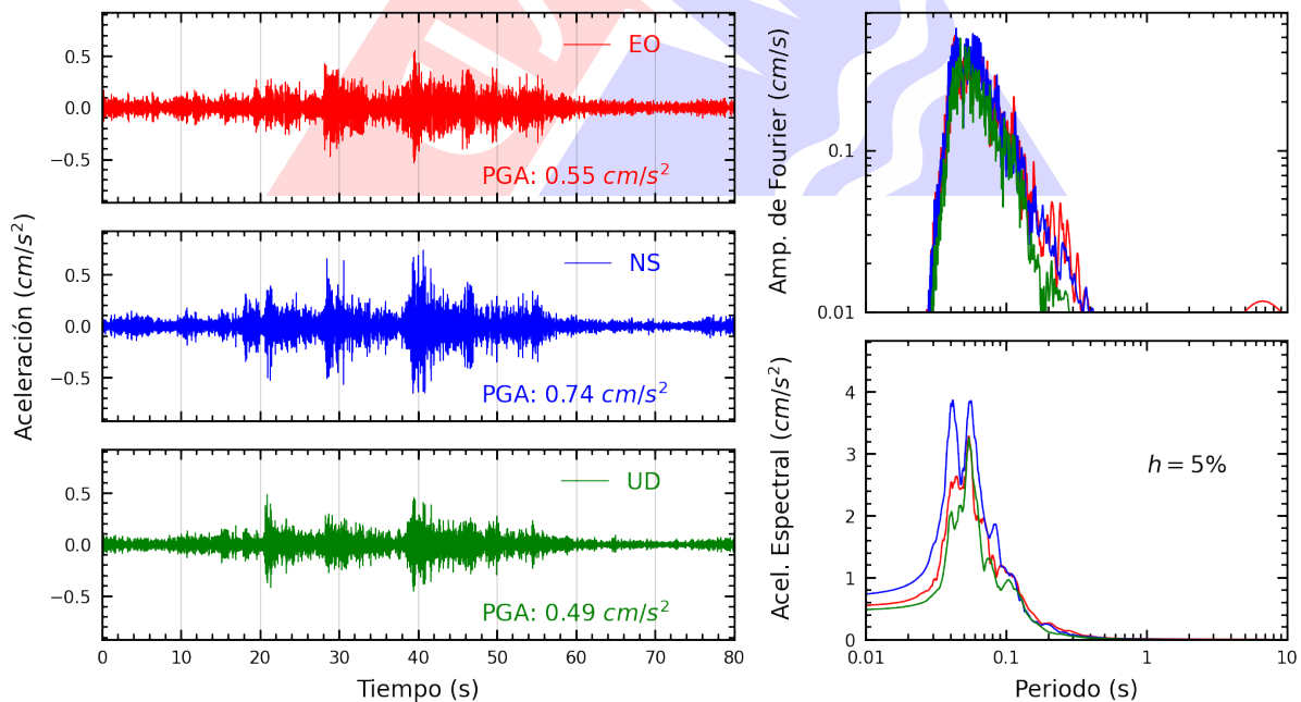
Figura A.22: Registros tiempo-historia, espectros de Fourier y de respuesta en las direcciones EO, NS y vertical de la estación PACHA. Sismo de Provincia Constitucional del Callao , Callao - Lima del 2022-12-22, 12:08:17 (Hora local)
