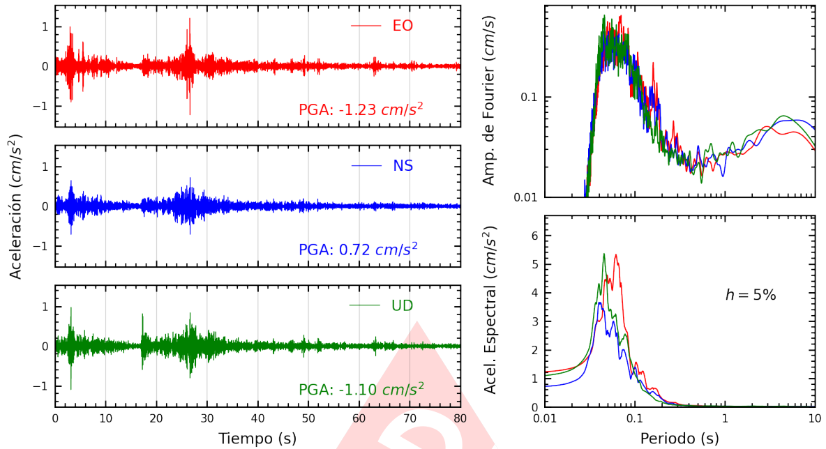
Figura A.17: Registros tiempo-historia, espectros de Fourier y de respuesta en las direcciones EO, NS y vertical de la estación PRADO. Sismo de Provincia Constitucional del Callao , Callao - Lima del 2022-12-22, 12:08:17 (Hora local)
