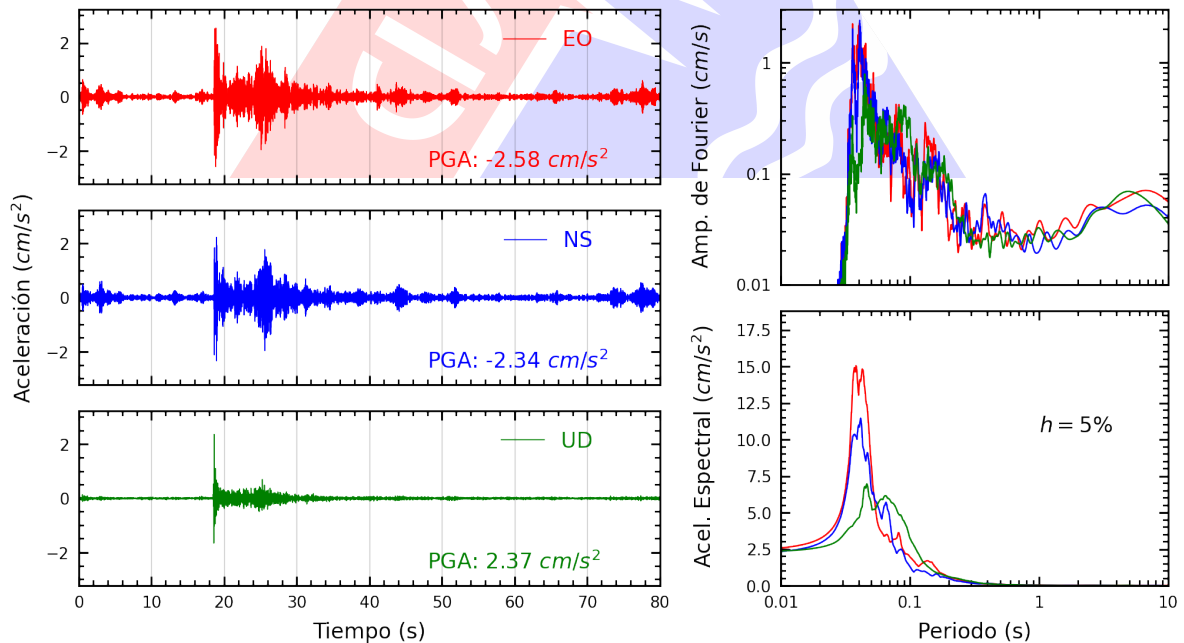
Figura A.6: Registros tiempo-historia, espectros de Fourier y de respuesta en las direcciones EO, NS y vertical de la estación DHNPE. Sismo de Provincia Constitucional del Callao , Callao - Lima del 2022-12-22, 12:08:17 (Hora local)
