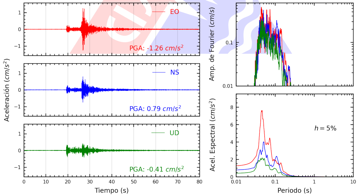
Figura A.16: Registros tiempo-historia, espectros de Fourier y de respuesta en las direcciones EO, NS y vertical de la estación ATARJ. Sismo de Provincia Constitucional del Callao , Callao - Lima del 2022-12-22, 12:08:17 (Hora local)
