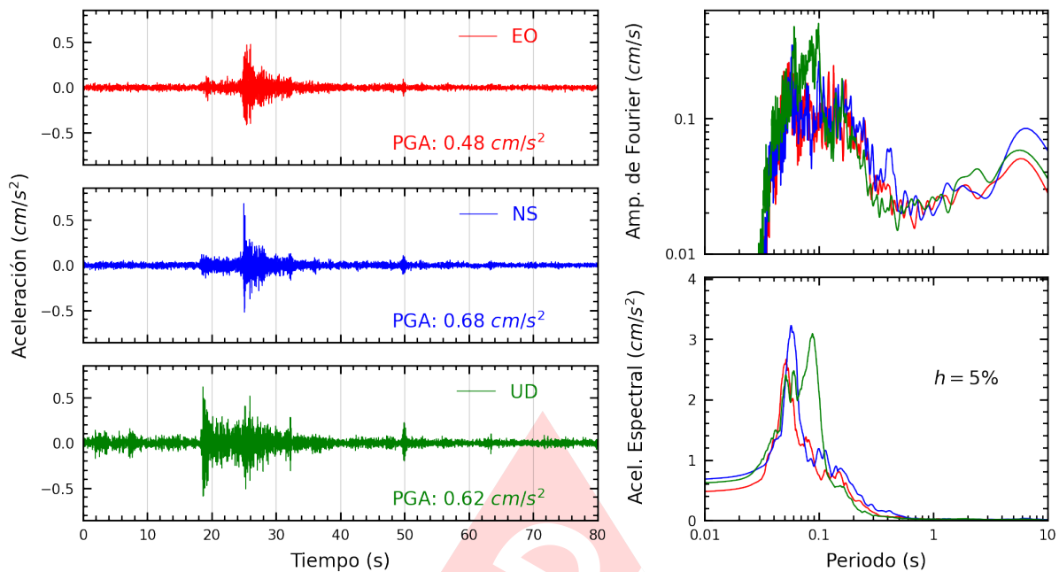
Figura A.23: Registros tiempo-historia, espectros de Fourier y de respuesta en las direcciones EO, NS y vertical de la estación RAMON. Sismo de Provincia Constitucional del Callao , Callao - Lima del 2022-12-22, 12:08:17 (Hora local)
