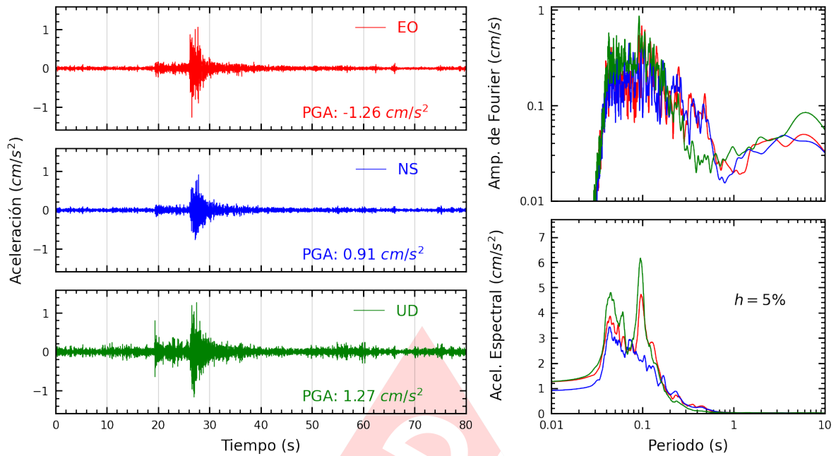
Figura A.15: Registros tiempo-historia, espectros de Fourier y de respuesta en las direcciones EO, NS y vertical de la estación MDPP. Sismo de Provincia Constitucional del Callao , Callao - Lima del 2022-12-22, 12:08:17 (Hora local)
