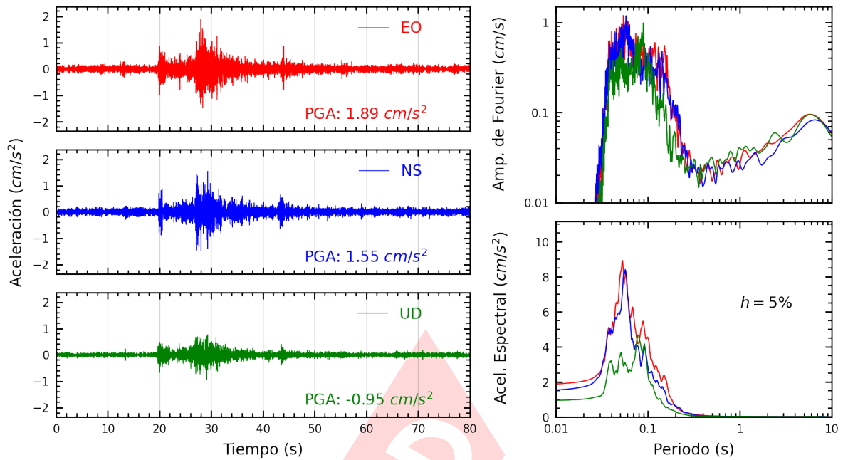
Figura A.9: Registros tiempo-historia, espectros de Fourier y de respuesta en las direcciones EO, NS y vertical de la estación USILM. Sismo de Provincia Constitucional del Callao , Callao - Lima del 2022-12-22, 12:08:17 (Hora local)
