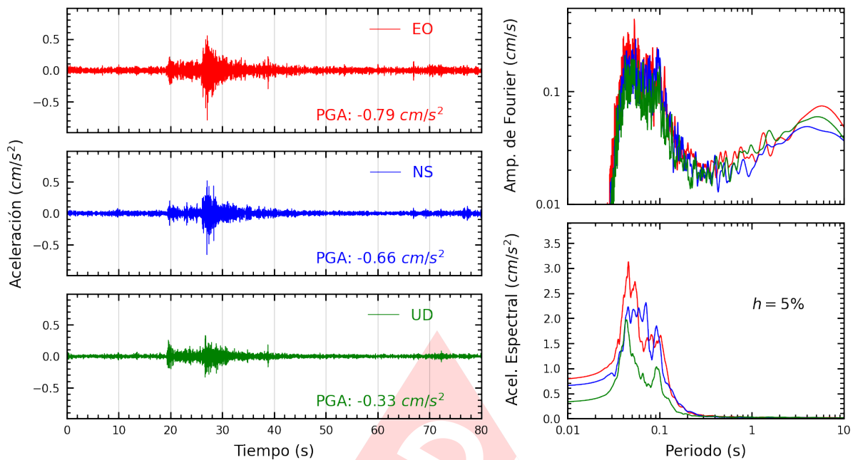
Figura A.21: Registros tiempo-historia, espectros de Fourier y de respuesta en las direcciones EO, NS y vertical de la estación INICT. Sismo de Provincia Constitucional del Callao , Callao - Lima del 2022-12-22, 12:08:17 (Hora local)
