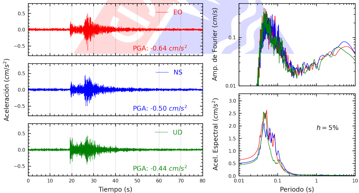
Figura A.24: Registros tiempo-historia, espectros de Fourier y de respuesta en las direcciones EO, NS y vertical de la estación CENEP. Sismo de Provincia Constitucional del Callao , Callao - Lima del 2022-12-22, 12:08:17 (Hora local)
