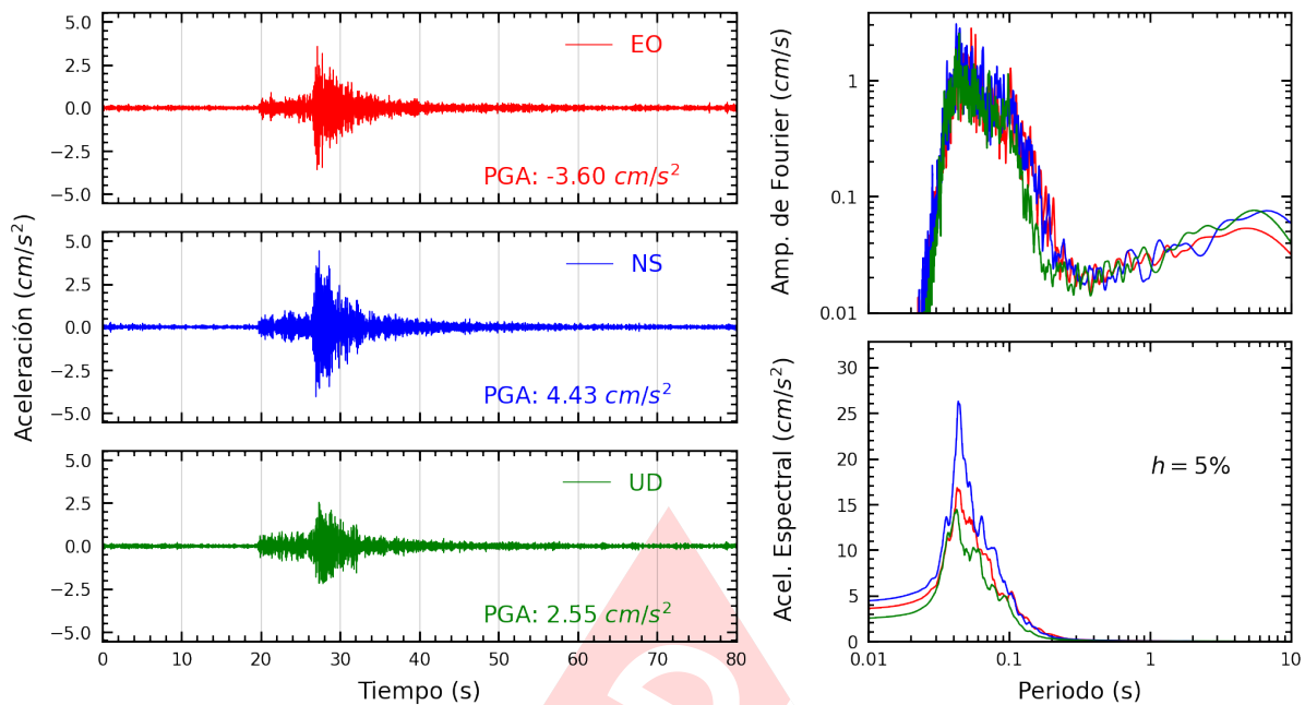
Figura A.3: Registros tiempo-historia, espectros de Fourier y de respuesta en las direcciones EO, NS y vertical de la estación SROSA. Sismo de Provincia Constitucional del Callao , Callao - Lima del 2022-12-22, 12:08:17 (Hora local)
