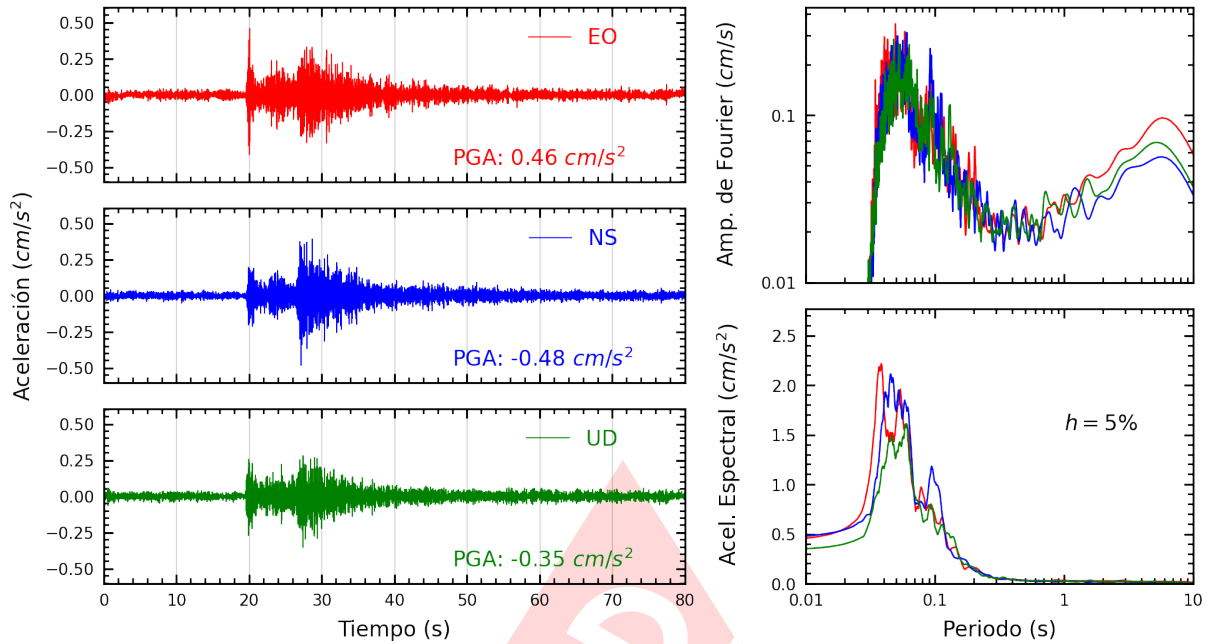
Figura A.29: Registros tiempo-historia, espectros de Fourier y de respuesta en las direcciones EO, NS y vertical de la estación IMCA. Sismo de Provincia Constitucional del Callao , Callao - Lima del 2022-12-22, 12:08:17 (Hora local)
