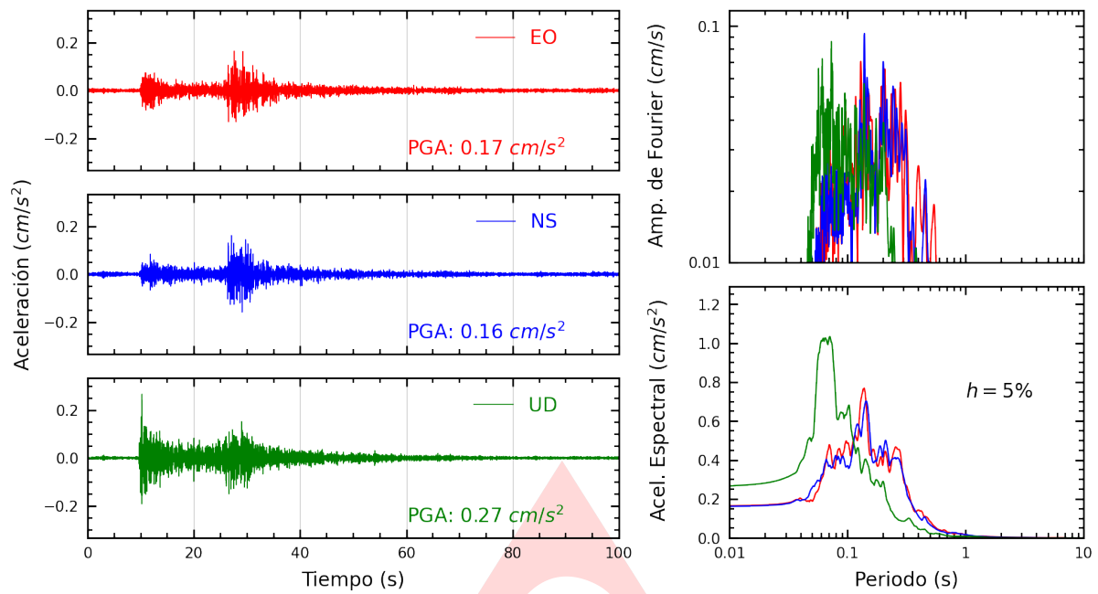
Figura A.1: Registros tiempo-historia, espectros de Fourier y de respuesta en las direcciones EO, NS y vertical de la estación UNAAA. Sismo de Rioja, Rioja - San Martín del 2023-01-20, 21:44:49 (Hora local)
