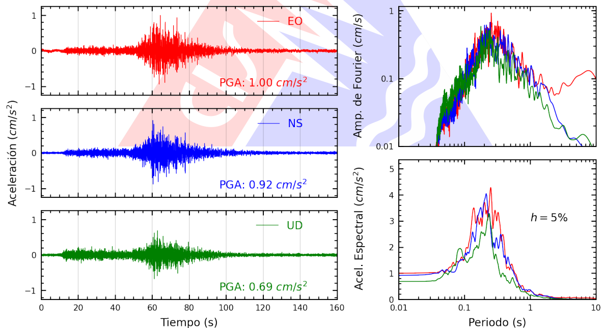
Figura A.2: Registros tiempo-historia, espectros de Fourier y de respuesta en las direcciones EO, NS y vertical de la estación UJB3. Sismo de Atico, Caraveli - Arequipa del 2023-03-05, 14:25:43 (Hora local)
