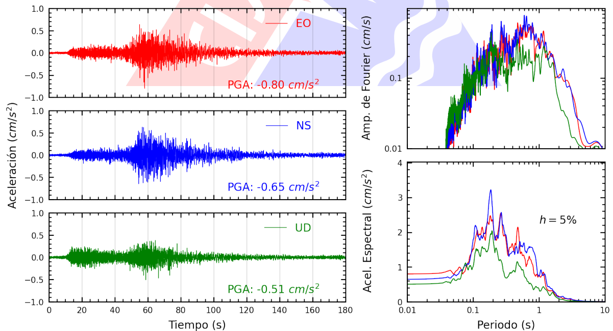
Figura A.4: Registros tiempo-historia, espectros de Fourier y de respuesta en las direcciones EO, NS y vertical de la estación UNICA. Sismo de Atico, Caraveli - Arequipa del 2023-03-05, 14:25:43 (Hora local)
