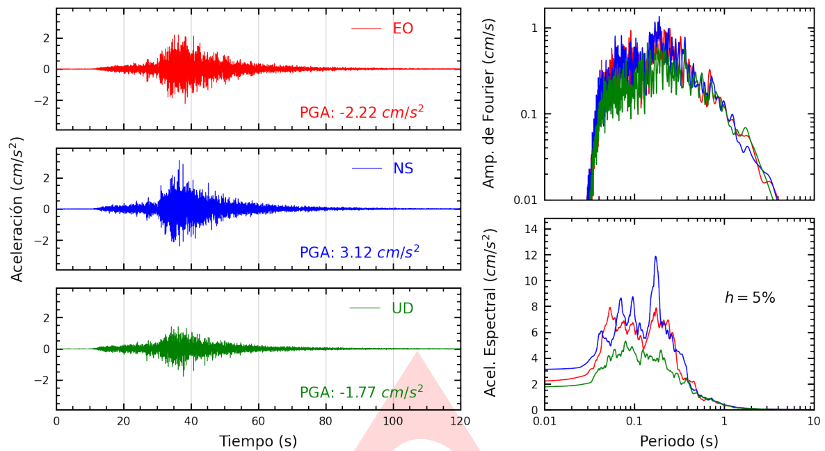
Figura A.1: Registros tiempo-historia, espectros de Fourier y de respuesta en las direcciones EO, NS y vertical de la estación UNSA. Sismo de Atico, Caraveli - Arequipa del 2023-03-05, 14:25:43 (Hora local)
