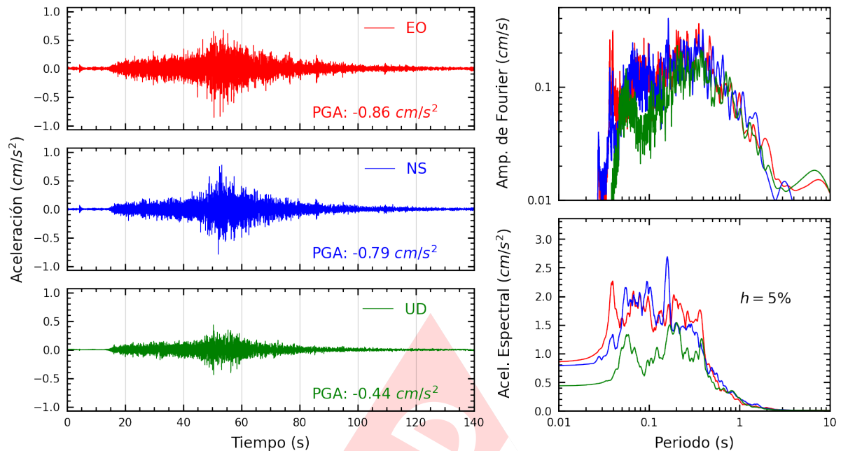
Figura A.3: Registros tiempo-historia, espectros de Fourier y de respuesta en las direcciones EO, NS y vertical de la estación UNAM. Sismo de Atico, Caraveli - Arequipa del 2023-03-05, 14:25:43 (Hora local)
