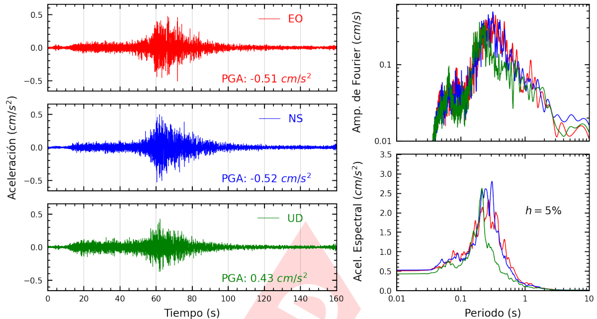
Figura A.5: Registros tiempo-historia, espectros de Fourier y de respuesta en las direcciones EO, NS y vertical de la estación CREY. Sismo de Atico, Caraveli - Arequipa del 2023-03-05, 14:25:43 (Hora local)
