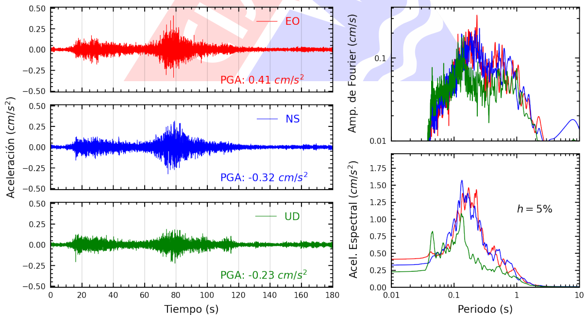
Figura A.6: Registros tiempo-historia, espectros de Fourier y de respuesta en las direcciones EO, NS y vertical de la estación ASIA. Sismo de Atico, Caraveli - Arequipa del 2023-03-05, 14:25:43 (Hora local)
