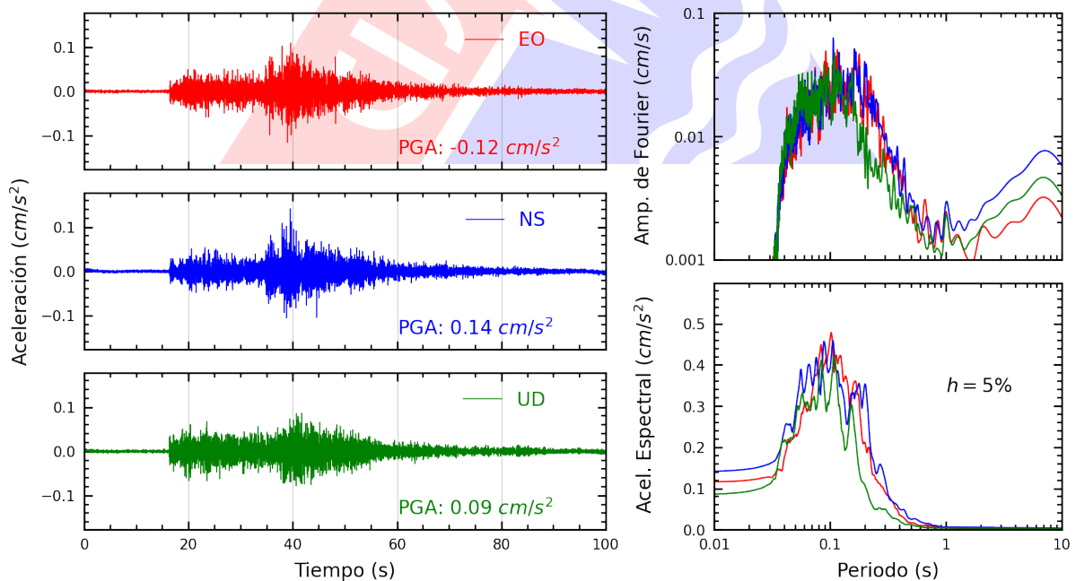
Figura A.28: Registros tiempo-historia, espectros de Fourier y de respuesta en las direcciones EO, NS y vertical de la estación ASIA. Sismo de Provincia Constitucional del Callao , Callao - Lima del 2023-03-20, 22:37:10 (Hora local)
