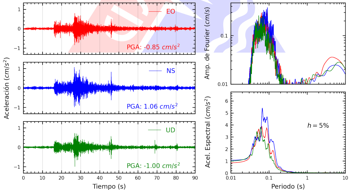
Figura A.8: Registros tiempo-historia, espectros de Fourier y de respuesta en las direcciones EO, NS y vertical de la estación JOSEO. Sismo de Provincia Constitucional del Callao , Callao - Lima del 2023-03-20, 22:37:10 (Hora local)
