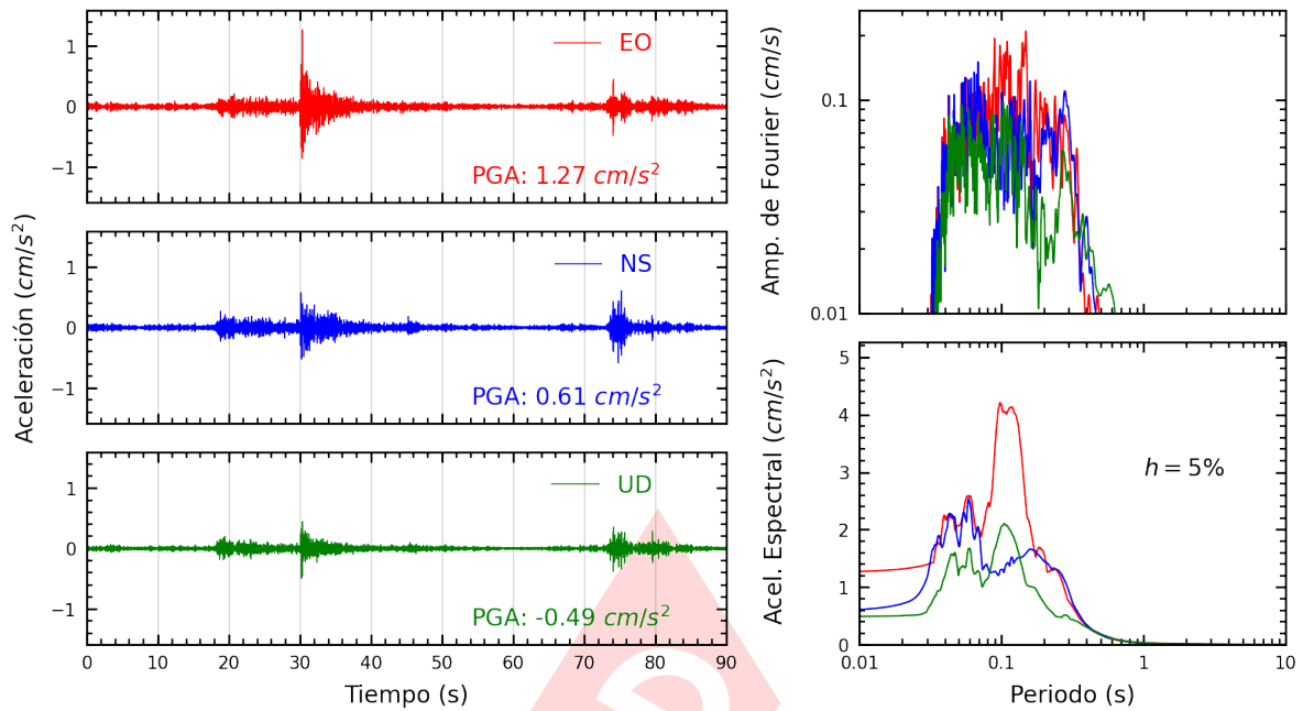
Figura A.5: Registros tiempo-historia, espectros de Fourier y de respuesta en las direcciones EO, NS y vertical de la estación PACHA. Sismo de Provincia Constitucional del Callao , Callao - Lima del 2023-03-20, 22:37:10 (Hora local)
