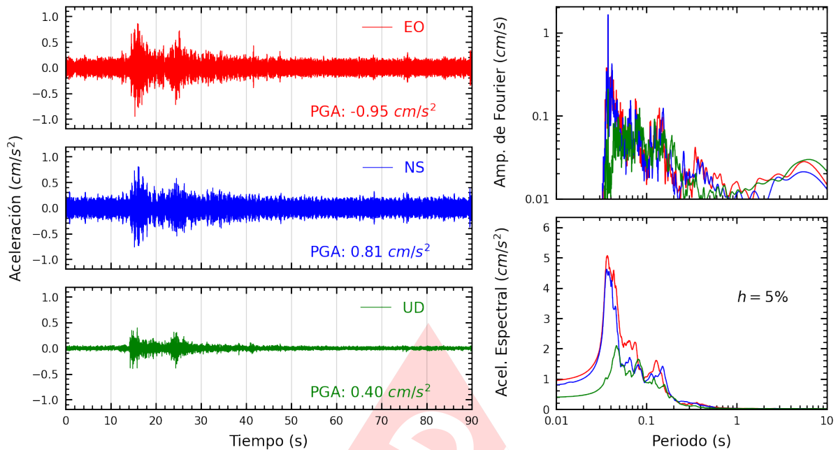
Figura A.11: Registros tiempo-historia, espectros de Fourier y de respuesta en las direcciones EO, NS y vertical de la estación DHNPE. Sismo de Provincia Constitucional del Callao , Callao - Lima del 2023-03-20, 22:37:10 (Hora local)
