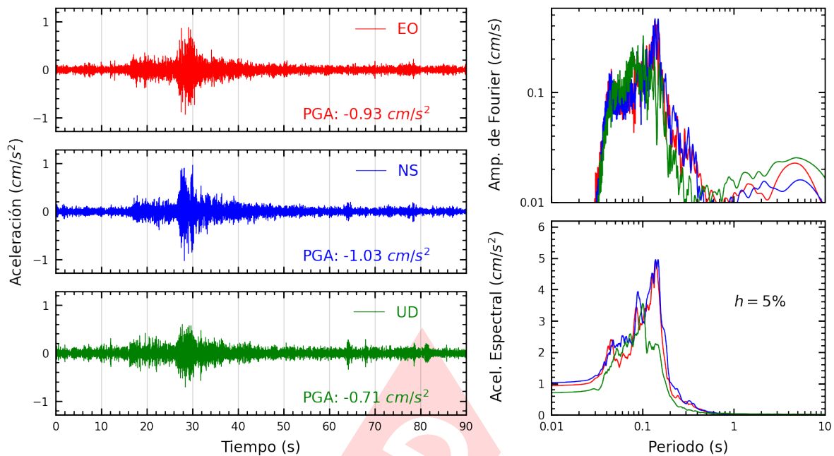
Figura A.9: Registros tiempo-historia, espectros de Fourier y de respuesta en las direcciones EO, NS y vertical de la estación CARAB. Sismo de Provincia Constitucional del Callao , Callao - Lima del 2023-03-20, 22:37:10 (Hora local)
