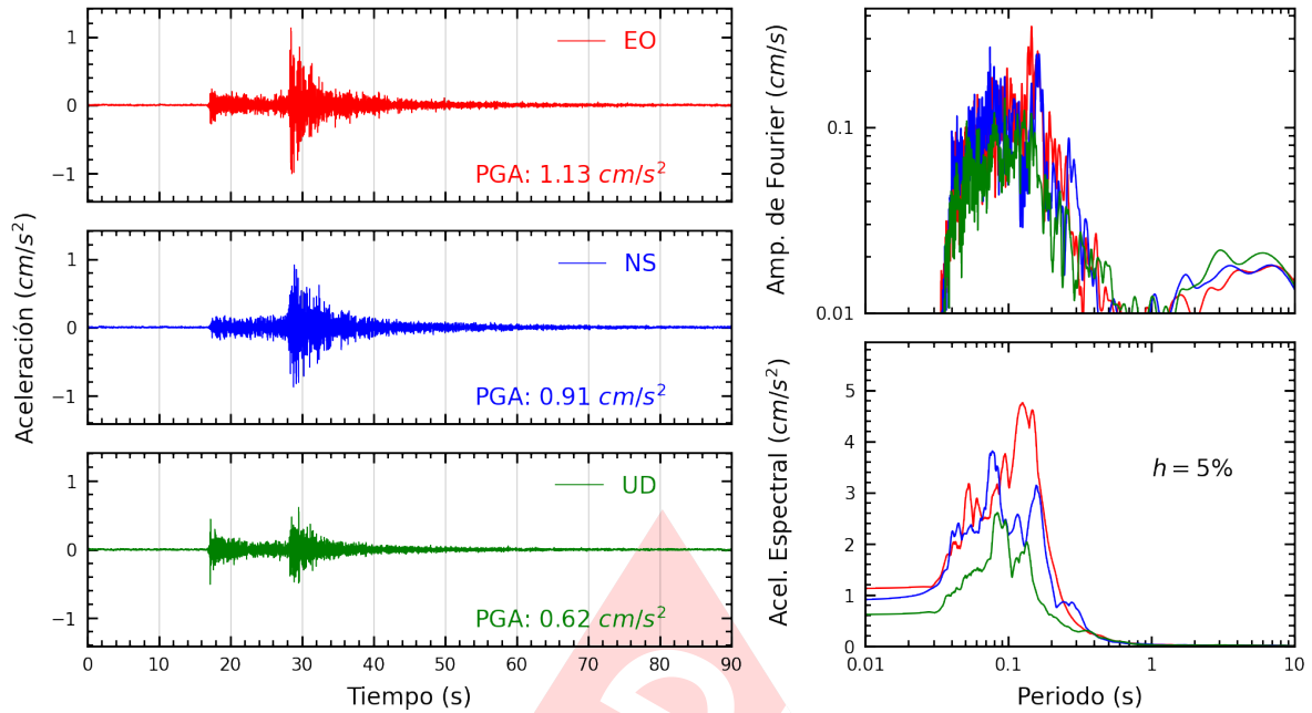
Figura A.7: Registros tiempo-historia, espectros de Fourier y de respuesta en las direcciones EO, NS y vertical de la estación IPEN. Sismo de Provincia Constitucional del Callao , Callao - Lima del 2023-03-20, 22:37:10 (Hora local)
