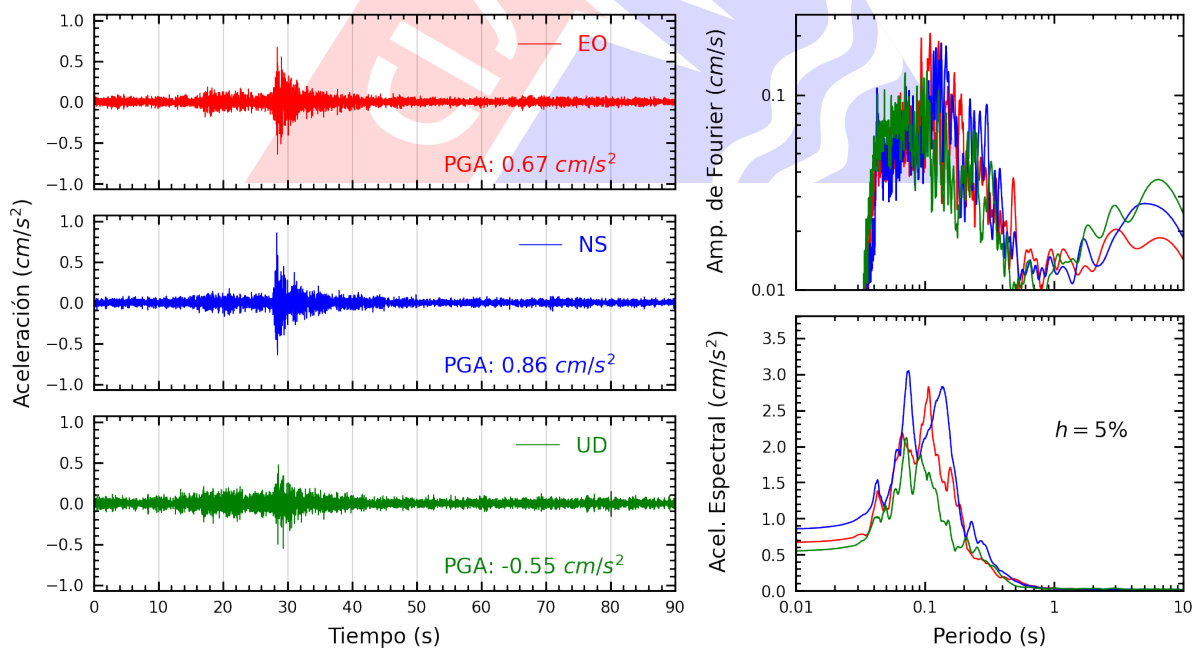
Figura A.14: Registros tiempo-historia, espectros de Fourier y de respuesta en las direcciones EO, NS y vertical de la estación URPE. Sismo de Provincia Constitucional del Callao , Callao - Lima del 2023-03-20, 22:37:10 (Hora local)
