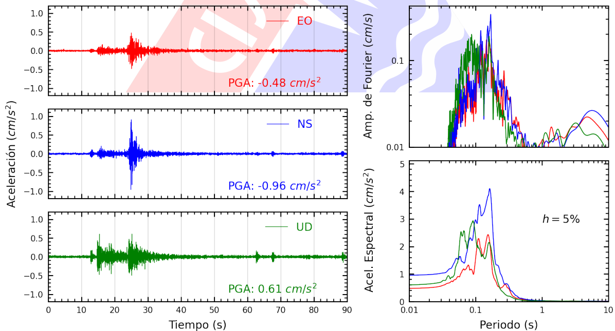
Figura A.10: Registros tiempo-historia, espectros de Fourier y de respuesta en las direcciones EO, NS y vertical de la estación RAMON. Sismo de Provincia Constitucional del Callao , Callao - Lima del 2023-03-20, 22:37:10 (Hora local)
