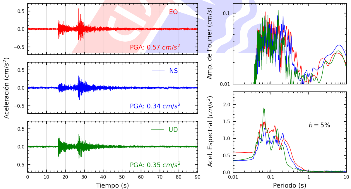
Figura A.20: Registros tiempo-historia, espectros de Fourier y de respuesta en las direcciones EO, NS y vertical de la estación CENEP. Sismo de Provincia Constitucional del Callao , Callao - Lima del 2023-03-20, 22:37:10 (Hora local)
