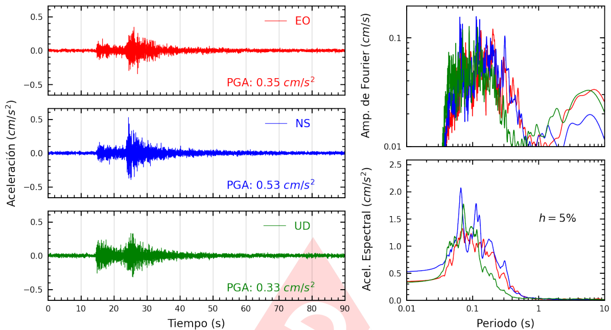
Figura A.21: Registros tiempo-historia, espectros de Fourier y de respuesta en las direcciones EO, NS y vertical de la estación VHAYA. Sismo de Provincia Constitucional del Callao , Callao - Lima del 2023-03-20, 22:37:10 (Hora local)
