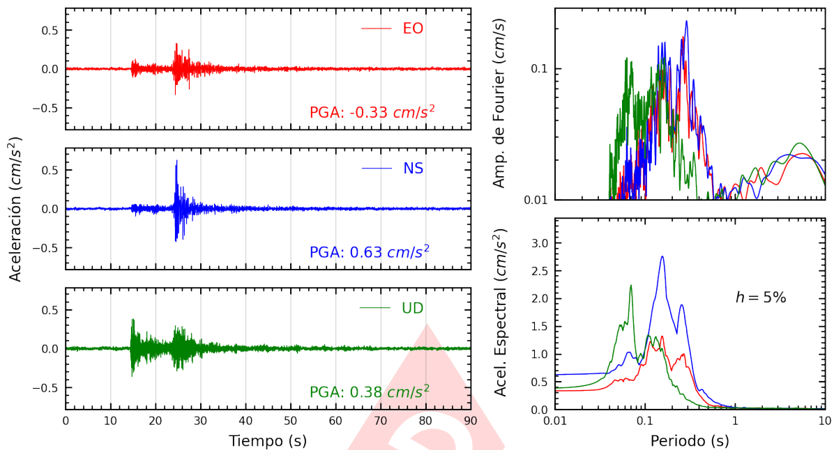
Figura A.17: Registros tiempo-historia, espectros de Fourier y de respuesta en las direcciones EO, NS y vertical de la estación ACAPU. Sismo de Provincia Constitucional del Callao , Callao - Lima del 2023-03-20, 22:37:10 (Hora local)
