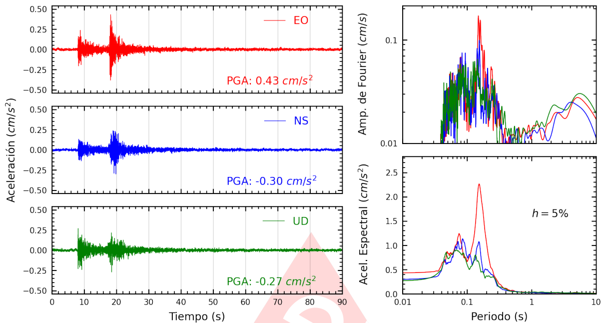
Figura A.25: Registros tiempo-historia, espectros de Fourier y de respuesta en las direcciones EO, NS y vertical de la estación UNMSM. Sismo de Provincia Constitucional del Callao , Callao - Lima del 2023-03-20, 22:37:10 (Hora local)
