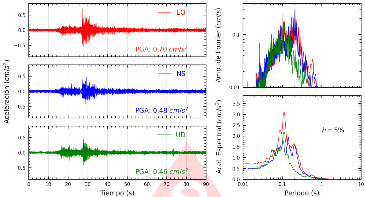
Figura A.15: Registros tiempo-historia, espectros de Fourier y de respuesta en las direcciones EO, NS y vertical de la estación SCCHO. Sismo de Provincia Constitucional del Callao , Callao - Lima del 2023-03-20, 22:37:10 (Hora local)
