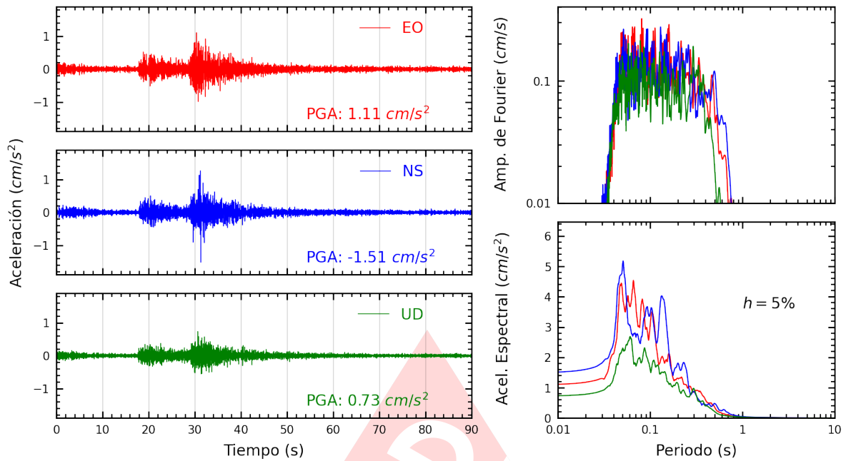
Figura A.3: Registros tiempo-historia, espectros de Fourier y de respuesta en las direcciones EO, NS y vertical de la estación UNTEL. Sismo de Provincia Constitucional del Callao , Callao - Lima del 2023-03-20, 22:37:10 (Hora local)
