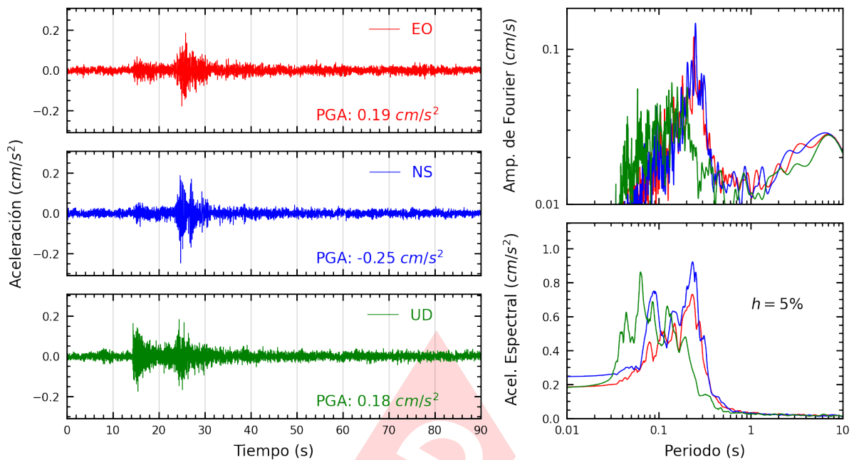
Figura A.27: Registros tiempo-historia, espectros de Fourier y de respuesta en las direcciones EO, NS y vertical de la estación DSMI. Sismo de Provincia Constitucional del Callao , Callao - Lima del 2023-03-20, 22:37:10 (Hora local)
