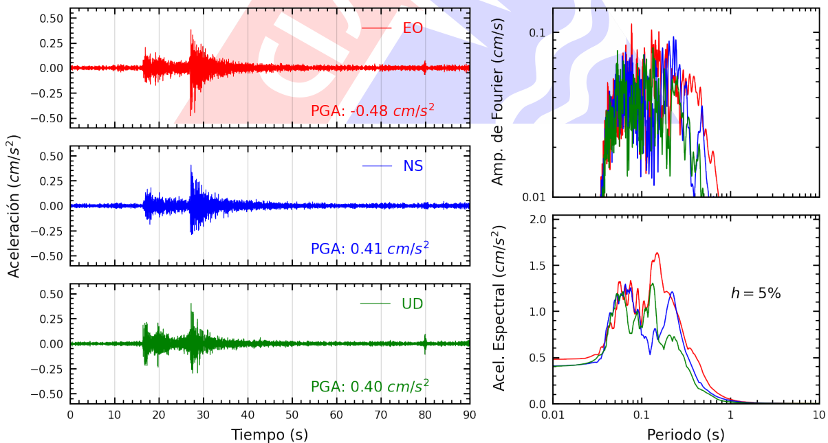
Figura A.22: Registros tiempo-historia, espectros de Fourier y de respuesta en las direcciones EO, NS y vertical de la estación BORJA. Sismo de Provincia Constitucional del Callao , Callao - Lima del 2023-03-20, 22:37:10 (Hora local)
