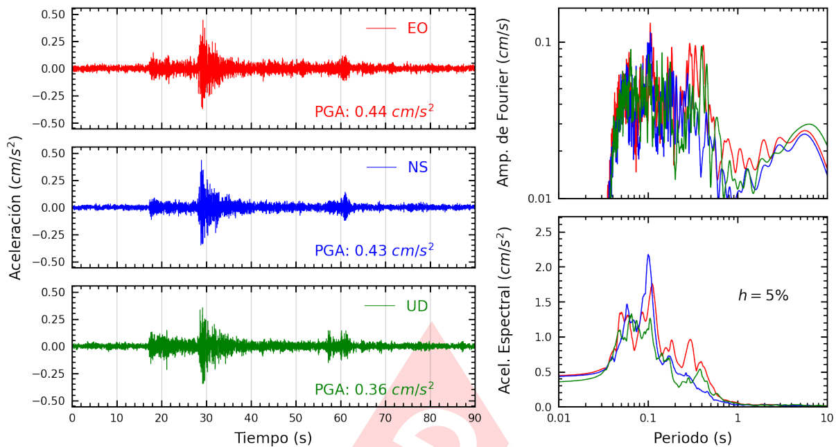
Figura A.23: Registros tiempo-historia, espectros de Fourier y de respuesta en las direcciones EO, NS y vertical de la estación IMCA. Sismo de Provincia Constitucional del Callao , Callao - Lima del 2023-03-20, 22:37:10 (Hora local)
