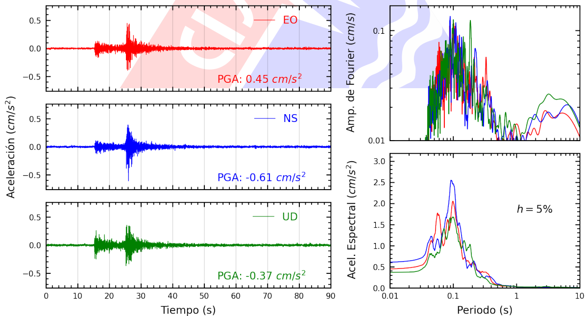
Figura A.18: Registros tiempo-historia, espectros de Fourier y de respuesta en las direcciones EO, NS y vertical de la estación UNFV. Sismo de Provincia Constitucional del Callao , Callao - Lima del 2023-03-20, 22:37:10 (Hora local)
