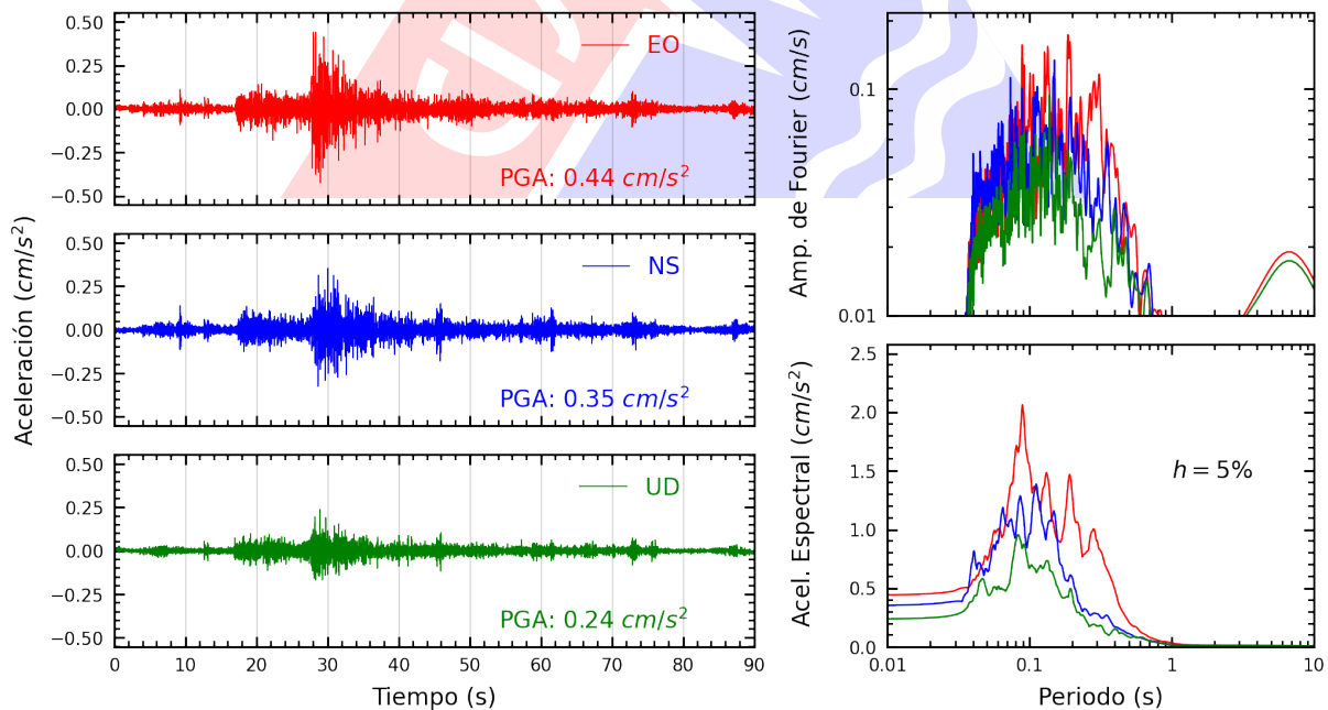
Figura A.24: Registros tiempo-historia, espectros de Fourier y de respuesta en las direcciones EO, NS y vertical de la estación BRISA. Sismo de Provincia Constitucional del Callao , Callao - Lima del 2023-03-20, 22:37:10 (Hora local)
