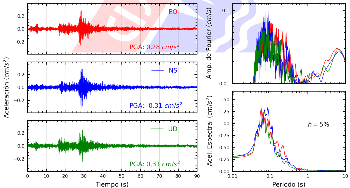
Figura A.26: Registros tiempo-historia, espectros de Fourier y de respuesta en las direcciones EO, NS y vertical de la estación SERVI. Sismo de Provincia Constitucional del Callao , Callao - Lima del 2023-03-20, 22:37:10 (Hora local)
