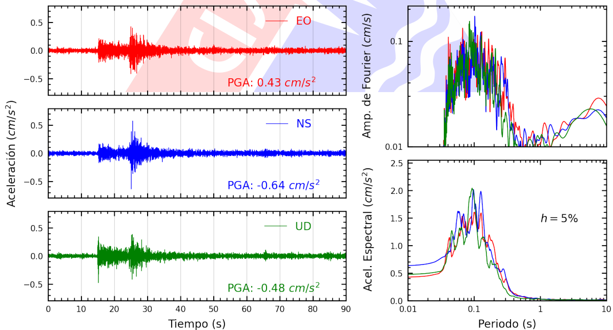
Figura A.16: Registros tiempo-historia, espectros de Fourier y de respuesta en las direcciones EO, NS y vertical de la estación MADRE. Sismo de Provincia Constitucional del Callao , Callao - Lima del 2023-03-20, 22:37:10 (Hora local)
