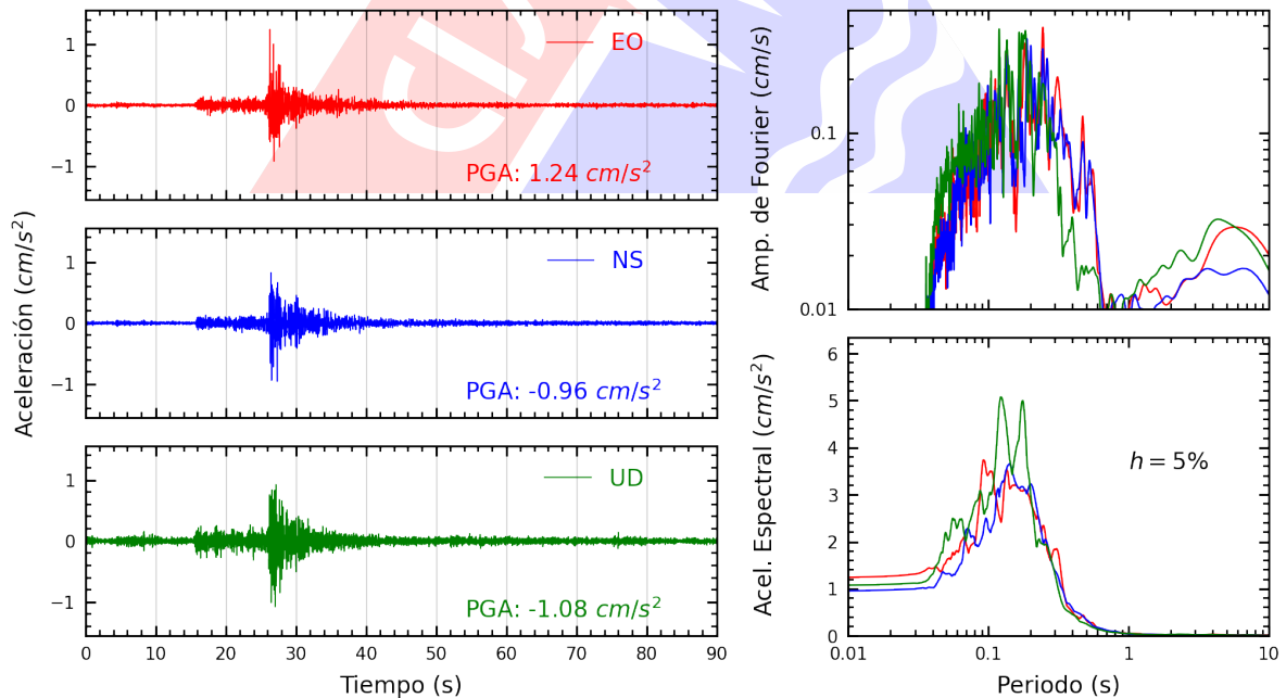
Figura A.6: Registros tiempo-historia, espectros de Fourier y de respuesta en las direcciones EO, NS y vertical de la estación MDPP. Sismo de Provincia Constitucional del Callao , Callao - Lima del 2023-03-20, 22:37:10 (Hora local)
