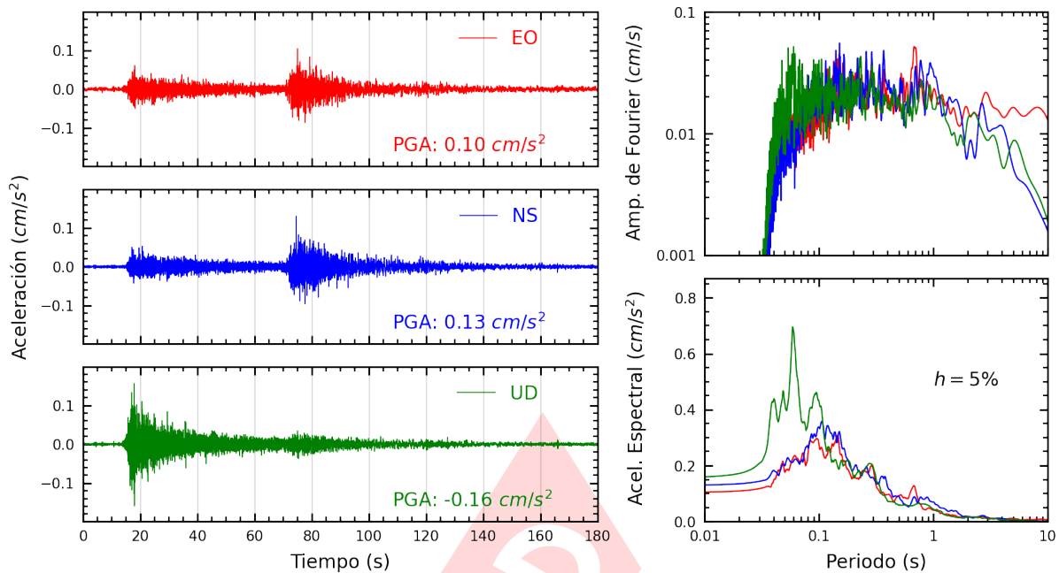
Figura A.17: Registros tiempo-historia, espectros de Fourier y de respuesta en las direcciones EO, NS y vertical de la estación SCCHL. Sismo de Contamana, Ucayali - Loreto del 2023-05-01, 04:31:06 (Hora local)
