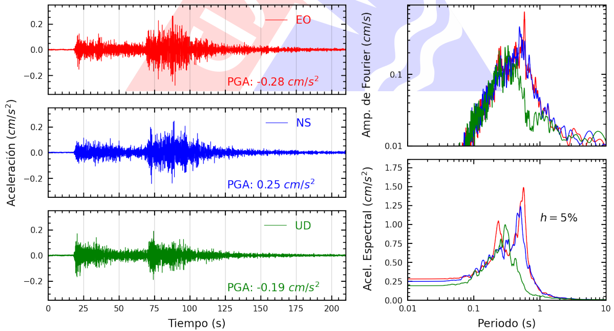
Figura A.10: Registros tiempo-historia, espectros de Fourier y de respuesta en las direcciones EO, NS y vertical de la estación CARAL. Sismo de Contamana, Ucayali - Loreto del 2023-05-01, 04:31:06 (Hora local)
