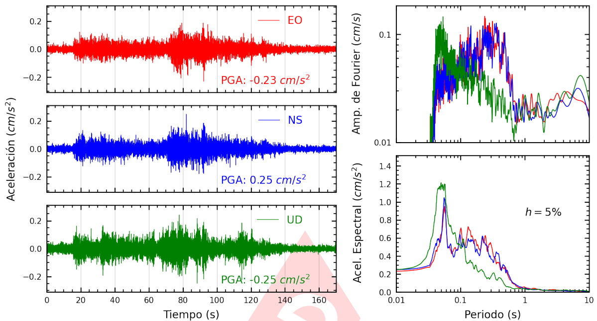
Figura A.13: Registros tiempo-historia, espectros de Fourier y de respuesta en las direcciones EO, NS y vertical de la estación ANCON. Sismo de Contamana, Ucayali - Loreto del 2023-05-01, 04:31:06 (Hora local)
