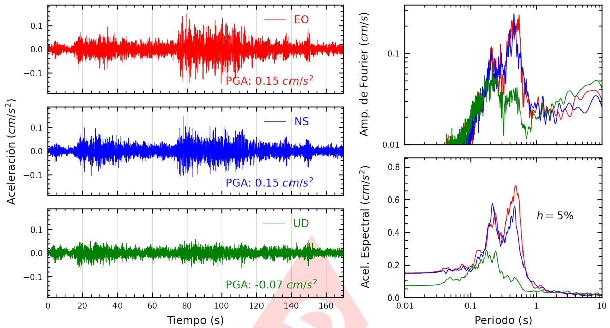
Figura A.19: Registros tiempo-historia, espectros de Fourier y de respuesta en las direcciones EO, NS y vertical de la estación VHAYA. Sismo de Contamana, Ucayali - Loreto del 2023-05-01, 04:31:06 (Hora local)
