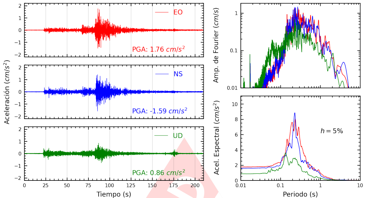
Figura A.3: Registros tiempo-historia, espectros de Fourier y de respuesta en las direcciones EO, NS y vertical de la estación SCIQU. Sismo de Contamana, Ucayali - Loreto del 2023-05-01, 04:31:06 (Hora local)
