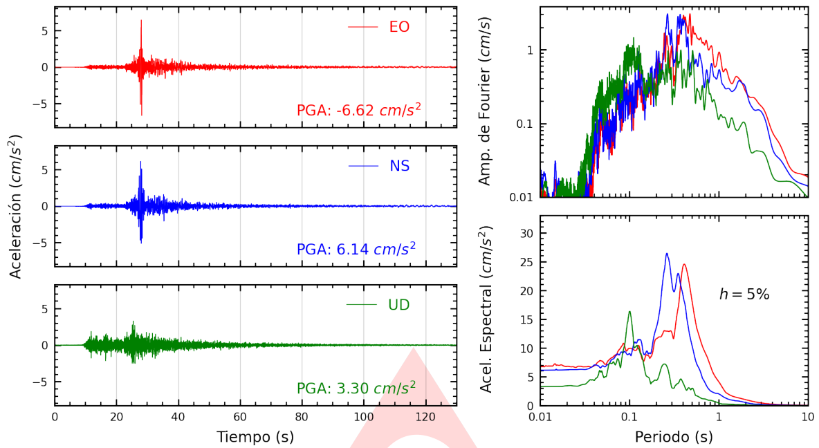
Figura A.1: Registros tiempo-historia, espectros de Fourier y de respuesta en las direcciones EO, NS y vertical de la estación SCPUC. Sismo de Contamana, Ucayali - Loreto del 2023-05-01, 04:31:06 (Hora local)
