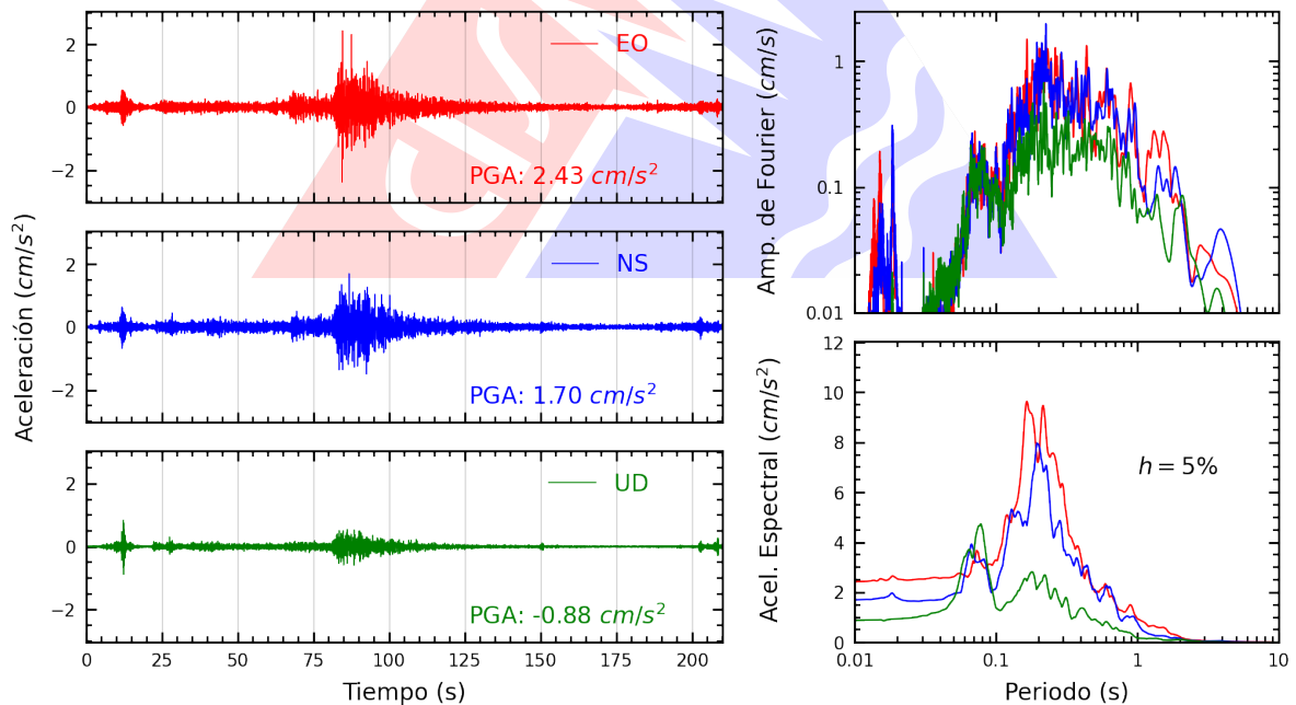
Figura A.2: Registros tiempo-historia, espectros de Fourier y de respuesta en las direcciones EO, NS y vertical de la estación UNAPI. Sismo de Contamana, Ucayali - Loreto del 2023-05-01, 04:31:06 (Hora local)
