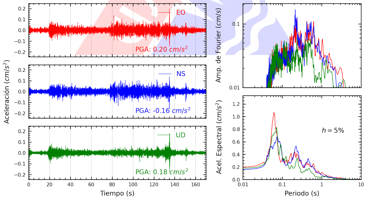
Figura A.16: Registros tiempo-historia, espectros de Fourier y de respuesta en las direcciones EO, NS y vertical de la estación SCCHO. Sismo de Contamana, Ucayali - Loreto del 2023-05-01, 04:31:06 (Hora local)
