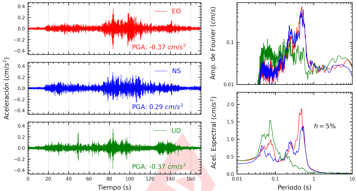
Figura A.7: Registros tiempo-historia, espectros de Fourier y de respuesta en las direcciones EO, NS y vertical de la estación MDPP. Sismo de Contamana, Ucayali - Loreto del 2023-05-01, 04:31:06 (Hora local)
