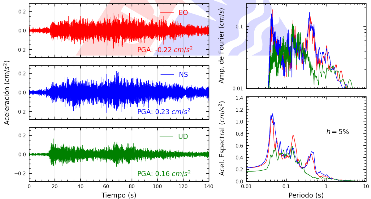
Figura A.14: Registros tiempo-historia, espectros de Fourier y de respuesta en las direcciones EO, NS y vertical de la estación SCTRU. Sismo de Contamana, Ucayali - Loreto del 2023-05-01, 04:31:06 (Hora local)
