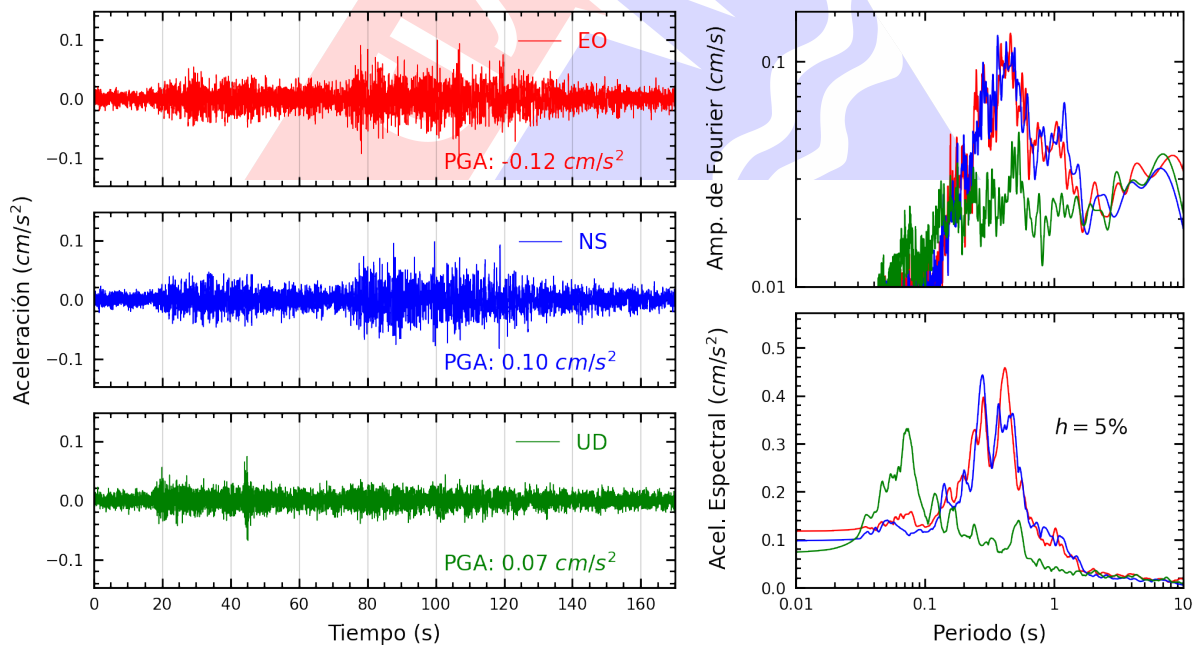
Figura A.20: Registros tiempo-historia, espectros de Fourier y de respuesta en las direcciones EO, NS y vertical de la estación ACAPU. Sismo de Contamana, Ucayali - Loreto del 2023-05-01, 04:31:06 (Hora local)
