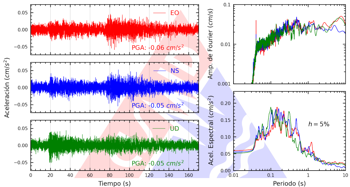
Figura A.23: Registros tiempo-historia, espectros de Fourier y de respuesta en las direcciones EO, NS y vertical de la estación SERVI. Sismo de Contamana, Ucayali - Loreto del 2023-05-01, 04:31:06 (Hora local)
