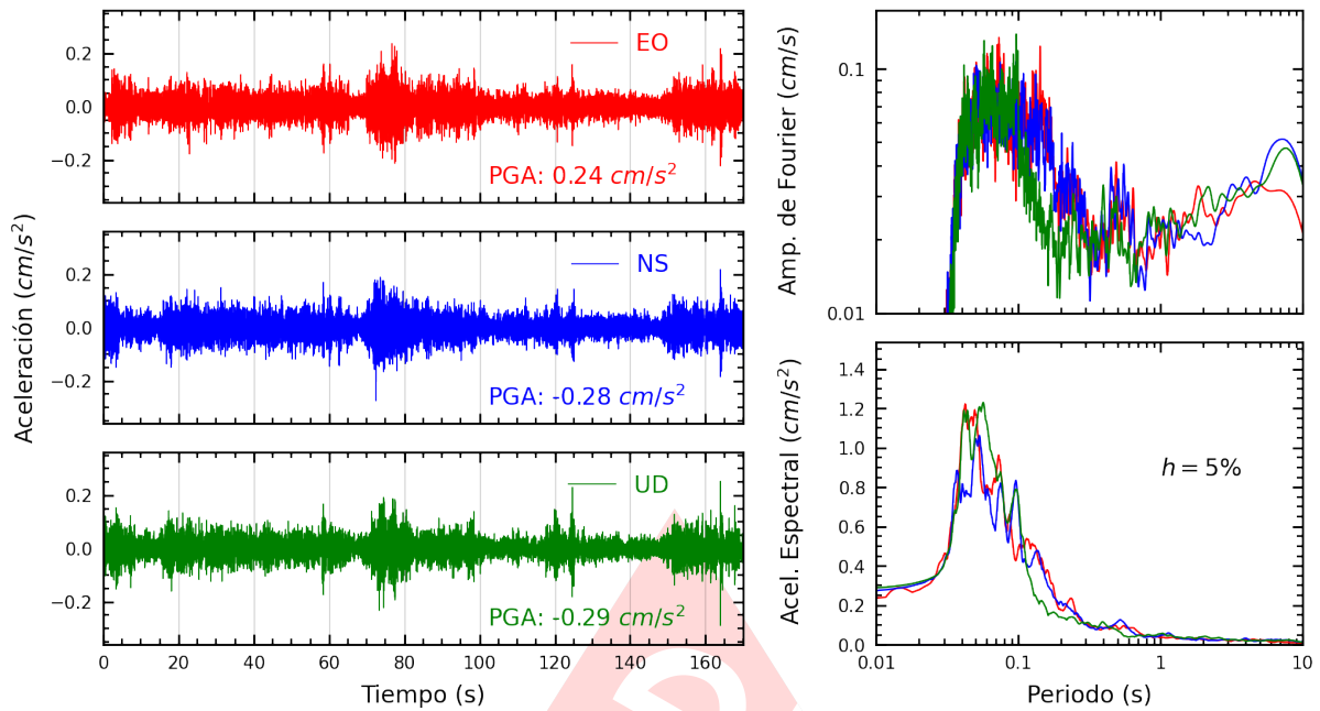
Figura A.9: Registros tiempo-historia, espectros de Fourier y de respuesta en las direcciones EO, NS y vertical de la estación SROSA. Sismo de Contamana, Ucayali - Loreto del 2023-05-01, 04:31:06 (Hora local)
