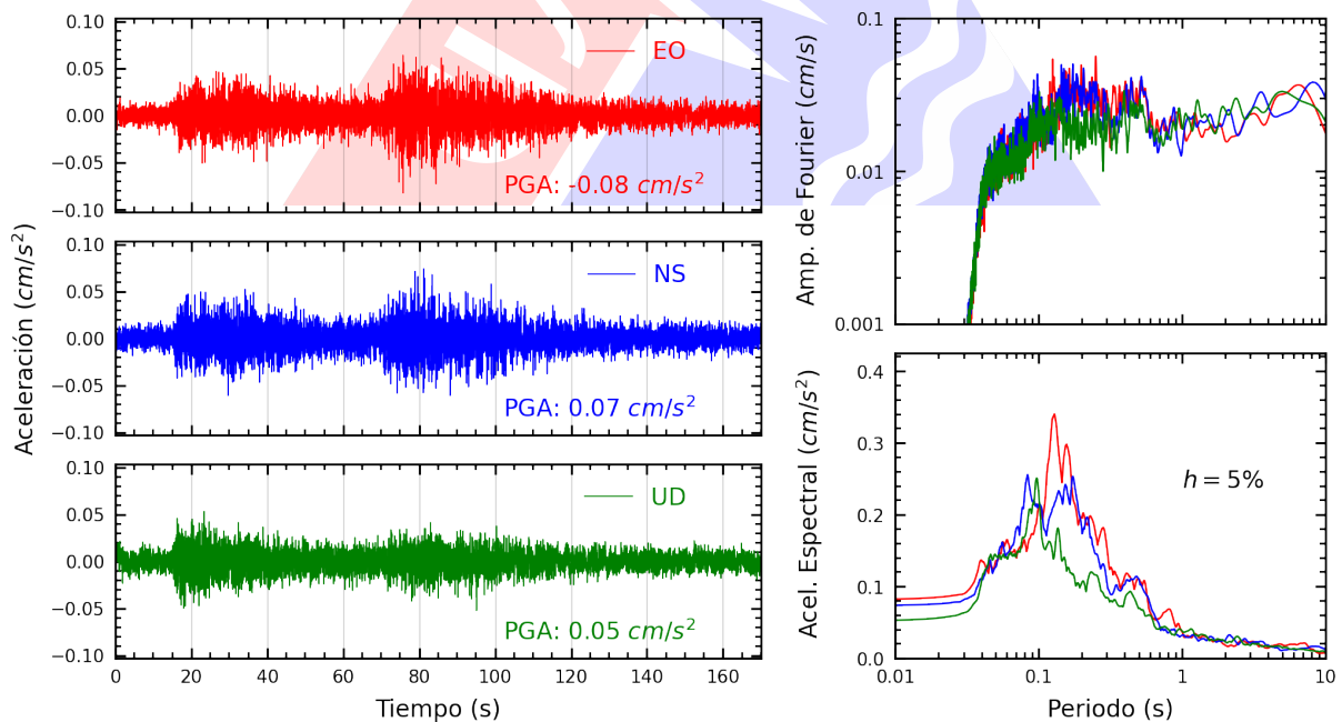
Figura A.22: Registros tiempo-historia, espectros de Fourier y de respuesta en las direcciones EO, NS y vertical de la estación IPEN. Sismo de Contamana, Ucayali - Loreto del 2023-05-01, 04:31:06 (Hora local)
