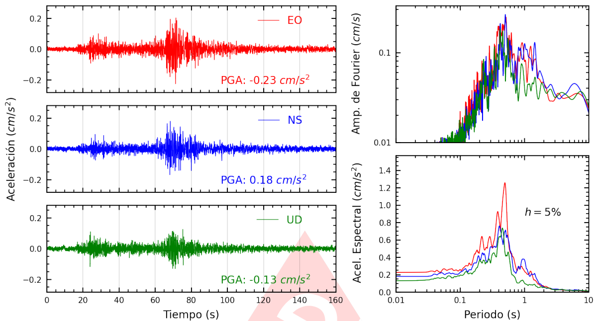
Figura A.15: Registros tiempo-historia, espectros de Fourier y de respuesta en las direcciones EO, NS y vertical de la estación UNASA. Sismo de Contamana, Ucayali - Loreto del 2023-05-01, 04:31:06 (Hora local)
