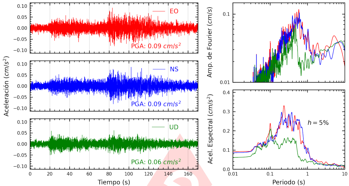
Figura A.21: Registros tiempo-historia, espectros de Fourier y de respuesta en las direcciones EO, NS y vertical de la estación USILP. Sismo de Contamana, Ucayali - Loreto del 2023-05-01, 04:31:06 (Hora local)
