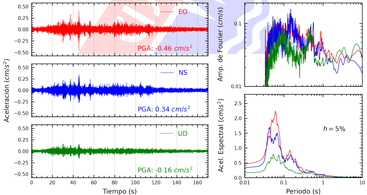
Figura A.6: Registros tiempo-historia, espectros de Fourier y de respuesta en las direcciones EO, NS y vertical de la estación USILM. Sismo de Contamana, Ucayali - Loreto del 2023-05-01, 04:31:06 (Hora local)
