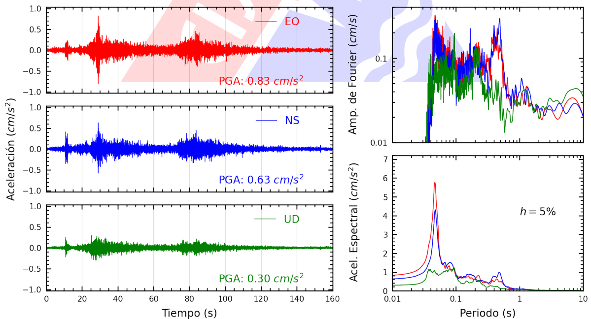
Figura A.4: Registros tiempo-historia, espectros de Fourier y de respuesta en las direcciones EO, NS y vertical de la estación USP. Sismo de Contamana, Ucayali - Loreto del 2023-05-01, 04:31:06 (Hora local)
