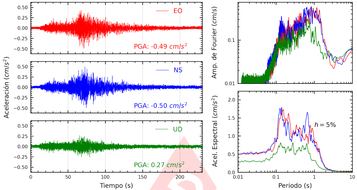
Figura A.5: Registros tiempo-historia, espectros de Fourier y de respuesta en las direcciones EO, NS y vertical de la estación UNTRM. Sismo de Contamana, Ucayali - Loreto del 2023-05-01, 04:31:06 (Hora local)
