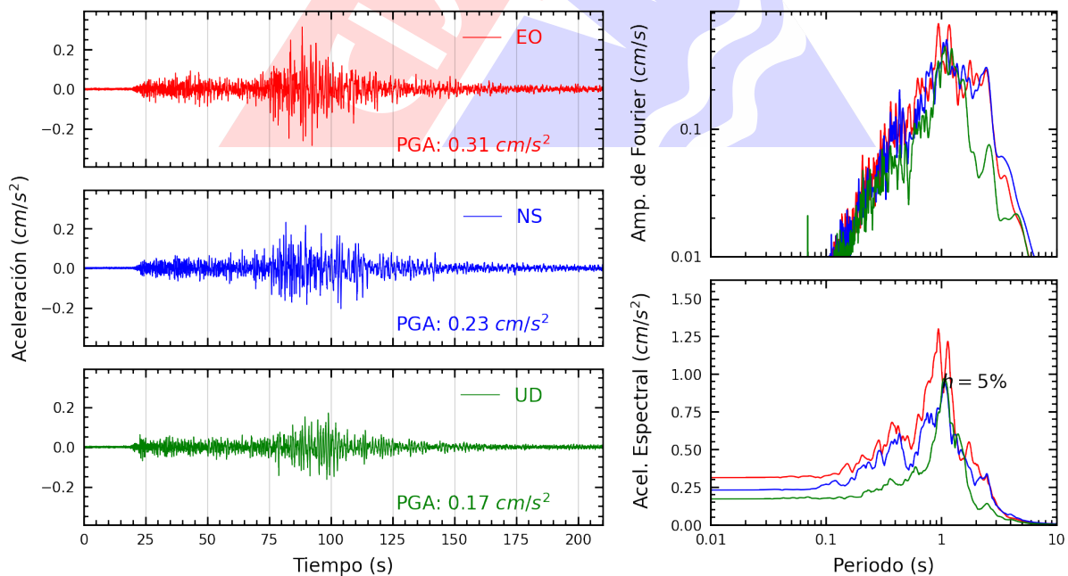
Figura A.8: Registros tiempo-historia, espectros de Fourier y de respuesta en las direcciones EO, NS y vertical de la estación UNC. Sismo de Contamana, Ucayali - Loreto del 2023-05-01, 04:31:06 (Hora local)
