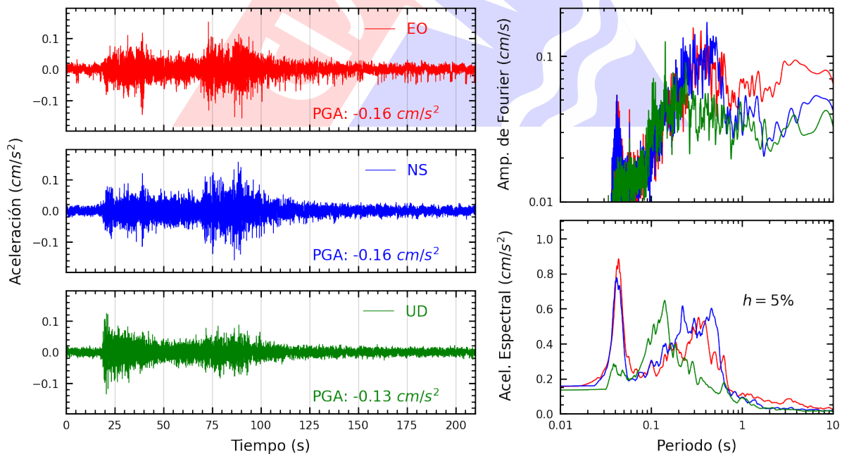
Figura A.18: Registros tiempo-historia, espectros de Fourier y de respuesta en las direcciones EO, NS y vertical de la estación UNAB. Sismo de Contamana, Ucayali - Loreto del 2023-05-01, 04:31:06 (Hora local)
