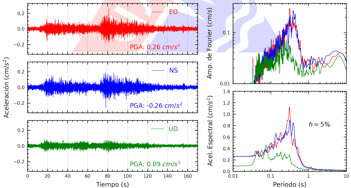
Figura A.12: Registros tiempo-historia, espectros de Fourier y de respuesta en las direcciones EO, NS y vertical de la estación DEFEN. Sismo de Contamana, Ucayali - Loreto del 2023-05-01, 04:31:06 (Hora local)
