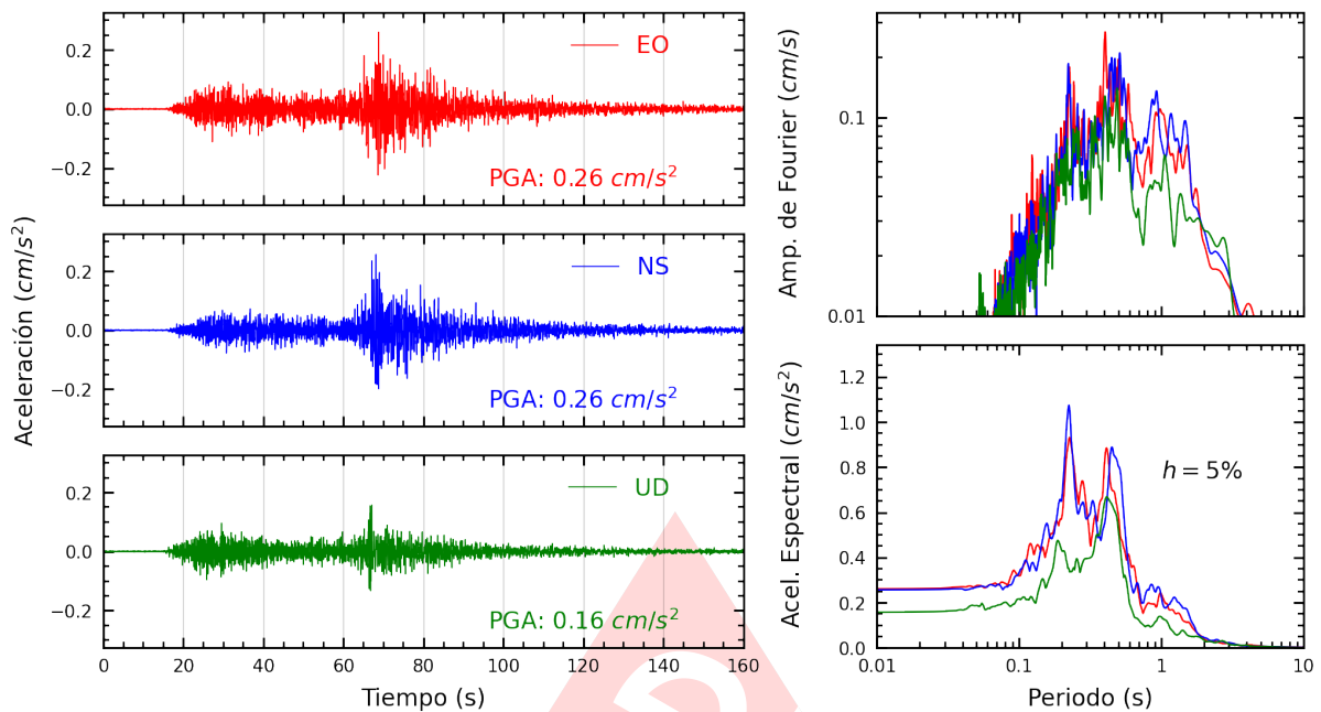
Figura A.11: Registros tiempo-historia, espectros de Fourier y de respuesta en las direcciones EO, NS y vertical de la estación YUNGA. Sismo de Contamana, Ucayali - Loreto del 2023-05-01, 04:31:06 (Hora local)
